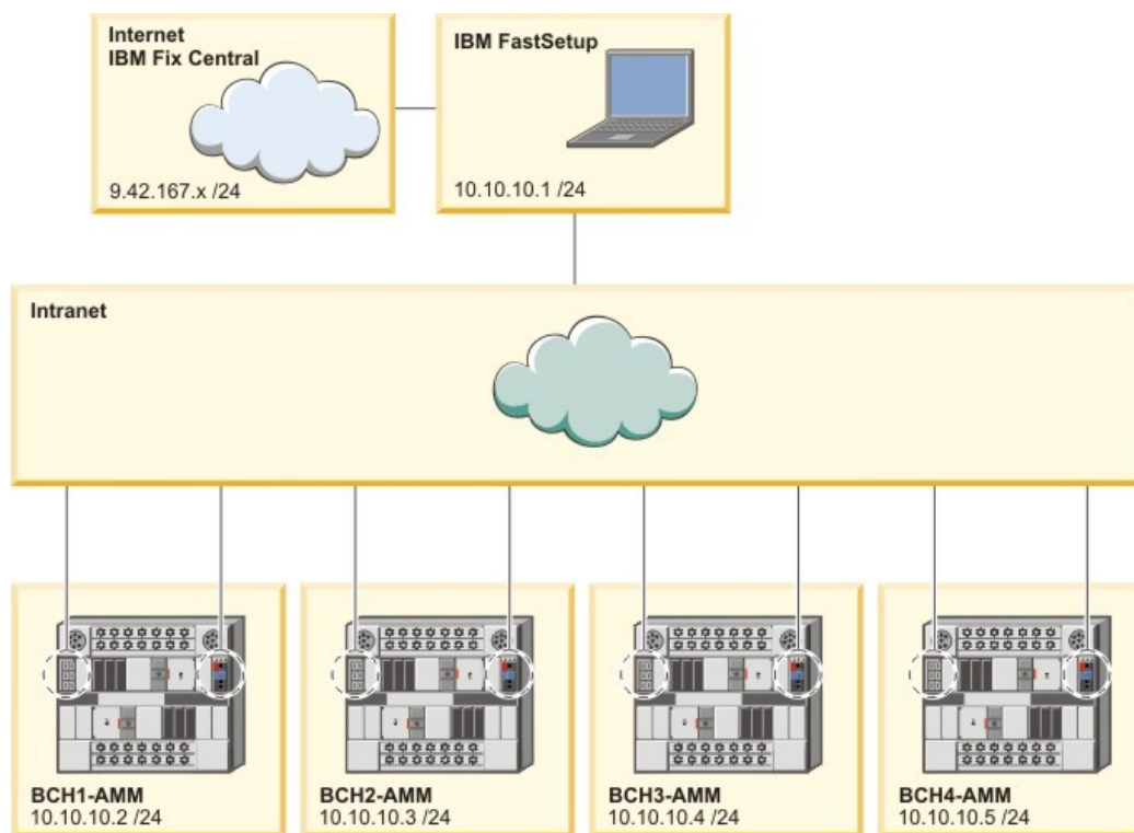
Figura 1: Cabeamento de rede do BladeCenter H
