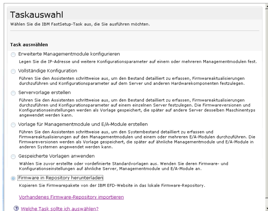
Abbildung 13: Anzeige "Taskauswahl"
