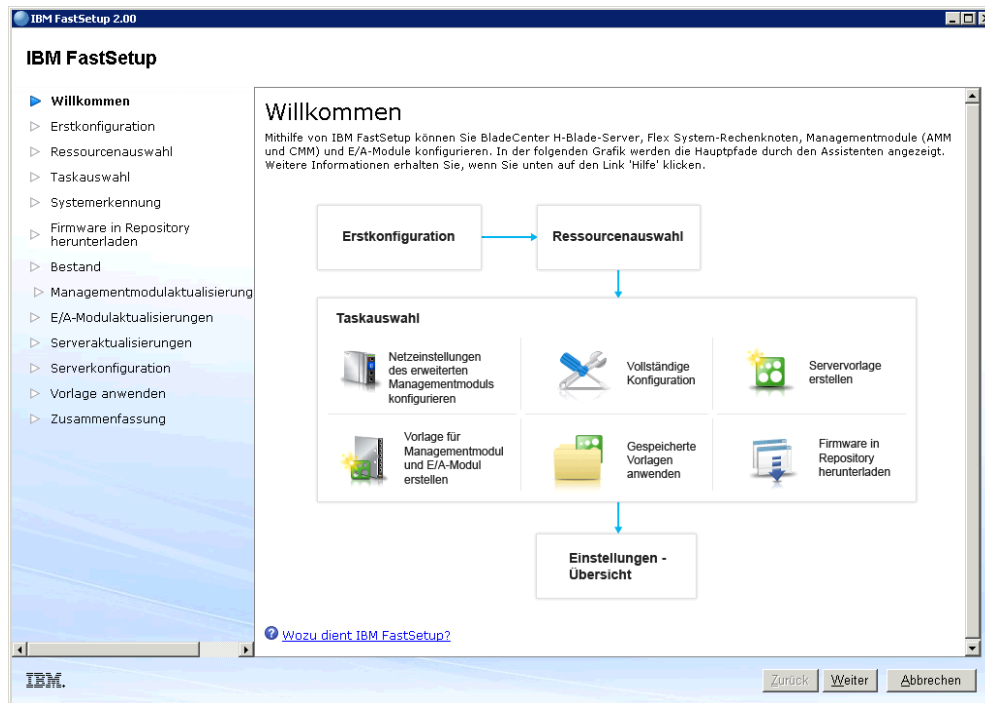
Abbildung 2: Eingangsanzeige
