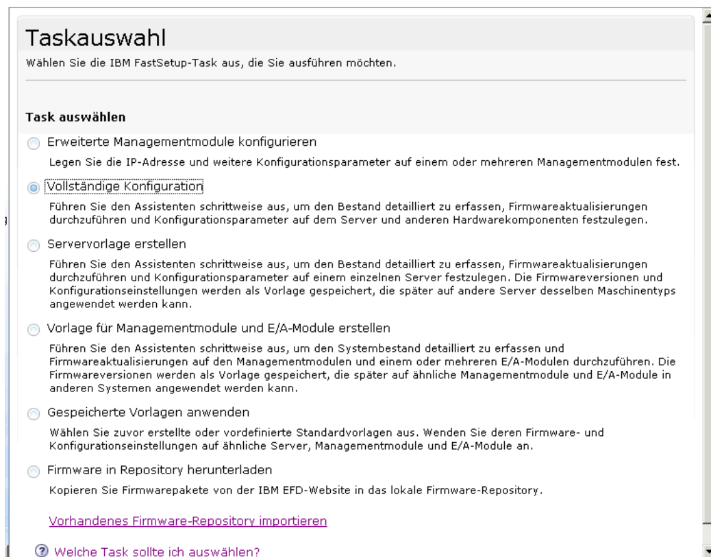
Abbildung 19: Anzeige "Taskauswahl"
