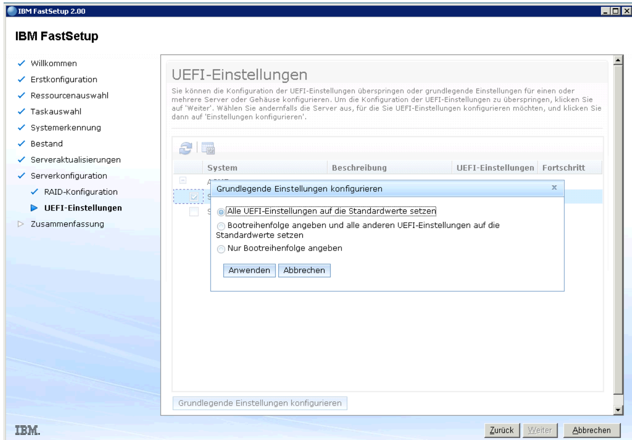
Abbildung 10: Anzeige "UEFI-Einstellungen"
