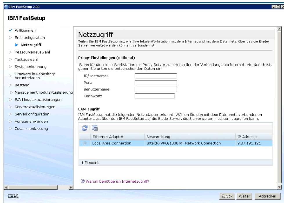
Abbildung 3: Netzzugriffsanzeige
