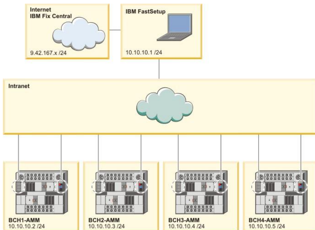
Figure 1 : Câblage réseau de BladeCenter H
