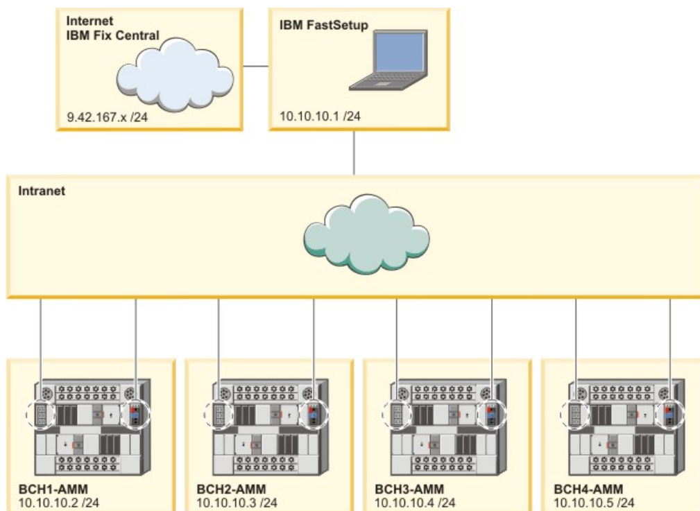
图1: BladeCenter H 网络布线
