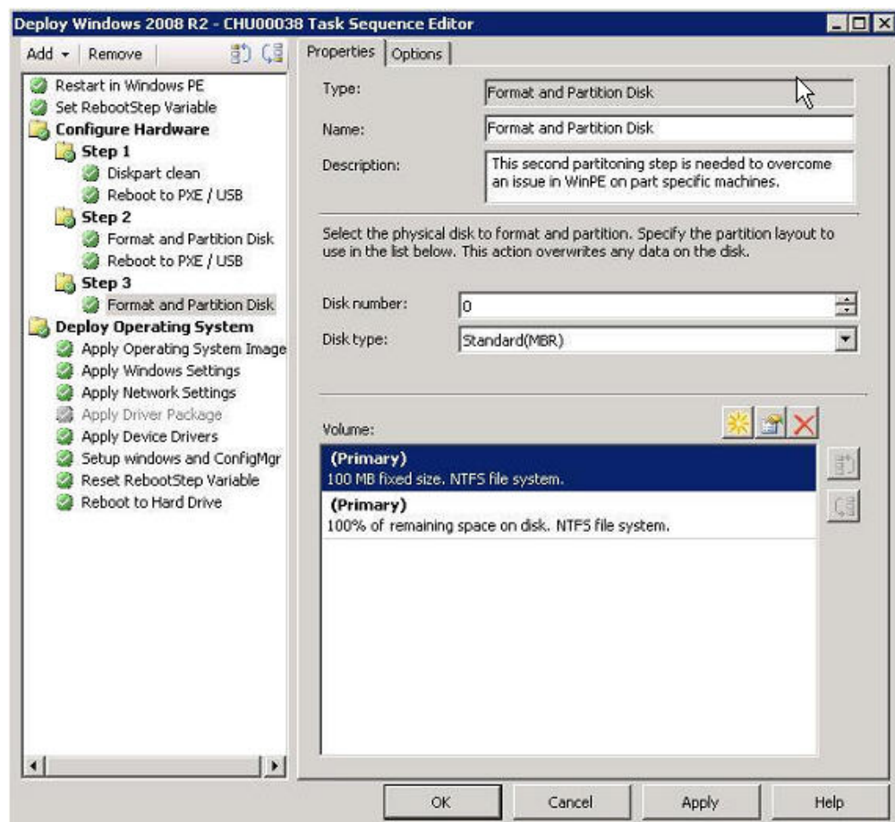
图 118. 任务序列
