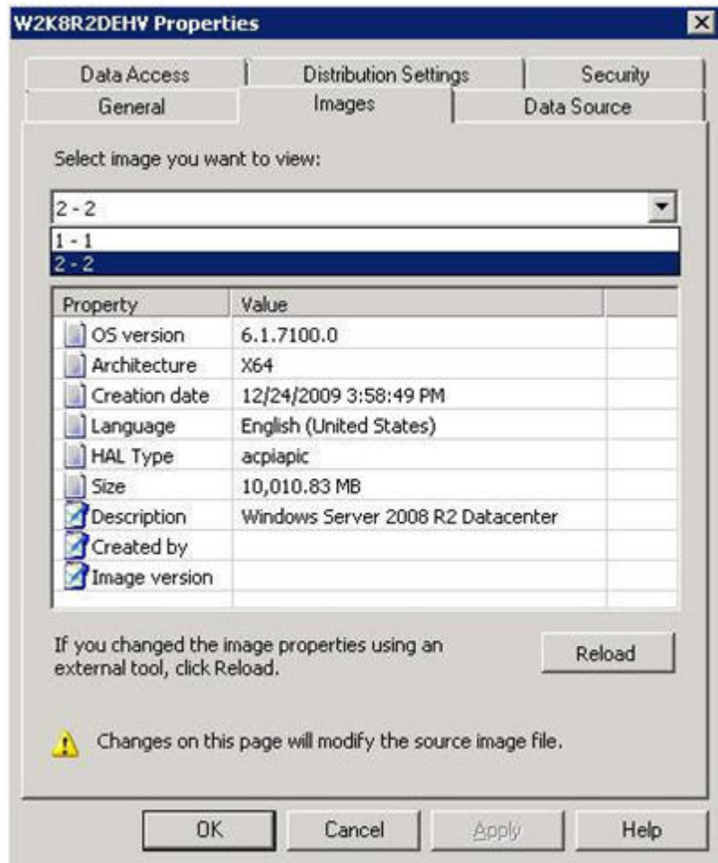
图 114. 映像列表
