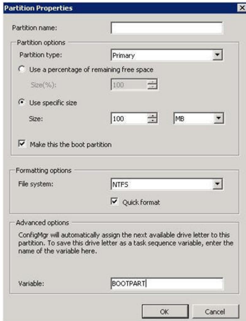
图 116. 分区属性
