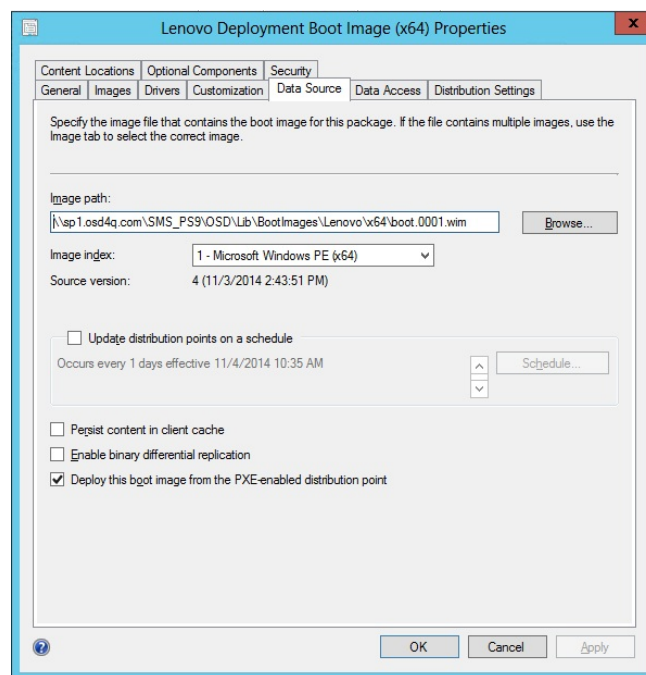
图 56. 配置数据源
