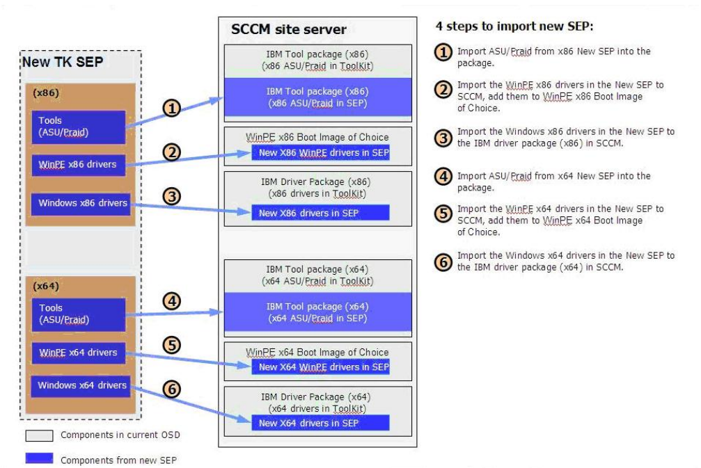
图 19. SEP 工作流程
