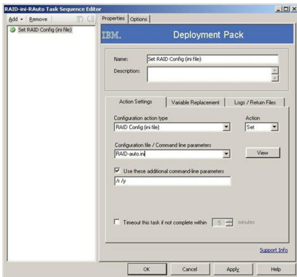
图 94. INI 文件的 RAID 配置任务序列
