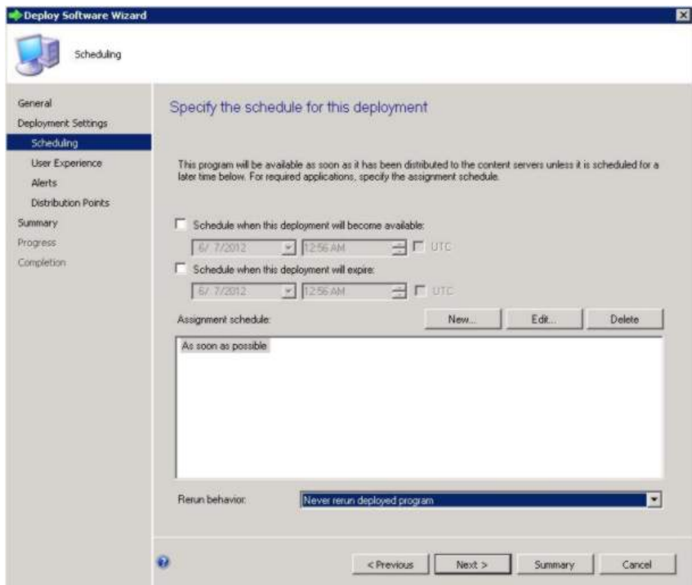
图 85. 安排部署
