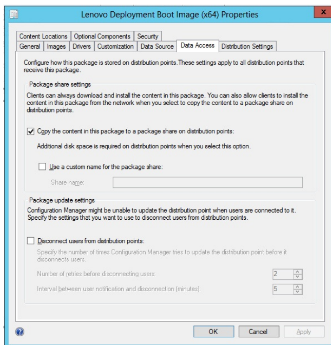
图 57. 包共享设置
