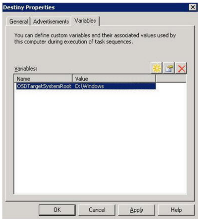
图 113. OSDTargetSystemRoot 属性
