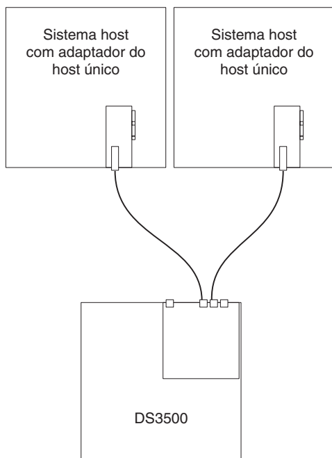
Figura 3-43. Conexão Fibre Channel Conectada Direta de Controlador Único a HBAs Únicos em Vários Hosts
