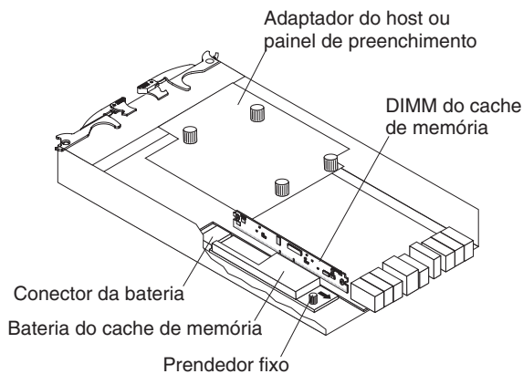
Figura 5-19. Local do DIMM do cache de memória
