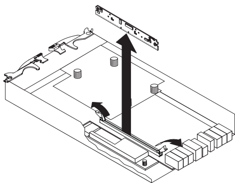
Figura 5-21. Removendo o DIMM do Controlador
