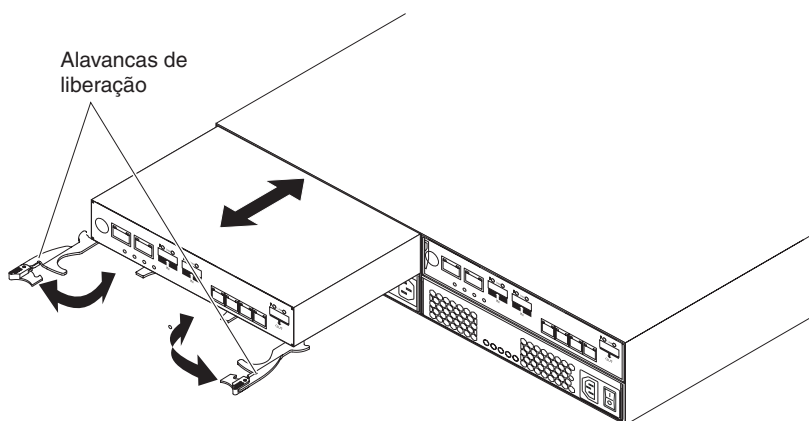
Figura 5-17. Removendo um controlador
