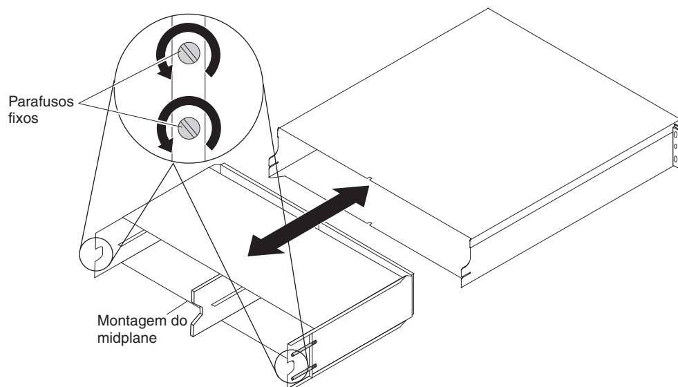
Figura 5-25. Substituindo uma Montagem do Painel Intermediário em um DS3512 ou EXP3512
