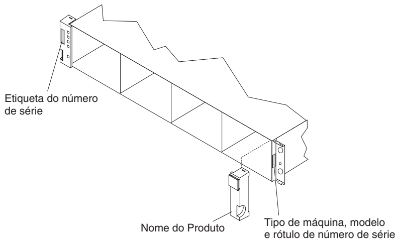
Figura 1-1. Locais da Etiqueta do Número de Série e da Etiqueta do Nome do Produto, do Tipo de Máquina e do Número do Modelo
