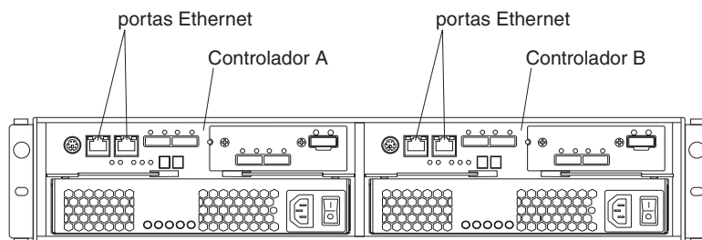
Figura 3-28. Locais de Porta Ethernet em um DS3500 de Controlador Dual
