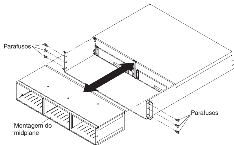
Figura 5-26. Substituindo uma Montagem do Painel Intermediário em um DS3524 ou EXP3524
