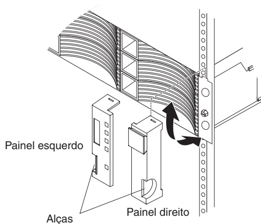
Figura 5-23. Removendo os Painéis
