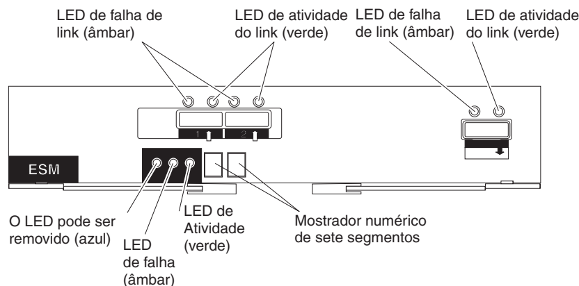
Figura 4-13. LEDs do ESM
