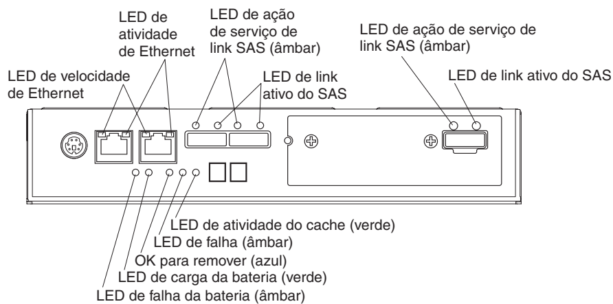
Figura 4-7. LEDs do controlador
