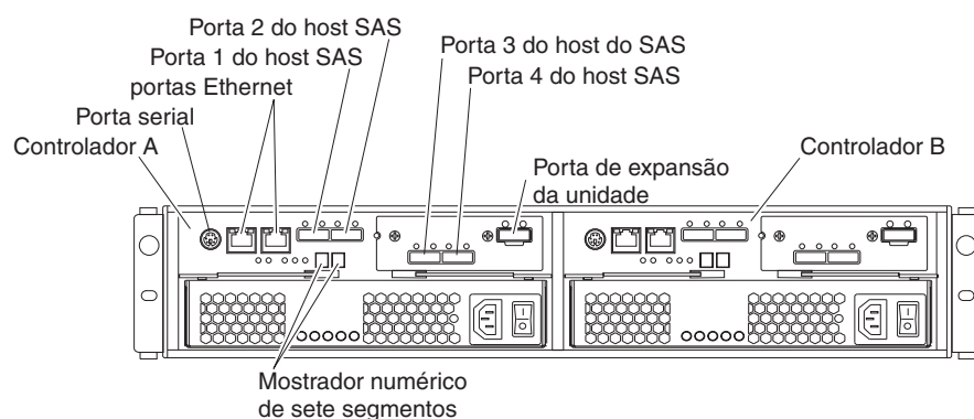
Figura 3-4. Portas e Controladores do Subsistema de Armazenamento DS3500 de Controlador Dual (com Adaptador de Porta do Host SAS Opcional)
