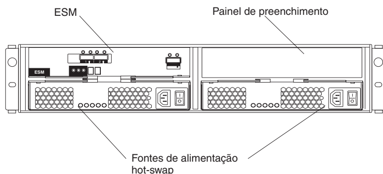
Figura 1-8. Vista Posterior, Gabinete de Armazenamento do Modelo ESM Único
