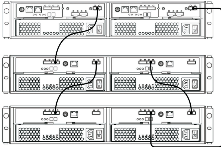
Figura 3-26. Um DS3500 de Controlador Dual e Dois Gabinetes de Armazenamento
