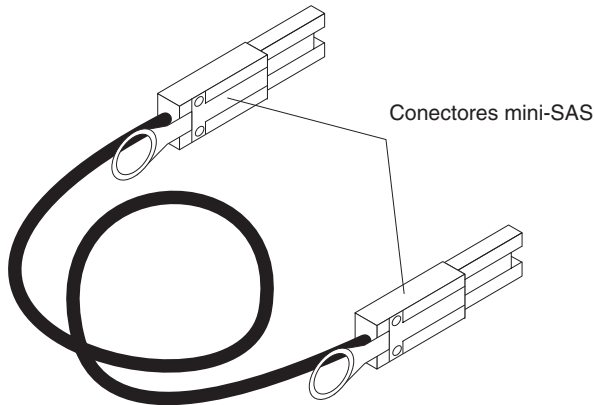
Figura 3-5. Cabo MiniSAS
