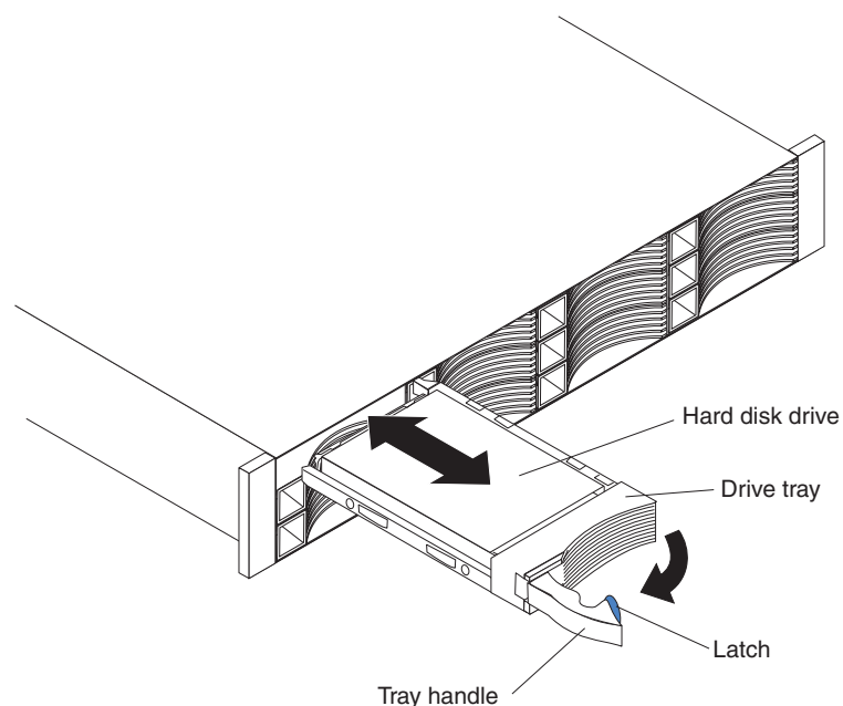
Figura 5-13. Instalando uma Unidade em um DS3512 ou EXP3512
