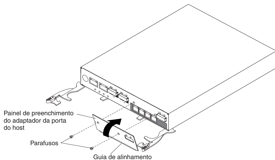
Figura 5-7. Removendo o Painel de Preenchimento do Adaptador de Porta do Host
