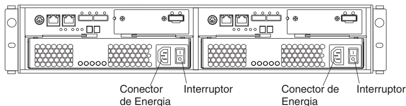
Figura 1-9. Componentes da Fonte de Alimentação AC
