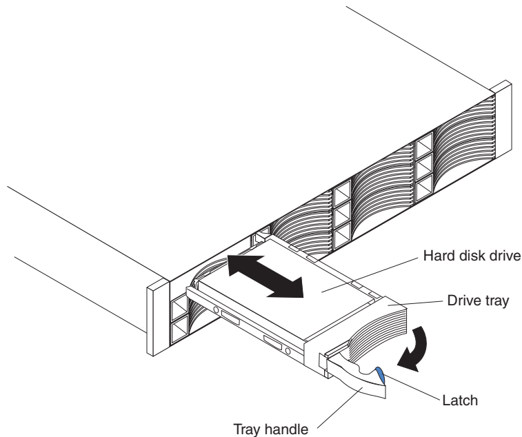
Figura 5-11. Removendo uma Unidade de um DS3512 ou EXP3512
