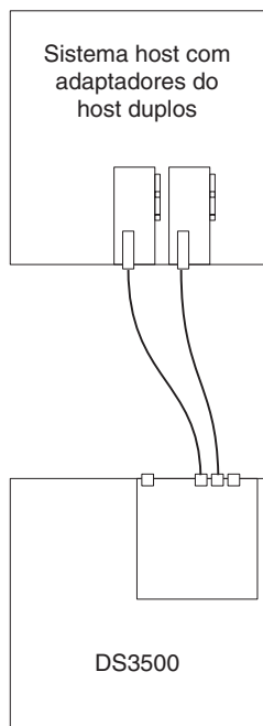
Figura 3-32. Conexão Direta SAS de Controlador Único a HBAs dual em um Host Único (Conexão de Host Redundante)
