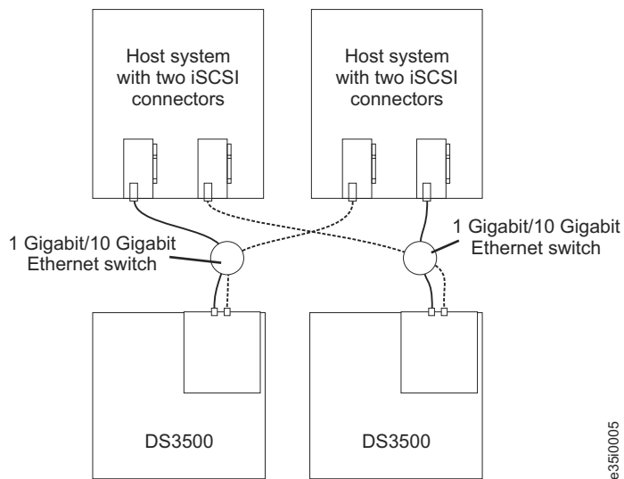
Figura 3-53. Configuração do iSCSI para diversos Subsistemas de Armazenamento com diversos Hosts e Portas
