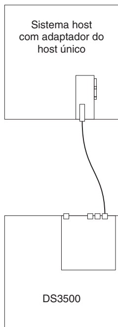
Figura 3-31. Conexão SAS com Conexão Direta de Controlador Único a um HBA de Host Único
