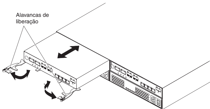
Figura 5-4. Removendo e Recolocando um Controlador
