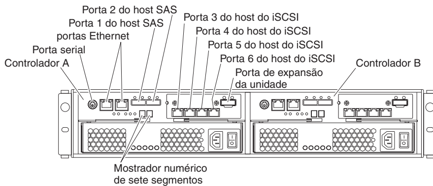
Figura 3-2. Portas e Controladores do Subsistema de Armazenamento DS3500 de Controlador Dual (com Adaptador de Porta do Host iSCSI Opcional)
