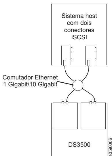
Figura 3-54. Configuração do iSCSI de Controlador Dual de Host Único com diversas Portas
