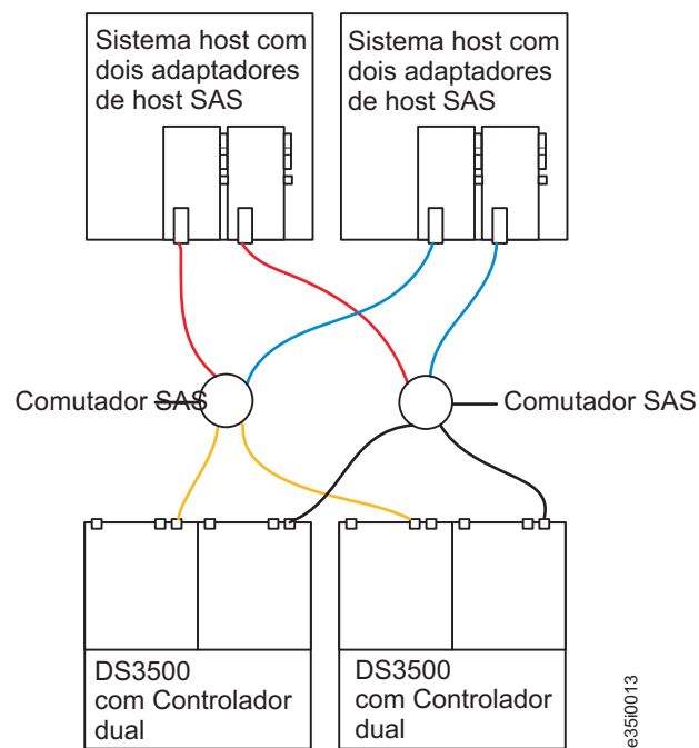
Figura 3-38. Conexão SAS DS3500 de Diversos Controladores Dual com Diversos Hosts Usando Dois Comutadores SAS Separados
