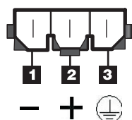
Figura 1-11. Conector da Fonte de Alimentação DC - Posições dos Pinos
