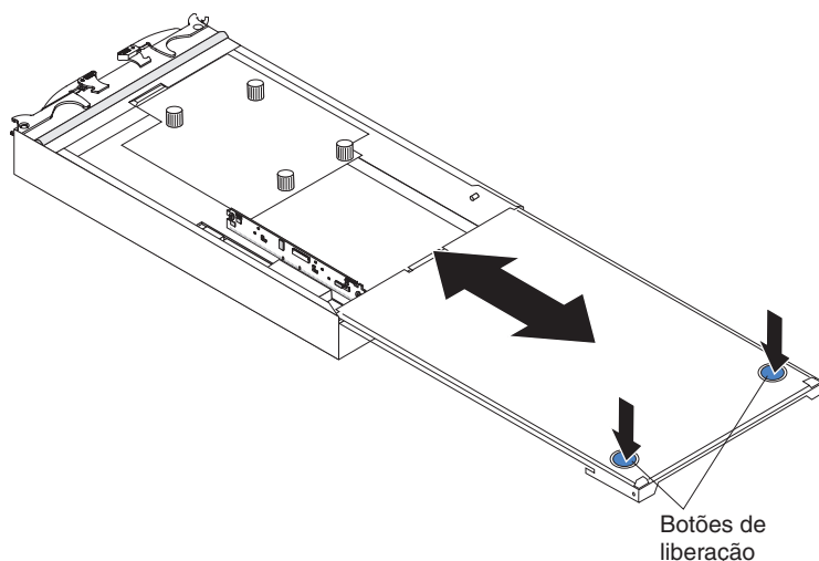
Figura 5-24. Removendo um Environmental Service Module
