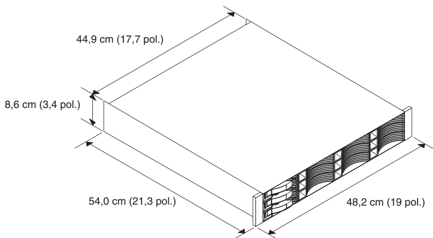
Figura 1-13. Dimensões do Subsistema de Armazenamento DS3512 e Gabinete de Armazenamento EXP3512
