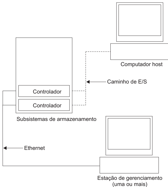
Figura 3-30. Subsistemas de Armazenamento Gerenciado Direto (Fora da Banda)
