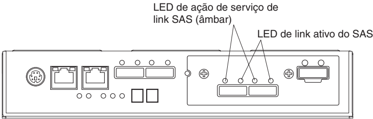
Figura 4-10. LEDs de Adaptador de Porta do Host SAS
