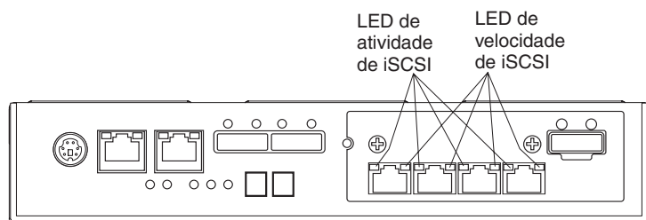
Figura 4-8. LEDs do Adaptador da Porta do Host iSCSI
