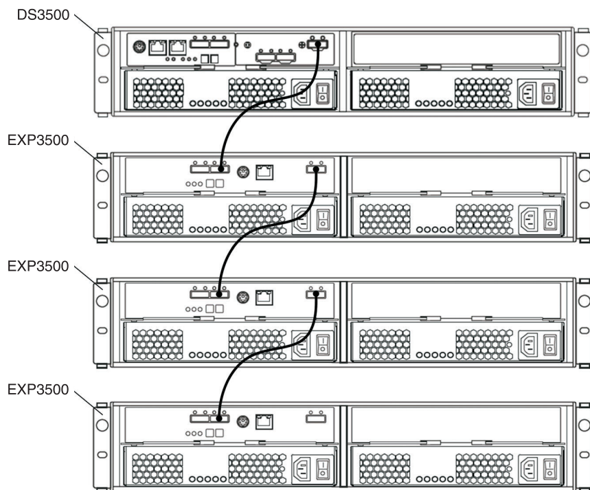
Figura 3-24. Um DS3500 de Controlador Único e diversos Gabinetes de Armazenamento ESM Únicos
