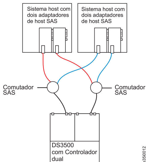
Figura 3-37. Conexão SAS DS3500 de Controlador Dual com Diversos Hosts Usando Dois Comutadores SAS Separados
