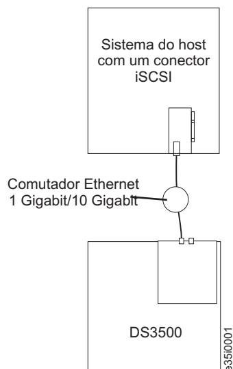
Figura 3-49. Host Único, Configuração iSCSI de Controlador Único
