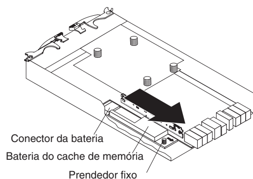
Figura 5-5. Removendo a Unidade de Bateria do Controlador
