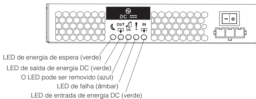
Figura 4-4. LEDs da Fonte de Alimentação DC
