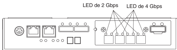
Figura 4-9. LEDs do Adaptador de Porta do Host Fibre Channel
