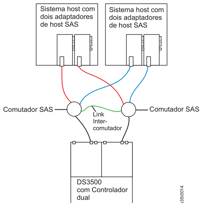
Figura 3-39. Conexão SAS DS3500 de Controlador Dual com Diversos Hosts Usando Dois Comutadores SAS que Estão Conectados Juntos por meio de um Comutador Interlink
