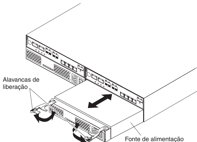
Figura 5-16. Substituindo uma fonte de alimentação
