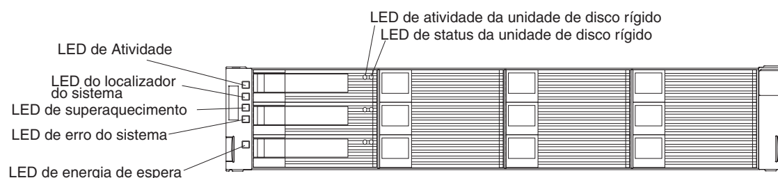
Figura 4-5. Controles e LEDs Frontais do Subsistema de Armazenamento DS3512 e Gabinete de Armazenamento EXP3512
