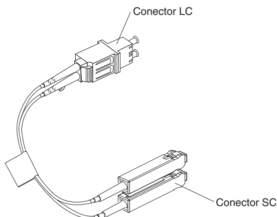
Figura 3-17. adaptador de cabo Fibre Channel LC-SC
