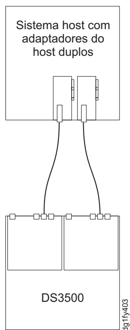
Figura 3-34. Conexão SAS Conectada Direto de Controlador Dual a Dois HBAs no Mesmo Host (Conexão de Host Redundante)
