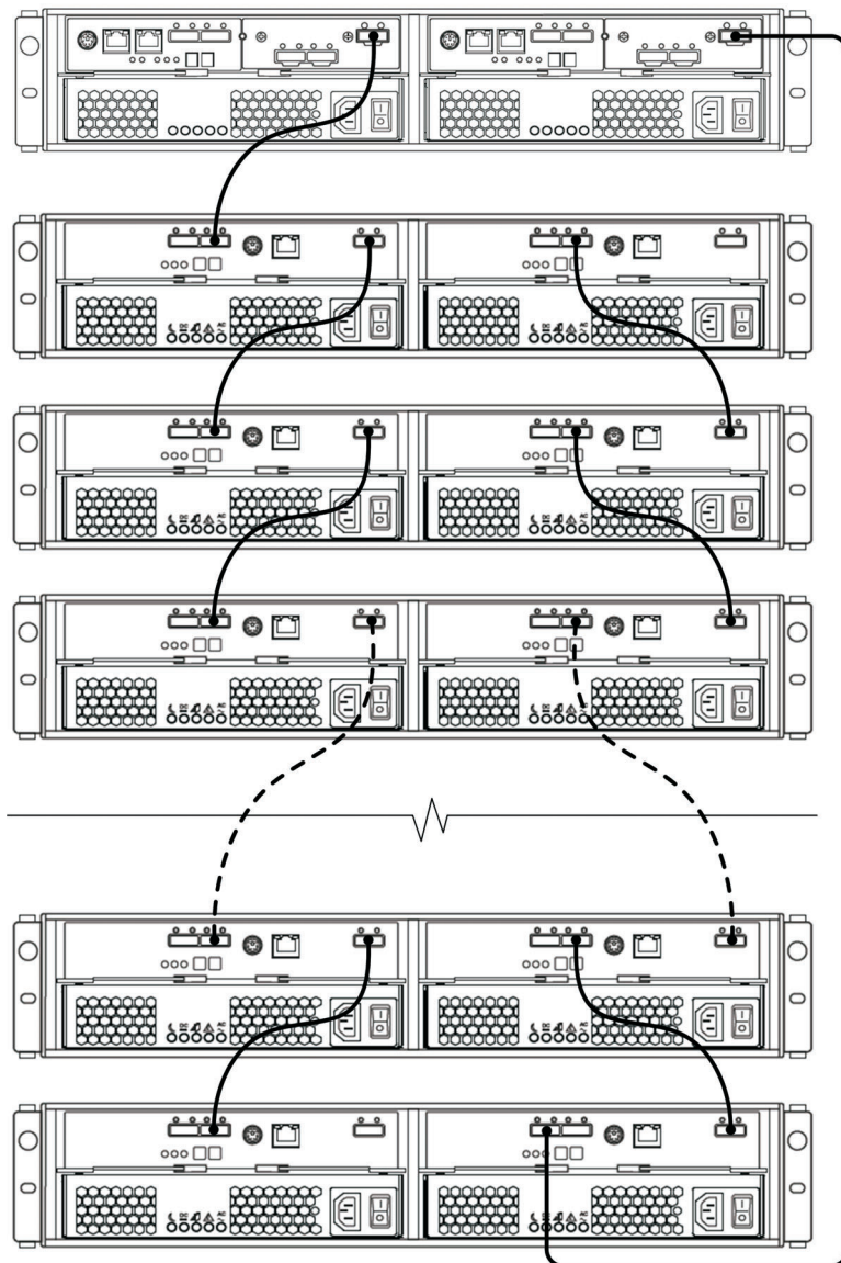
Figura 3-27. Um DS3500 de Controlador Duplo e Oito gabinete de armazenamentos
