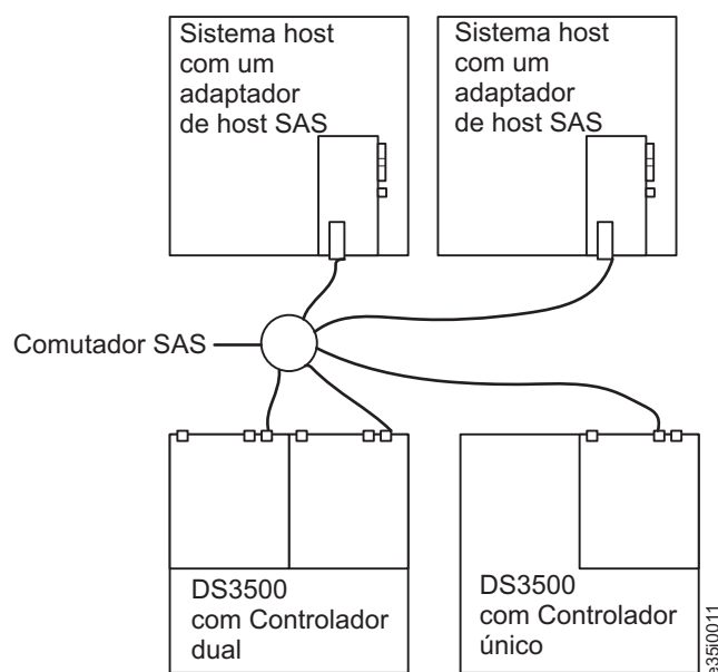
Figura 3-36. O Controlador Duplo DS3500 ou Controlador Único SAS DS3500 SAS com Diversos Hosts Usando um Comutador SAS
