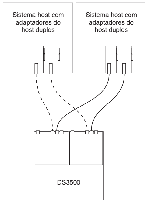
Figura 3-35. Conexões Diretas SAS de Controlador Dual a Vários HBAs em Vários Hosts
