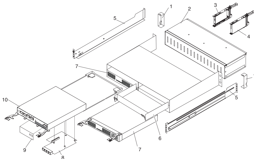
Figura 7-2. Peças do Subsistema de Armazenamento DS3524 e do Gabinete de Armazenamento EXP3524
