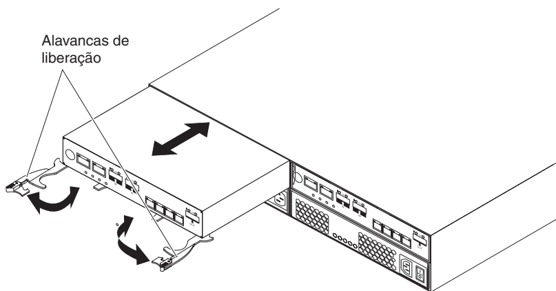
Figura 5-20. Removendo um controlador
