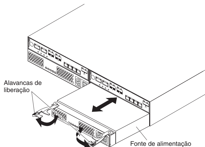
Figura 5-15. Substituindo uma fonte de alimentação
