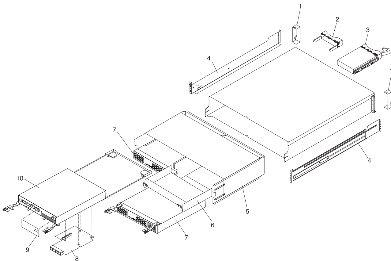
Figura 7-1. Peças do Subsistema de Armazenamento DS3512 e do Subsistema de Armazenamento do Gabinete de Armazenamento EXP3512
