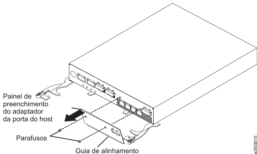
Figura 5-8. Instalando um Adaptador de Porta do Host
