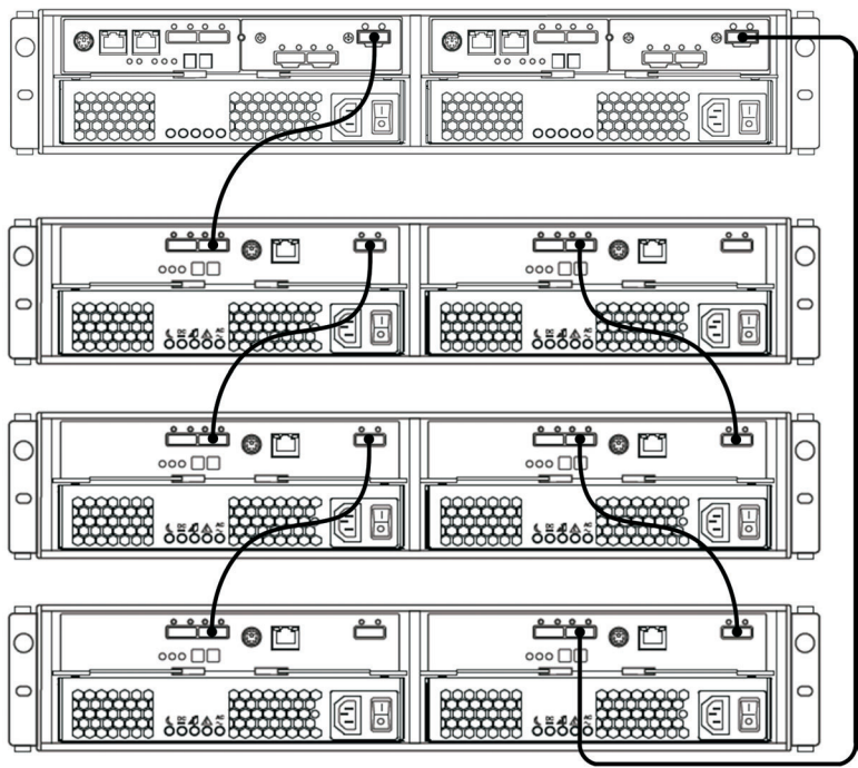
Figura 3-23. Exemplo de um Caminho de Unidade Redundante
