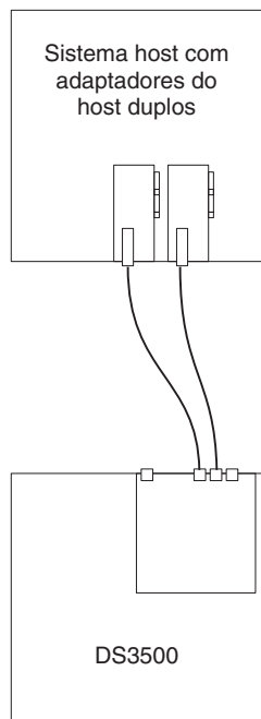
Figura 3-42. Conexão Fibre Channel Conectada Direta de Controlador Único com HBAs Dual (Conexão de Host Redundante)
