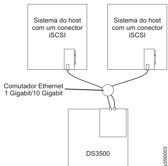
Figura 3-51. Vários Hosts de Porta Única, Configuração iSCSI de Controlador Único
