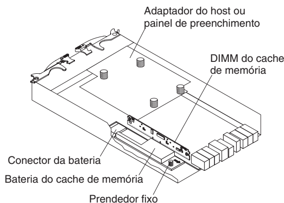
Figura 1-12. Unidade da Bateria
