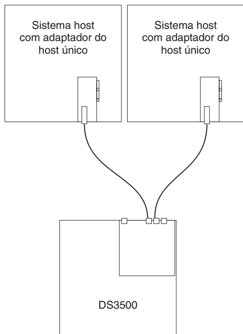
Figura 3-33. Conexão Direta SAS de Controlador Único a HBAs únicos em Vários Hosts
