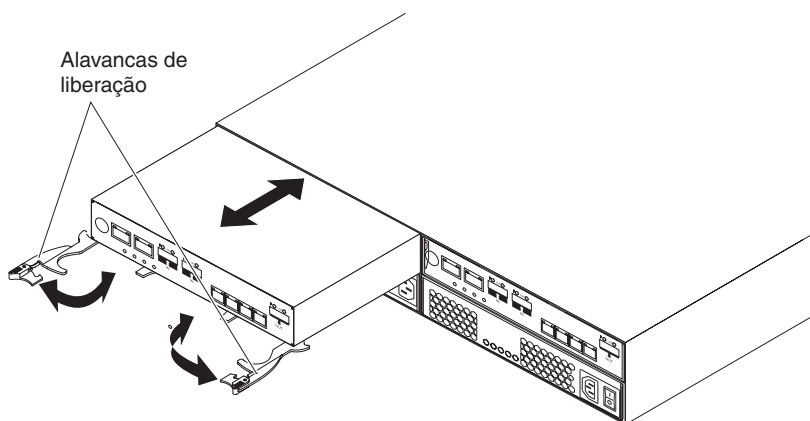
Figura 5-6. Removendo um controlador
