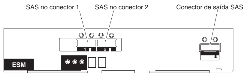
Figura 3-22. Conectores ESM
