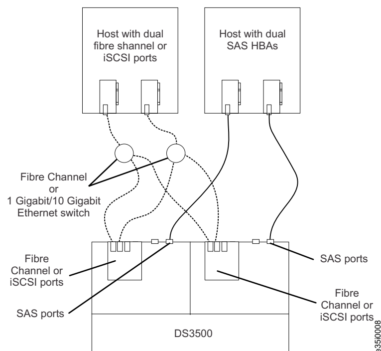
Figura 3-56. Exemplo de uma Configuração de Vários Hosts, Várias Portas e Várias Malhas (Fibre Channel ou iSCSI e SAS)
