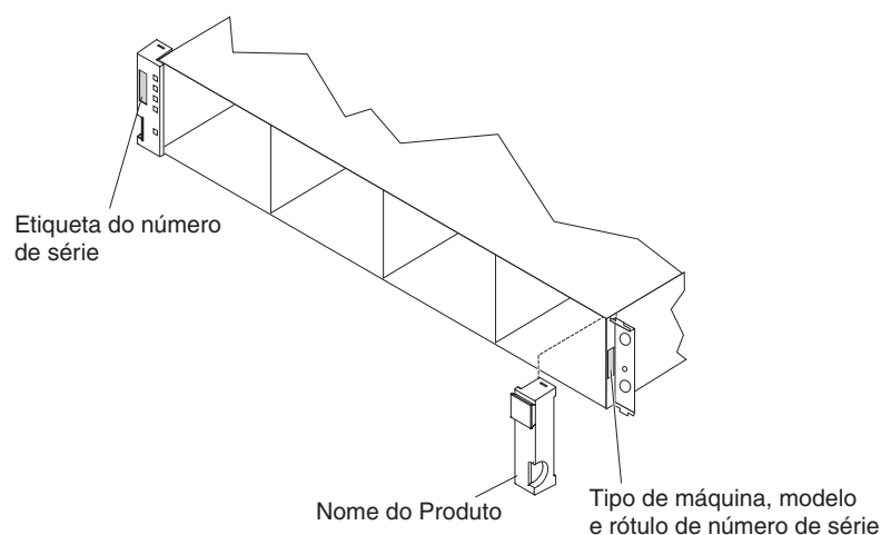
Figura A-1. Local do número de série no DS3500
