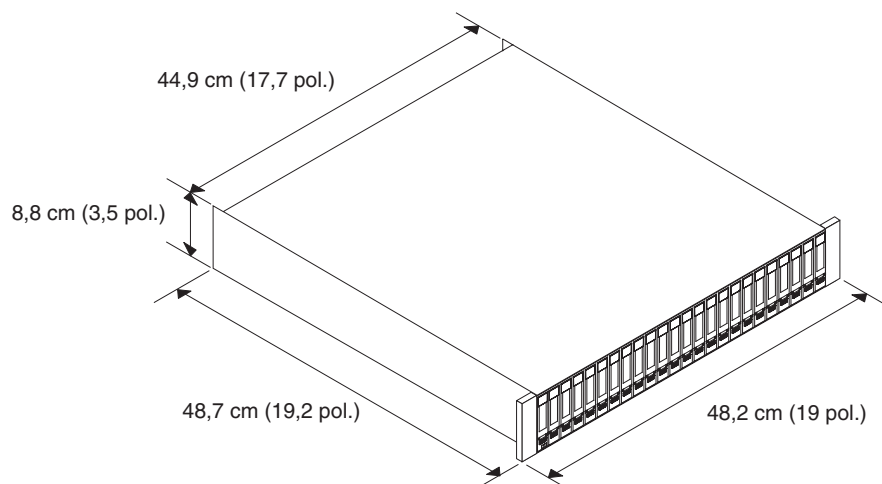
Figura 1-14. Dimensões do Subsistema de Armazenamento DS3524 e Gabinete de Armazenamento EXP3524
