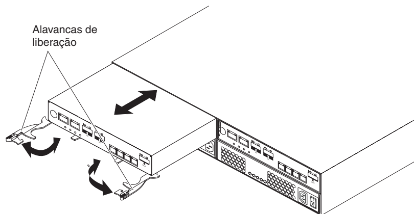
Figura 5-1. Removendo um controlador
