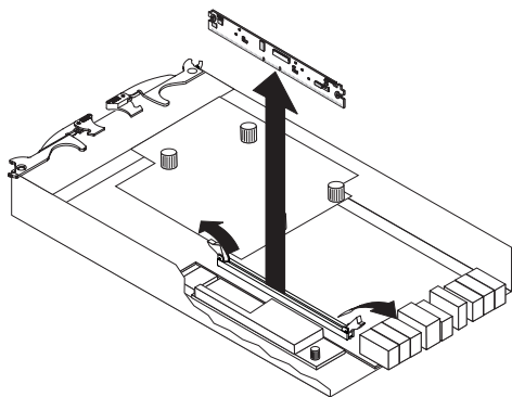
Figura 5-22. Instalando o DIMM no controlador
