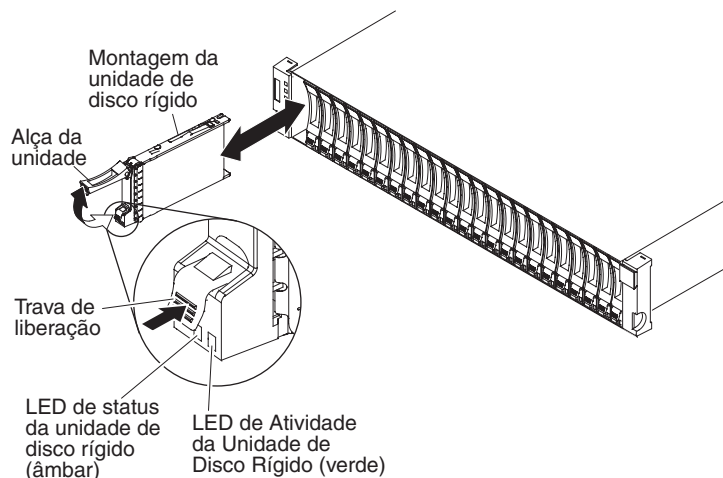
Figura 5-12. Removendo uma Unidade de um DS3524 ou EXP3524
