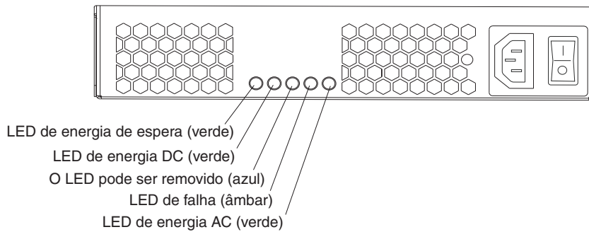
Figura 4-3. LEDs de Fonte de Alimentação AC
