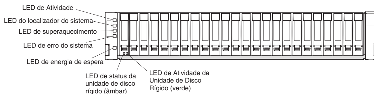
Figura 4-6. LEDs Frontais do Subsistema de Armazenamento DS3524 e Gabinete de Armazenamento EXP3524
