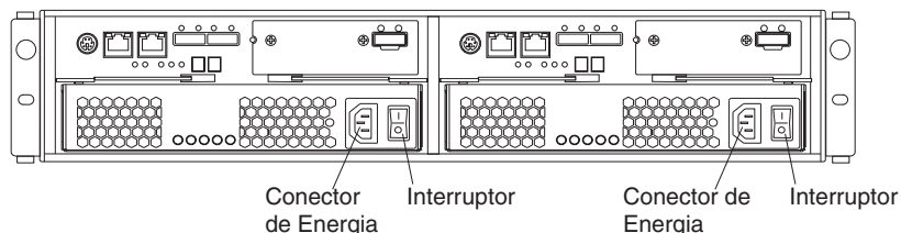
Figura 4-1. Conectores e Comutadores de Fonte de Alimentação para Modelos de AC do DS3500
