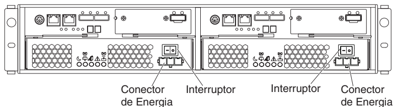
Figura 4-2. Conectores e Comutadores de Fonte de Alimentação para Modelos de DC do DS3500
