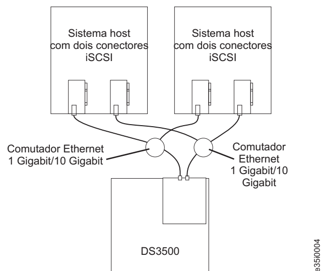
Figura 3-52. Configuração do iSCSI de Controlador Único com diversos Hosts e Portas e Caminho Redundante
