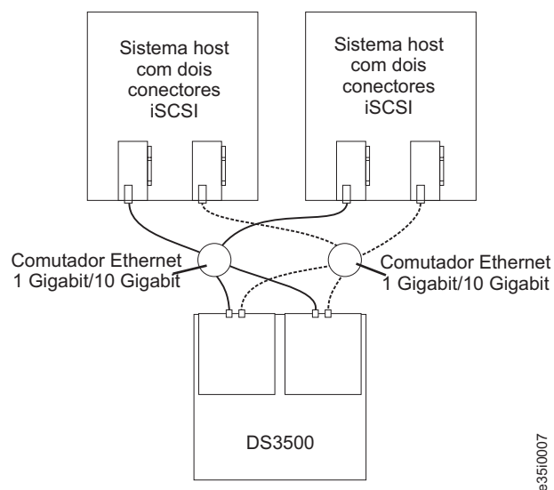
Figura 3-55. Configuração do iSCSI de Controlador Dual com diversos Hosts e Portas
