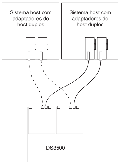
Figura 3-45. Conexões Diretas Fibre Channel do Controlador Dual a Vários HBAs em Vários Hosts
