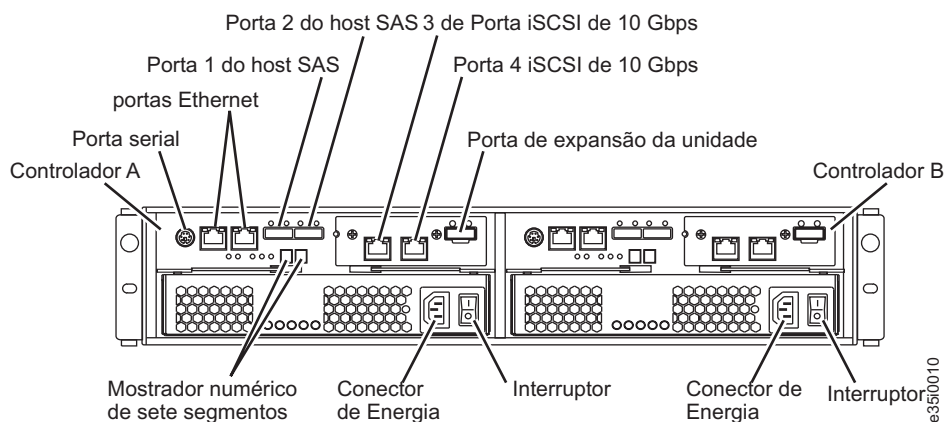
Figura 3-3. Portas e Controladores do Subsistema de Armazenamento DS3500 de Controlador Dual (com Adaptador de Porta do Host iSCSI de 10 Gbps Opcional)
