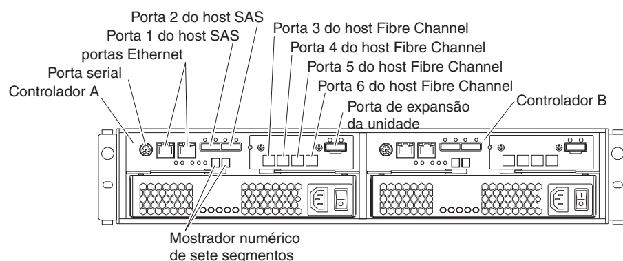
Figura 3-1. Portas e Controladores do Subsistema de Armazenamento DS3500 de Controlador Dual (com Adaptador de Porta do Host Fibre Channel Opcional)
