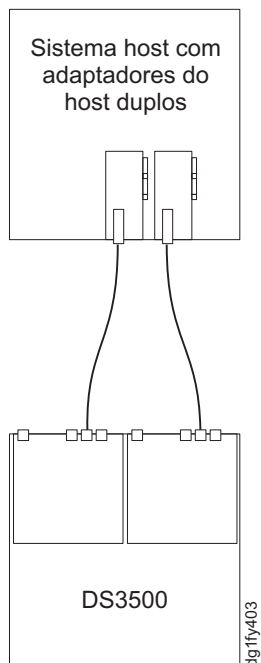
Figura 3-44. Conexão Fibre Channel Conectada Direta de Controlador Dual a Dois HBAs no Mesmo Host (Conexão de Host Redundante)
