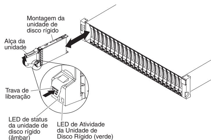
Figura 5-14. Instalando uma Unidade em um DS3524 ou EXP3524
