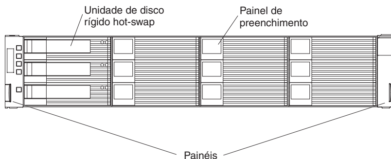
Figura 1-2. Painéis e compartimentos de unidades hot swap do subsistema de armazenamento DS3512 e gabinete de armazenamento EXP3512
