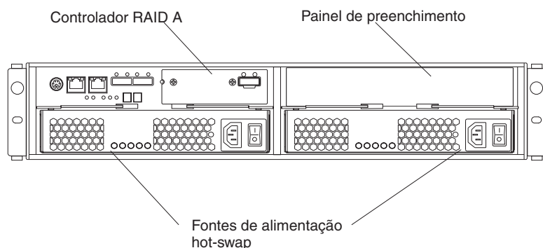
Figura 1-7. Vista Posterior, Modelo de Controlador Único (Mostrado sem um Adaptador de Porta do Host Opcional)
