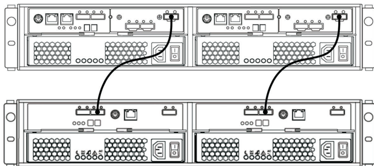
Figura 3-25. Um DS3500 de Controlador Dual e um gabinete de armazenamento
