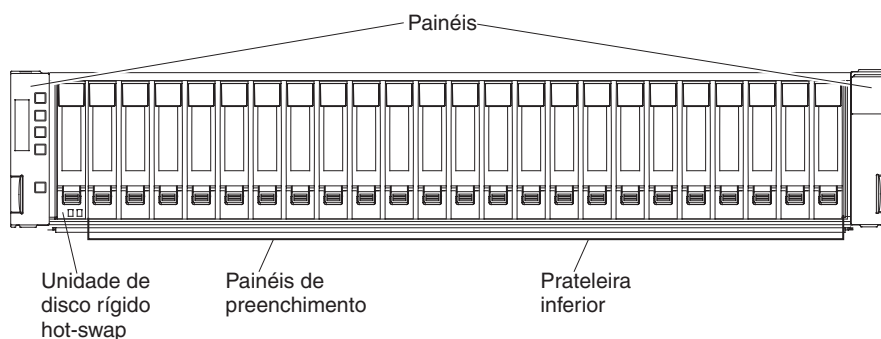
Figura 1-3. Painéis e compartimentos de unidades hot swap do subsistema de armazenamento DS3524 e gabinete de armazenamento EXP3524
