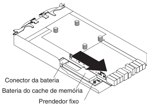
Figura 5-18. Removendo uma Unidade de Bateria do Controlador
