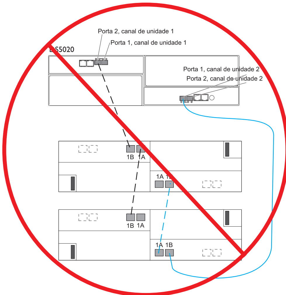
Figura 39. Cabeamento incorreto de um DS5020 e dois gabinete de expansão de armazenamentos
