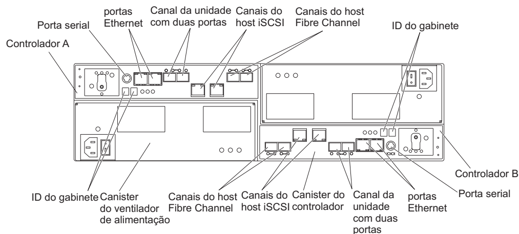
Figura 4. Vista posterior; controladores com dois canais de expansão de host padrão Fibre Channel e dois canais de expansão de host opcional iSCSI
