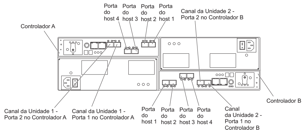
Figura 36. Portas e controladores do subsistema de armazenamento DS5020
