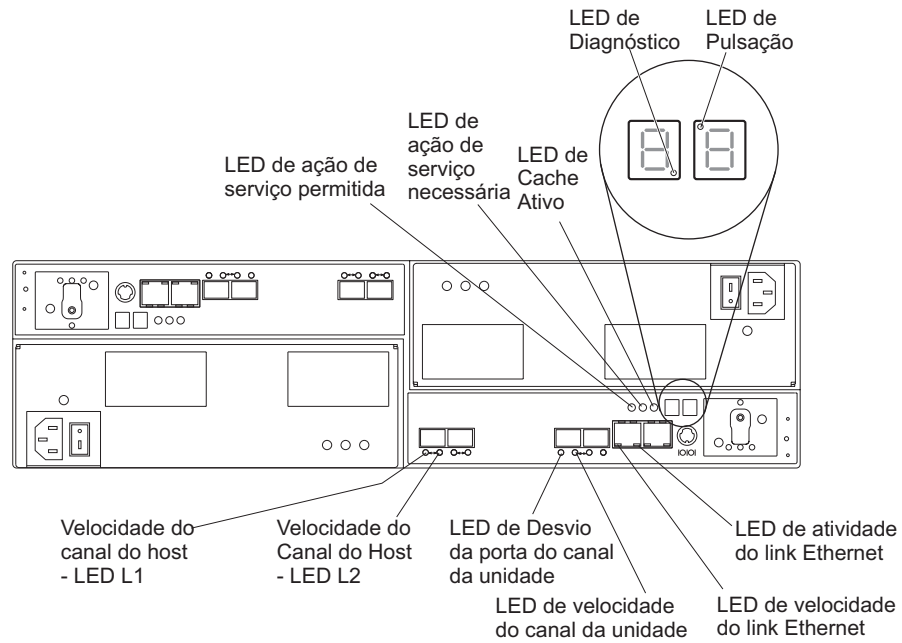
Figura 69. LEDs, controles e conectores de controladores com dois canais padrão de expansão de host Fibre Channel
