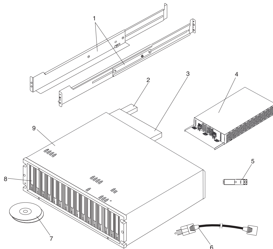
Figura 88. Lista de Peças do Subsistema de Armazenamento DS5020
