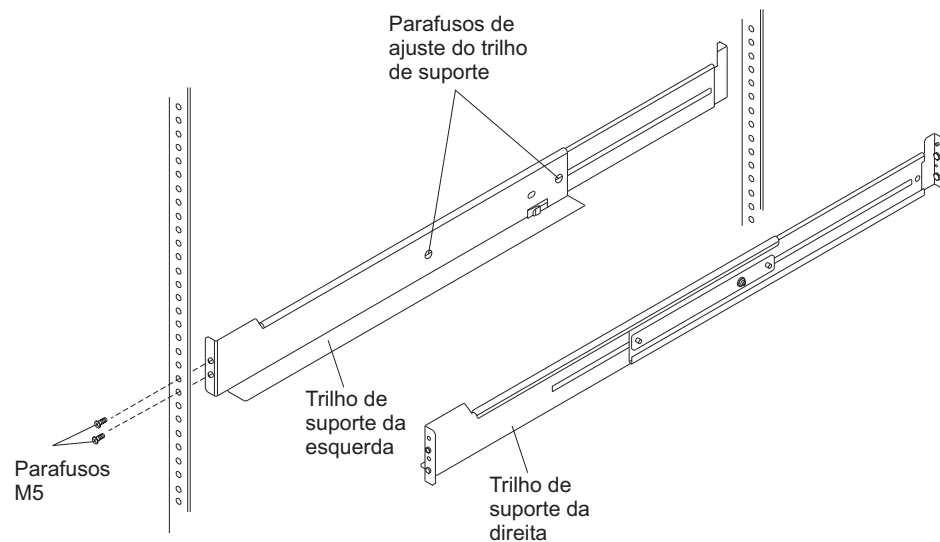
Figura 15. Instalando os Trilhos de Suporte
