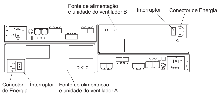
Figura 5. Componentes da unidade de fonte de alimentação e refrigeração para o DS5020
