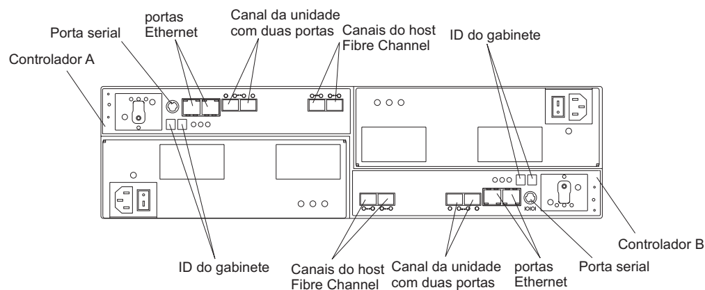
Figura 2. Vista posterior; controladores com dois canais de expansão de host padrão Fibre Channel
