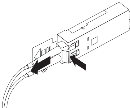
Figura 34. Removendo o cabo Fibre Channel LC-LC
