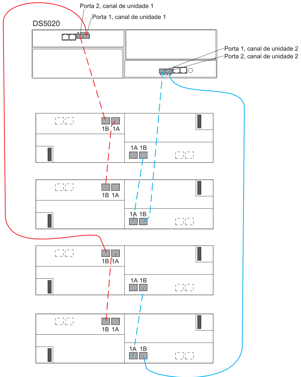
Figura 41. Cabeamento para um DS5020 e quatro gabinete de expansão de armazenamentos
