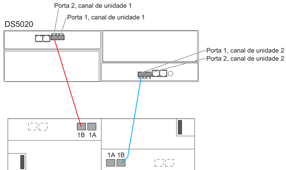
Figura 37. Cabeamento para um DS5020 e um gabinete de expansão de armazenamento
