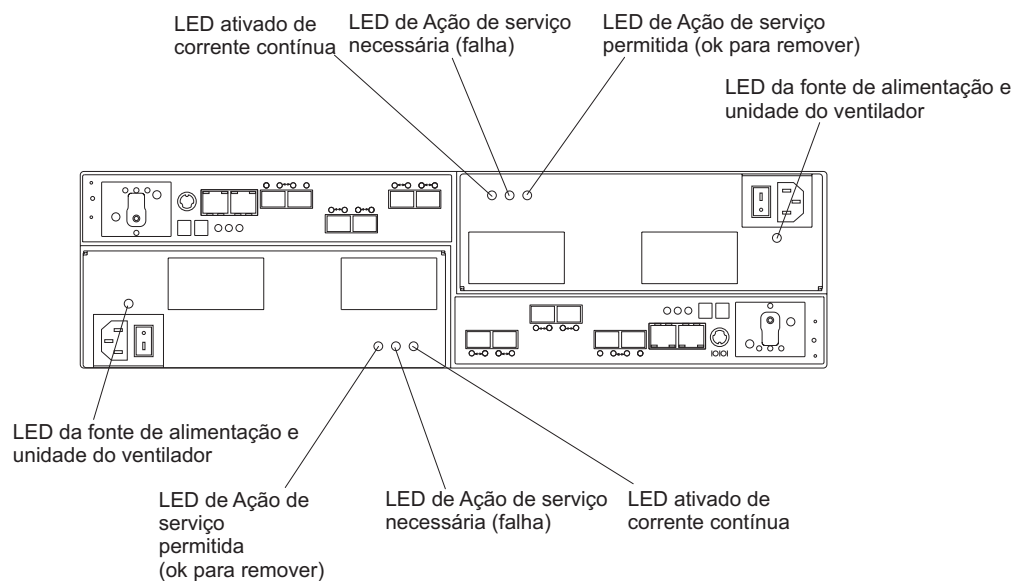
Figura 66. LEDs da Unidade de Fonte de Alimentação e de Ventilador
