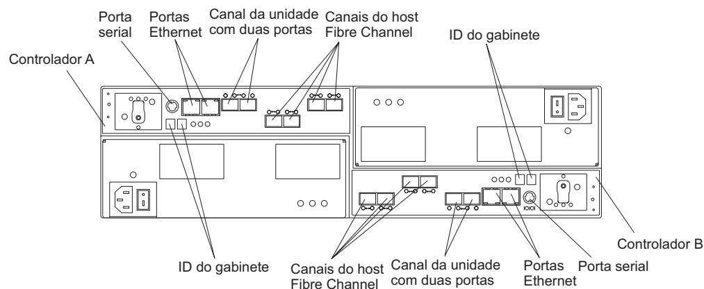
Figura 3. Vista posterior; controladores com dois canais de expansão de host padrão e dois opcionais Fibre Channel
