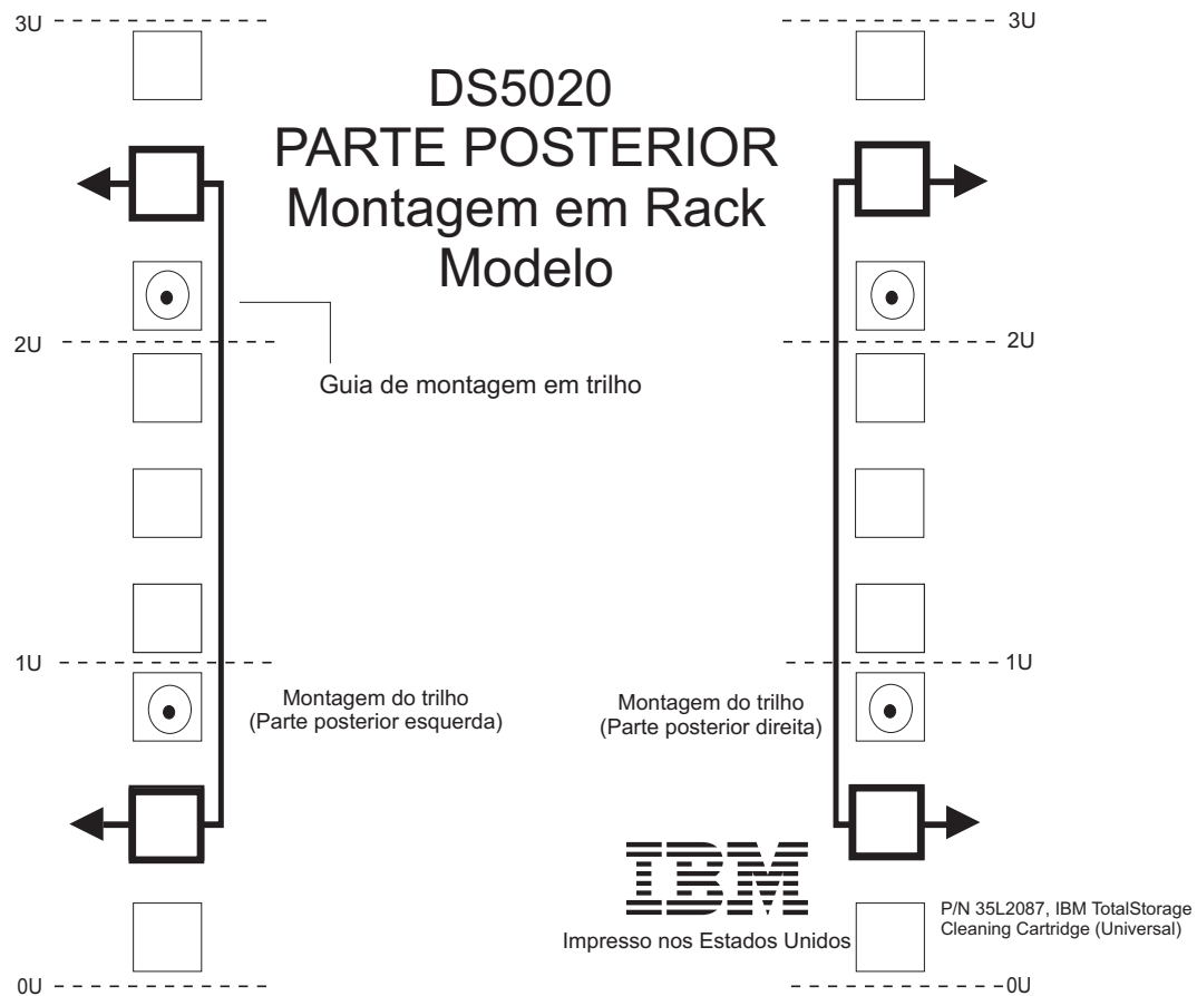
Figura 90. Gabarito de Montagem da Parte Traseira do Rack
