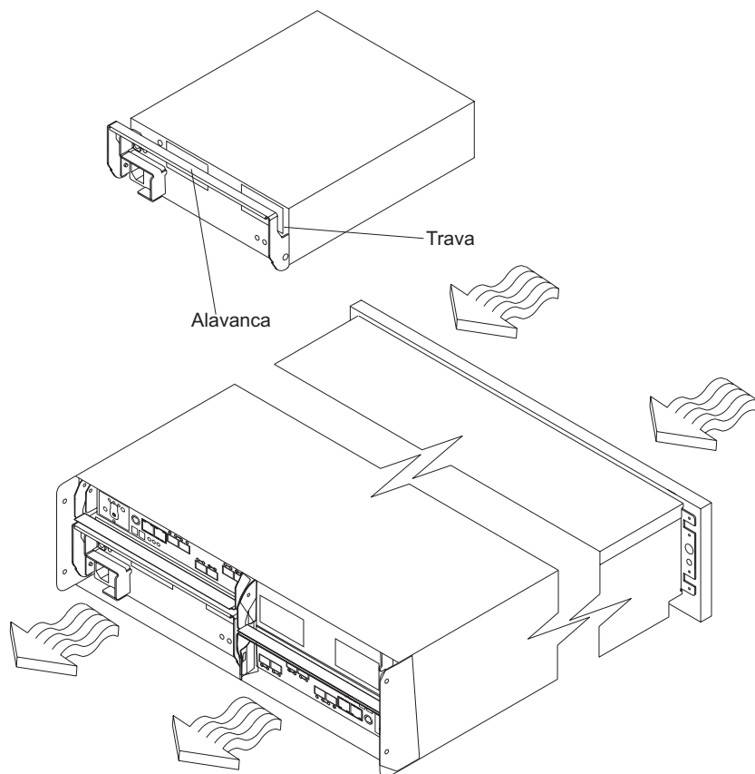
Figura 6. Fluxo de Ar da Unidade de Fonte de Alimentação e de Ventilador
