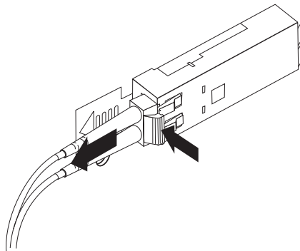
圖 34. 移除「LC-LC 光纖通道」纜線
