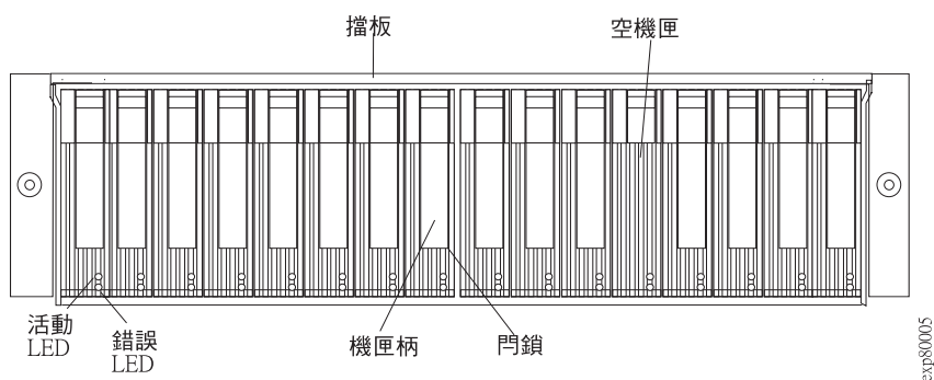
圖 79. 熱抽換 E-DDM LED
