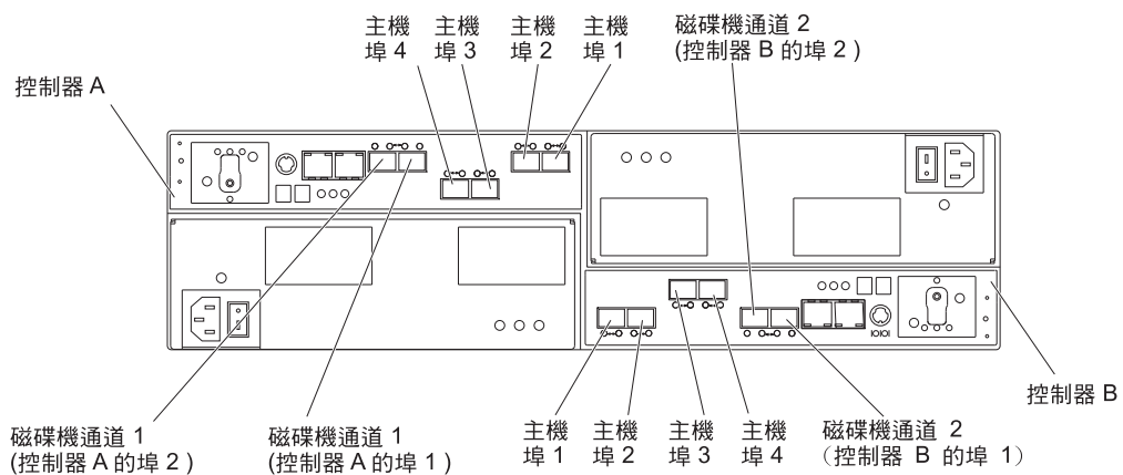
圖 36. DS5020 儲存體子系統埠及控制器
