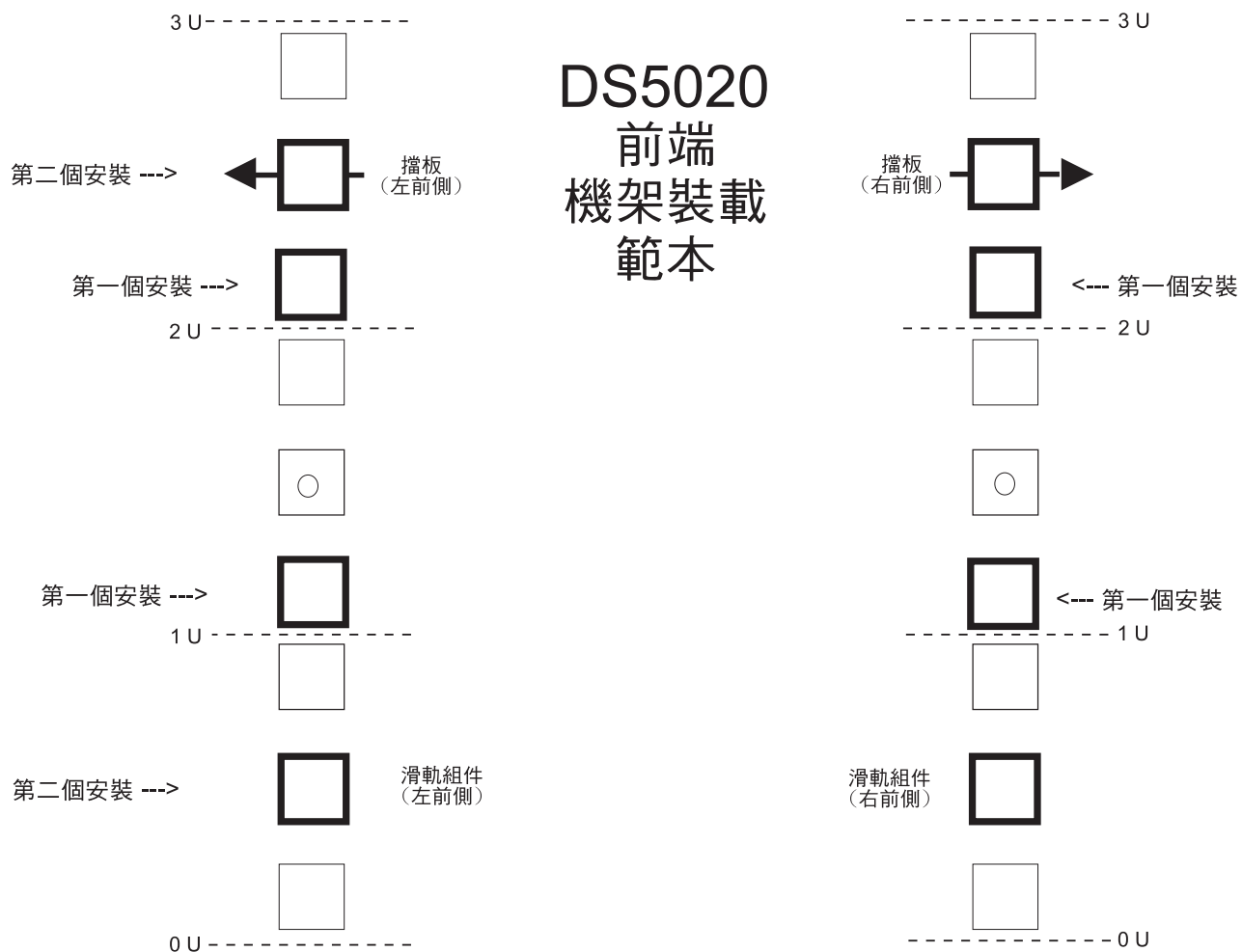
圖 89. 前端機架裝載範本
