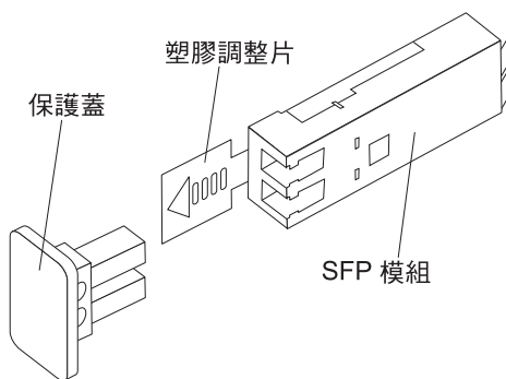
圖 27. 將 SFP 模組安裝至主機埠
