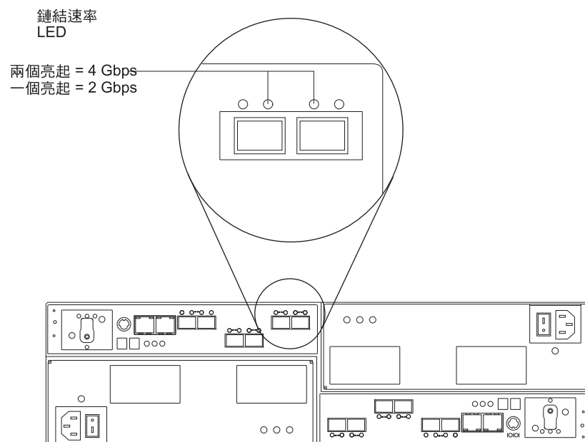
圖 81. 鏈結速率 LED
