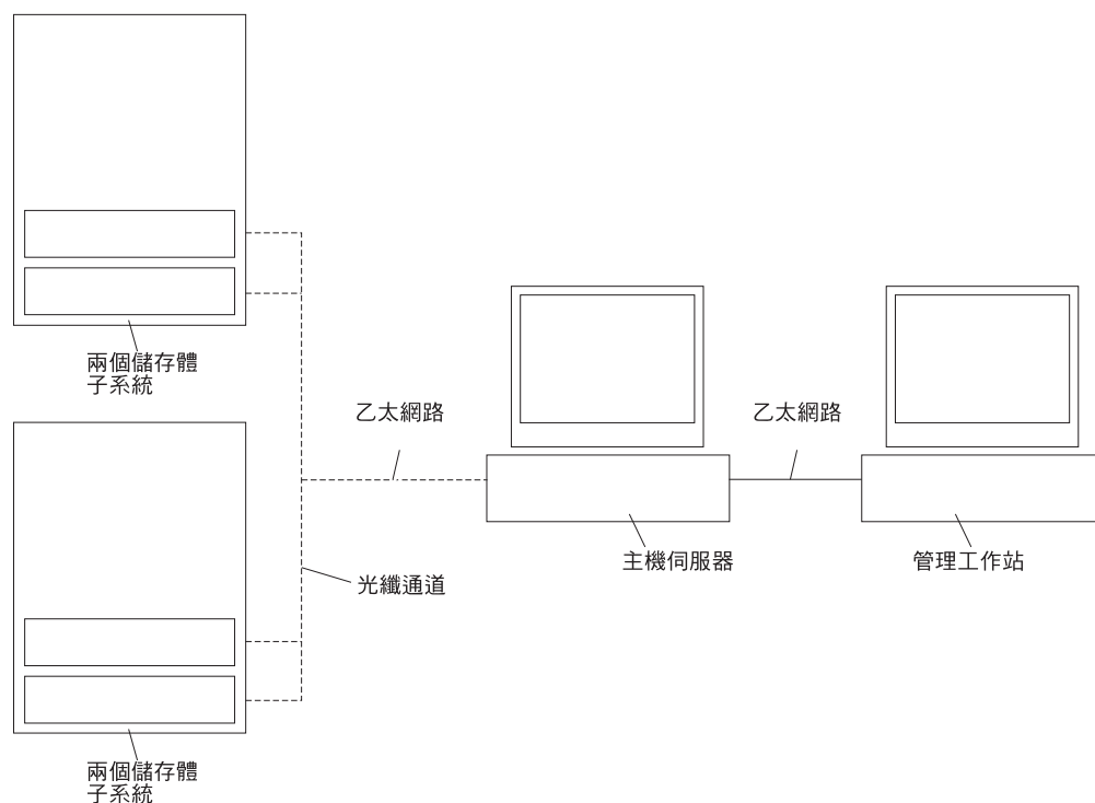
圖 52. 主機代理程式 (頻內) 管理的儲存體子系統
