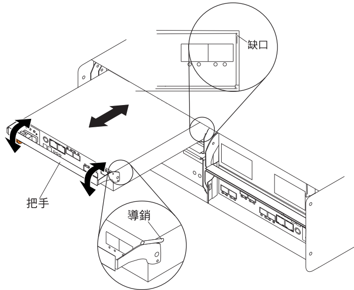
圖 21. 移出及裝回控制器
