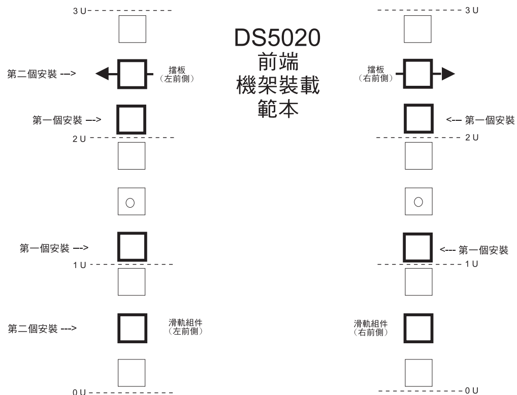
圖 13. 前端機架裝載範本
