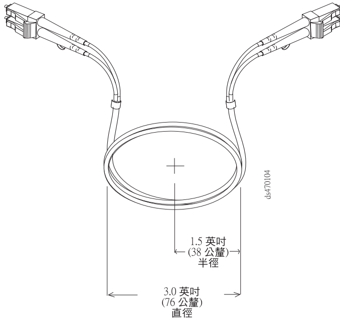
圖 25. 光纖纜線的彎曲及線圈規格
