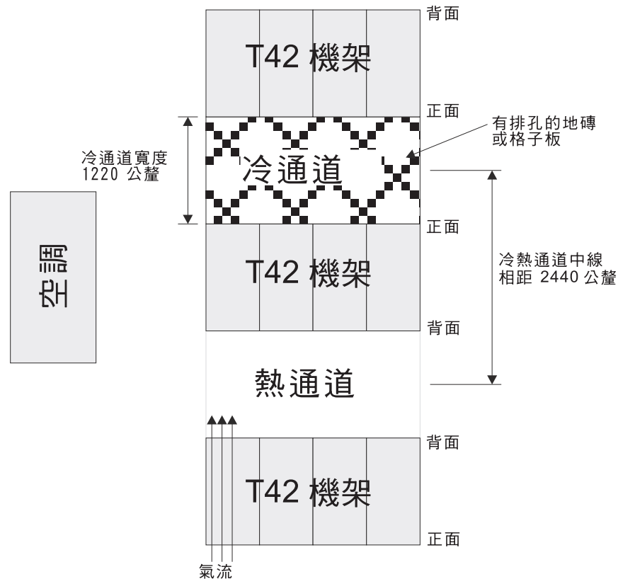
圖 11. 冷通道/熱通道機架配置的範例
