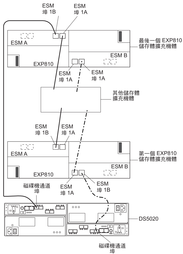
圖 45. 連接至 EXP810 ESM 埠且標籤為 1B 的 DS5020 磁碟機埠
