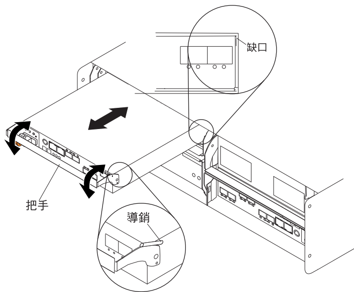
圖 78. 安裝控制器
