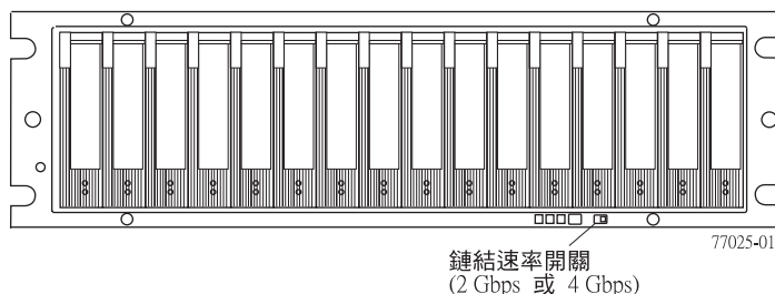
圖 82. 鏈結速率開關
