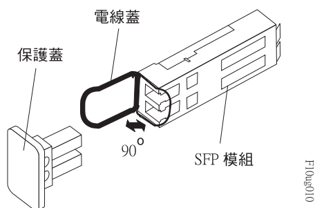
圖 76. 鬆開 SFP 模組門鎖 - 金屬種類
