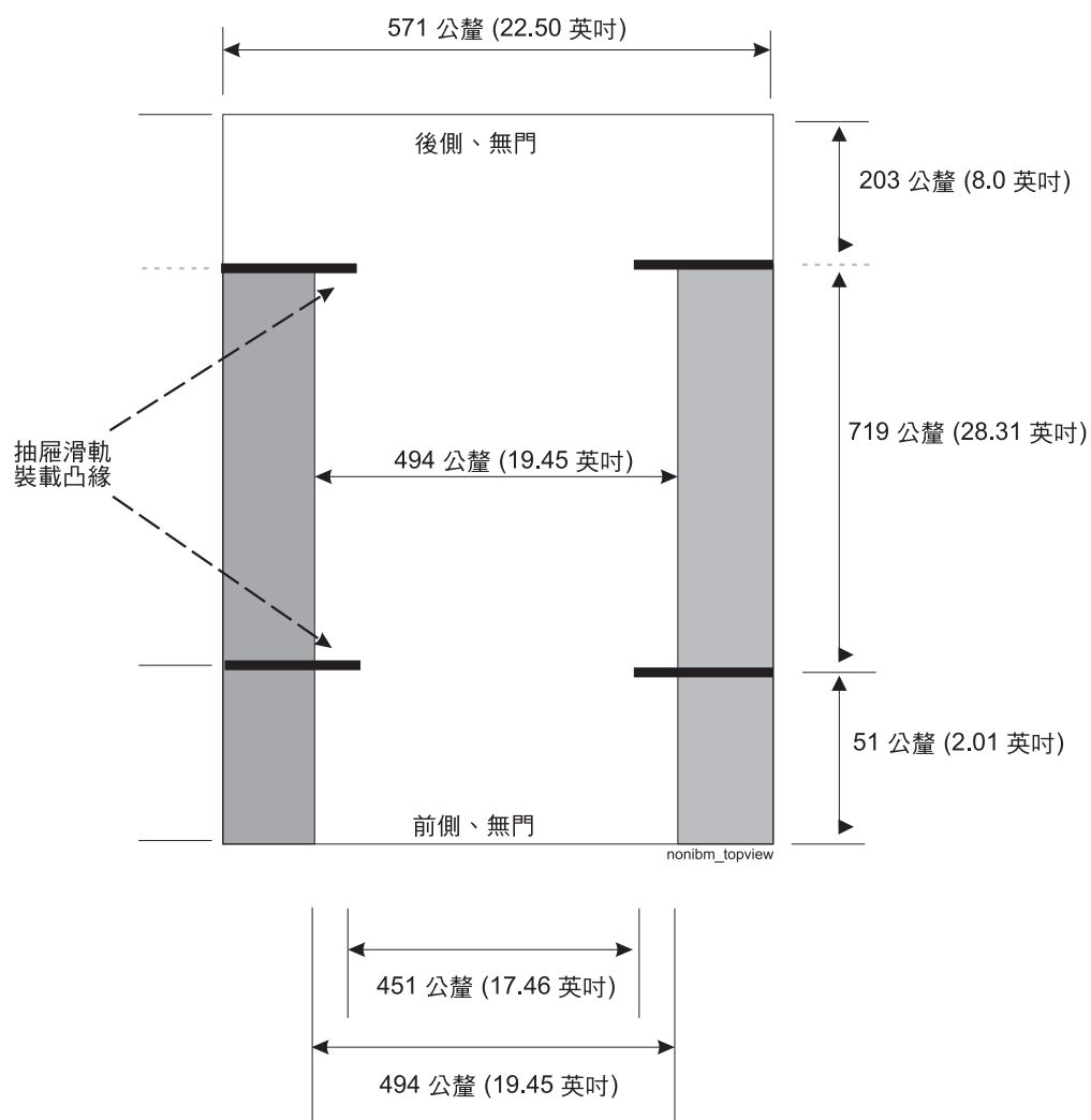
圖 91. 非 IBM 機架規格尺寸的頂端視圖
