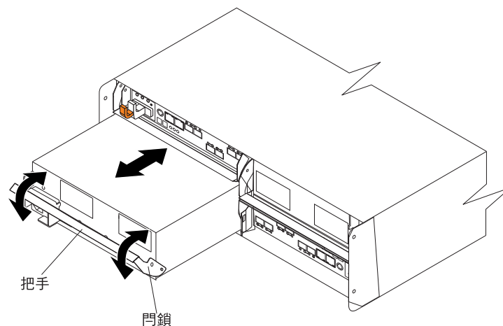
圖 17. 移除電源供應器及風扇裝置
