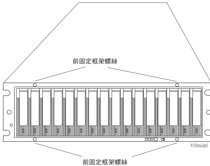
圖 86. 前固定框架螺絲位置
