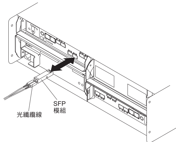
圖 85. 更換 SFP 模組
