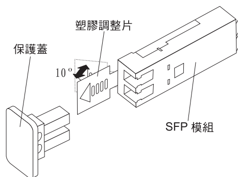
圖 28. 鬆開 SFP 模組門鎖 - 塑膠種類
