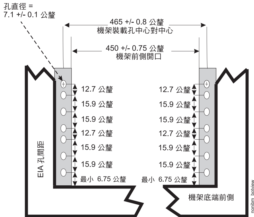
圖 93. 機架規格尺寸，底端前側視圖
