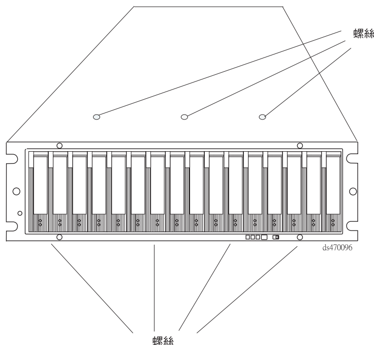
圖 87. 將機箱頂端及底端與固定框架固定在一起的螺絲
