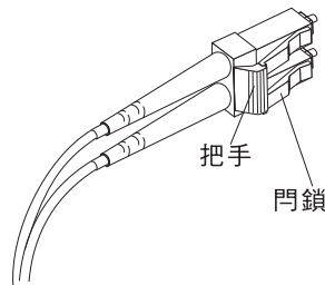
圖 33. 「LC-LC 光纖通道」纜線把手及門鎖
