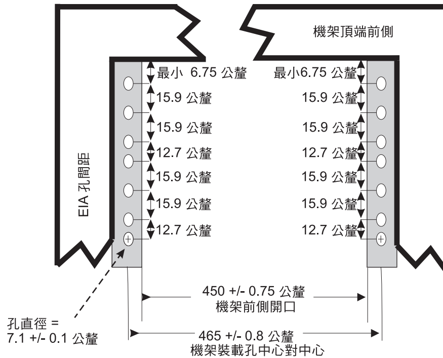
圖 92. 機架規格尺寸，頂端前側視圖
