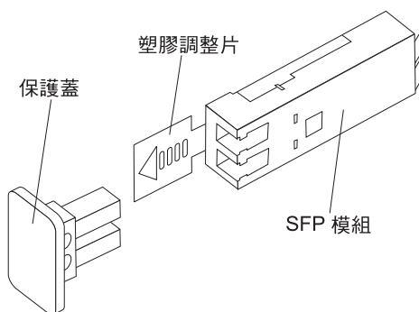
圖 26. SFP 模組及保護蓋
