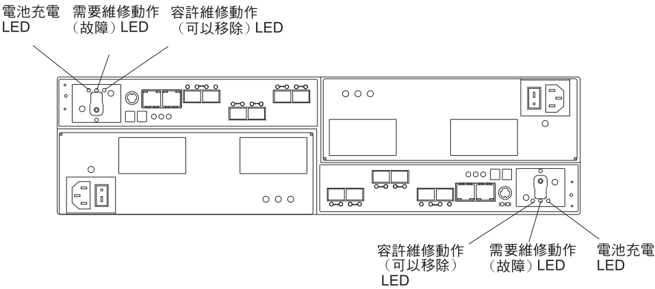
圖 68. 電池裝置 LED
