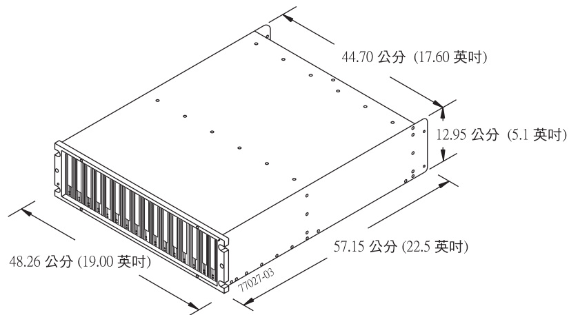
圖 9. DS5020 尺寸
