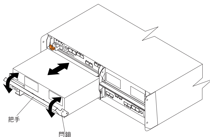
圖 83. 更換電源供應器及風扇裝置
