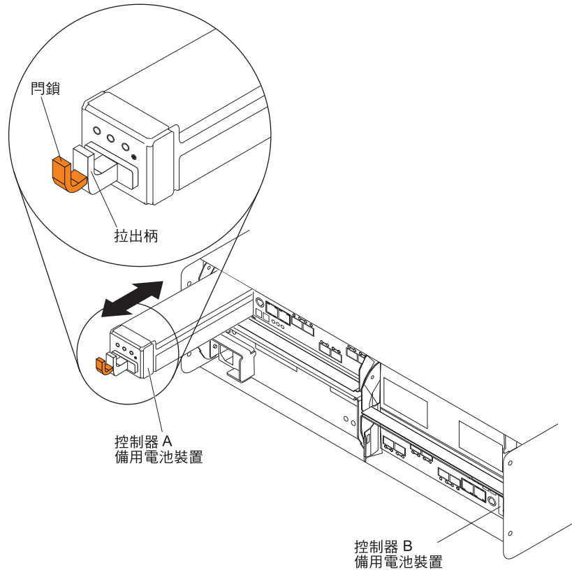
圖 84. 移除並更換控制器機箱中的電池裝置
