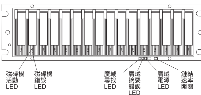
圖 67. 正面的 LED 及控制項
