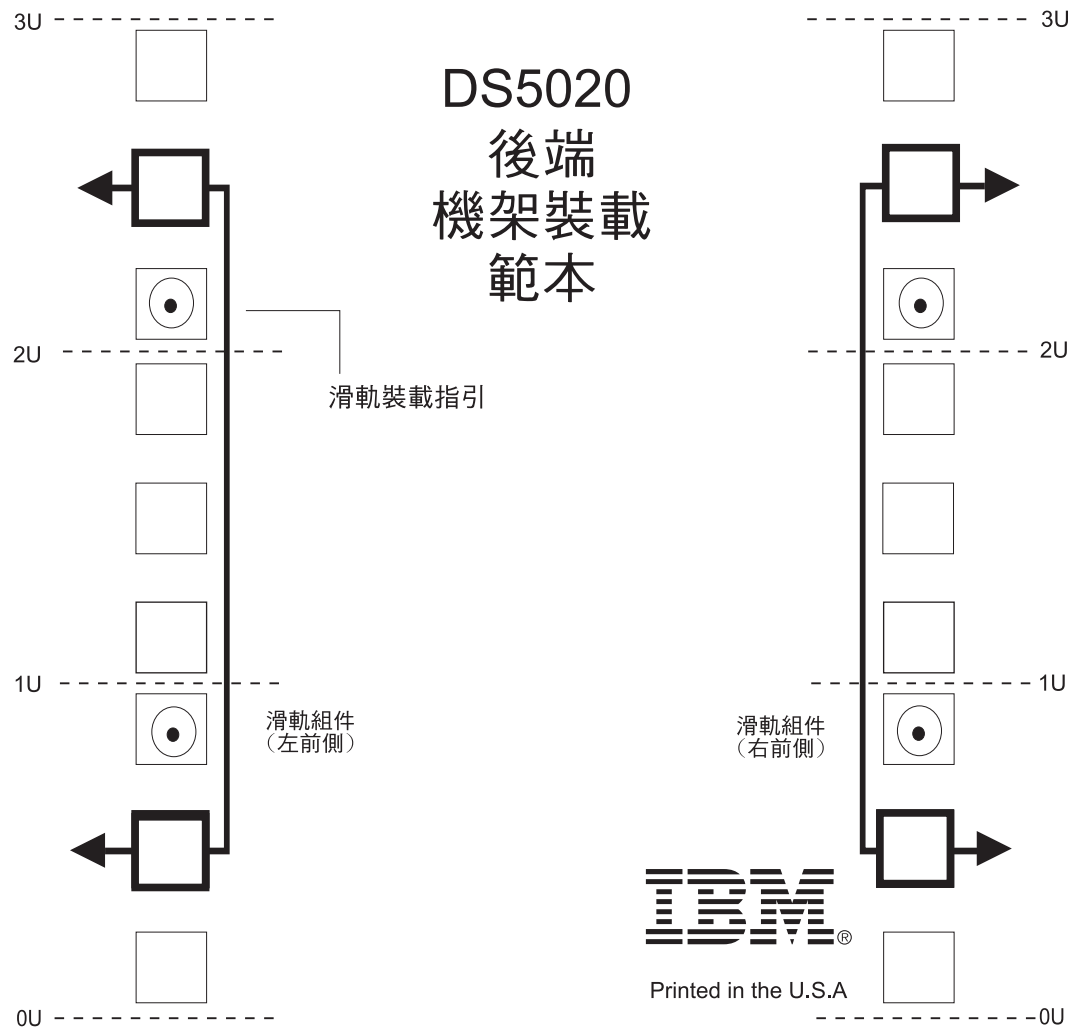
圖 90. 後端機架裝載範本
