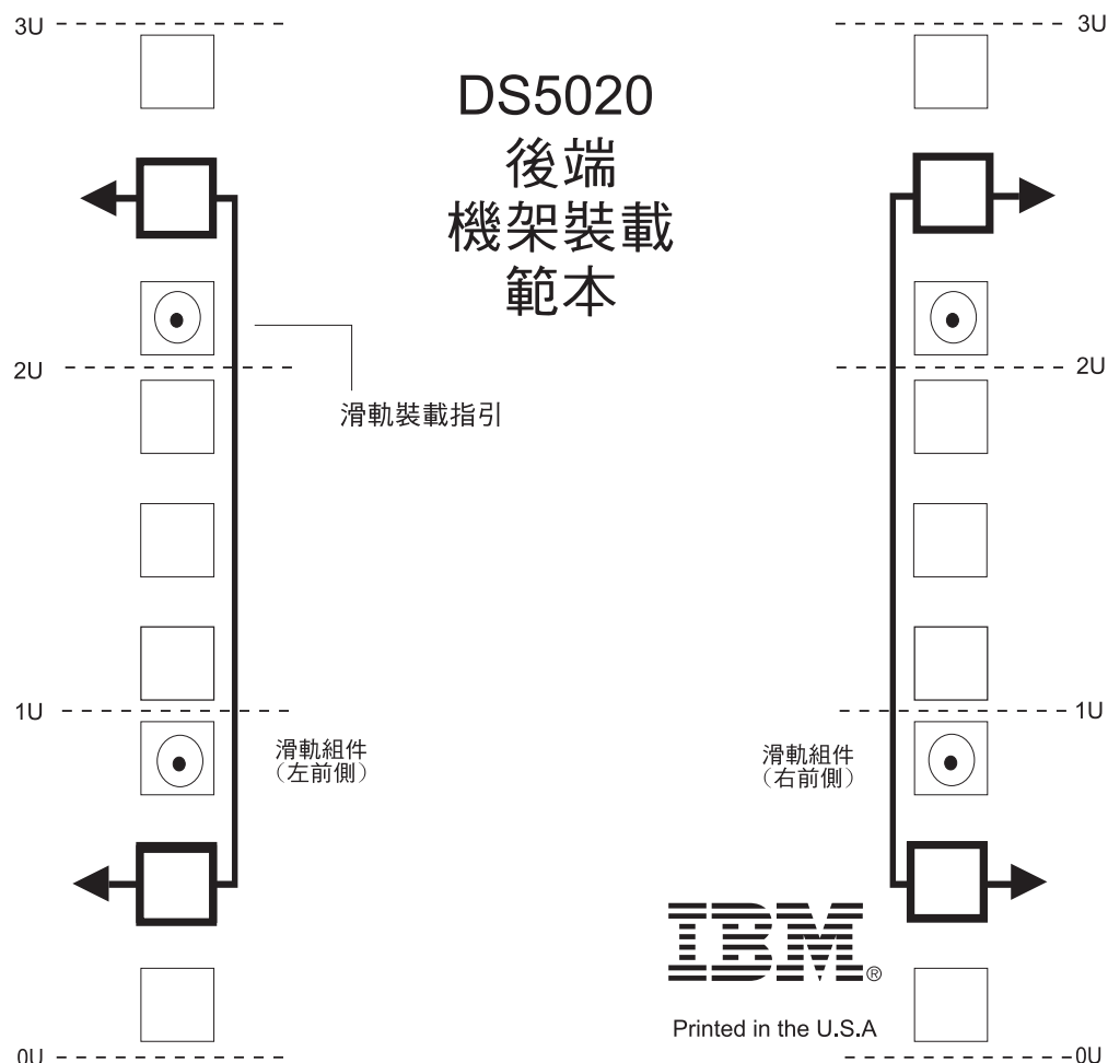
圖 14. 後端機架裝載範本
