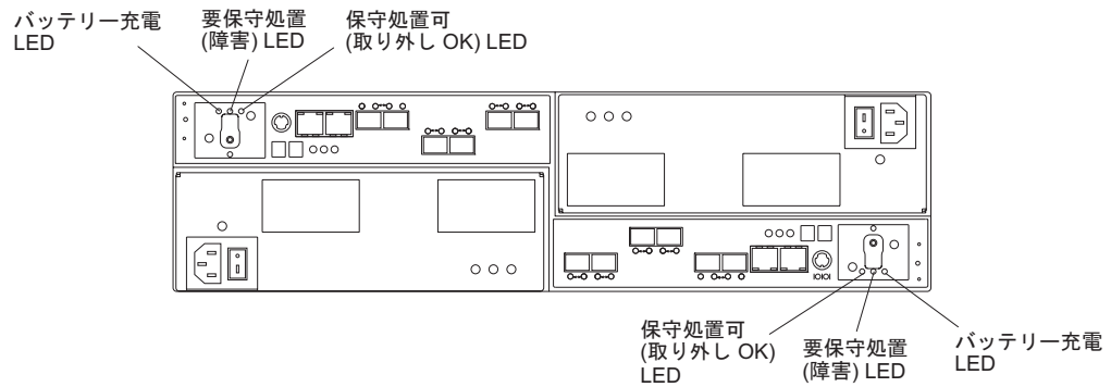
図 68. バッテリー・ユニット LED
