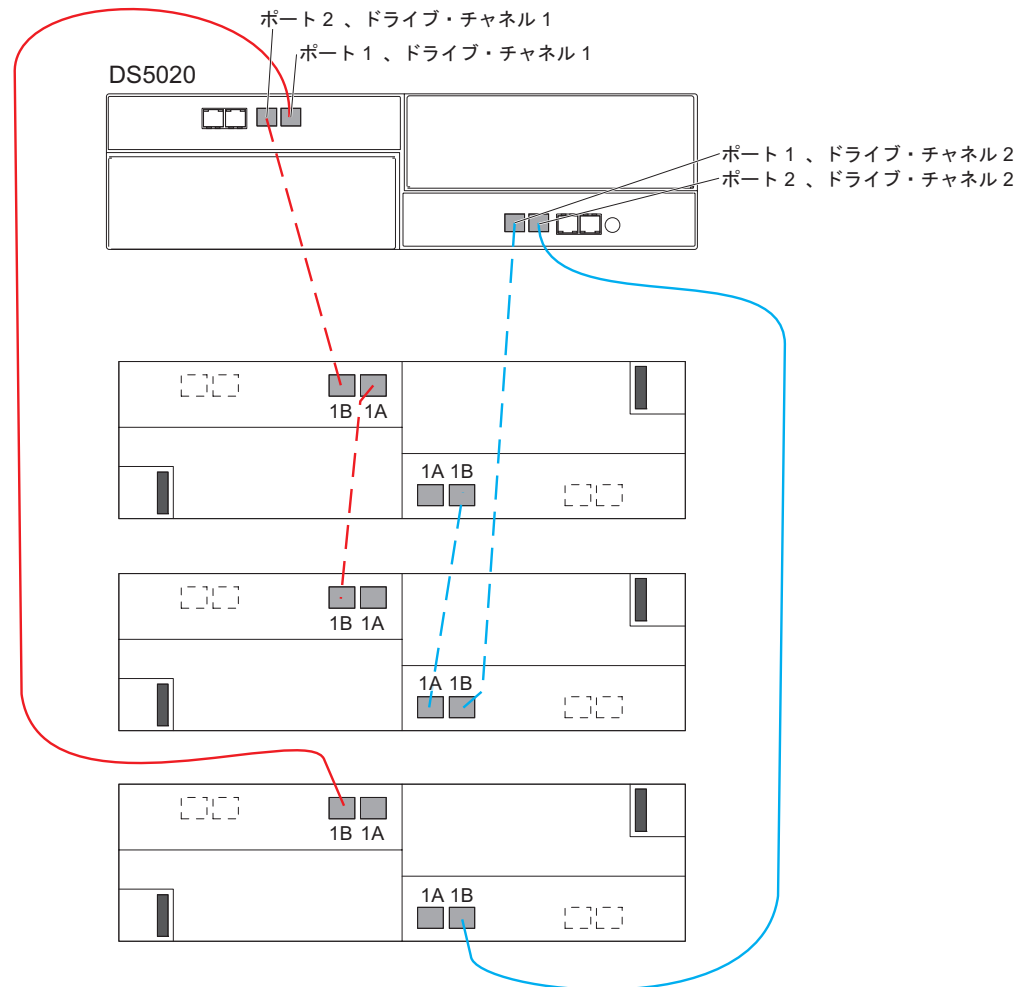
図 40. 1 つの DS5020 と 3 つのストレージ拡張エンクロージャーのケーブル接続
