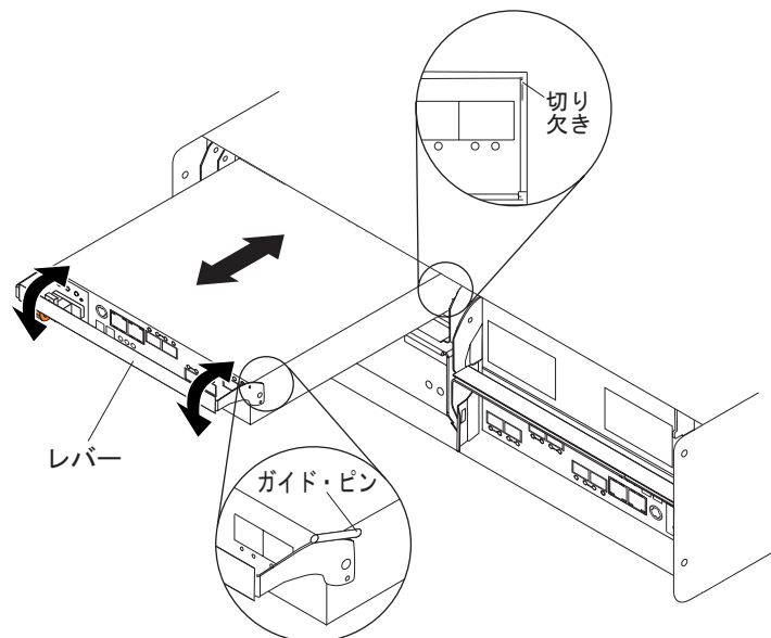
図 78. コントローラーの取り付け
