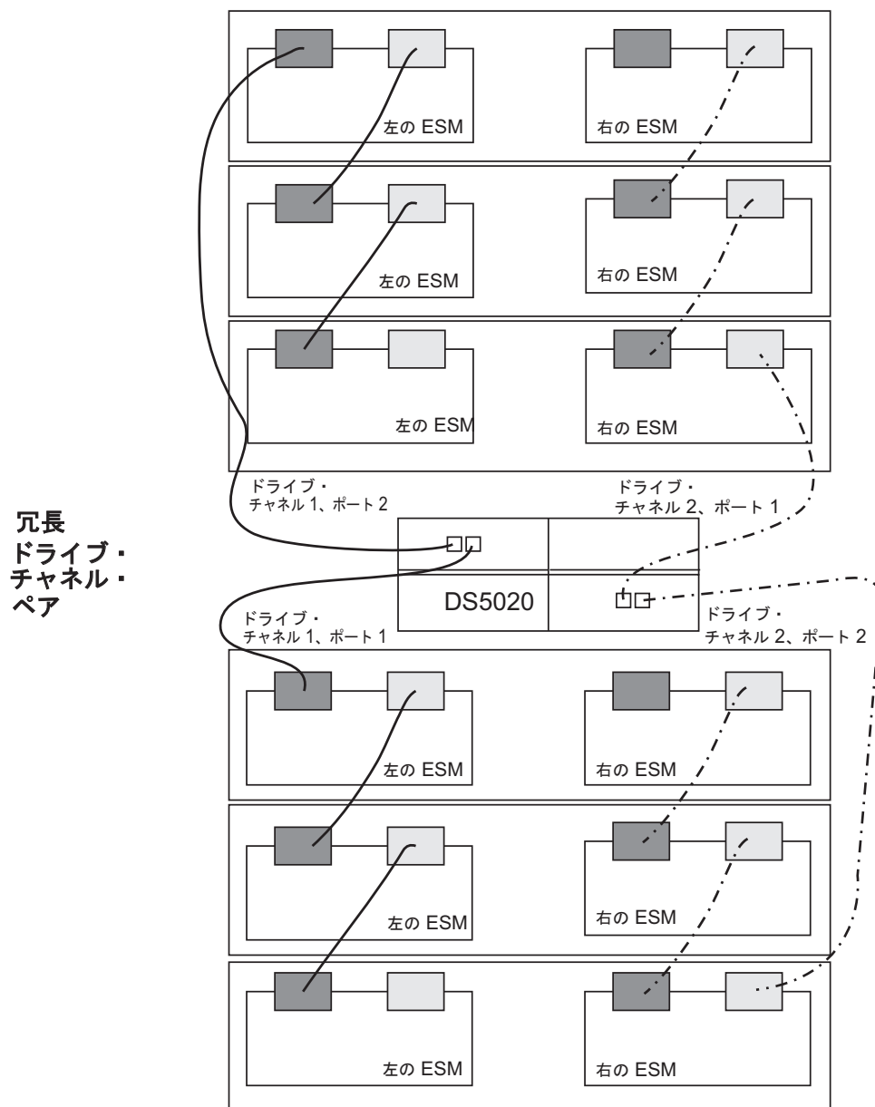
図 35. 冗長ドライブ・チャンネル・ペアの例
