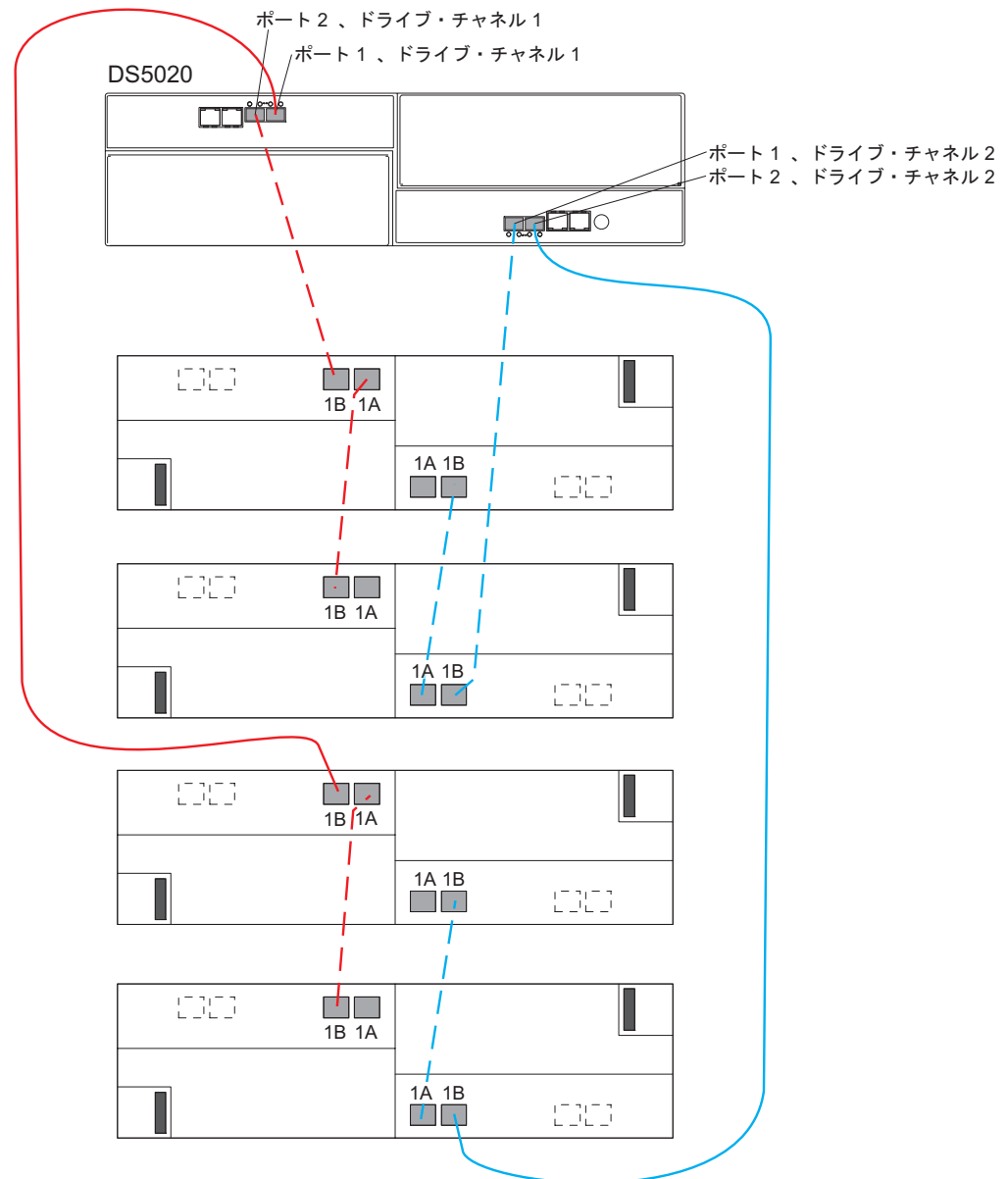
図 41. 1 つの DS5020 と 4 つのストレージ拡張エンクロージャのケーブル接続
