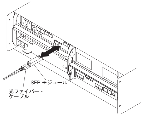
図 8. SFP モジュールと光ファイバー・ケーブル
