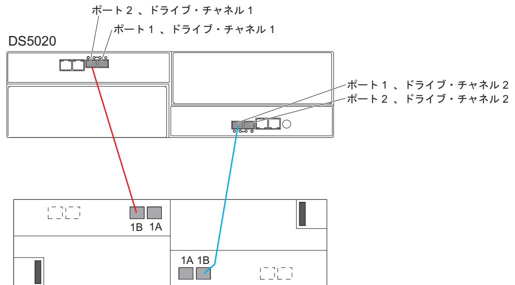
図 37. 1 つの DS5020 と 1 つのストレージ拡張エンクロージャのケーブル接続
