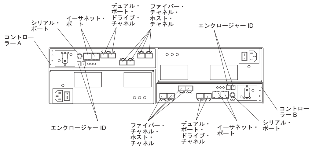
図 3. 2 つの標準および 2 つのオプションのファイバー・チャンネル・ホスト拡張チャンネルを搭載したコントローラーの背面図
