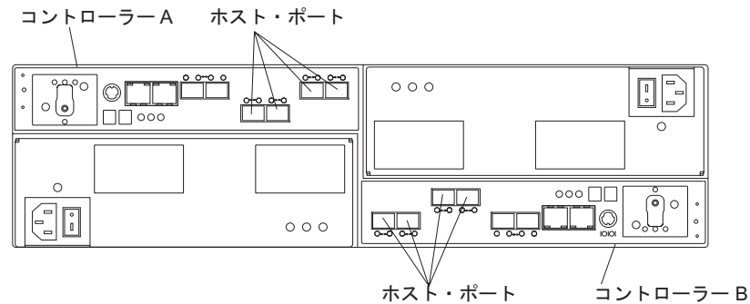
図 54. DS5020 の RAID コントローラー上のホスト・ケーブルの位置
