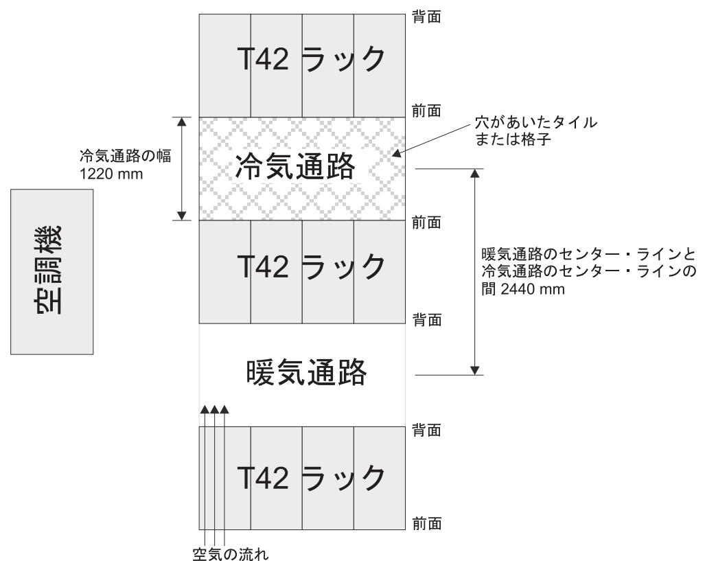
図 11. 冷気通路/暖気通路ラック構成の例
