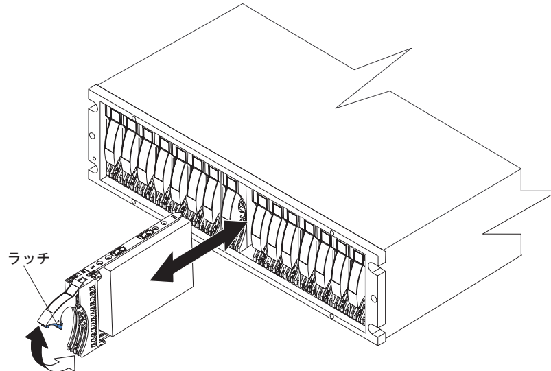
図 18. E-DDM CRU の取り外し
