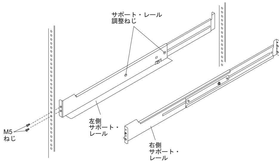
図 15. サポート・レールの取り付け
