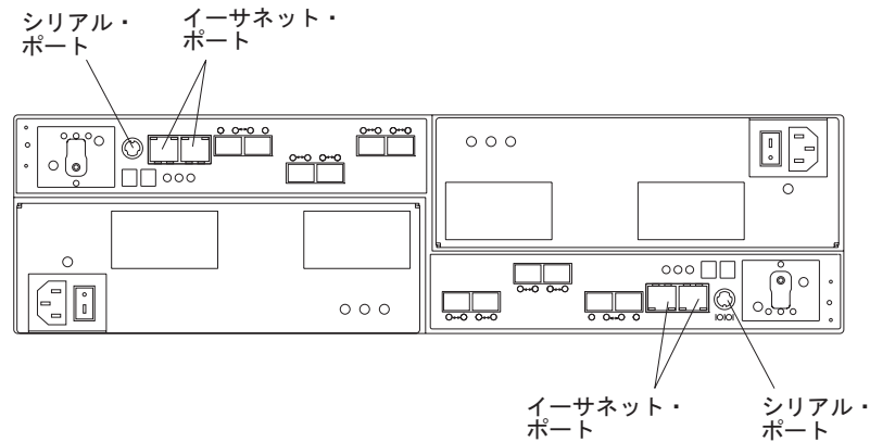
図 51. DS5020 のイーサネットおよびシリアル・ポートの位置
