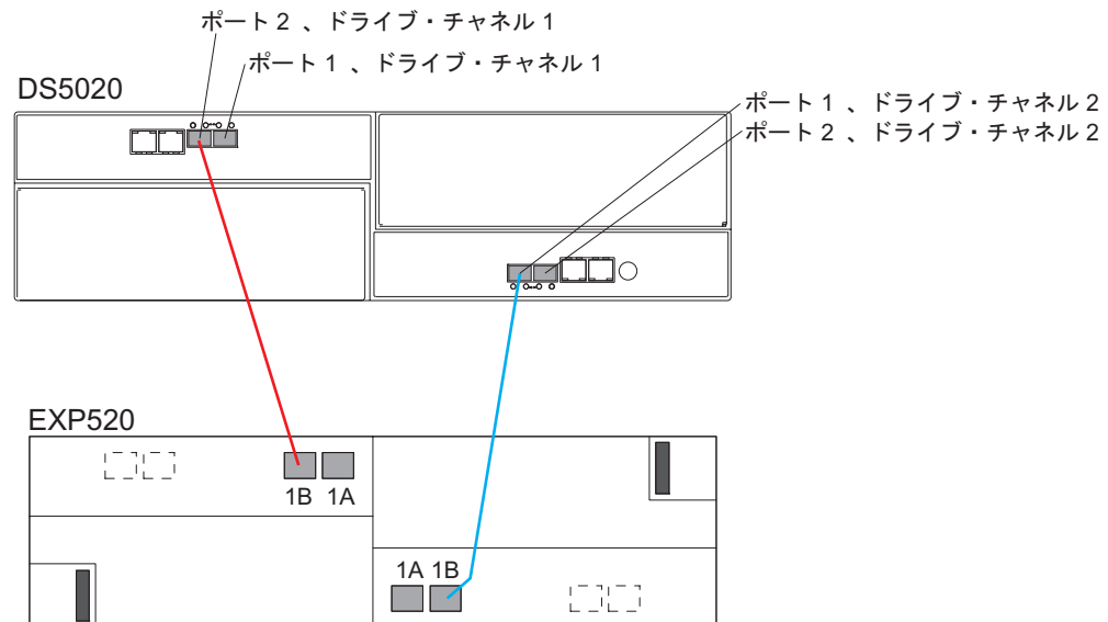
図 46. 1 つの DS5020 と 1 つの EXP520 ストレージ拡張エンクロージャのケーブル接続
