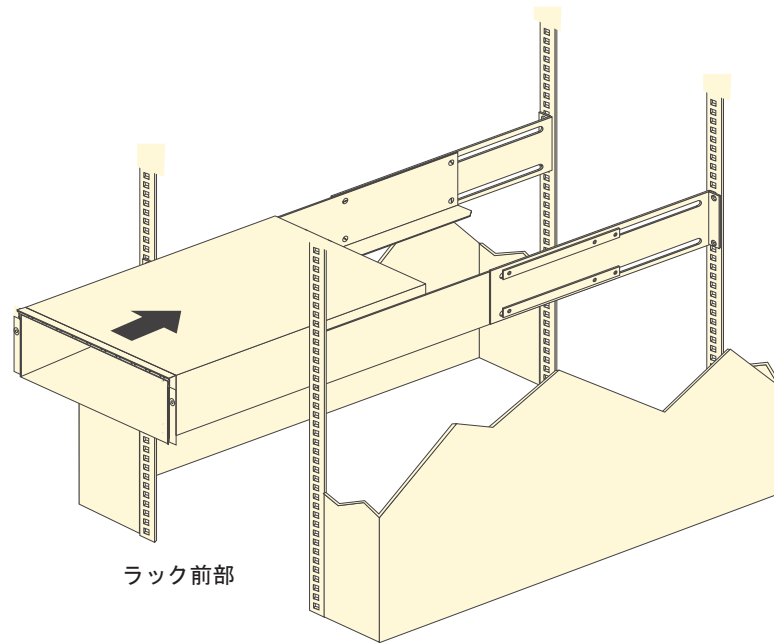
図 19. DS5020 の取り付け
