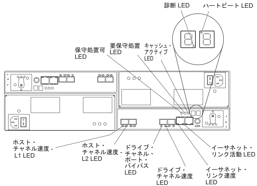
図 69. 2 つの標準ファイバー・チャンネル・ホスト拡張チャンネルを搭載したコントローラーの LED、制御、およびコネクタ
