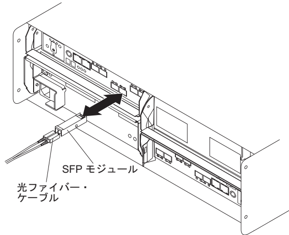
図 85. SFP モジュールの交換
