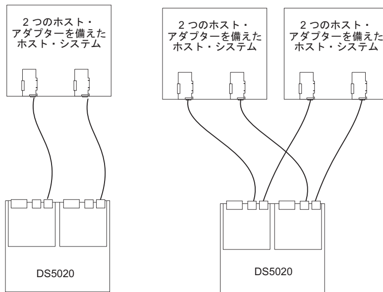
図 56. 冗長ホスト直接接続ファイバー・チャンネル構成の例
