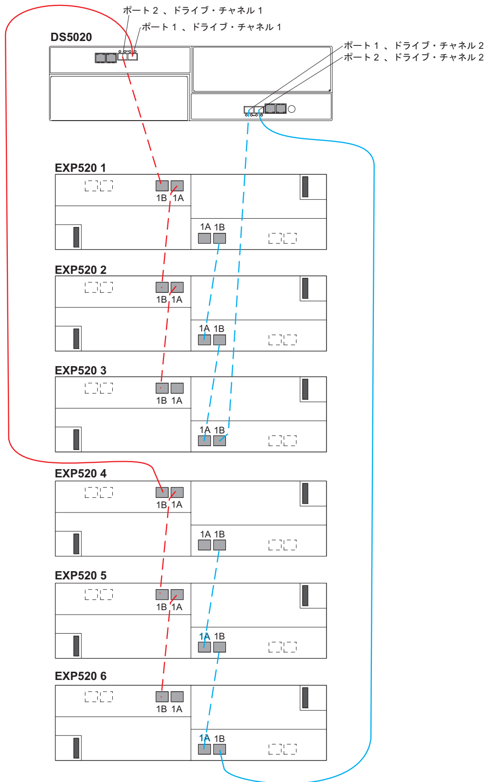
図 50. 1 組の DS5020 ドライブ・ポートの後ろでの 1 つの DS5020 と最大 6 つの EXP520 ストレージ拡張エンクロージャー
