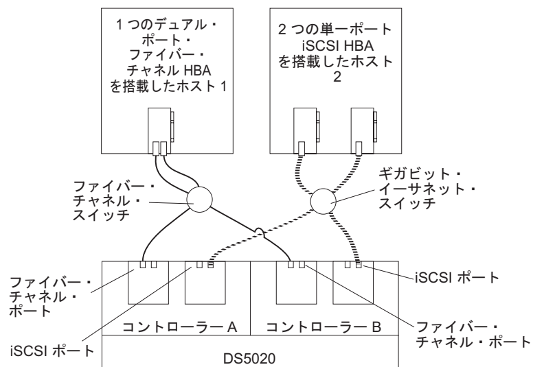
図 63. iSCSI およびファイバー・チャネル・ホスト、複数ポート構成の例
