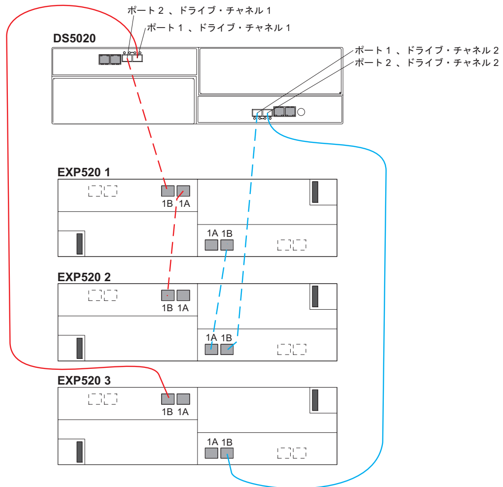
図 48. 1 組の DS5020 ドライブ・ポートの後ろでの 1 つの DS5020 と 3 つの EXP520 ストレージ拡張エンクロージャー
