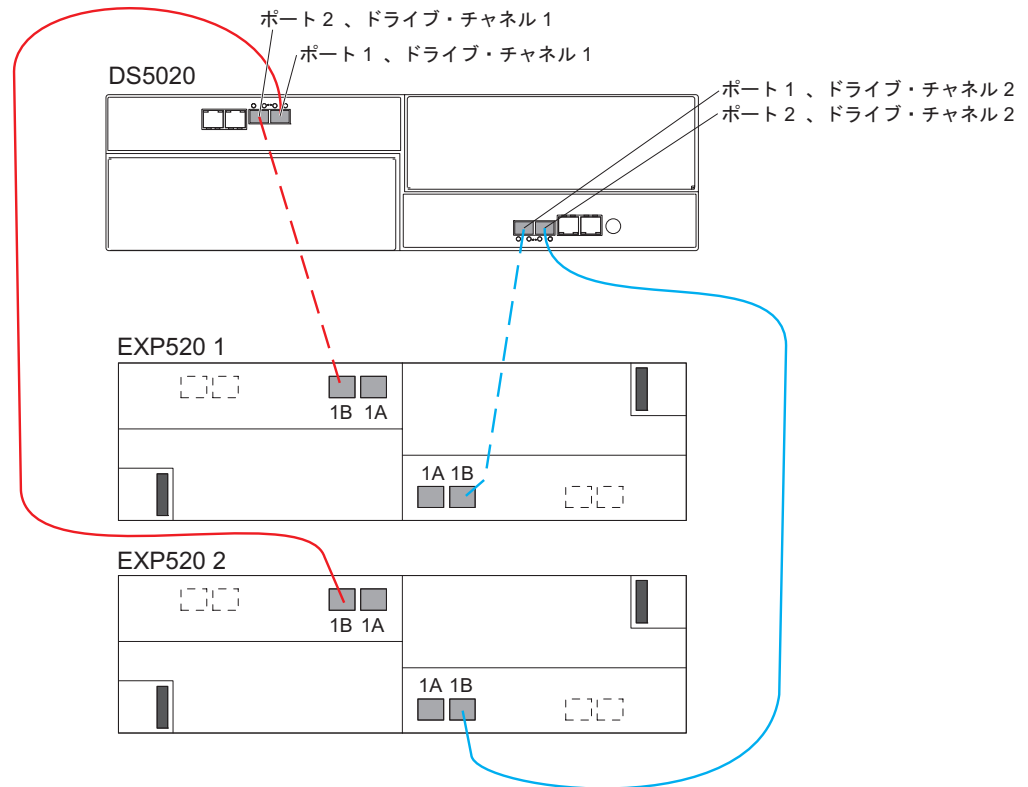
図 47. 1 組の DS5020 ドライブ・ポートの後ろでの 1 つの DS5020 と 2 つの EXP520 ストレージ拡張エンクロージャ
