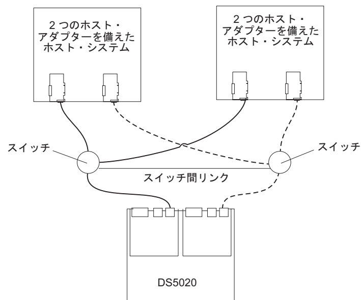
図 57. 単一 SAN ファブリック構成の例
