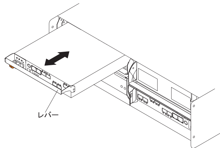
図 16. コントローラーの取り外しと再取り付け
