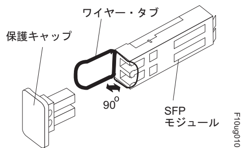
図 76. SFP モジュール・ラッチのアンロック - ワイヤー・タブの場合
