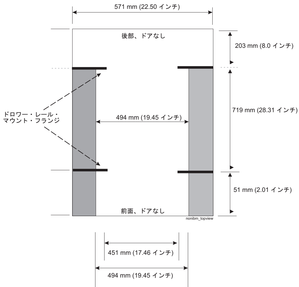
図 91. IBM 以外のラックの仕様寸法の平面図
