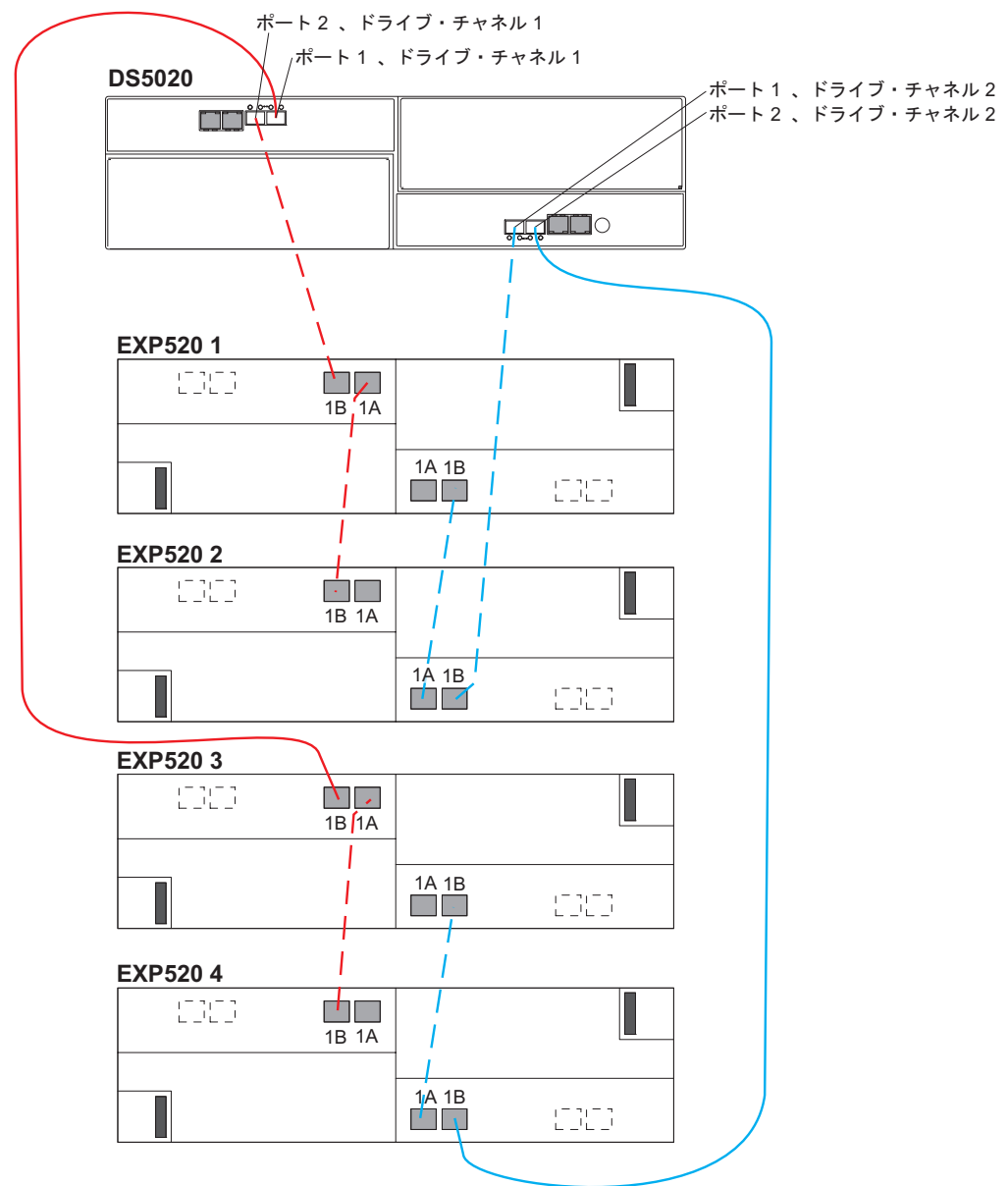
図 49. 1 組の DS5020 ドライブ・ポートの後ろでの 1 つの DS5020 と 4 つの EXP520 ストレージ拡張エンクロージャ
