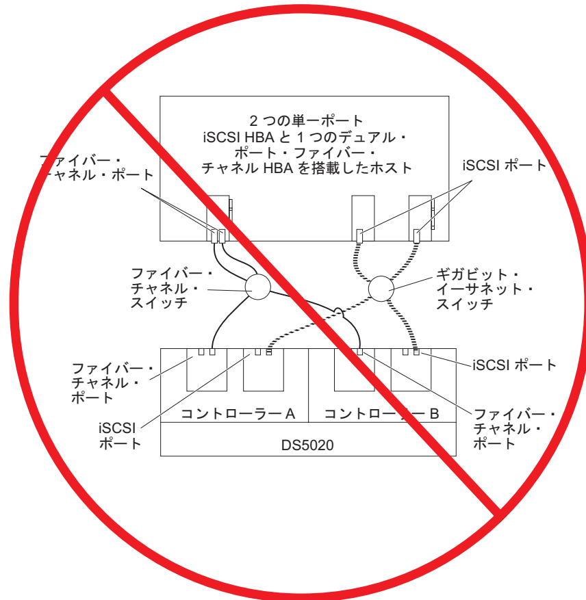
図 64. 誤った構成の例: 単一ホスト、iSCSI およびファイバー・チャネル
