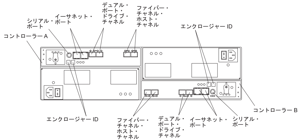
図 2. 2 つの標準ファイバー・チャンネル・ホスト拡張チャンネルを搭載したコントローラーの背面図
