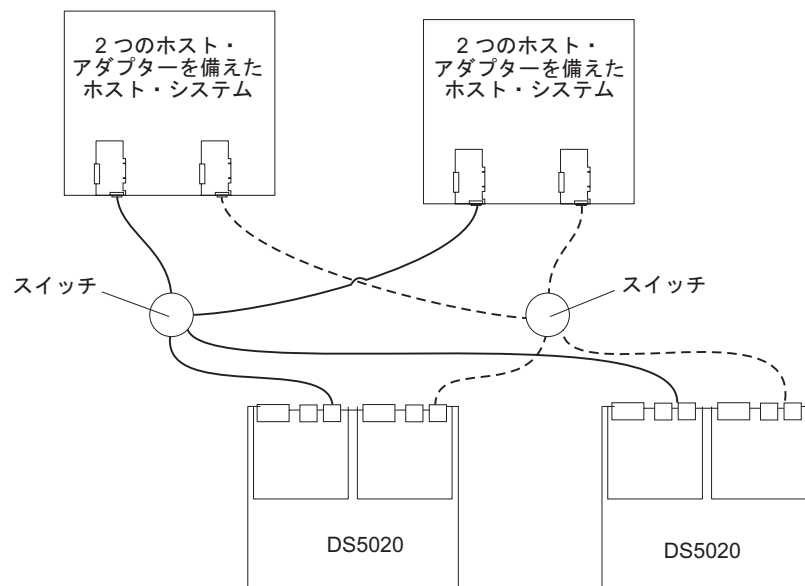
図 59. 二重 SAN 環境の 2 つのストレージ・サブシステムの例
