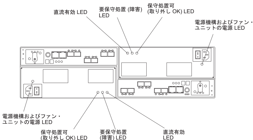
図 66. 電源機構およびファン・ユニット LED
