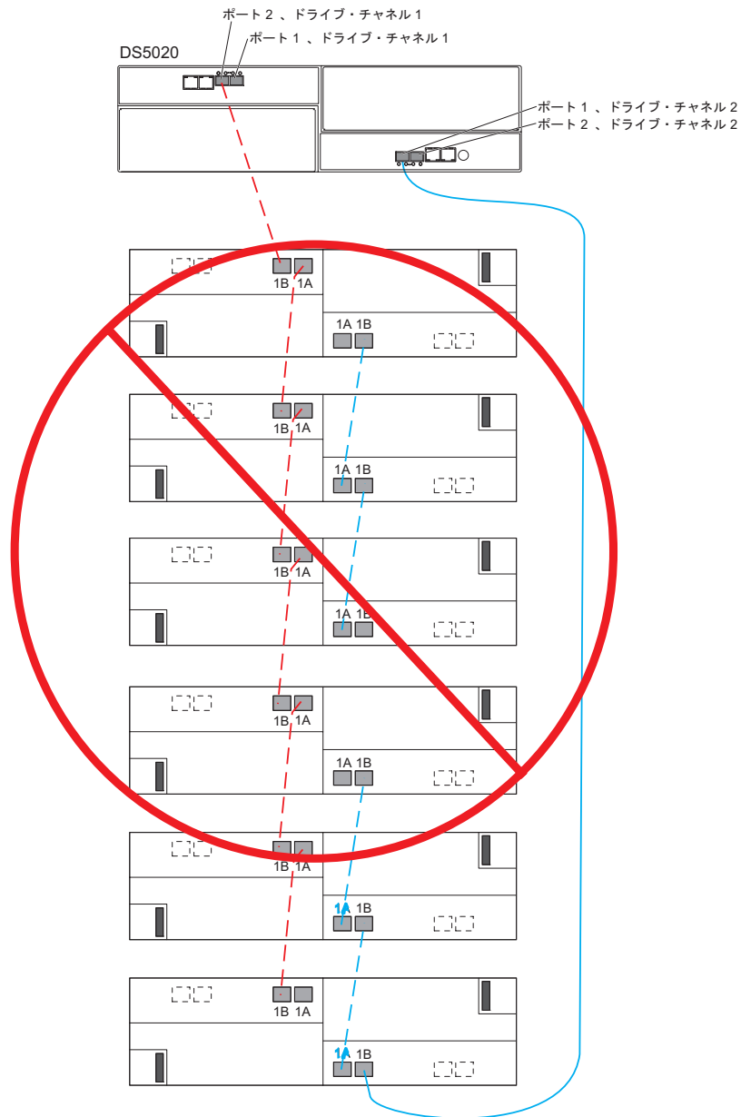
図 43. 1 つの DS5020 と最大 6 つのストレージ拡張エンクロージャーのケーブル接続
