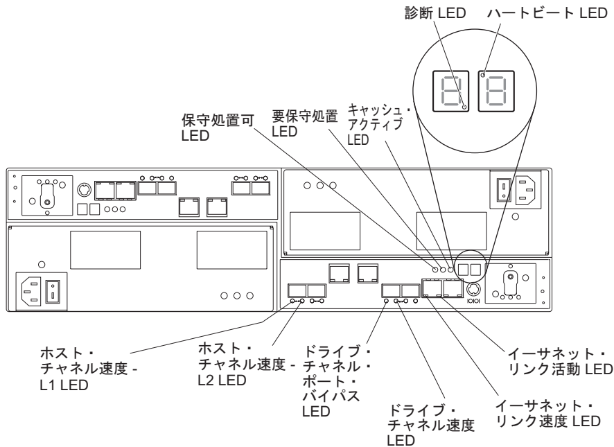
図 71. 2 つの標準ファイバー・チャンネル・ホスト拡張チャンネルおよび 2 つのオプション iSCSI ホスト通信路チャンネルを搭載したコントローラーの LED、制御、およびコネクタ
