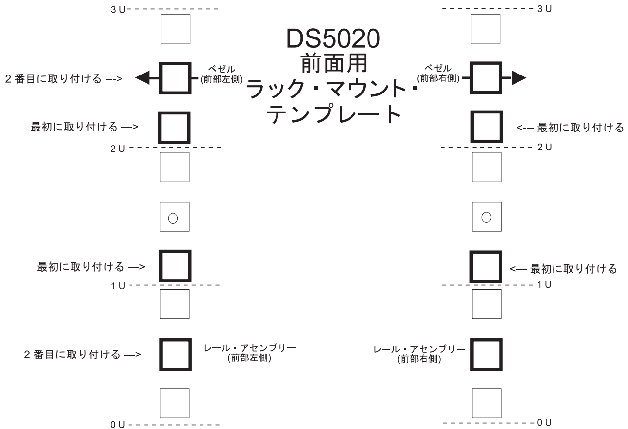
図 89. 前面用ラック・マウント・テンプレート
