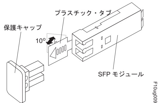
図 75. SFP モジュール・ラッチのアンロック - プラスチック・タブの場合
