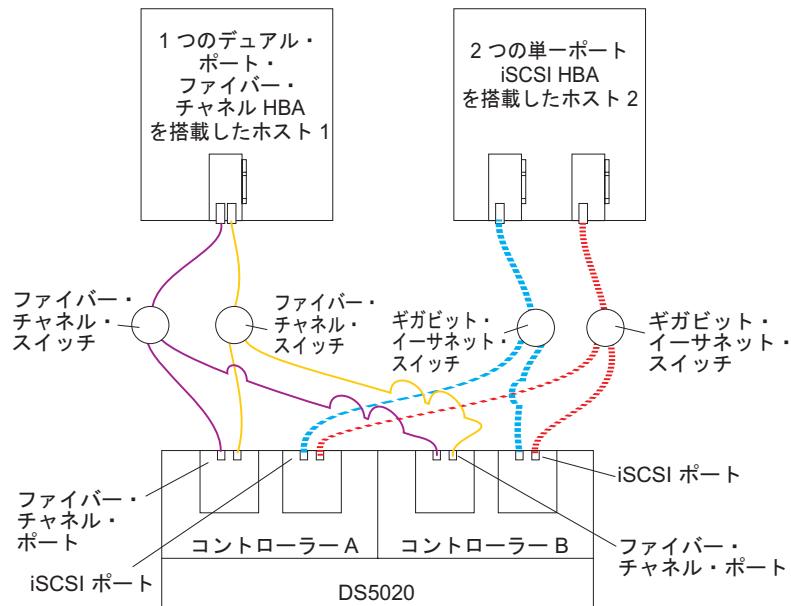
図 65. 複数ホスト、複数ポート、複数スイッチ構成の例
