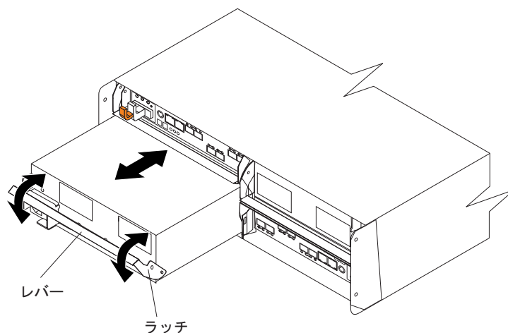
図 83. 電源機構およびファン・ユニットの交換
