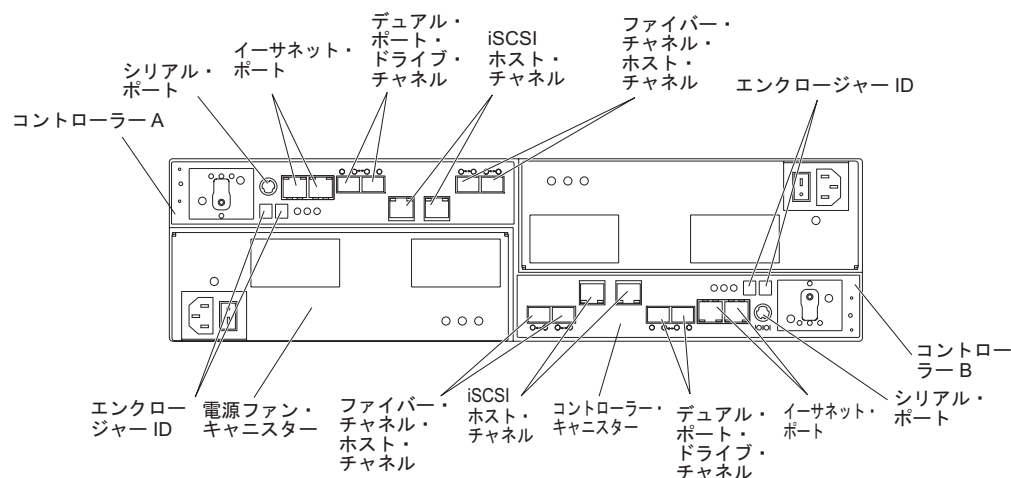
図 4. 2 つの標準ファイバー・チャンネル・ホスト拡張チャンネルおよび 2 つのオプション iSCSI ホスト拡張チャンネルを搭載したコントローラーの背面図
