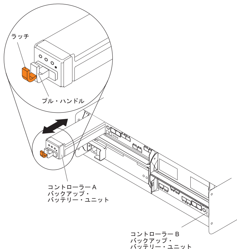
図7. バックアップ・バッテリー・ユニット
