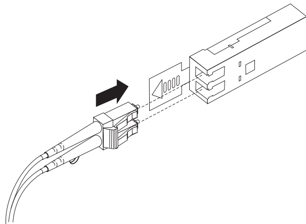
図 32. LC-LC ファイバー・チャネル・ケーブルの SFP モジュールへの挿入
