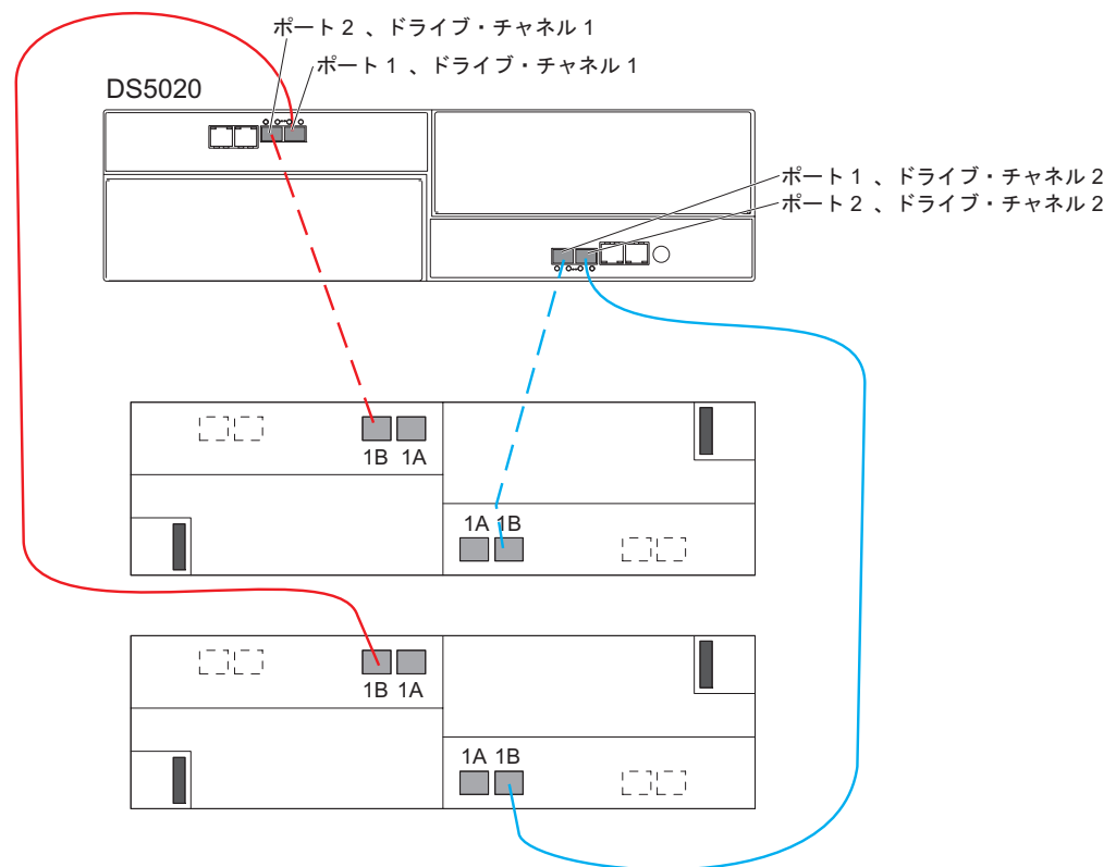
図 38. 1 つの DS5020 と 2 つのストレージ拡張エンクロージャーのケーブル接続
