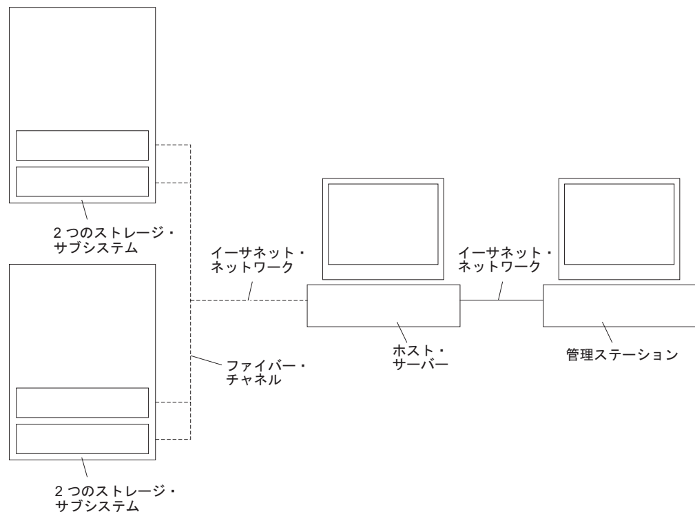
図 52. ホスト・エージェント (インバンド) 管理対象ストレージ・サブシステム
