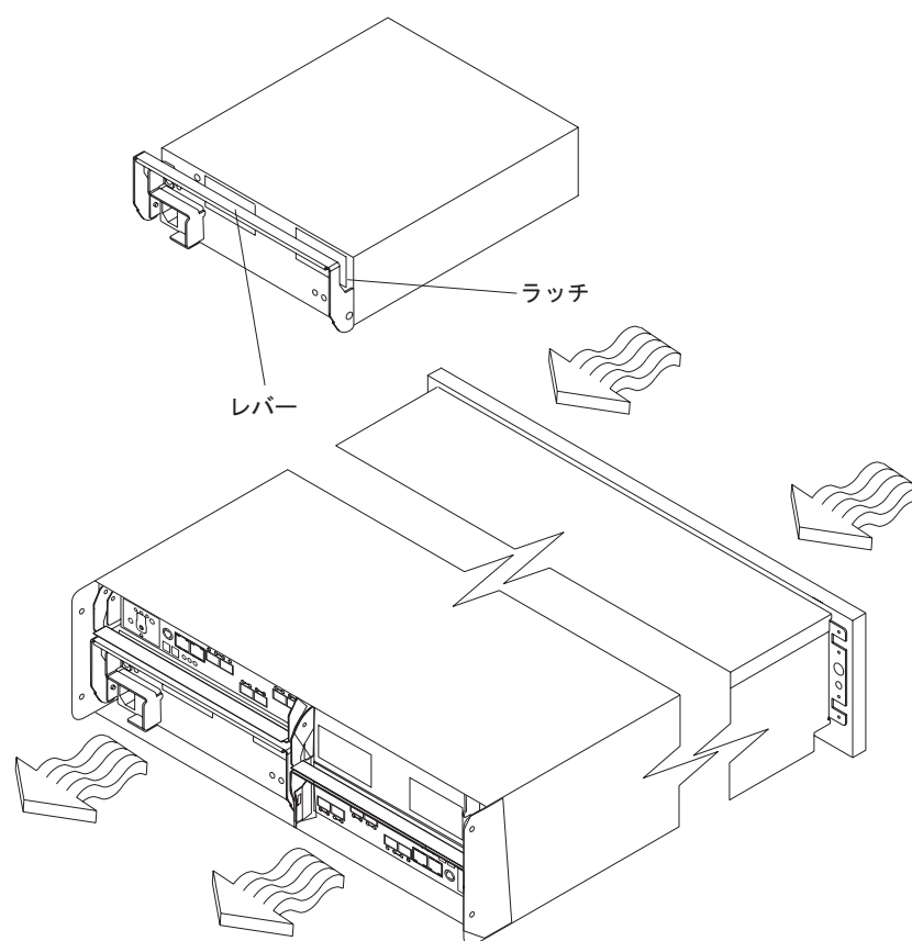
図 6. 電源機構およびファン・ユニットと空気の流れ
