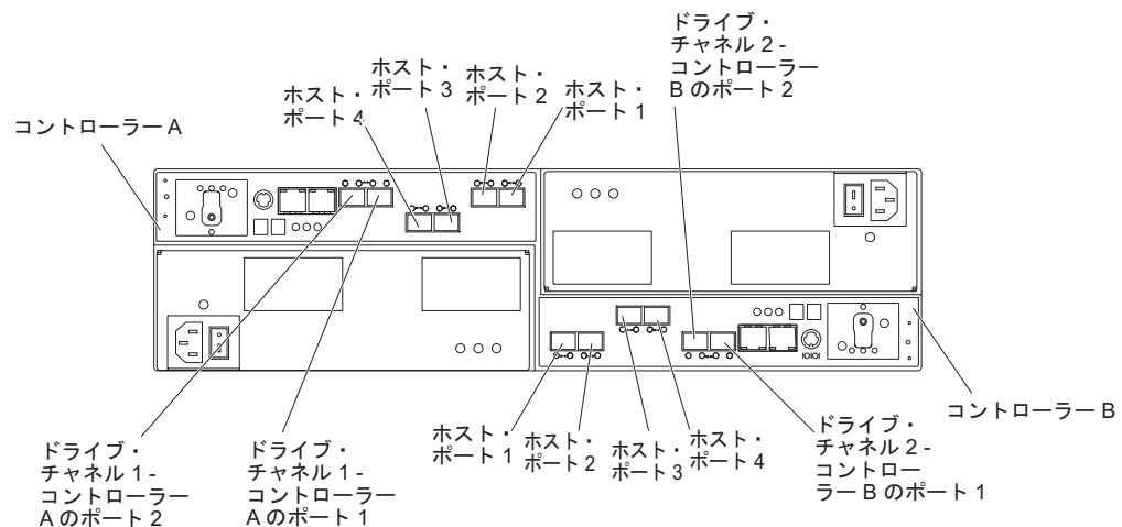
図 36. DS5020 ストレージ・サブシステムのポートとコントローラー
