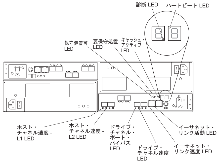
図 70. 2 つの標準および 2 つのオプションのファイバー・チャンネル・ホスト拡張チャンネルを搭載したコントローラーの LED、制御、およびコネクタ
