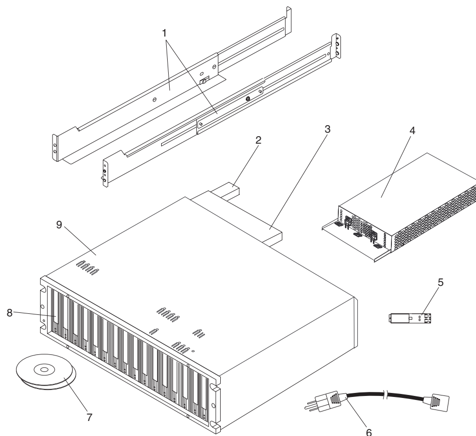
図 88. DS5020 ストレージ・サブシステム部品リスト
