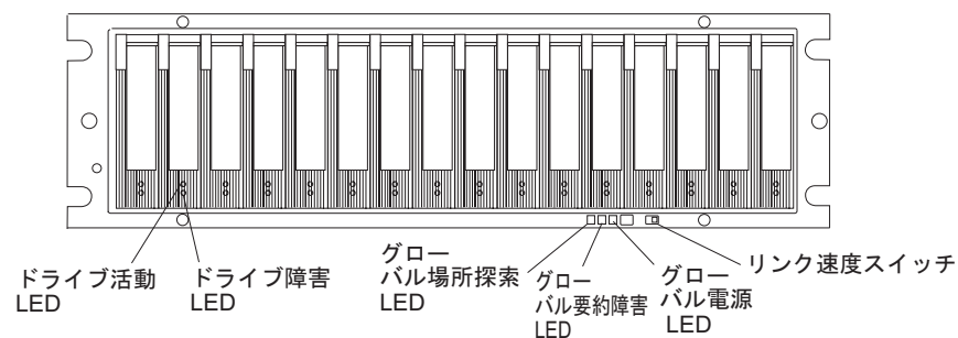
図 67. 前面 LED およびコントロール
