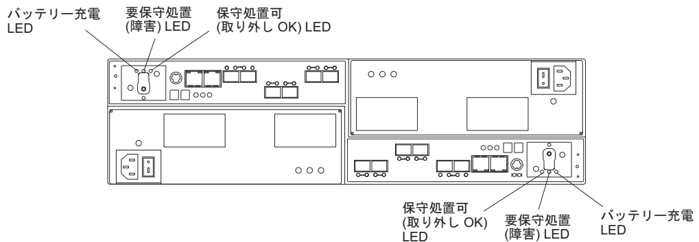
図 74. バッテリー・ユニット LED
