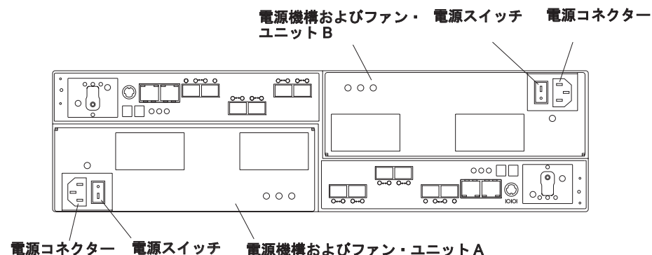
図 5. DS5020 の電源機構およびファン・ユニットのコンポーネント
