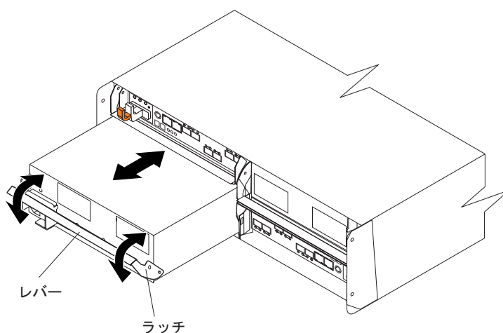
図 17. 電源機構およびファン・ユニットの取り外し
