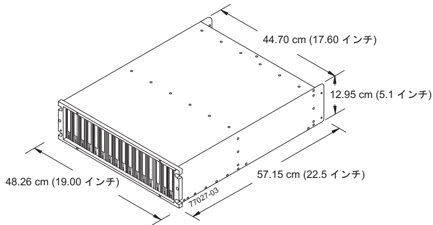
図 9. DS5020 寸法
