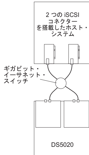
図 61. 単一ホスト、複数ポート構成の例
