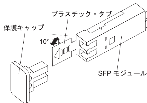
図 28. SFP モジュール・ラッチのアンロック - プラスチック・タブの場合
