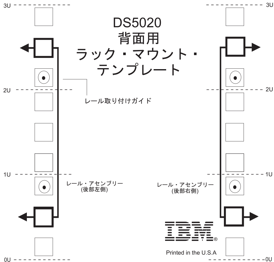
図 90. 背面用ラック・マウント・テンプレート
