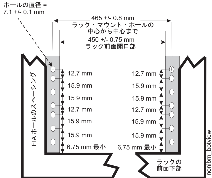
図 93. ラックの仕様寸法 (下部正面図)
