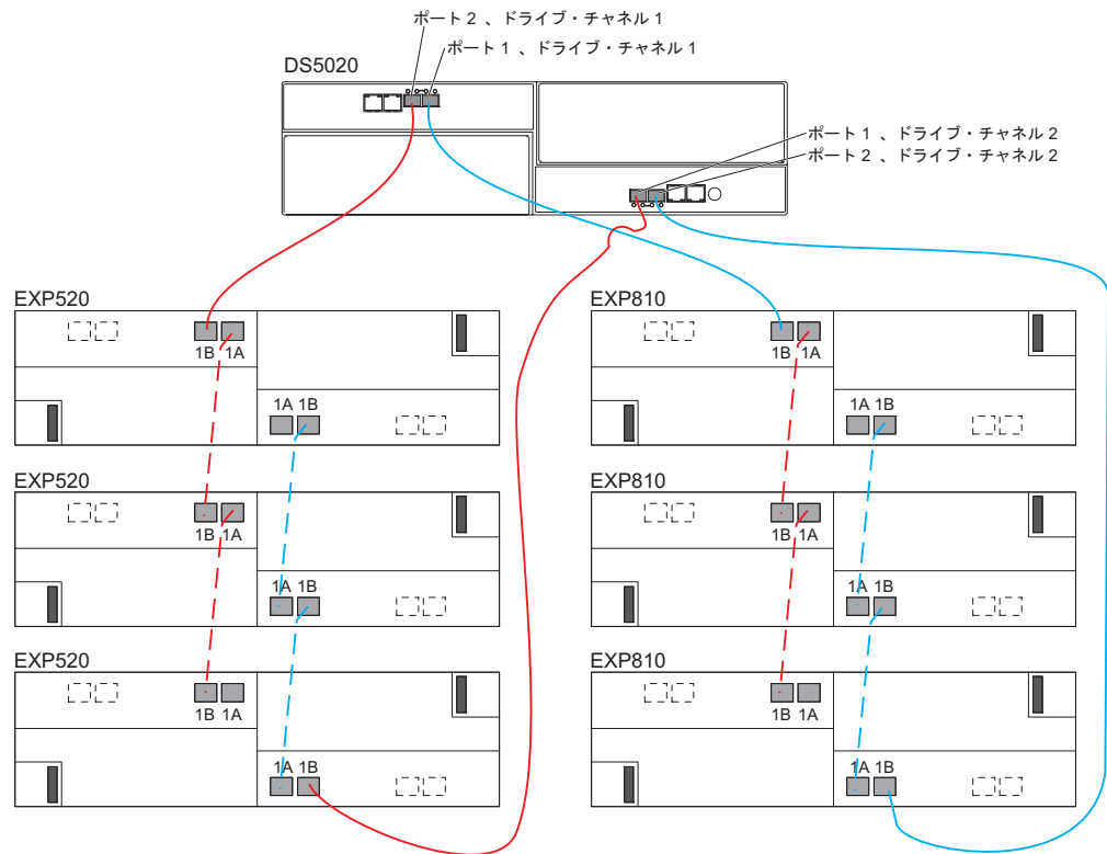
図 44. 混合環境での 1 つの DS5020 と複数のストレージ拡張エンクロージャのケーブル接続
