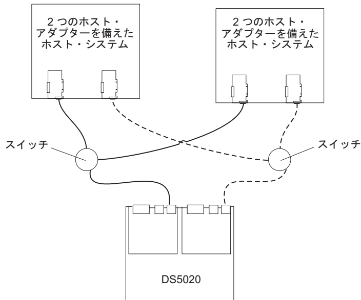
図 58. 二重 SAN ファブリック構成の例
