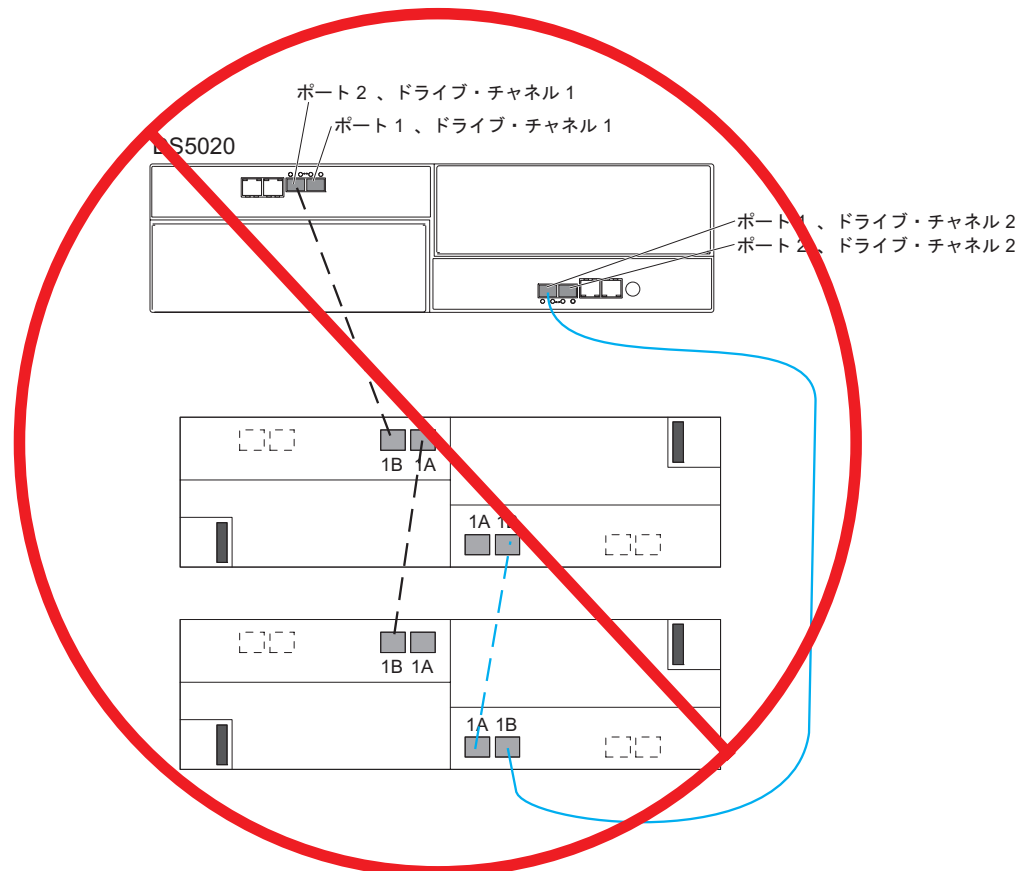
図 39. 1 つの DS5020 と 2 つのストレージ拡張エンクロージャーの誤ったケーブル接続
