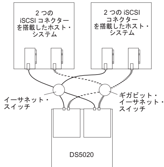
図 62. 複数ホスト、複数ポート構成の例
