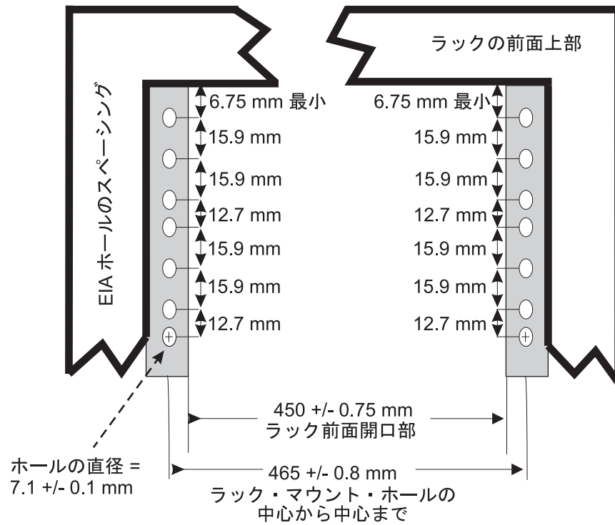
図 92. ラックの仕様寸法 (正面図)
