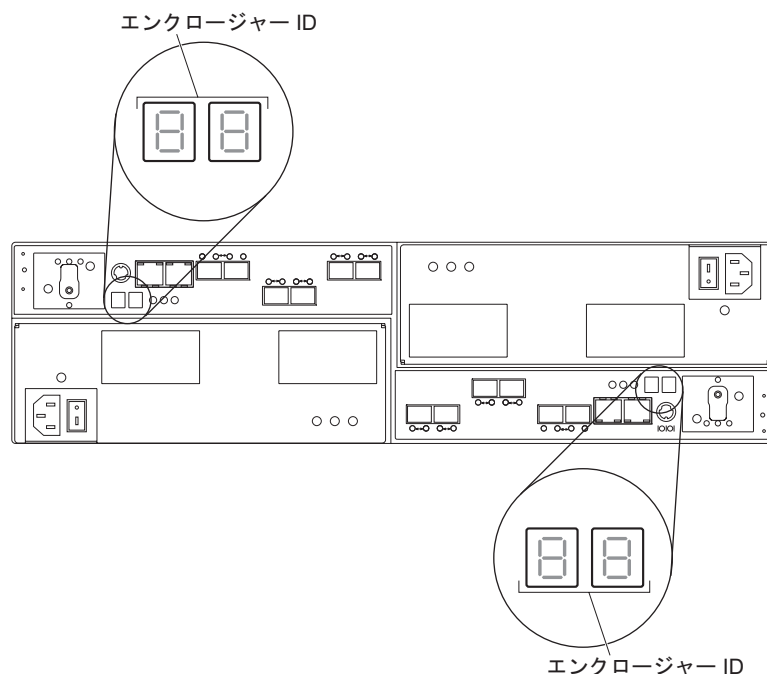
図 24. ストレージ・サブシステム 7 セグメント・エンクロージャー ID
