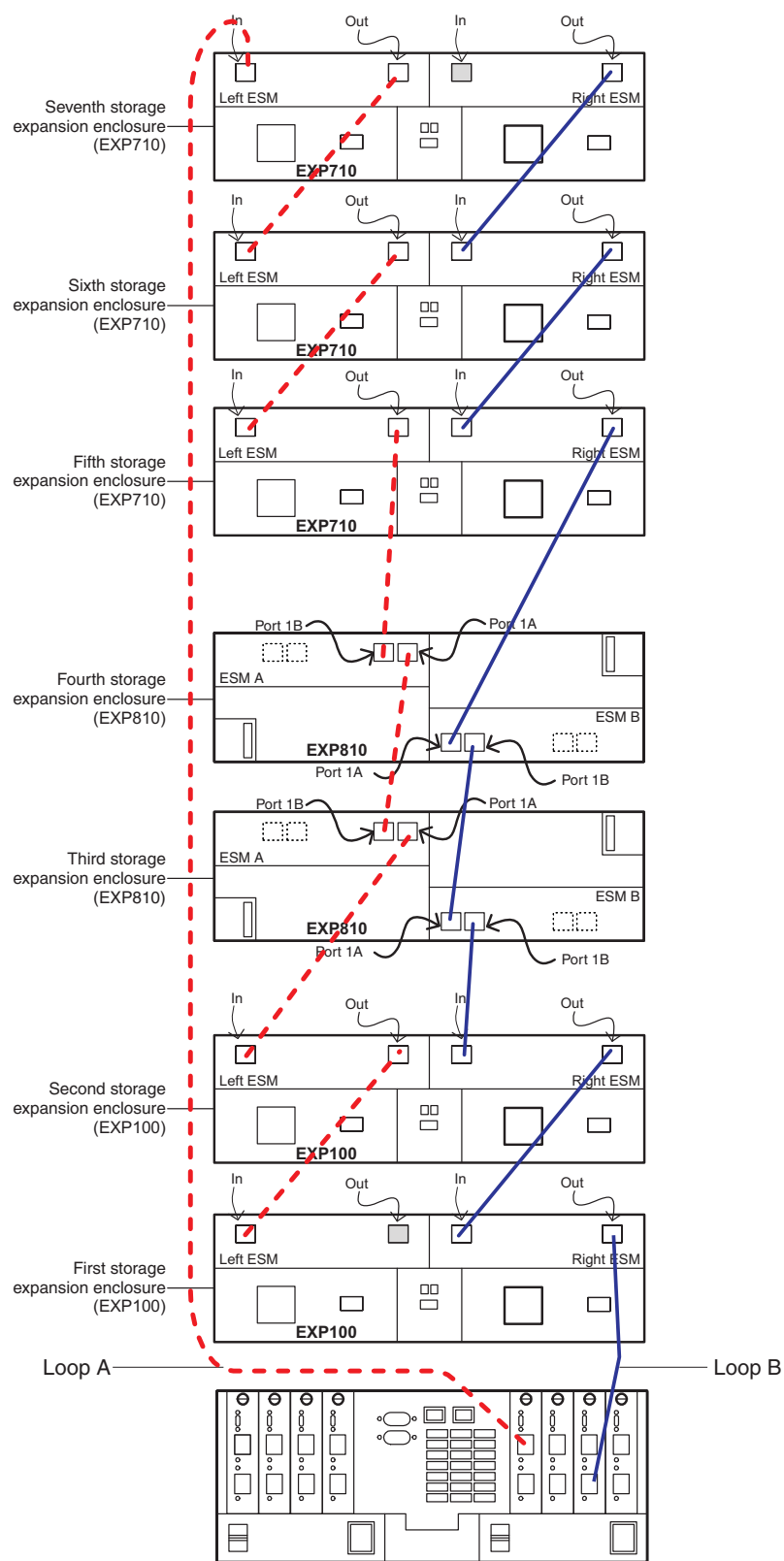
图 13. 混用 EXP100、EXP710 和 EXP810 存储机柜的受支持连线方案（示例 2）
