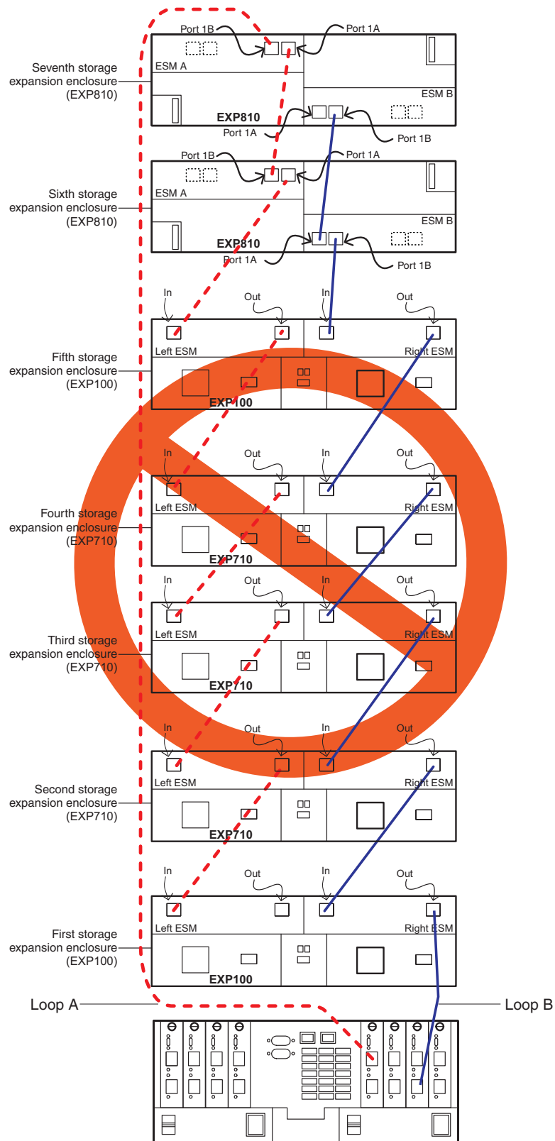
图 14. 混用 EXP100、EXP710 和 EXP810 存储机柜的不受支持连线方案 (示例 1)
