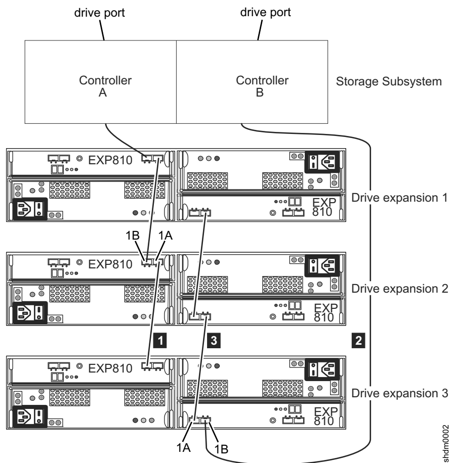
图 29. 连线要添加的 EXP5000、EXP520、EXP395、EXP810 或 EXP420 存储机柜
