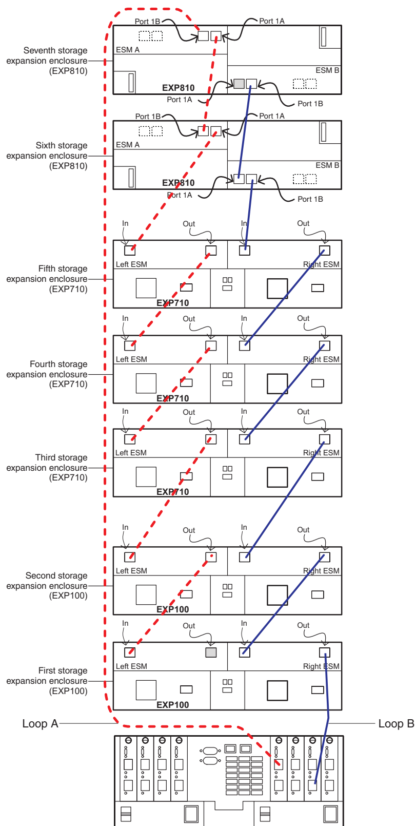
图 12. 混用 EXP100、EXP710 和 EXP810 存储机柜的受支持连线方案（示例 1）
