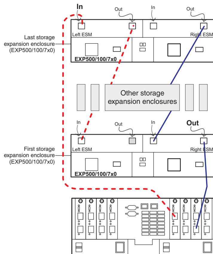
图 18. 到 EXP500/EXP100/EXP700/EXP710 存储机柜端口的受支持连线方案
