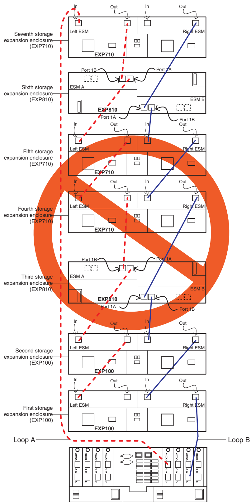
图 15. 混用 EXP100、EXP710 和 EXP810 存储机柜的不受支持连线方案（示例 2）
