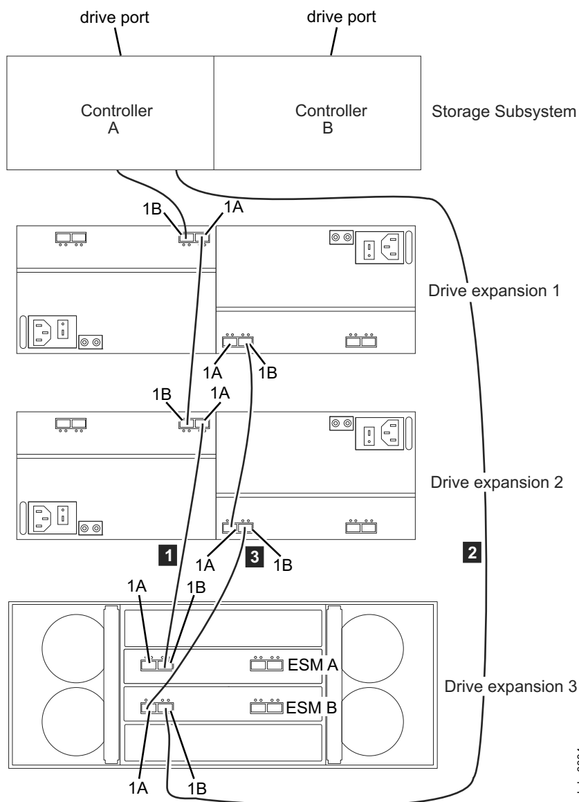
图 31. 连线要添加的 EXP5060 存储机柜
