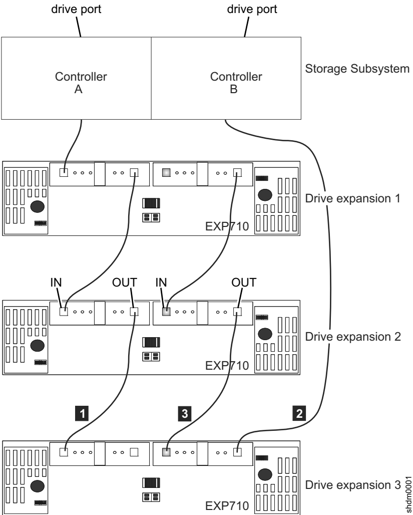
图 28. 连线要添加的 EXP700/EXP710/EXP100/EXP500 存储机柜
