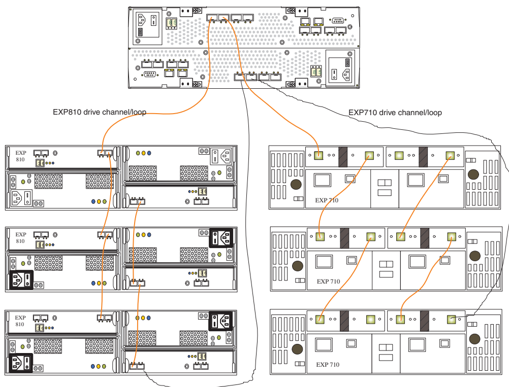
图 8. 连接到 EXP710 和 EXP810 存储机柜的混用 DS4000 存储子系统环路最佳配置
