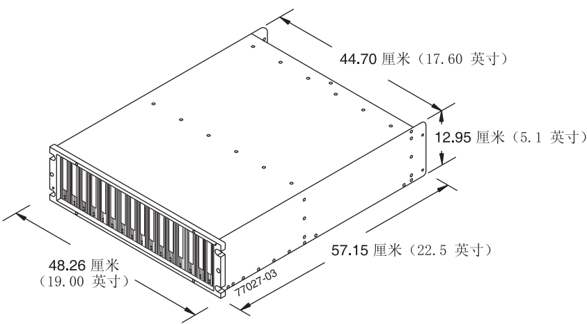
图 6. EXP520 尺寸
