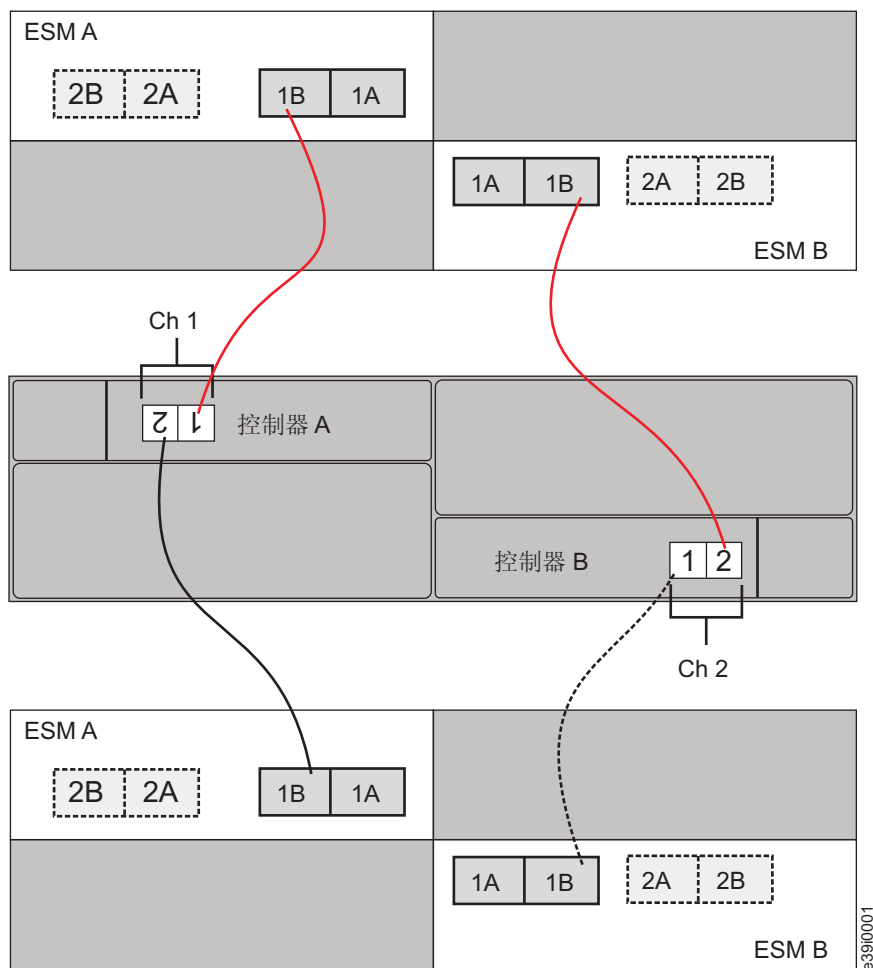
图 25. 以循环法方式对 EXP520 布线
