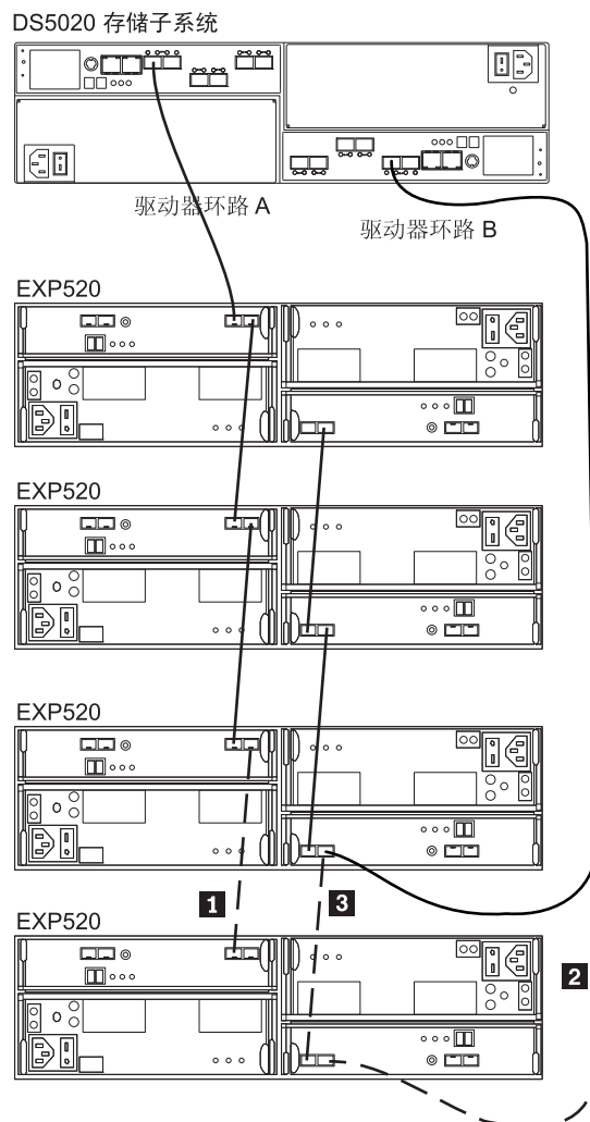
图 33. 将 EXP520 用电缆连接到现有的和已配置的驱动器环路
