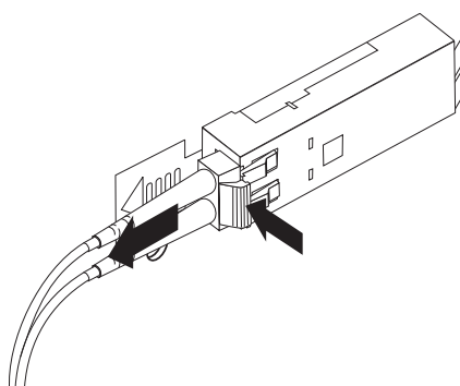
图 24. 拔下 LC-LC 光纤通道电缆
