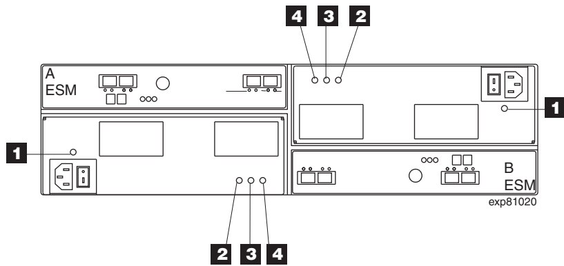
图 29. 电源和风扇单元指示灯
