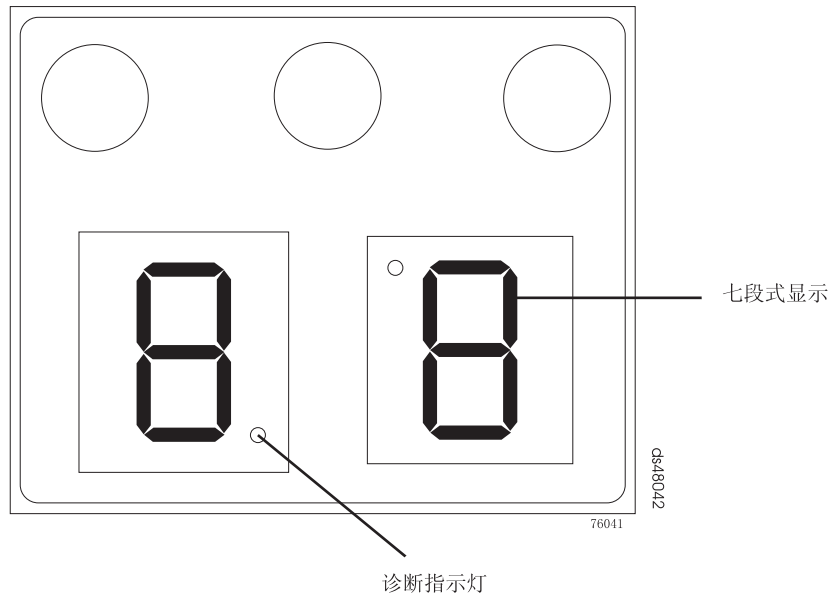
图 32. 数字显示器指示灯
