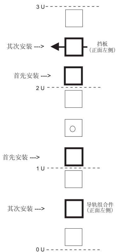
图 9. 前部机架安装模板
