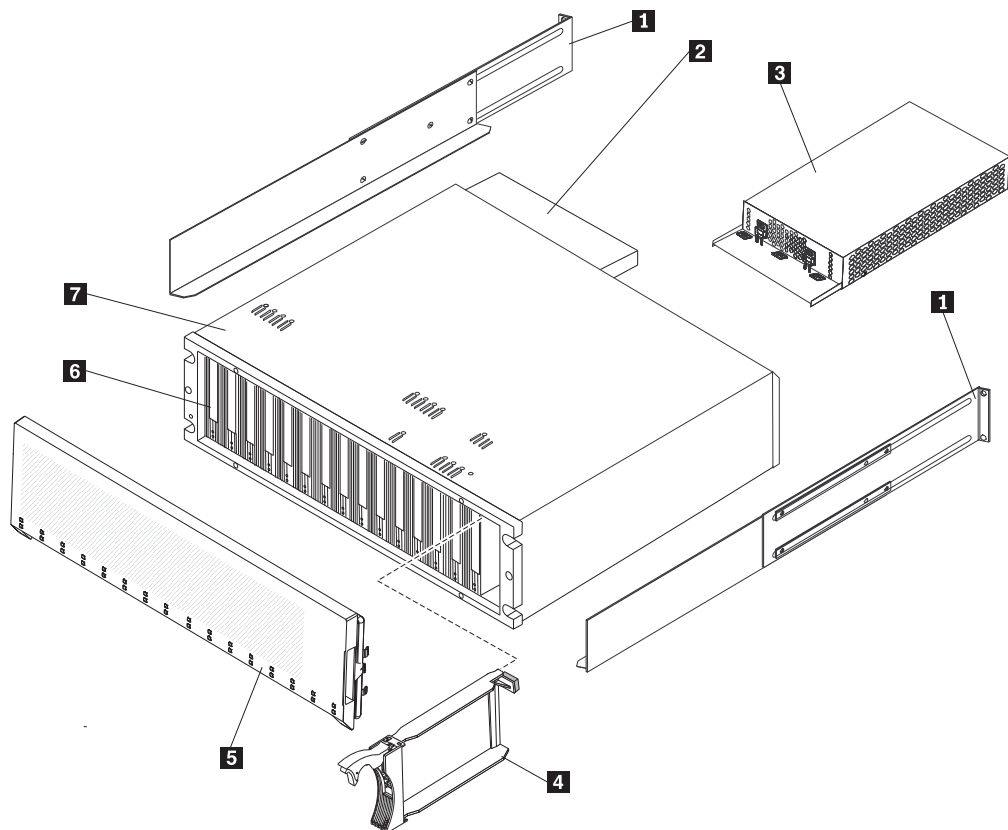
图 41. EXP520 存储扩展机柜部件列表
