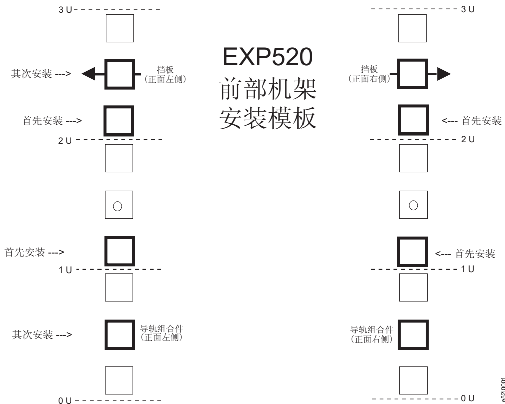
图 43. 前部机架安装模板
