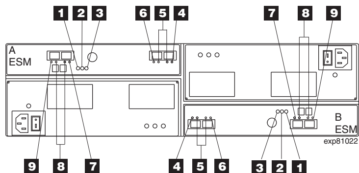
图 31. 后部指示灯、控制器和接口
