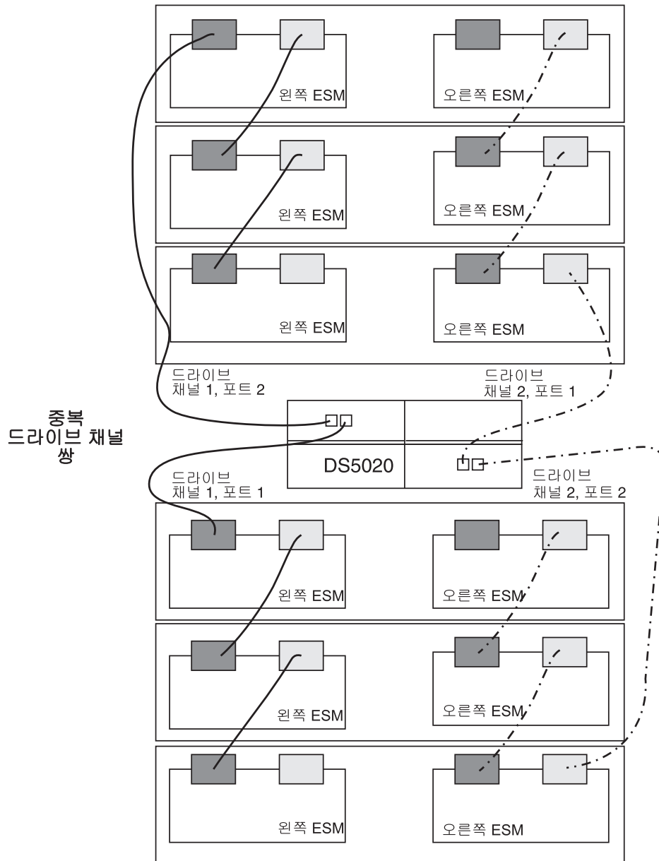
그림 35. 중복 드라이브 채널 쌍 예제
