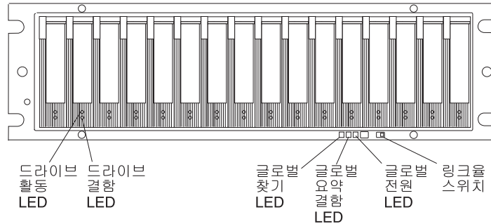
그림 67. 앞면 LED 및 제어
