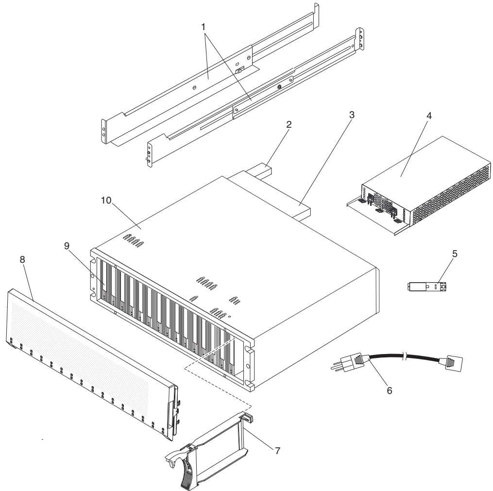
그림 90. DS5020 스토리지 서브시스템 부품 목록
