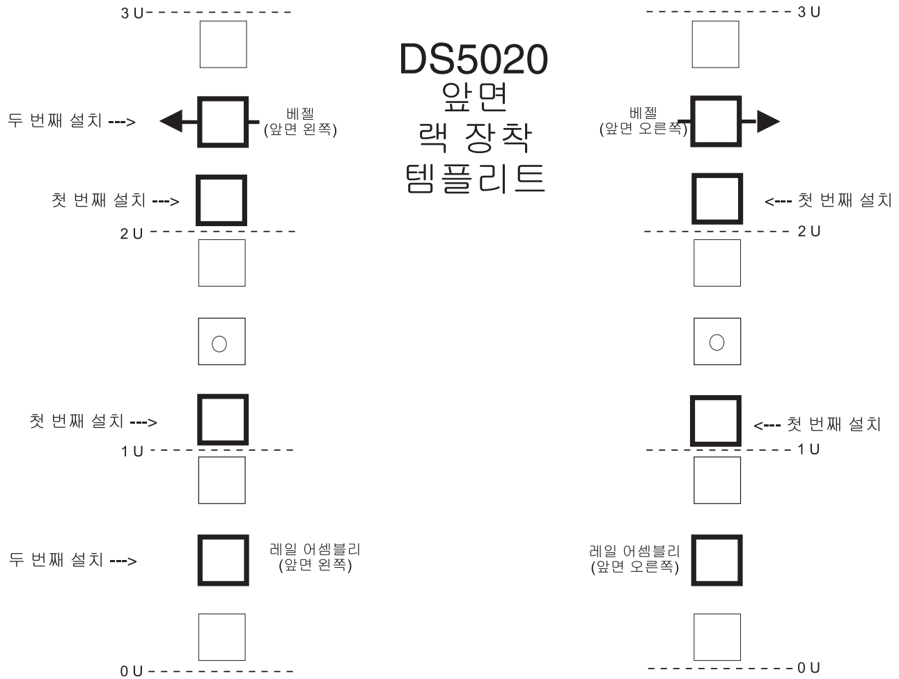
그림 92. 앞면 랙 마운팅 템플리트
