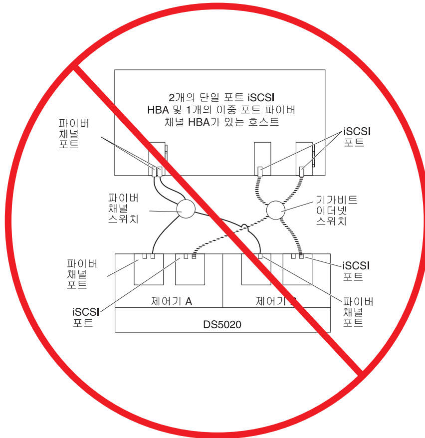
그림 64. 올바르게 않은 구성의 예제: 단일 호스트, iSCSI 및 파이버 채널
