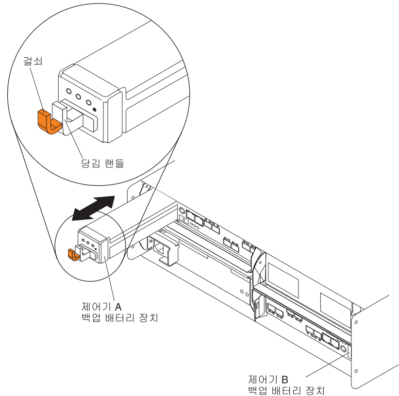
그림 86. 제어기 새시에서 배터리 장치 제거 및 교체
