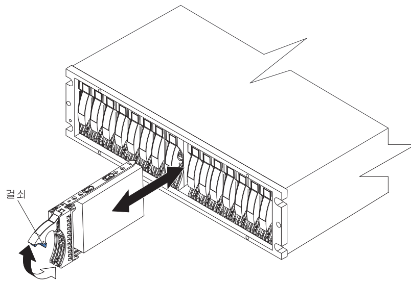
그림 23. E-DDM 교체
