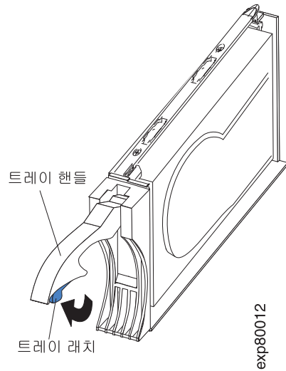
그림 82. E-DDM CRU 핸들
