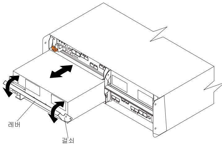
그림 85. 전원 공급 장치 및 팬 장치 교체
