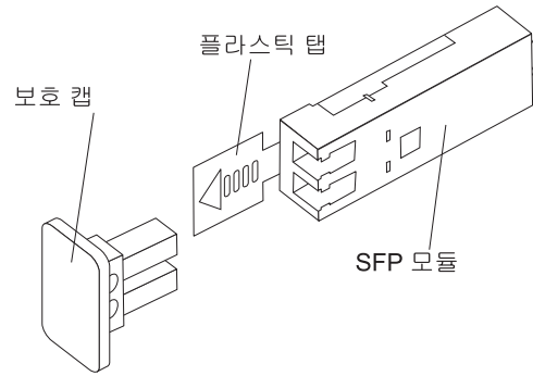
그림 26. SFP 모듈 및 보호 캡
