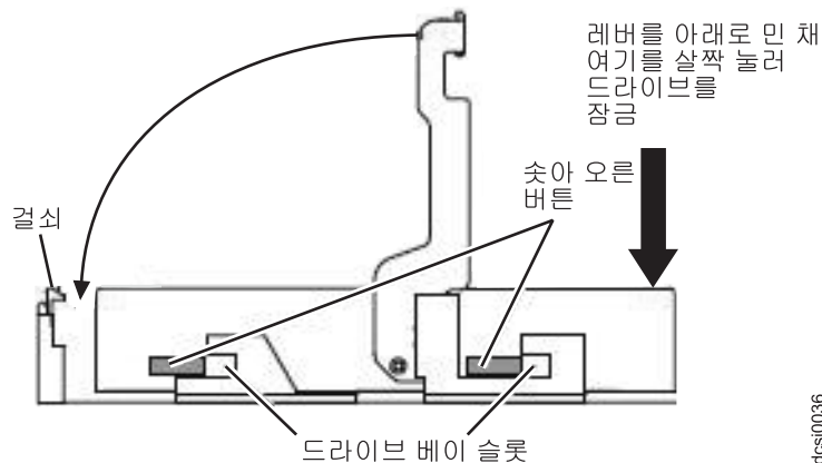
그림 80. 커넥터에 하드 디스크 드라이브 삽입
