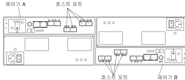
그림 54. DS5020의 RAID 제어기에서 호스트 케이블의 위치
