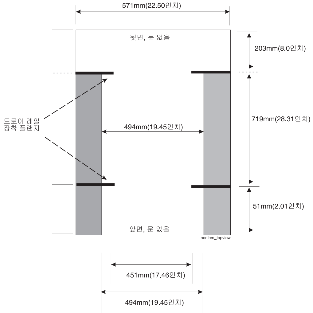
그림 94. 비IBM 랙 스펙 차원의 맨 위 보기
