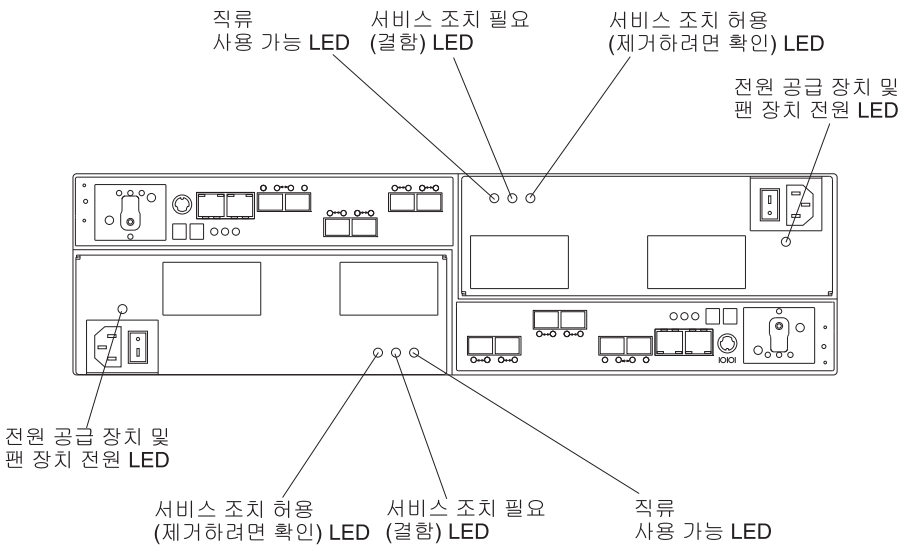
그림 66. 전원 공급 장치 및 팬 장치 LED
