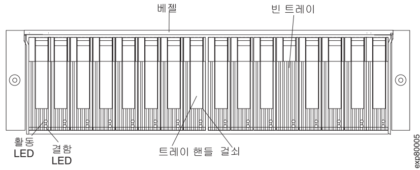
그림 81. 핫 스왑 E-DDM LED
