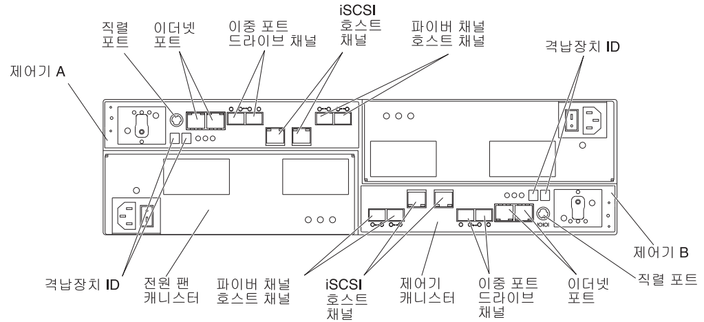
그림 4. 뒷면 보기 - 2개의 표준 파이버 채널 호스트 확장 채널 및 2개의 선택적 iSCSI 호스트 확장 채널이 있는 제어기
