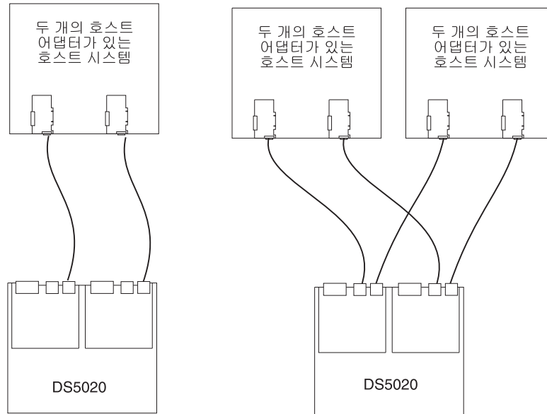
그림 56. 중복 호스트 직접 연결 파이버 채널 SAN 구성의 예제
