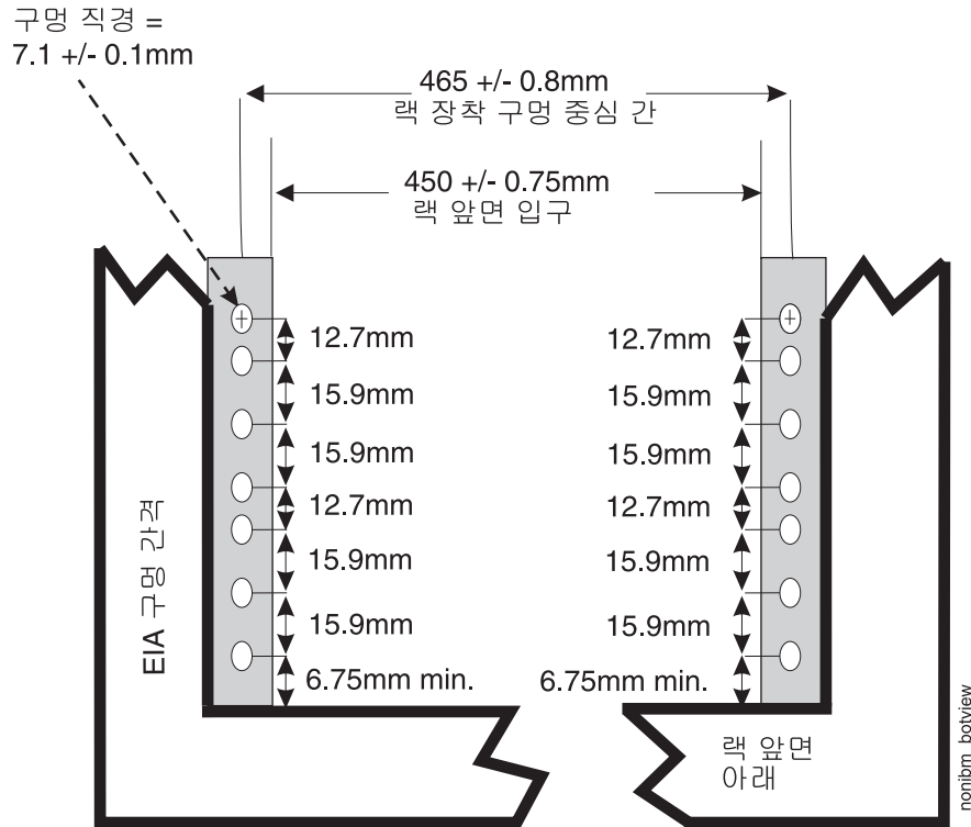
그림 96. 랙 스펙 차원, 맨 아래 앞면 보기
