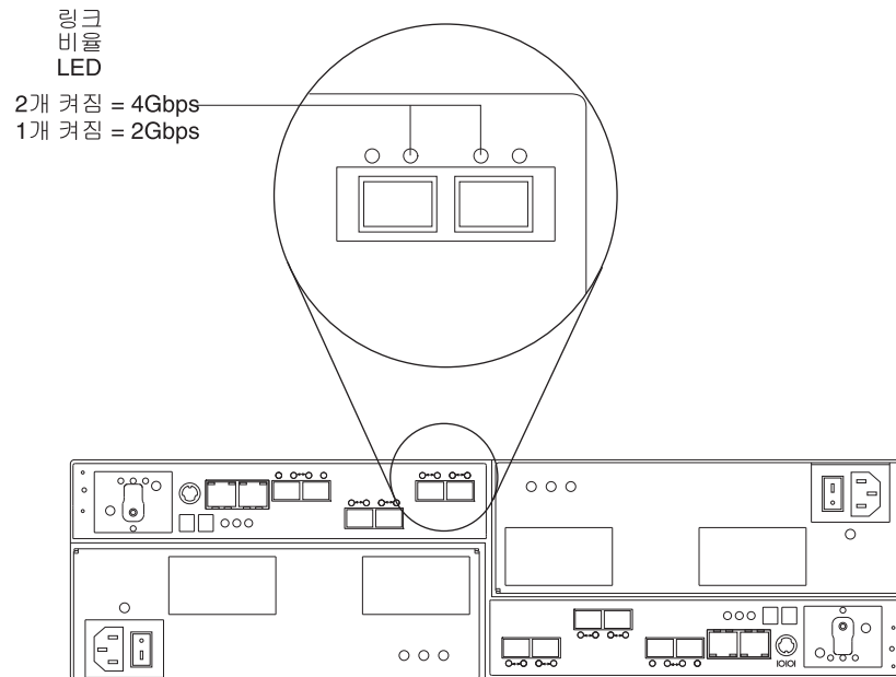
그림 83. 링크율 LED
