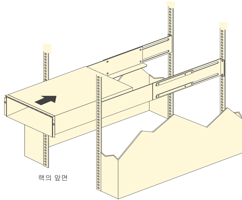
그림 19. DS5020 설치
