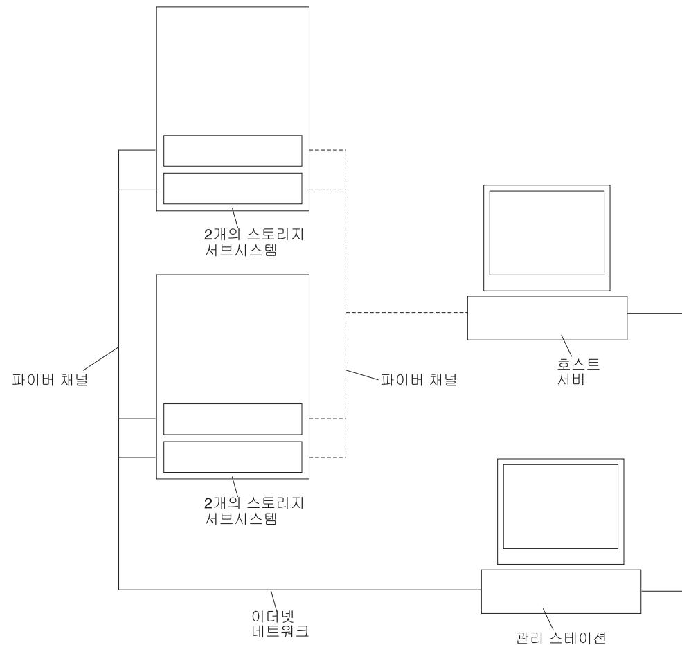
그림 53. 직접(아웃오브밴드) 관리 스토리지 서브시스템
