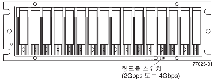
그림 84. 링크율 스위치
