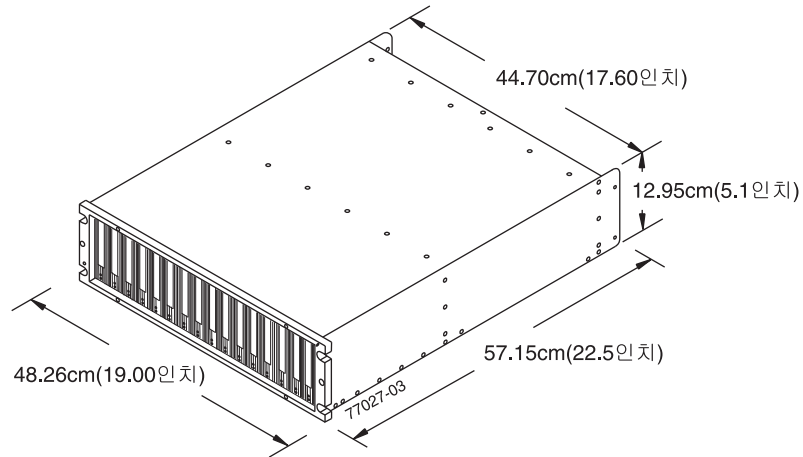
그림 9. DS5020 차원
