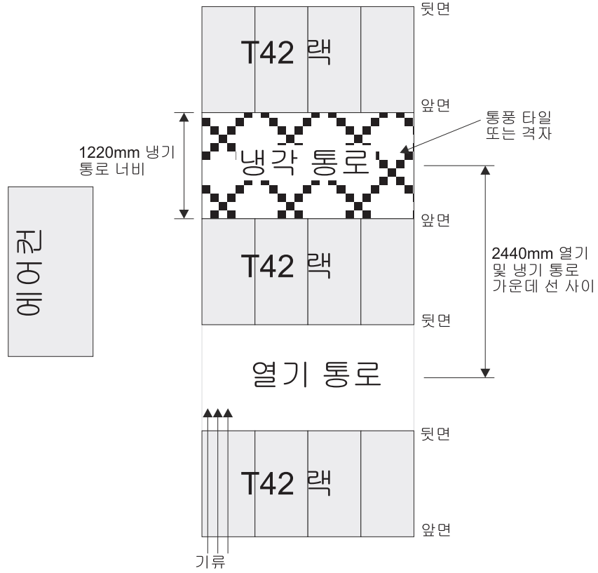
그림 11. 냉각 통로/열 통로 랙 구성 예제
