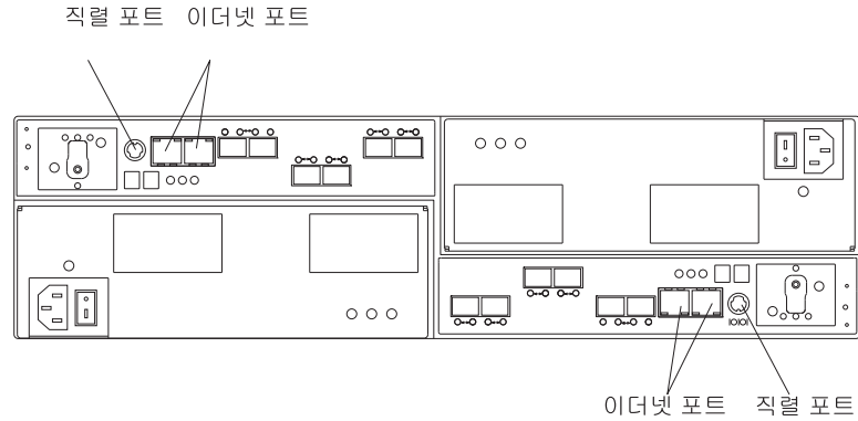
그림 51. DS5020의 이더넷 및 직렬 포트 위치
