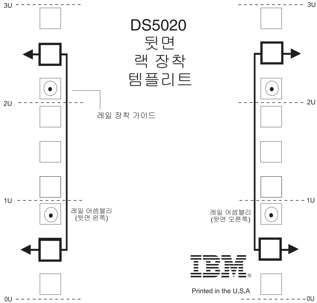
그림 93. 뒷면 랙 마운팅 템플리트
