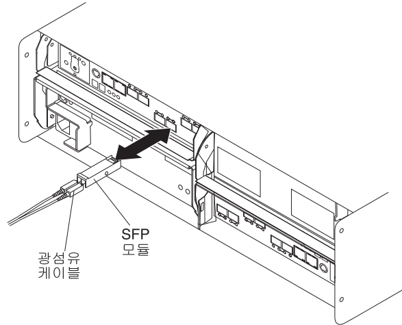
그림 87. SFP 모듈 교체
