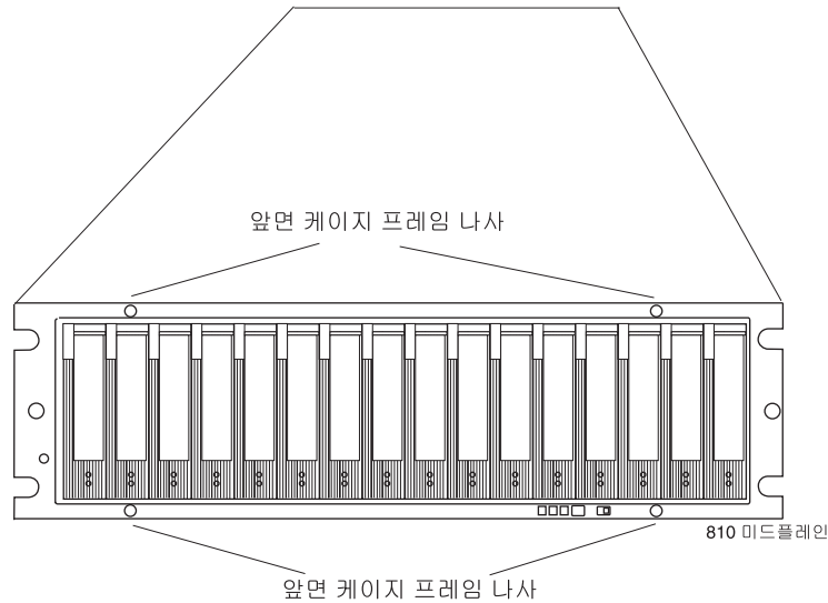
그림 88. 앞면 케이지 프레임 나사 위치
