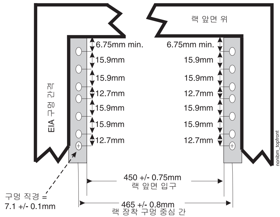
그림 95. 랙 스펙 차원, 맨 위 앞면 보기
