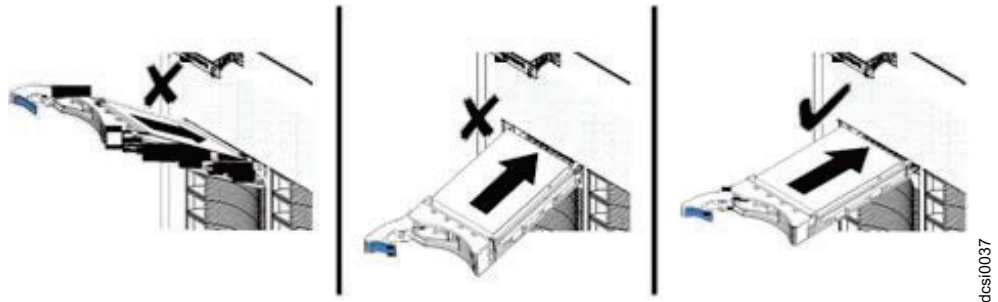
그림 79. 드라이브 슬롯에 하드 디스크 드라이브 삽입
