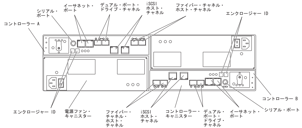
図 4. 2 つの標準ファイバー・チャンネル・ホスト拡張チャンネルおよび 2 つのオプション iSCSI ホスト拡張チャンネルを搭載したコントローラーの背面図
