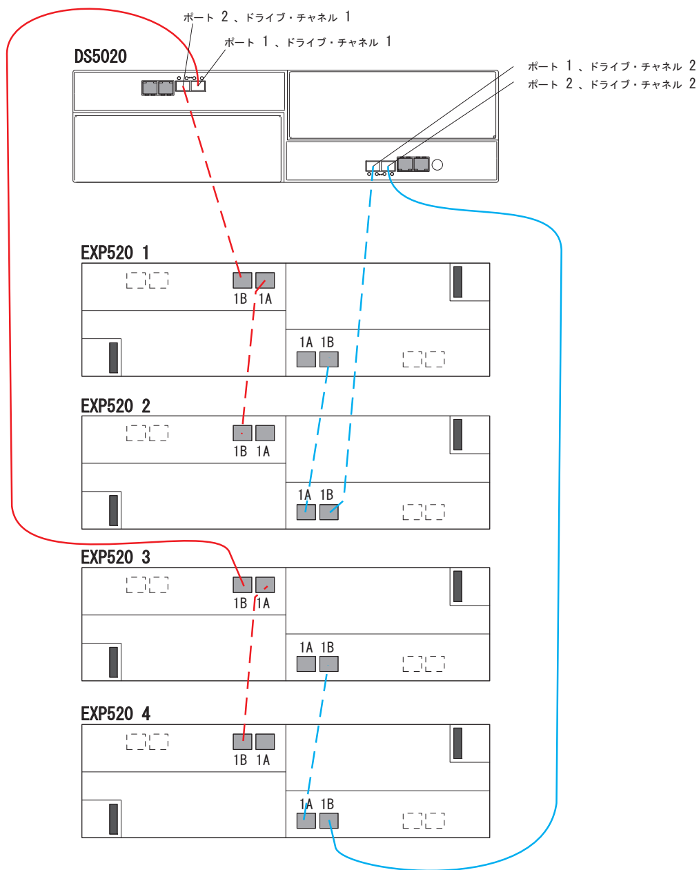
図 49. 1 組の DS5020 ドライブ・ポートの後ろでの 1 つの DS5020 と 4 つの EXP520 ストレージ拡張エンクロージャー
