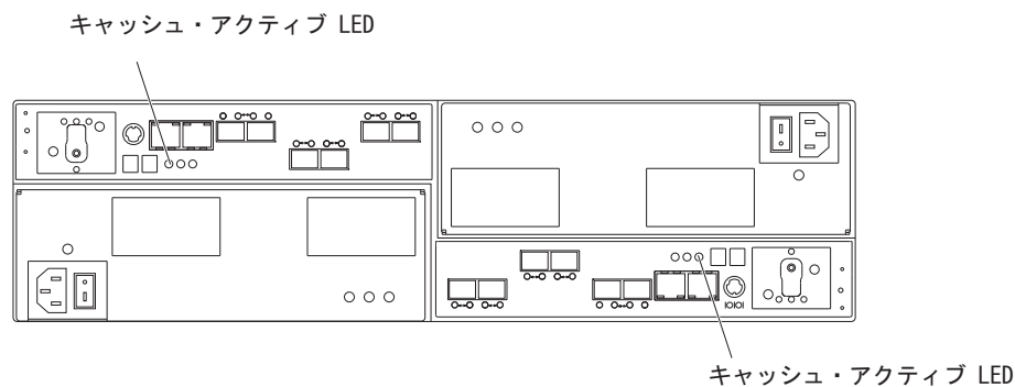
図 73. キャッシュ・アクティブ LED
