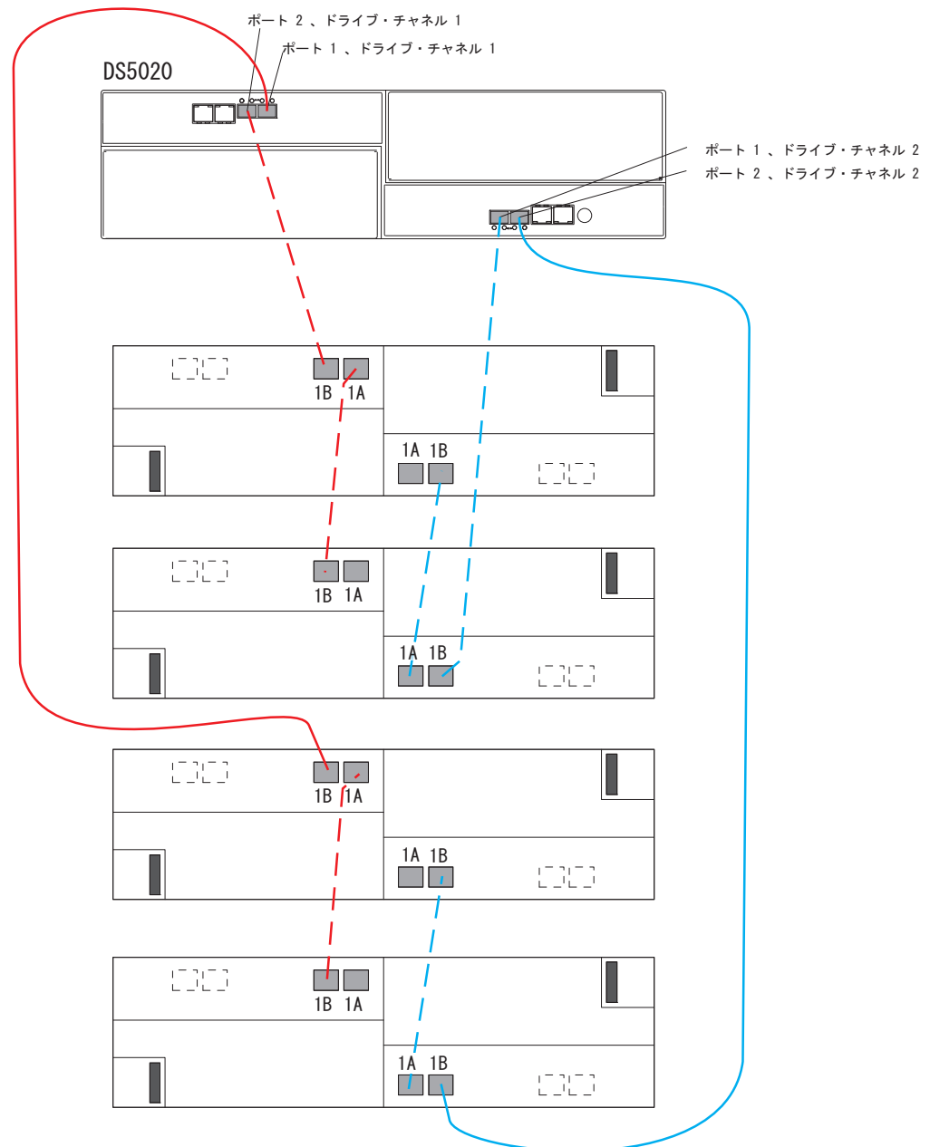
図 41. 1 つの DS5020 と 4 つのストレージ拡張エンクロージャーのケーブル接続
