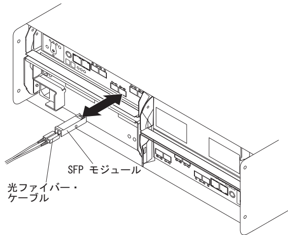
図 87. SFP モジュールの交換
