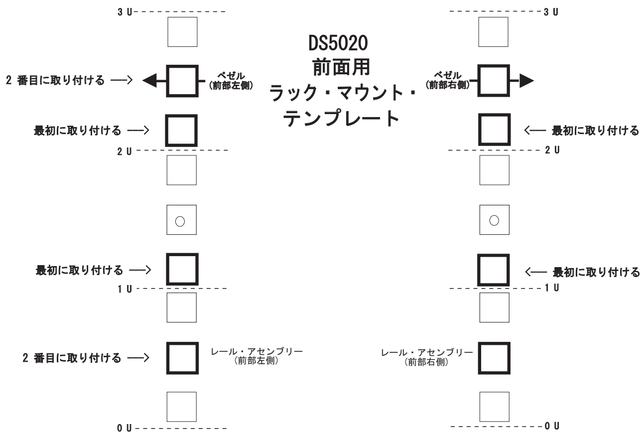
図 92. 前面用ラック・マウント・テンプレート
