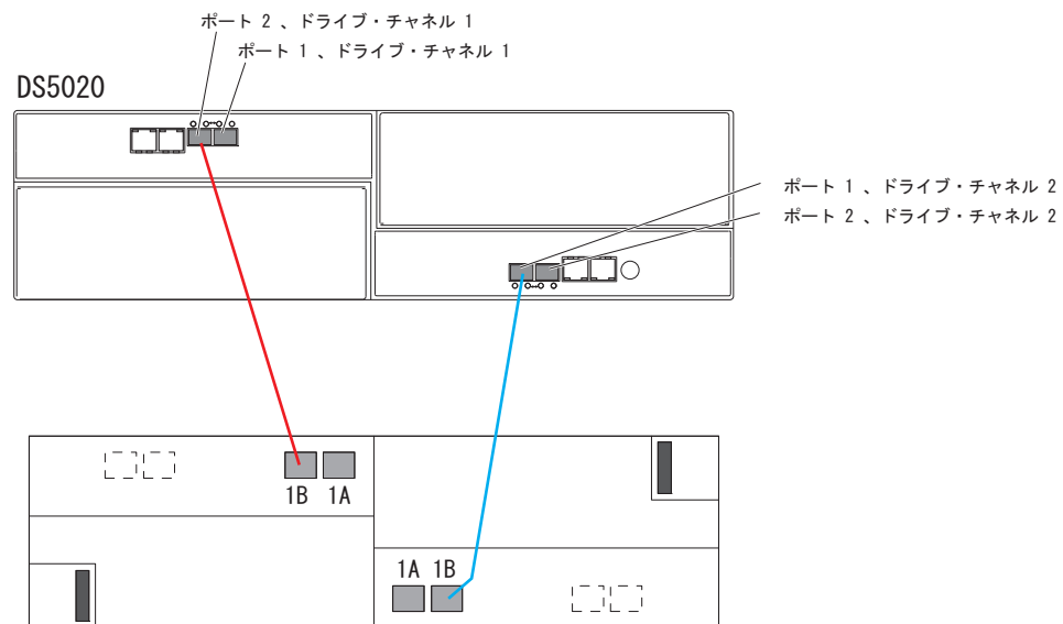
図 37. 1 つの DS5020 と 1 つのストレージ拡張エンクロージャーのケーブル接続
