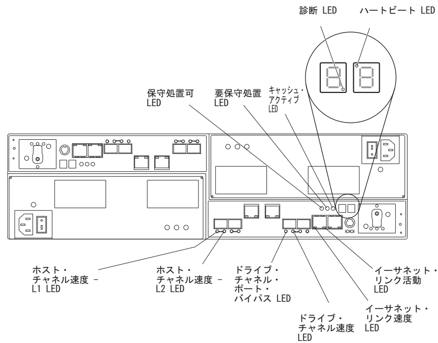
図 71. 2 つの標準ファイバー・チャンネル・ホスト拡張チャンネルおよび 2 つのオプション iSCSI ホスト通信路チャンネルを搭載したコントローラーの LED、制御、およびコネクタ
