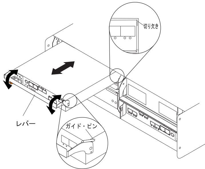
図 21. コントローラーの取り外しと交換
