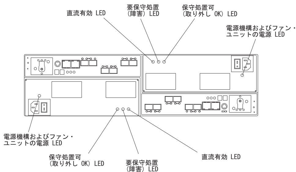
図 66. 電源機構およびファン・ユニット LED
