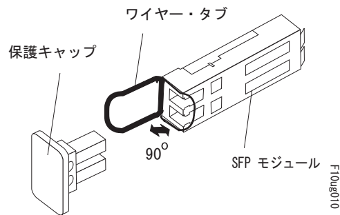
図 76. SFP モジュール・ラッチのアンロック - ワイヤー・タブの場合
