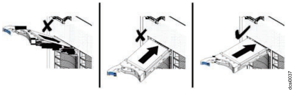
図79. ハード・ディスクのドライブ・スロットへの挿入
