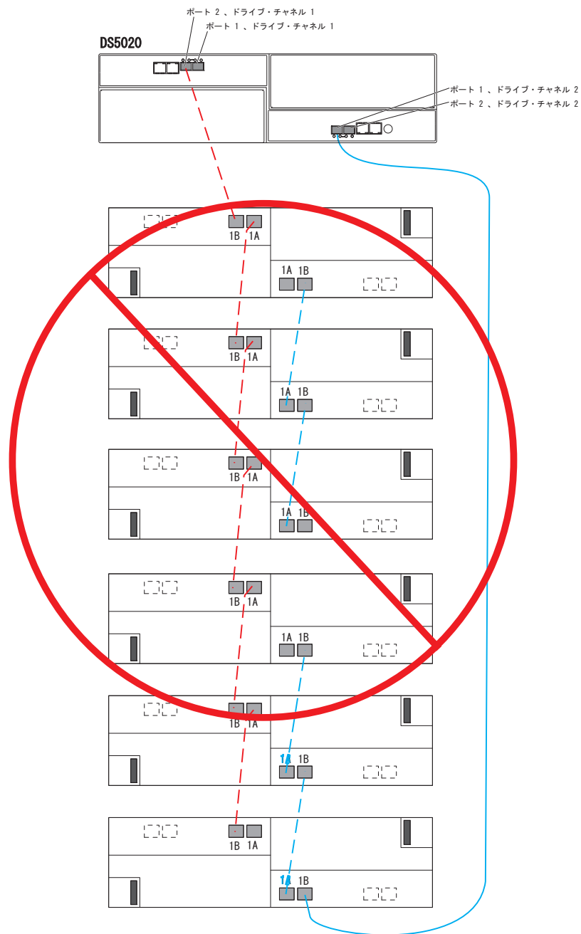
図 43. 1 つの DS5020 と最大 6 つのストレージ拡張エンクロージャーのケーブル接続
