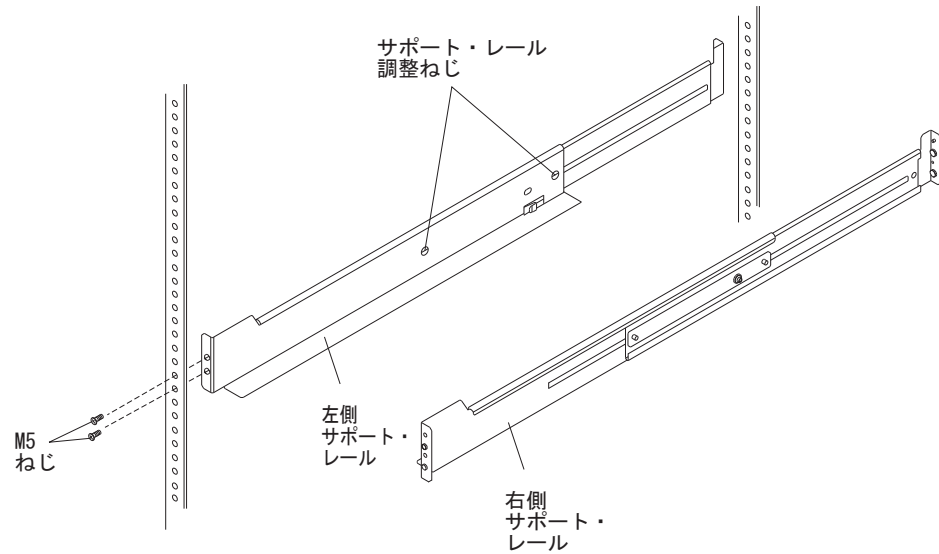
図 15. サポート・レールの取り付け
