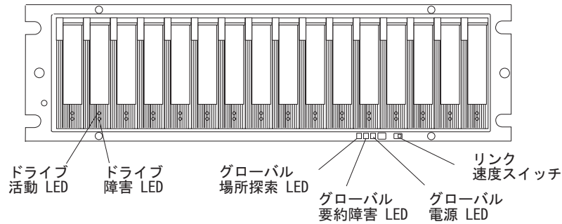
図 67. 前面 LED およびコントロール
