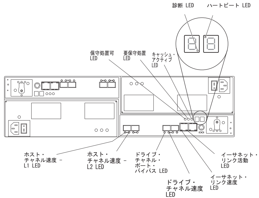
図 69. 2 つの標準ファイバー・チャンネル・ホスト拡張チャンネルを搭載したコントローラーの LED、制御、およびコネクタ
