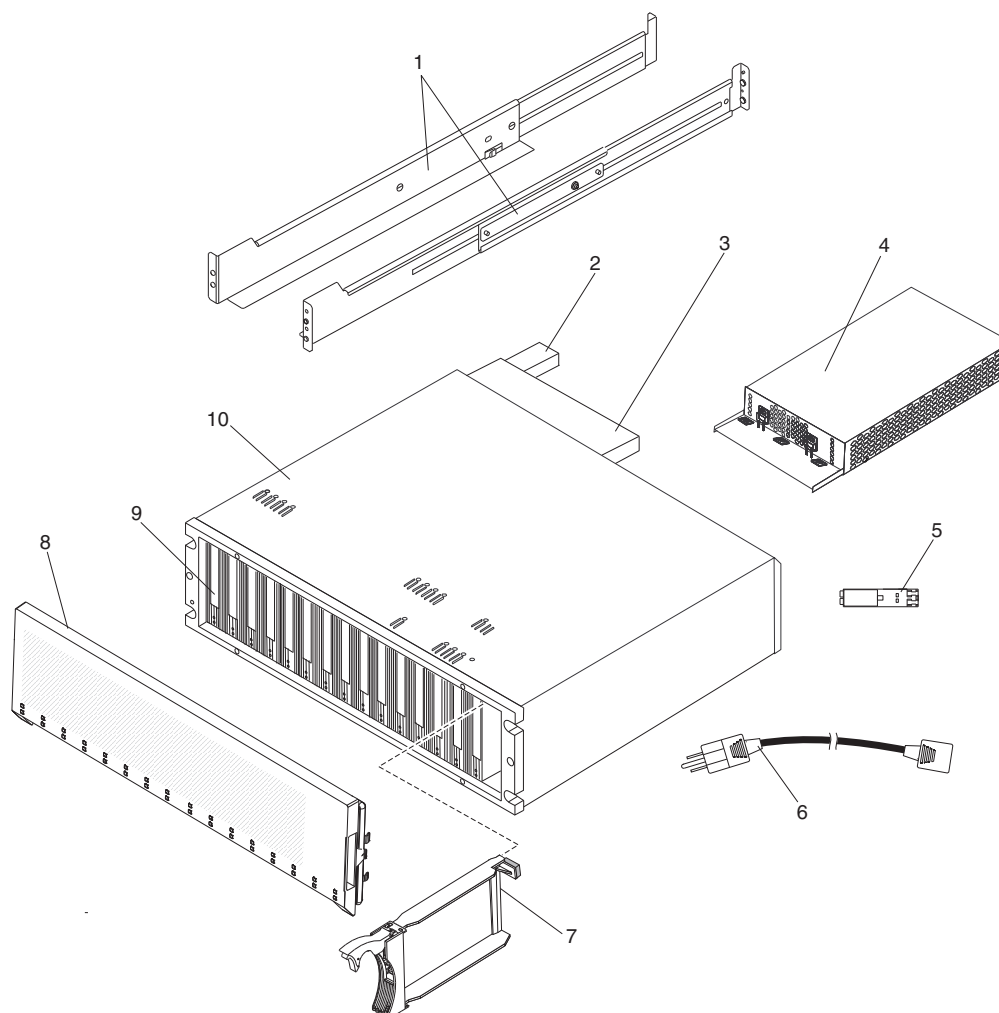
図 90. DS5020 ストレージ・サブシステム部品リスト
