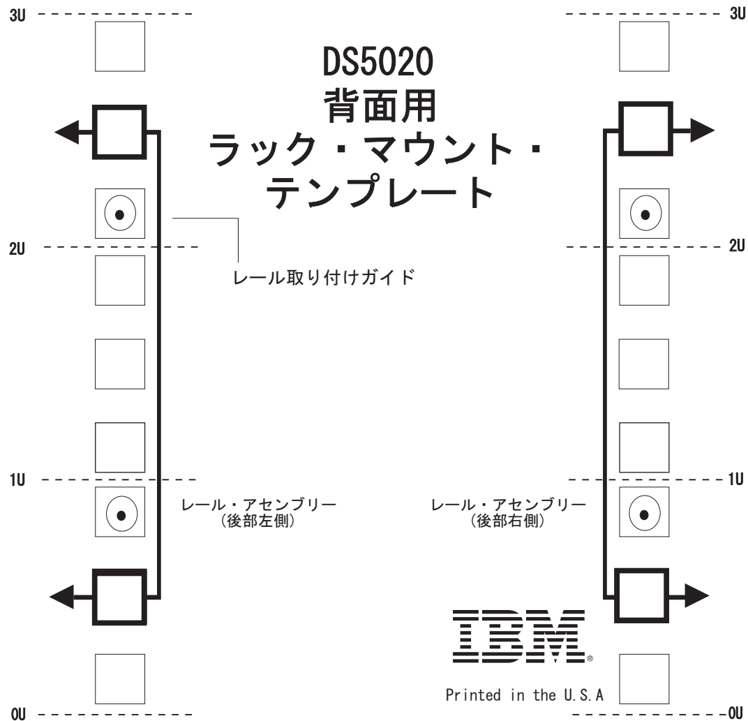
図 93. 背面用ラック・マウント・テンプレート
