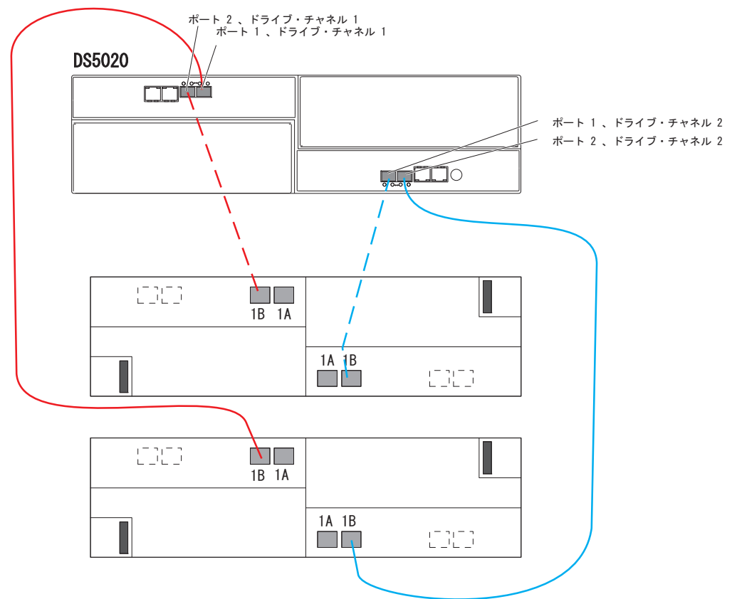
図 38. 1 つの DS5020 と 2 つのストレージ拡張エンクロージャーのケーブル接続
