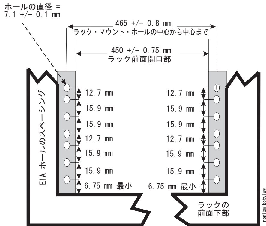
図 96. ラックの仕様寸法 (下部正面図)
