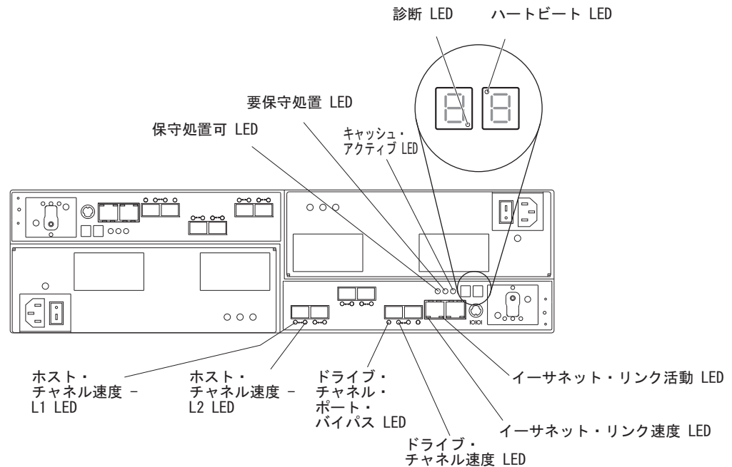
図 70. 2 つの標準および 2 つのオプションのファイバー・チャンネル・ホスト拡張チャンネルを搭載したコントローラーの LED、制御、およびコネクタ
