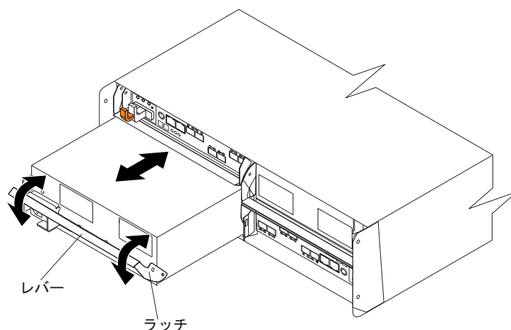
図 22. 電源機構およびファン・ユニットの交換
