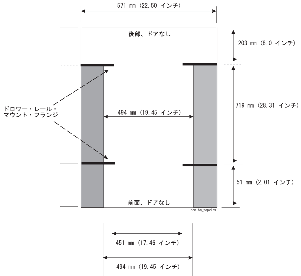
図 94. IBM 以外のラックの仕様寸法の平面図
