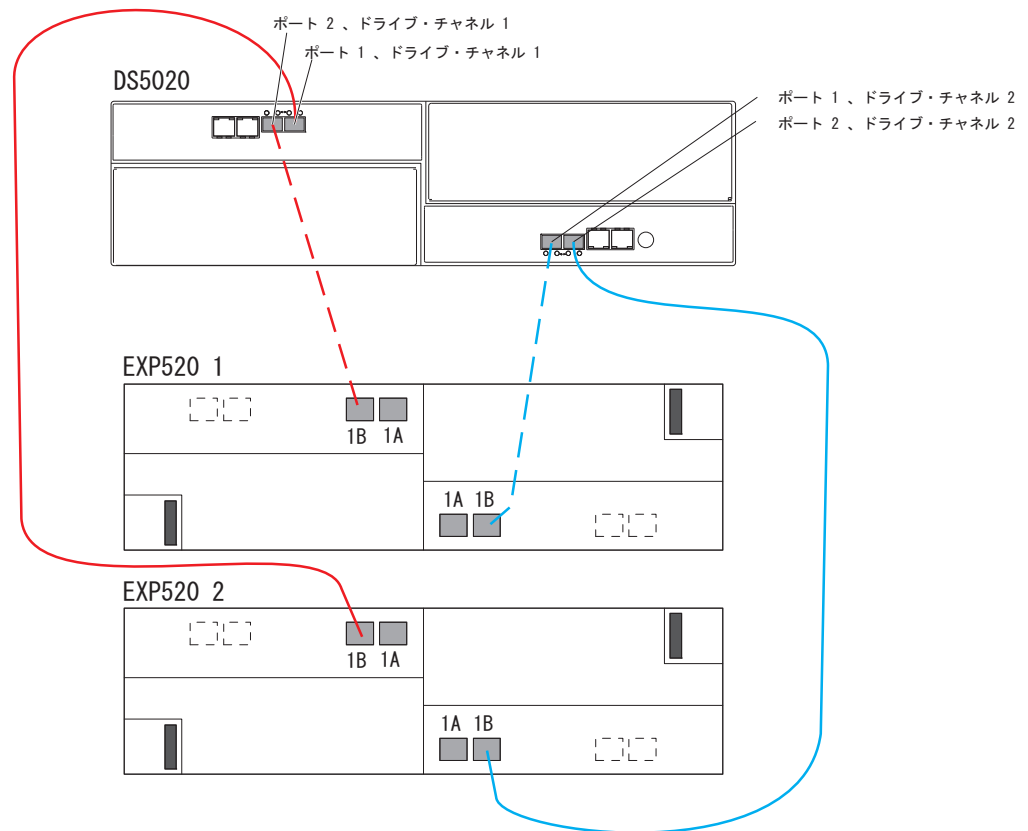
図 47. 1 組の DS5020 ドライブ・ポートの後ろでの 1 つの DS5020 と 2 つの EXP520 ストレージ拡張エンクロージャ
