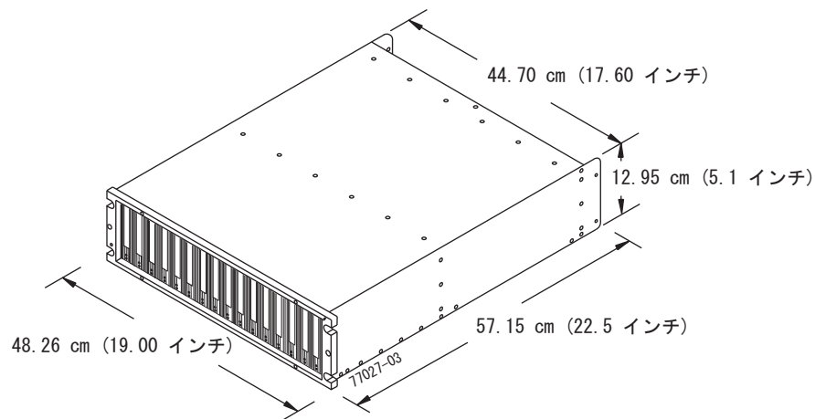
図 9. DS5020 寸法
