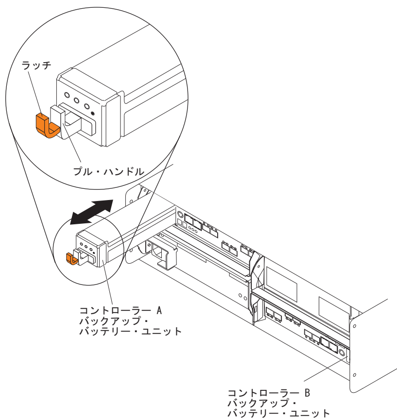
図 86. コントローラー・シャーシからのバッテリーの取り外しと再取り付け
