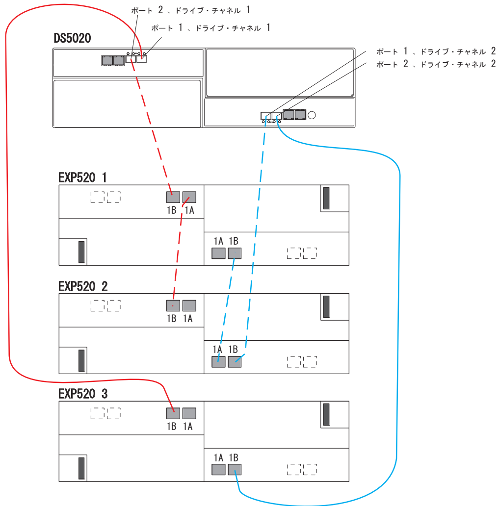
図 48. 1 組の DS5020 ドライブ・ポートの後ろでの 1 つの DS5020 と 3 つの EXP520 ストレージ拡張エンクロージャー
