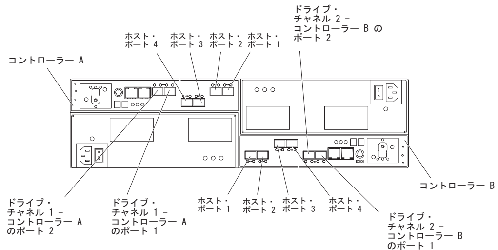
図 36. DS5020 ストレージ・サブシステムのポートとコントローラー
