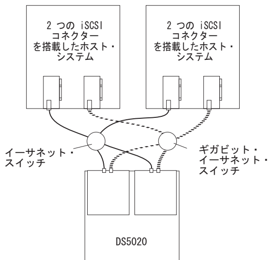
図 62. 複数ホスト、複数ポート構成の例
