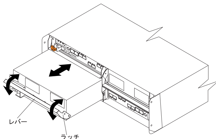
図 17. 電源機構およびファン・ユニットの取り外し
