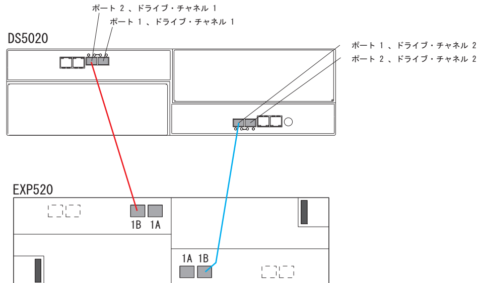
図 46. 1 つの DS5020 と 1 つの EXP520 ストレージ拡張エンクロージャのケーブル接続
