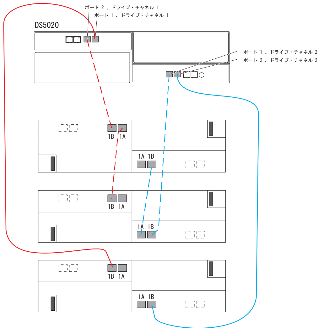
図 40. 1 つの DS5020 と 3 つのストレージ拡張エンクロージャのケーブル接続
