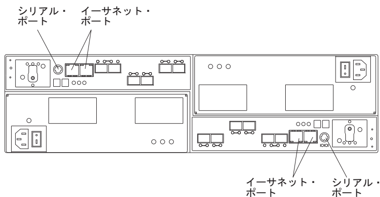
図 51. DS5020 のイーサネットおよびシリアル・ポートの位置
