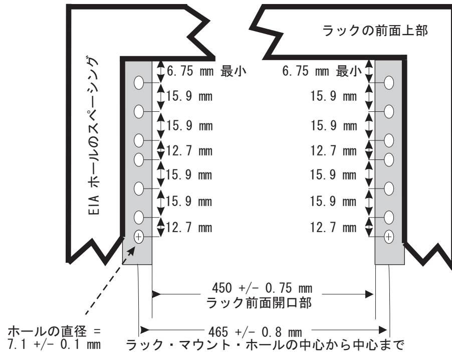
図 95. ラックの仕様寸法 (正面図)
