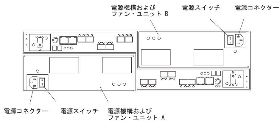
図 5. DS5020 の電源機構およびファン・ユニットのコンポーネント
