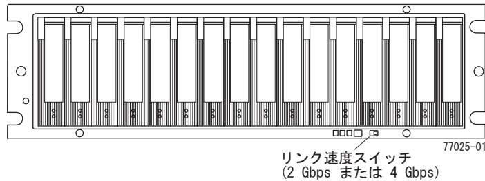
図 84. リンク速度スイッチ
