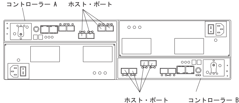
図 54. DS5020 の RAID コントローラー上のホスト・ケーブルの位置
