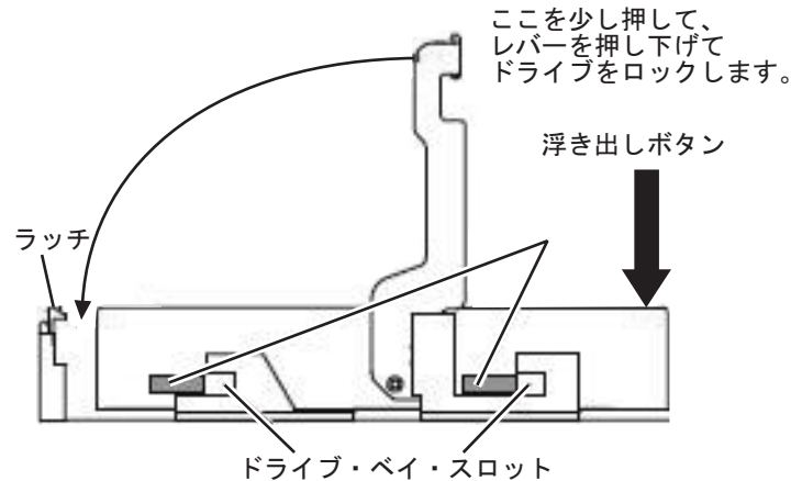
図 80. ハード・ディスクのコネクターへの挿入
