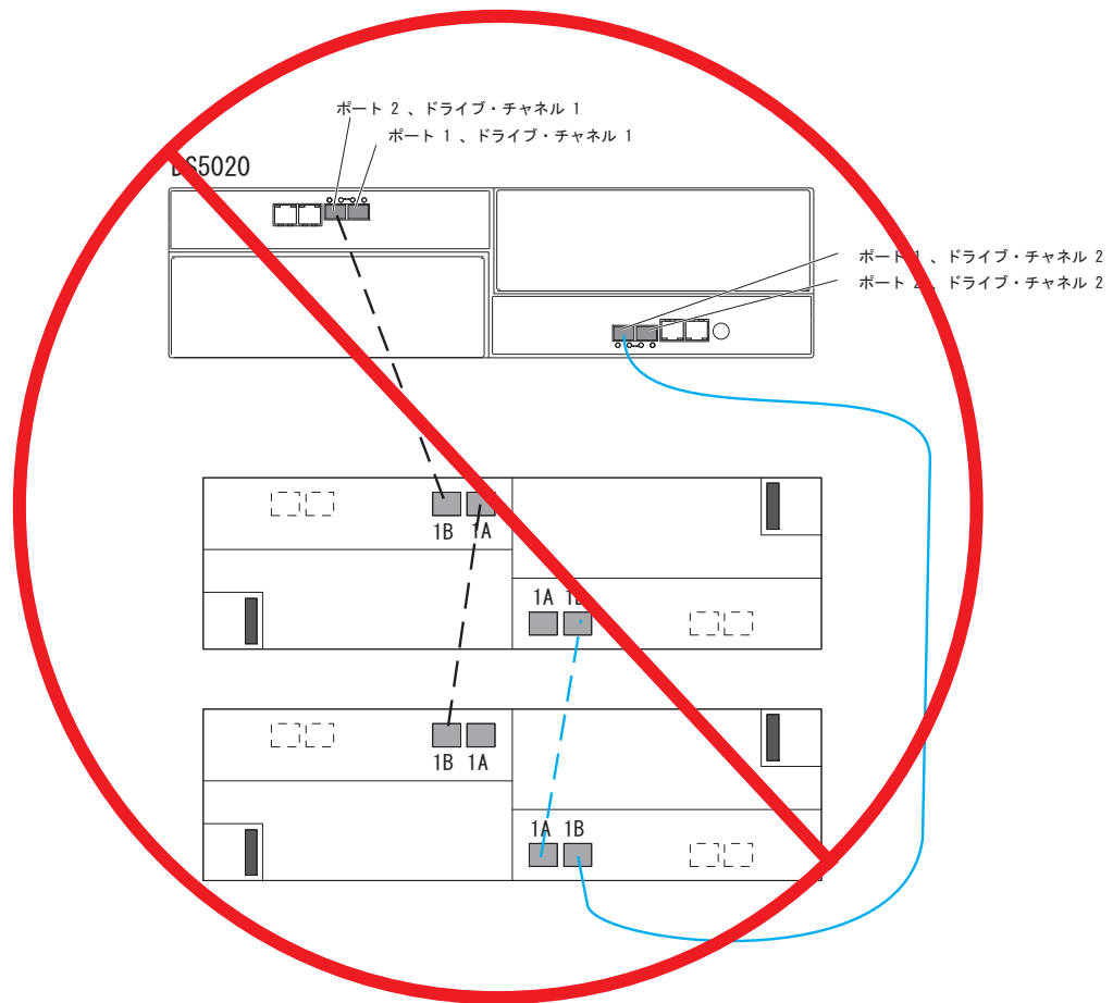
図 39. 1 つの DS5020 と 2 つのストレージ拡張エンクロージャーの誤ったケーブル接続
