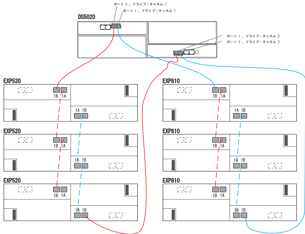
図 44. 混合環境での 1 つの DS5020 と複数のストレージ拡張エンクロージャーのケーブル接続
