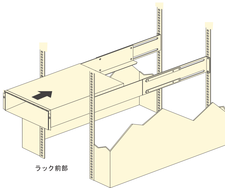
図 19. DS5020 の取り付け
