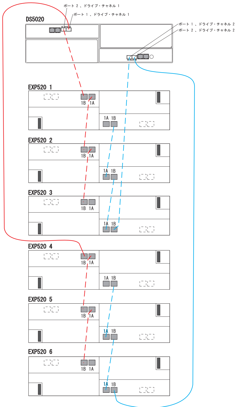
図 50. 1 組の DS5020 ドライブ・ポートの後ろでの 1 つの DS5020 と最大 6 つの EXP520 ストレージ拡張エンクロージャー
