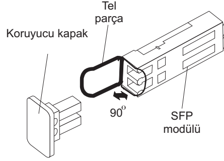
Şekil 30. SFP modül mandalının kilidinin açılması - kablo parçalı
