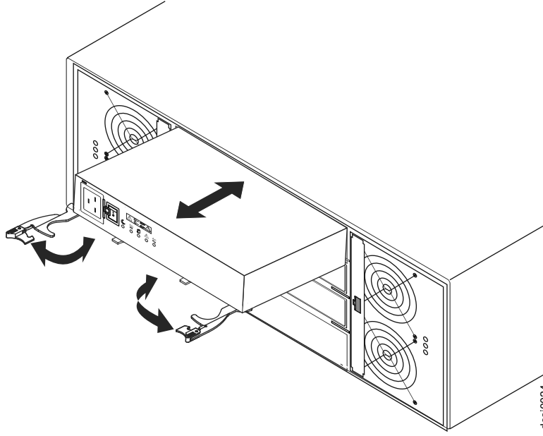
Şekil 76. Güç kaynağının değiştirilmesi
