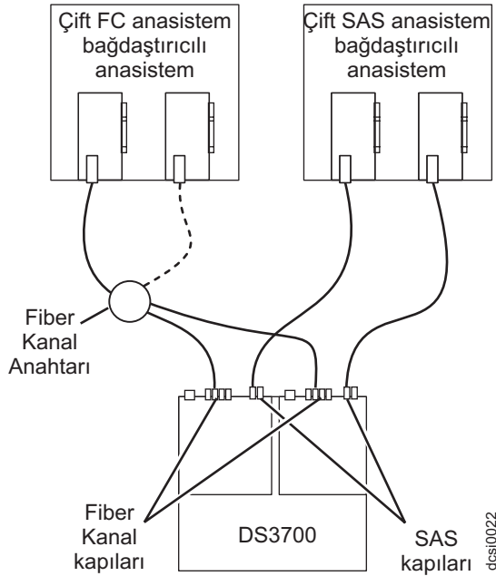
Şekil 48. Birden çok anasistemli, birden çok kapılı ve birden çok yönlü yapıya sahip (Fiber Kanal ve SAS) bir yapılandırma örneği
