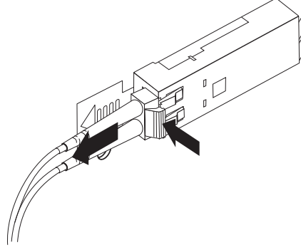
Şekil 36. LC-LC Fiber Kanal kablosunun çıkarılması
