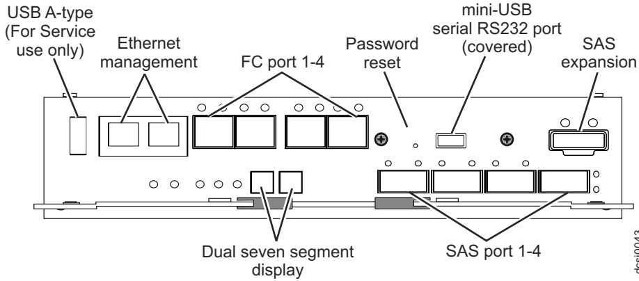
Şekil 20. Performans Modülü Denetleyicilerine sahip DCS3700 depolama altsistemi (SAS kapısı, SAS genişletmesi olarak listelenmiş)
