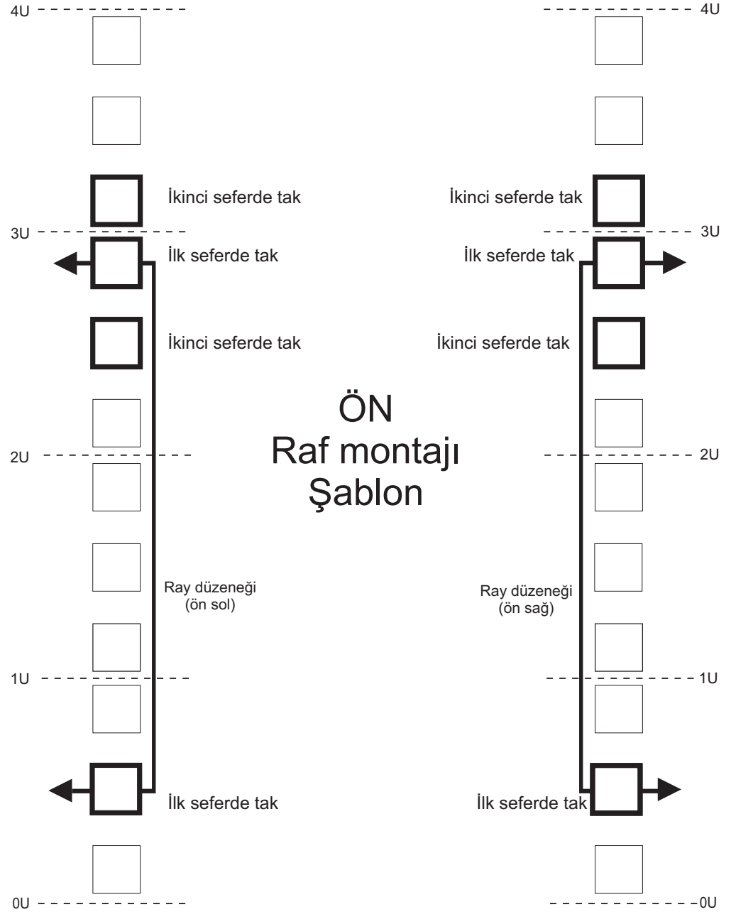
Şekil 16. Ön raf montaj şablonu
