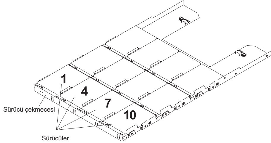
Şekil 18. etiketlenmiş disk sürücüler ile DCS3700 sürücü çekmecesinin
