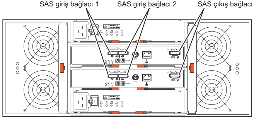
Şekil 8. ESM SAS kapı konumları
