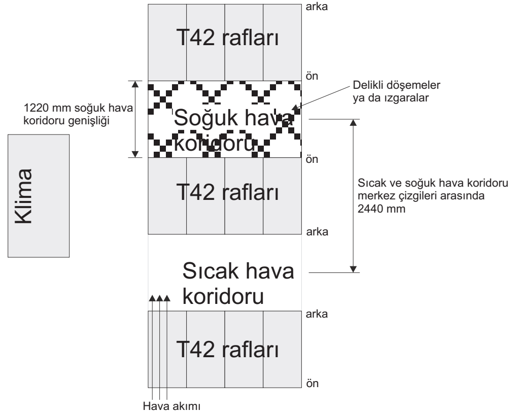
Şekil 15. Soğuk hava koridoru/sıcak hava koridoru raf yapılandırması örneği
