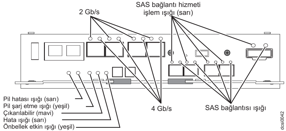
Şekil 53. Performans Modülü Denetleyicilerine sahip bir altsistemdeki denetleyici ışıkları
