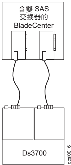
圖 44. 連接至單一 BladeCenter 裝置的 DCS3700 範例
