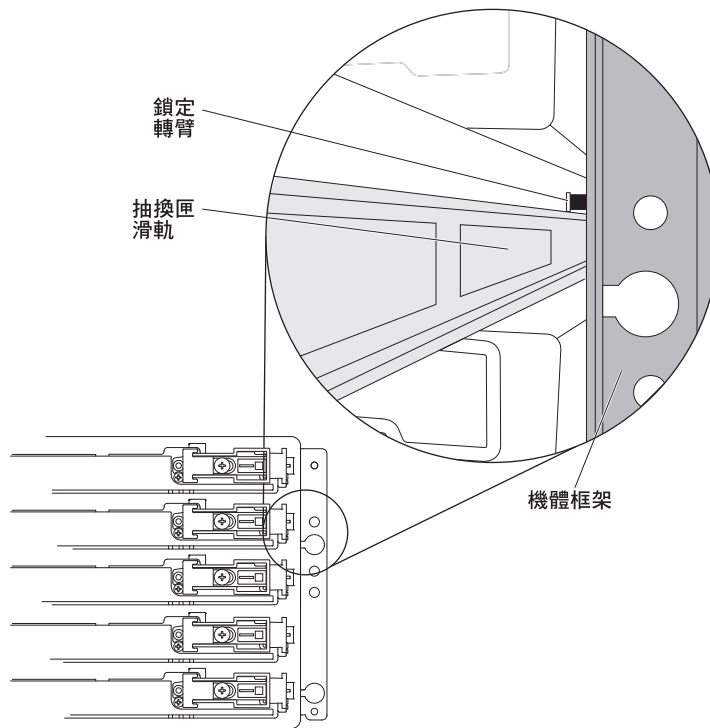
圖 97. 位於抽換匣導軌上面的鎖定桿鎖簧
