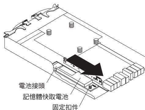
圖 78. 從控制器卸下電池裝置
