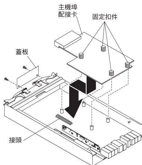
圖 69. 安裝主機埠配接卡
