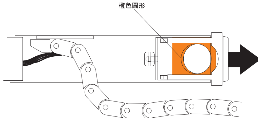
圖 95. 連接至磁碟機抽換匣的水平裝載托架
