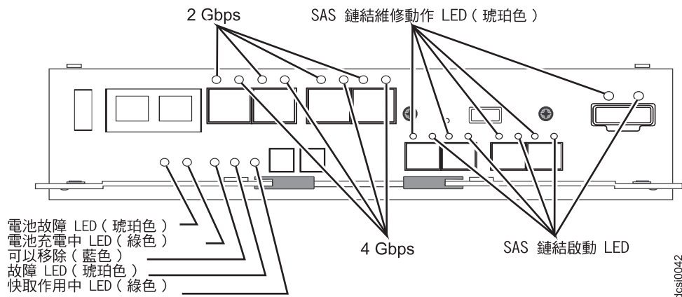
圖 53. 配有效能模組控制器的子系統上的控制器 LED
