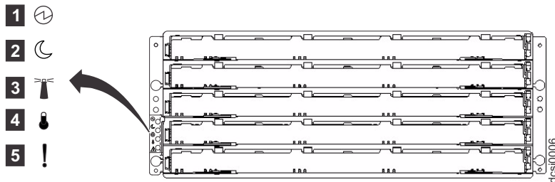
圖 50. DCS3700 正面 LED 及控制項
