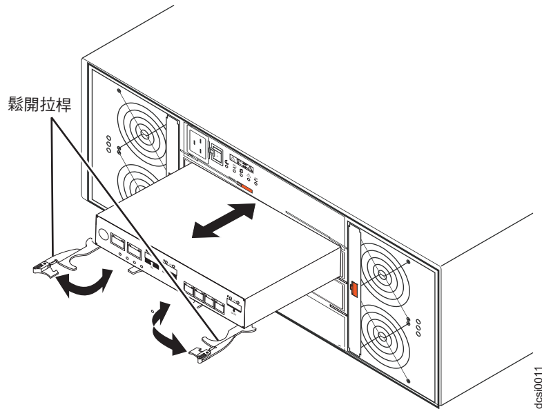
圖 85. 卸下環境服務模組
