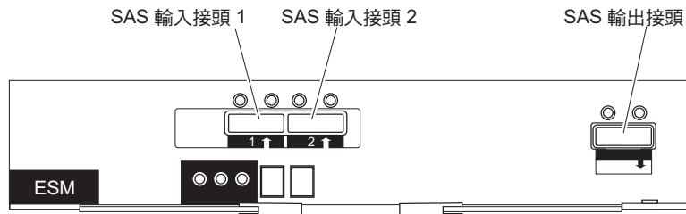
圖 37. ESM 接頭
