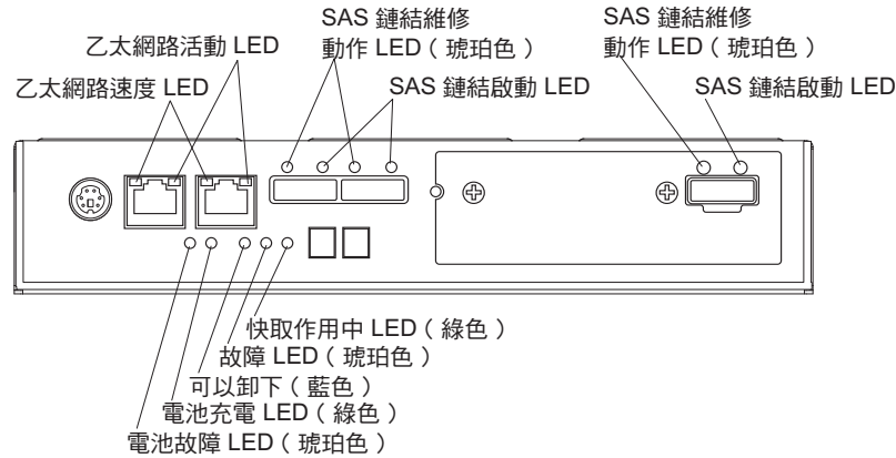
圖 52. 控制器 LED
