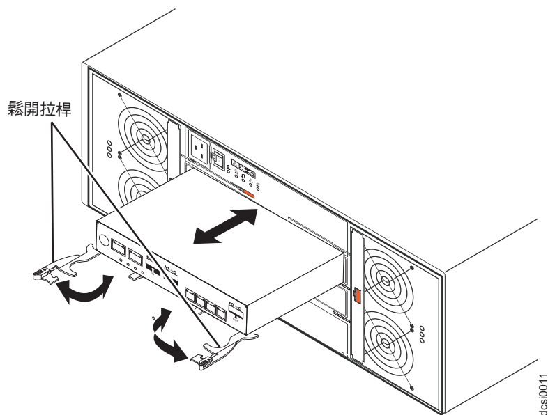
圖 80. 卸下控制器
