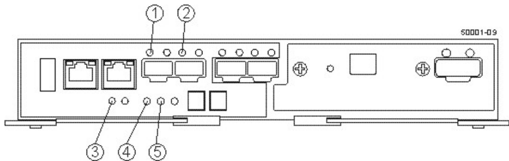
圖 113. 控制器 LED
