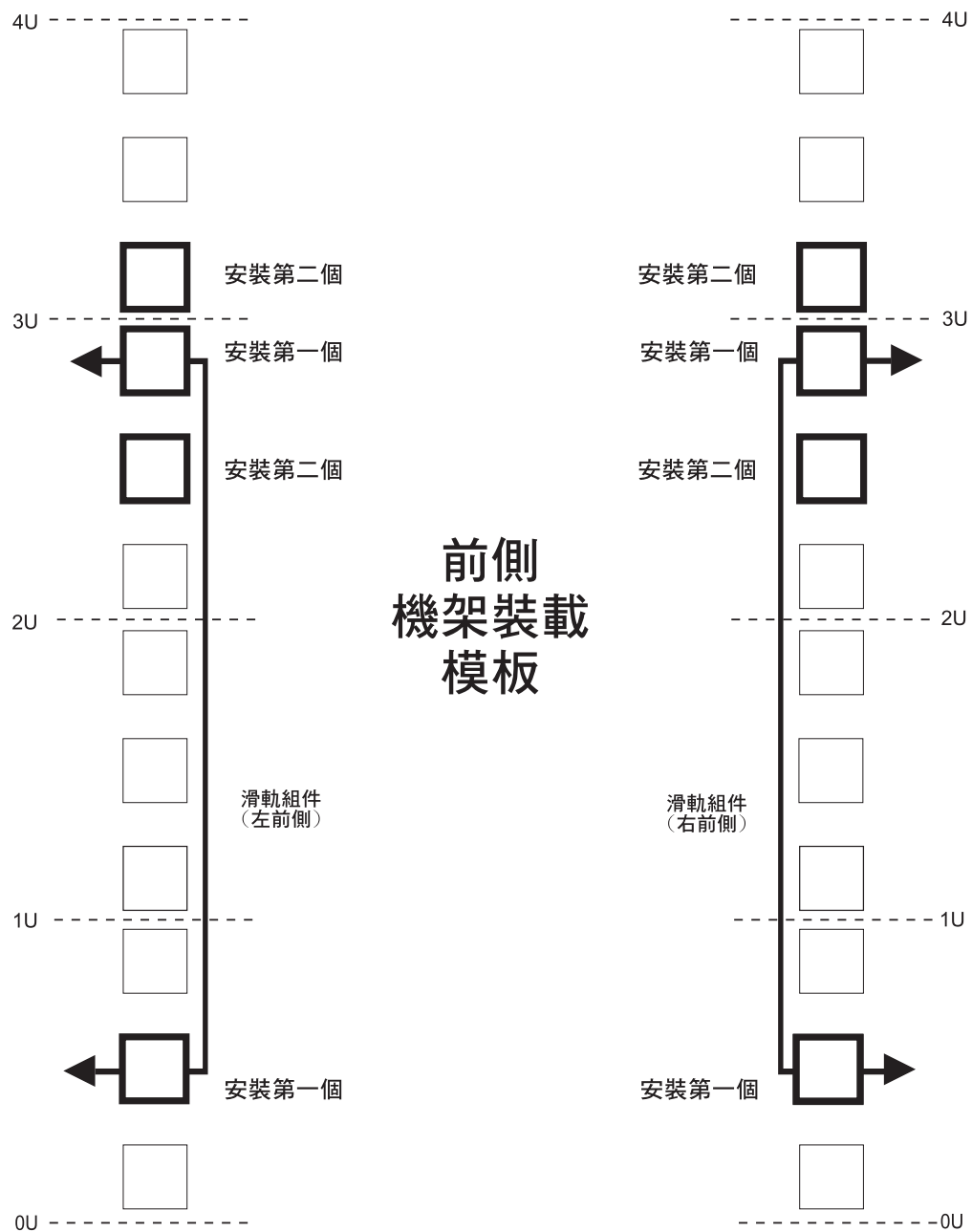
圖 122. 正面機架裝載模板
