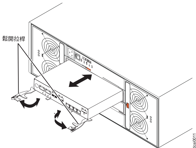
圖 64. 卸下及更換控制器
