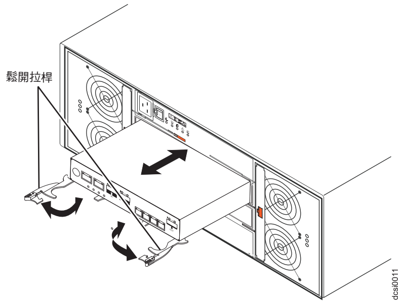
圖 98. 卸下及更換控制器
