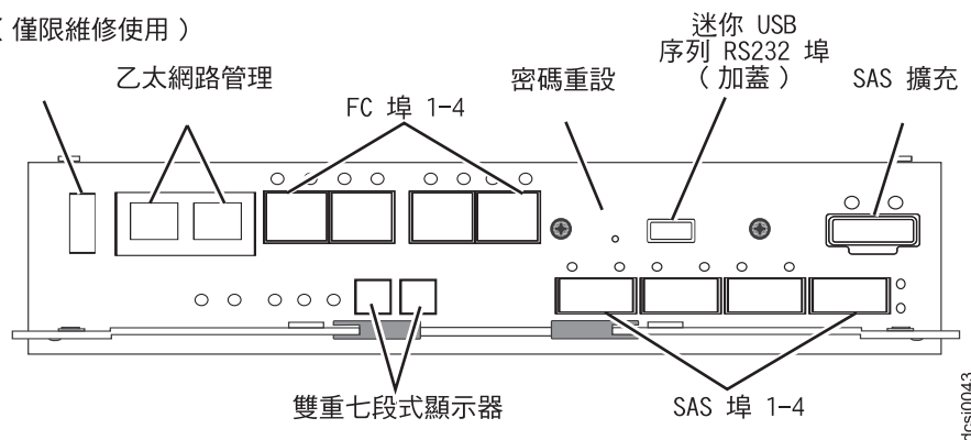
圖 20. 配有效能模組控制器的 DCS3700 儲存體子系統（列示為 SAS 擴充的 SAS 埠）
