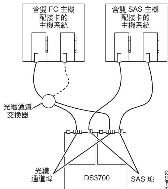
圖 48. 多部主機、多個埠及多個光纖（光纖通道及 SAS）配置的範例
