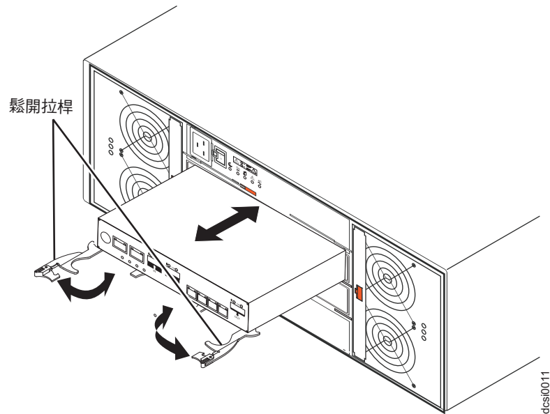
圖 62. 卸下控制器
