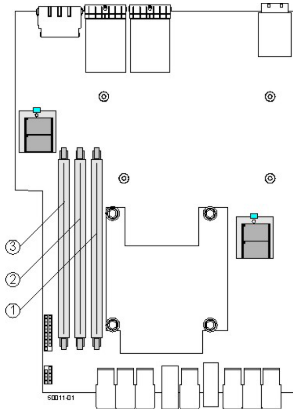
圖 103. 三個快取記憶體 DIMM 插槽
