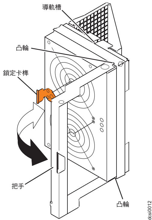
圖 86. 卸下風扇組件
