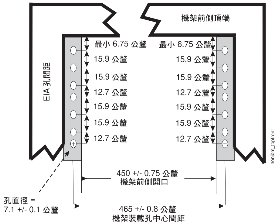
圖 125. 機架規格尺寸，頂端前視圖
