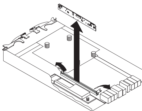
圖 82. 在控制器中安裝 DIMM
