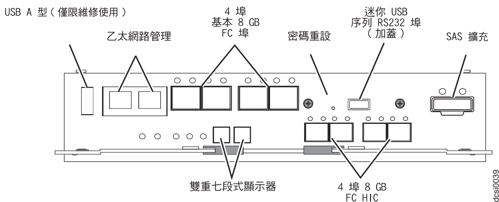
圖 6. 含有效能模組控制器的 DCS3700 儲存體系系統上的接頭
