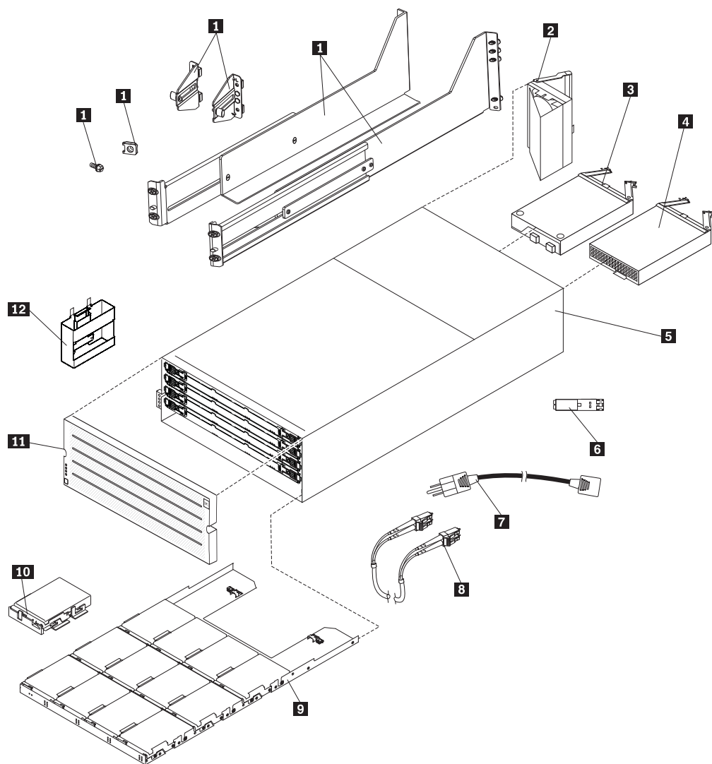
圖 119. DCS3700 儲存體系系統機體零件清單
