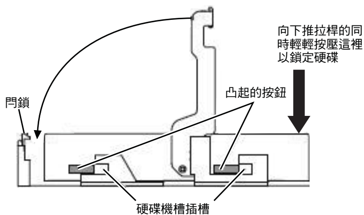
圖 72. 將硬碟插入接頭中
