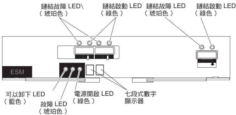
圖 56. ESM LED
