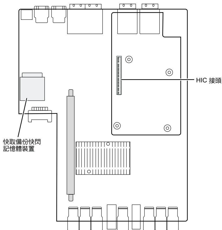
圖 70. 對齊 HIC 接頭
