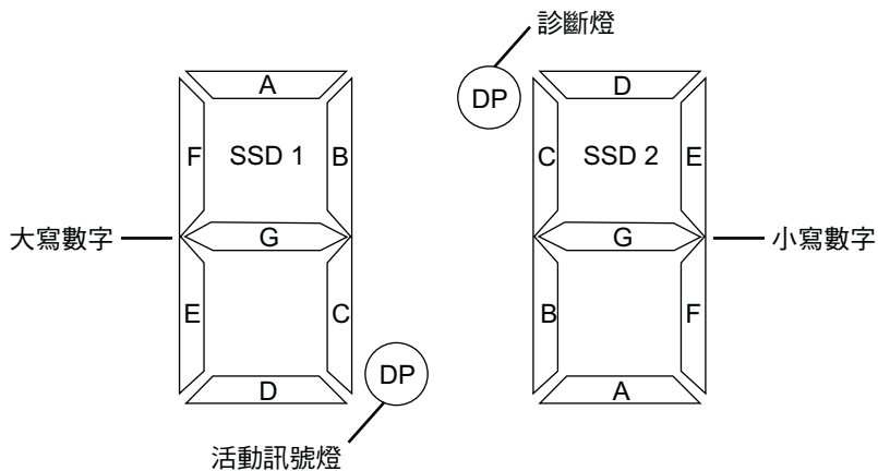
圖 61. 數字顯示器 LED
