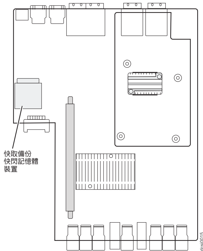
圖 83. 快取備份快閃記憶體裝置
