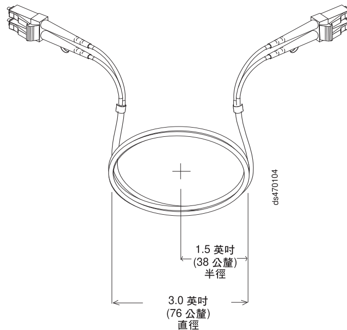
圖 31. 建議的光纖纜線彎曲及線圈規格
