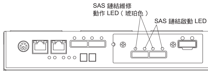
圖 55. SAS 主機埠配接卡 LED
