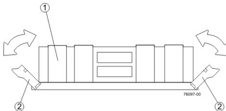
圖 104. 取出快取記憶體 DIMM
