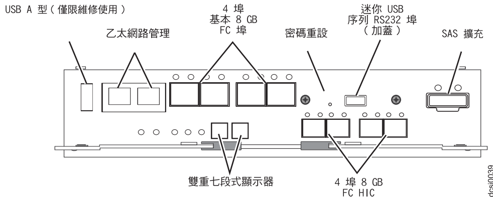
圖 23. 配有效能模組控制器的 DCS3700 子系統上的 FC HIC 埠
