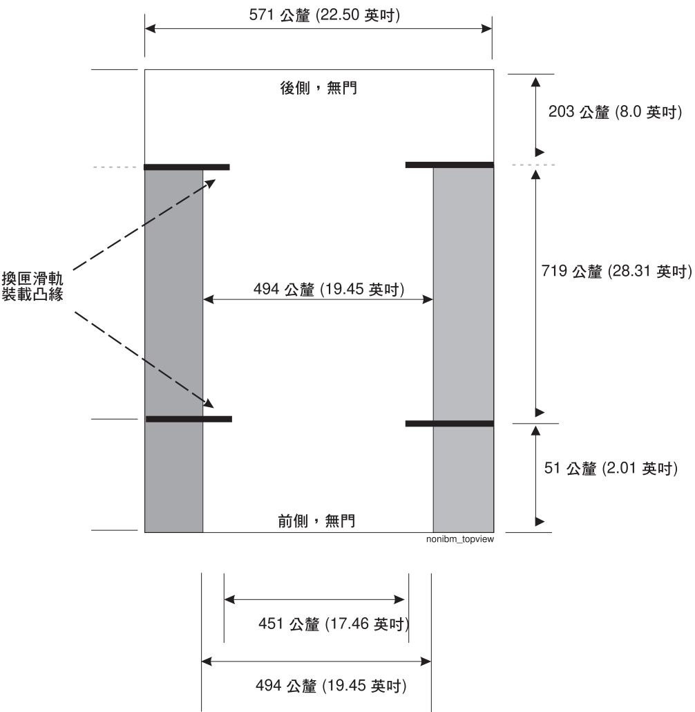
圖 124. 非 IBM 機架規格尺寸的頂端視圖
