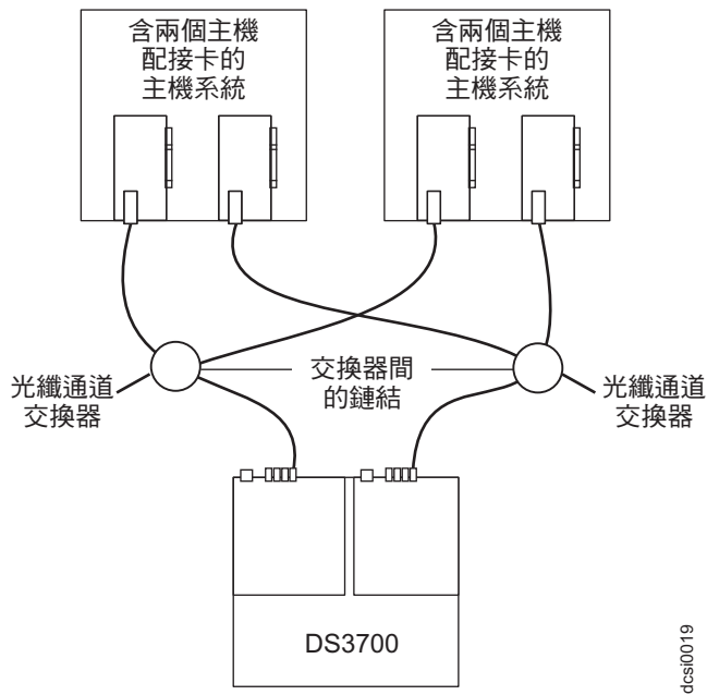
圖 45. 單一光纖通道 SAN 光纖配置的範例
