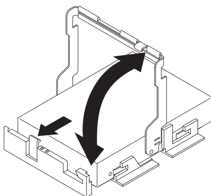
圖 73. 提升磁碟機把手
