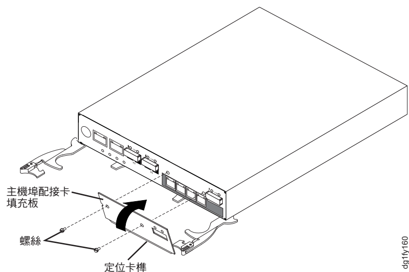
圖 68. 卸下主機埠配接卡填充板
