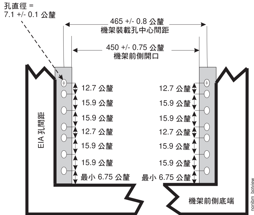
圖 126. 機架規格尺寸，底端前視圖
