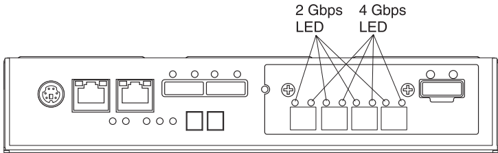
圖 54. 光纖通道主機埠配接卡 LED
