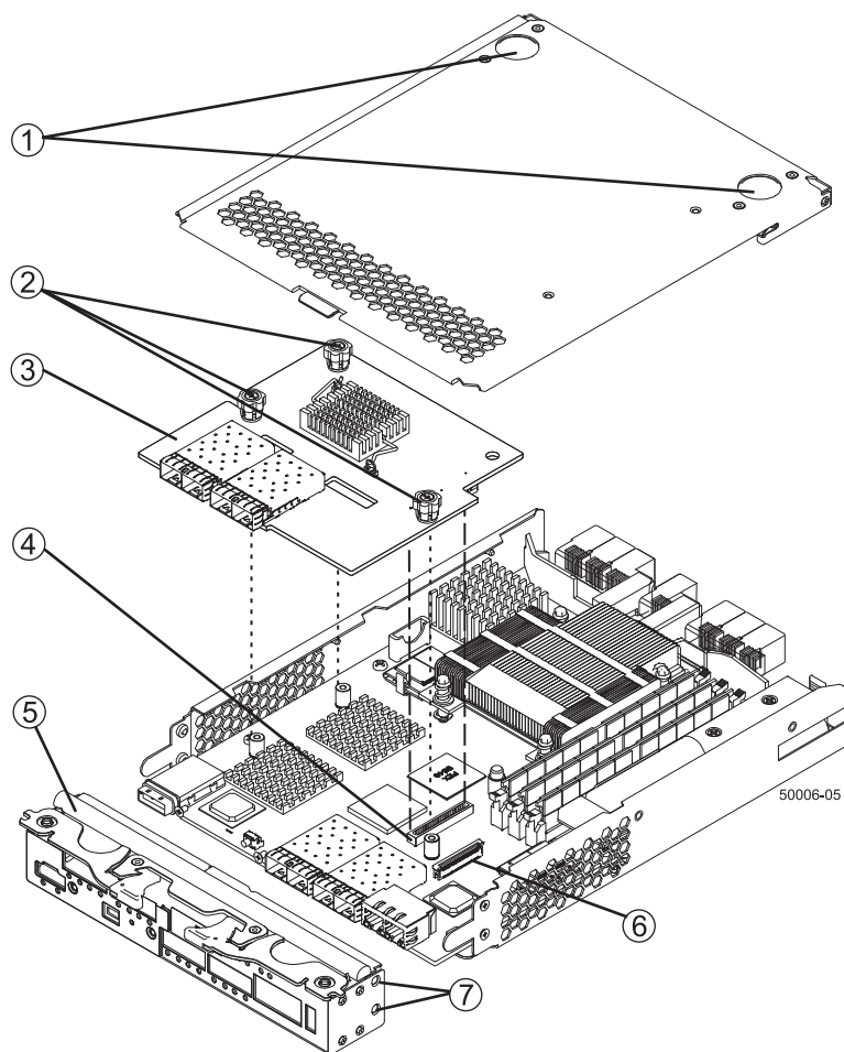
圖 117. 更換主機介面卡
