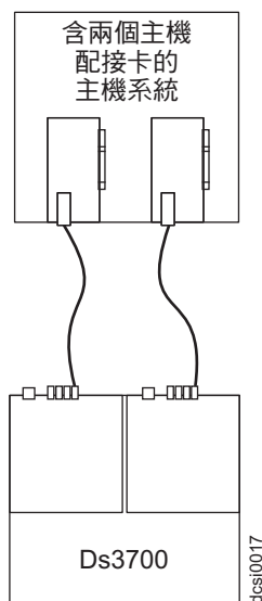
圖 42. 相同主機中兩個 HBA 的雙控制器直接連接型光纖通道連線（備用主機連線）
