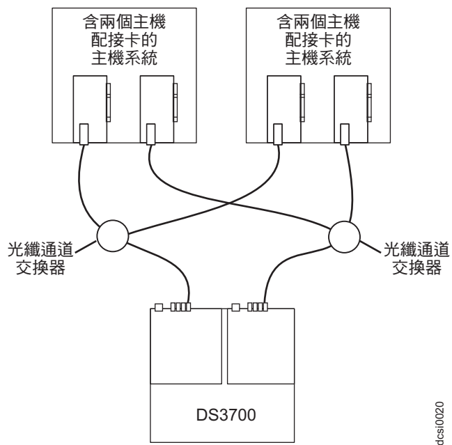
圖 46. 雙光纖通道 SAN 光纖配置的範例
