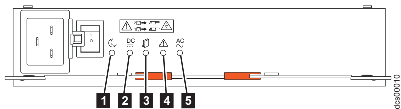
圖 58. AC 電源供應器 LED
