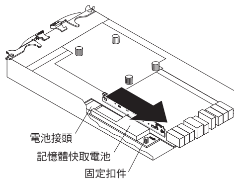
圖 65. 從控制器卸下電池裝置
