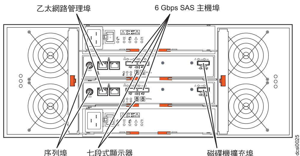
圖 5. DCS3700 接頭
