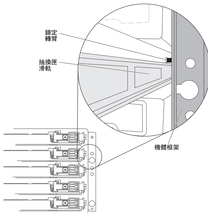
圖 91. 位於抽換匣導軌上面的鎖定桿鎖簧
