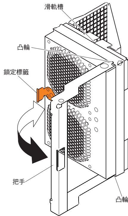
圖 92. 卸下風扇組件
