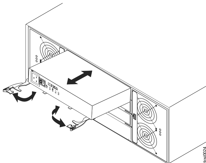
圖 76. 更換電源供應器
