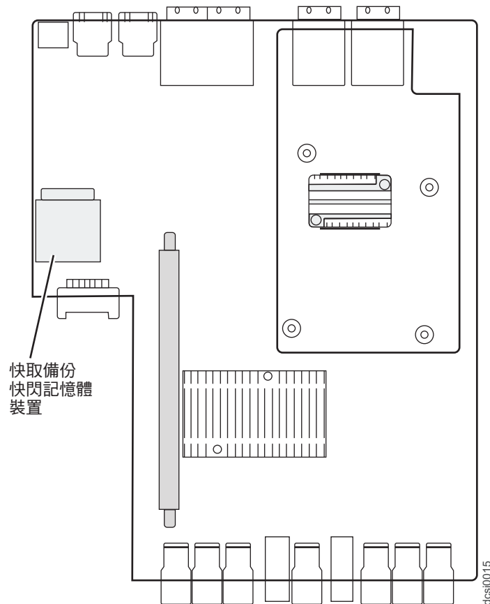
圖 66. 快取備份的快閃記憶體裝置位置
