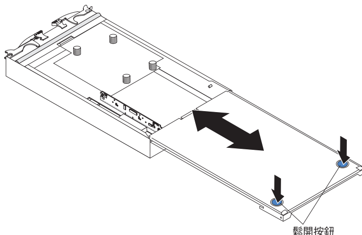
圖 63. 卸下蓋板
