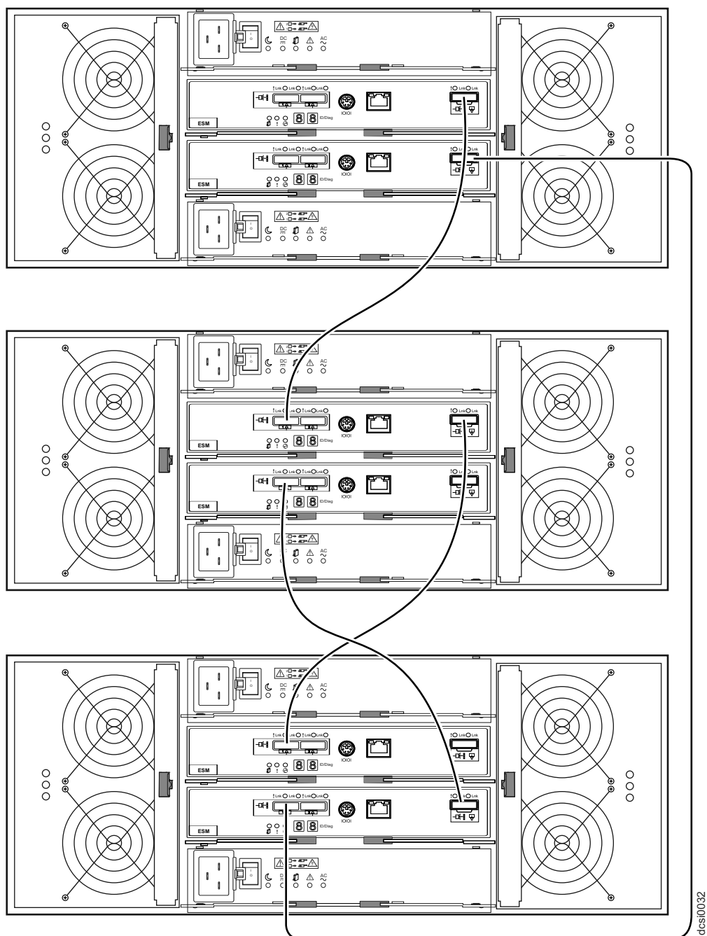
圖 39. 雙擴充機體
