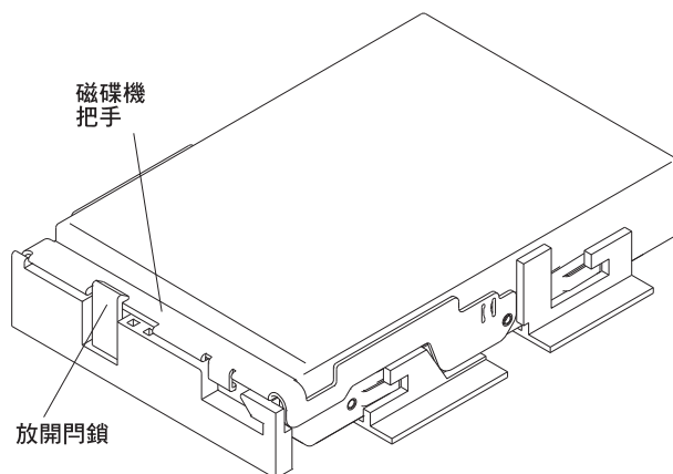
圖 75. 將磁碟機鎖在定位
