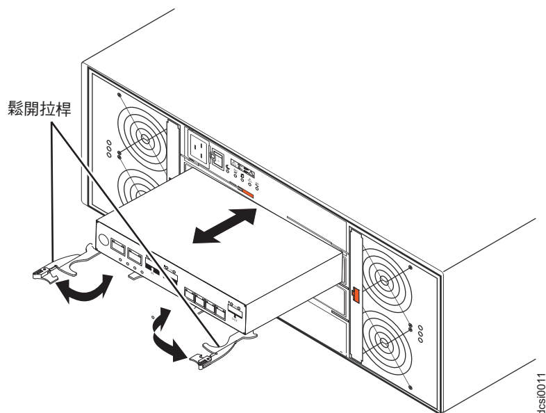
圖 77. 卸下控制器
