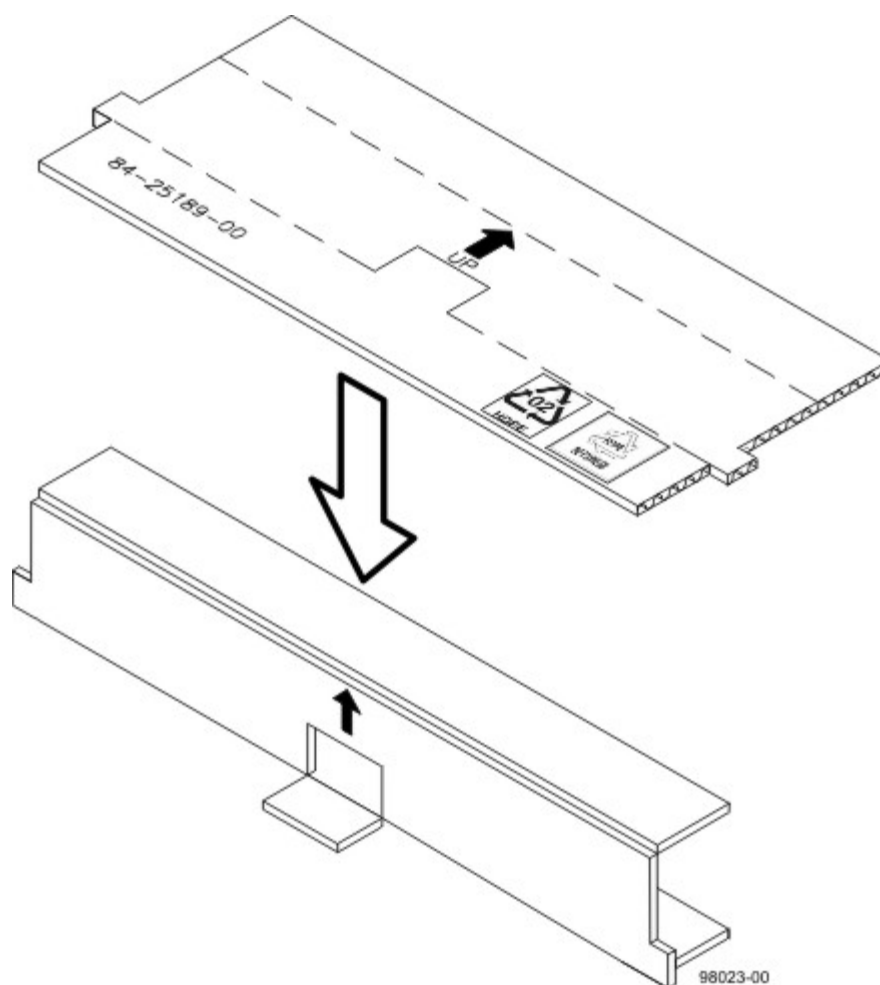
圖 99. 控制器空氣分向閥
