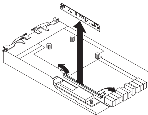
圖 81. 從控制器卸下 DIMM
