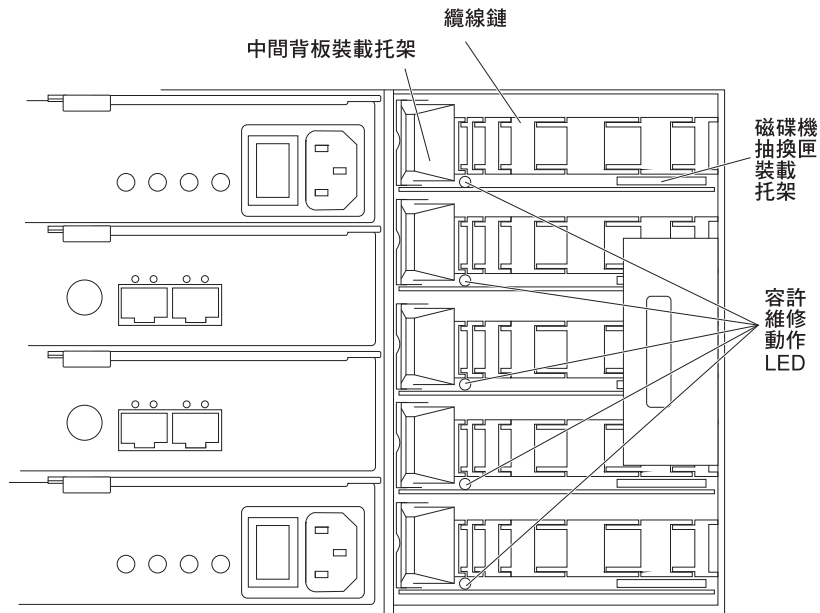
圖 87. 已卸下右側風扇組件的儲存體擴充機體背面視圖
