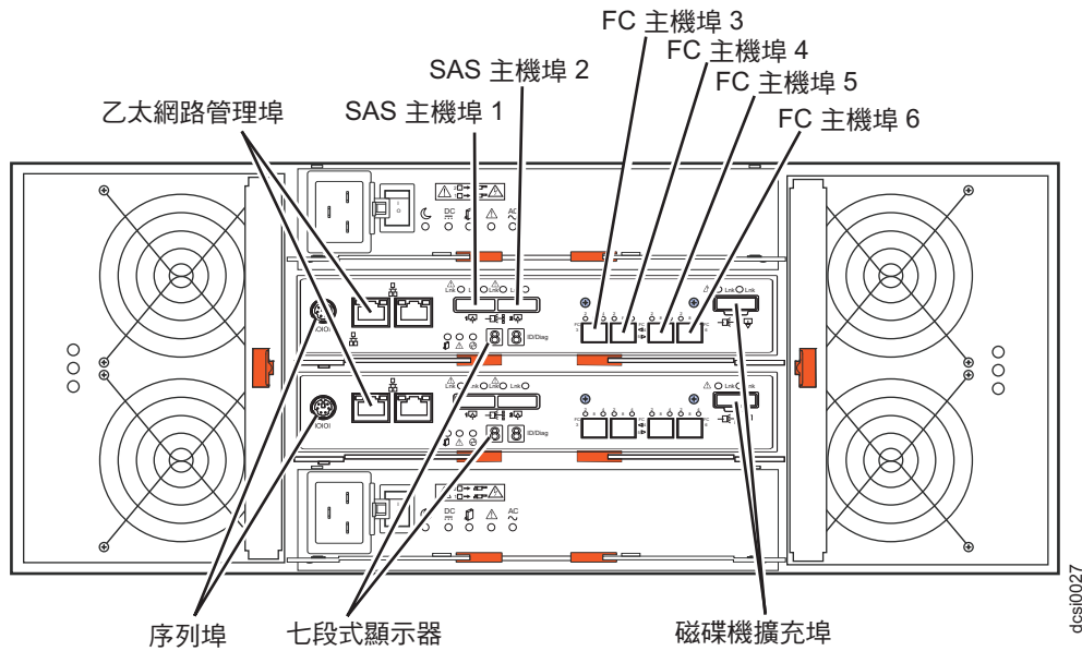
圖 22. 雙控制器 DCS3700 儲存體系系統埠及控制器（含選用光纖通道主機埠配接卡）
