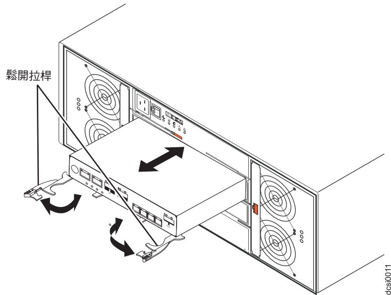
圖 67. 卸下控制器
