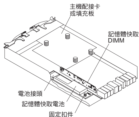
圖 79. 記憶體快取 DIMM 位置
