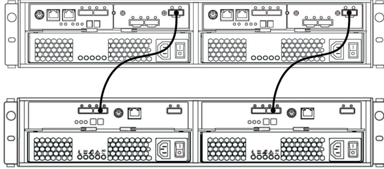
Şekil 40. Çift denetleyicili DS3500 ve depolama kasası
