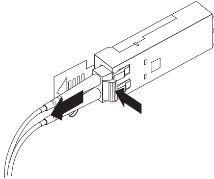
Şekil 31. LC-LC Fiber Kanal kablosunun çıkarılması
