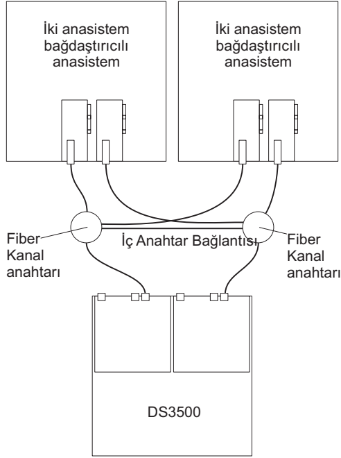
Şekil 61. Tek Fiber Kanal SAN yöneltme yapısı yapılandırması örneği
