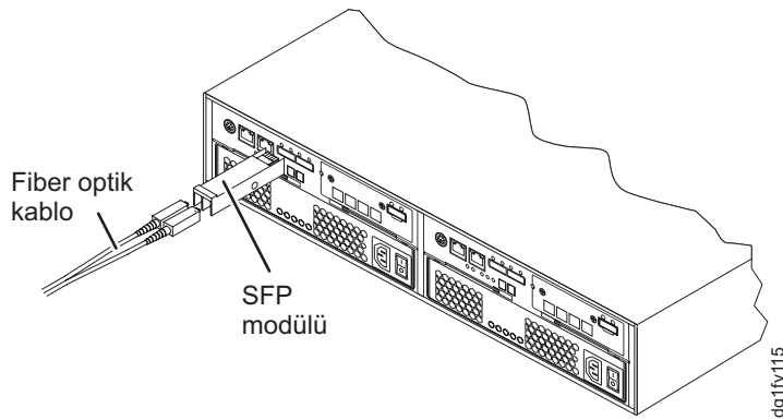
Şekil 121. SFP modülünün anasistem kapağına takılması
