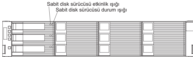
Şekil 98. DS3512 depolama altsistemi ve EXP3512 depolama kasası sürücüsünün ışıkları
