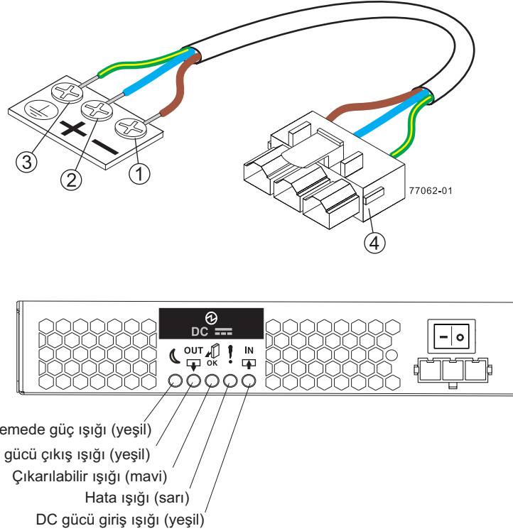
Şekil 110. DS3500 DC modellerine ilişkin DC güç bağlaçları
