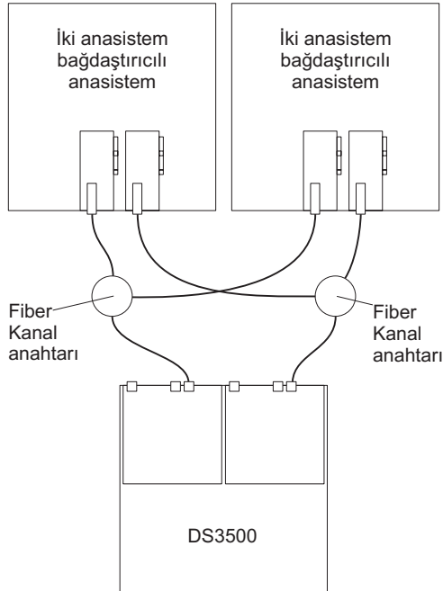
Şekil 62. Çift Fiber Kanal SAN yöneltme yapısı yapılandırması örneği
