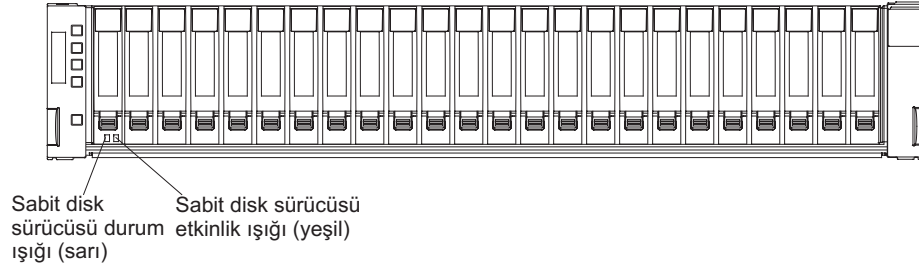
Şekil 99. DS3524 depolama altsistemi ve EXP3524 depolama kasası sürücü ışıkları
