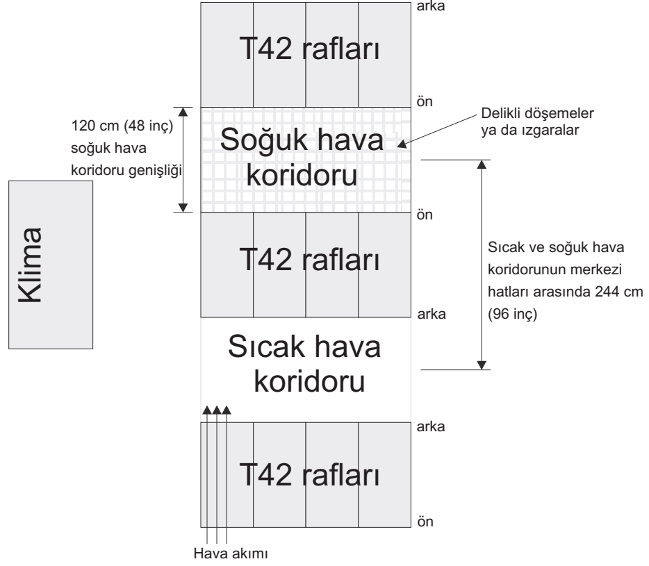
Şekil 15. Soğuk hava koridoru/sıcak hava koridoru raf yapılandırması örneği
