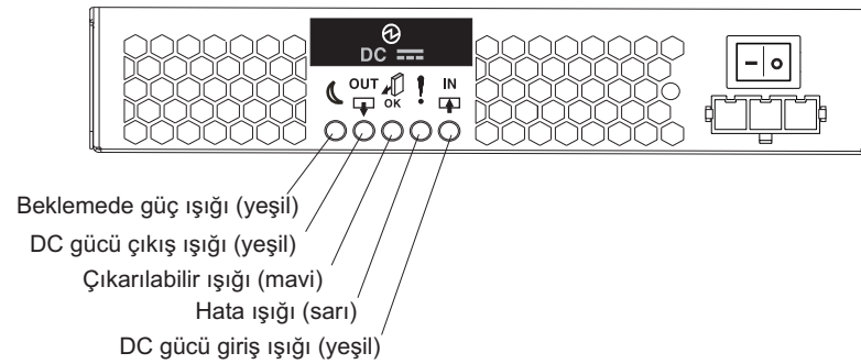
Şekil 109. DC güç kaynağı ışıkları
