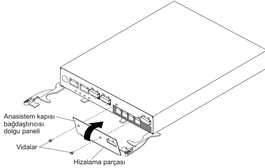
Şekil 96. Anasistem kapısı bağdaştırıcısı dolgu panelinin çıkarılması
