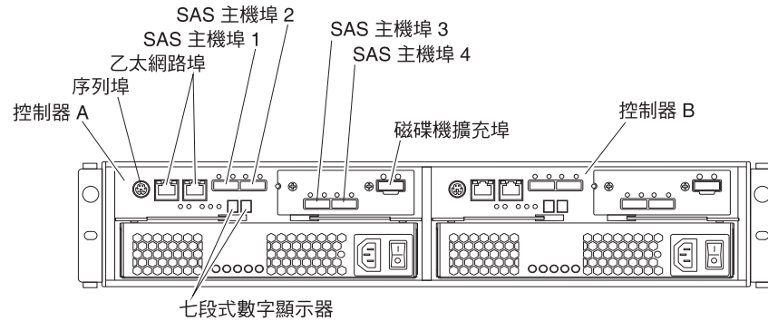
圖 19. 雙控制器 DS3500 儲存體子系統埠及控制器（含選用 SAS 主機埠配接卡）
