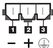
圖 73. DC 電源接頭 - 插腳位置
