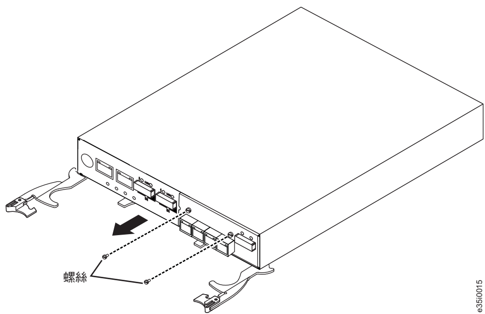
圖 97. 安裝主機埠配接卡
