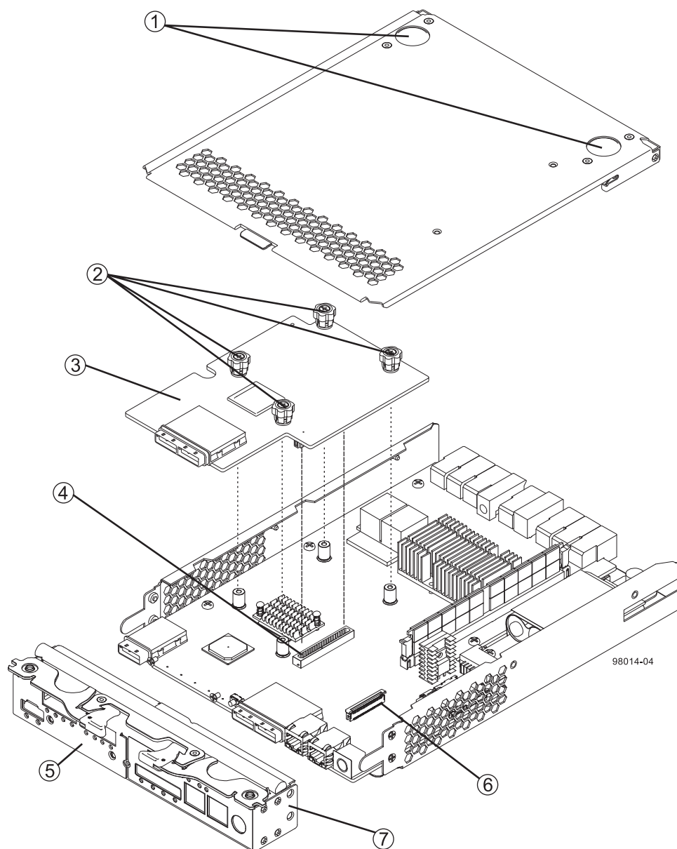
圖 94. 卸下控制器元件的順序
