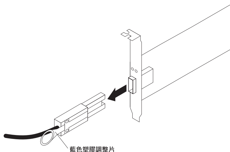
圖 22. 拔掉迷你 SAS 纜線
