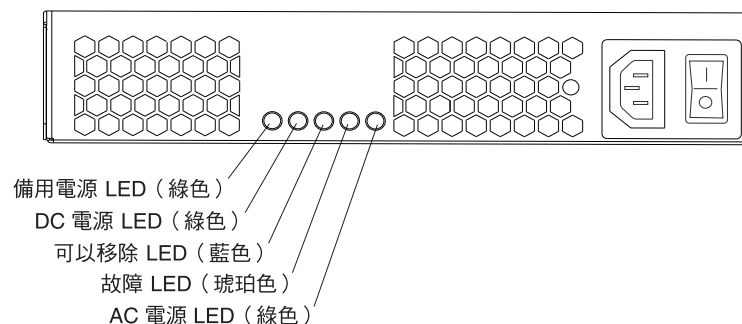
圖 77. AC 電源供應器 LED
