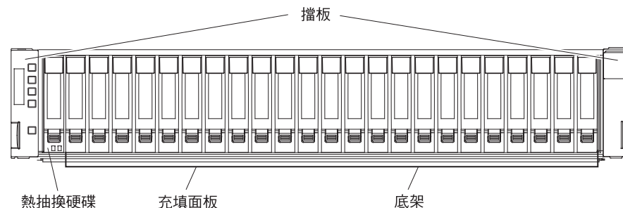
圖 3. DS3524 儲存體子系統和 EXP3524 儲存體機體熱抽換硬碟機槽和隔板
