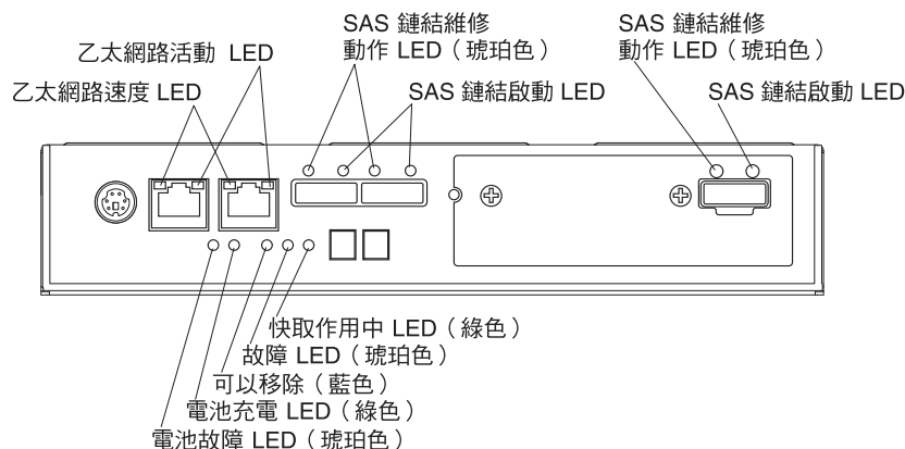
圖 81. 控制器 LED
