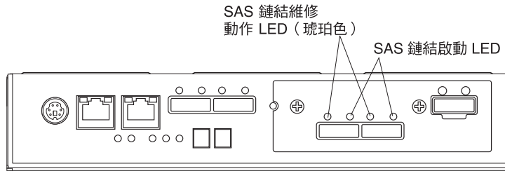
圖 84. SAS 主機埠配接卡 LED
