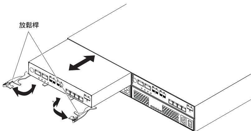
圖 113. 卸下控制器
