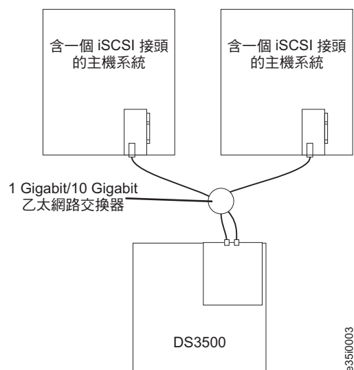
圖 66. 多個單一埠主機、單控制器 iSCSI 配置
