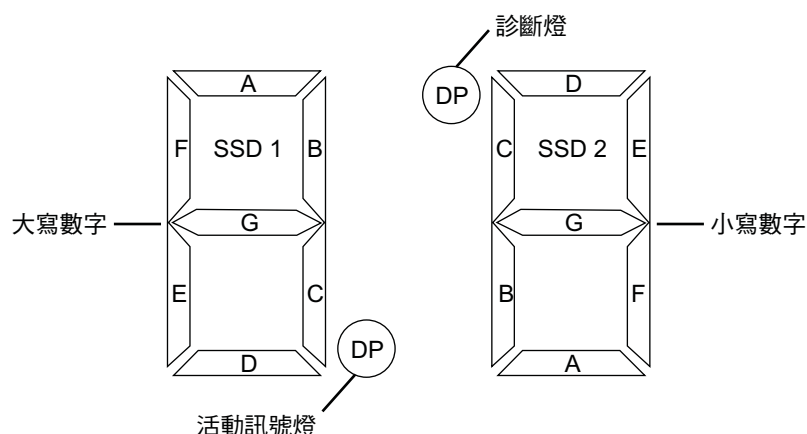
圖 86. 數字顯示器 LED
