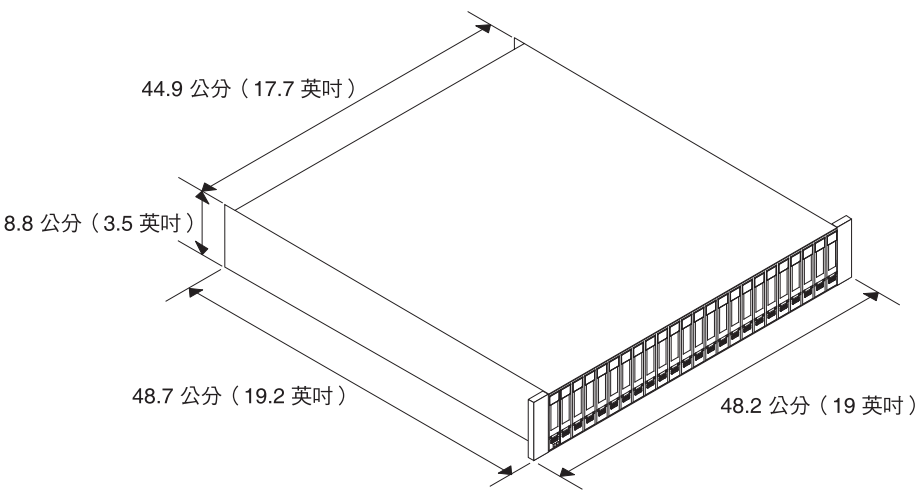
圖 14. DS3524 儲存體子系統和 EXP3524 儲存體機體尺寸
