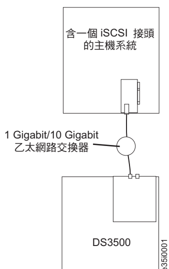
圖 64. 單一主機、單控制器 iSCSI 配置
