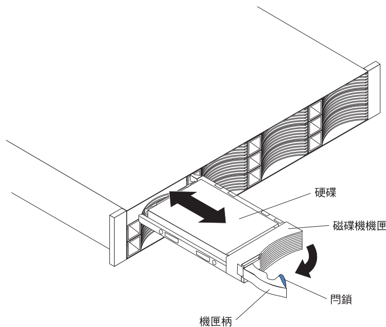
圖 100. 從 DS3512 或 EXP3512 卸下硬碟
