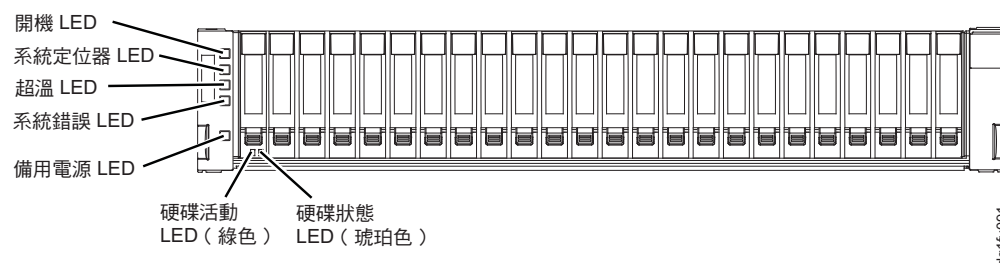
圖 119. DS3524 儲存體子系統和 EXP3524 儲存體機體正面 LED
