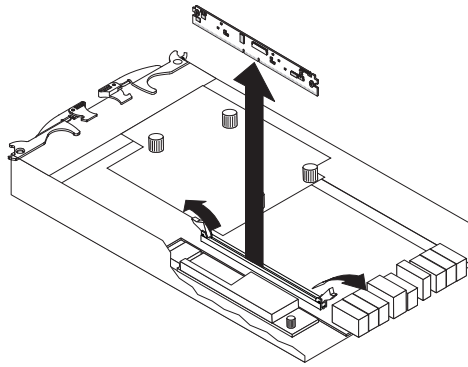
圖 118. 在控制器中安裝 DIMM
