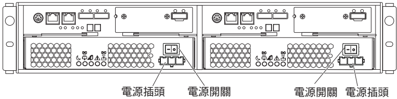
圖 10. DC 電源供應器元件
