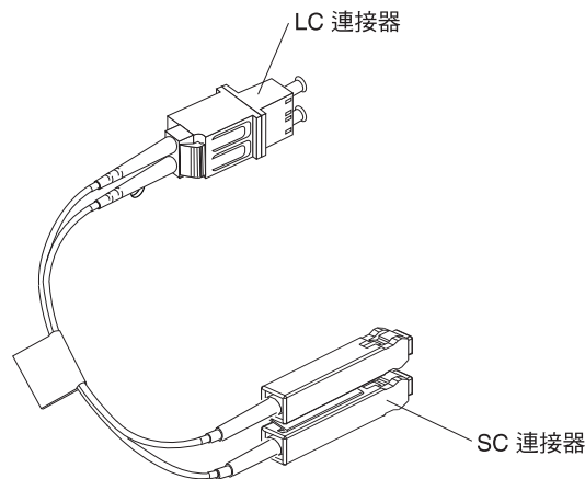
圖 32. 「LC-SC 光纖通道」纜線轉接器
