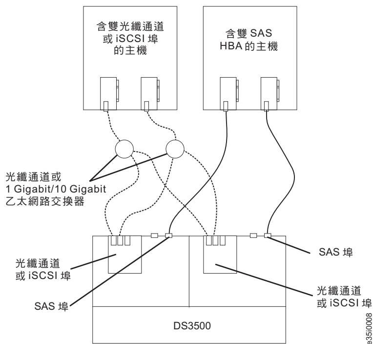
圖 71. 多個主機、多個埠及多個光纖（「光纖通道」或 iSCSI 及 SAS）配置的範例
