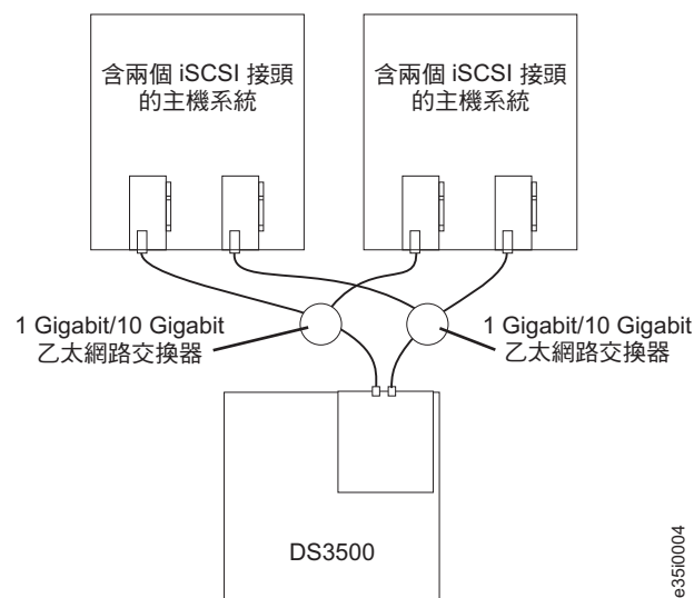
圖 67. 多個主機、多個埠、單控制器及備用路徑 iSCSI 配置
