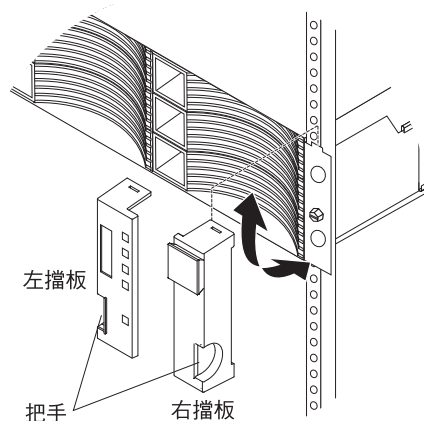
圖 122. 卸下隔板
