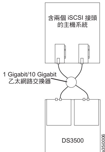
圖 69. 單一主機、多個埠、雙控制器 iSCSI 配置
