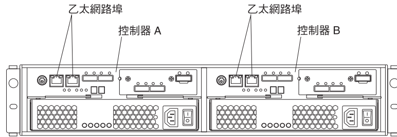
圖 43. 雙控制器 DS3500 上的乙太網路埠位置
