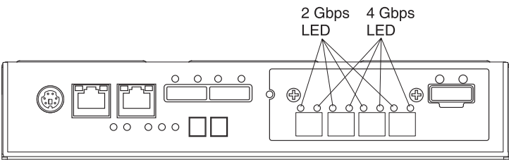
圖 83. 「光纖通道」主機埠配接卡 LED
