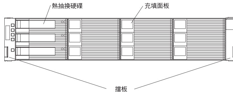
圖 2. DS3512 儲存體子系統和 EXP3512 儲存體機體熱抽換硬碟機槽和隔板
