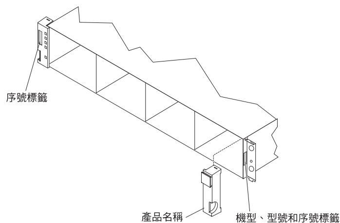
圖 130. DS3500 上的序號位置
