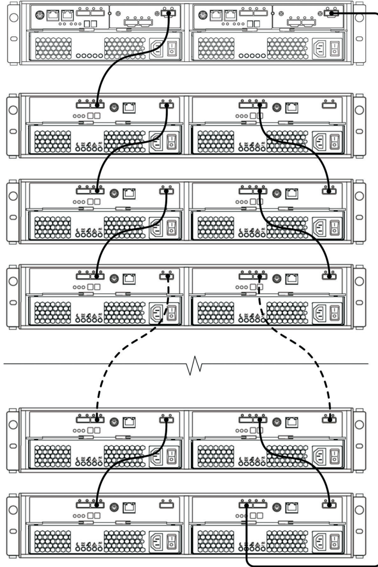
圖 42. 一個雙控制器 DS3500 及八個 儲存體機體
