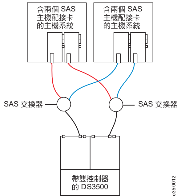
圖 52. 使用兩個獨立的 SAS 交換器連接至多部主機的双控制器 DS3500 SAS 連線
