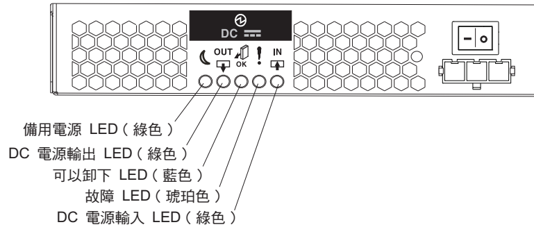
圖 78. DC 電源供應器 LED
