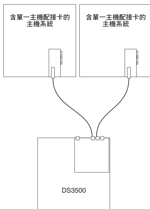
圖 58. 多個主機中單一 HBA 的單控制器直接連接型「光纖通道」連線
