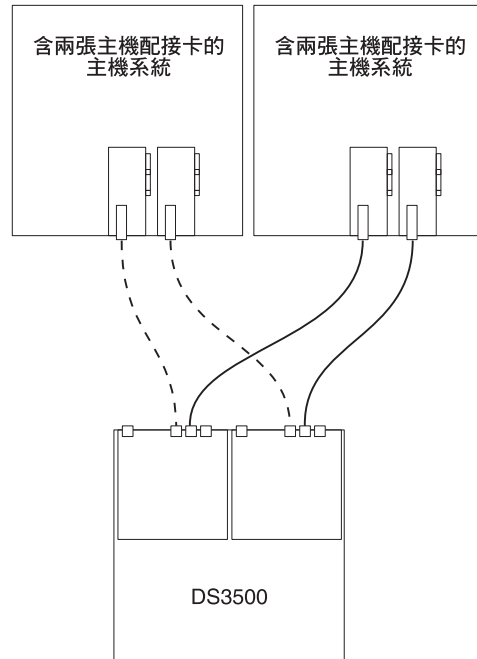
圖 50. 多個主機中多個 HBA 的雙控制器直接連接的 SAS 連線
