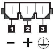
圖 11. DC 電源供應器接頭 - 插腳位置
