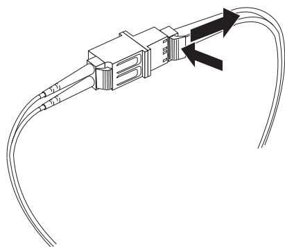
圖 36. 從「LC-SC 光纖通道」纜線轉接器拔掉「LC-LC 光纖通道」纜線
