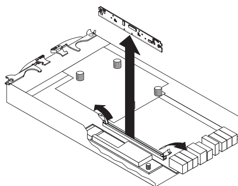
圖 117. 從控制器卸下 DIMM
