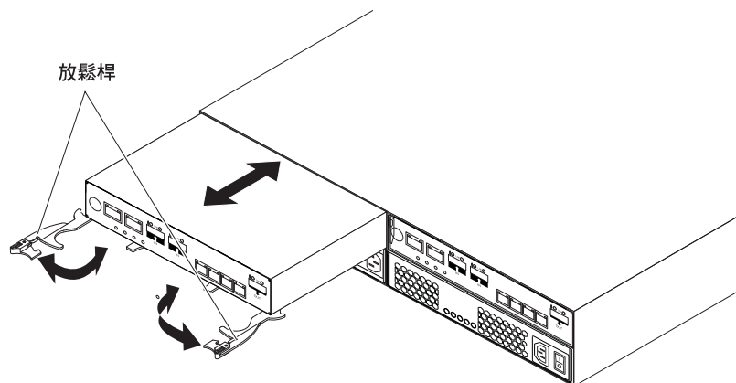
圖 91. 卸下及更換控制器
