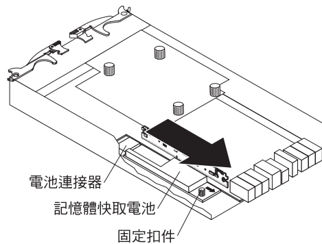
圖 114. 卸下控制器中的電池裝置
