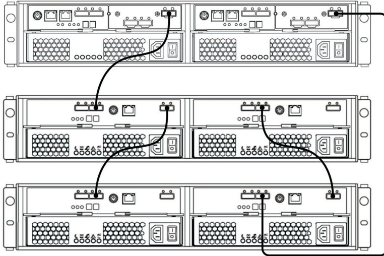
圖 41. 一個雙控制器 DS3500 及兩個儲存體機體
