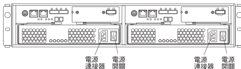
圖 75. DS3500 AC 型號的電源供應器開關及接頭
