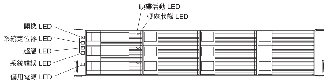
圖 79. DS3512 儲存體子系統和 EXP3512 儲存體機體正面 LED 及控制項
