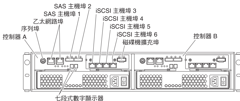
圖 17. 雙控制器 DS3500 儲存體子系統埠及控制器（含選用 iSCSI 主機埠配接卡）
