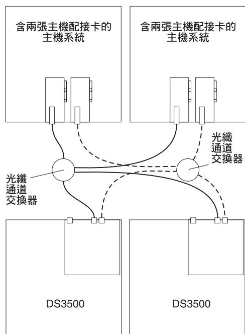
圖 63. 雙重「光纖通道」SAN 環境中兩個儲存體子系統的範例
