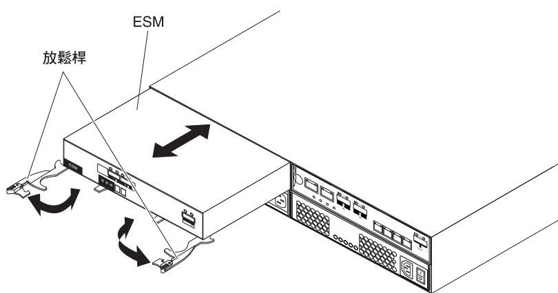
圖 123. 卸下環境服務模組
