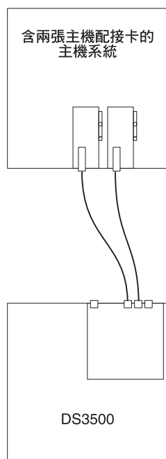
圖 57. 雙重 HBA 的單控制器直接連接型「光纖通道」連線（備用主機連線）
