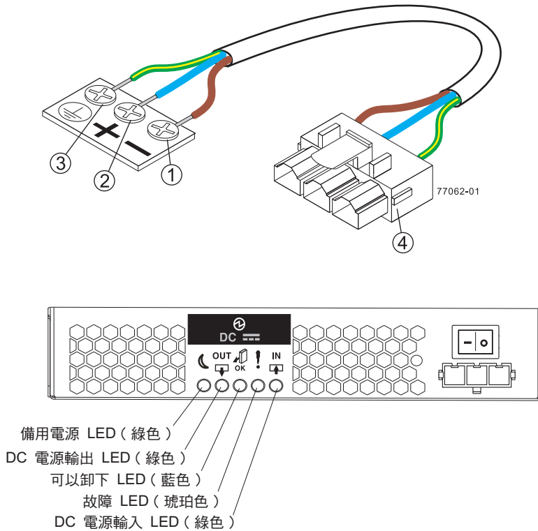
圖 110. DS3500 DC 型號的 DC 電源接頭
