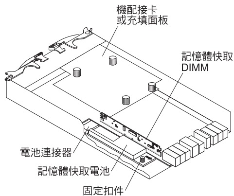
圖 12. 電池裝置
