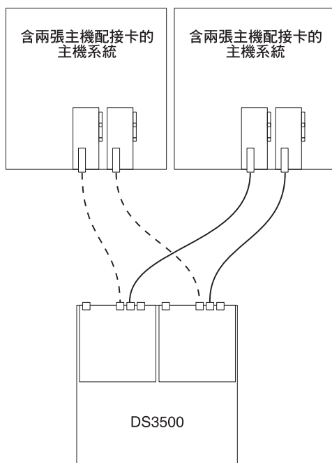
圖 60. 多個主機中多個 HBA 的雙控制器直接連接型「光纖通道」連線
