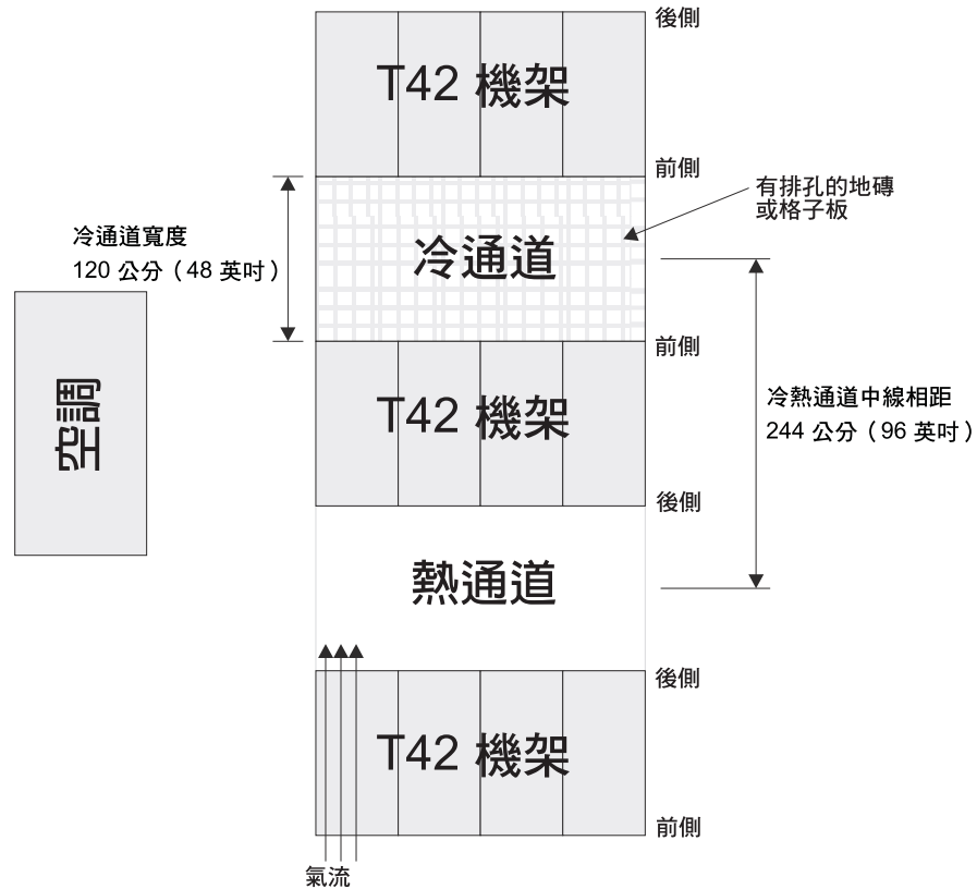
圖 15. 冷通道/熱通道機櫃配置的範例
