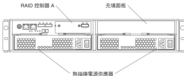
圖 7. 背面圖，單控制器型號（不含選用主機埠配接卡）
