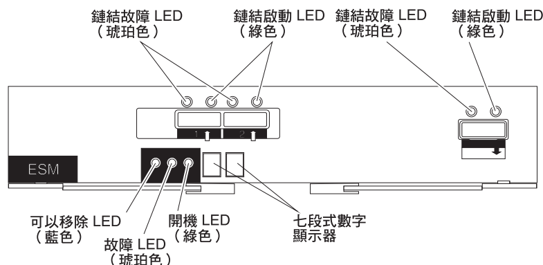
圖 87. ESM LED
