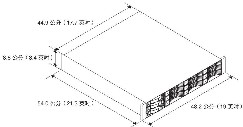
圖 13. DS3512 儲存體子系統和 EXP3512 儲存體機體尺寸
