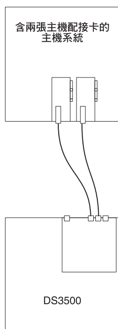
圖 47. 單一主機中雙重 HBA 的單控制器直接連接型 SAS 連線（備用主機連線）
