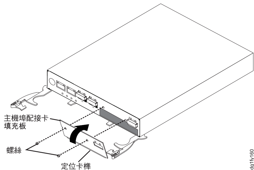
圖 96. 卸下主機埠配接卡填充板
