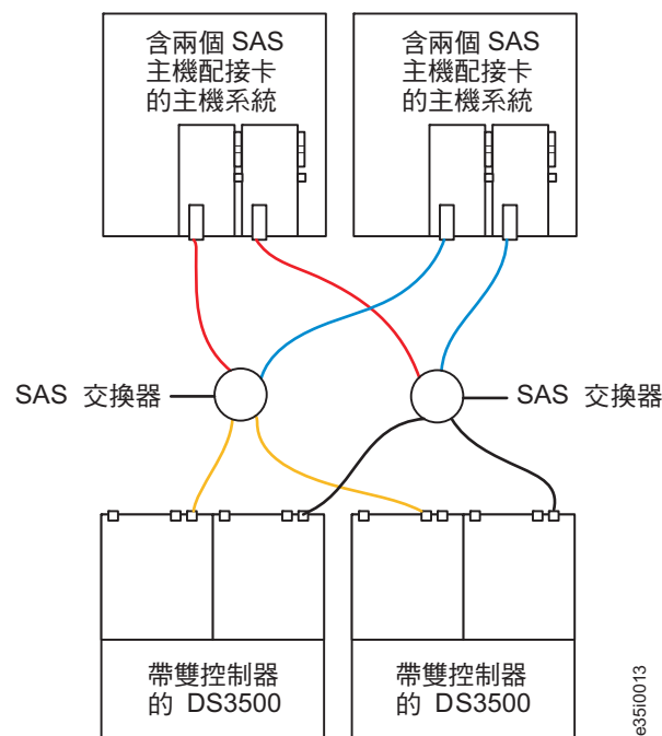
圖 53. 使用兩個獨立的 SAS 交換器連接至多部主機的多個雙控制器 DS3500 SAS 連線
