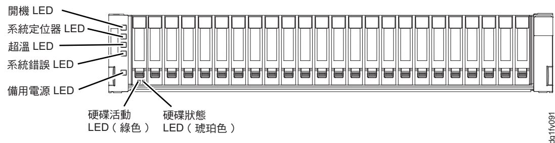
圖 80. DS3524 儲存體子系統和 EXP3524 儲存體機體正面 LED
