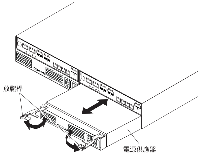
圖 104. 更換電源供應器
