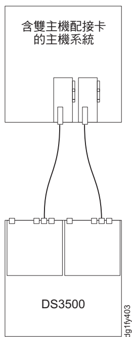
圖 59. 相同主機中兩個 HBA 的雙控制器直接連接型「光纖通道」連線（備用主機連線）
