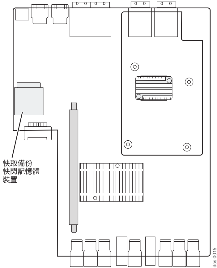
圖 93. 快取備份快閃記憶體裝置
