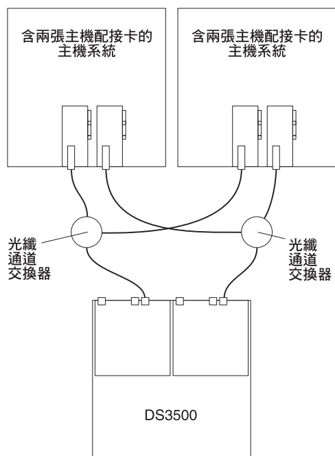
圖 62. 雙重「光纖通道」SAN 光纖配置的範例
