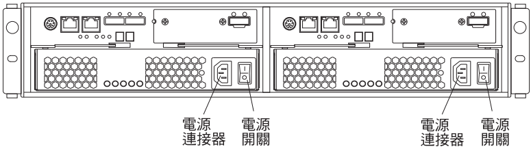
圖 9. AC 電源供應器元件
