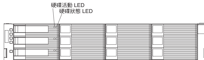
圖 98. DS3512 儲存體子系統和 EXP3512 儲存體機體硬碟 LED
