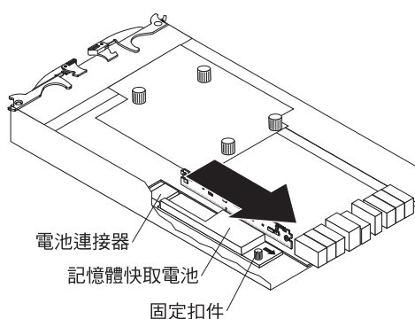
圖 92. 從控制器卸下電池裝置
