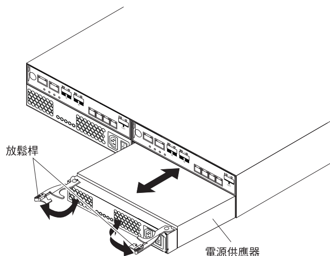
圖 112. 更換電源供應器
