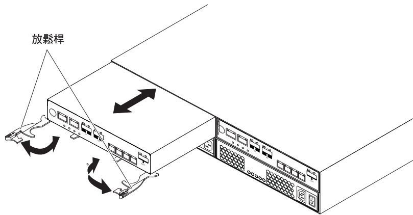
圖 88. 卸下控制器
