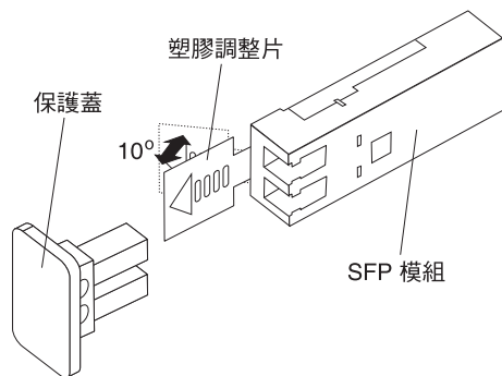
圖 25. 鬆開 SFP 模組門鎖 - 塑膠類
