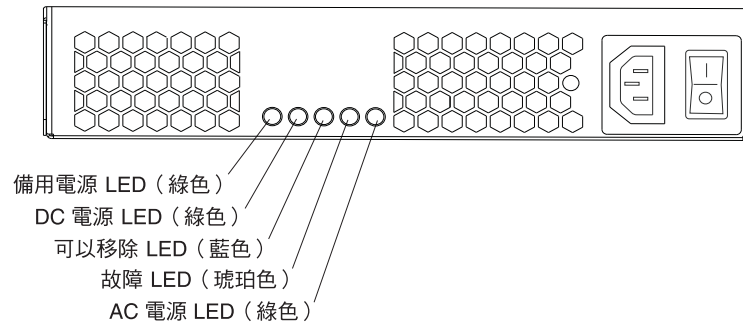
圖 106. AC 電源供應器 LED
