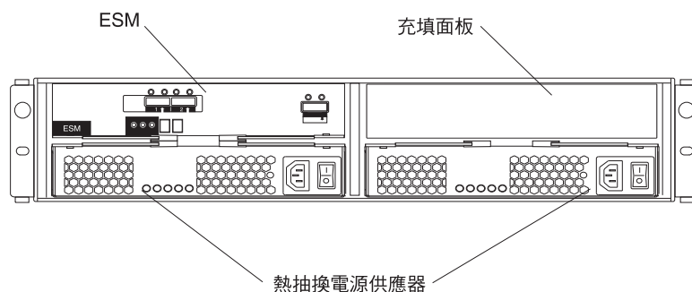
圖 8. 背面圖，單一 ESM 型號儲存體機體
