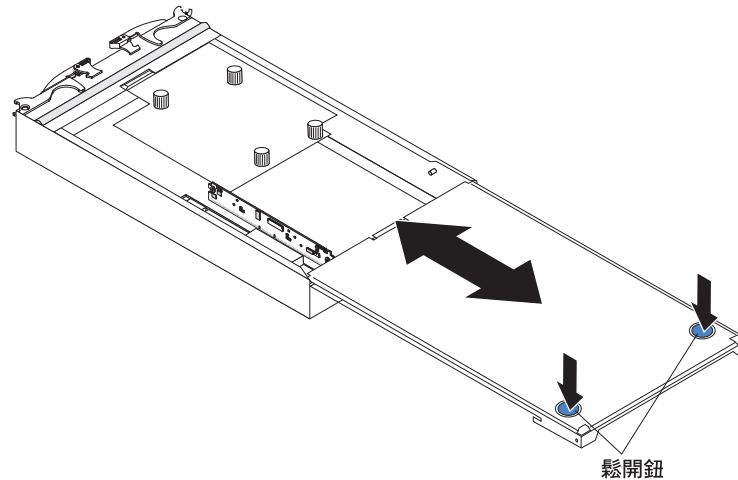
圖 89. 卸下蓋板
