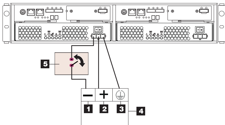
圖 74. 從 DS3500 至中斷連接裝置及 DC 電源的 DC 佈線
