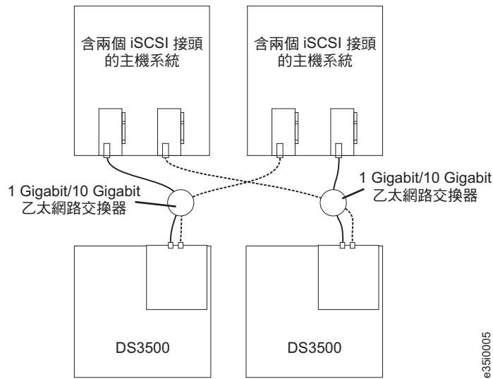
圖 68. 多個主機、多個埠、多個儲存體子系統 iSCSI 配置
