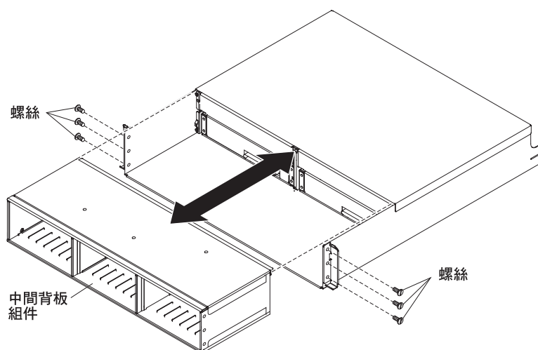
圖 125. 更換 DS3524 或 EXP3524 中的中間背板組件
