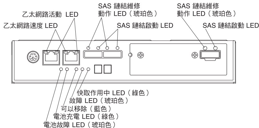
圖 120. 控制器 LED
