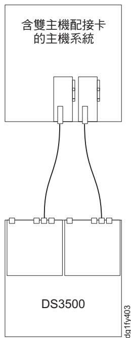
圖 49. 相同主機中兩個 HBA 的雙控制器直接連接型 SAS 連線（備用主機連線）
