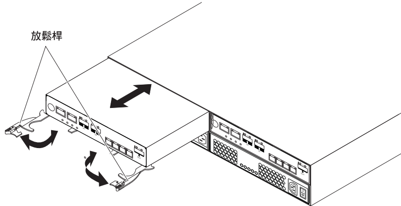
圖 95. 卸下控制器
