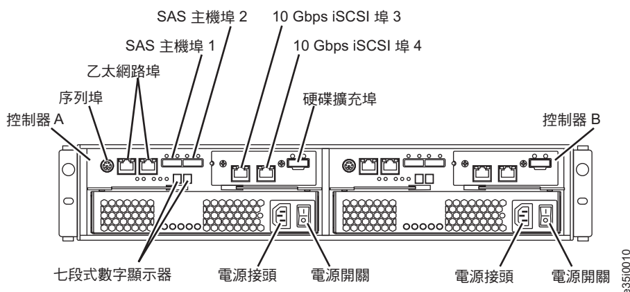
圖 18. 雙控制器 DS3500 儲存體子系統埠及控制器（含選用 10 Gbps iSCSI 主機埠配接卡）
