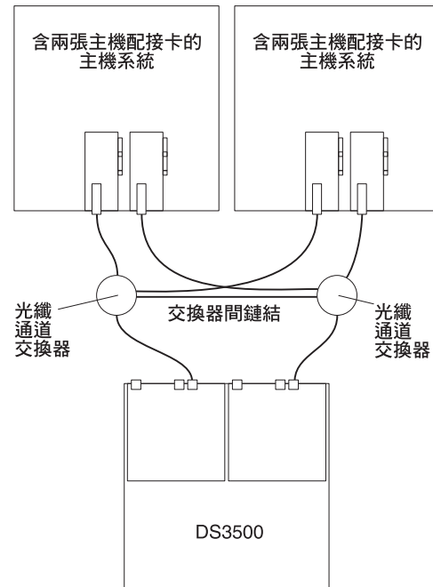
圖 61. 單一「光纖通道」SAN 光纖配置的範例
