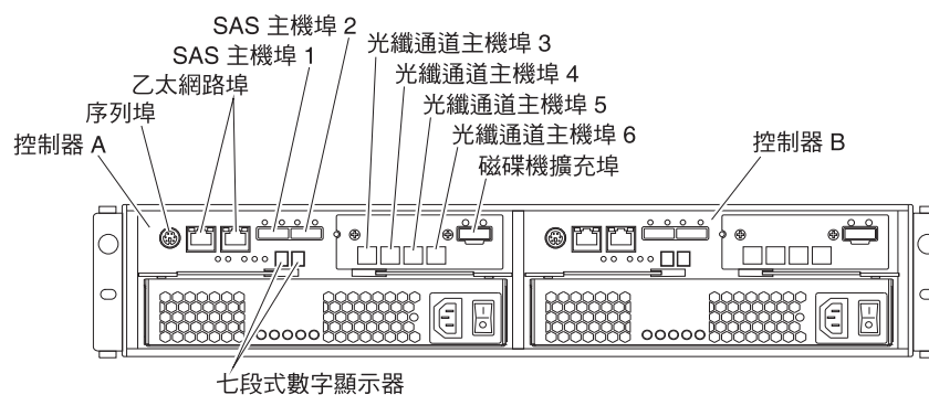
圖 16. 雙控制器 DS3500 儲存體子系統埠及控制器（含選用「光纖通道」主機埠配接卡）
