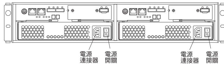
圖 107. DS3500 AC 型號的電源供應器開關及接頭
