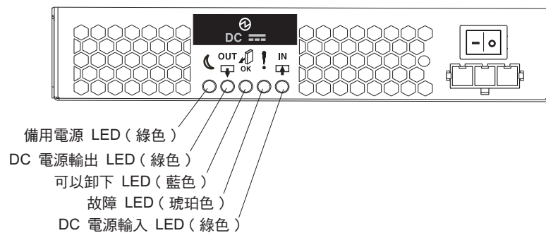
圖 109. DC 電源供應器 LED
