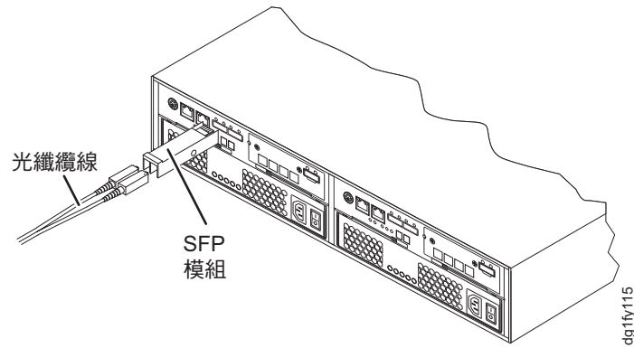
圖 121. 將 SFP 模組安裝至主機埠
