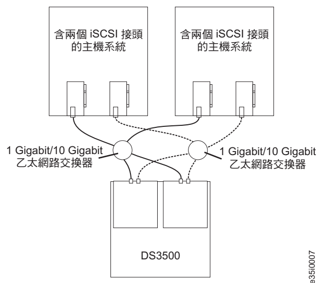
圖 70. 多個主機、多個埠、雙控制器 iSCSI 配置
