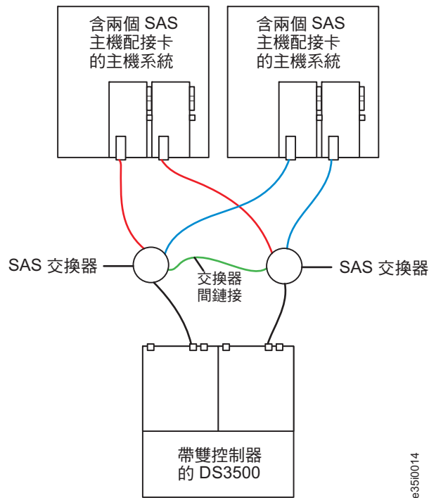
圖 54. 使用透過交換器間鏈結來互連的兩個 SAS 交換器，連接至多部主機的雙控制器 DS3500 SAS 連線
