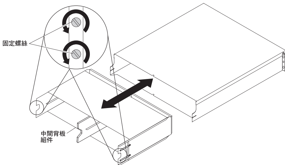
圖 124. 更換 DS3512 或 EXP3512 中的中間背板組件
