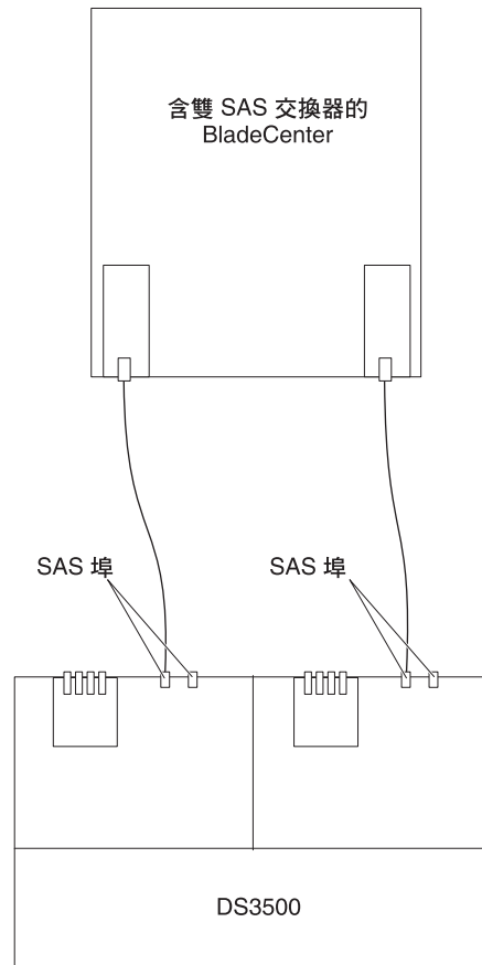
圖 72. 連接到 BladeCenter 裝置的 DS3500 的範例
