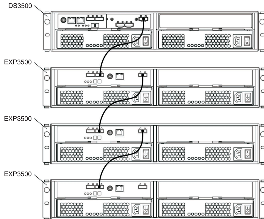
圖 39. 一個單控制器 DS3500 及多個單一 ESM 儲存體機體
