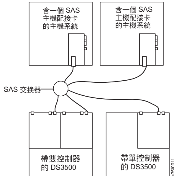
圖 51. 使用一個 SAS 交換器連接至多部主機的雙控制器 DS3500 或單控制器 DS3500 SAS 連線
