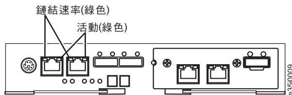
圖 85. 10 Gbps iSCSI 埠 LED
