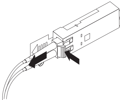
圖 31. 拔掉「LC-LC 光纖通道」纜線
