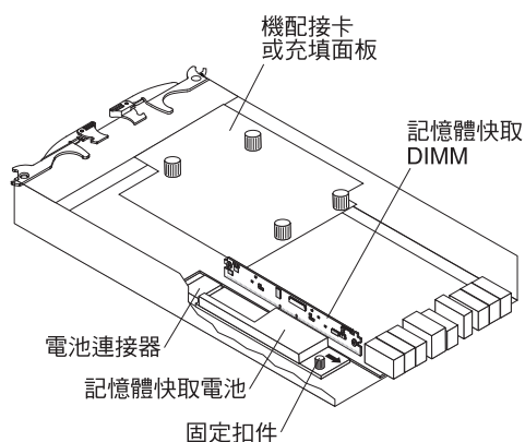
圖 115. 記憶體快取 DIMM 位置
