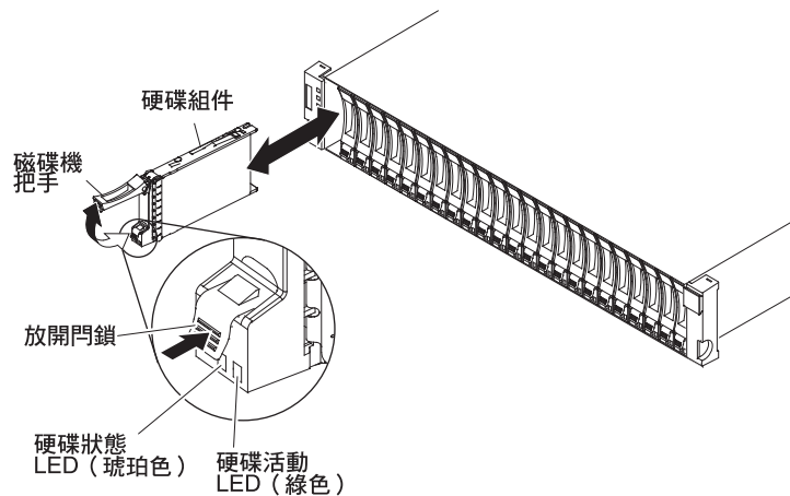
圖 103. 在 DS3524 或 EXP3524 中安裝硬碟
