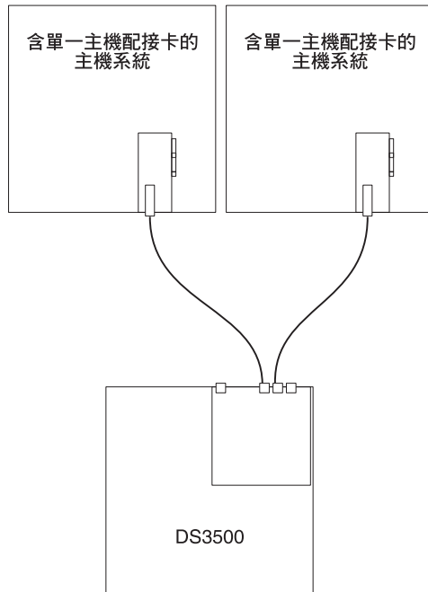
圖 48. 多個主機中單一 HBA 的單控制器直接連接型 SAS 連線
