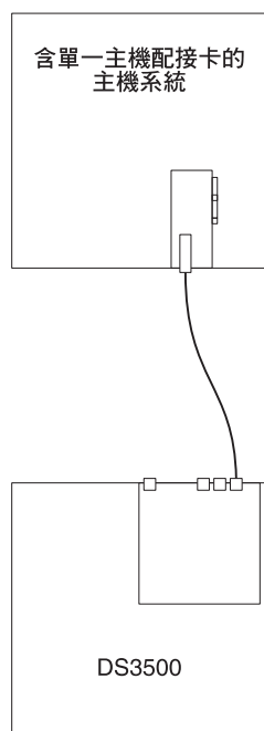
圖 46. 單一主機 HBA 的單控制器直接連接型 SAS 連線
