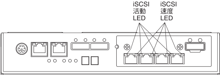
圖 82. iSCSI 主機埠配接卡 LED
