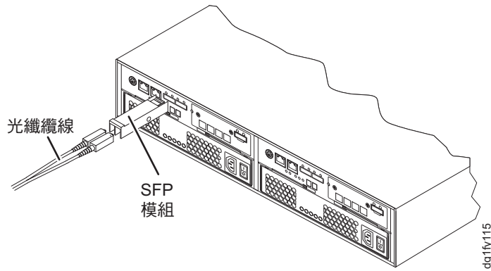
圖 24. 將 SFP 模組安裝至主機埠
