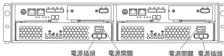
圖 76. DS3500 DC 型號的電源供應器開關及接頭
