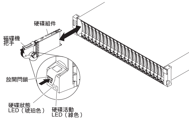
圖 101. 從 DS3524 或 EXP3524 卸下硬碟
