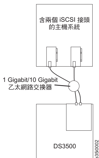
圖 65. 多個埠、單控制器 iSCSI 配置
