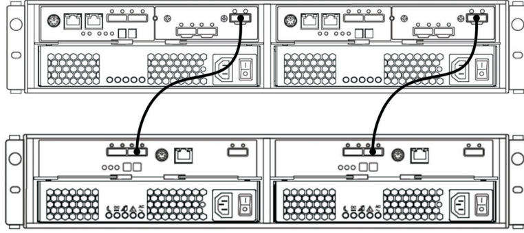
圖 40. 一個雙控制器 DS3500 及一個 儲存體機體
