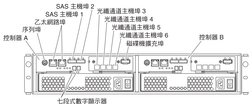
圖 55. 儲存體控制器上的主機接頭位置
