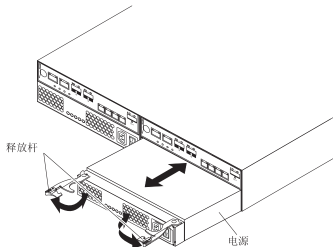
图 104. 更换电源
