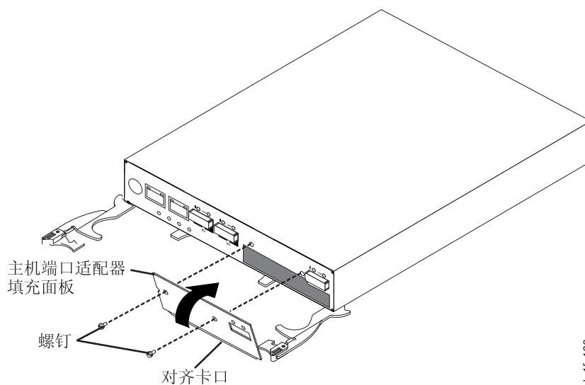
图 96. 卸下主机端口适配器填充面板
