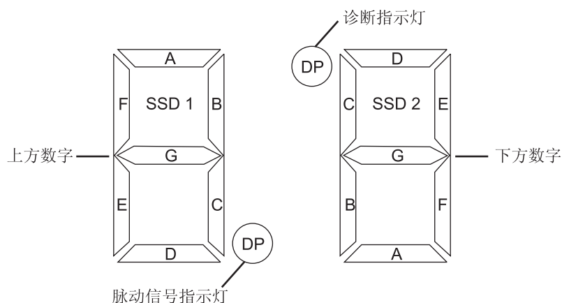
图 86. 数字显示屏指示灯
