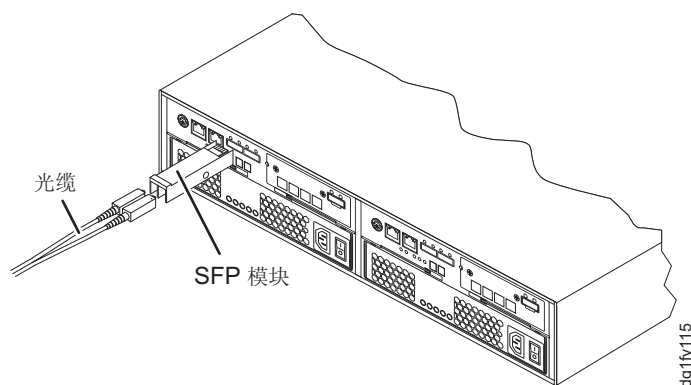
图 24. 将 SFP 模块安装到主机端口中
