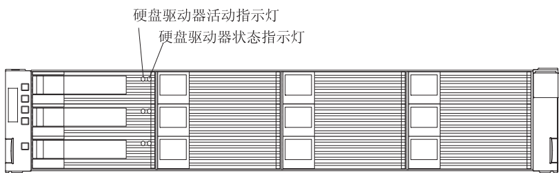
图 98. DS3512 存储子系统和 EXP3512 存储机柜驱动器指示灯
