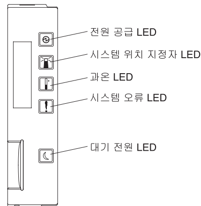
그림 4. 왼쪽 베젤
