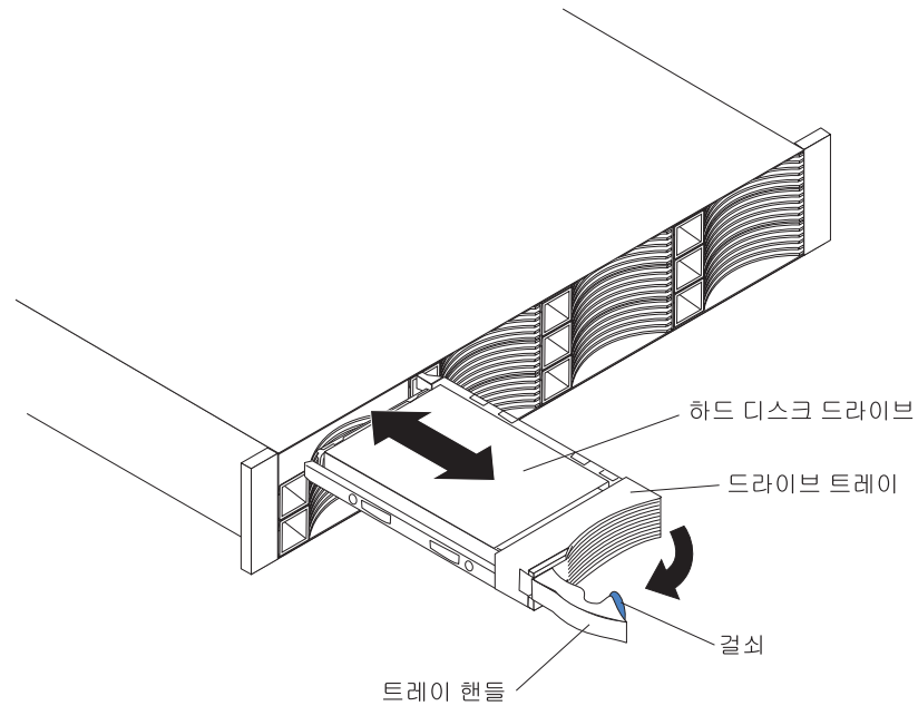
그림 100. DS3512 또는 EXP3512에서 드라이브 제거
