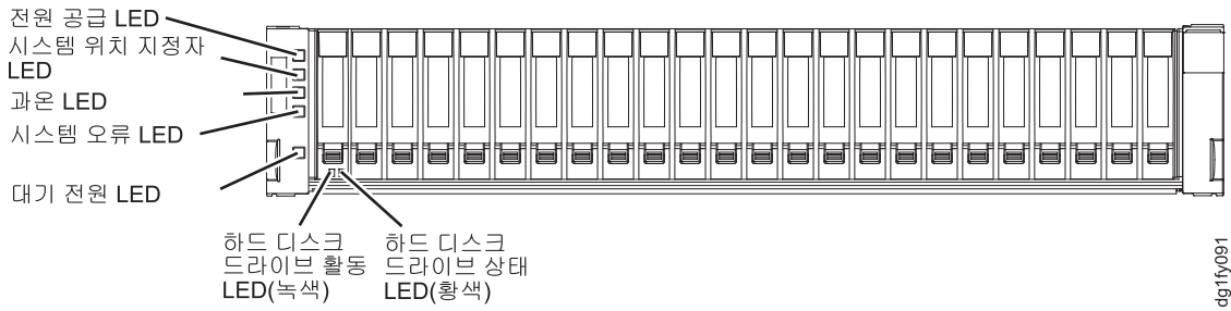
그림 80. DS3524 스토리지 서브시스템 및 EXP3524 스토리지 격납장치 앞면 LED
