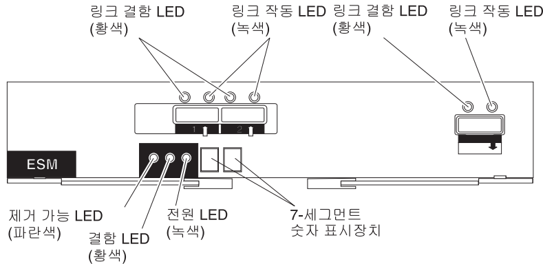
그림 87. ESM LED
