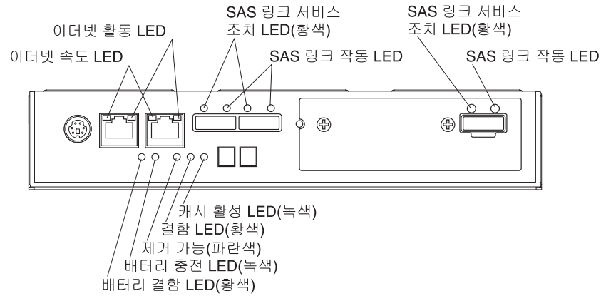
그림 81. 제어기 LED
