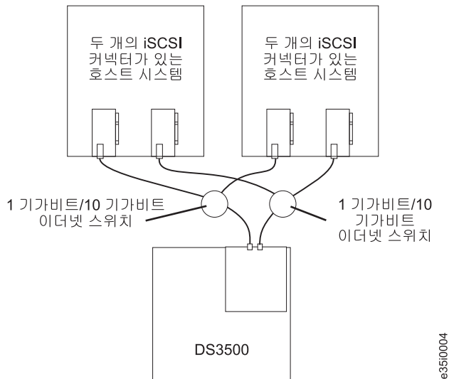
그림 67. 다중 호스트, 다중 포트, 단일 제어기 및 중복 경로 iSCSI 구성
