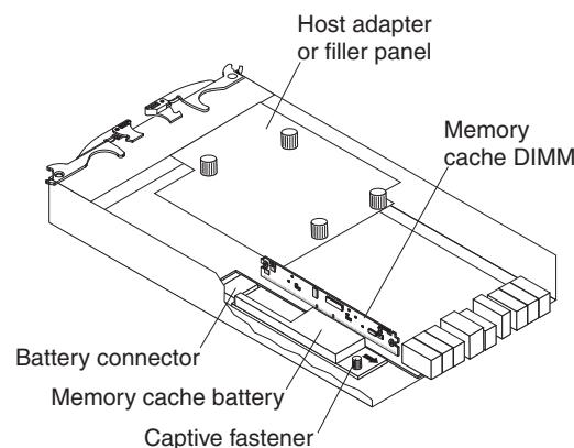
그림 115. 메모리 캐시 DIMM 위치
