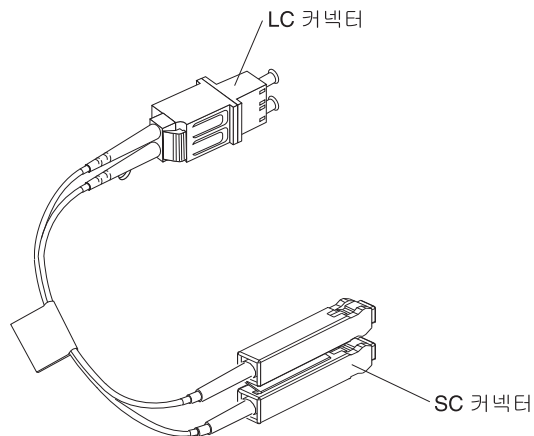
그림 32. LC-SC 파이버 채널 케이블 어댑터
