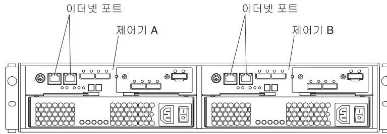
그림 43. 듀얼 제어기 DS3500의 이더넷 포트 위치
