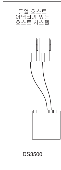
그림 47. 단일 호스트의 듀얼 HBA에 대한 단일 제어기의 직접 연결된 SAS 연결(중복 호스트 연결)
