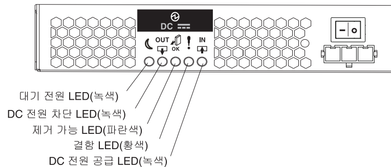
그림 109. DC 전원 공급 장치 LED
