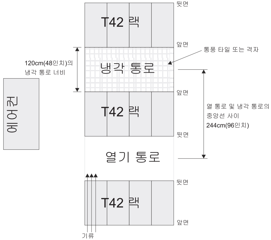
그림 15. 냉각 통로/열 통로 랙 구성 예
