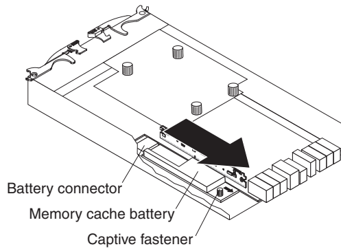
그림 114. 제어기에서 배터리 장치 제거
