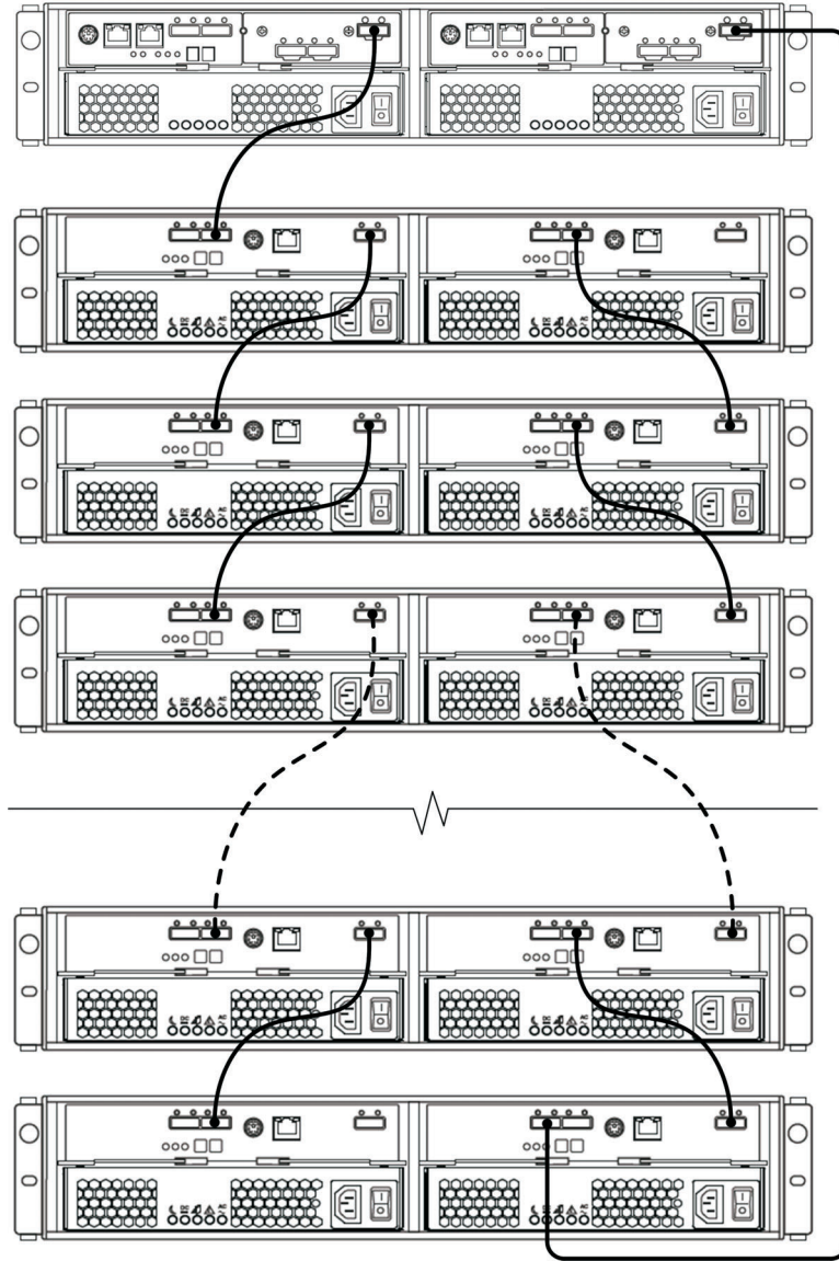
그림 45. 직접(아웃오브밴드) 관리 스토리지 서브시스템
