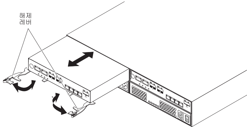
그림 116. 제어기 제거
