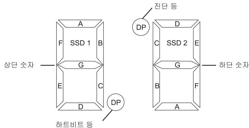
그림 86. 숫자 표시 LED
