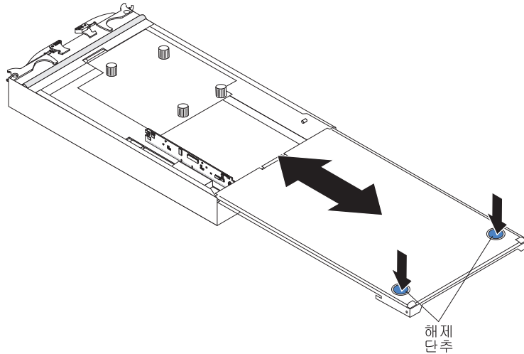
그림 89. 덮개 제거
