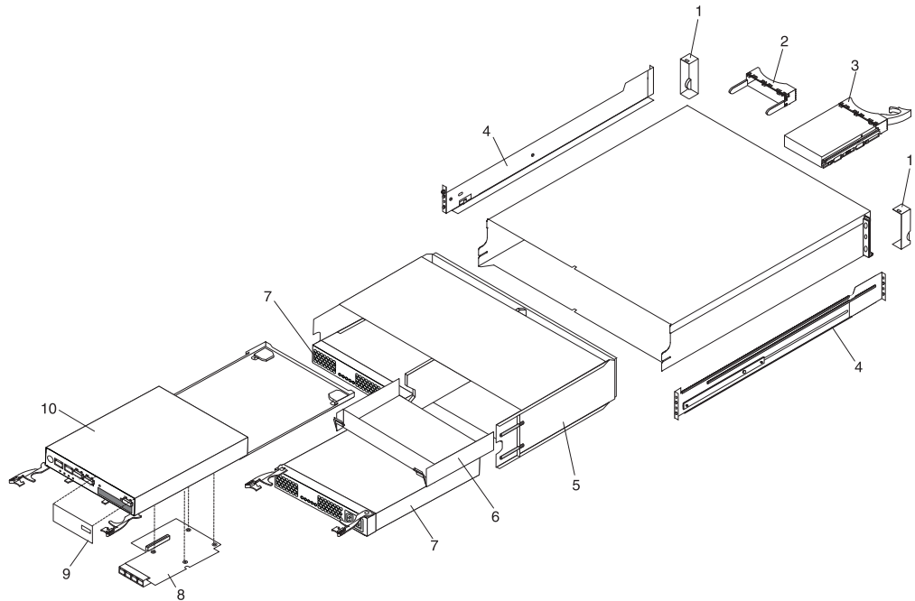
그림 127. DS3512 스토리지 서브시스템 및 EXP3512 스토리지 격납장치 스토리지 서브시스템 부품
