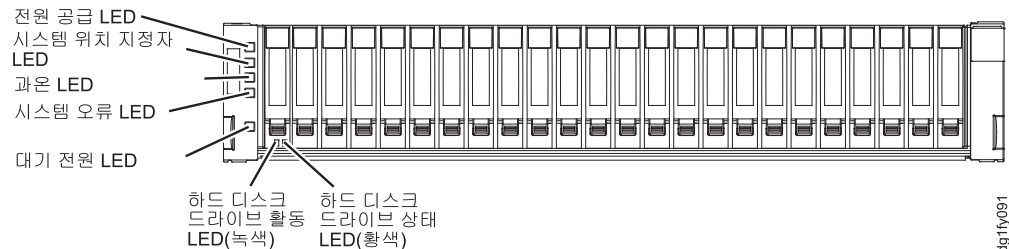
그림 119. DS3524 스토리지 서브시스템 및 EXP3524 스토리지 격납장치 전면 LED
