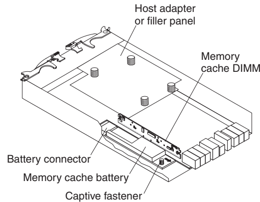
그림 12. 배터리 장치
