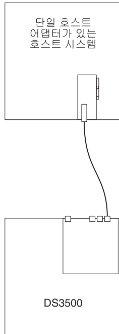
그림 56. 단일 호스트 HBA에 대한 단일 제어기의 직접 연결된 파이버 채널 연결
