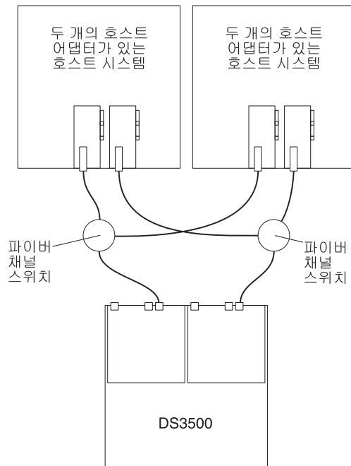
그림 62. 듀얼 파이버 채널 SAN 패브릭 구성 예제
