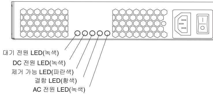
그림 77. AC 전원 공급 장치 LED
