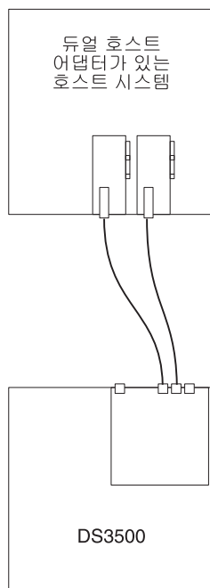
그림 57. 듀얼 HBA에 대한 단일 제어기의 직접 연결된 파이버 채널 연결(중복 호스트 연결)
