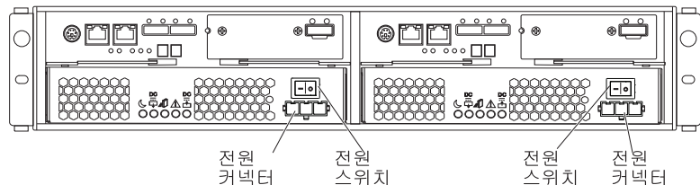
그림 76. DS3500 DC 모델의 전원 공급 장치 스위치 및 커넥터
