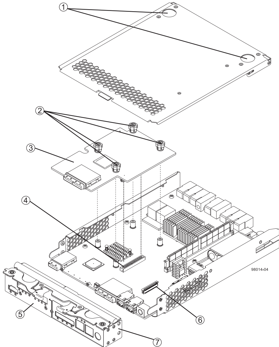
그림 94. 제어기 구성요소 제거 순서
