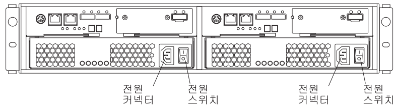
그림 107. DS3500 AC 모델의 전원 공급 장치 스위치 및 커넥터
