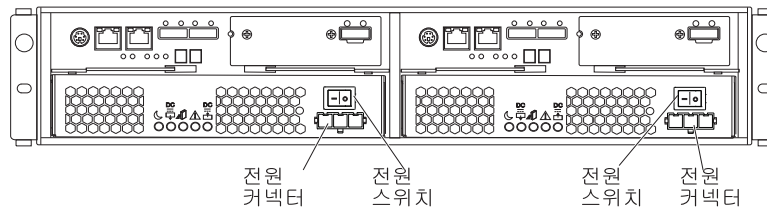
그림 111. DS3500 DC 모델의 전원 공급 장치 스위치 및 커넥터
