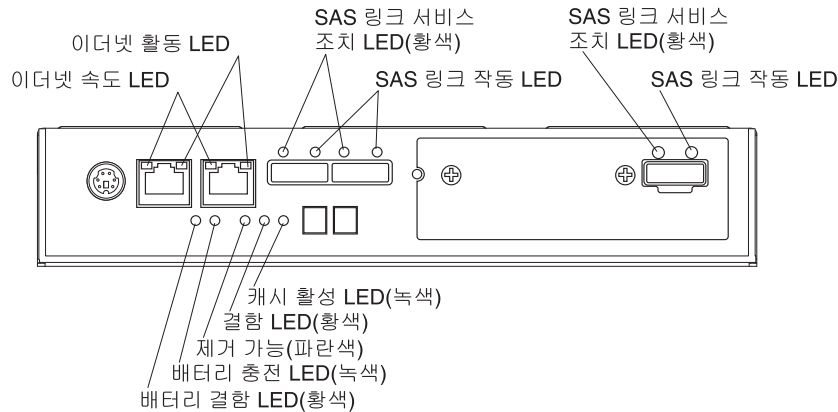
그림 120. 제어기 LED
