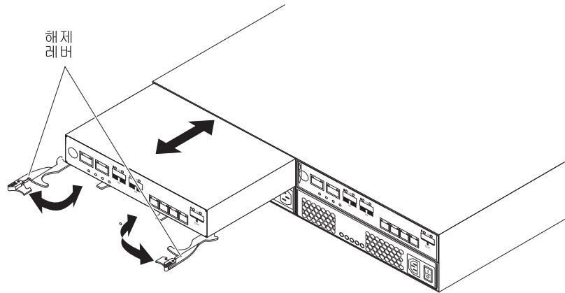
그림 95. 제어기 제거
