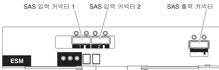
그림 37. ESM 커넥터
