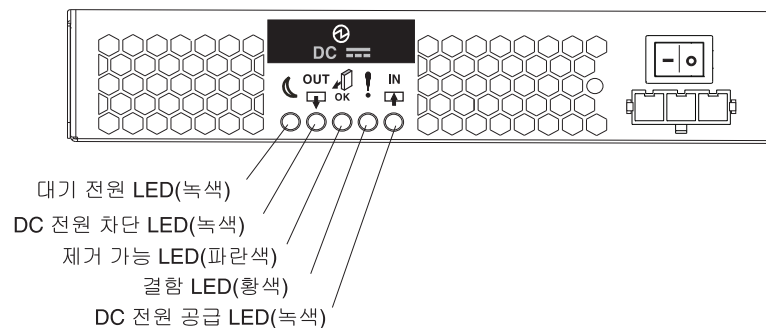
그림 78. DC 전원 공급 장치 LED
