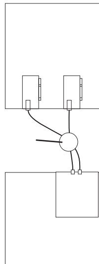
그림 65. 다중 포트, 단일 제어기 iSCSI 구성
