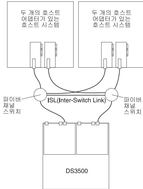
그림 61. 단일 파이버 채널 SAN 패브릭 구성 예제
