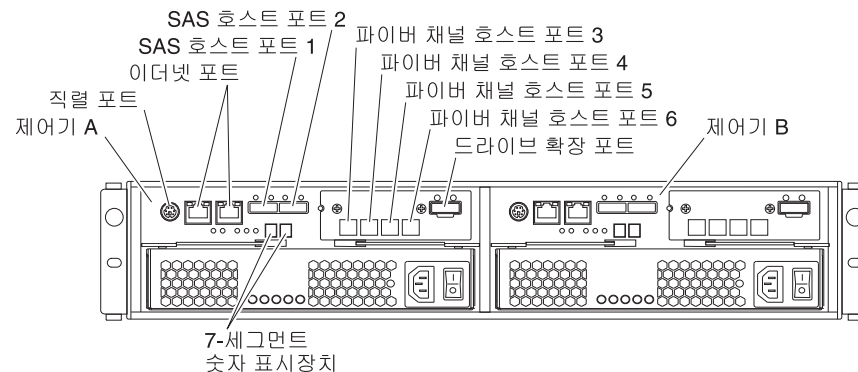
그림 16. 듀얼 제어기 DS3500 스토리지 서브시스템 포트 및 제어기(선택적 파이버 채널 호스트 포트 어댑터 포함)
