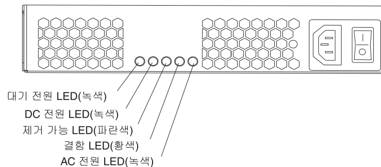
그림 106. AC 전원 공급 장치 LED
