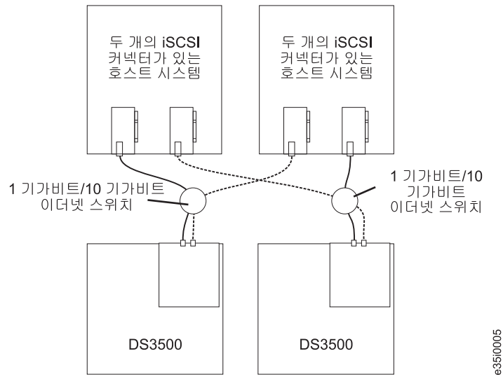
그림 68. 다중 호스트, 다중 포트, 다중 스토리지 서브시스템 iSCSI 구성
