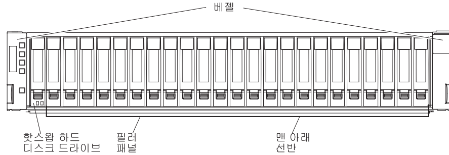
그림 3. DS3524 스토리지 서브시스템 및 EXP3524 스토리지 격납장치 핫스왑 드라이브 베이 및 베젤
