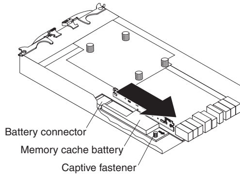
그림 92. 제어기에서 배터리 장치 제거
