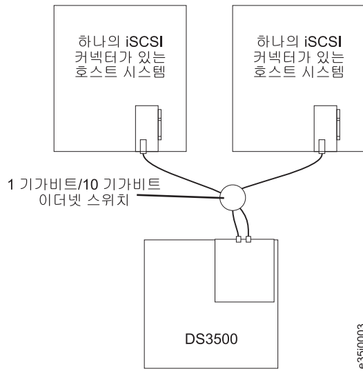
그림 66. 여러 단일 포트 호스트, 단일 제어기 iSCSI 구성
