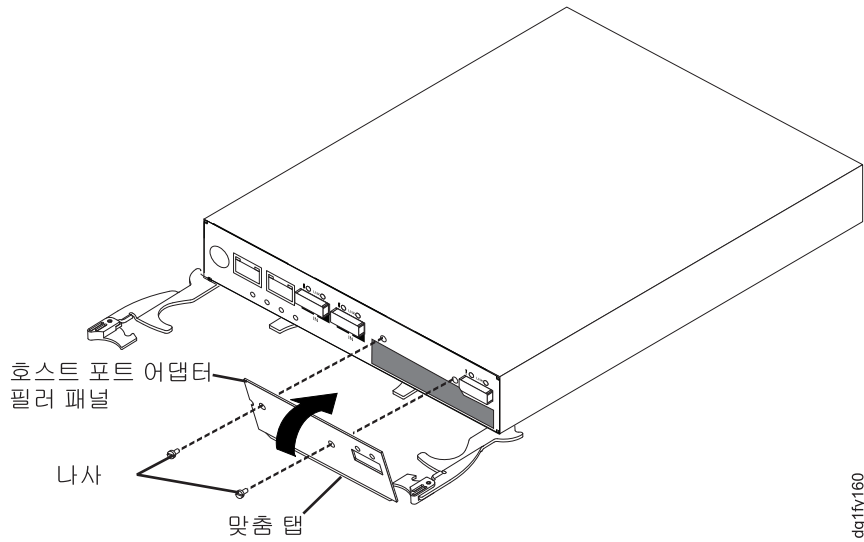
그림 96. 호스트 포트 어댑터 필터 패널 제거
