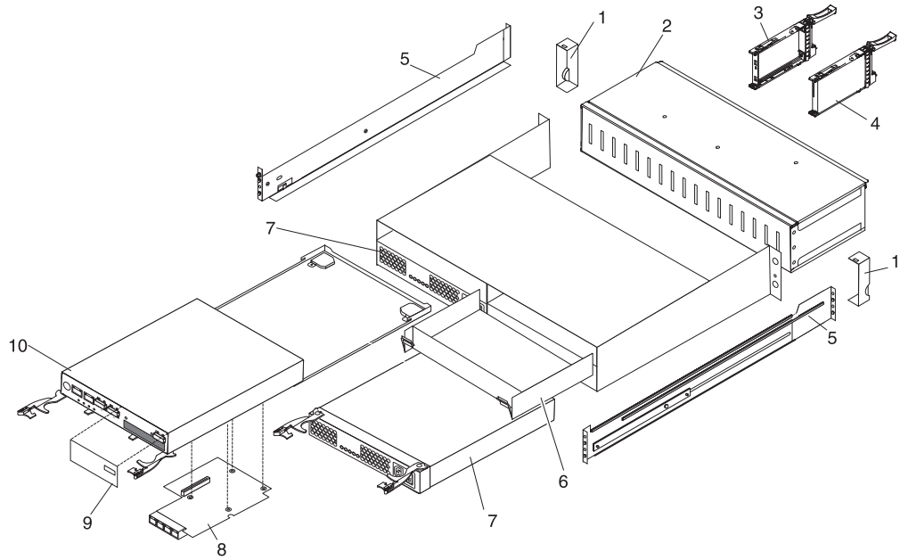
그림 128. DS3524 스토리지 서브시스템 및 EXP3524 스토리지 격납장치 부품
