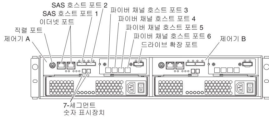
그림 55. 스토리지 제어기에서 호스트 커넥터의 위치
