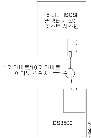
그림 64. 단일 호스트, 단일 제어기 iSCSI 구성
