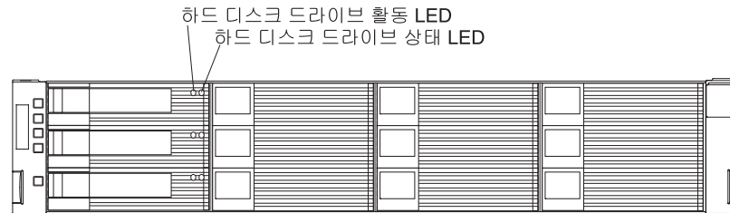
그림 98. DS3512 스토리지 서브시스템 및 EXP3512 스토리지 격납장치 드라이브 LED
