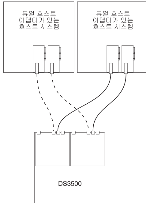
그림 50. 여러 호스트의 다중 HBA에 대한 듀얼 제어기의 직접 연결된 SAS 연결
