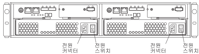
그림 9. AC 전원 공급 장치 구성요소
