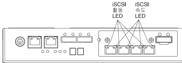
그림 82. iSCSI 호스트 포트 어댑터 LED
