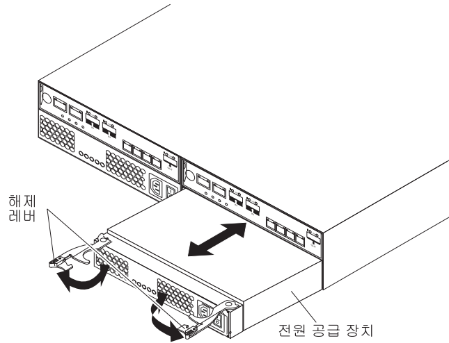
그림 105. 전원 공급 장치 교체
