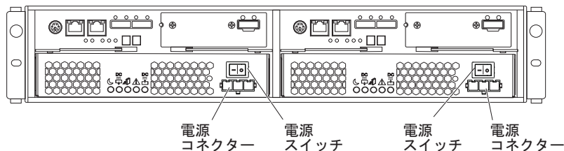
図 111. DS3500 DC モデルの電源機構のスイッチとコネクタ
