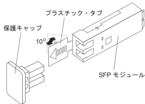
図 25. SFP モジュール・ラッチのアンロック - プラスチック・タブの場合
