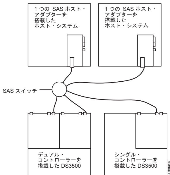
図 51. 1 つの SAS スイッチを使用した複数のホストへのデュアル・コントローラー DS3500 またはシングル・コントローラー DS3500 の SAS 接続
