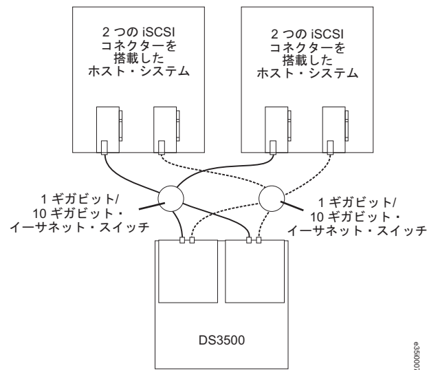
図 70. 複数ホスト、複数ポート、デュアル・コントローラー iSCSI 構成
