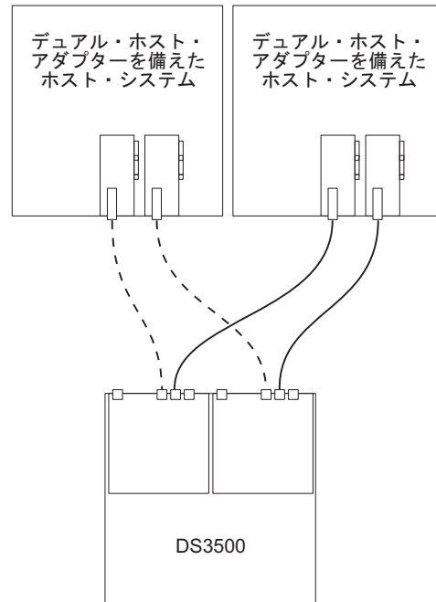
図 50. 複数のホスト内の複数の HBA へのデュアル・コントローラー直接 SAS 接続による接続
