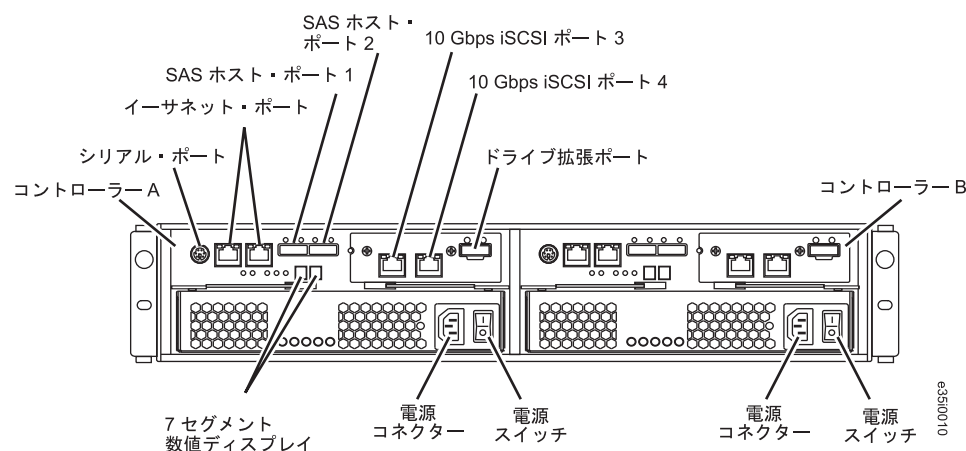
図 18. デュアル・コントローラー DS3500 ストレージ・サブシステムのポートとコントローラー (オプションの 10 Gbps iSCSI ホスト・ポート・アダプターを装備)
