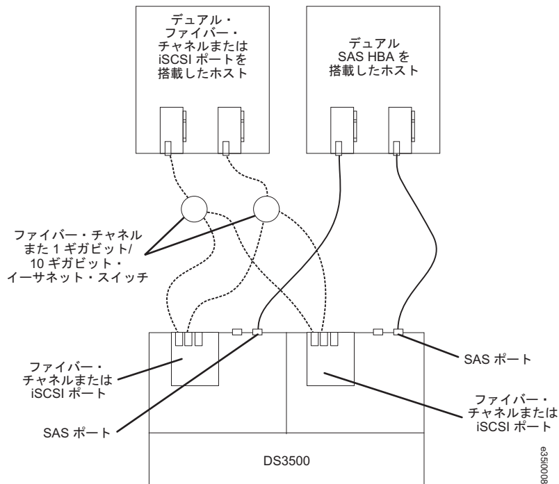
図 71. 複数ホスト、複数ポート、および複数ファブリック (ファイバー・チャネルまたは iSCSI、および SAS) 構成の例
