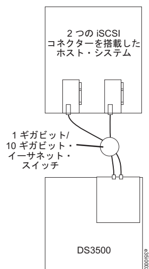
図 65. 複数ポート、シングル・コントローラー iSCSI 構成
