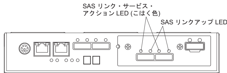
図 84. SAS ホスト・ポート・アダプター LED
