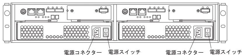
図 75. DS3500 AC モデルの電源機構のスイッチとコネクタ
