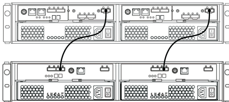
図 40. デュアル・コントローラー DS3500 とストレージ・エンクロージャー
