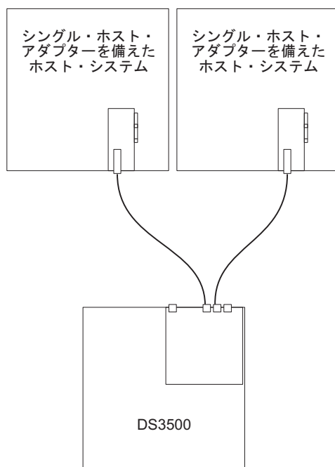
図 48. 複数のホスト内のシングル HBA へのシングル・コントローラー直接 SAS 接続による接続
