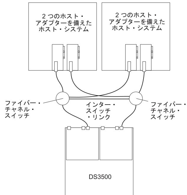
図 61. 単一ファイバー・チャンネル SAN ファブリック構成の例
