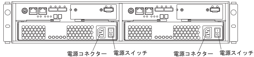
図 107. DS3500 AC モデルの電源機構のスイッチとコネクタ
