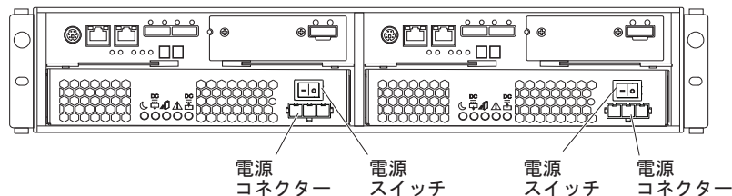
図 76. DS3500 DC モデルの電源機構のスイッチとコネクタ
