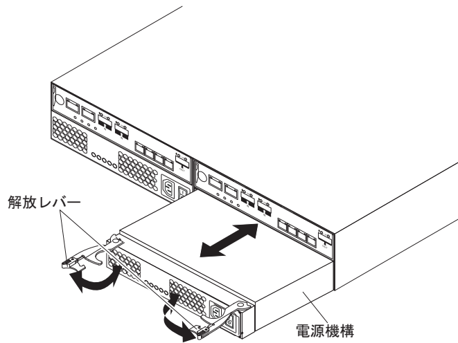
図 105. 電源機構の交換
