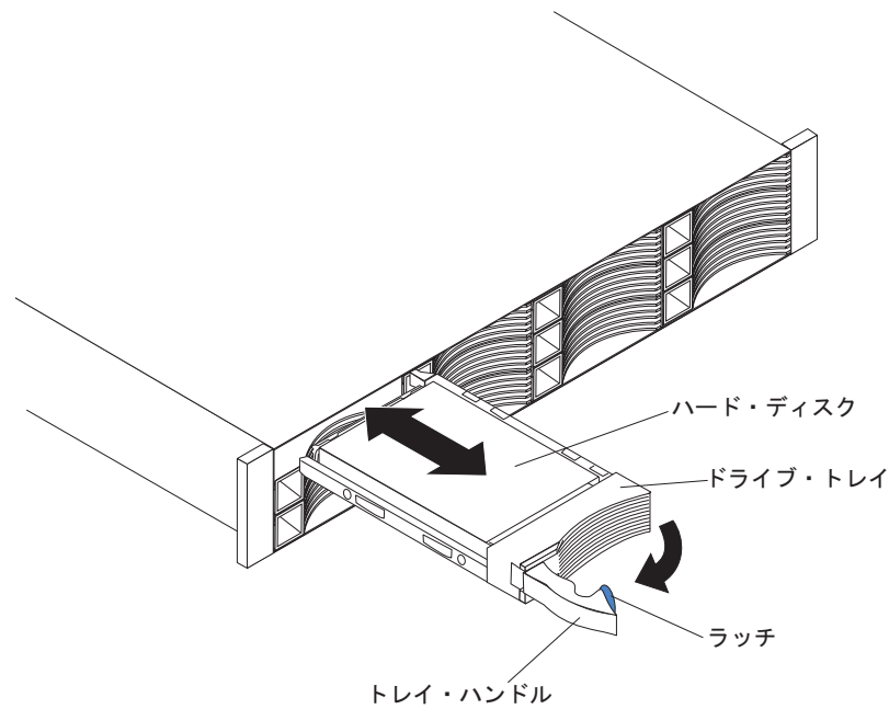
図 102. DS3512 または EXP3512 へのドライブの取り付け
