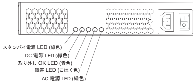
図 106. AC 電源機構 LED
