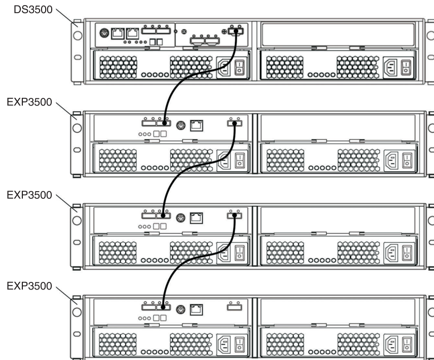
図 39. 1 つのシングル・コントローラー DS3500 と複数のシングル ESM ストレージ・エンクロージャー
