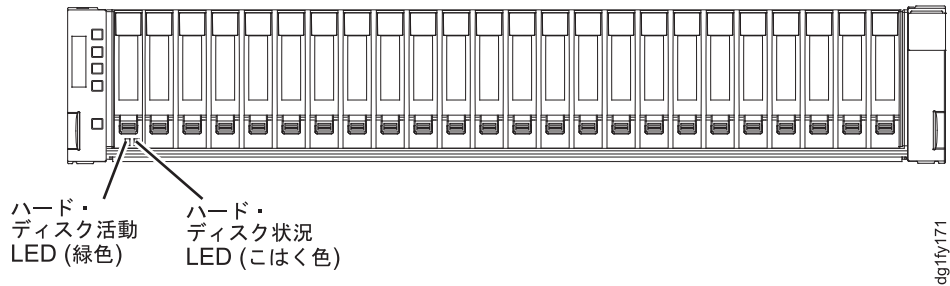
図 99. DS3524 ストレージ・サブシステムおよび EXP3524 ストレージ・エンクロージャー・ドライブ LED
