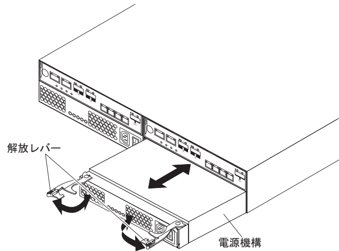
図 112. 電源機構の交換
