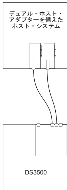
図 57. デュアル HBA へのシングル・コントローラー直接ファイバー・チャンネル接続による接続 (冗長ホスト接続)
