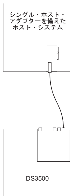
図 46. シングル・ホスト HBA とのシングル・コントローラー直接 SAS 接続
