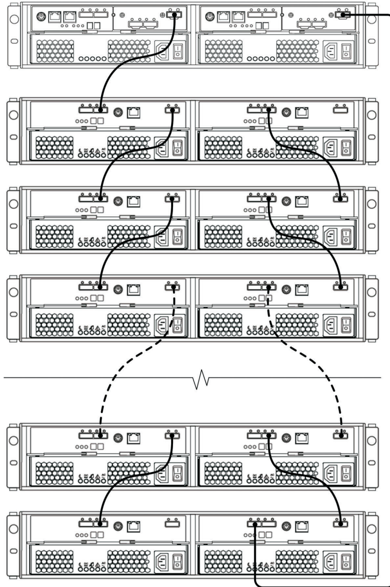
図45. 直接 (アウト・オブ・バンド) 管理ストレージ・サブシステム
