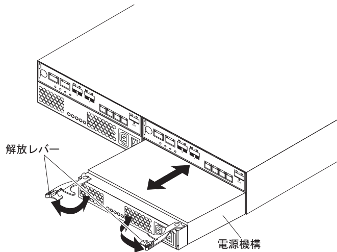
図 104. 電源機構の交換
