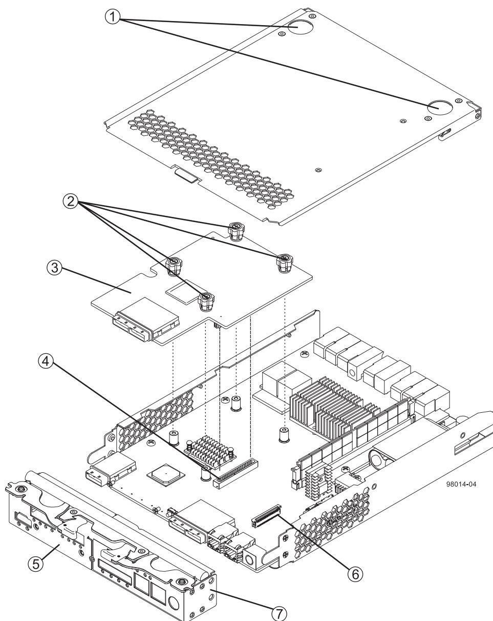
図 94. コントローラー・コンポーネントの取り外し手順
