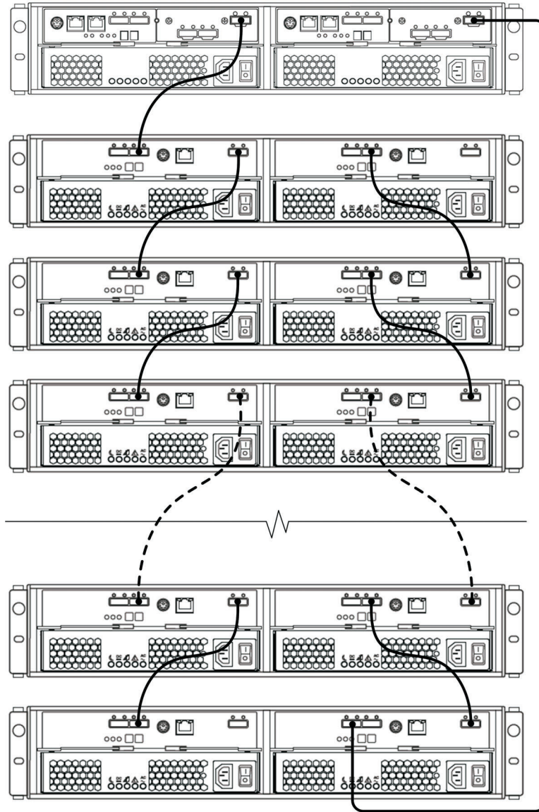
図42. デュアル・コントローラー DS3500 と 8 つのストレージ・エンクロージャー
