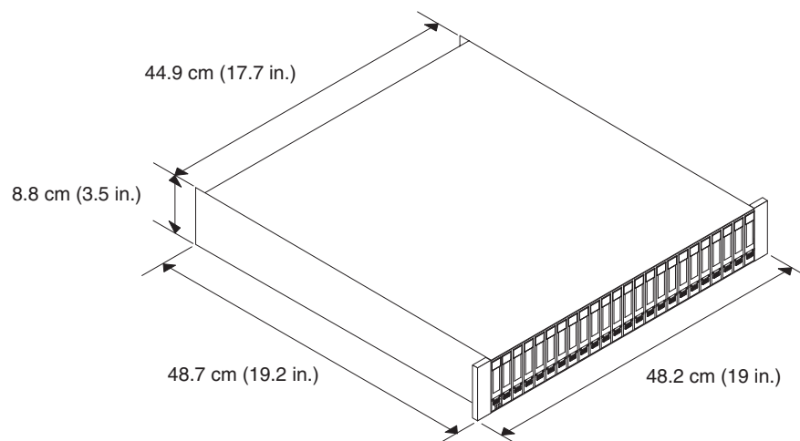
図 14. DS3524 ストレージ・サブシステムおよび EXP3524 ストレージ・エンクロージャーの寸法
