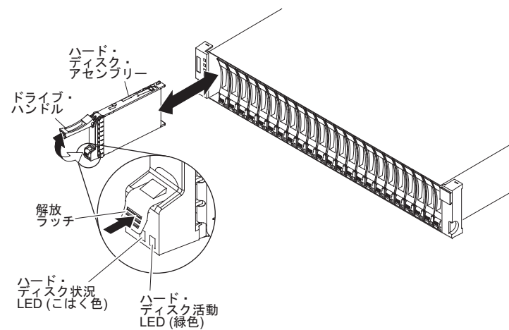
図 101. DS3524 または EXP3524 からのドライブの取り外し
