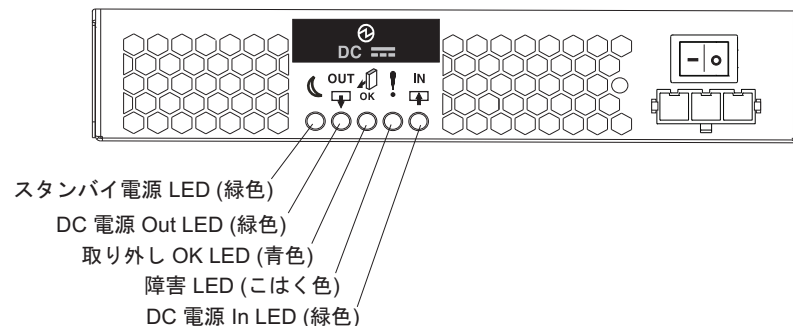
図 109. DC 電源機構 LED
