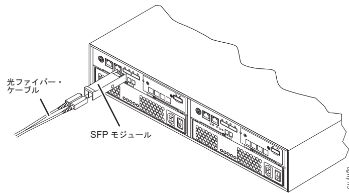
図 121. SFP モジュールのホスト・ポートへの取り付け
