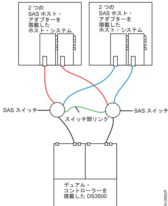
図 54. インターリンク・スイッチを介して一緒に接続された 2 つの SAS スイッチを使用した複数のホストへのデュアル・コントローラー DS3500 の SAS 接続
