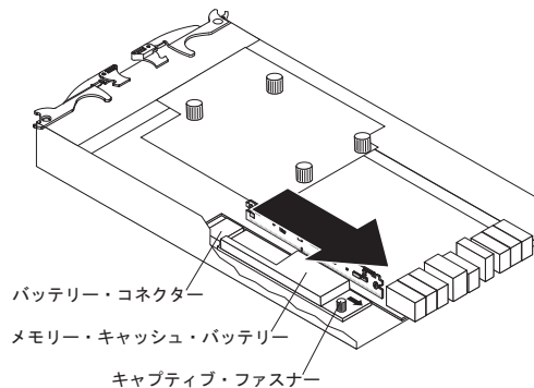
図 92. コントローラーからのバッテリー・ユニットの取り外し
