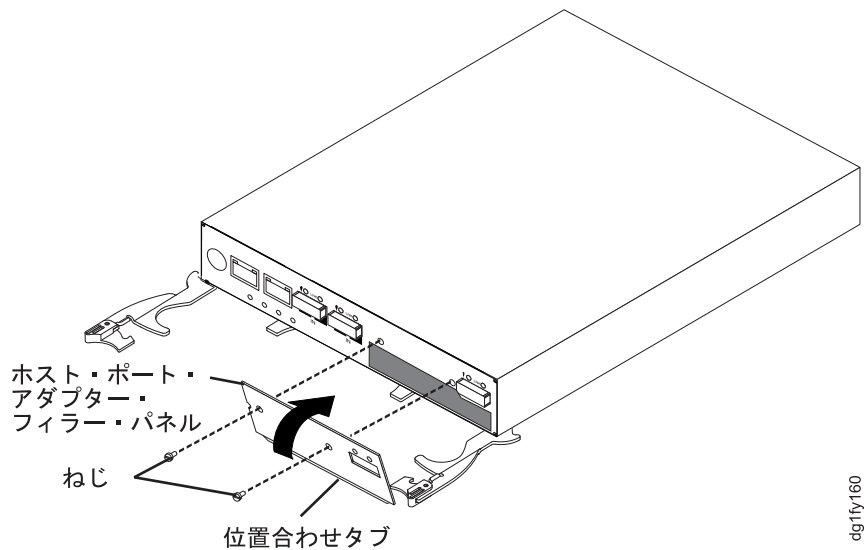
図 96. ホスト・ポート・アダプター・フィルラー・パネルの取り外し
