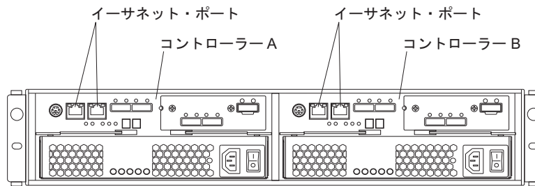
図 43. デュアル・コントローラー DS3500 上のイーサネット・ポートの位置
