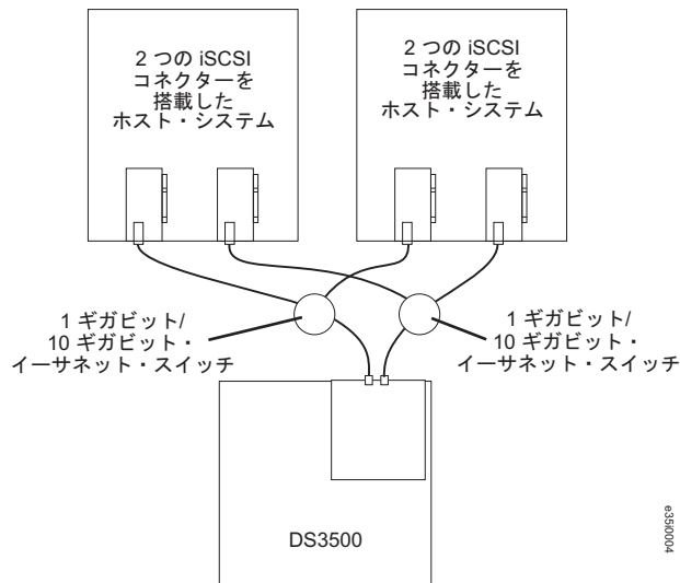
図 67. 複数ホスト、複数ポート、シングル・コントローラー、および冗長パス iSCSI 構成
