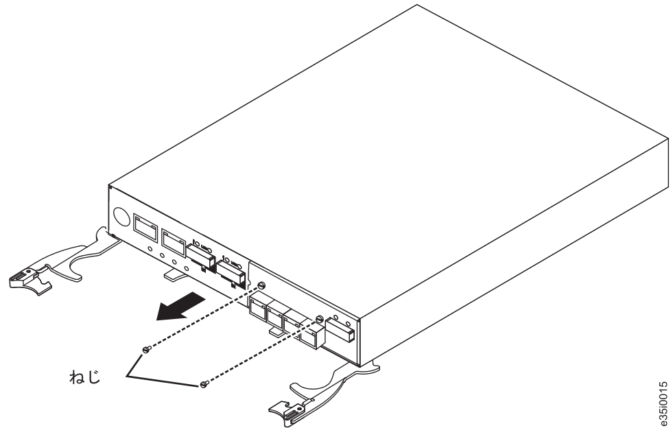
図 97. ホスト・ポート・アダプターの取り付け
