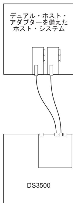
図 47. シングル・ホスト内のデュアル HBA とのシングル・コントローラー直接 SAS 接続 (冗長ホスト接続)
