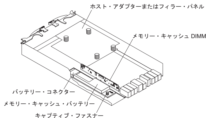
図 12. バッテリー・ユニット
