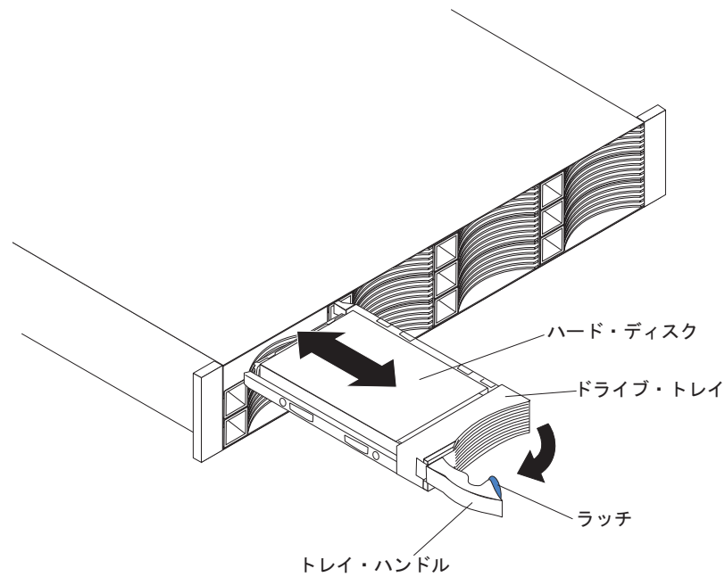
図 100. DS3512 または EXP3512 からのドライブの取り外し
