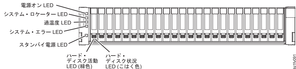
図 119. DS3524 ストレージ・サブシステムおよび EXP3524 ストレージ・エンクロージャーの前面 LED
