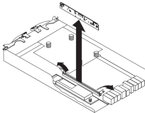
図 118. コントローラーへの DIMM のインストール
