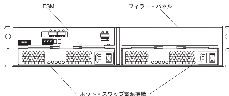
図 8. 背面図、シングル ESM モデル・ストレージ・エンクロージャー
