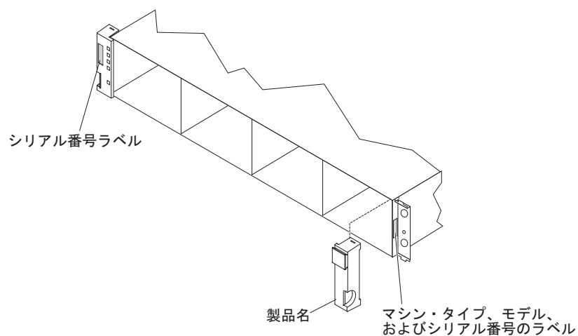
図 130. DS3500 のシリアル番号の位置
