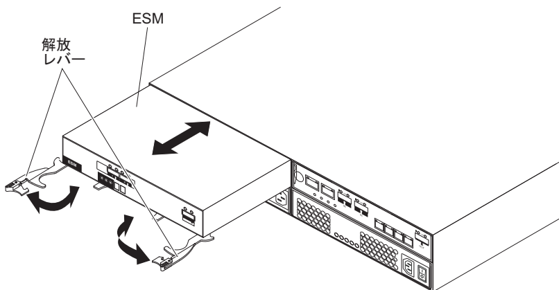
図 123. 環境サービス・モジュールの取り外し
