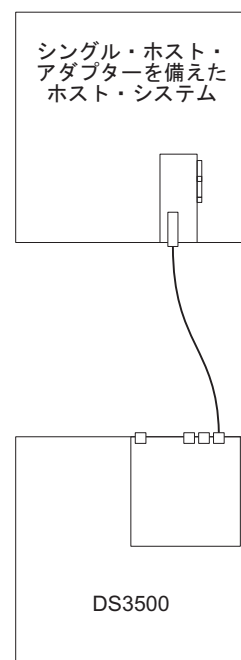
図 56. シングル・ホスト HBA へのシングル・コントローラー直接ファイバー・チャネル接続による接続
