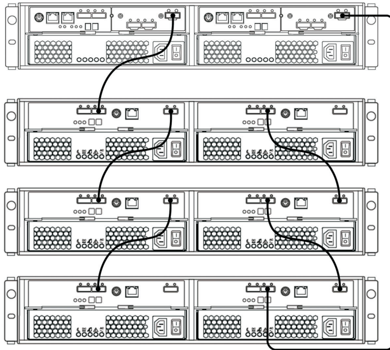
図 38. 冗長ドライブ・パスの例
