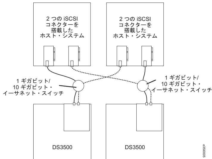
図 68. 複数ホスト、複数ポート、複数ストレージ・サブシステム iSCSI 構成
