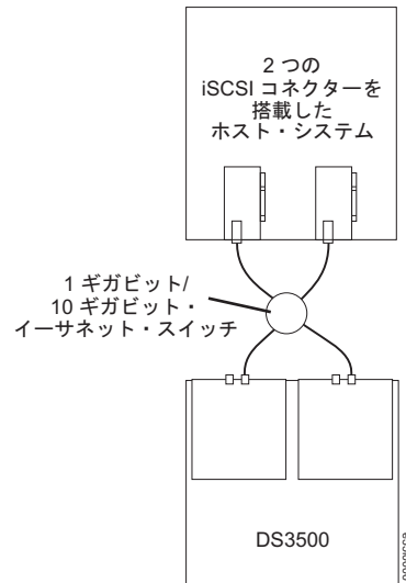
図 69. 単一ホスト、複数ポート、デュアル・コントローラー iSCSI 構成
