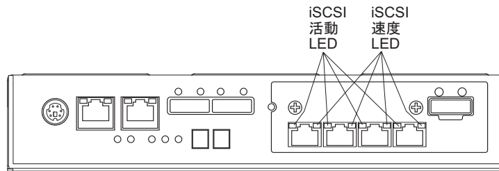
図 82. iSCSI ホスト・ポート・アダプター LED
