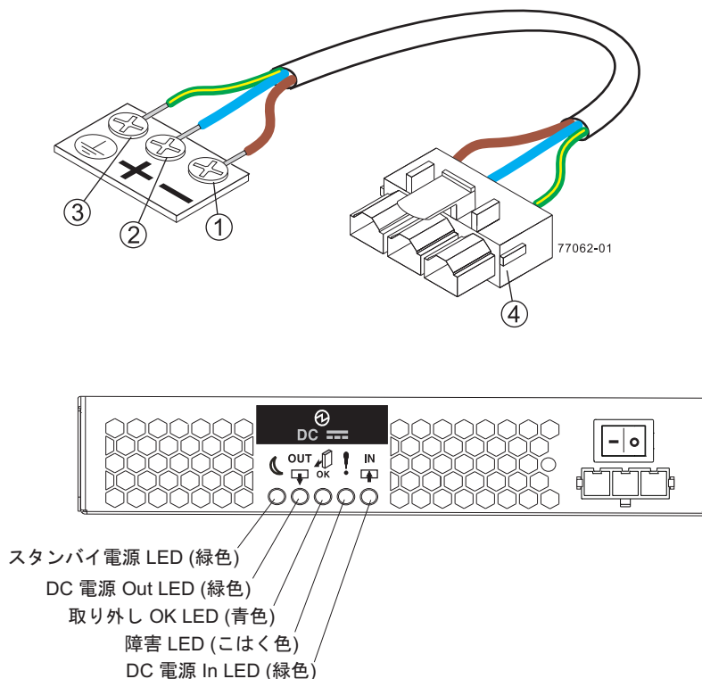
図 110. DS3500 DC モデルの DC 電源コネクタ
