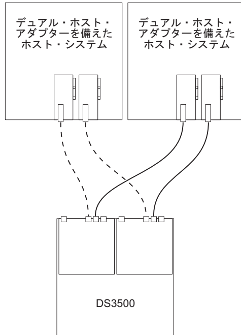
図 60. 複数のホスト内の複数の HBA へのデュアル・コントローラー直接ファイバー・チャンネル接続による接続
