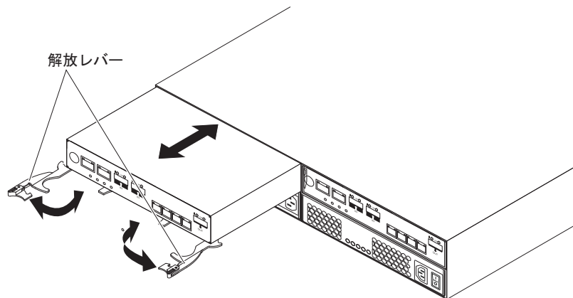
図 113. コントローラーの取り外し
