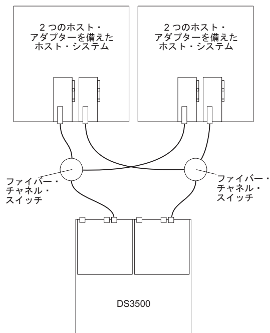
図 62. 二重ファイバー・チャンネル SAN ファブリック構成の例
