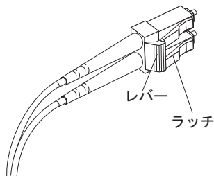
図 35. LC-LC ファイバー・チャンネル・ケーブルのレバーおよびラッチ
