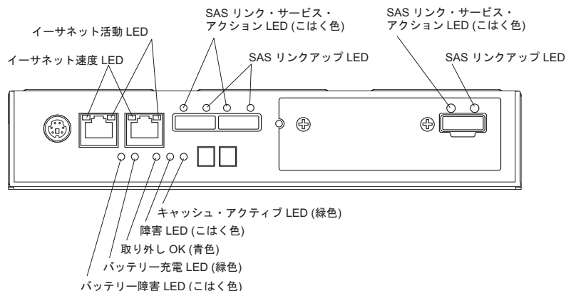
図 81. コントローラー LED
