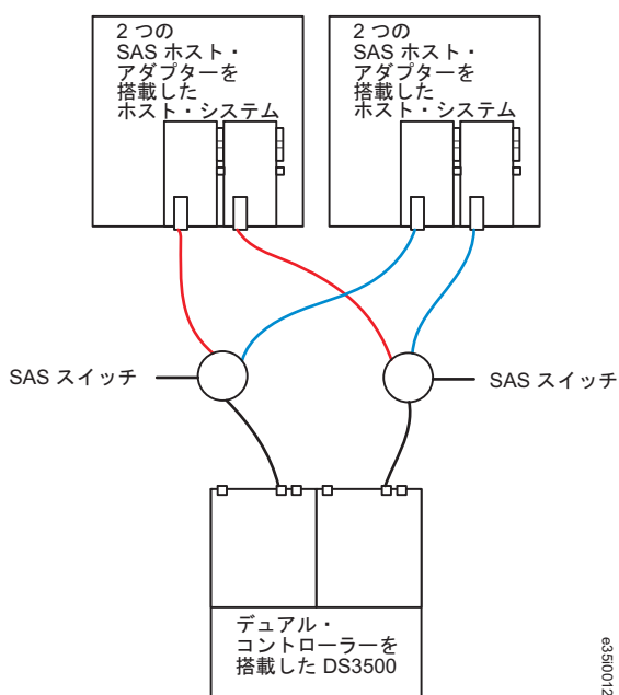
図 52. 2 つの独立した SAS スイッチを使用した複数のホストへのデュアル・コントローラー DS3500 の SAS 接続
