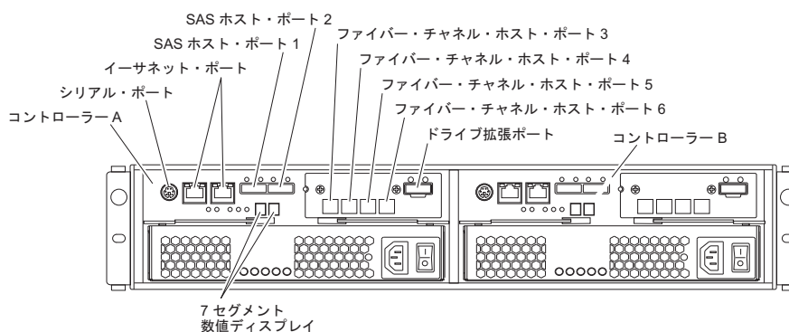
図 16. デュアル・コントローラー DS3500 ストレージ・サブシステムのポートとコントローラー (オプションのファイバー・チャネル・ホスト・ポート・アダプターを装備)
