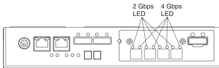
図 83. ファイバー・チャネル・ホスト・ポート・アダプター LED
