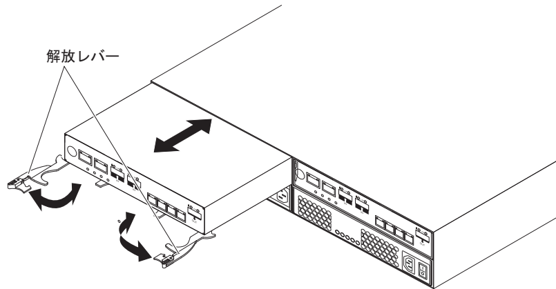
図 95. コントローラーの取り外し
