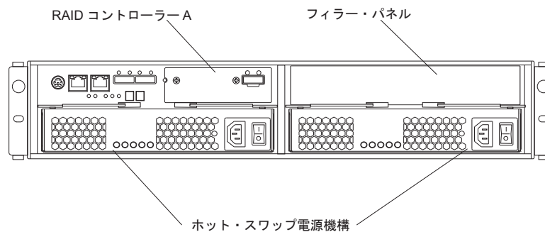
図 7. 背面図、シングル・コントローラー・モデル (オプションのホスト・ポート・アダプターなしで表示)
