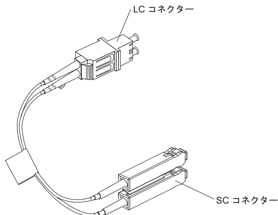
図 32. LC-SC ファイバー・チャネル・ケーブル・アダプター
