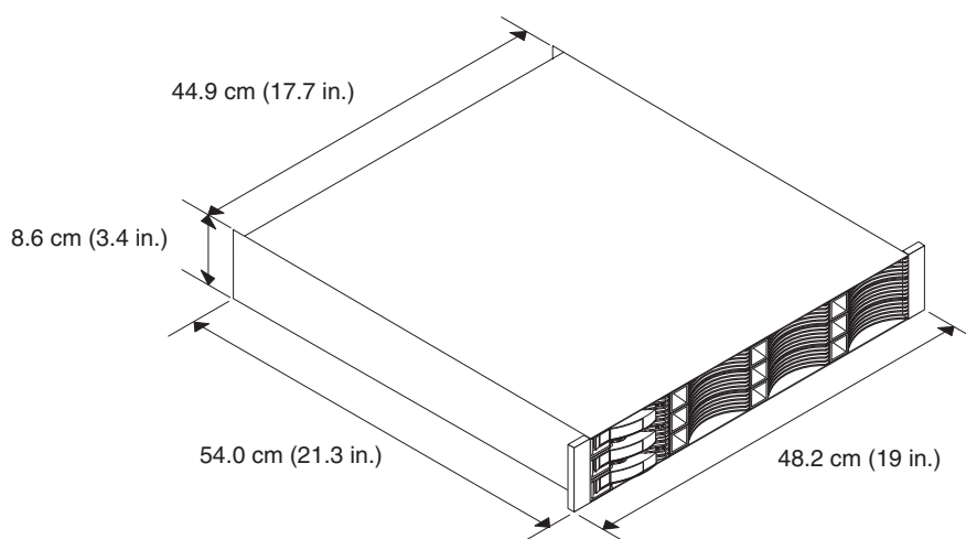
図 13. DS3512 ストレージ・サブシステムおよび EXP3512 ストレージ・エンクロージャーの寸法
