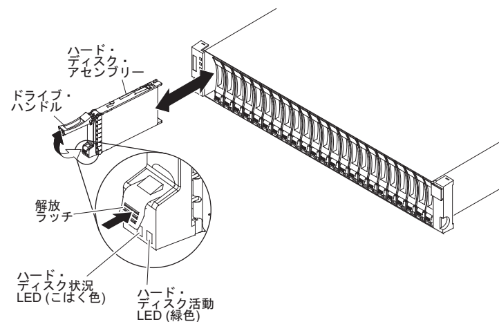
図 103. DS3524 または EXP3524 へのドライブの取り付け
