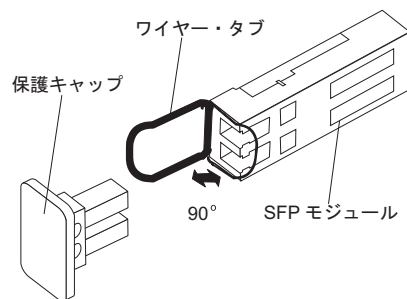
図 26. SFP モジュール・ラッチのアンロック - ワイヤー・タブの場合
