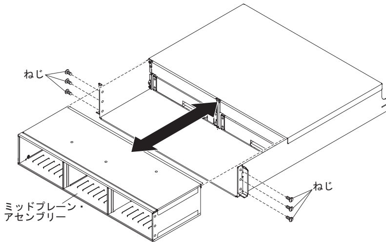
図 125. DS3524 または EXP3524 でのミッドプレーン・アセンブリーの交換
