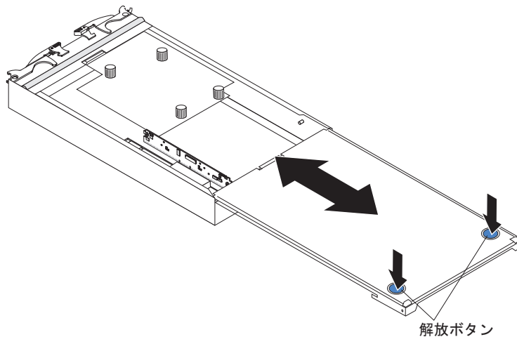
図 89. カバーの取り外し
