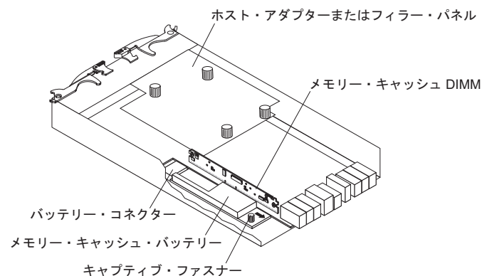
図 115. メモリー・キャッシュ DIMM の位置
