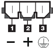
図 73. DC 電源コネクター - ピンの位置
