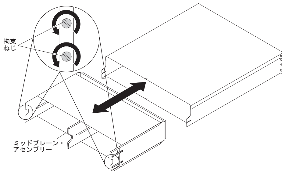
図 124. DS3512 または EXP3512 でのミッドプレーン・アセンブリーの交換
