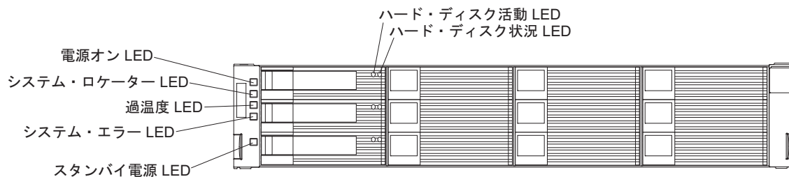
図 79. DS3512 ストレージ・サブシステムおよび EXP3512 ストレージ・エンクロージャの前面 LED およびコントロール
