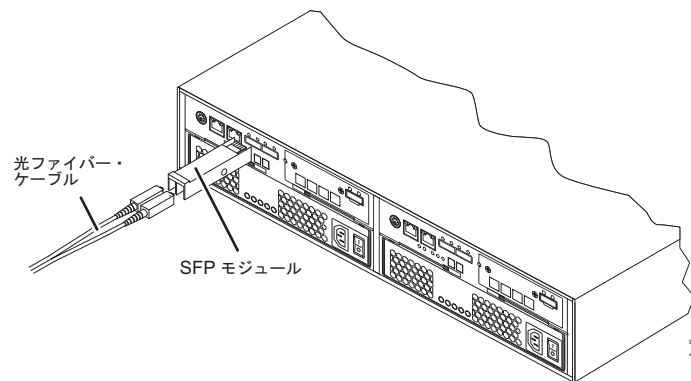
図 24. SFP モジュールのホスト・ポートへの取り付け
