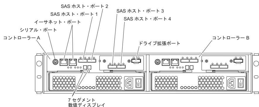
図 19. デュアル・コントローラー DS3500 ストレージ・サブシステムのポートとコントローラー (オプションの SAS ホスト・ポート・アダプターを装備)
