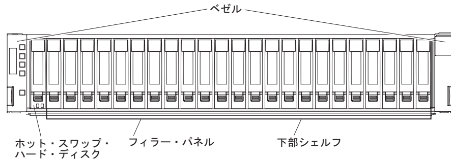
図3. DS3524 ストレージ・サブシステムおよび EXP3524 ストレージ・エンクロージャのホット・スワップ・ドライブ・ベイおよびベゼル
