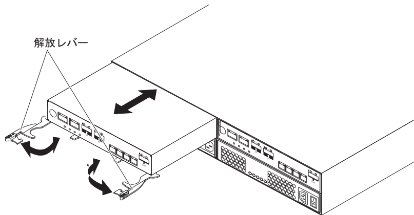
図 116. コントローラーの取り外し
