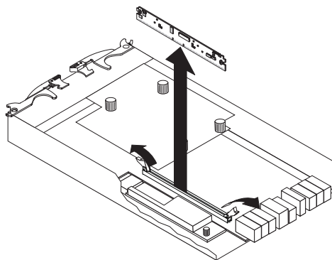
図 117. コントローラーからの DIMM の取り外し
