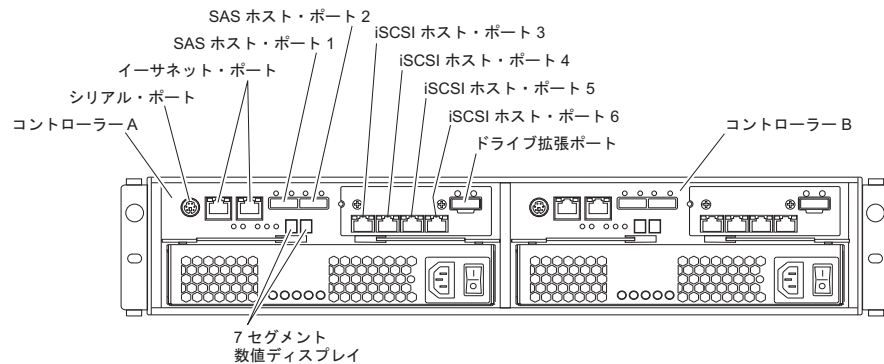
図 17. デュアル・コントローラー DS3500 ストレージ・サブシステムのポートとコントローラー (オプションの iSCSI ホスト・ポート・アダプターを装備)
