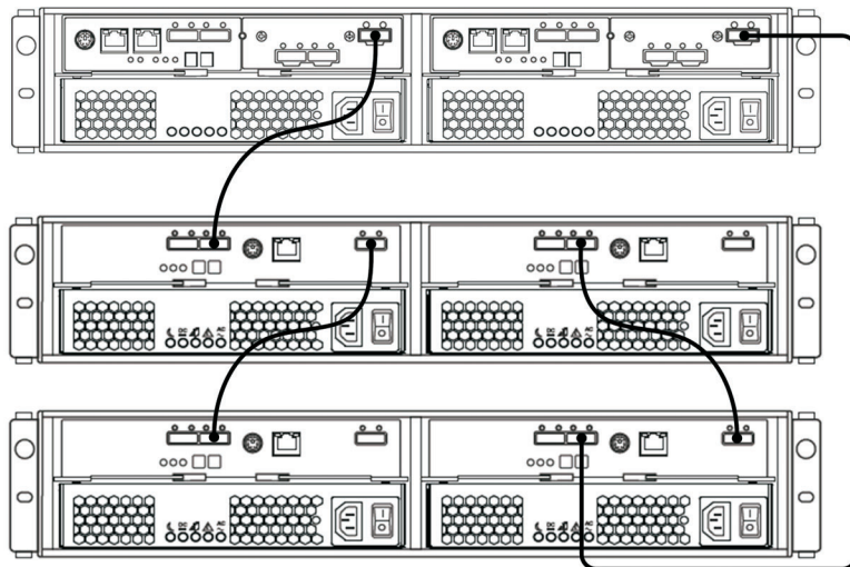
図 41. デュアル・コントローラー DS3500 と 2 つのストレージ・エンクロージャー
