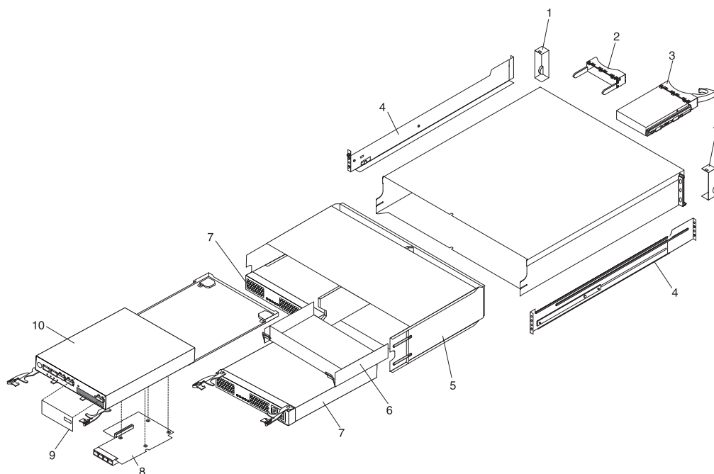
図 127. DS3512 ストレージ・サブシステムおよび EXP3512 ストレージ・エンクロージャー・ストレージ・サブシステムの部品
