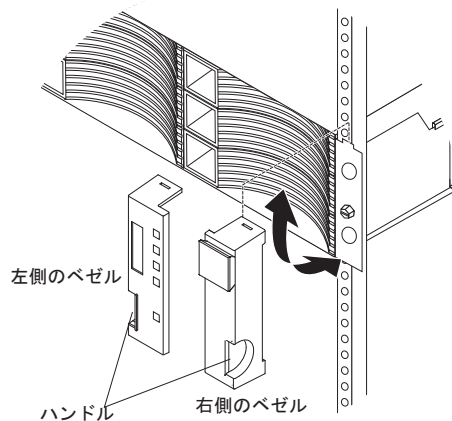
図 122. ベゼルの取り外し
