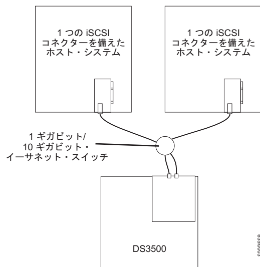
図 66. 単一ポート搭載の複数ホスト、シングル・コントローラー iSCSI 構成
