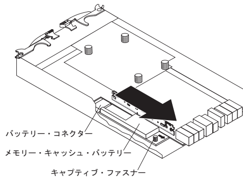
図 114. コントローラーからのバッテリー・ユニットの取り外し
