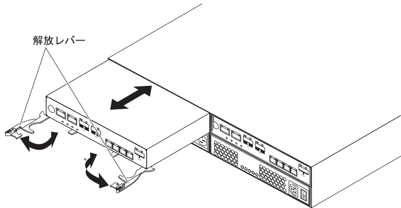
図 91. コントローラーの取り外しと交換
