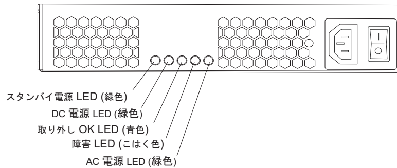
図 77. AC 電源機構 LED
