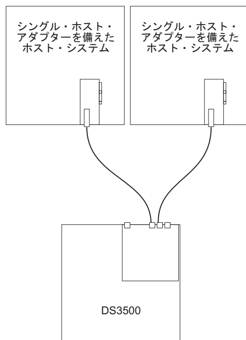
図 58. 複数のホスト内のシングル HBA へのシングル・コントローラー直接ファイバー・チャネル接続による接続
