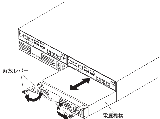
図 108. 電源機構の交換
