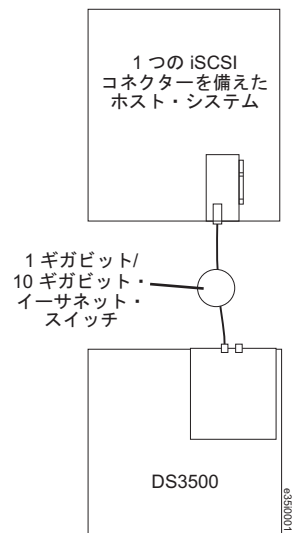
図 64. 単一ホスト、シングル・コントローラー iSCSI 構成
