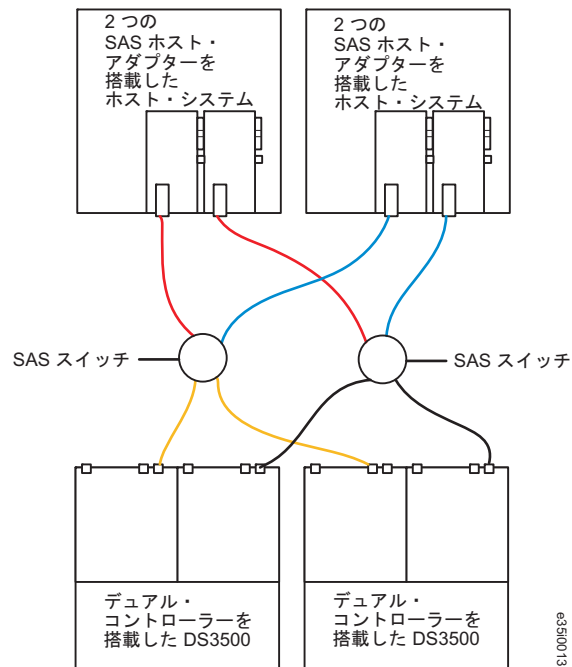
図 53. 2 つの独立した SAS スイッチを使用した複数のホストへの複数のデュアル・コントローラー DS3500 の SAS 接続
