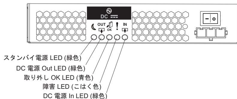
図 78. DC 電源機構 LED
