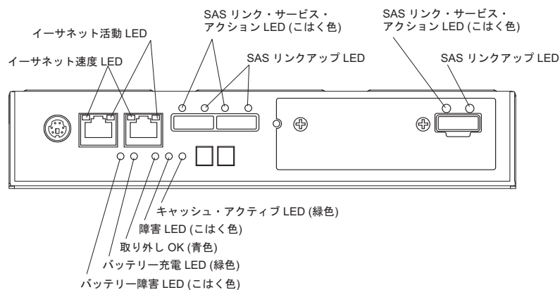
図 120. コントローラー LED
