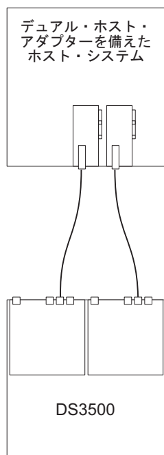
図 59. 同一ホスト内の 2 つの HBA へのデュアル・コントローラー直接ファイバー・チャネル接続による接続 (冗長ホスト接続)
