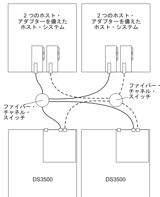
図 63. 二重ファイバー・チャンネル SAN 環境の 2 つのストレージ・サブシステムの例
