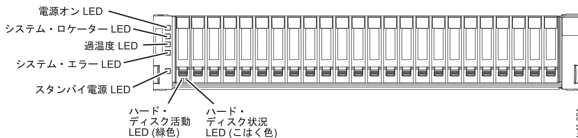
図 80. DS3524 ストレージ・サブシステムおよび EXP3524 ストレージ・エンクロージャの前面 LED
