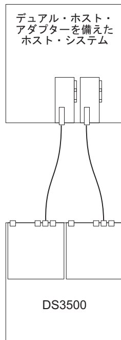
図 49. 同一ホスト内の 2 つの HBA へのデュアル・コントローラー直接 SAS 接続による接続 (冗長ホスト接続)
