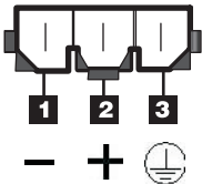
図 11. DC 電源機構コネクタ - ピンの位置
