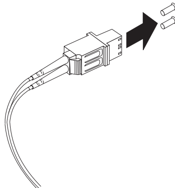
図 33. LC-SC ケーブル・アダプターの保護キャップの取り外し
