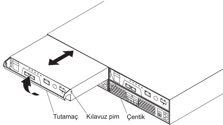
Şekil 37. Denetleyicinin çıkarılması ve geri takılması
