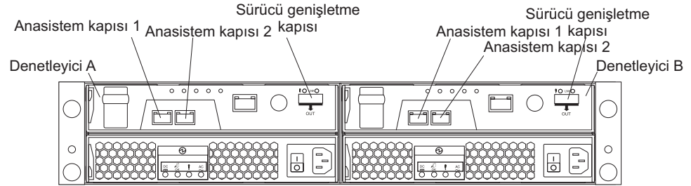
Şekil 13. DS3300 depolama altsisteminin kapıları ve denetleyicileri
