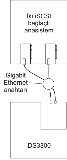
Şekil 24. Birden çok kapılı, tek denetleyicili yapılandırma
