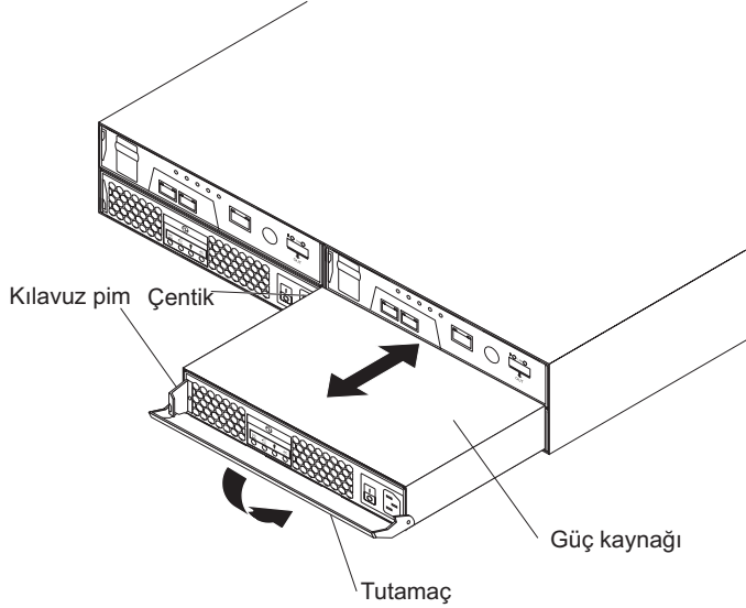
Şekil 42. Güç kaynağı biriminin yeniden takılması
