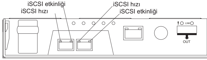
Şekil 34. iSCSI ışıkları
