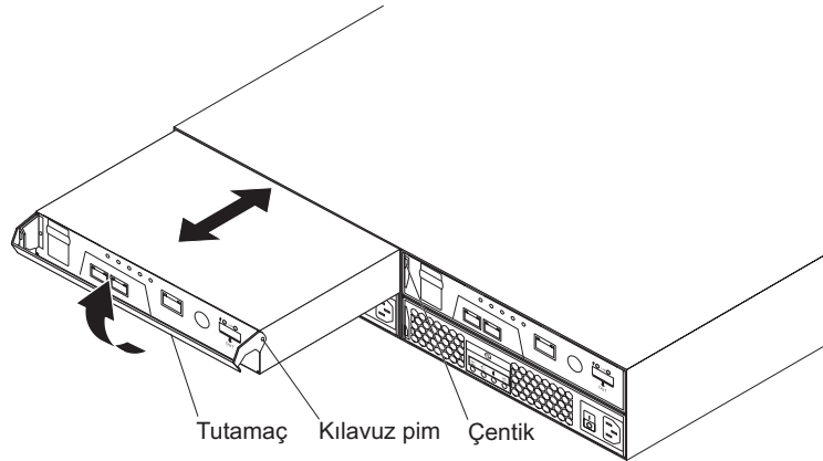
Şekil 36. Denetleyicinin takılması
