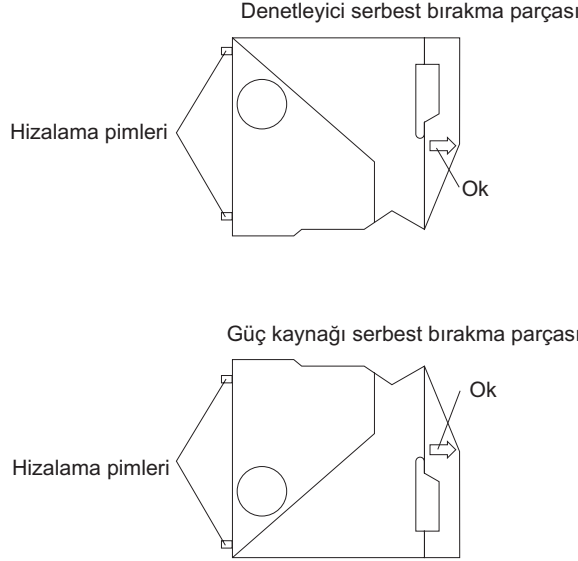
Şekil 52. Denetleyici ve güç kaynağı serbest bırakma parçaları
