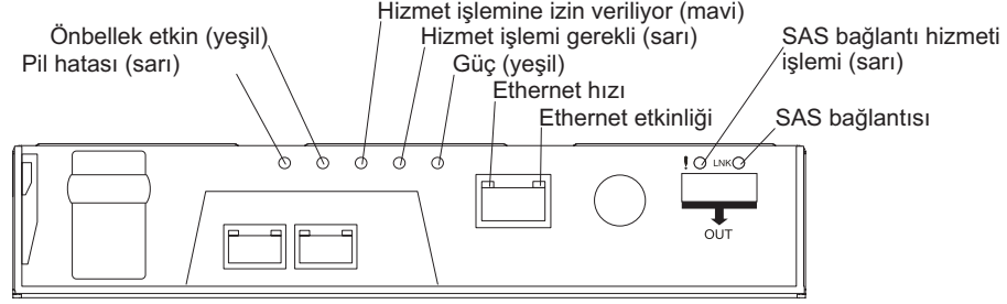
Şekil 33. Denetleyici ışıkları
