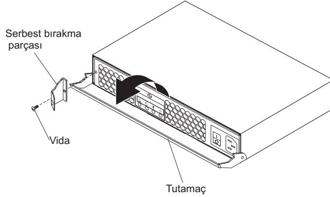
Şekil 53. Güç kaynağındaki serbest bırakma parçasını çıkarma
