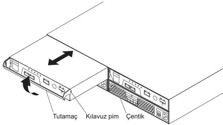
řekil 50. Denetleyicinin yeniden takılması
