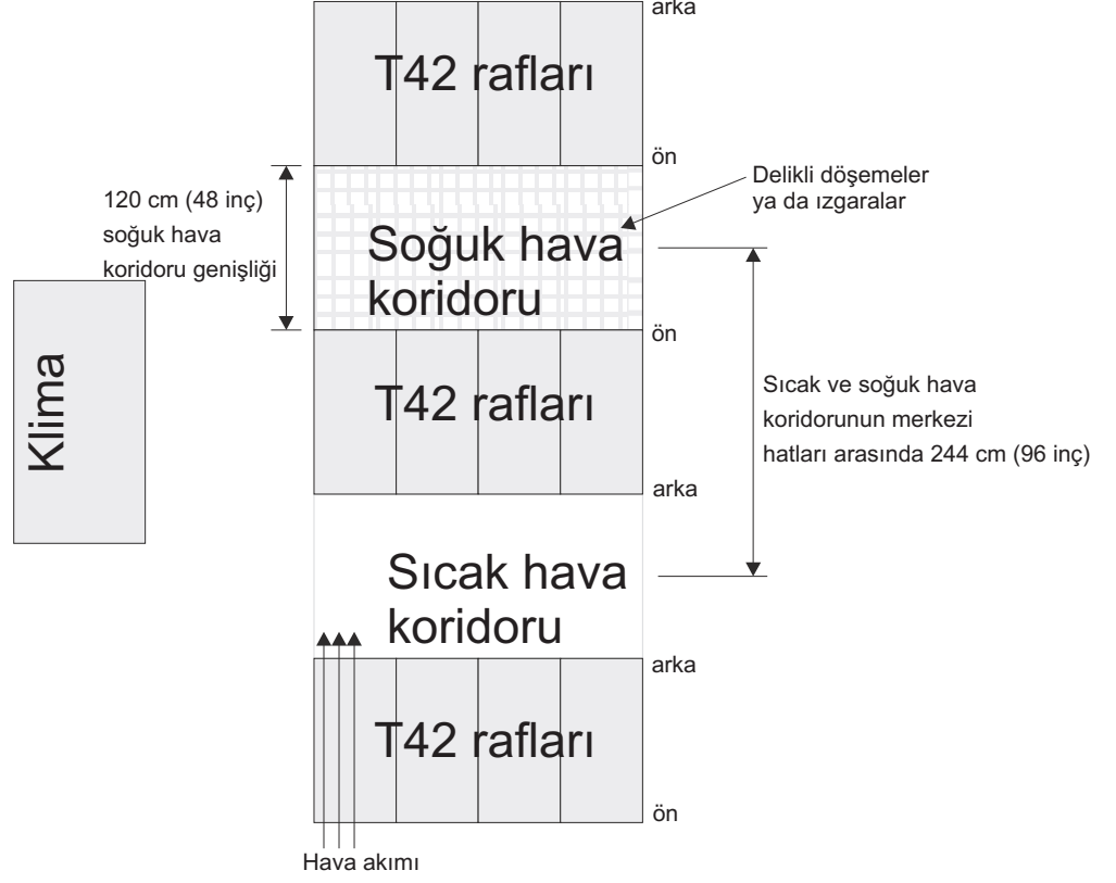
Şekil 12. Soğuk hava koridoru/sıcak hava koridoru raf yapılandırması örneği
