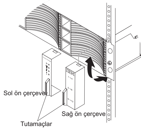
Şekil 51. Ön çerçeveleri çıkarma
