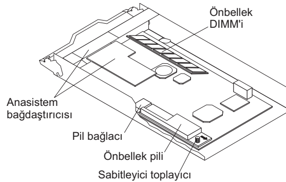
Şekil 45. Pil birimi
