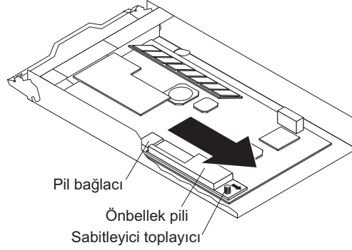
Şekil 38. Pil biriminin denetleyiciden çıkarılması
