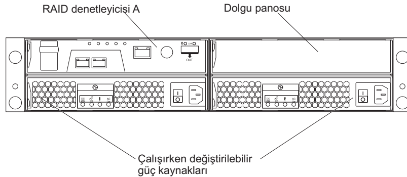
Şekil 5. Arkadan görünüm, tek denetleyicili model
