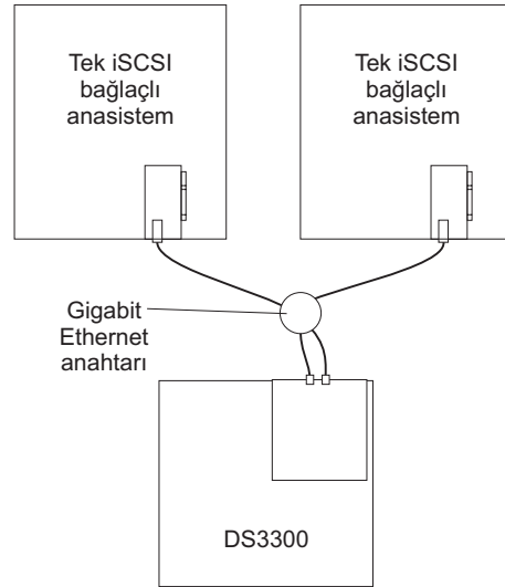
Şekil 25. Birden çok tek kapılı anasistem, tek denetleyicili yapılandırma
