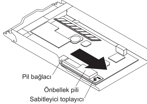
Şekil 47. Pili denetleyiciden çıkarılması
