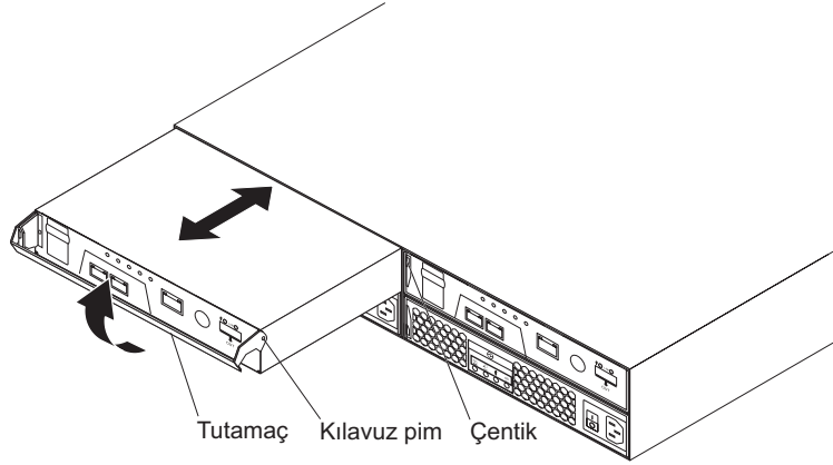
Şekil 43. Denetleyicinin çıkarılması ve geri takılması
