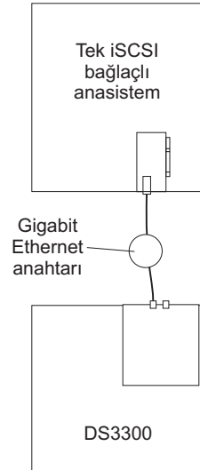
Şekil 23. Tek anasistem, tek denetleyici yapılandırması
