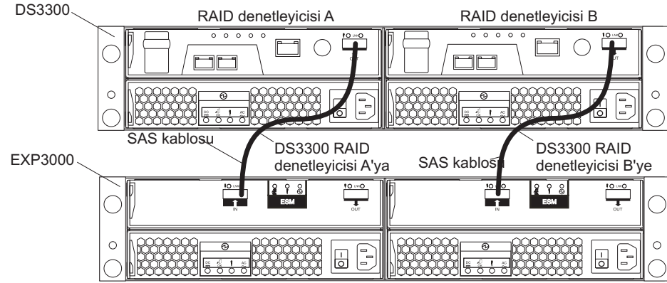
Şekil 17. Çift denetleyicili DS3300 ve bir depolama genişletme kasası
