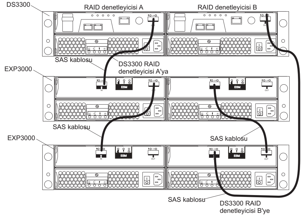
Şekil 18. Çift denetleyicili DS3300 ve iki depolama genişletme kasası
