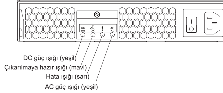
Şekil 31. Güç kaynağı ışıkları
