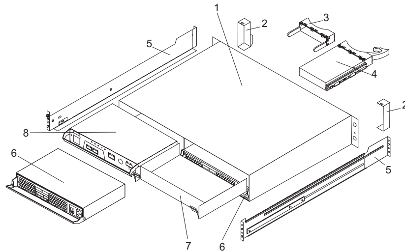
Şekil 56. DS3300 depolama altsistemi parçaları
