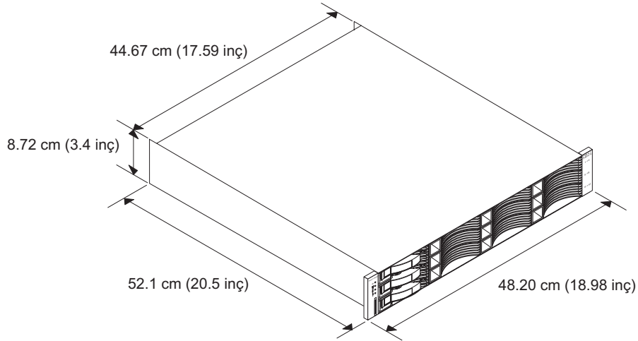
Şekil 10. DS3300 boyutları
