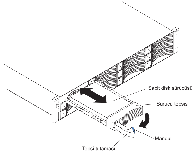
Şekil 40. Sürücünün çıkarılması
