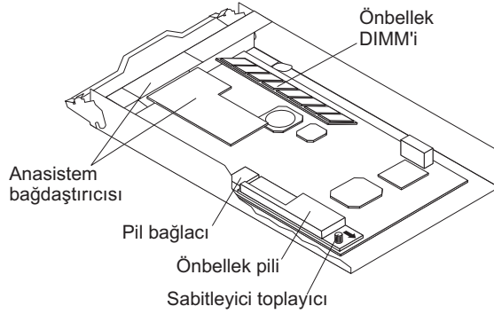
Şekil 9. Pil birimi
