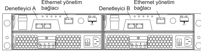
Şekil 20. Çift denetleyicili DS3300 üzerindeki Ethernet kapılarının yerleri
