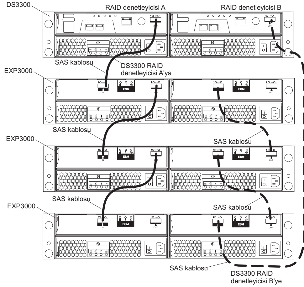
Şekil 15. Yedek sürücü yolu örneği
