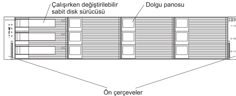
Şekil 2. DS3300 çalışırken değiştirilebilir sürücü bölmeleri ve ön çerçeveler
