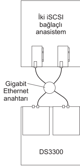
Şekil 28. Tek anasistem, birden çok kapı, çift denetleyici yapılandırması
