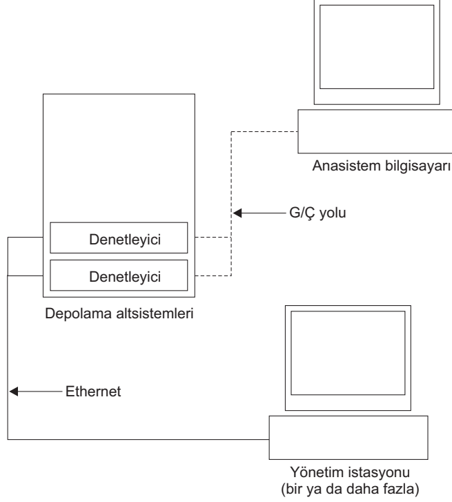
Şekil 22. Doğrudan (bant dışı) yönetim yöntemiyle yönetilen depolama altsistemleri
