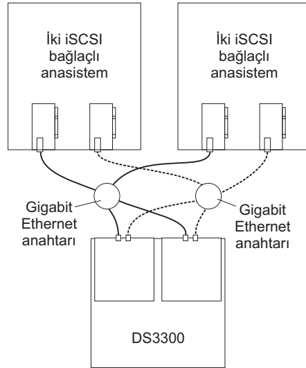
Şekil 29. Birden çok anasistem, birden çok kapı, çift denetleyici yapılandırması
