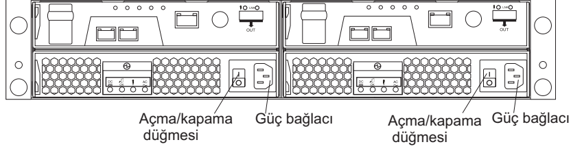
Şekil 30. DS3300 için güç kaynağı anahtarları ve bağlaçları
