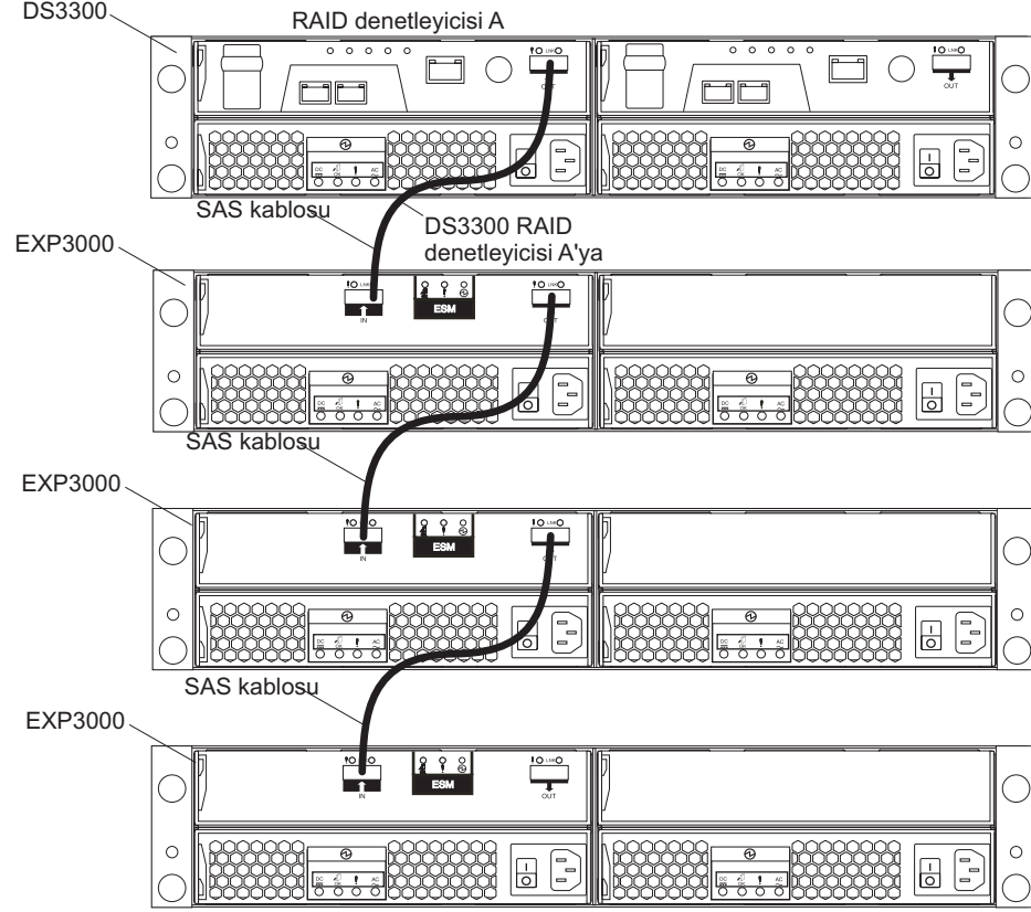
Şekil 16. Tek denetleyicili DS3300 ve birden çok tek ESM'li depolama genişletme kasası
