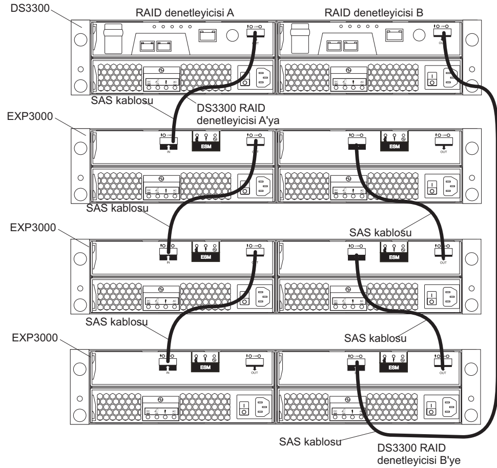
Şekil 19. Çift denetleyicili DS3300 ve üç depolama genişletme kasası
