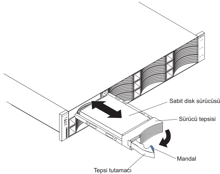
Şekil 41. Sabit disk sürücüsünün takılması ve çıkarılması
