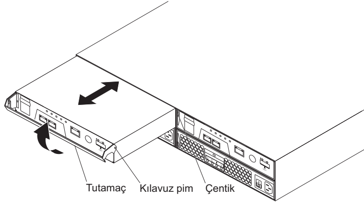
Şekil 35. Denetleyicinin çıkarılması
