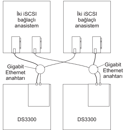
Şekil 27. Birden çok anasistem, birden çok kapı, birden çok depolama altsistemi yapılandırması
