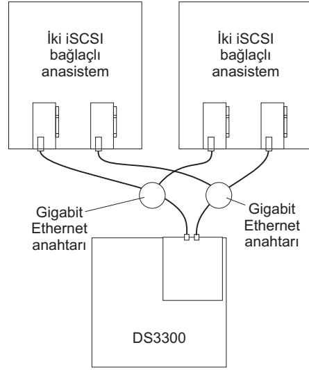
Şekil 26. Birden çok anasistem, birden çok kapı, tek denetleyici ve yedek yol yapılandırması
