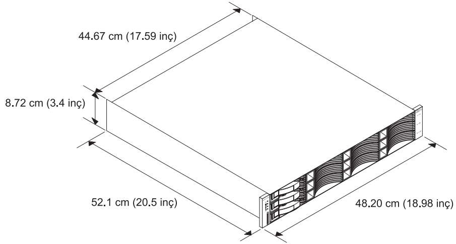
Şekil 10. DS3200 boyutları
