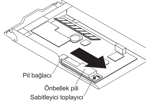
Şekil 53. Pili denetleyiciden çıkarılması
