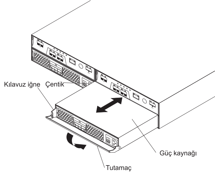
Şekil 48. Güç kaynağı biriminin yeniden takılması
