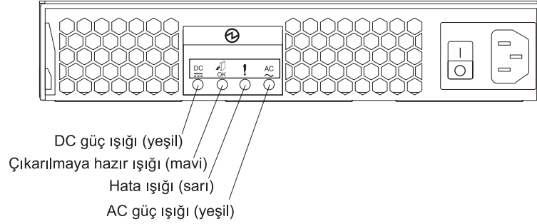
Şekil 34. Güç kaynağı ışıkları
