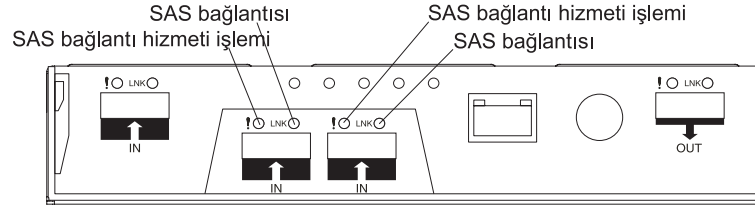
Şekil 37. Anasistem kapısı bağdaştırıcısı ışıkları
