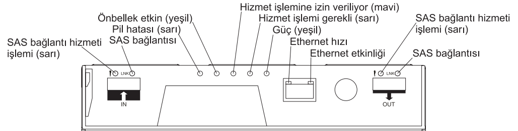
Şekil 36. Denetleyici ışıkları
