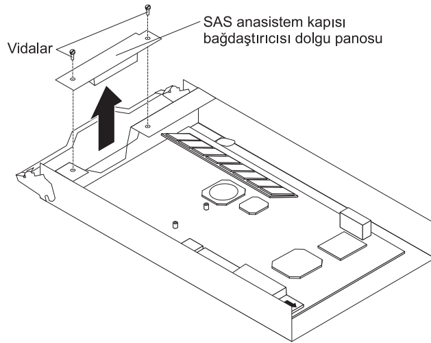
Şekil 43. SAS anasistem kapısı bağdaştırıcısı dolgu panosunun çıkarılması
