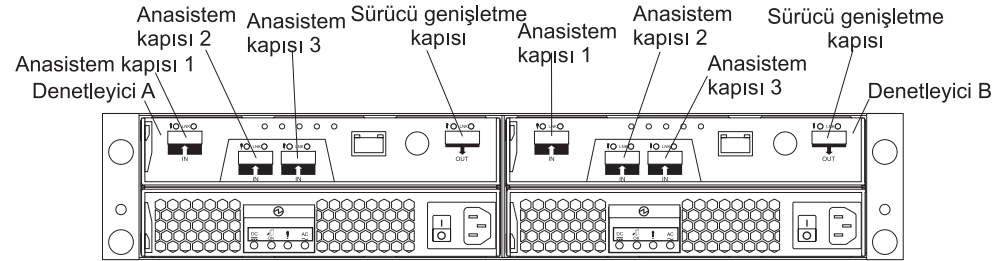
Şekil 14. Çift denetleyicili DS3200 depolama altsisteminin kapıları ve denetleyicileri (isteğe bağlı bir anasistem kapısı bağdaştırıcısı ile birlikte)
