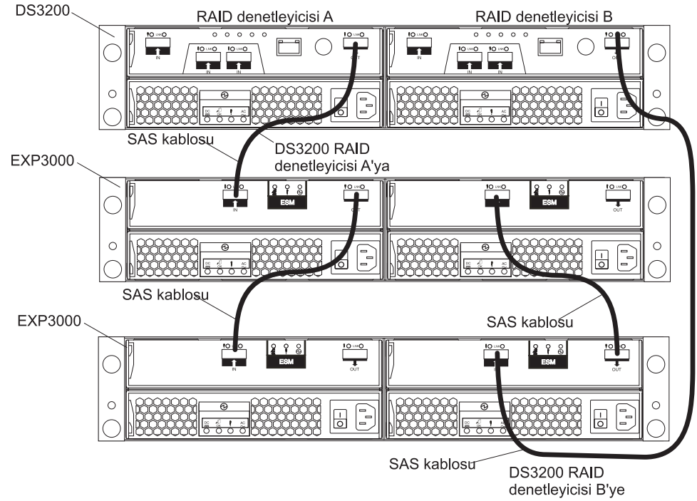
Şekil 21. Bir adet çift denetleyicili DS3200 ve iki adet depolama genişletme kasası
