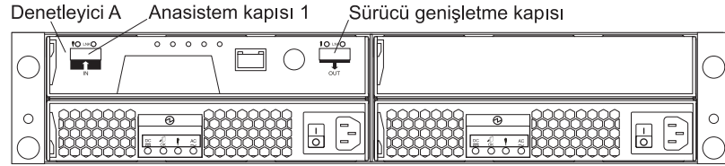
Şekil 13. Tek denetleyicili DS3200 depolama altsistemi kapıları ve denetleyici
