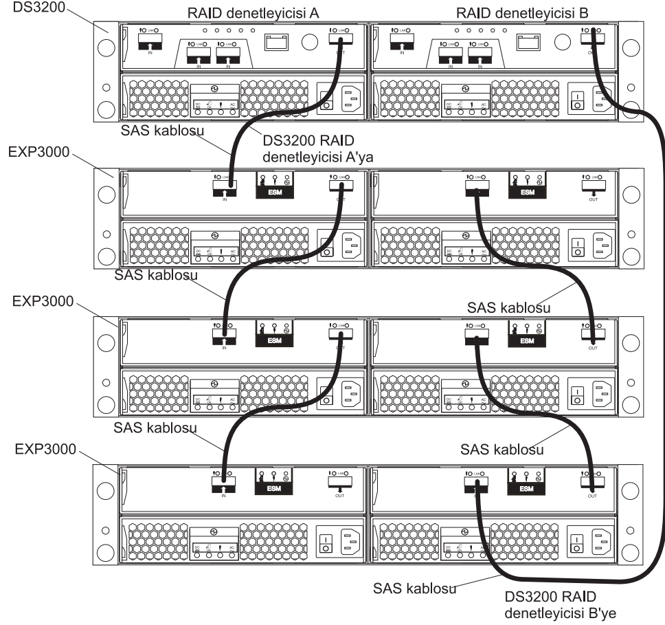
Şekil 22. Bir adet çift denetleyicili DS3200 ve üç adet depolama genişletme kasası
