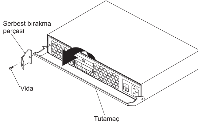
Şekil 59. Güç kaynağındaki serbest bırakma parçasını çıkarma
