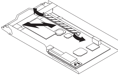
Şekil 55. DIMM'in denetleyiciye takılması
