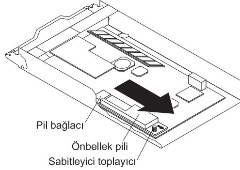
Şekil 41. Pil biriminin denetleyiciden çıkarılması
