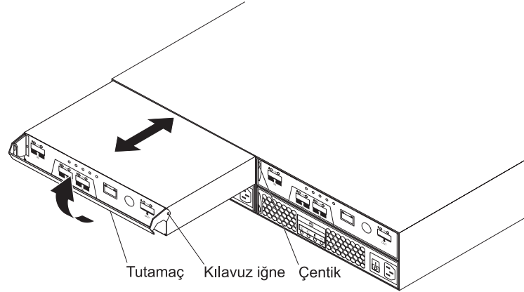
Şekil 52. Denetleyicinin çıkarılması
