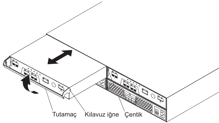
řekil 56. Denetleyicinin yeniden takılması
