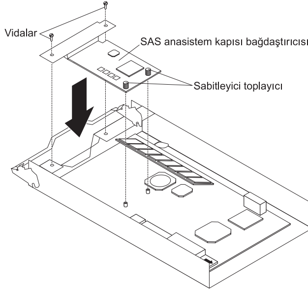
Şekil 44. SAS anasistem kapısı bağdaştırıcısının takılması
