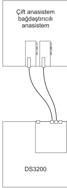
Şekil 27. Tek denetleyiciden, tek anasistemdeki (yedek anasistem bağlantısı) çift HBA'ya doğrudan yapılmış bağlantı
