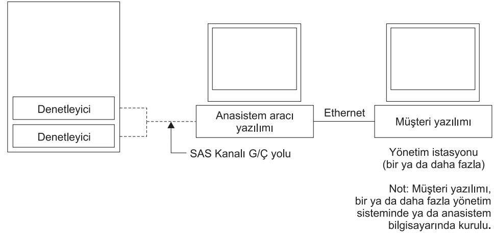
Şekil 24. Anasistem-aracı (bant içi) tarafından yönetilen depolama altsistemleri
