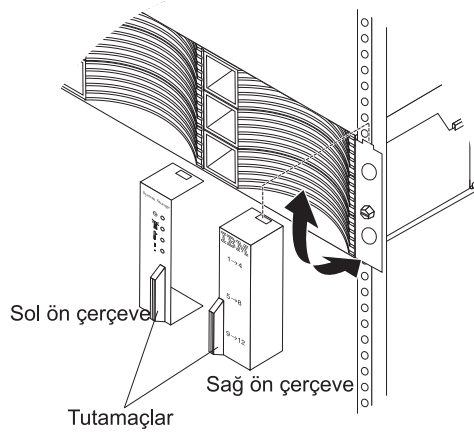
Şekil 57. Ön çerçeveleri çıkarma
