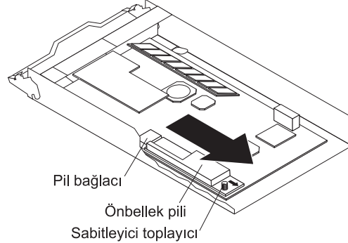
Şekil 50. Pil biriminin denetleyiciden çıkarılması
