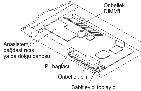
Şekil 9. Pil birimi
