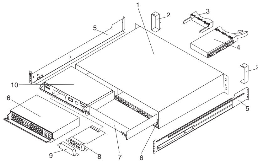
Şekil 62. DS3200 depolama altsistemi parçaları
