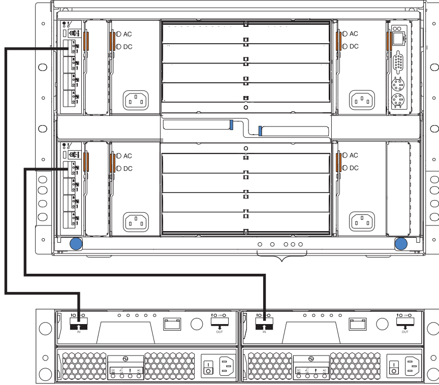
Şekil 32. Bir BladeCenter birimine bağlı DS3200 örneği
