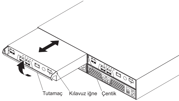
Şekil 38. Denetleyicinin çıkarılması
