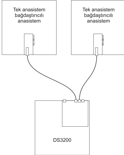
Şekil 28. Birden çok anasistemdeki tek HBA'lara tek denetleyicinin doğrudan bağlantısı
