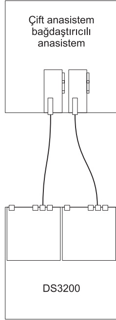
Şekil 29. Çift denetleyiciden aynı anasistemdeki (yedek anasistem bağlantısı) iki HBA'ya doğrudan yapılmış bağlantı
