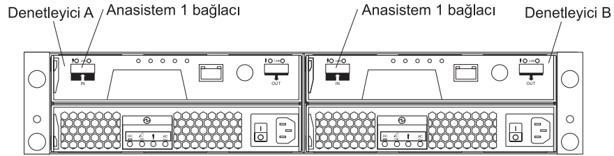
Şekil 31. DS3200 denetleyicisi bağlaçları
