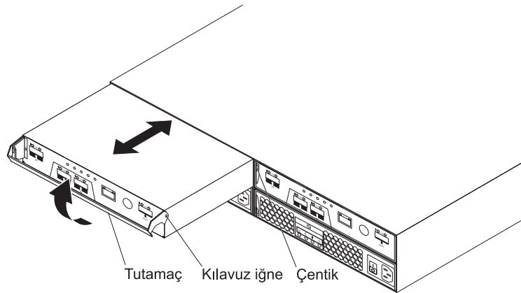
Şekil 40. Denetleyicinin çıkarılması ve geri takılması
