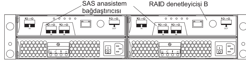
Şekil 6. Arkadan görünüm, çift denetleyicili model (takılı olan isteğe bağlı SAS anasistem kapısı bağdaştırıcıları ile gösterilir)
