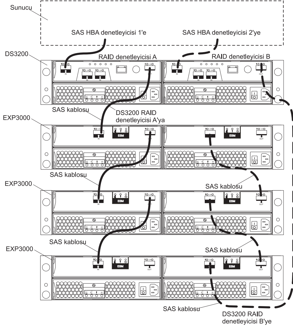
Şekil 18. Yedek sürücü yolu örneği
