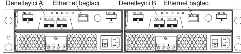
Şekil 23. Çift denetleyicili DS3200 üzerindeki Ethernet kapılarının yerleri
