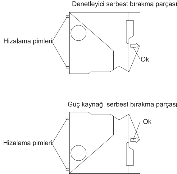
Şekil 58. Denetleyici ve güç kaynağı serbest bırakma parçaları
