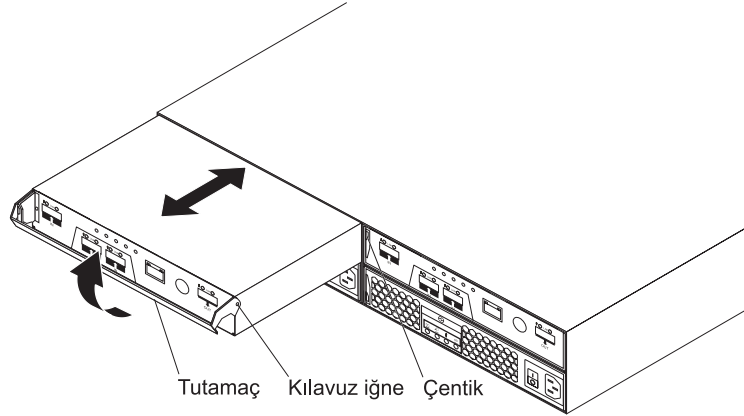
Şekil 49. Denetleyicinin çıkarılması ve geri takılması
