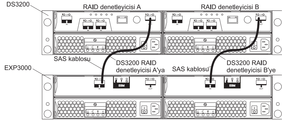
Şekil 20. Çift denetleyicili DS3200 ve bir depolama genişletme kasası
