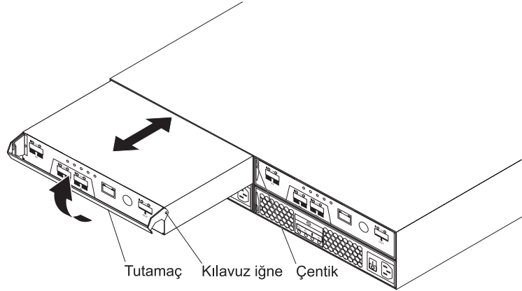
Şekil 42. Denetleyici A'nın çıkarılması ve değiştirilmesi
