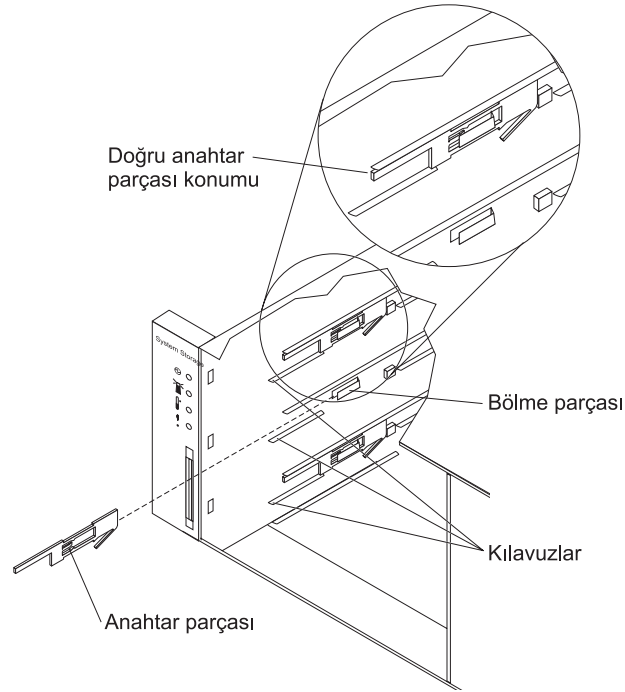
Şekil 61. Sürücü uyumluluğu anahtarı takma
