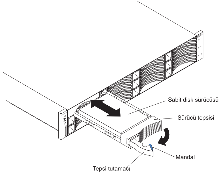
Şekil 47. Sabit disk sürücüsünün takılması ve çıkarılması
