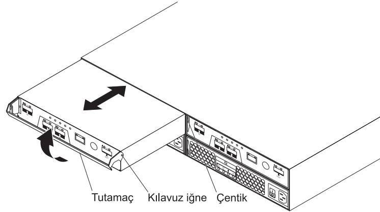
Şekil 39. Denetleyicinin takılması
