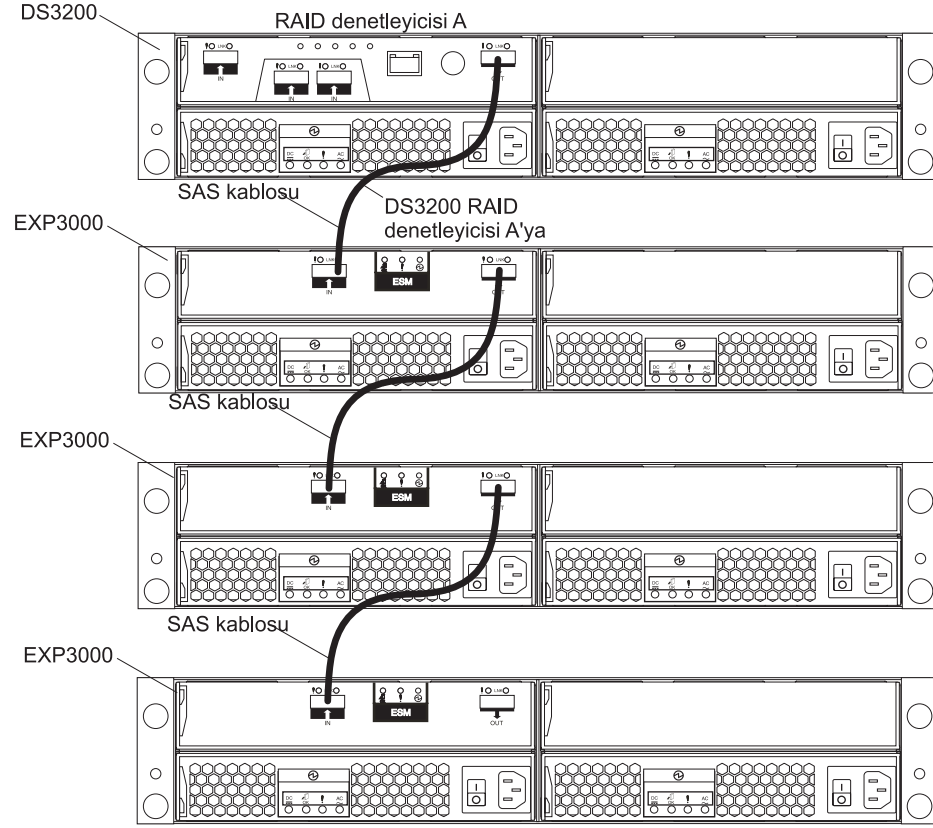
Şekil 19. Tek denetleyicili DS3200 ve birden çok tek ESM'li depolama genişletme kasası
