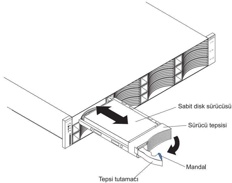
Şekil 46. Sürücünün çıkarılması
