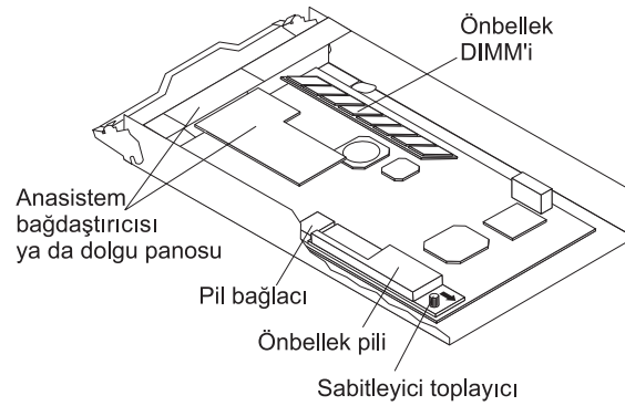
Şekil 51. Önbellek DIMM'inin yeri
