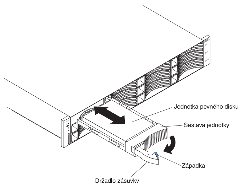
Obrázek 47. Instalace a odstranění jednotky pevného disku
