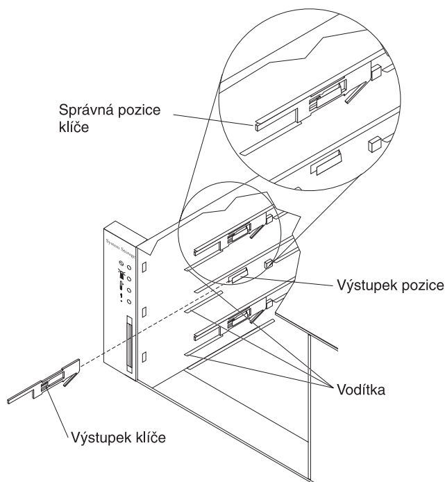
Obrázek 61. Instalace klíče kompatibility jednotek
