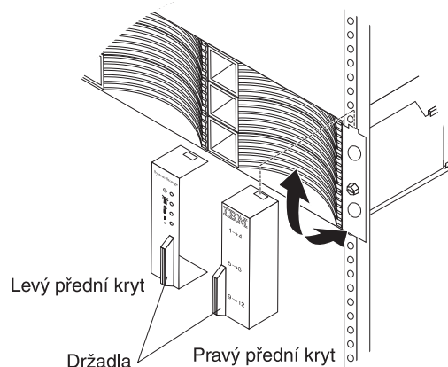
Obrázek 57. Odstranění předních krytů
