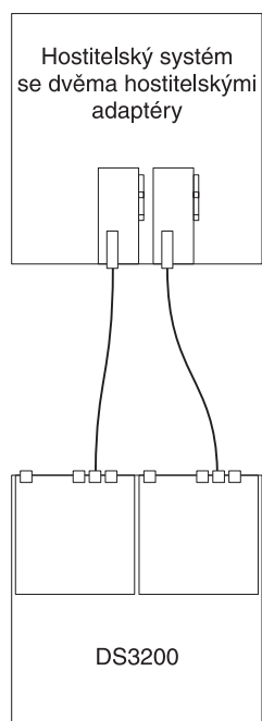
Obrázek 29. Přímé spojení dvou řadičů s dvěma adaptéry hostitelské sběrnice na jednom hostiteli (redundantní hostitelské spojení)
