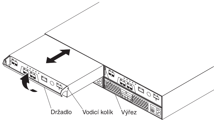
Obrázek 38. Vyjmutí řadiče
