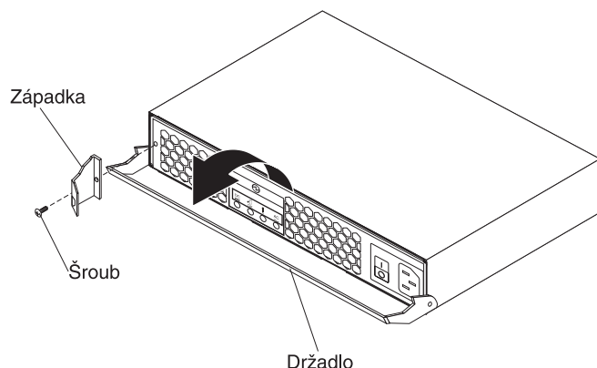
Obrázek 59. Odstranění západky zdroje napájení
