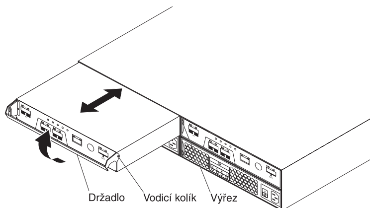
Obrázek 40. Vyjmutí a výměna řadiče
