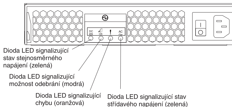
Obrázek 34. Diody LED zdroje napájení
