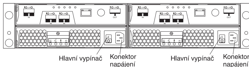
Obrázek 33. Vypínače a konektory napájení úložného subsystému DS3200
