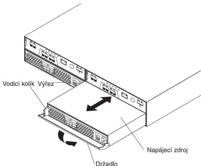
Obrázek 48. Výměna zdroje napájení
