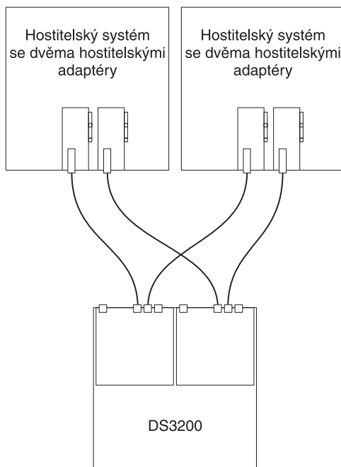
Obrázek 30. Přímé spojení dvou řadičů s více adaptéry hostitelské sběrnice na více hostitelích
