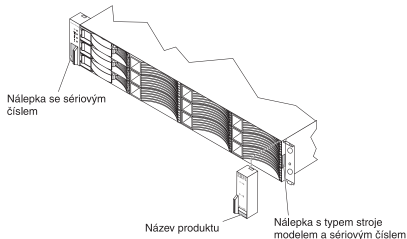
Obrázek 1. Umístění sériového čísla, názvu produktu, typu stroje a modelu subsystému DS3200
