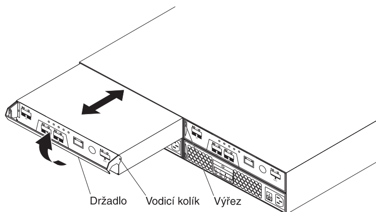
Obrázek 39. Instalace řadiče
