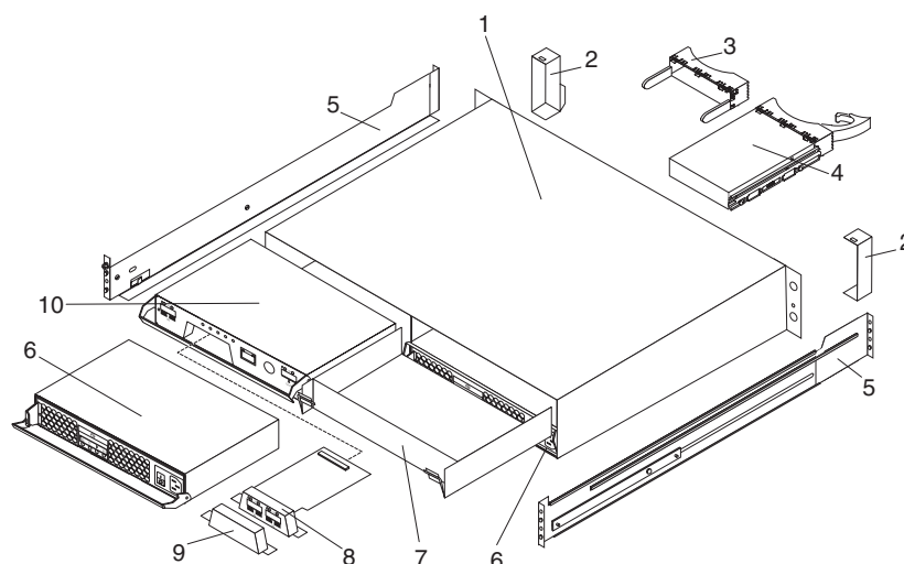
Obrázek 62. Součásti subsystému DS3200
