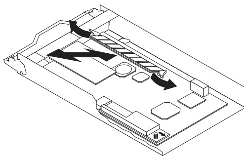
Obrázek 54. Vyjmutí modulu DIMM z řadiče
