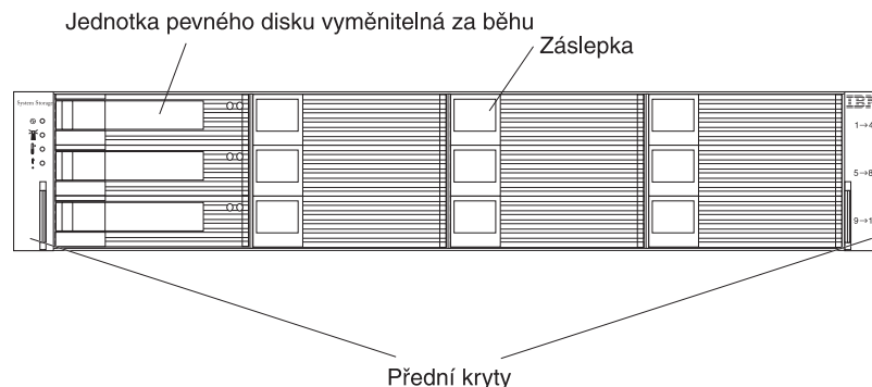
Obrázek 2. pozice diskových jednotek vyměnitelných za běhu a přední kryty subsystému DS3200
