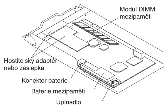
Obrázek 51. Umístění modulu DIMM mezipaměti
