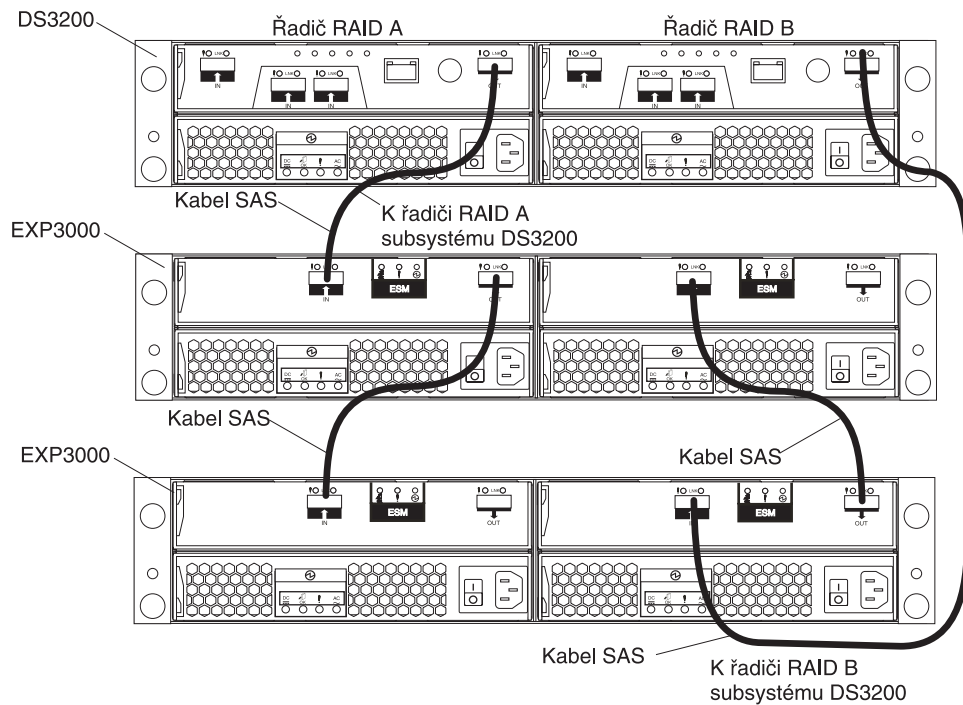
Obrázek 21. Jeden subsystém DS3200 s dvěma řadiči a dvě jednotky rozšíření
