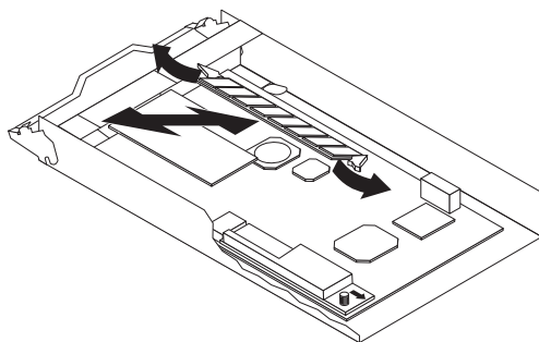
Obrázek 55. Instalace modulu DIMM do řadiče
