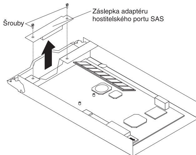
Obrázek 43. Odstranění adaptéru hostitelského portu
