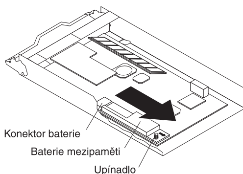
Obrázek 50. Vyjmutí baterie z řadiče
