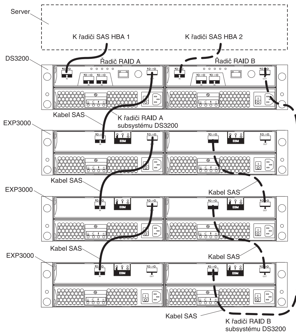
Obrázek 18. Příklad redundantního páru kanálů jednotek
