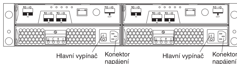
Obrázek 7. Prvky zdrojů napájení subsystému for DS3200
