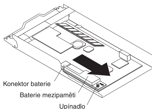
Obrázek 41. Vyjmutí baterie z řadiče
