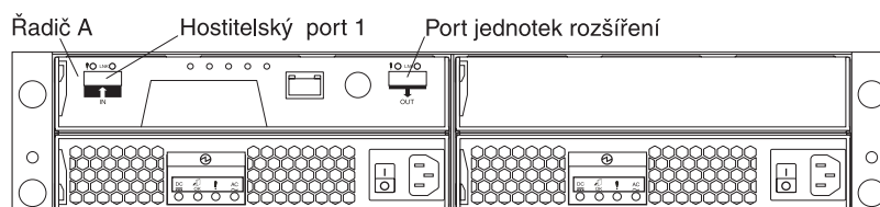
Obrázek 13. Konektory a řadič úložného subsystému DS3200 s jedním řadičem
