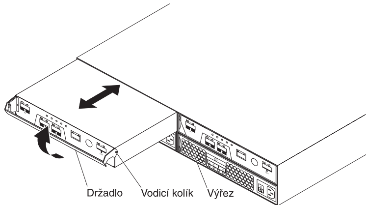
Obrázek 42. Vyjmutí a výměna řadiče A
