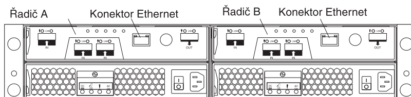
Obrázek 23. Umístění konektorů Ethernet úložného subsystému DS3200 s dvěma řadiči
