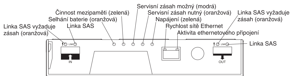
Obrázek 36. Diody LED řadiče
