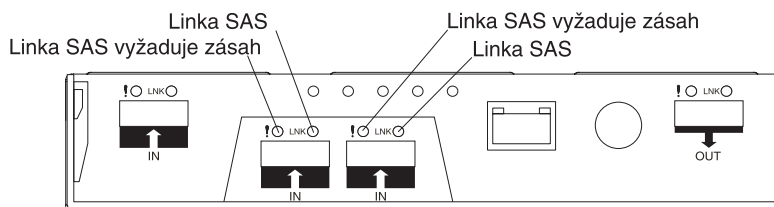
Obrázek 37. Diody LED adaptéru hostitelského portu
