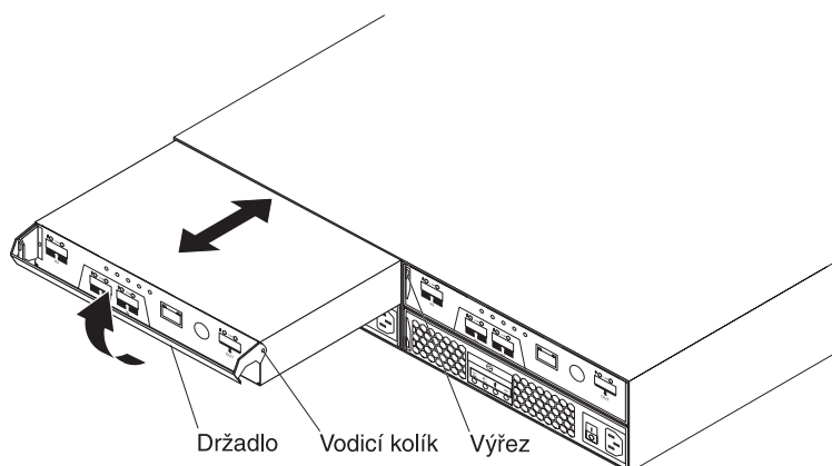
Obrázek 49. Vyjmutí a výměna řadiče
