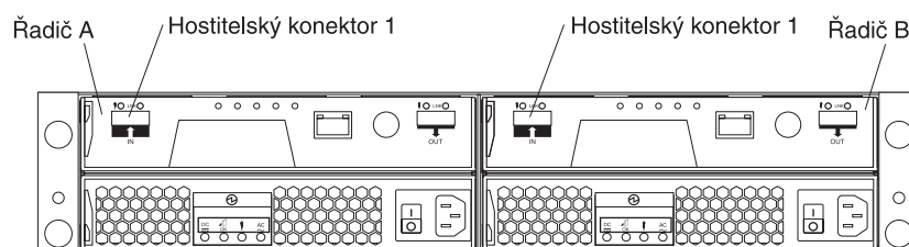
Obrázek 31. Konektory řadičů subsystému DS3200
