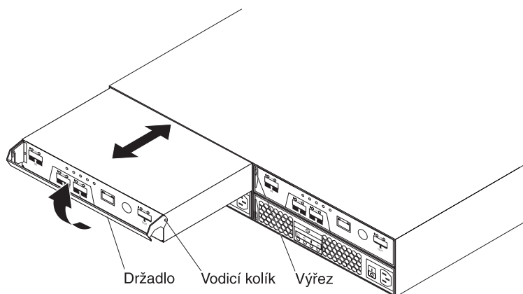
Obrázek 56. Instalace řadiče
