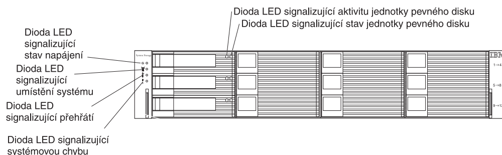
Obrázek 35. Diody LED a ovládací prvky na přední části
