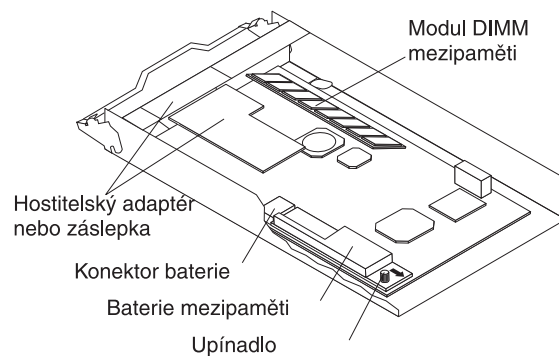
Obrázek 9. Baterie
