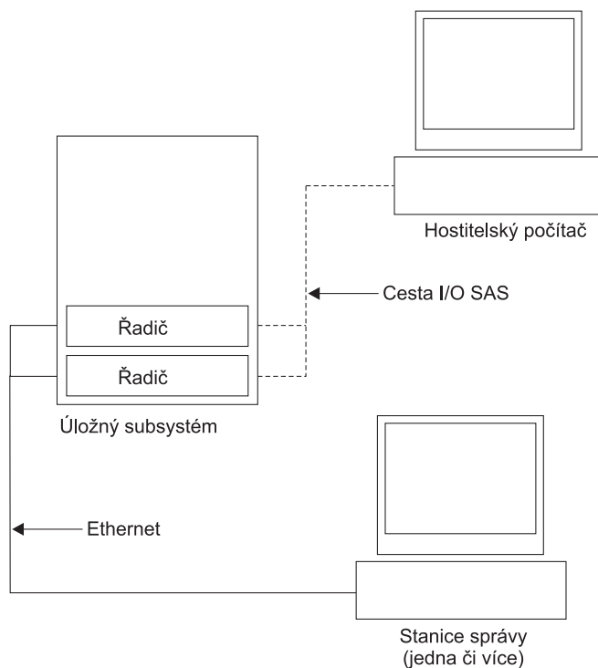
Obrázek 25. Přímá správa
