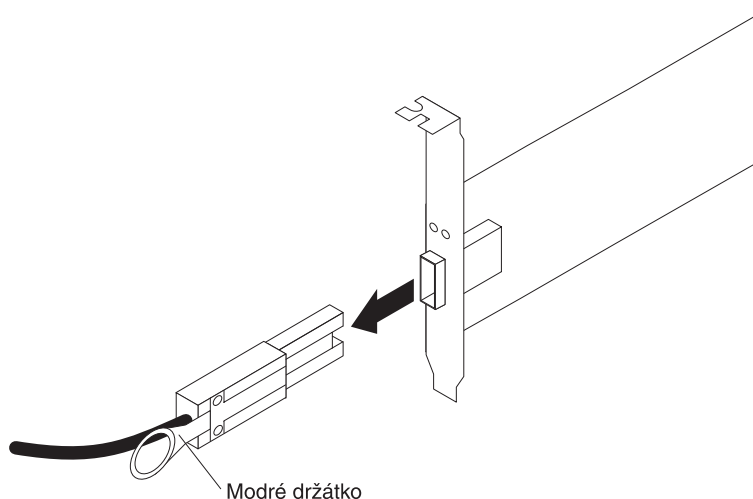
Obrázek 17. Odpojení kabelu mini-SAS
