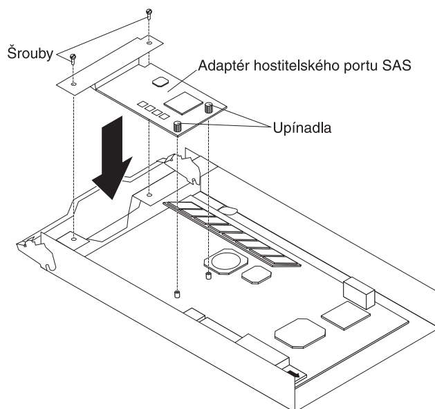
Obrázek 44. Instalace adaptéru hostitelského portu SAS
