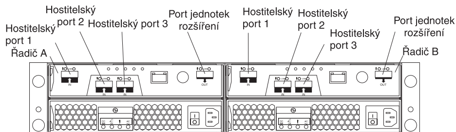
Obrázek 14. Konektory a řadiče úložného subsystému DS3200 se dvěma řadiči (s volitelnými adaptéry hostitelských portů)
