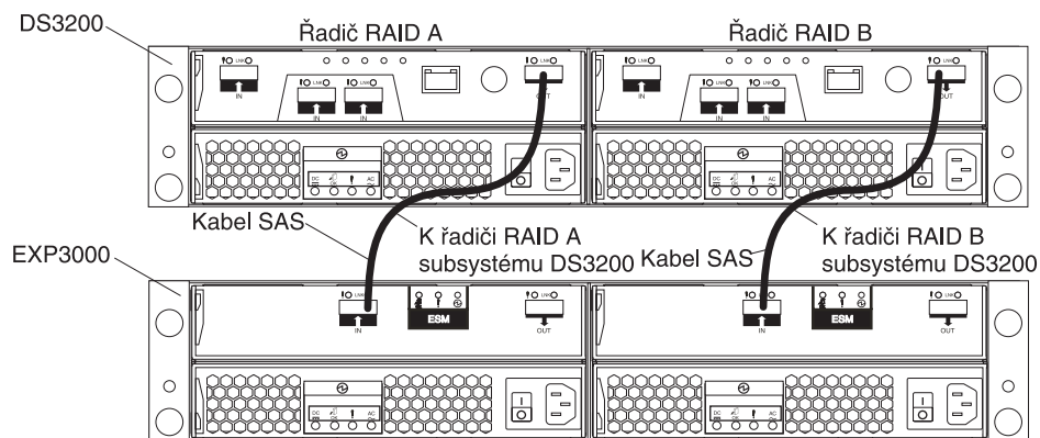
Obrázek 20. Jeden subsystém DS3200 s dvěma řadiči a jedna jednotka rozšíření
