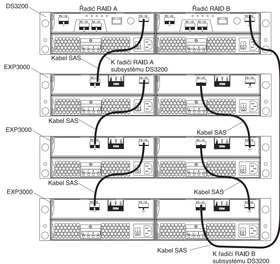
Obrázek 22. Jeden subsystém DS3200 s dvěma řadiči a tři jednotky rozšíření
