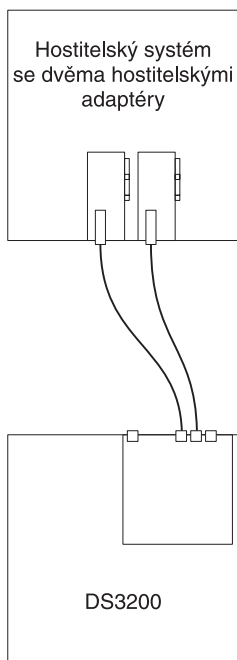
Obrázek 27. Přímé spojení jednoho řadiče s dvěma adaptéry hostitelské sběrnice na jednom hostiteli (redundantní hostitelské spojení)
