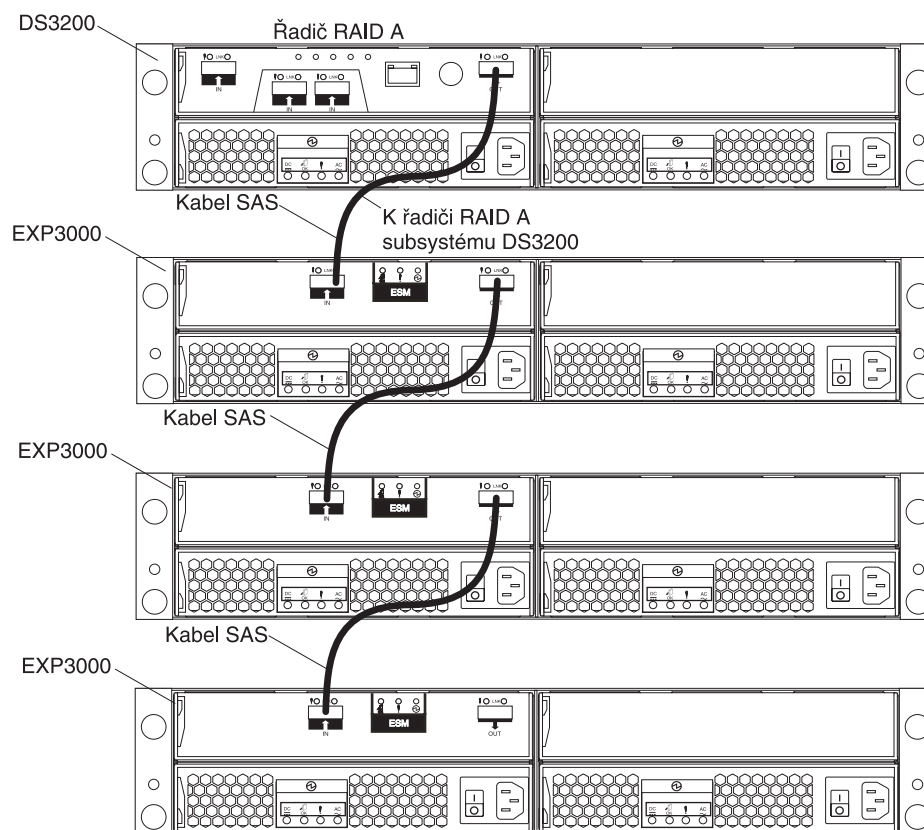
Obrázek 19. Subsystém DS3200 s jedním řadičem a několik jednotek rozšíření s jedním modulem ESM
