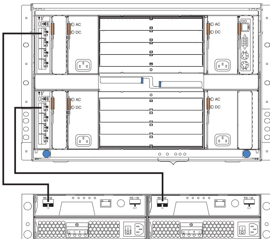
Obrázek 32. Příklad připojení subsystému DS3200 k jednotce BladeCenter
