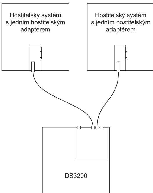
Obrázek 28. Přímé spojení jednoho řadiče s jednotlivými adaptéry hostitelské sběrnice na více hostitelích
