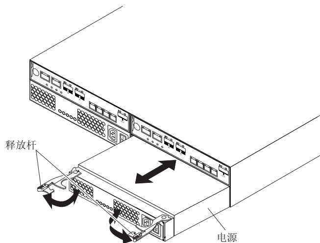
图 4. 从 DS3500 存储子系统或 EXP3500 扩展机柜中卸下电源
