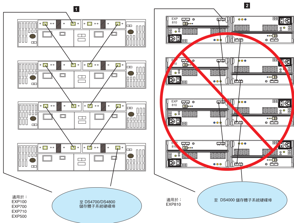
圖 38. 適用於連接儲存裝置的替代纜線迴圈方法
