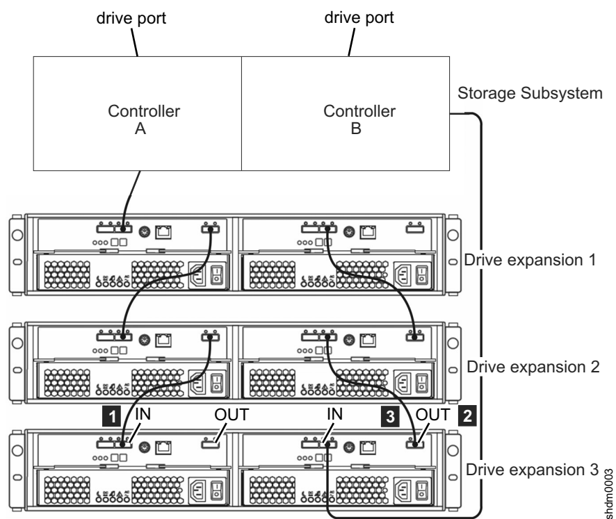
図 30. 追加の EXP3000、EXP3512、または EXP3524 ストレージ・エンクロージャーのケーブル接続
