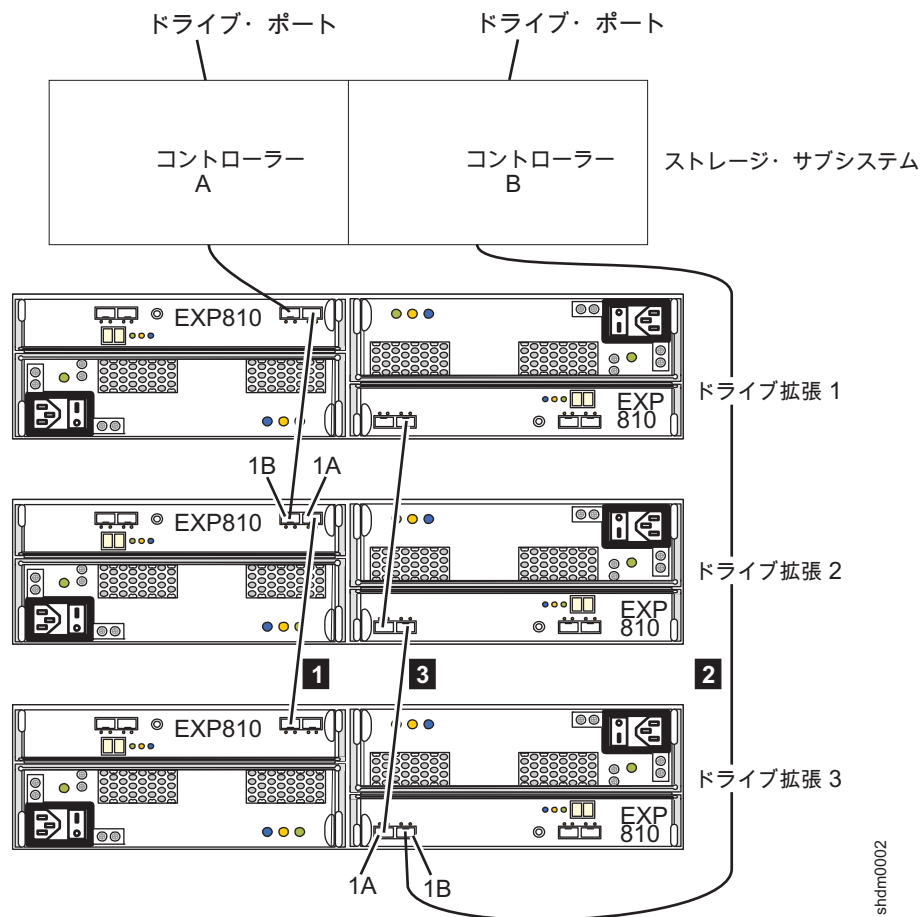
図 29. 追加の EXP5000、EXP520、EXP395、EXP810、または EXP420 ストレージ・エンクロージャーのケーブル接続
