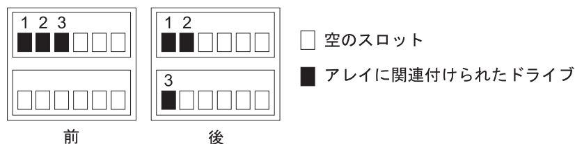
図 22. 2 つのストレージ・エンクロージャー内で空のベイを使用して定義済みアレイを再配列する場合のベスト・プラクティス
