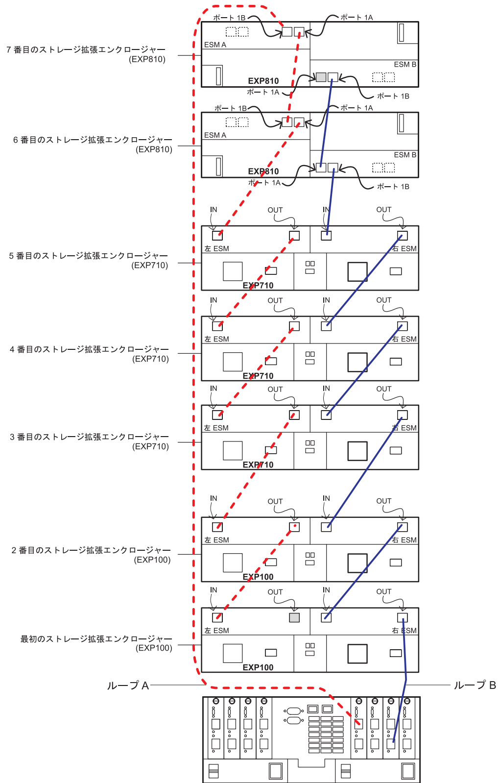
図 12. EXP100、EXP710、および EXP810 ストレージ・エンクロージャーを混用する際のサポートされるケーブル接続 (例 1)
