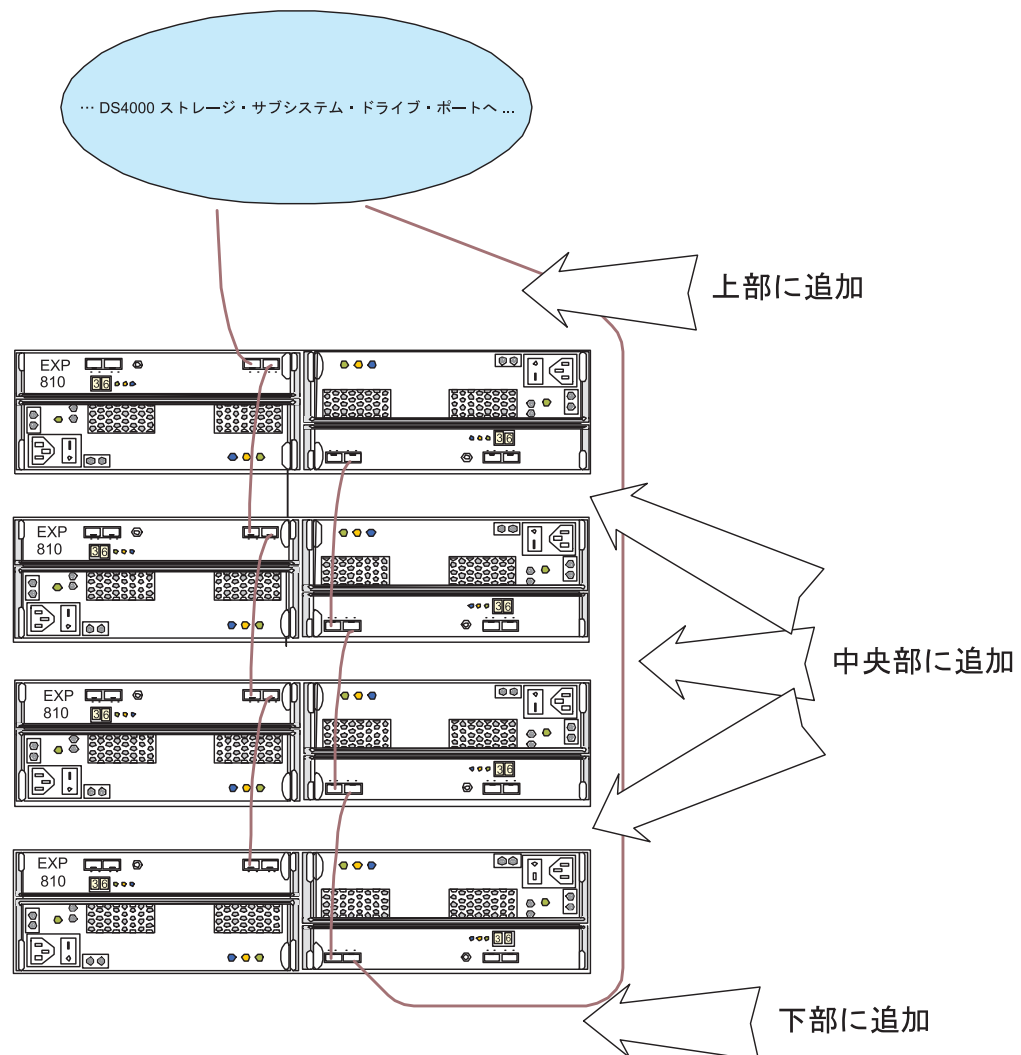
図 27. ドライブ・ループ内のストレージ・エンクロージャの位置を追加する例
