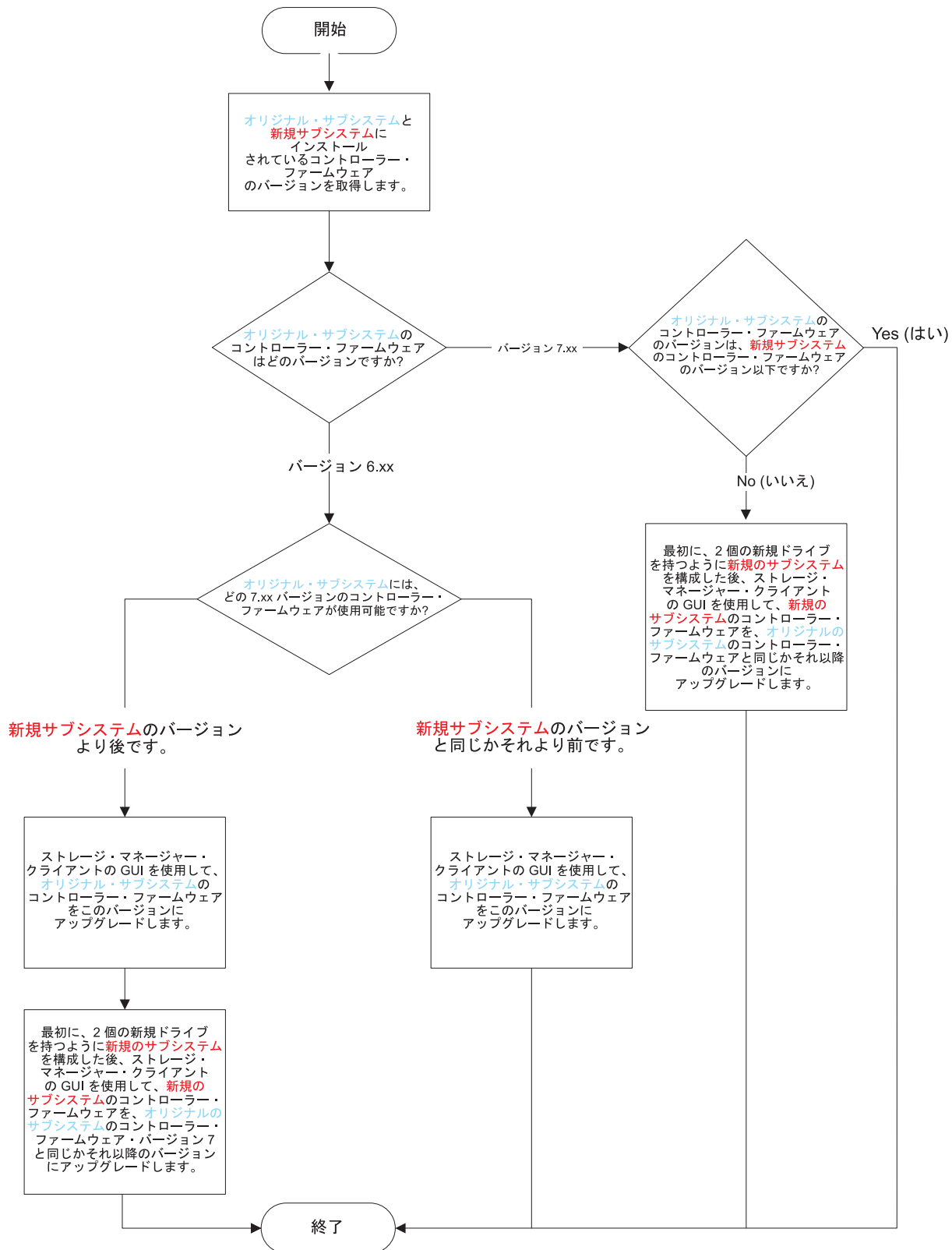
図 46. DS4700 または DS4800 から DS5000 ストレージ・サブシステムへのアップグレード用のファームウェア互換性フローチャート
