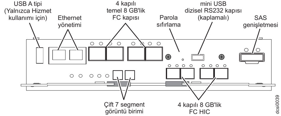
Şekil 6. Performans Modülü Denetleyicilerine sahip DCS3700 depolama altsistemindeki bağlaçlar
