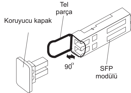
Şekil 27. SFP modülü ve koruyucu kapak
