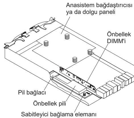
Şekil 79. Önbellek DIMM'inin yeri
