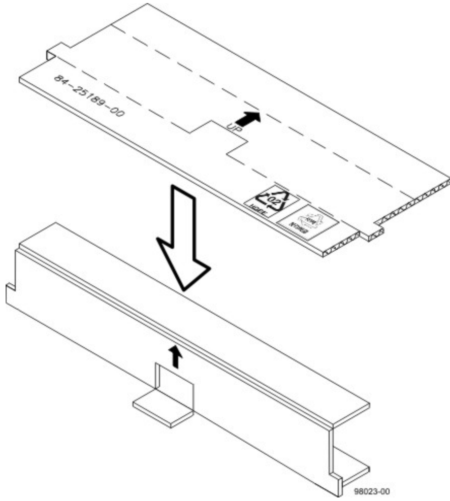
Şekil 115. Denetleyici hava yön değıştiricisi
