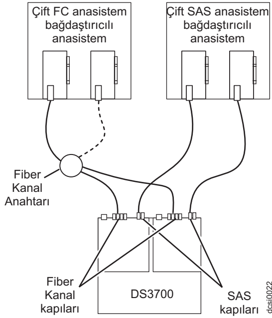
Şekil 48. Birden çok anasistemli, birden çok kapılı ve birden çok yönlüme yapısına sahip (Fiber Kanal ve SAS) bir yapılandırma örneği
