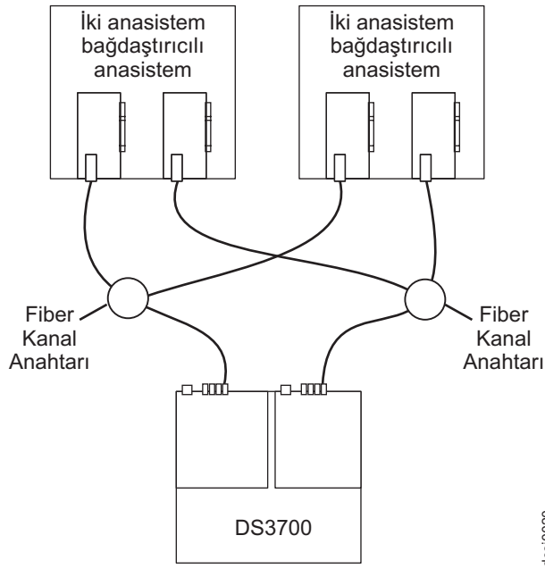
Şekil 46. Çift Fiber Kanal SAN yöneltme yapısı yapılandırması örneği
