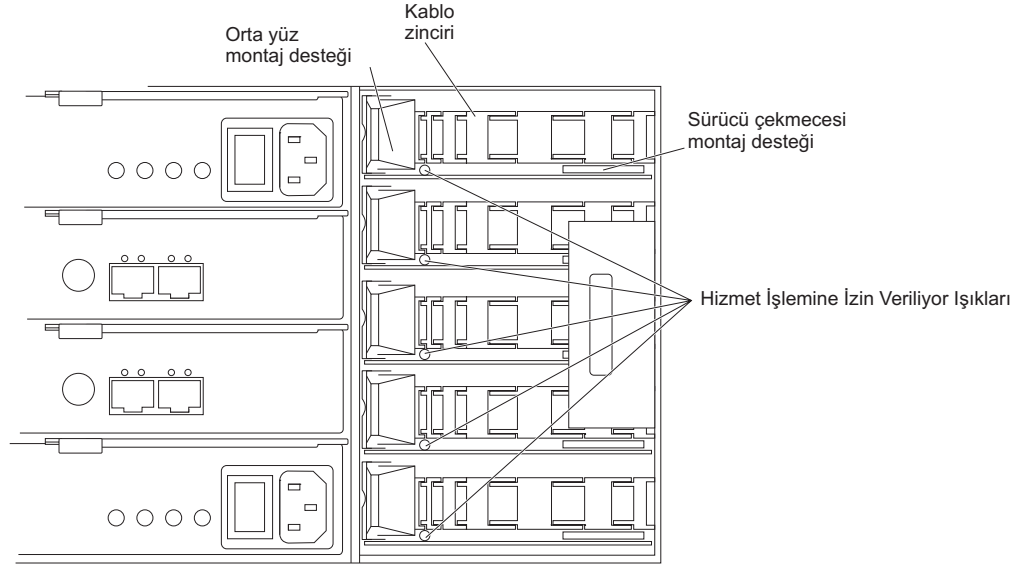
Şekil 87. Sağ fan düzeneği çıkarılmış olarak, depolama genişletme kasasının arkadan görünümü
