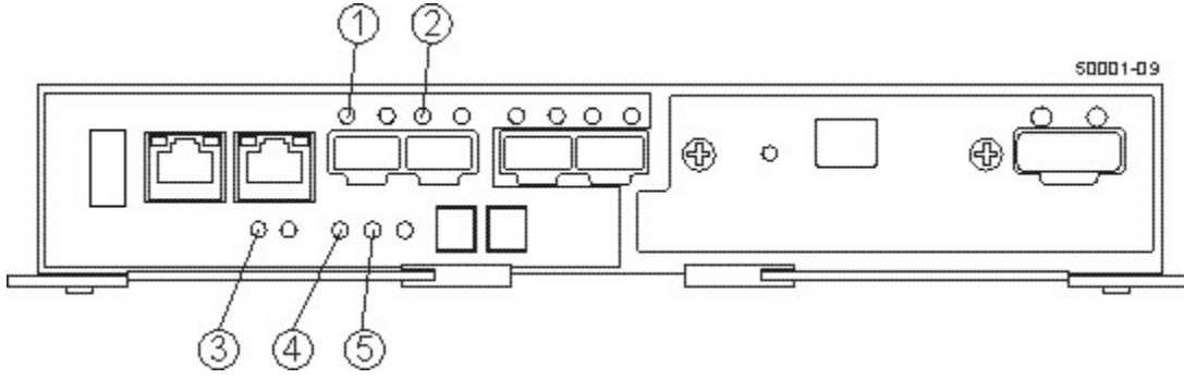
Şekil 111. Denetleyici ışıkları
