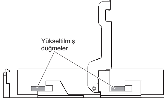
Şekil 74. Sürücüyü hizalama
