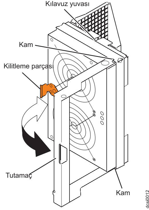
Şekil 86. Fan düzeneğini çıkarma
