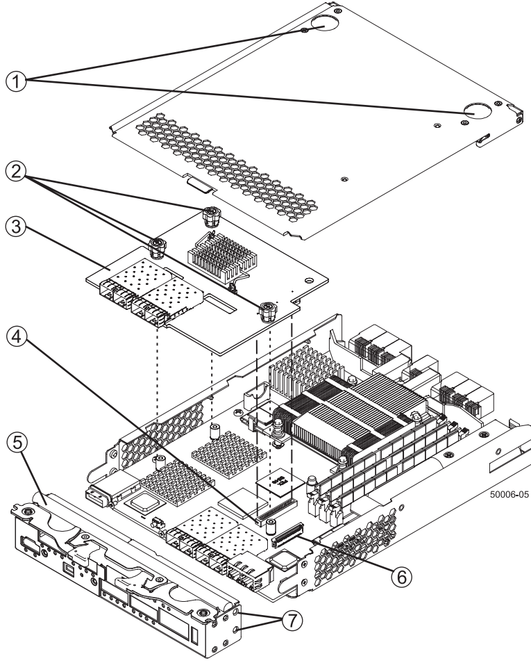
Şekil 117. Anasistem Arabirim Kartını değiştirme
