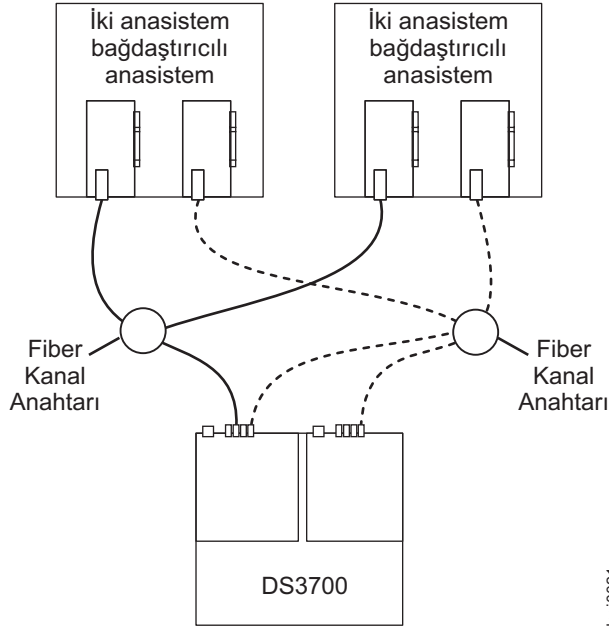
Şekil 47. Çift Fiber Kanal SAN ortamındaki iki depolama alt sistemi örneği
