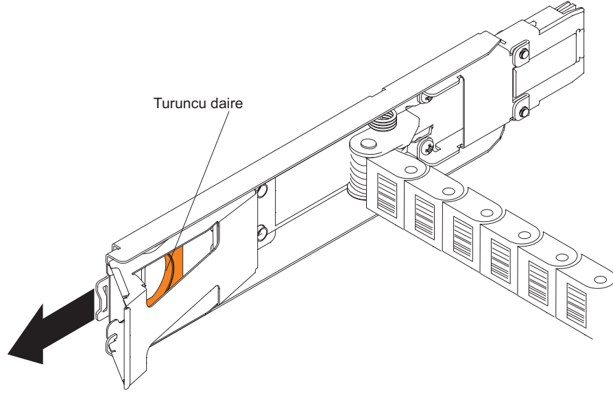
Şekil 88. Orta yüze bağlanan dikey montaj desteği
