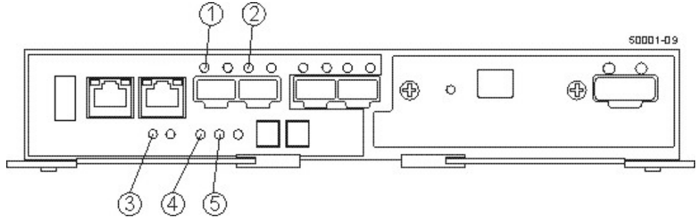
Şekil 113. Denetleyici ışıkları
