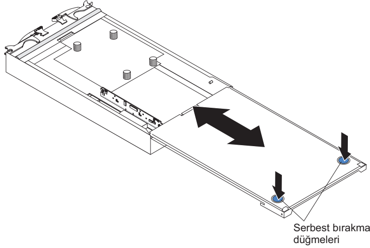
Şekil 63. Kapağın çıkarılması
