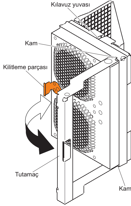
Şekil 92. Fan düzeneğini çıkarma
