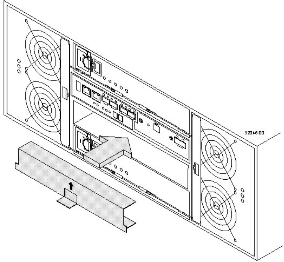
Şekil 100. Denetleyici hava yön değiştiricisinin açık denetleyici yuvasına takılması
