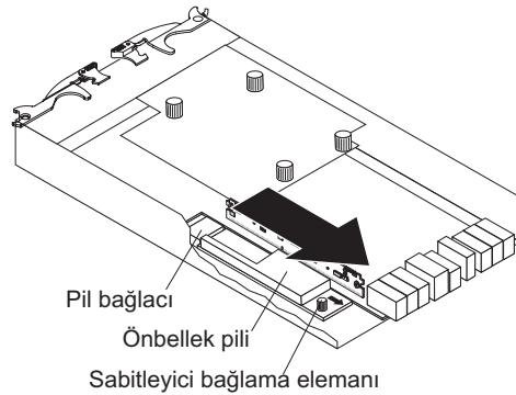
Şekil 65. Pil biriminin denetleyiciden çıkarılması
