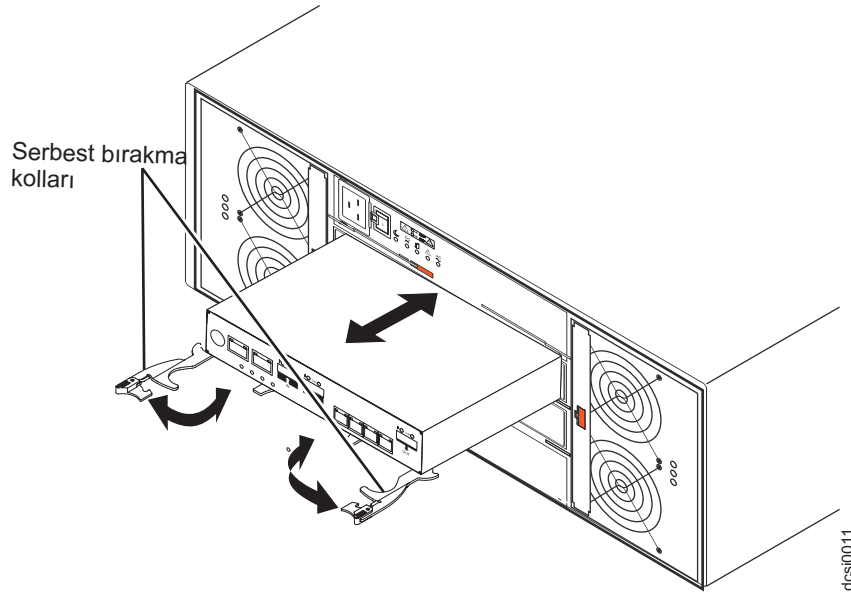
Şekil 67. Denetleyicinin çıkarılması
