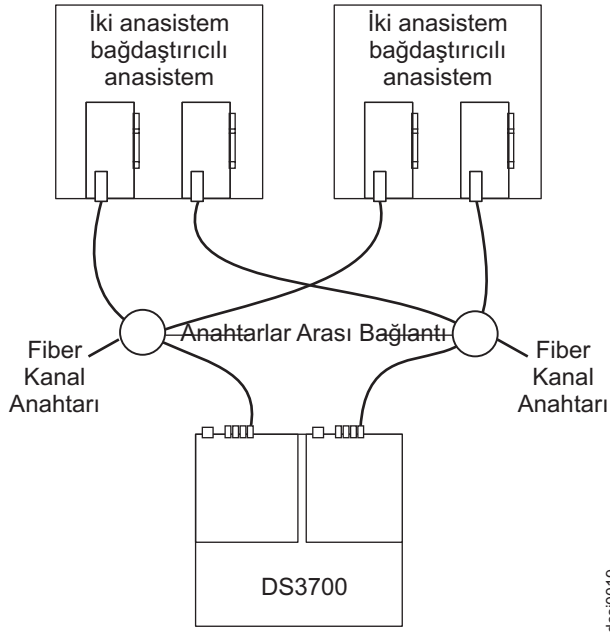
Şekil 45. Tek Fiber Kanal SAN yöneltme yapısı yapılandırması örneği
