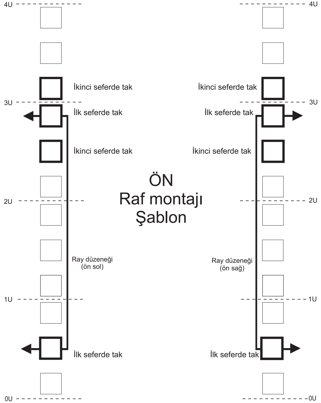
Şekil 122. Ön raf montaj şablonu
