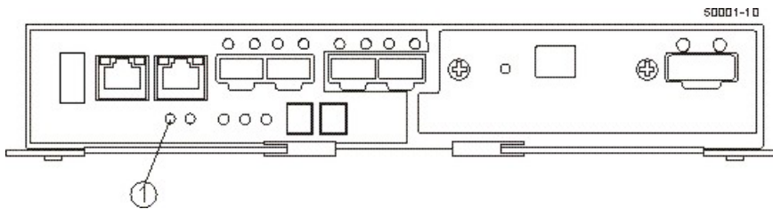
Şekil 105. Denetleyici üzerindeki Pil Hizmet İşlemi Gerekiyor Işığı
