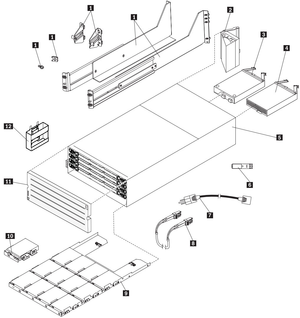
Şekil 119. DCS3700 depolama altsistem kasası parça listesi
