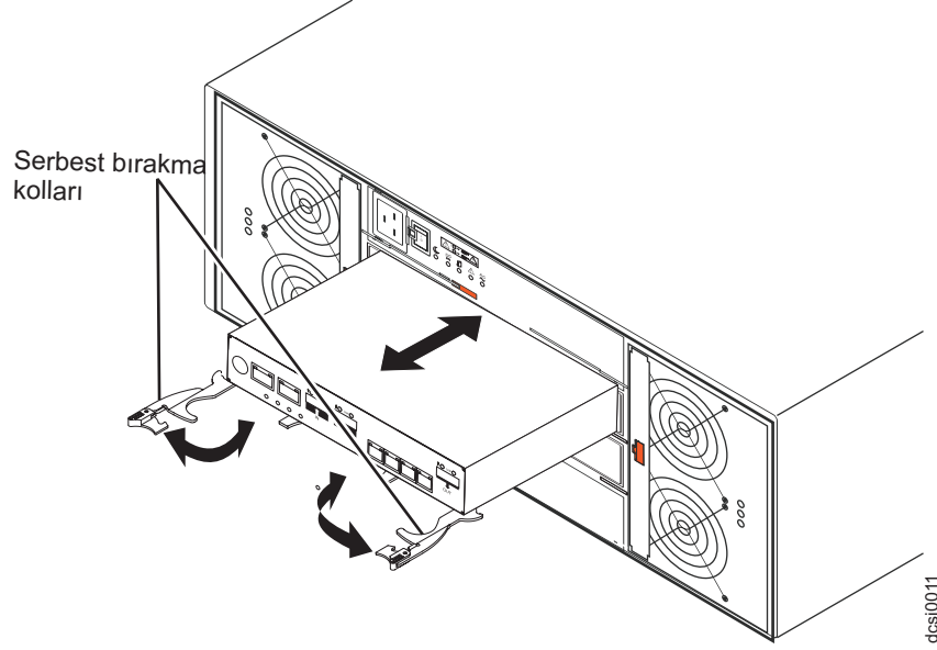
Şekil 98. Denetleyicinin çıkarılması ve geri takılması
