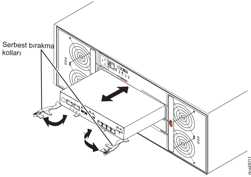
Şekil 85. Ortam hizmet modülünün çıkarılması
