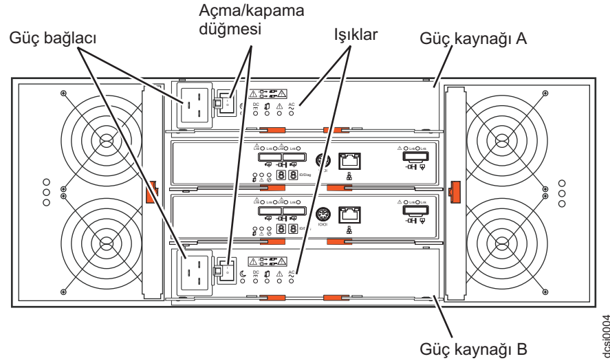
Şekil 10. Güç kaynağı bileşenleri
