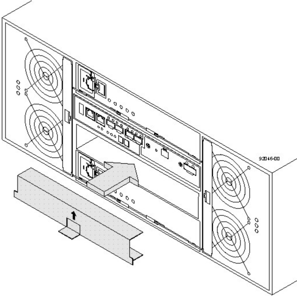
Şekil 109. Denetleyici hava yön değiştiricisinin açık denetleyici yuvasına takılması
