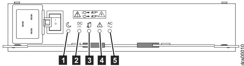
Şekil 58. AC güç kaynağı ışıkları
