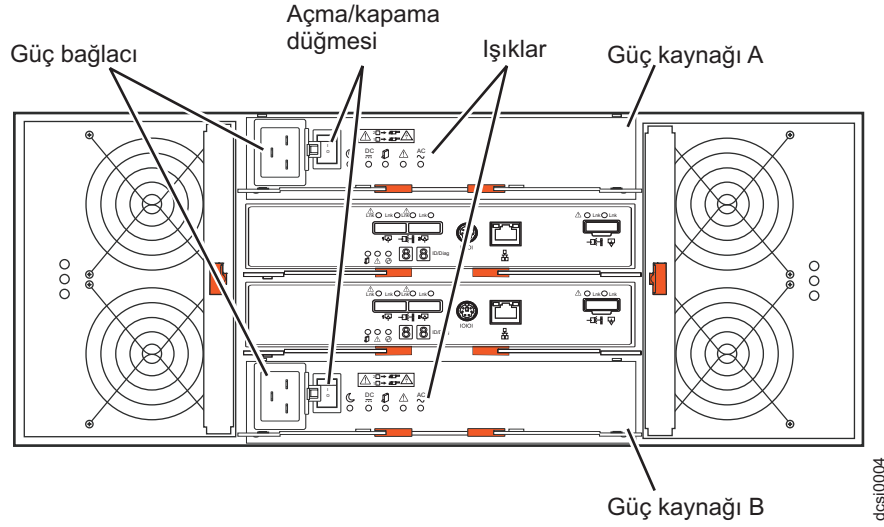
Şekil 49. DS3500 dc modellerine ilişkin güç kaynağı düğmeleri ve bağlaçlar
