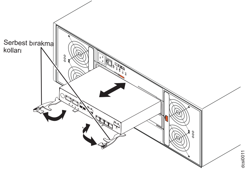
Şekil 62. Denetleyicinin çıkarılması
