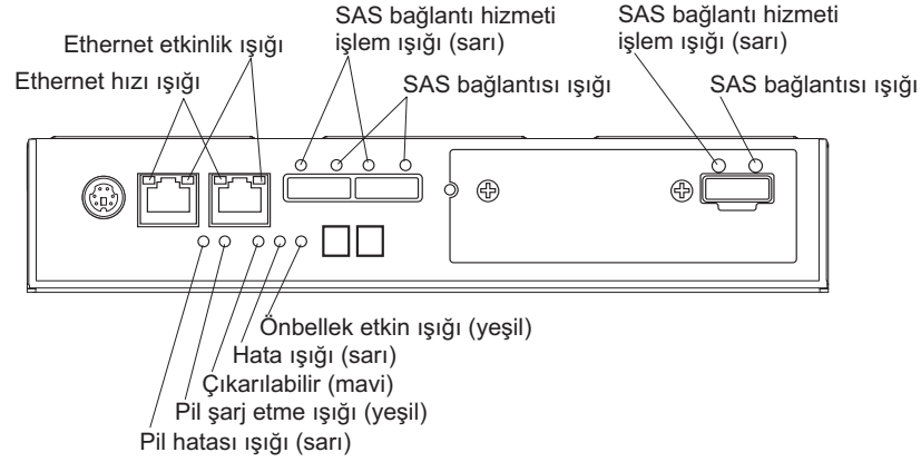
Şekil 52. Denetleyici ışıkları
