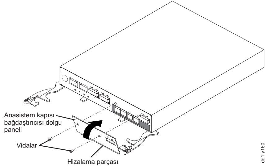
Şekil 68. Anasistem kapısı bağdaştırıcısı dolgu panelinin çıkarılması
