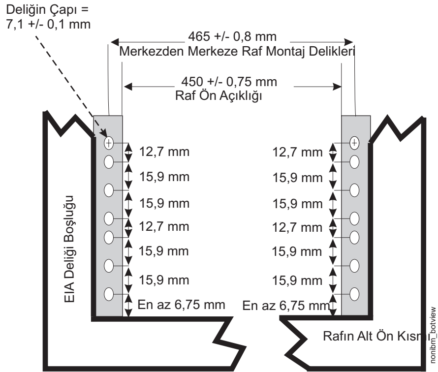
Şekil 126. Raf belirtileri boyutları, alttan ön görünüm
