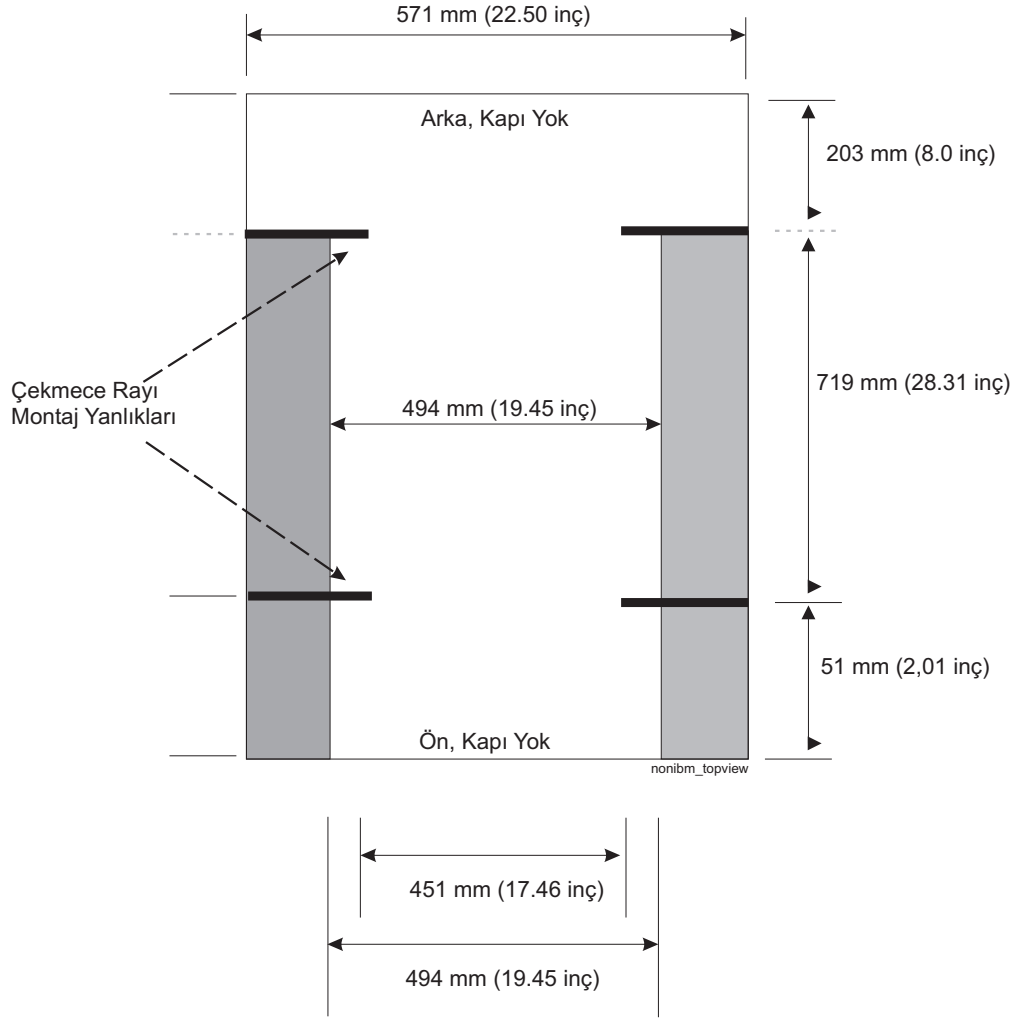
Şekil 124. IBM Ürünü Olmayan Raf Belirtileri Boyutlarının Üstten Görünümü
