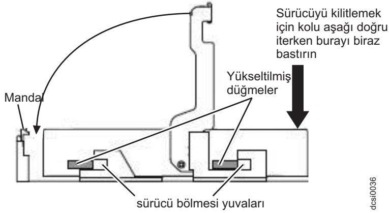
Şekil 72. Bağlaca sabit disk sürücüsü takma
