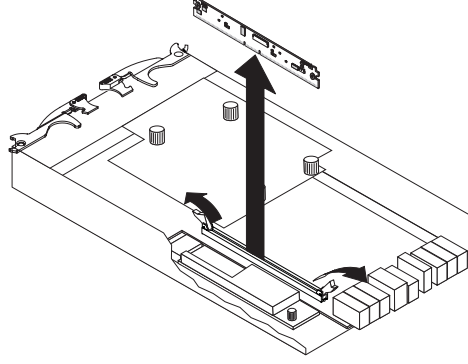
Şekil 82. DIMM'in denetleyiciye takılması
