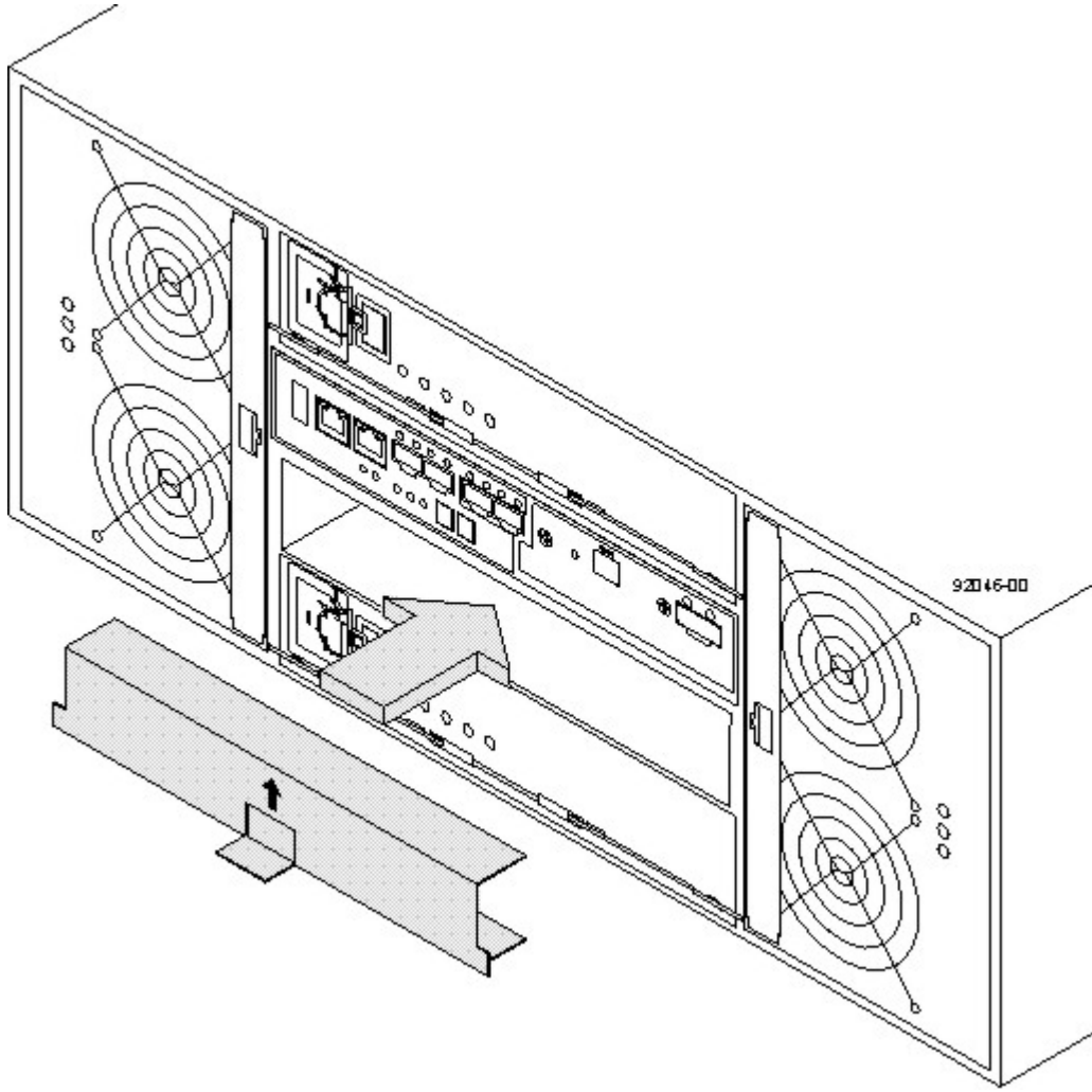
Şekil 102. Denetleyici hava yön değıştiricisinin açık denetleyici yuvasına takılması
