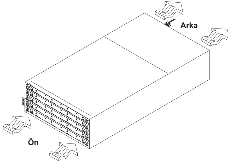
Şekil 14. DCS3700 hava akımı
