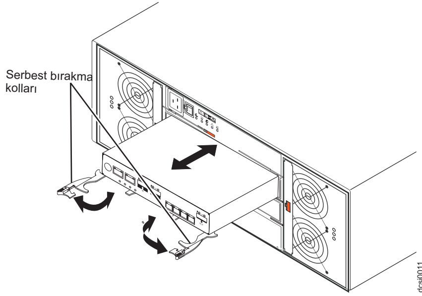
Şekil 64. Denetleyicinin çıkarılması ve geri takılması
