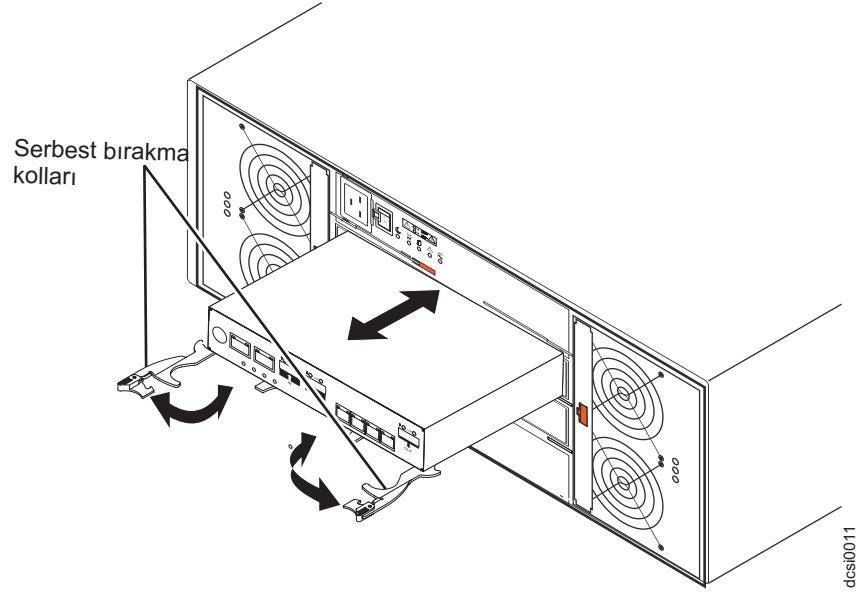
Şekil 80. Denetleyicinin çıkarılması
