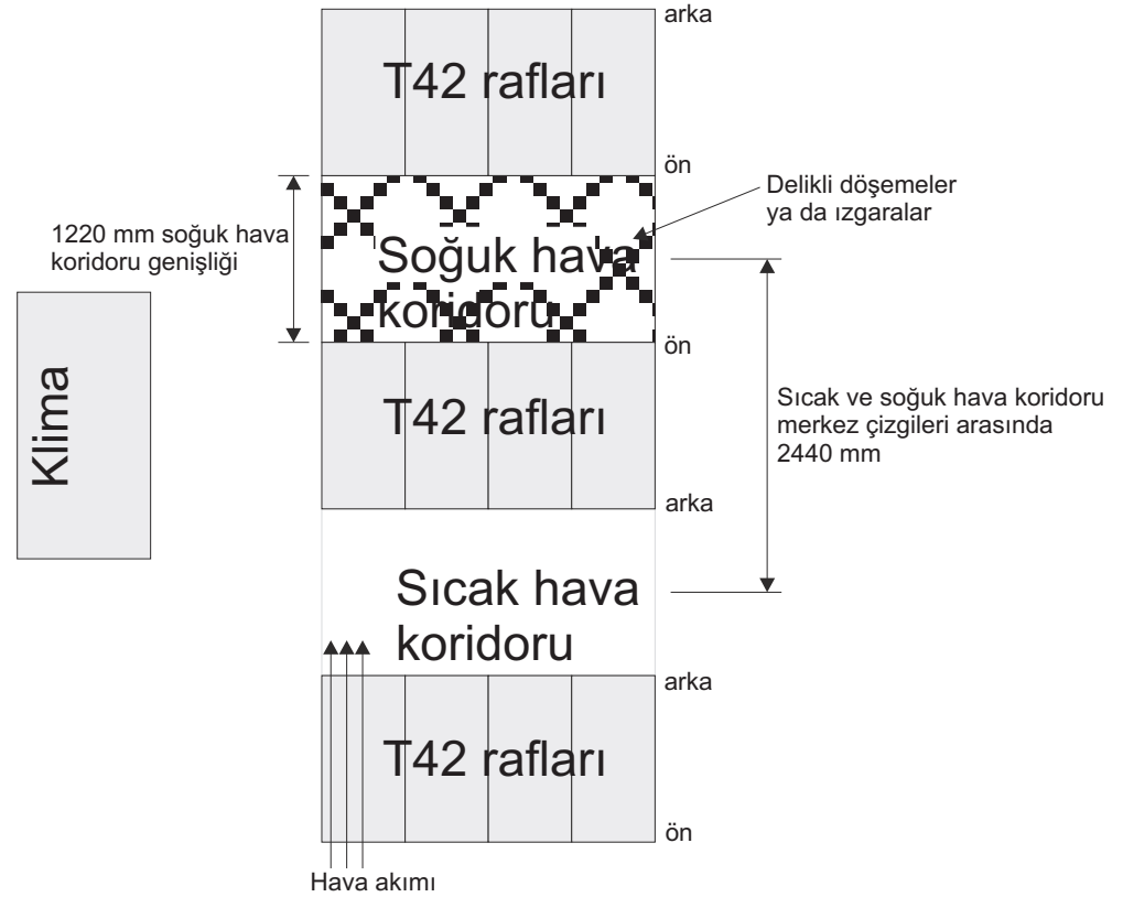
Şekil 15. Soğuk hava koridoru/sıcak hava koridoru raf yapılandırması örneği
