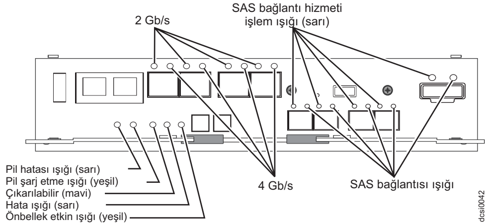
Şekil 53. Performans Modülü Denetleyicilerine sahip bir altsistemdeki denetleyici ışıkları
