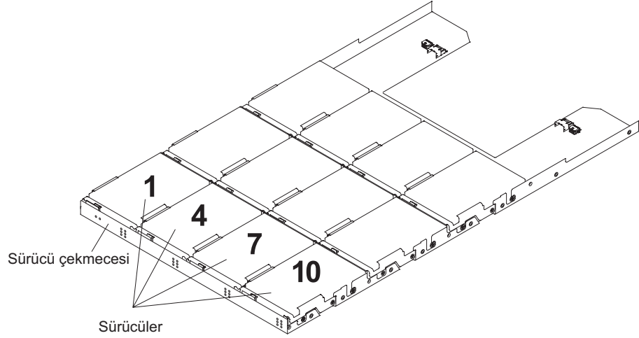
Şekil 18. etiketlenmiş disk sürücüleriyle DCS3700 sürücü çekmecesini
