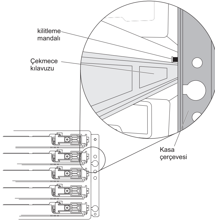
Şekil 91. Çekmece kılavuzunun üstünde bulunan kilitleme mandalı
