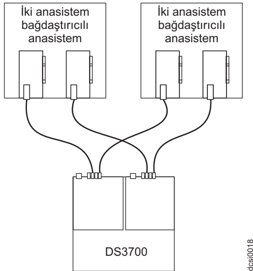
Şekil 43. Birden çok anasistemdeki birden çok HBA'ya çift denetleyicili doğrudan bağlı Fiber Kanal bağlantısı
