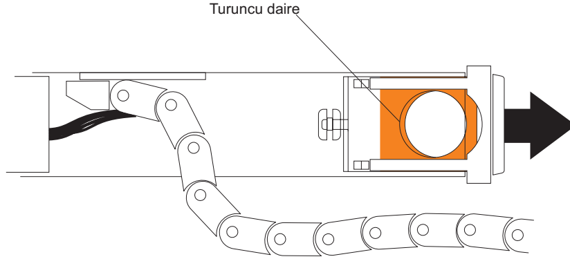
Şekil 89. Sürücü çekmecesine bağlanan yatay montaj desteği
