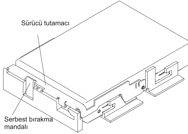
Şekil 75. Sürücüyü yerine kilitleme
