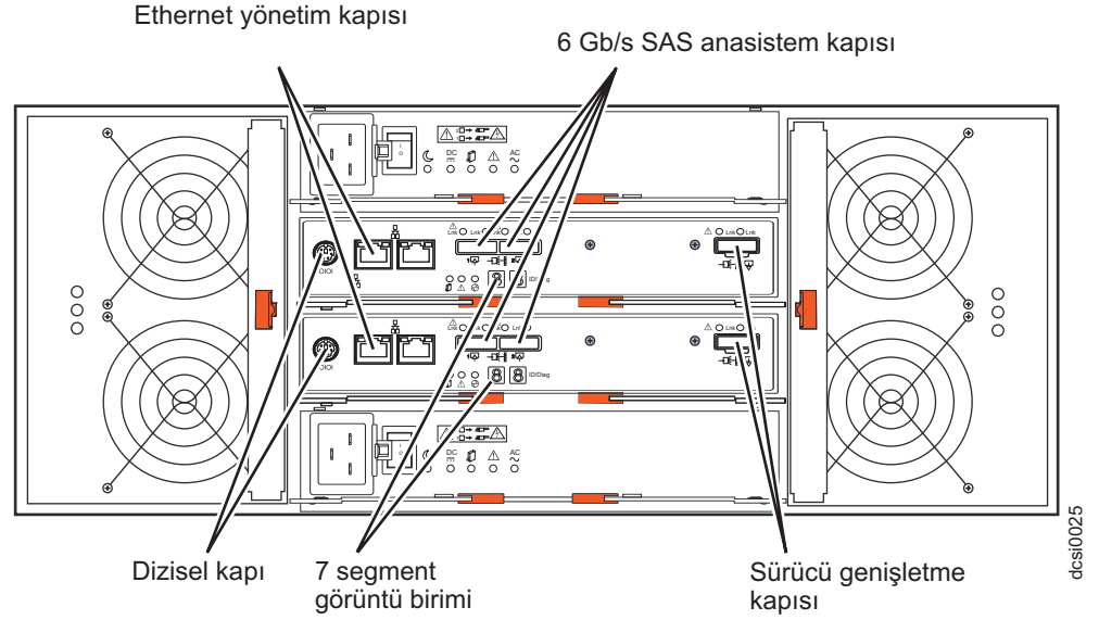
Şekil 5. DCS3700 bağlaçları
