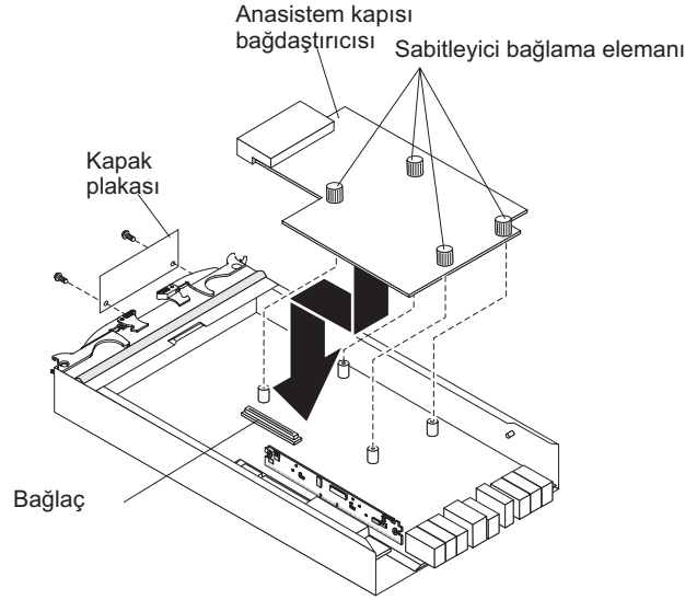
Şekil 69. Anasistem kapısı bağdaştırıcısının takılması
