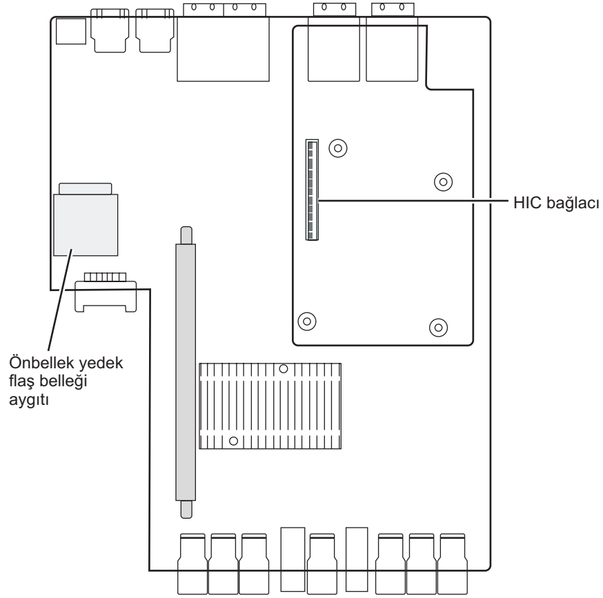
Şekil 70. HIC bağlacını hizalama
