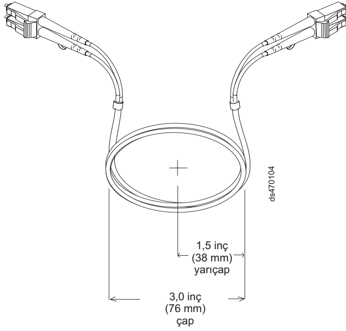
Şekil 31. Fiber optik kablolarla ilişkin önerilen bükülme ve döngü belirtileri
