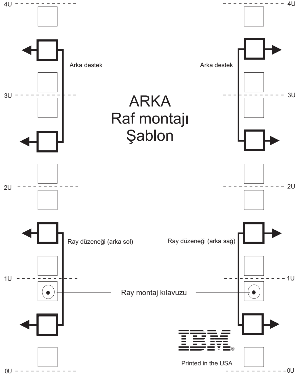
Şekil 123. Arka raf montaj şablonu
