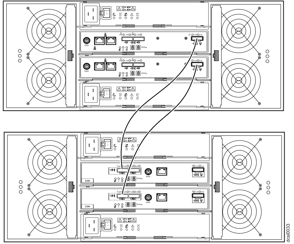
Şekil 38. Tekli Genişletme Kasaları
