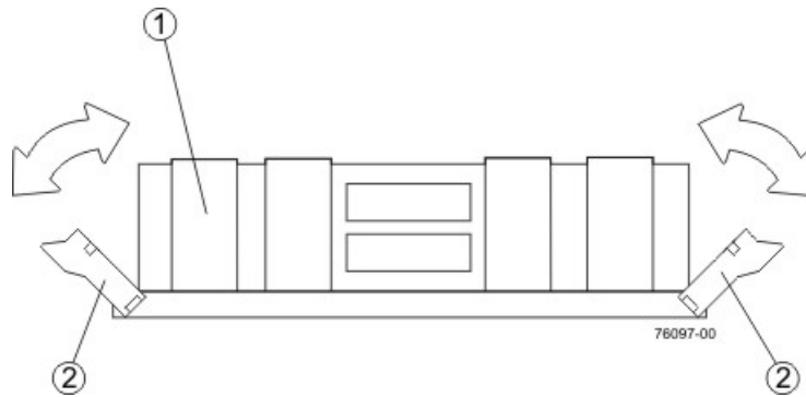
Şekil 104. Ön bellek DIMM'inin çıkarılması
