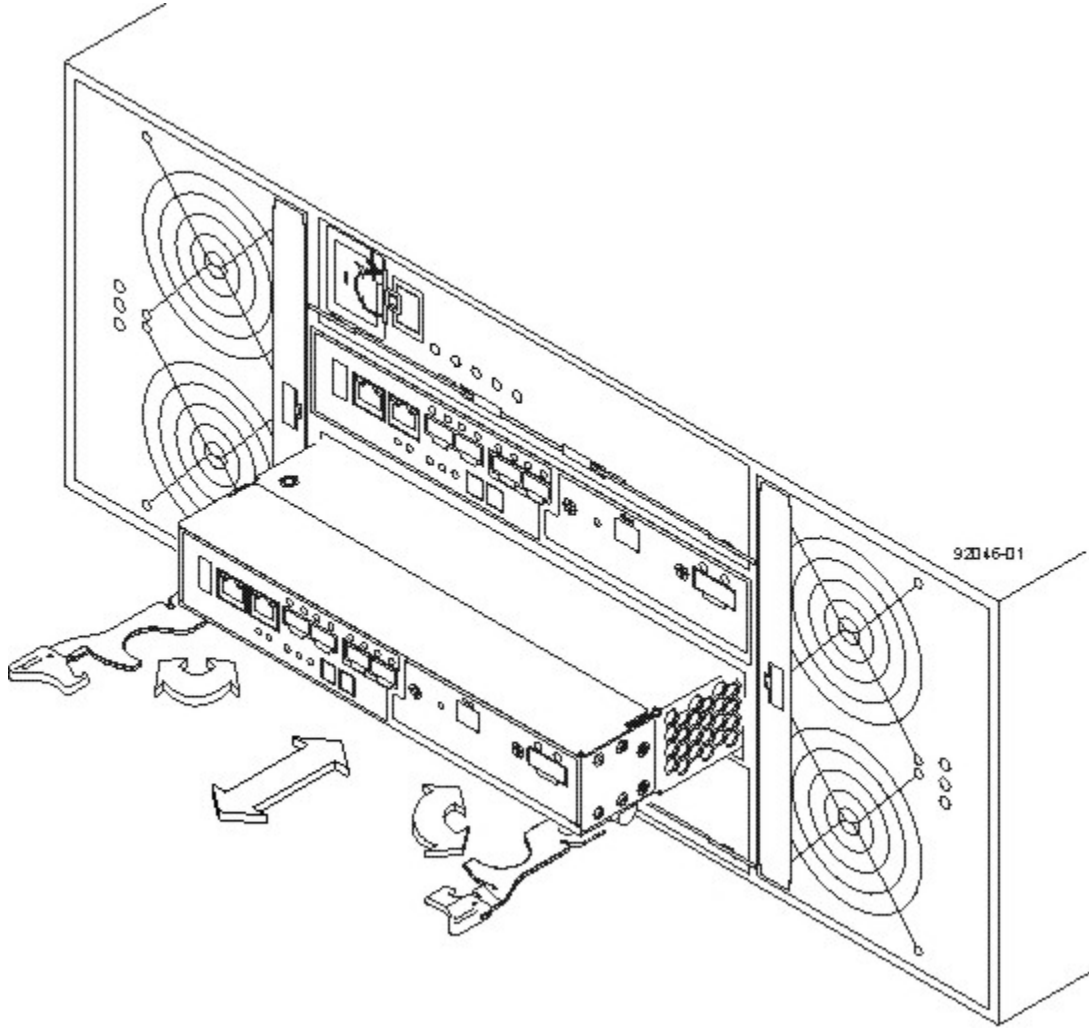
Şekil 107. Denetleyicinin çıkarılması ve geri takılması
