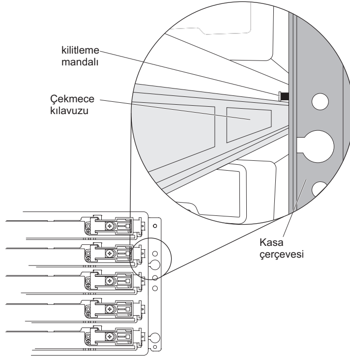
Şekil 97. Çekmece kılavuzunun üstünde bulunan kilitleme mandalı
