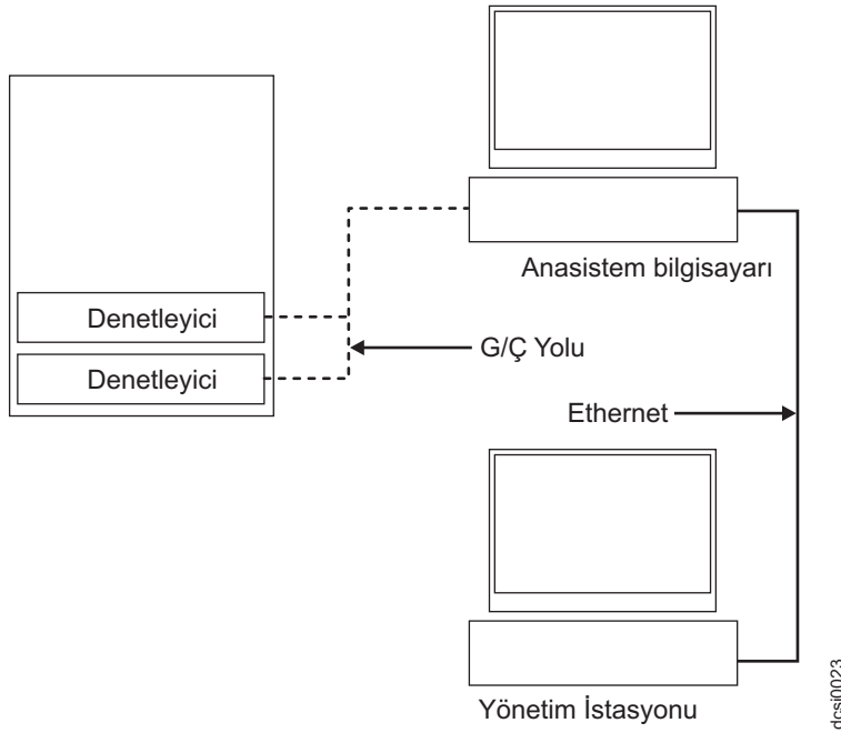
Şekil 40. Anasistem-Aracı (Bant İçi) Yönetim
