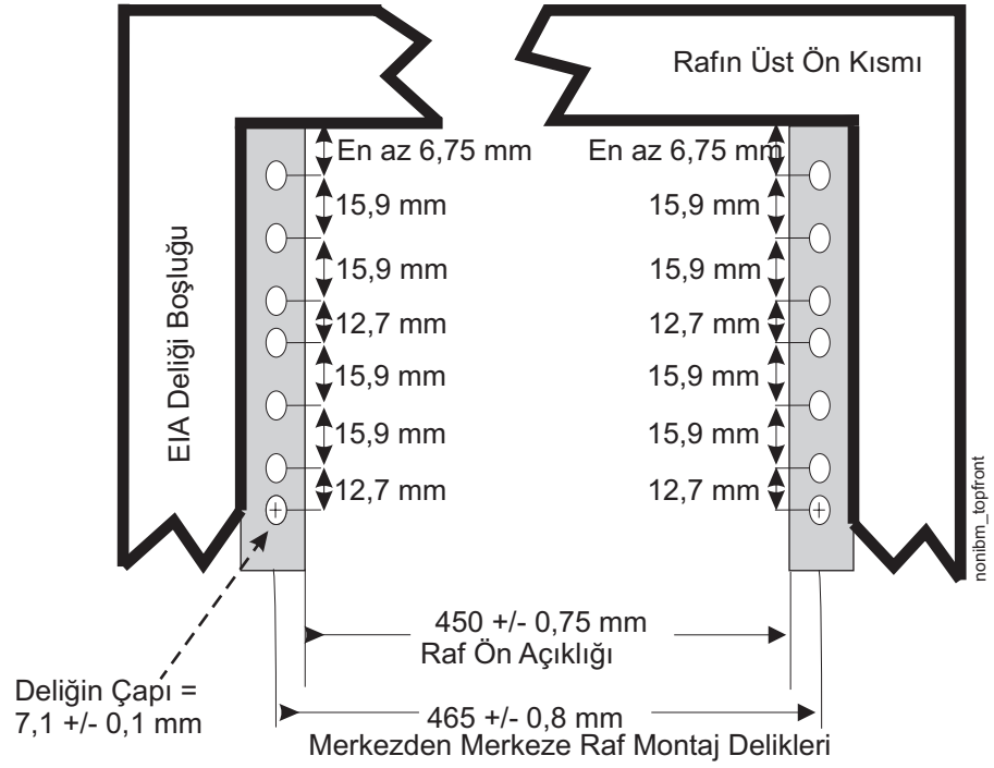
Şekil 125. Raf belirtileri boyutları, üstten ön görünüm
