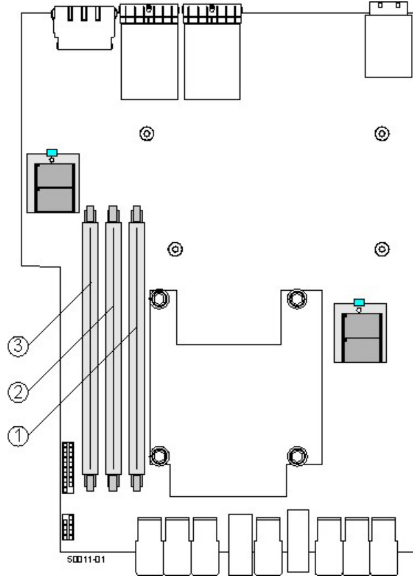
Şekil 103. Üç ön bellek DIMM yuvası
