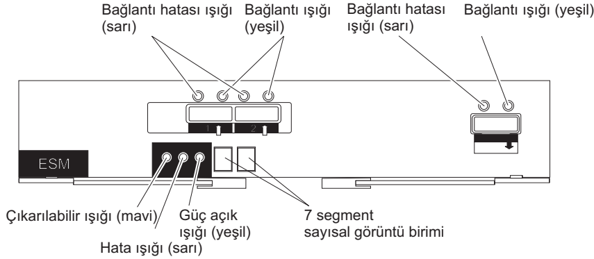
Şekil 56. ESM ışıkları
