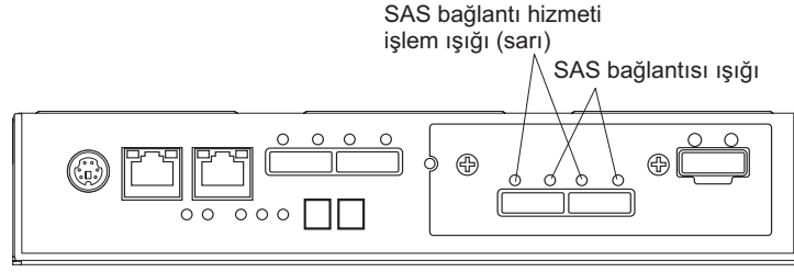
Şekil 55. SAS anasistem kapısı bağdaştırıcısı ışıkları
