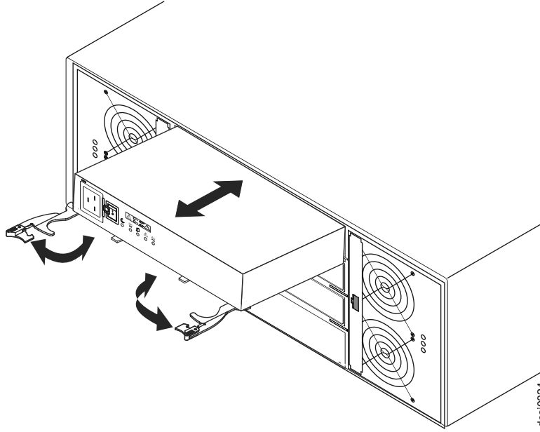
Şekil 76. Güç kaynağının değiştirilmesi
