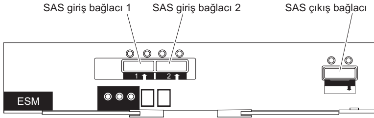
Şekil 37. ESM bağlaçları
