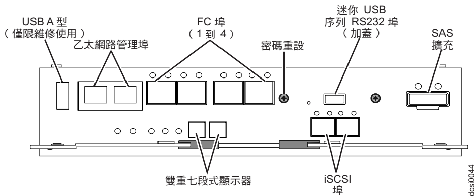
圖 21. 含有效能模組控制器的 DCS3700 儲存體系系統（列出 FC 埠）
