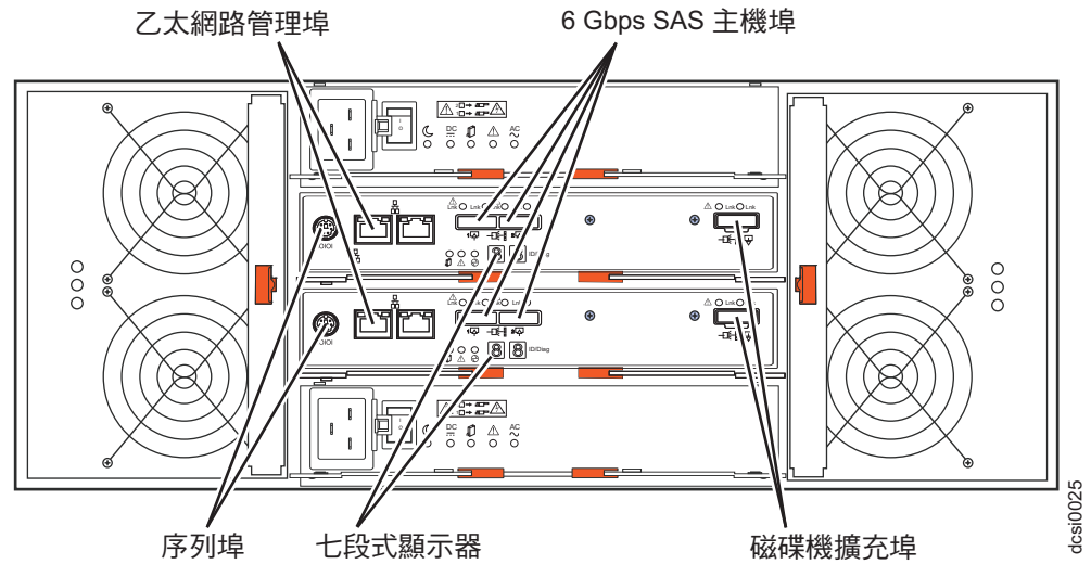
圖 5. DCS3700 接頭
