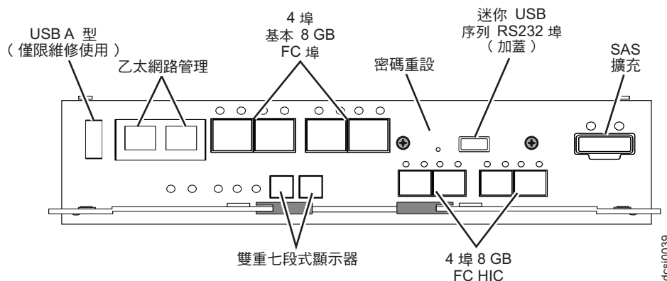
圖 23. 配有效能模組控制器的 DCS3700 子系統上的 FC HIC 埠
