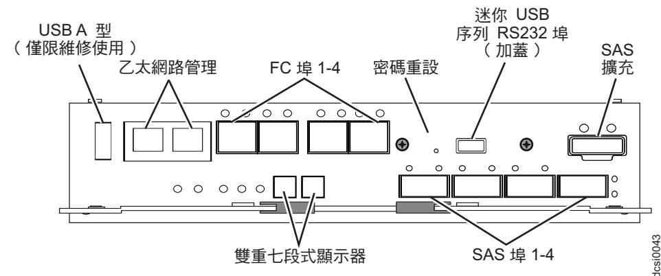
圖 20. 配有效能模組控制器的 DCS3700 儲存體子系統（列示為 SAS 擴充的 SAS 埠）
