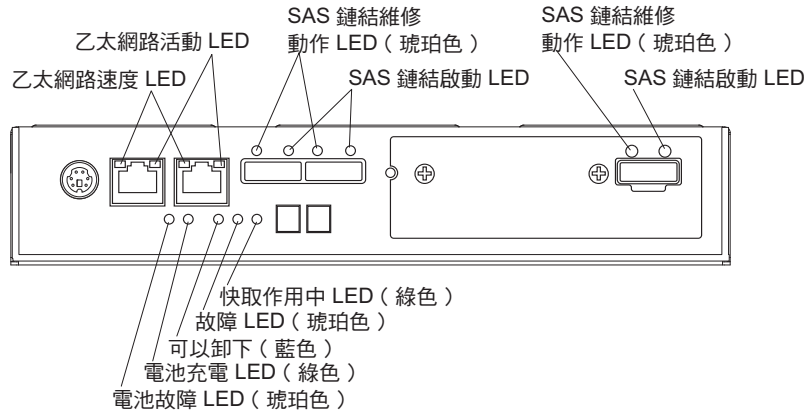
圖 52. 控制器 LED
