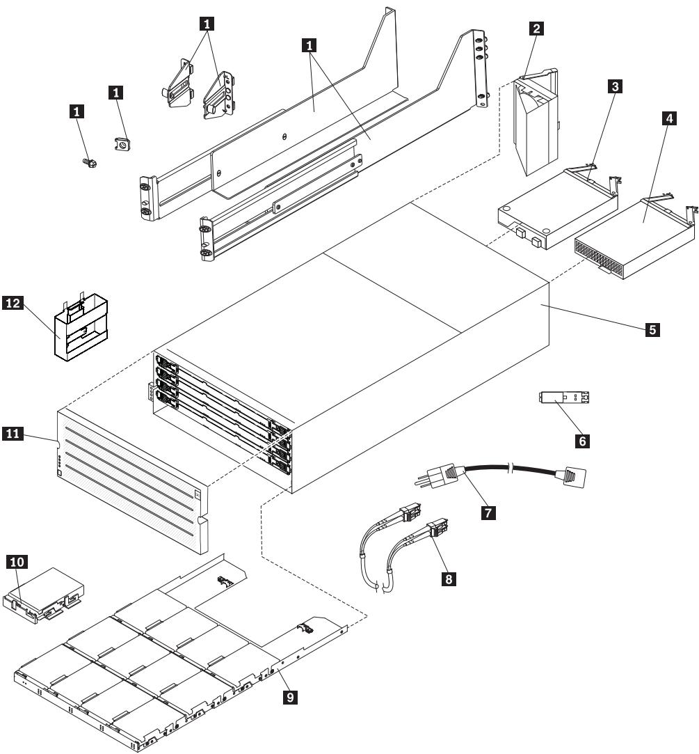
圖 119. DCS3700 儲存體子系統機體零件清單
