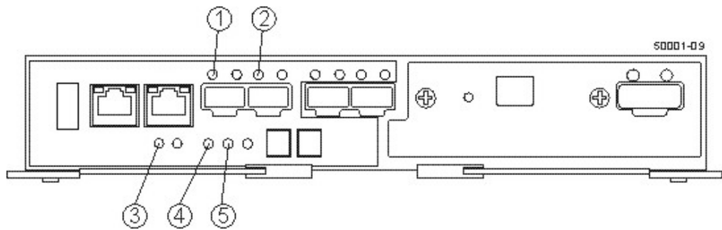
圖 113. 控制器 LED
