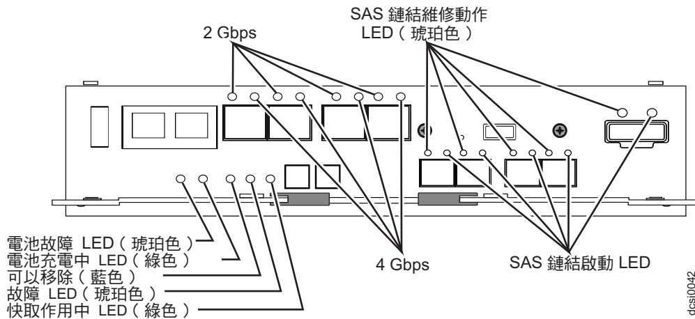
圖 53. 配有效能模組控制器的子系統上的控制器 LED
