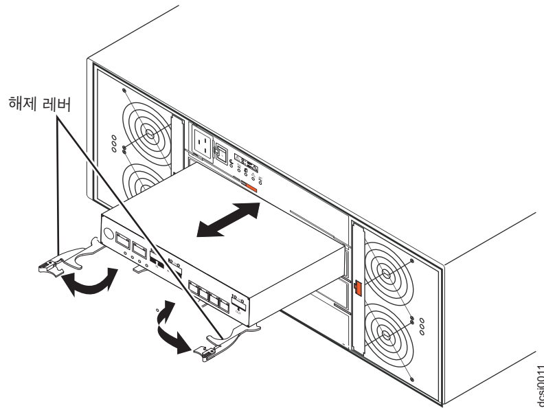
그림 67. 제어기 제거
