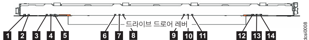
그림 59. 드라이브 드로어 LED
