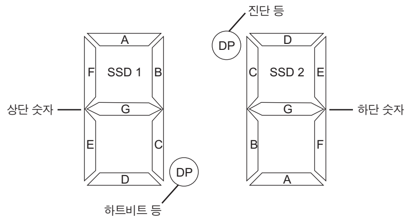
그림 61. 숫자 표시 LED
