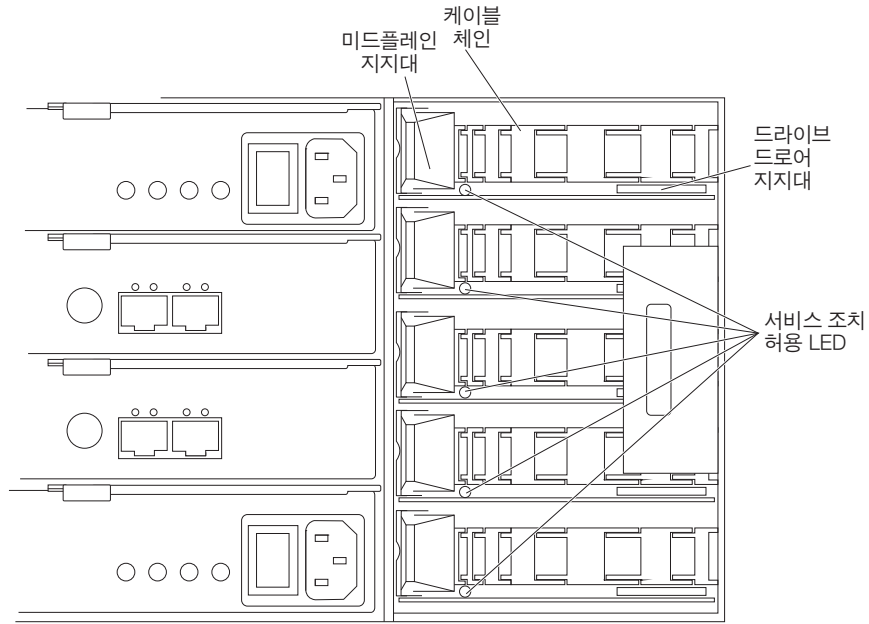
그림 93. 오른쪽 팬 조립품이 제거된 스토리지 확장 격납장치의 뒷면 보기
