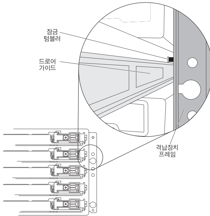
그림 91. 드로어 가이드 위에 있는 잠금 텀블러
