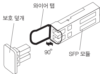
그림 30. SFP 모듈 결쇠 잠금 해제 - 와이어 유형
