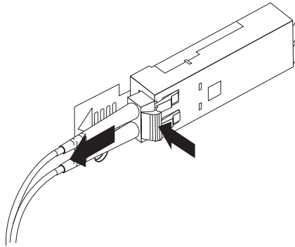
그림 36. LC-LC 파이버 채널 케이블 제거
