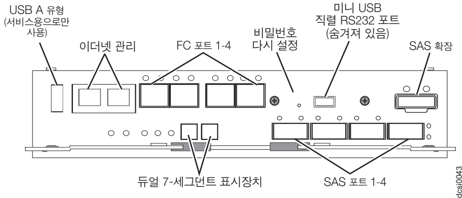
그림 20. 성능 모듈 제어기가 있는 DCS3700 스토리지 서브시스템(SAS 확장으로 나열된 SAS 포트)
