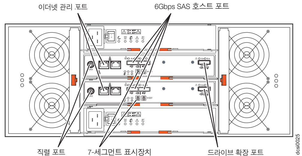
그림 5. DCS3700 커넥터
