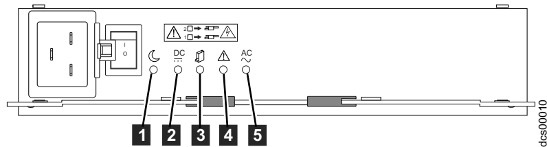
그림 58. AC 전원 공급 장치 LED
