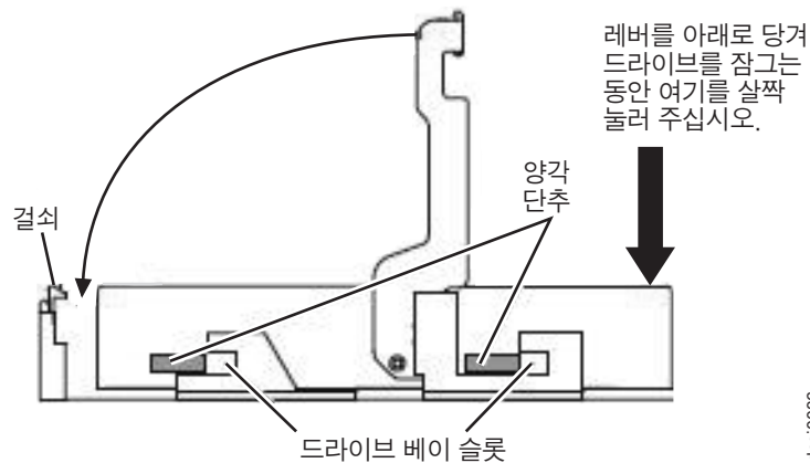
그림 72. 커넥터에 하드 디스크 드라이브 삽입
