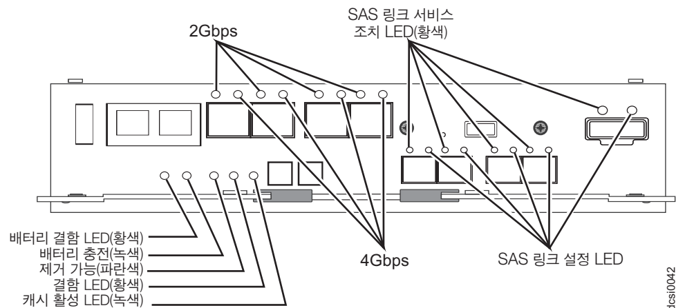
그림 53. 성능 모듈 제어기가 있는 서브시스템의 제어기 LED
