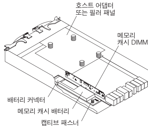
그림 7. 캐시 배터리 및 메모리 캐시 DIMM 위치
