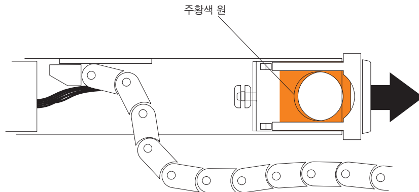
그림 95. 드라이브 드로어에 연결하는 수평 지지대
