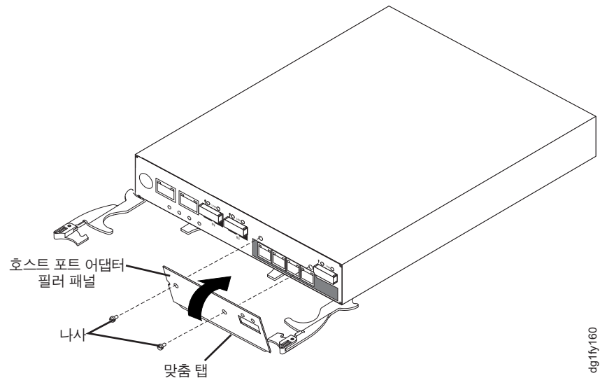
그림 68. 호스트 포트 어댑터 필터 패널 제거
