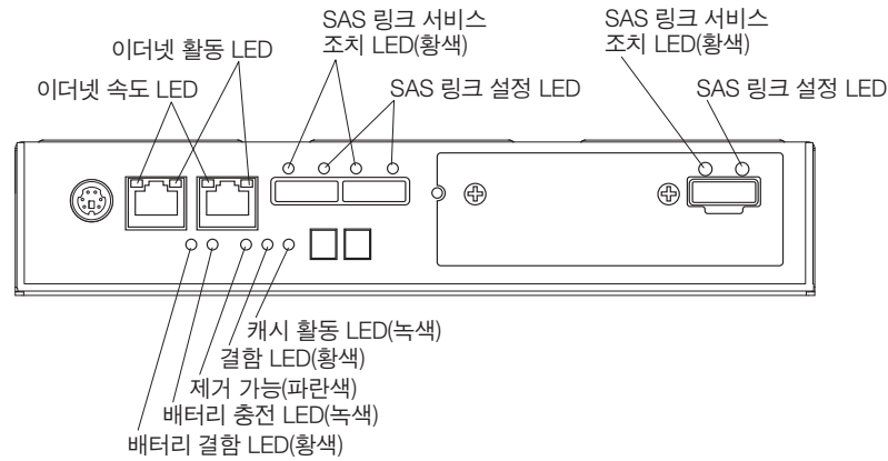
그림 52. 제어기 LED
