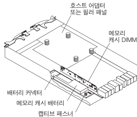
그림 79. 메모리 캐시 DIMM 위치
