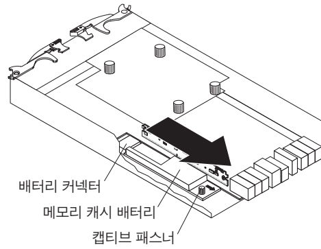
그림 65. 제어기에서 배터리 장치 제거
