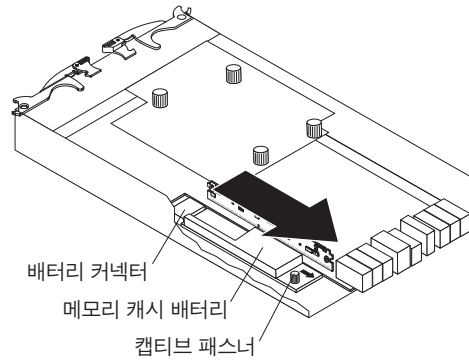
그림 78. 제어기에서 배터리 장치 제거
