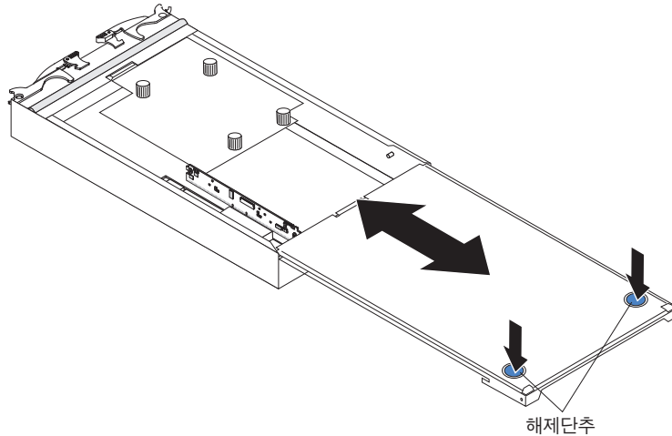
그림 63. 덮개 제거
