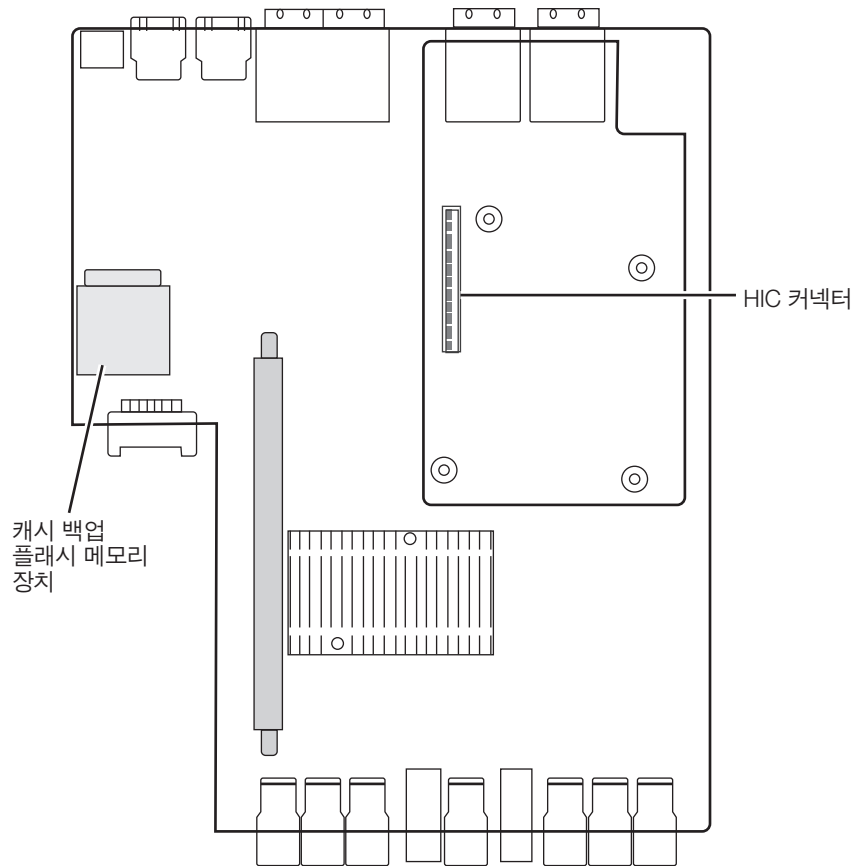
그림 70. HIC 커넥터 맞추기
