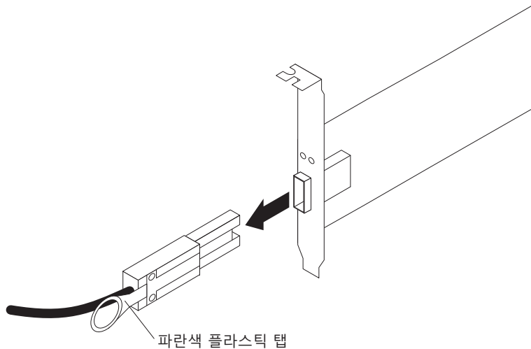
그림 26. Mini-SAS 케이블 제거
