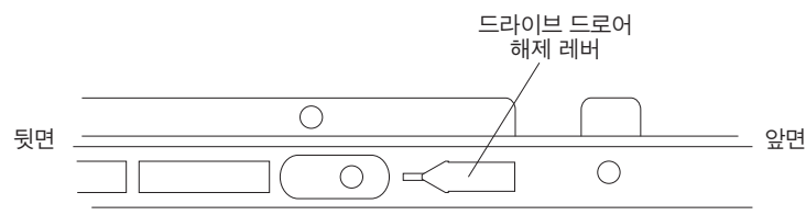
그림 90. 드라이브 드로어 옆면에 있는 드라이브 드로어 해제 레버
