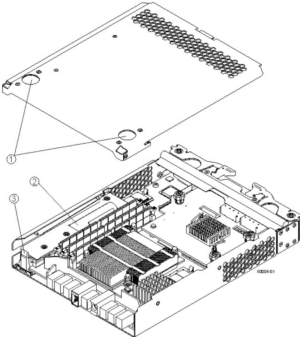
그림 110. 제어기 상단 덮개 결쇠 버튼
