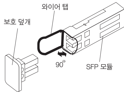
그림 28. 호스트 포트에 SFP 모듈 설치
