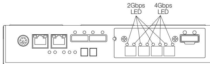
그림 54. 파이버 채널 호스트 포트 어댑터 LED
