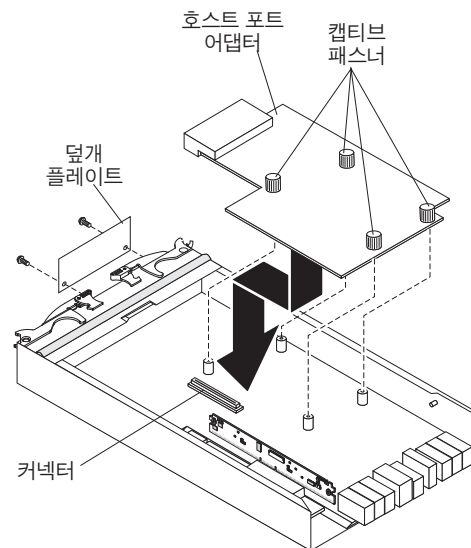
그림 69. 호스트 포트 어댑터 설치
