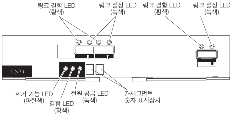
그림 56. ESM LED
