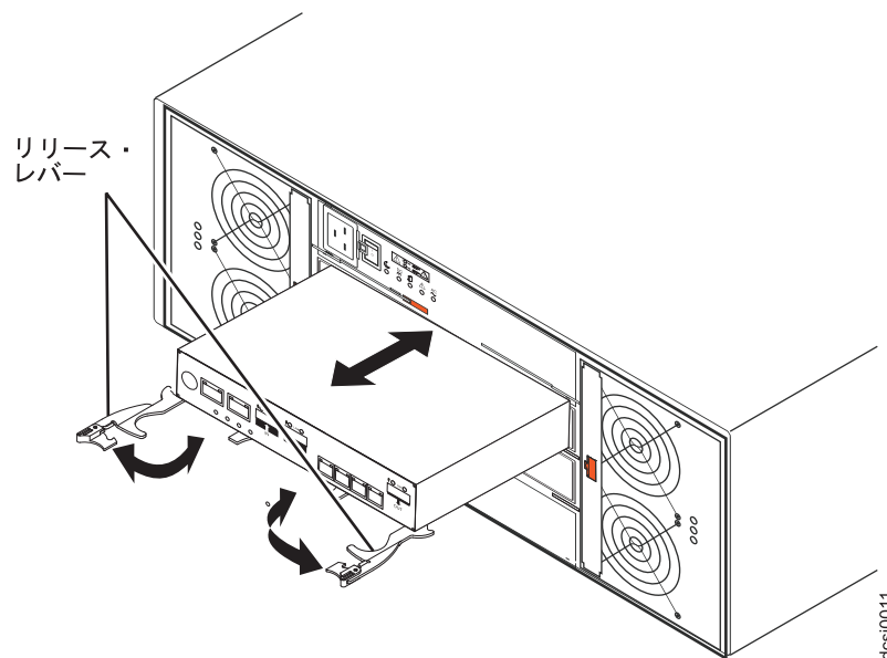
図 98. コントローラーの取り外しと交換
