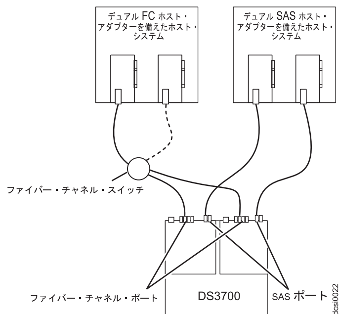
図 48. 複数ホスト、複数ポート、および複数ファブリック（ファイバー・チャンネルおよび SAS）構成の例
