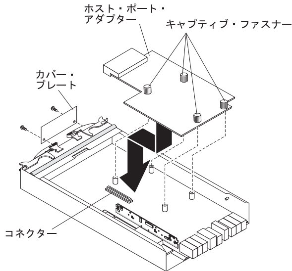
図 69. ホスト・ポート・アダプターの取り付け
