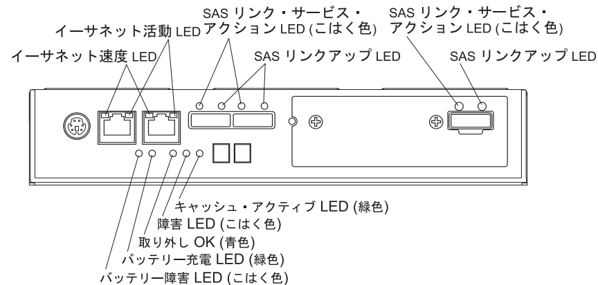
図 52. コントローラー LED
