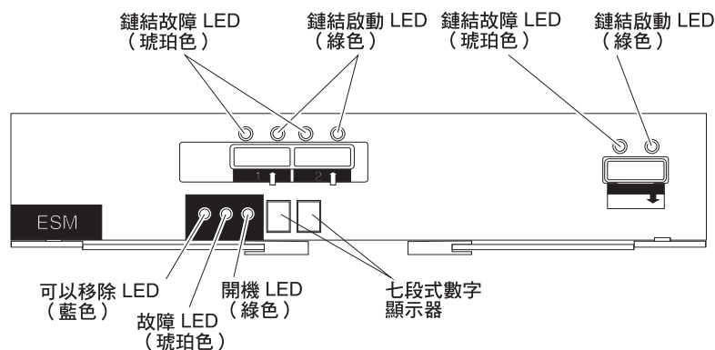
圖 87. ESM LED
