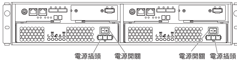
圖 111. DS3500 DC 型號的電源供應器開關及接頭
