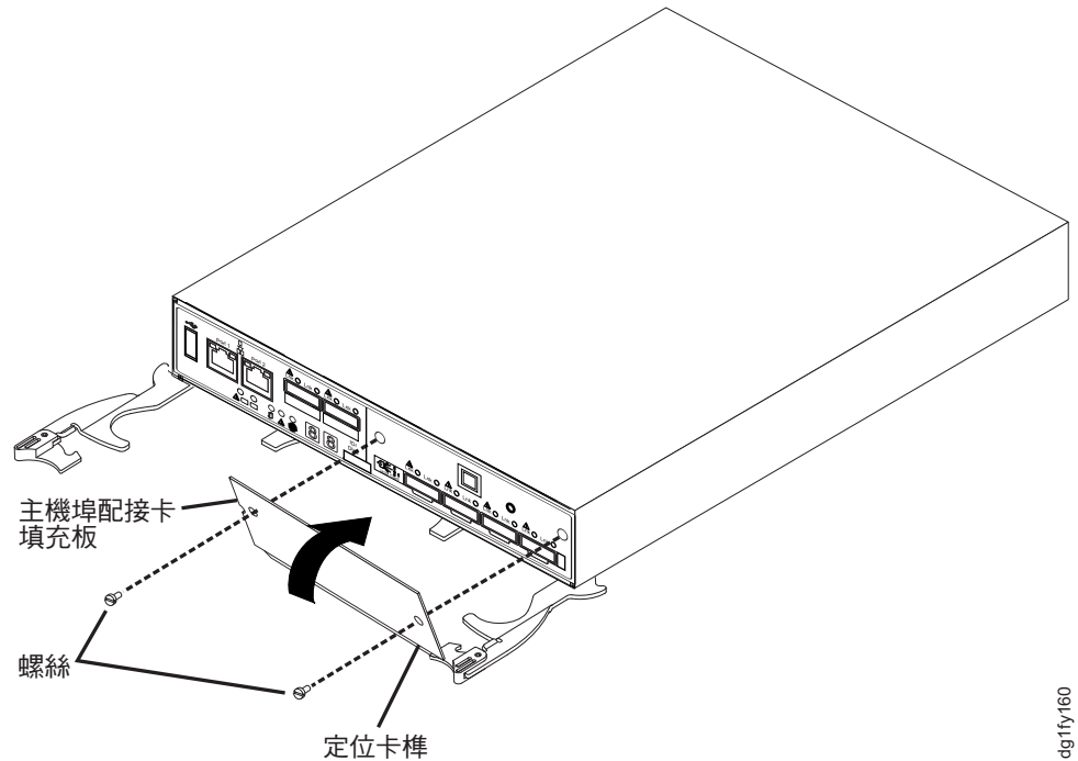
圖 96. 卸下主機埠配接卡填充板
