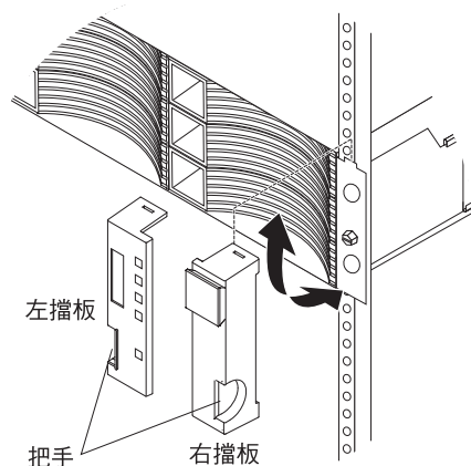
圖 122. 卸下隔板
