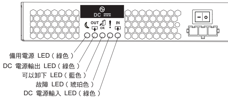
圖 110. DS3500 DC 型號的 DC 電源接頭
