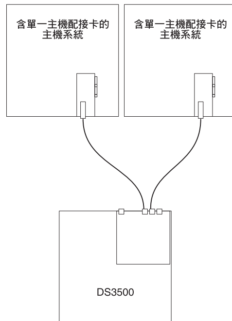
圖 58. 多個主機中單一 HBA 的單控制器直接連接型「光纖通道」連線
