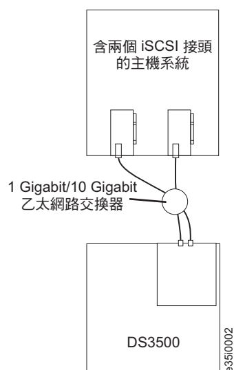
圖 65. 多個埠、單控制器 iSCSI 配置
