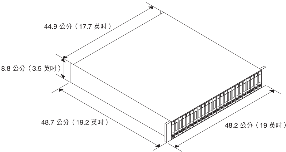
圖 14. DS3524 儲存體子系統和 EXP3524 儲存體機體尺寸
