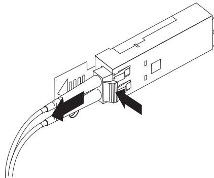
圖 31. 拔掉「LC-LC 光纖通道」纜線
