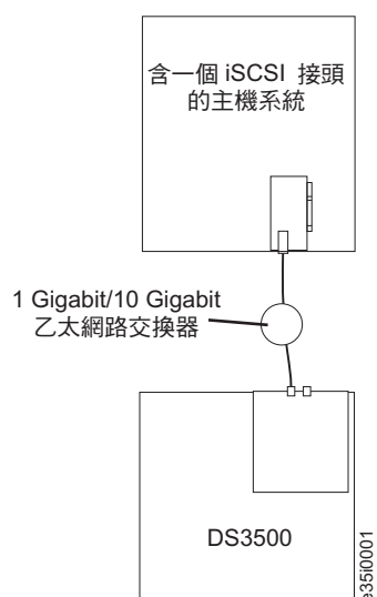
圖 64. 單一主機、單控制器 iSCSI 配置
