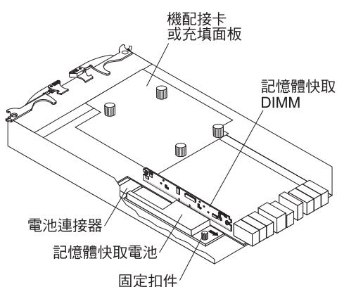
圖 12. 電池裝置
