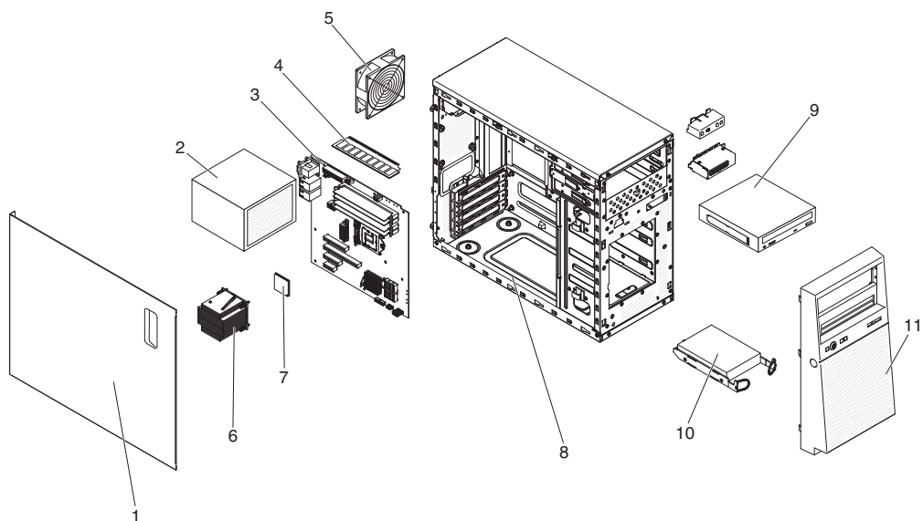
圖 12. 伺服器元件
