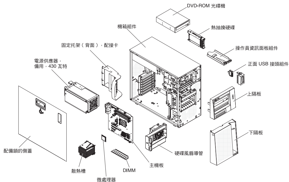
圖 6. 5U 伺服器的伺服器元件
