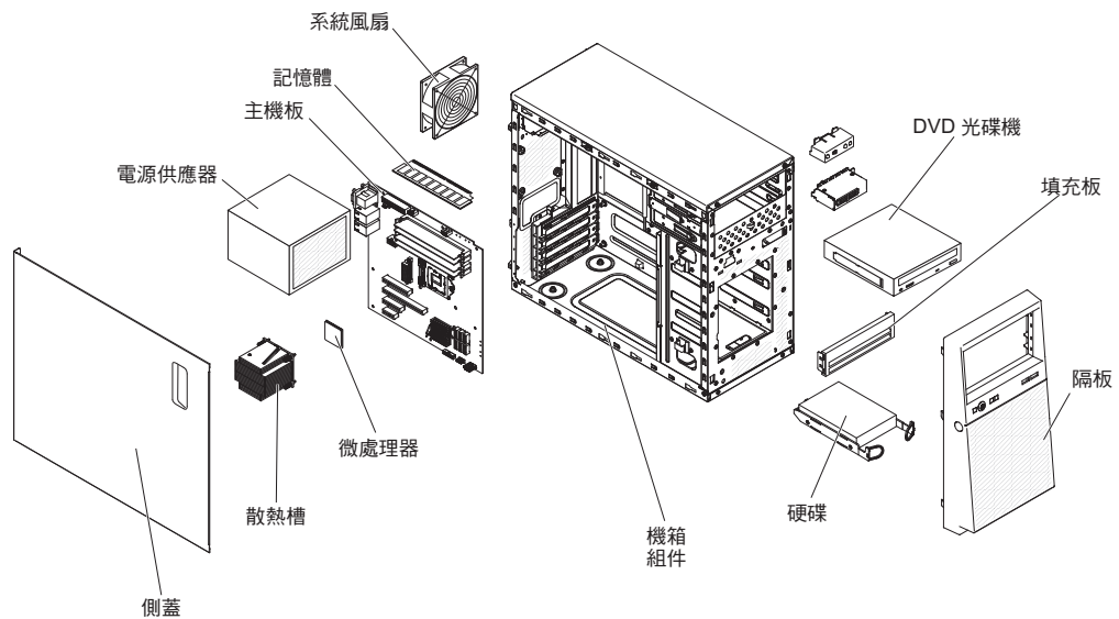
圖 5. 4U 伺服器的伺服器元件
