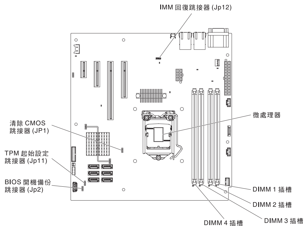
圖 9. 開關及跳接器的位置和說明
