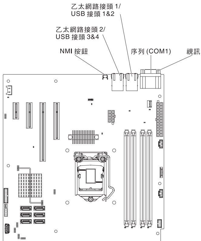
圖 8. 主機板上的外部接頭
