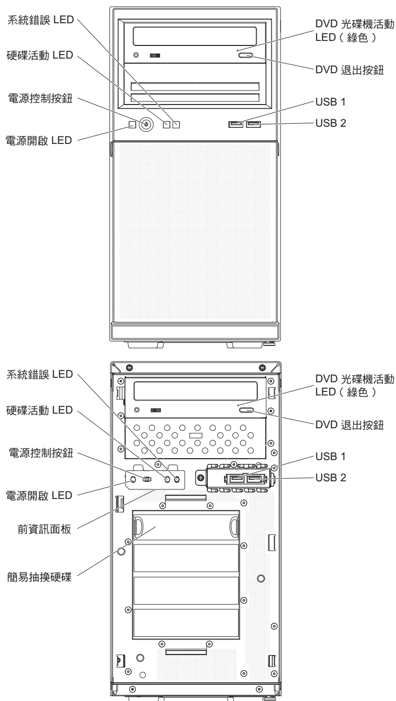
圖 1. 伺服器前視圖
