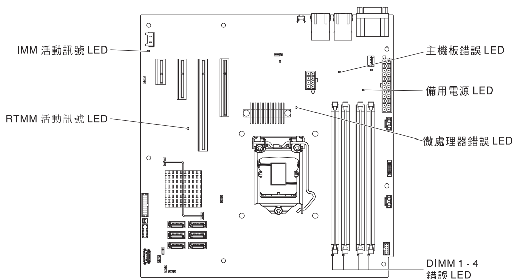
圖 10. 主機板上的 LED
