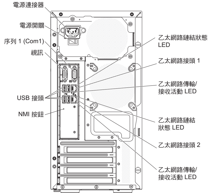
圖 3. 4U 伺服器背面圖
