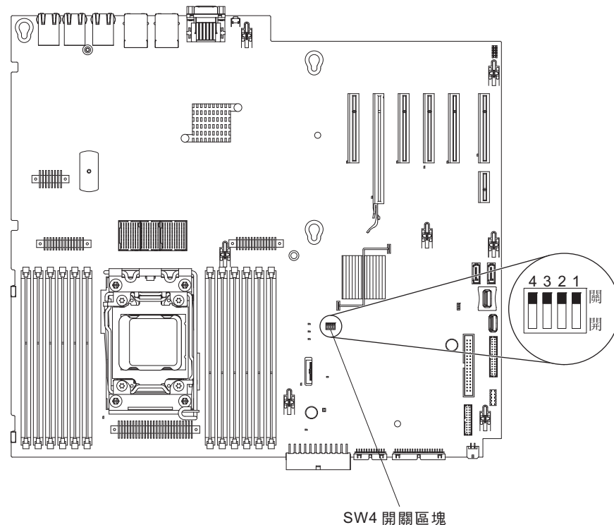
圖 11. 開機密碼開關
