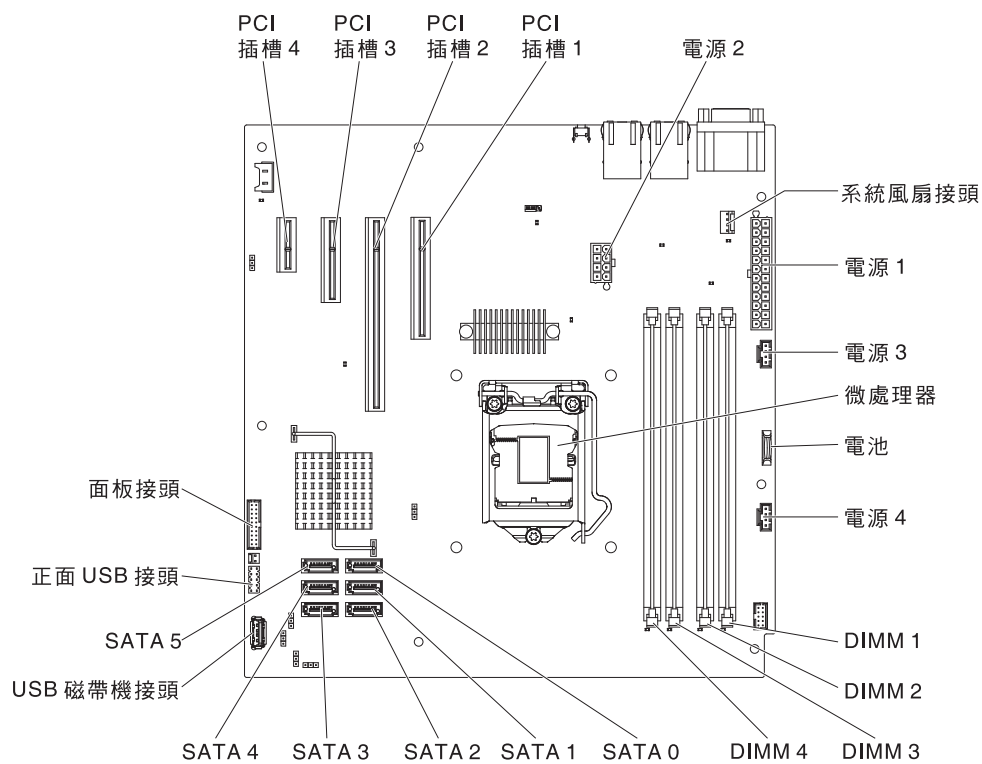
圖 7. 主機板上的內部接頭
