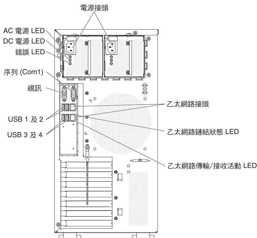
圖 4. 5U 伺服器背面圖
