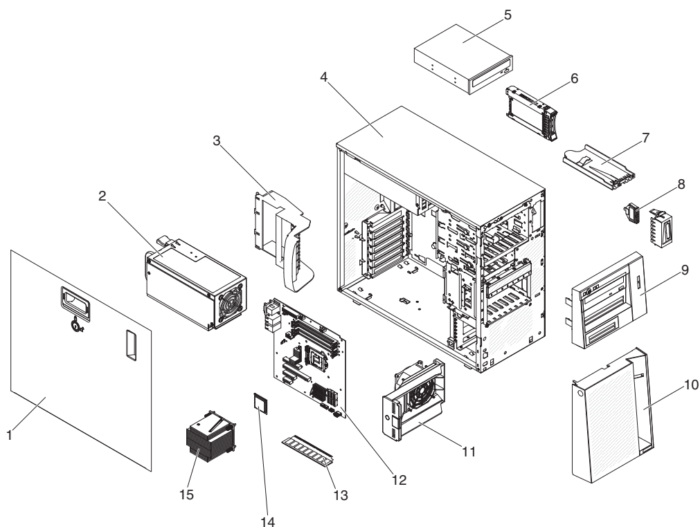
圖 13. 伺服器元件
