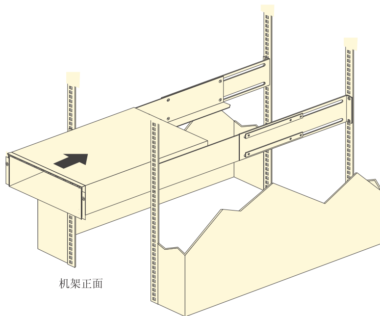
图 12. 安装 EXP520
