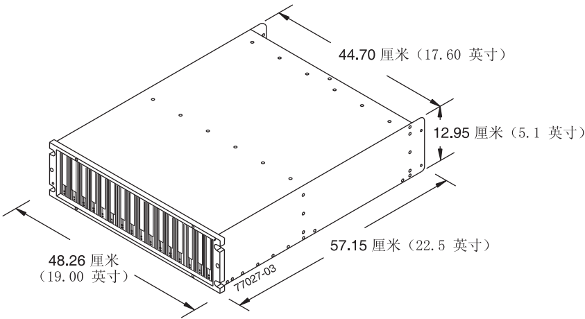
图 6. EXP520 尺寸
