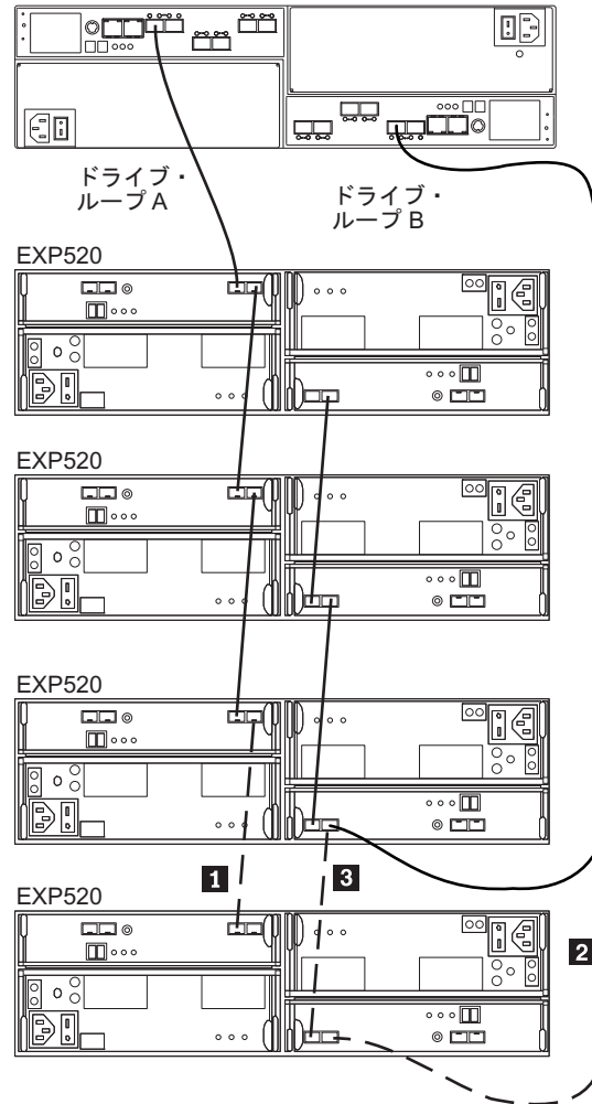
図 33. 既存の構成済みドライブ・ループへの EXP520 のケーブル接続
