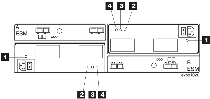
図 29. 電源機構およびファン・ユニット LED
