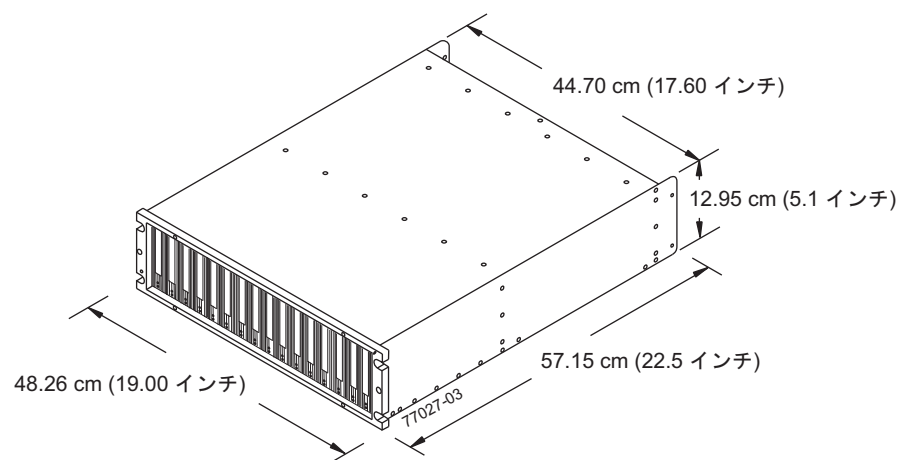
図 6. EXP520 寸法
