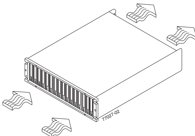
図 7. EXP520 空気の流れ
