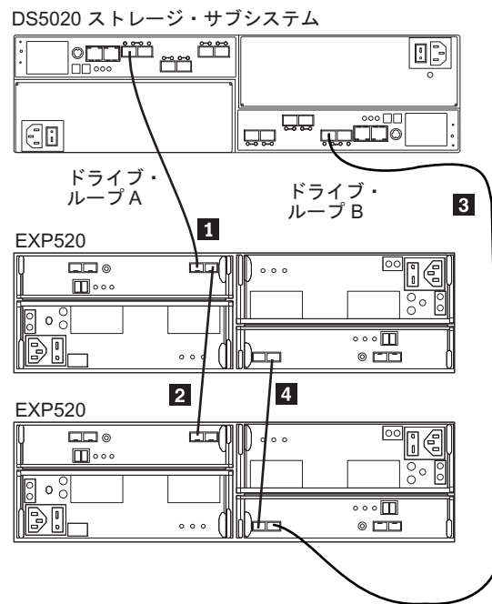
図 28. 正しい EXP520 冗長ドライブ・ループ構成
