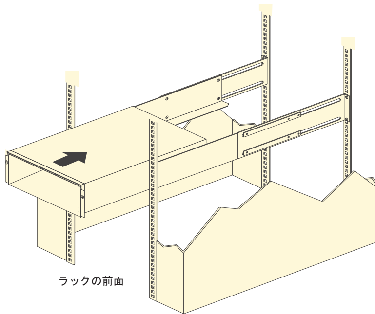
図 12. EXP520 の取り付け
