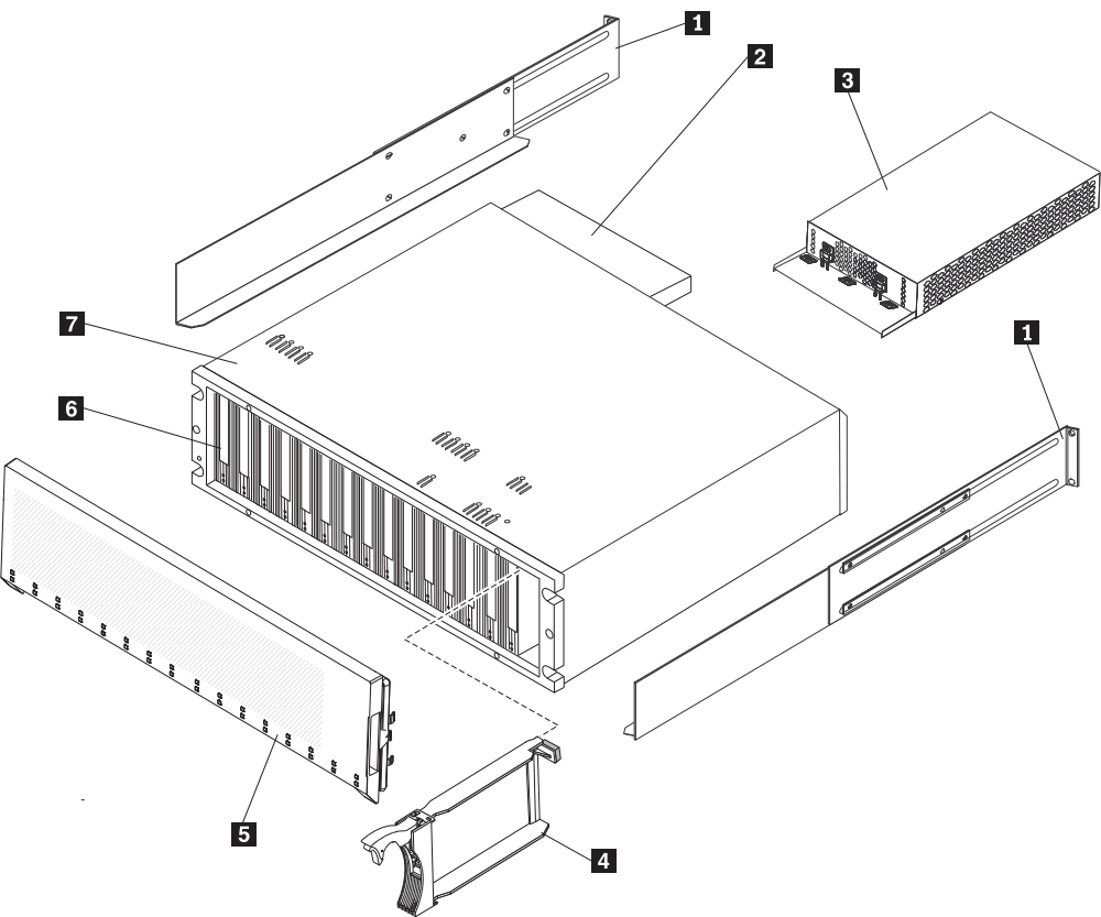
図 41. EXP520 ストレージ拡張エンクロージャー部品リスト
