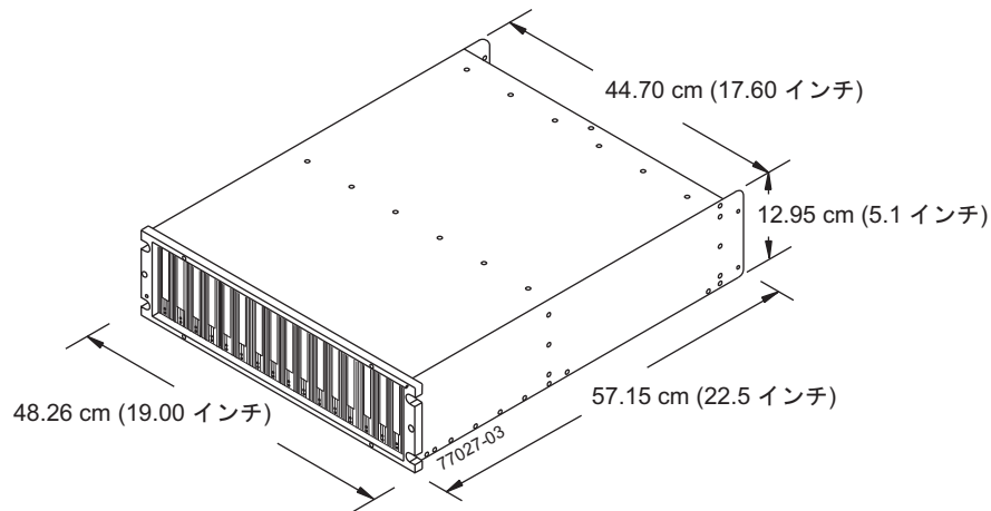
図 6. EXP5000 寸法
