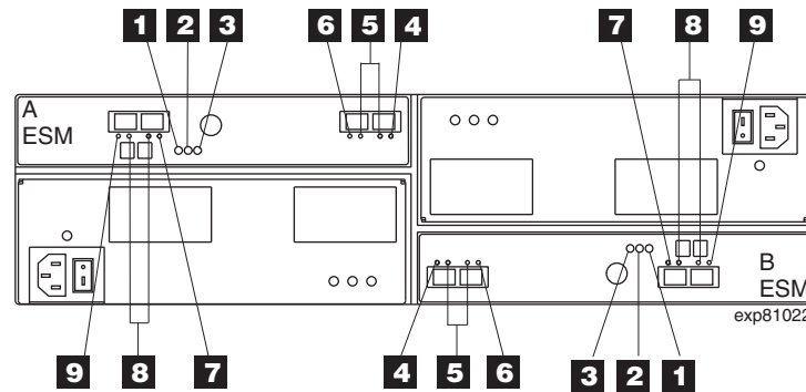
図 30. 背面 LED、コントロール、およびコネクタ
