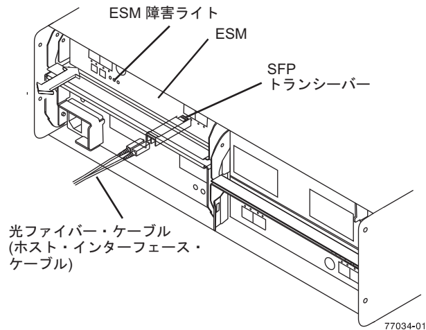
図 38. SFP モジュールの交換
