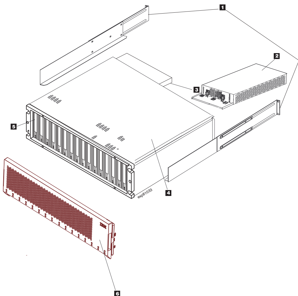
図 41. EXP5000 ストレージ拡張エンクロージャー部品リスト
