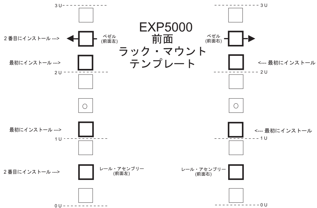
図 43. 前面用ラック・マウント・テンプレート
