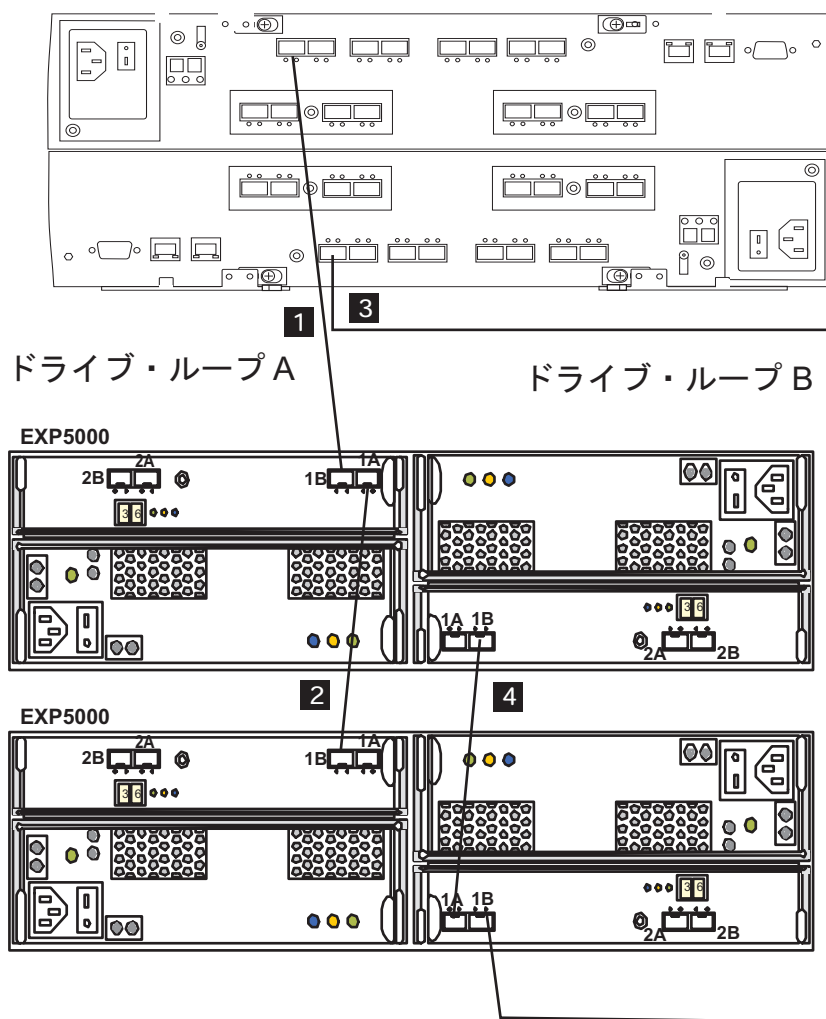
図 27. 正しい EXP5000 冗長ドライブ・ループ構成
