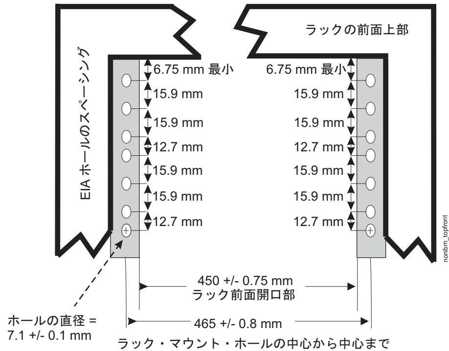
図 46. ラックの仕様寸法 (正面図)
