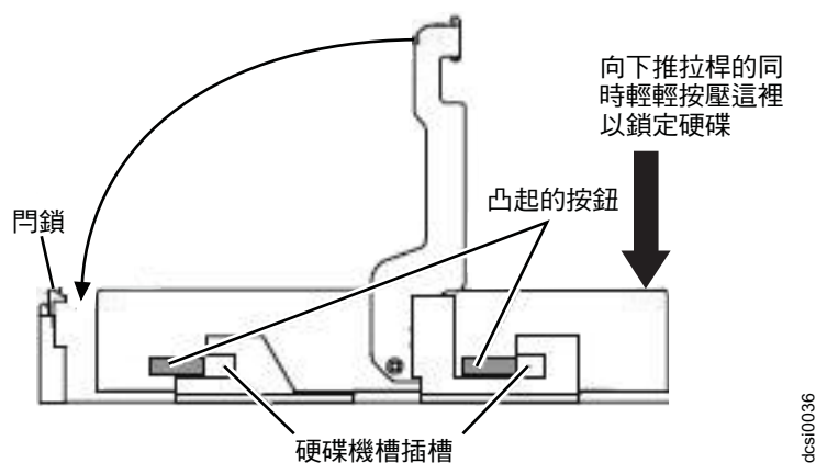
圖 80. 將硬碟插入接頭
