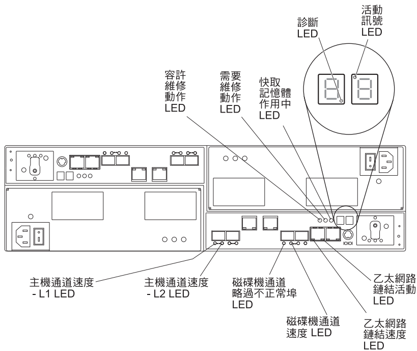
圖 71. 具有兩個標準「光纖通道」主機擴充通道及兩個選用 iSCSI 主機擴充通道之控制器的 LED、控制項及接頭
