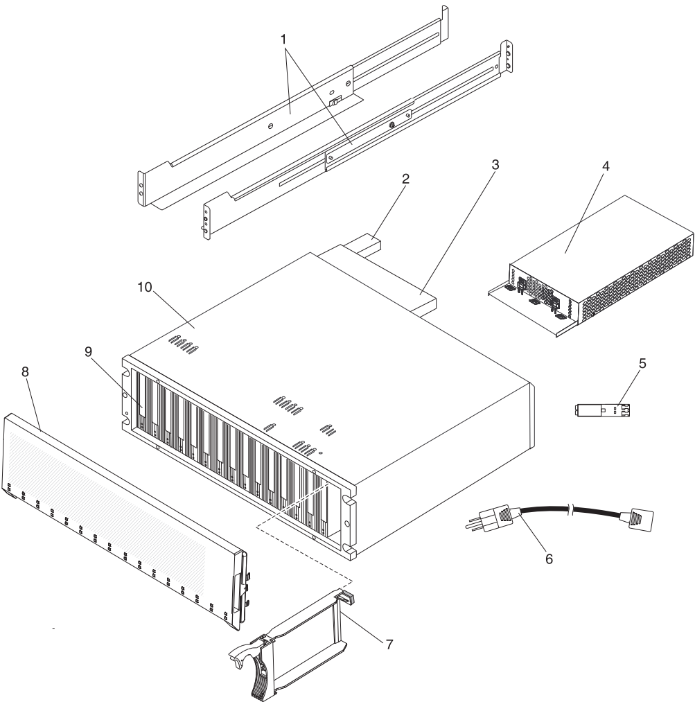
圖 90. DS5020 儲存體子系零件清單
