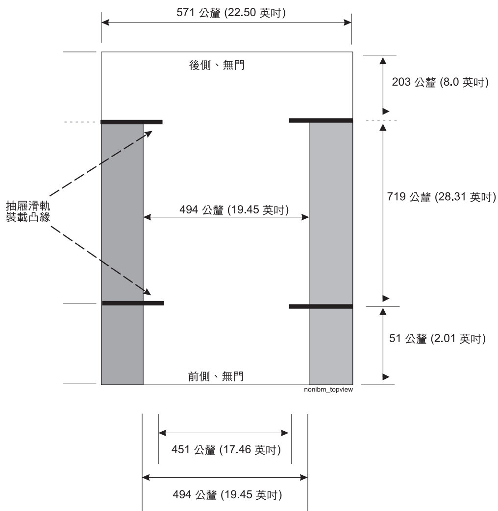
圖 94. 非 IBM 機架規格尺寸的頂端視圖
