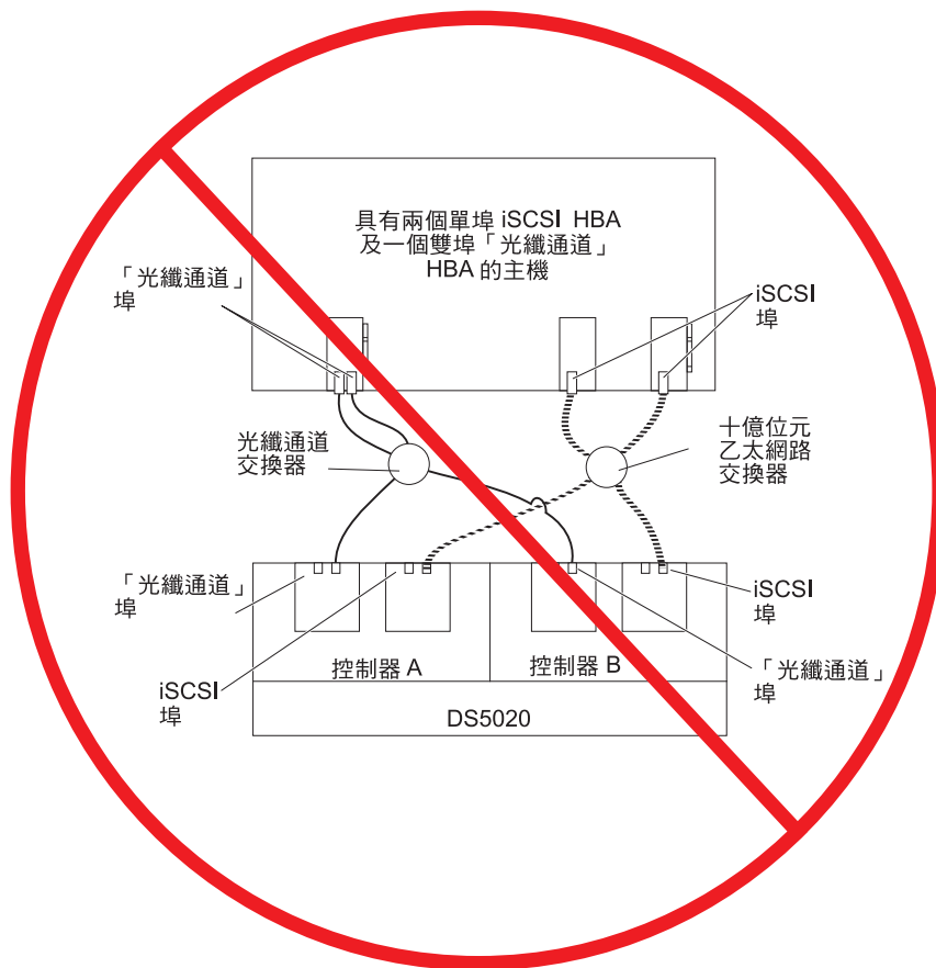
圖 64. 不正確配置的範例：單一主機、iSCSI 及「光纖通道」
