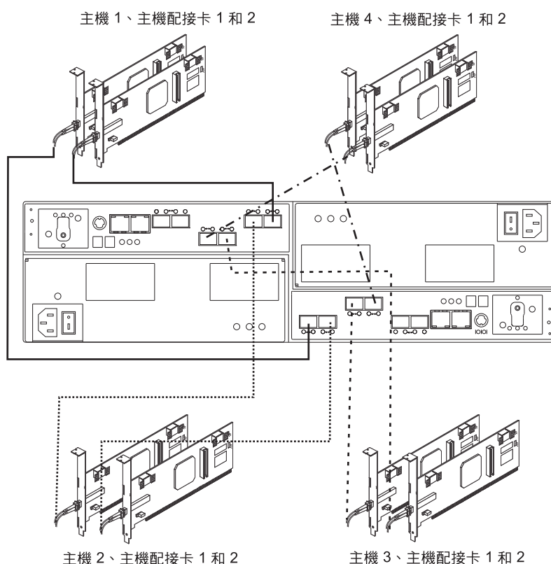
圖 55. 兩個備用主機連線的纜線安裝圖解
