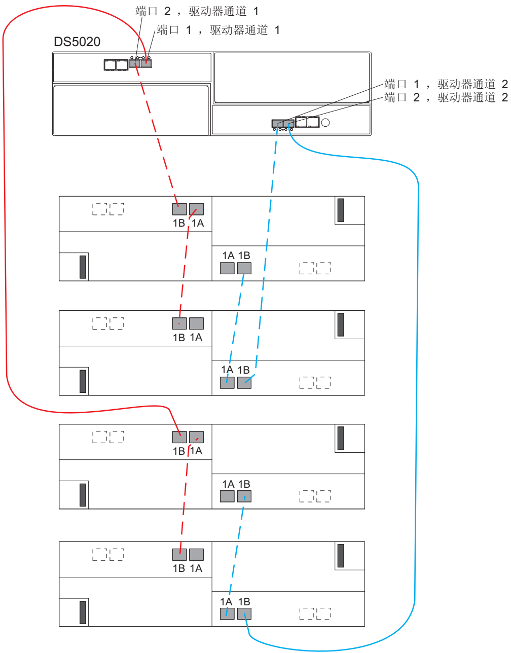
图 41. 用电缆连接一个 DS5020 和四个存储扩展机柜
