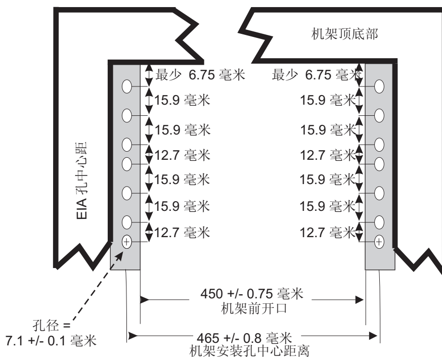
图 95. 机架规格尺寸，顶视图（前部）
