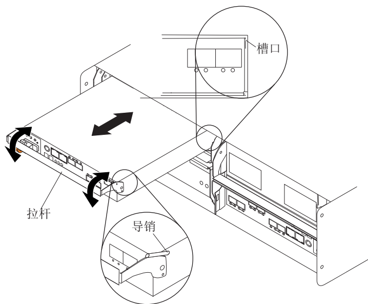
图 78. 安装控制器
