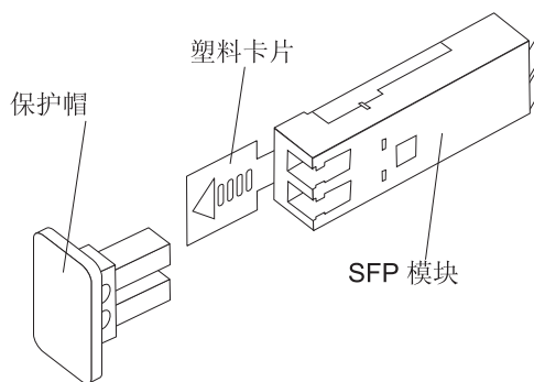
图 27. 将 SFP 模块安装到主机端口中
