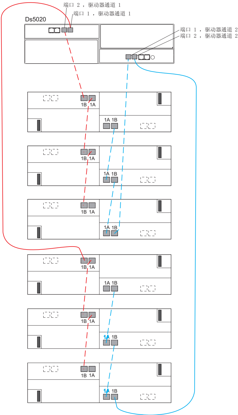
图 42. 用电缆连接一个 DS5020 和最多六个存储扩展机柜
