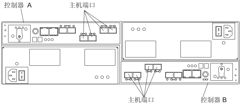
图 54. DS5020 的 RAID 控制器上的主机电缆位置
