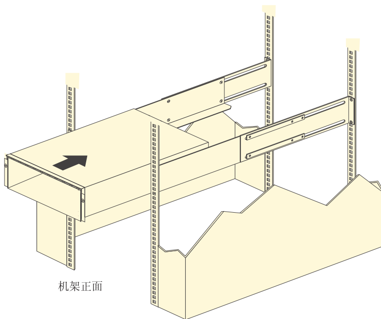
图 19. 安装 DS5020
