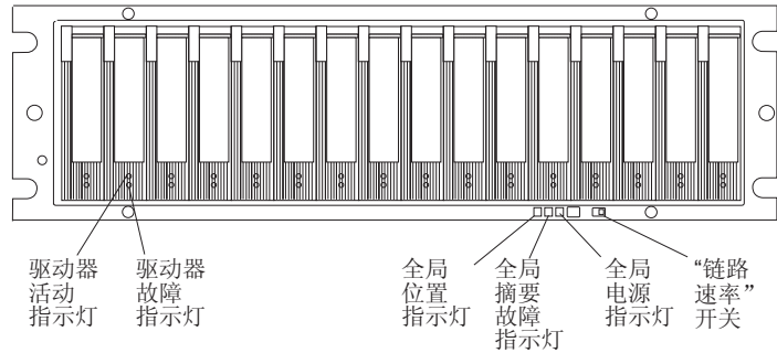
图 67. 前部指示灯和控件
