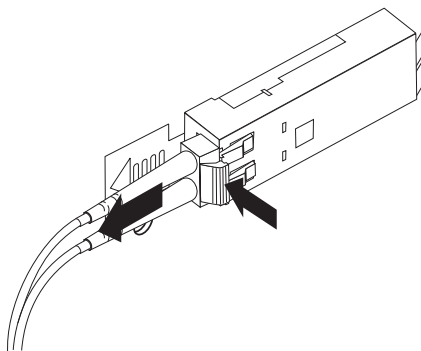
图 34. 卸下 LC-LC 光线通道电缆
