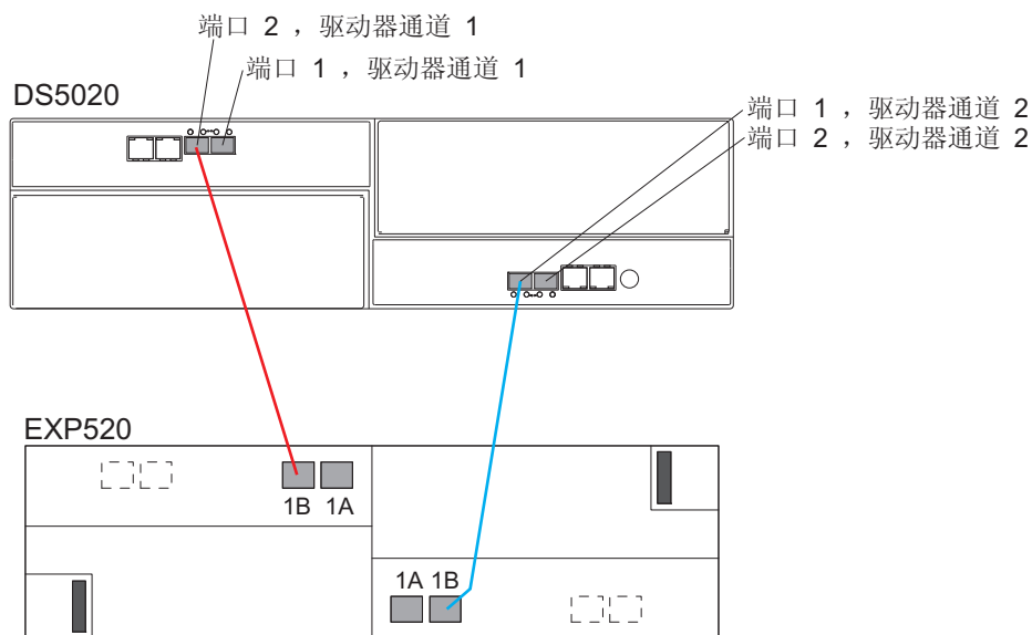
图 46. 用电缆连接一个 DS5020 和一个 EXP520 存储扩展机柜
