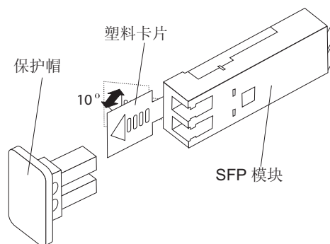
图 28. 松开塑料类 SFP 模块滑锁
