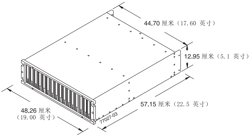
图 9. DS5020 尺寸
