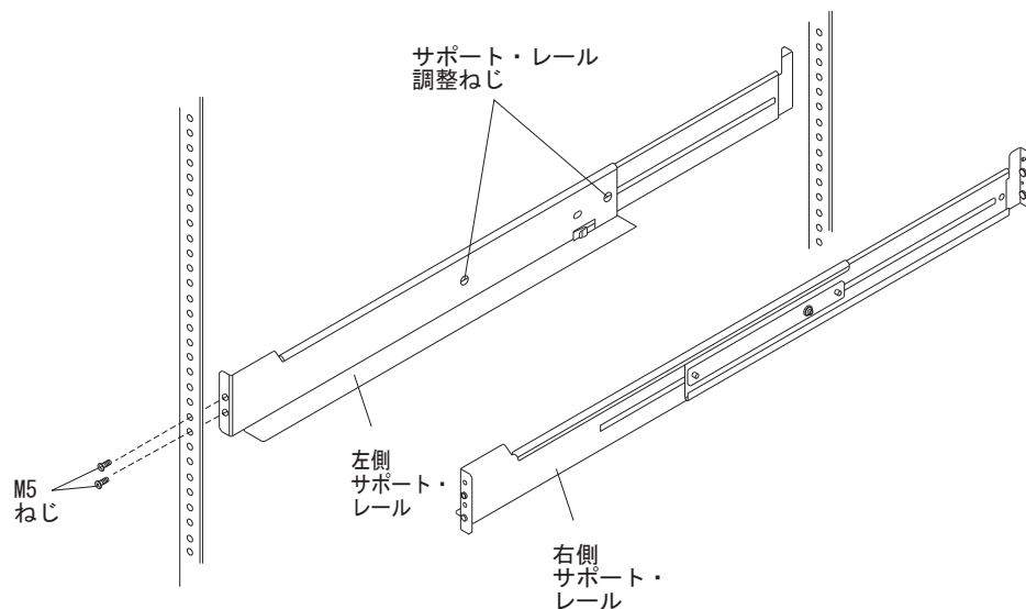
図 15. サポート・レールの取り付け
