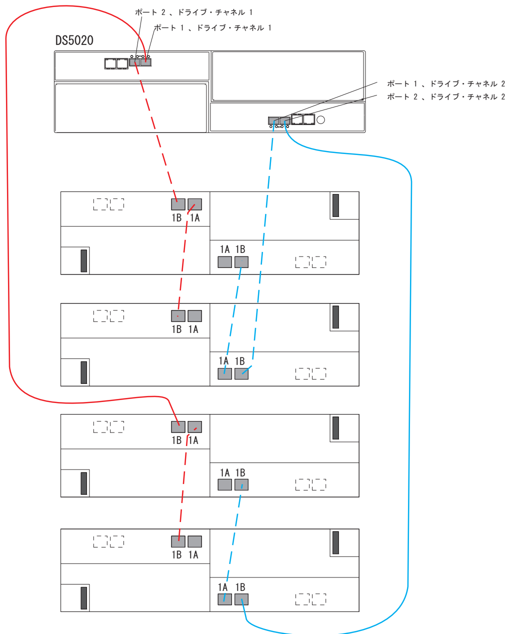
図 41. 1 つの DS5020 と 4 つのストレージ拡張エンクロージャのケーブル接続
