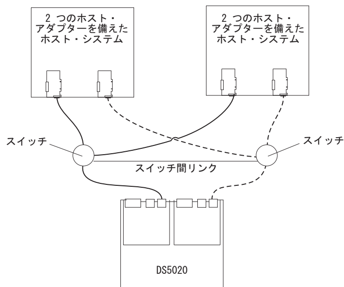
図 57. 単一 SAN ファブリック構成の例
