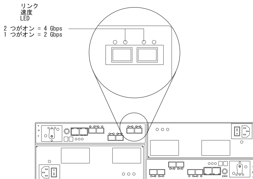
図 83. リンク速度 LED
