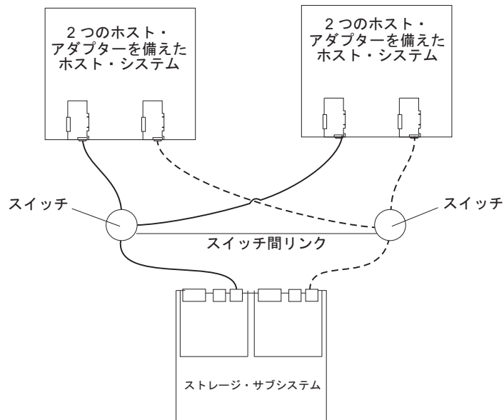
図 56. 単一 SAN ファブリック構成の例
