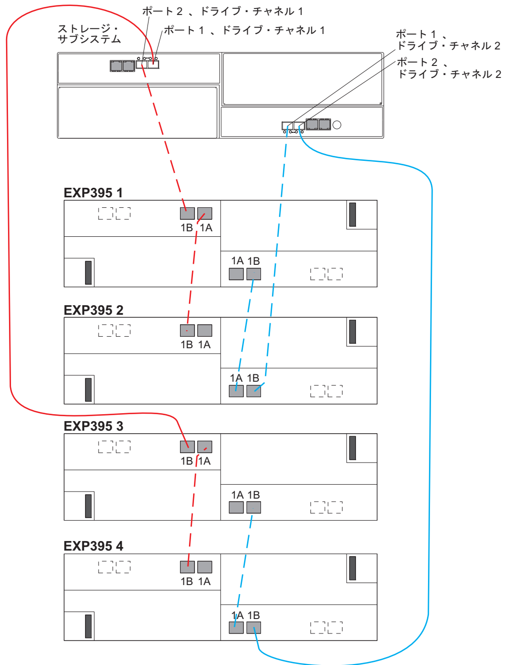
図 48. 1 組の DS3950 ドライブ・ポートの後ろでの 1 つの DS3950 と 4 つの EXP395 ストレージ拡張エンクロージャー
