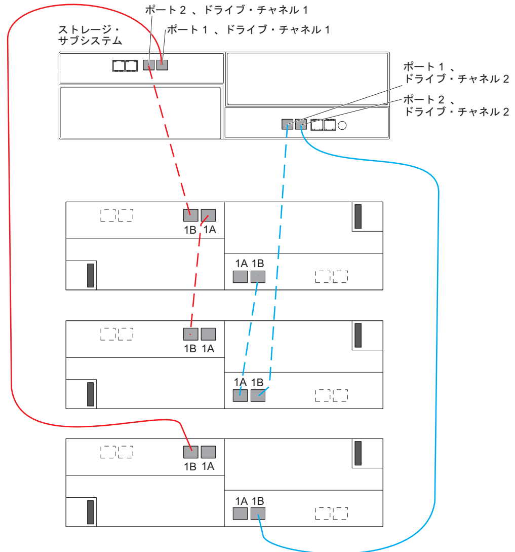
図 39. 1 つの DS3950 と 3 つのストレージ拡張エンクロージャのケーブル接続
