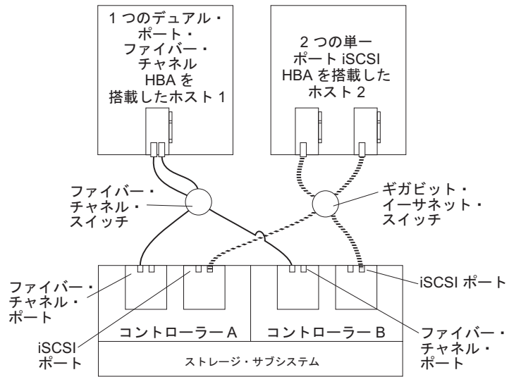
図 62. iSCSI およびファイバー・チャンネル・ホスト、複数ポート構成の例
