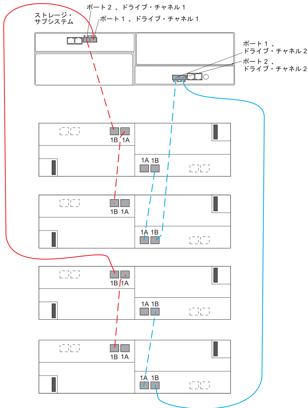
図 40. 1 つの DS3950 と 4 つのストレージ拡張エンクロージャのケーブル接続
