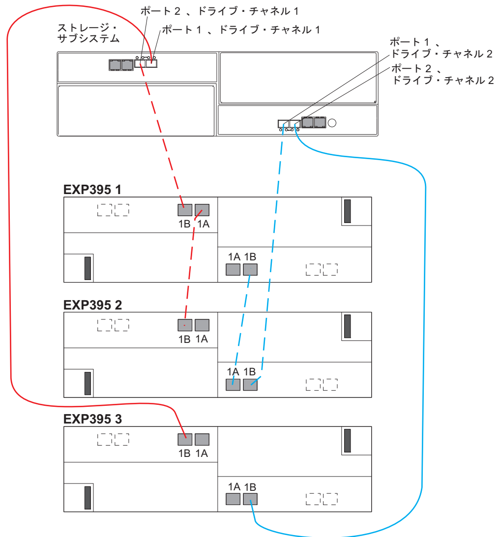
図 47. 1 組の DS3950 ドライブ・ポートの後ろでの 1 つの DS3950 と 3 つの EXP395 ストレージ拡張エンクロージャー
