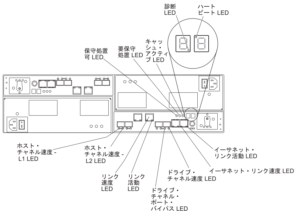
図 69. モデル 98H: 2 つの標準ファイバー・チャンネル・ホスト拡張チャンネルおよび 2 つのオプション iSCSI ホスト拡張チャンネルを搭載したコントローラーの LED、制御、およびコネクタ
