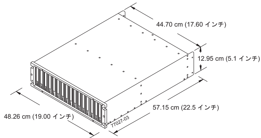
図 8. DS3950 寸法
