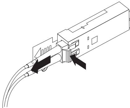
図 33. LC-LC ファイバー・チャネル・ケーブルの取り外し
