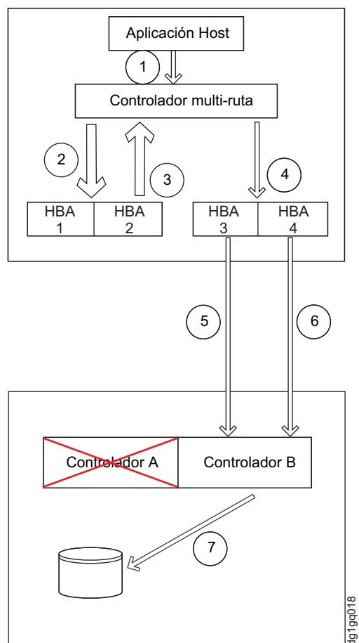
Figura 20. Todas las rutas al controlador fallan en modo ALUA. Cinco minutos de error
