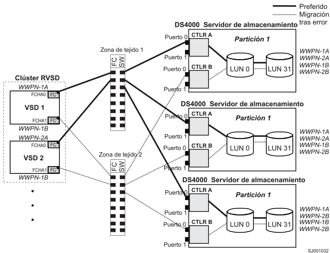
Figura 37. Configuración de clúster con tres subsistemas de almacenamiento - una partición por subsistema
