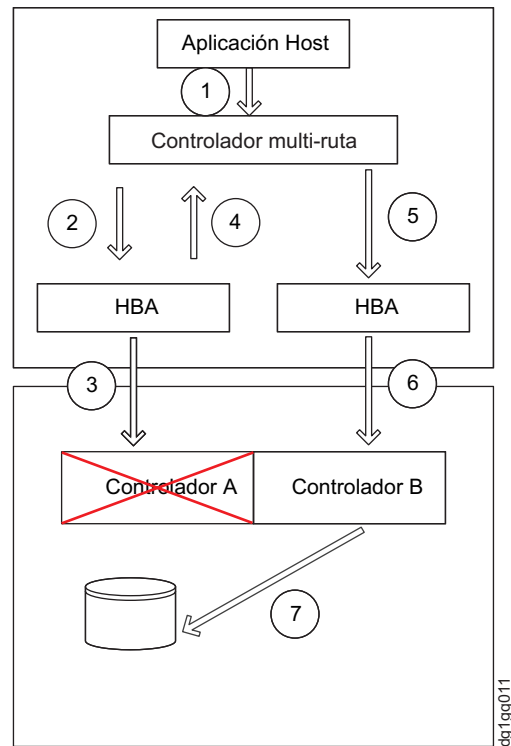
Figura 16. Migración tras error de E/S en un entorno de ruta única
