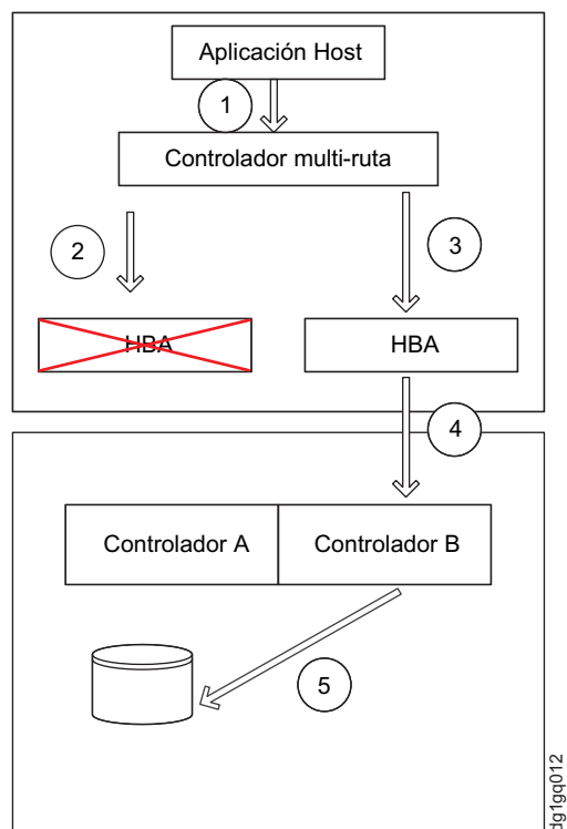
Figura 18. Todas las rutas al controlador fallan en modo de migración tras error AVT/ADT y RDAC
