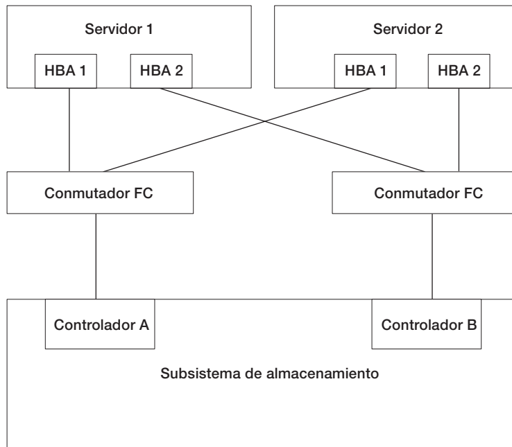
Figura 22. Ejemplo de configuración de HBA de host a subsistema de almacenamiento para controladores multi-ruta AIX fcp_array y Solaris RDAC
