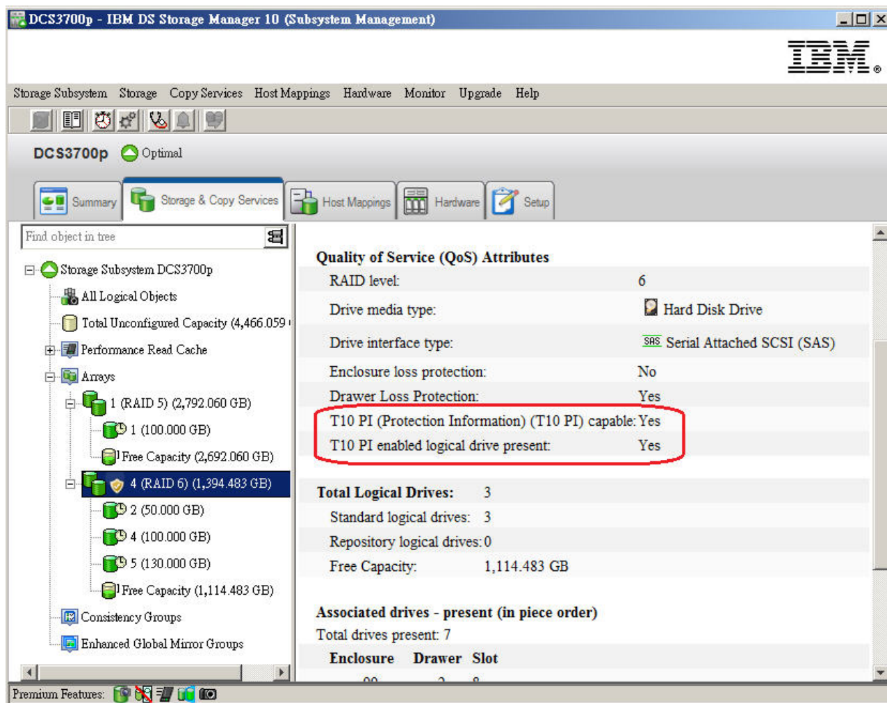
Figura 7. Ejemplo - Unidad lógica 4 de matriz RAID 4 - T10PI no habilitada
