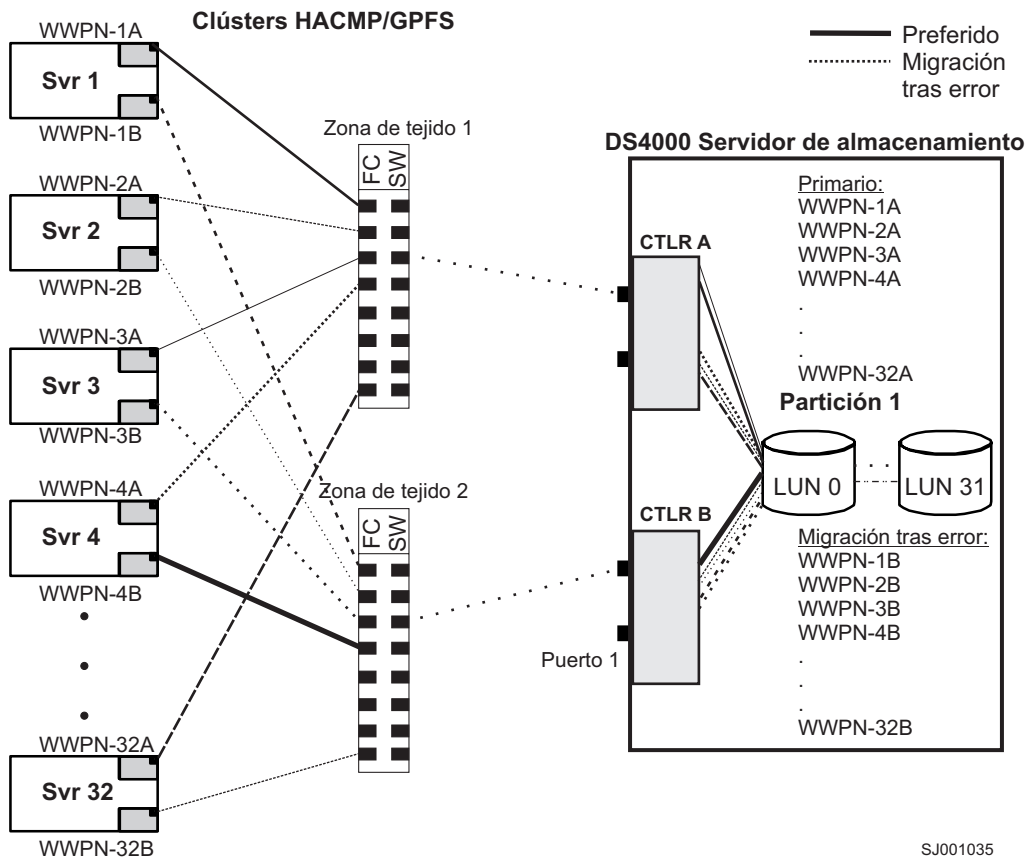
Figura 40. Configuración de clúster HACMP/GPFS con un subsistema de almacenamiento - una partición
