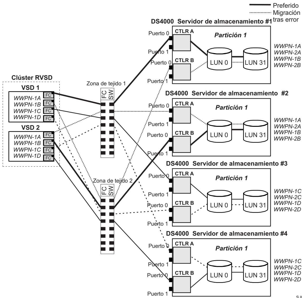
Figura 38. Configuración de clúster con cuatro subsistemas de almacenamiento - una partición por subsistema
