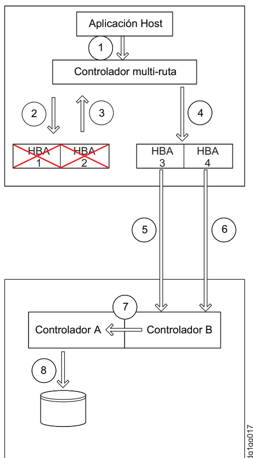
Figura 19. Todas las rutas al controlador fallan en modo de migración tras error ALUA. Cinco primeros minutos de la migración tras error.
