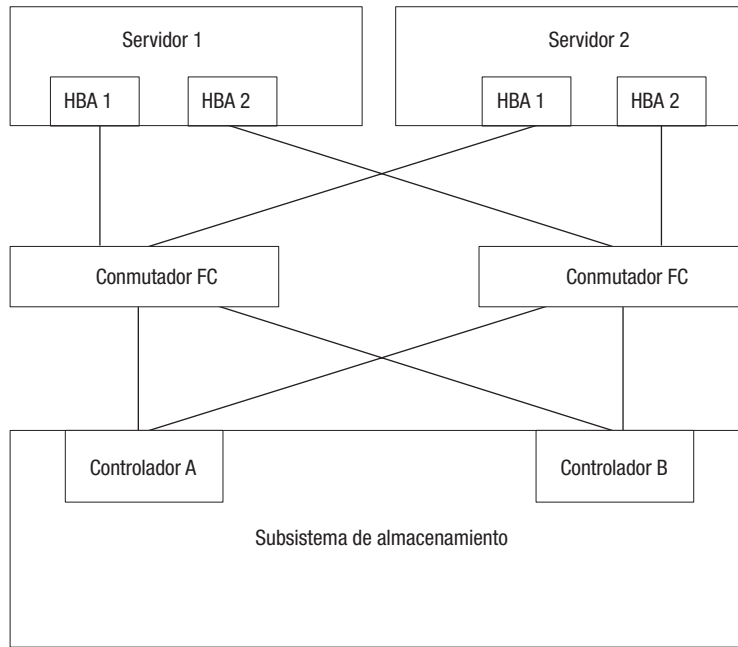
Figura 21. Ejemplo de configuración de HBA de host a subsistema de almacenamiento para todos los controladores multi-ruta excepto AIX fcp_array y Solaris RDAC
