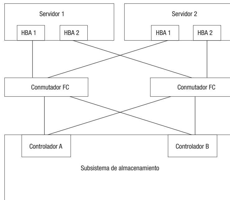
Figura 35. Configuración de conexiones cruzadas para conexiones VMware
