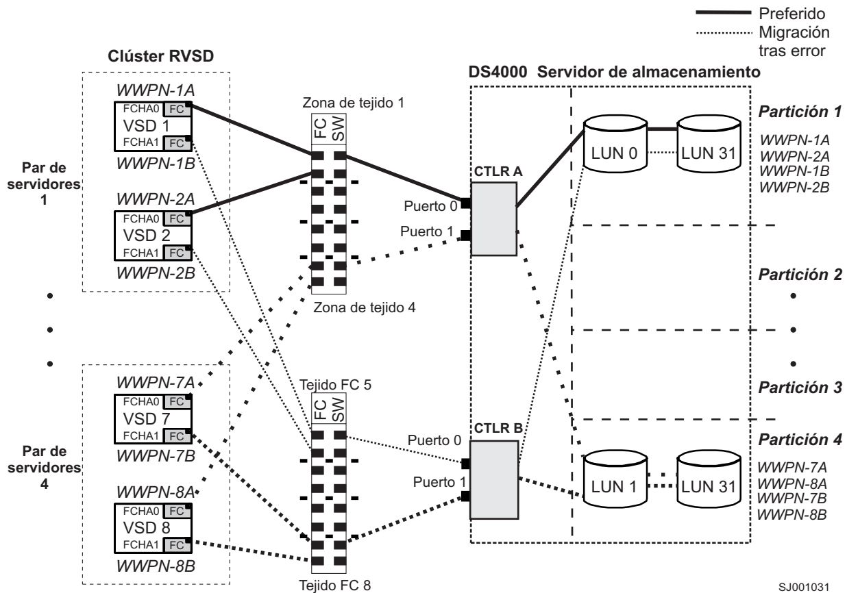
Figura 36. Configuración de clúster con un subsistema de almacenamiento individual - una a cuatro particiones
