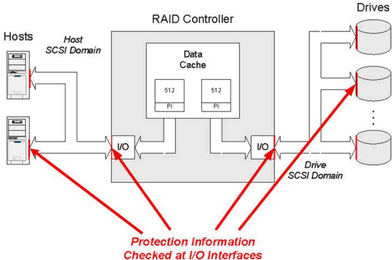
Figura 4. Puntos de comprobación de Protection Information (P)
