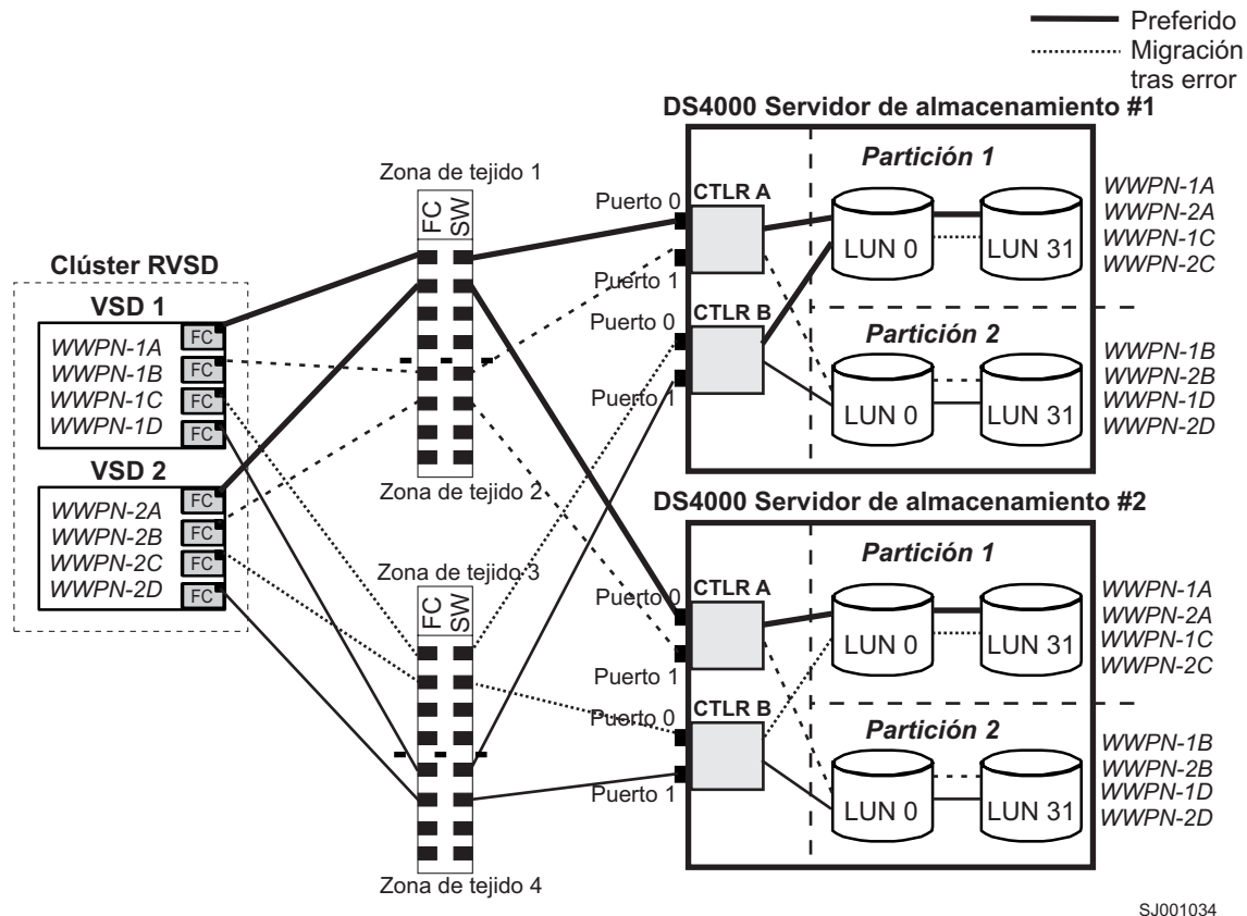
Figura 39. Configuración de clúster RVSD con dos subsistemas de almacenamiento - dos particiones por subsistema
