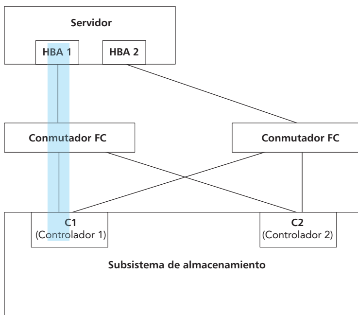
Figura 23. Esquema de distribución en zonas uno a uno
