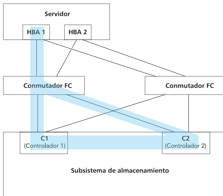
Figura 24. Esquema de distribución en zonas uno a dos
