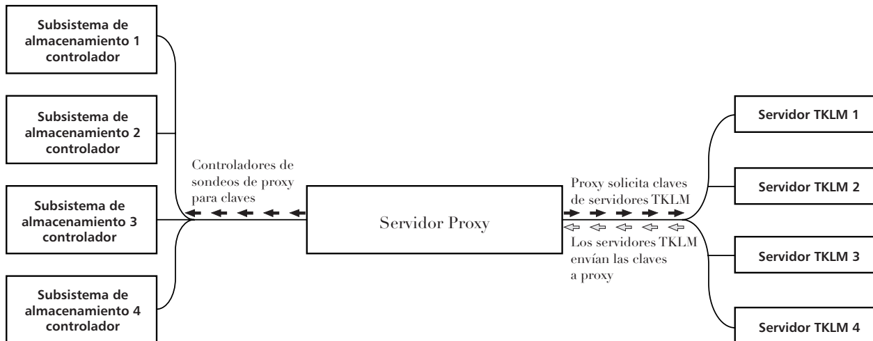
Figura 33. Topología de gestión externa de claves de seguridad
