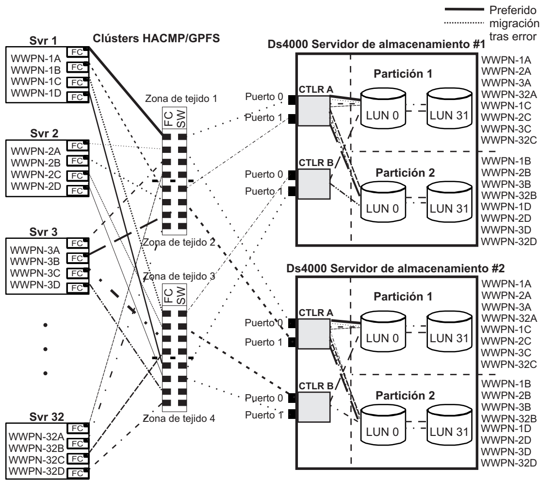
Figura 41. Configuración de clúster HACMP/GPFS con dos subsistemas de almacenamiento - dos particiones por subsistema
