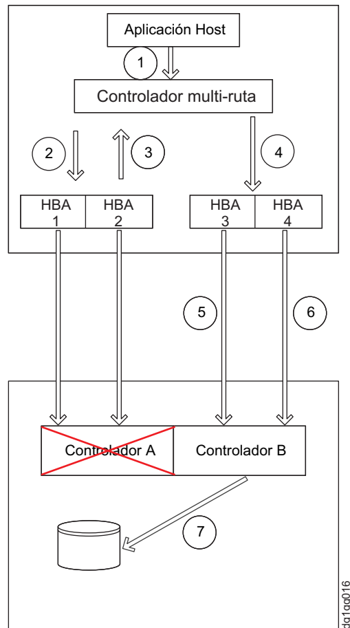
Figura 17. Migración tras error de E/S en un entorno multi-ruta
