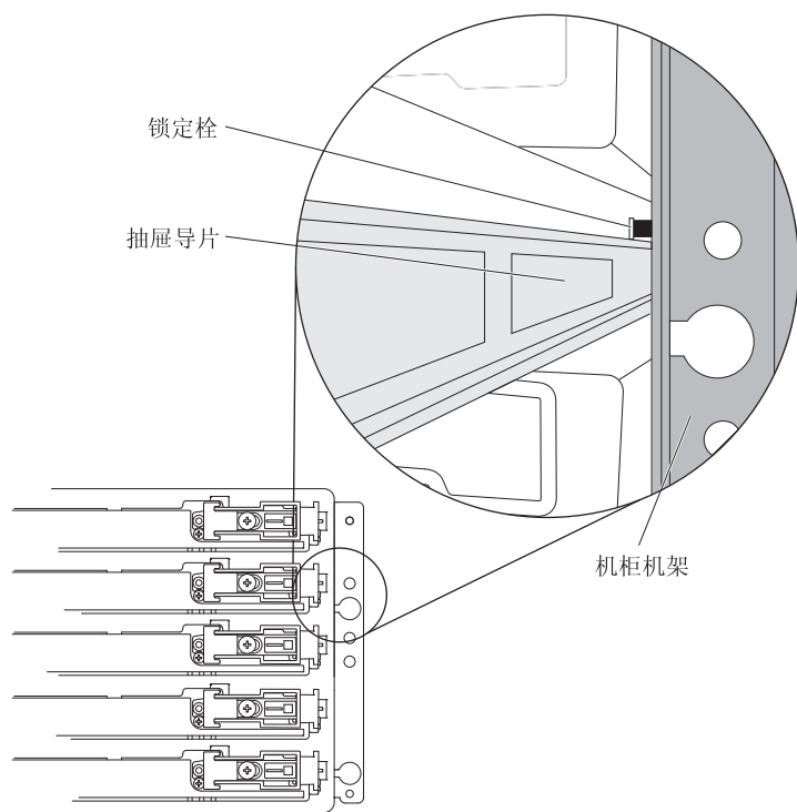
图 99. 位于抽屉导销上方的锁定滚轮
