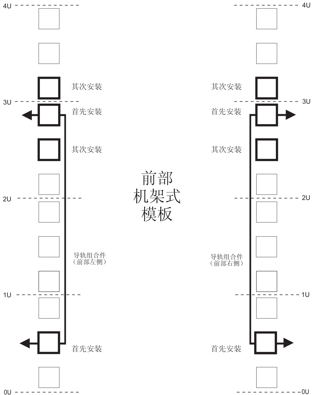
图 124. 前部机架安装模板
