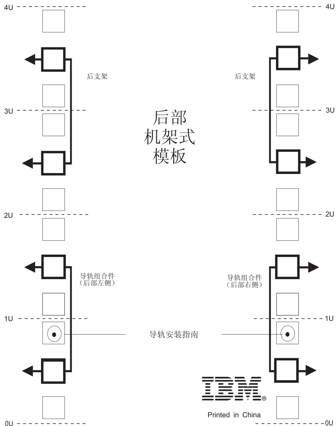
图 125. 后部机架安装模板
