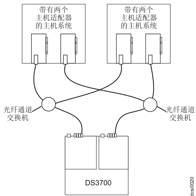
图 48. 双光纤通道 SAN 光纤网配置的示例
