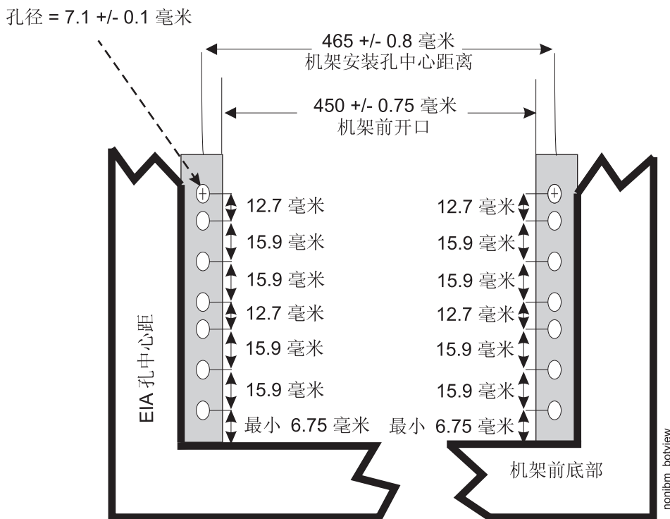
图 128. 机架规格尺寸，底视图（前部）
