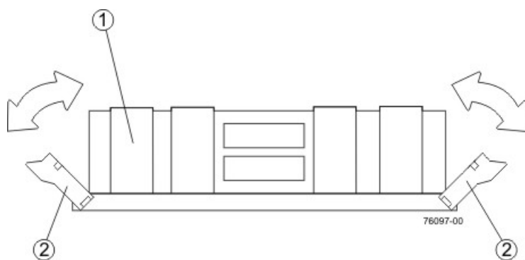
图 106. 卸下高速缓存内存 DIMM
