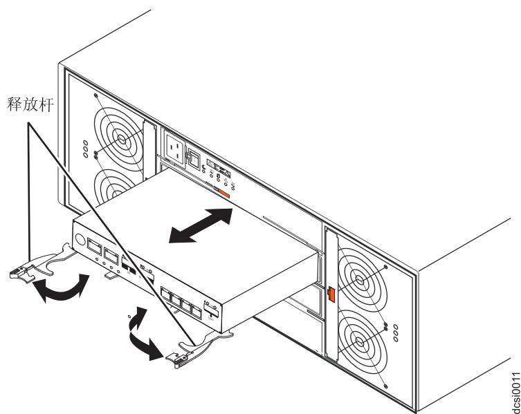
图 66. 卸下并重新安装控制器
