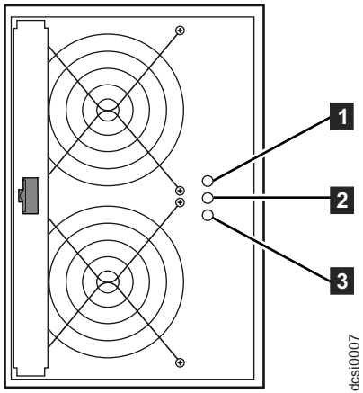
图 59. 风扇组件指示灯
