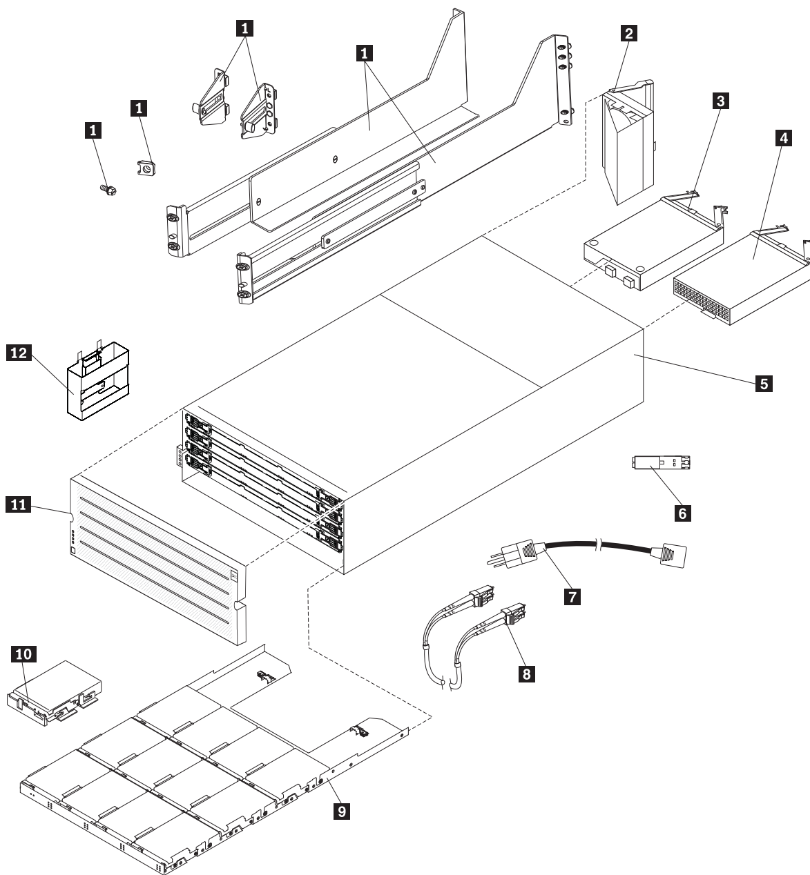
图 121. DCS3700 存储子系统机柜部件列表
