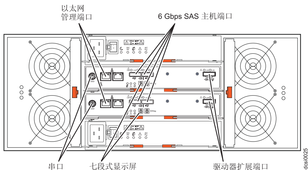
图 5. DCS3700 接口
