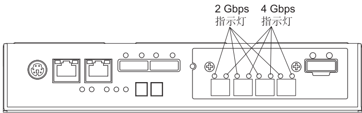
图 56. 光纤通道主机端口适配器指示灯
