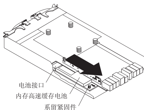
图 67. 从控制器上卸下电池单元
