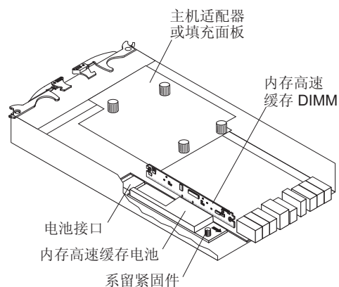
图 81. 内存高速缓存 DIMM 的位置
