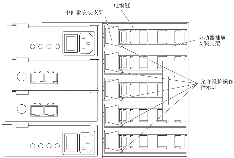
图 95. 已卸下右侧风扇组合件的存储扩展机柜的后视图
