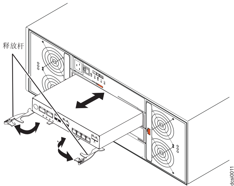
图 82. 卸下控制器
