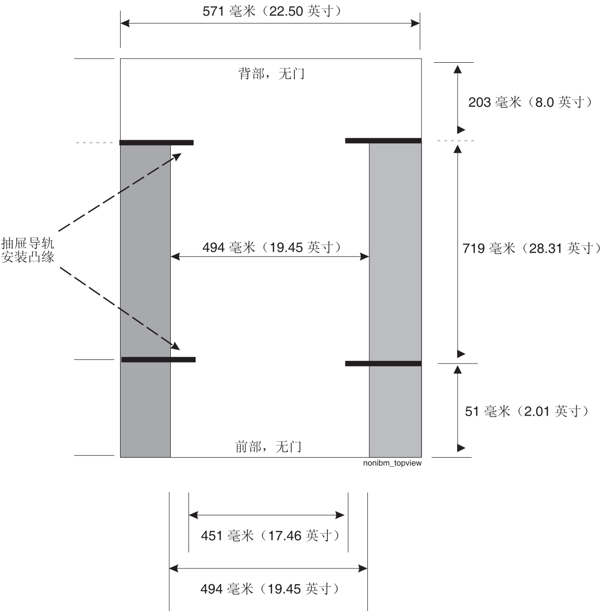
图 126. 非 IBM 机架规格尺寸的顶视图
