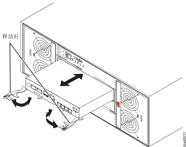
图 87. 卸下环境维护模块
