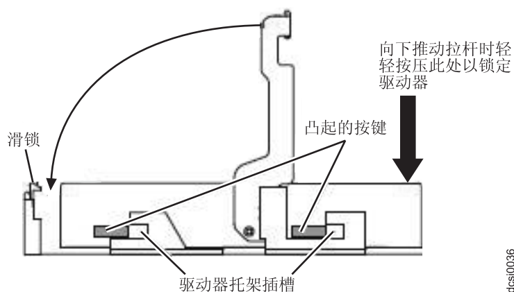
图 74. 将硬盘驱动器插入接口
