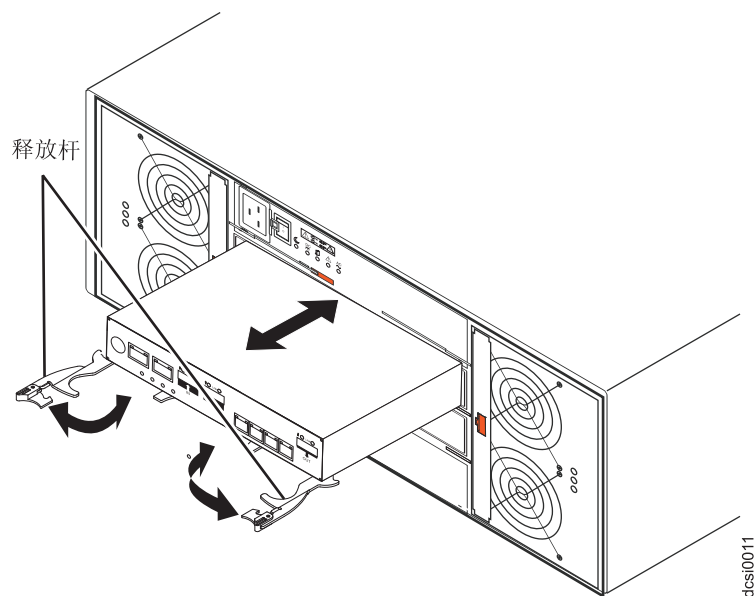
图 69. 卸下控制器
