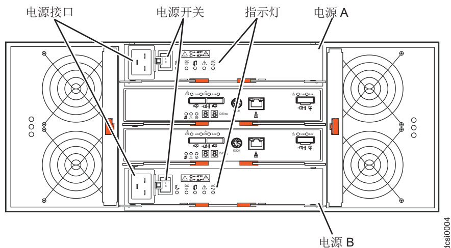
图 10. 电源组件
