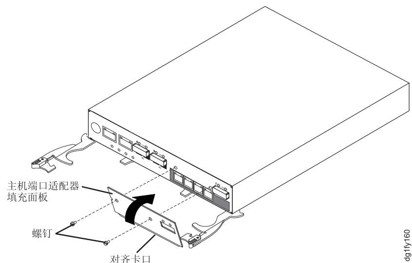
图 70. 卸下主机端口适配器填充面板
