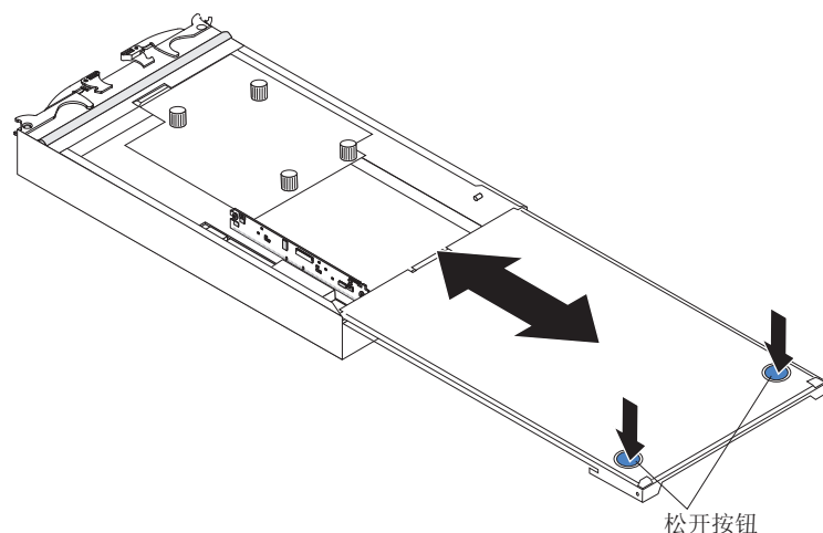
图 65. 卸下外盖
