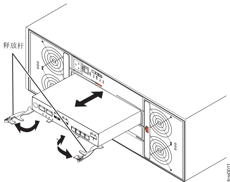
图 64. 卸下控制器
