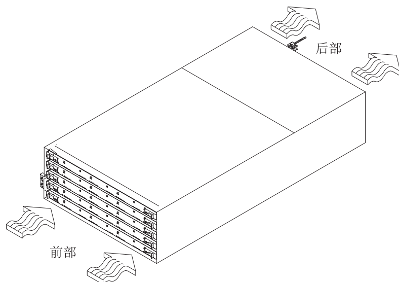
图 14. DCS3700 气流
