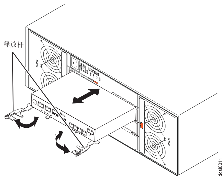
图 100. 卸下并重新安装控制器
