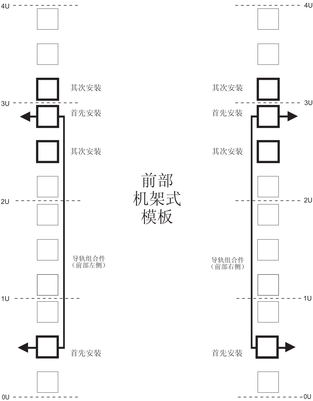
图 16. 前部机架安裝模板
