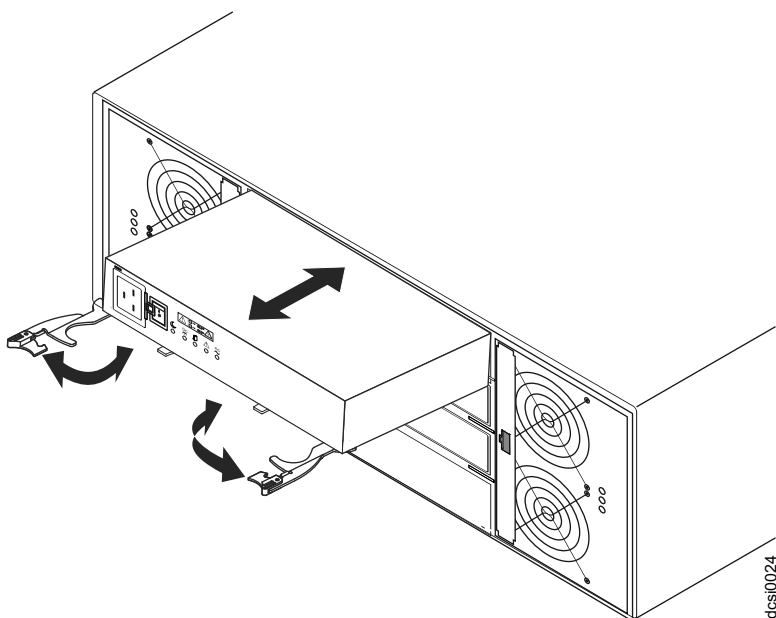
图 78. 更换电源
