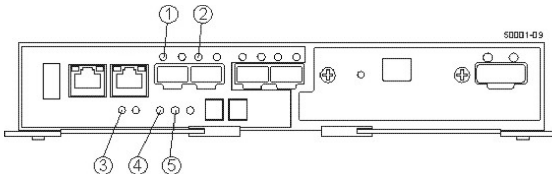
图 120. 控制器指示灯
