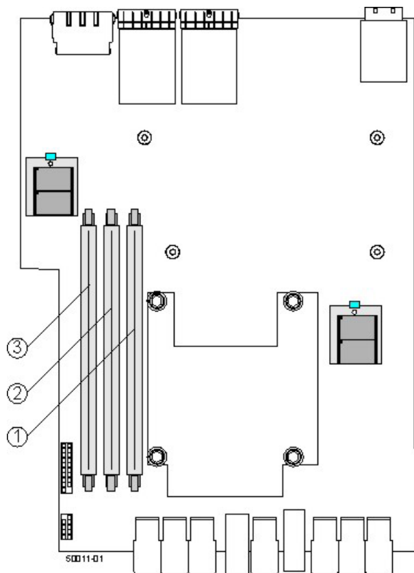
图 105. 三个高速缓存内存 DIMM 插槽
