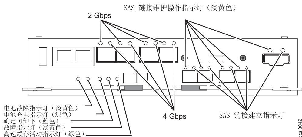
图 55. 带有性能模块控制器的子系统上的控制器指示灯
