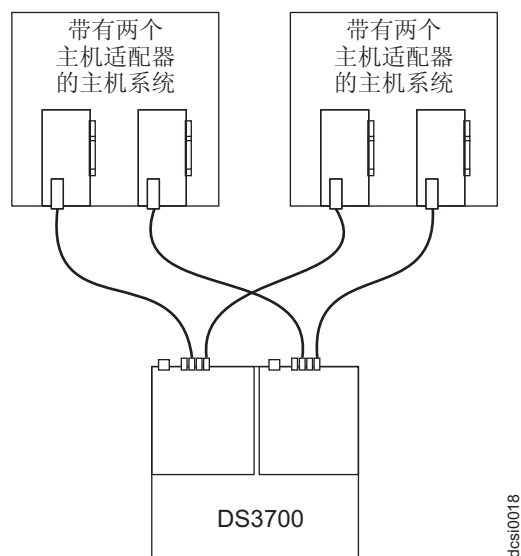
图 46. 与多主机中多个 HBA 的双控制器直接连接的光纤通道连接
