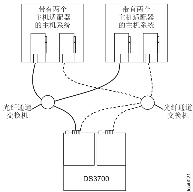
图 49. 双光纤通道 SAN 环境中两个存储子系统的示例
