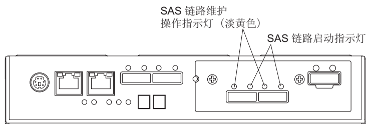
图 57. SAS 主机端口适配器指示灯
