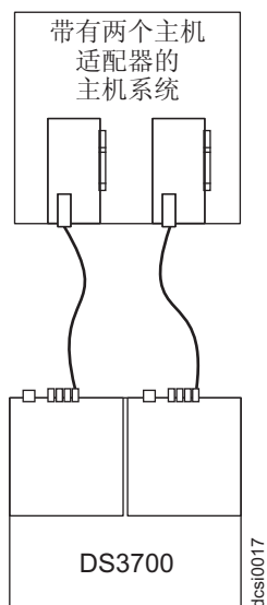
图 42. 与同一主机中两个 HBA 的双控制器直接连接的光纤通道连接（冗余主机连接）
