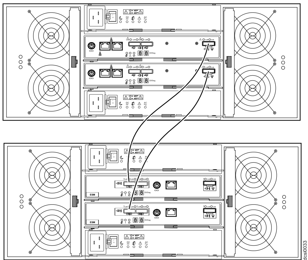
图 38. 单扩展机柜
