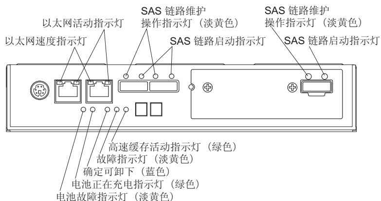
图 54. 控制器指示灯
