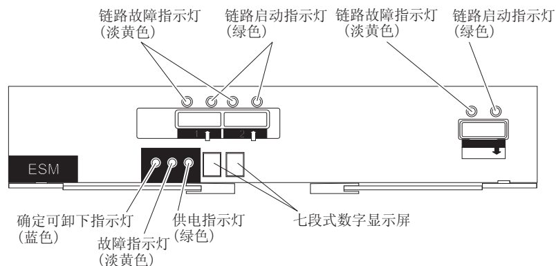
图 58. ESM 指示灯
