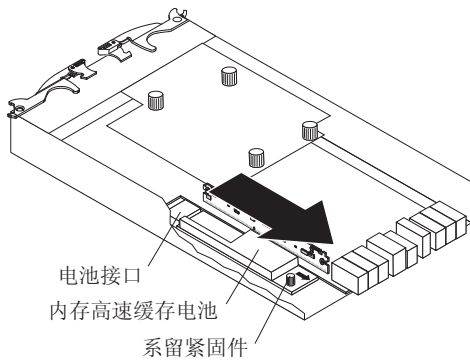
图 80. 从控制器上卸下电池单元
