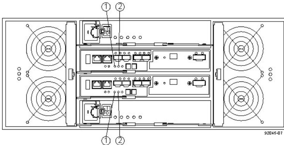
图 114. “控制器维护操作”指示灯
