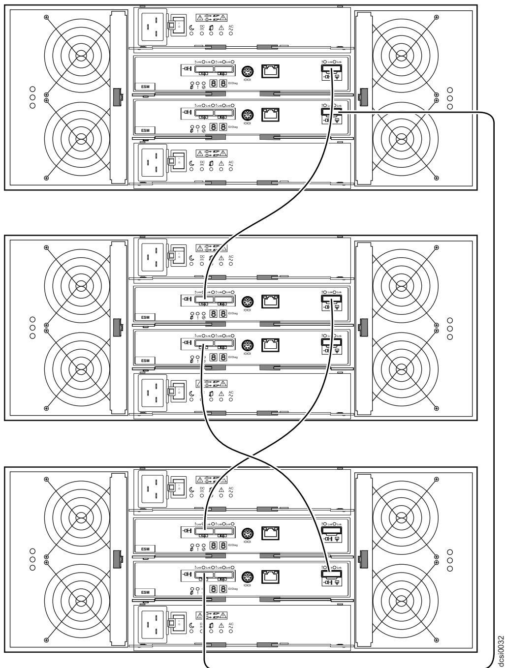
图 39. 双扩展机柜
