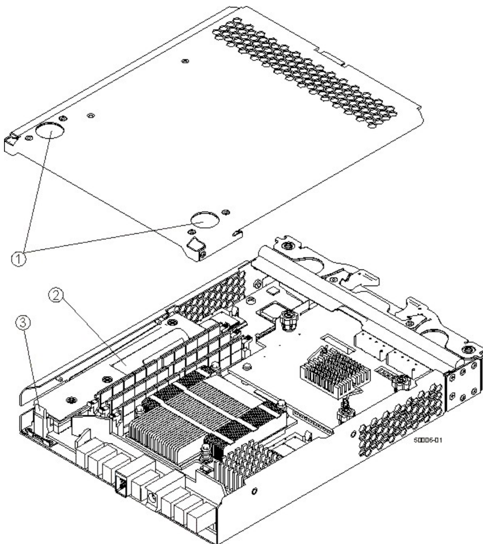
图 112. 控制器顶盖滑锁按钮
