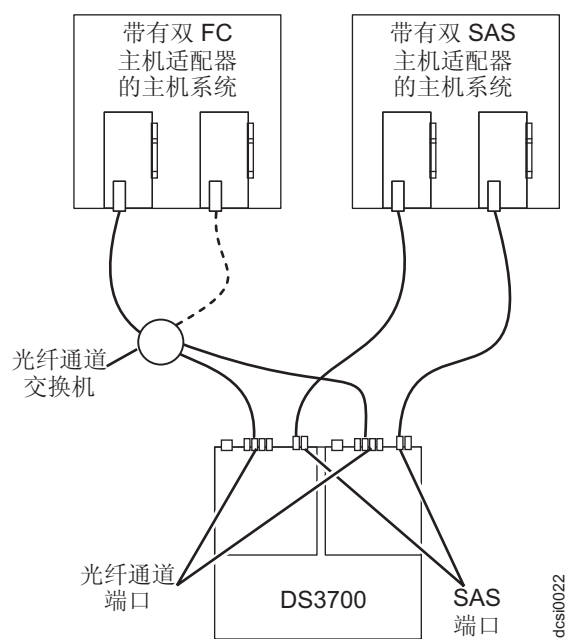
图 50. 多主机、多端口和多光纤网（光纤通道和 SAS）配置的示例
