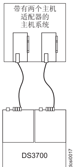
图 45. 与同一主机中两个 HBA 的双控制器直接连接的光纤通道连接（冗余主机连接）
