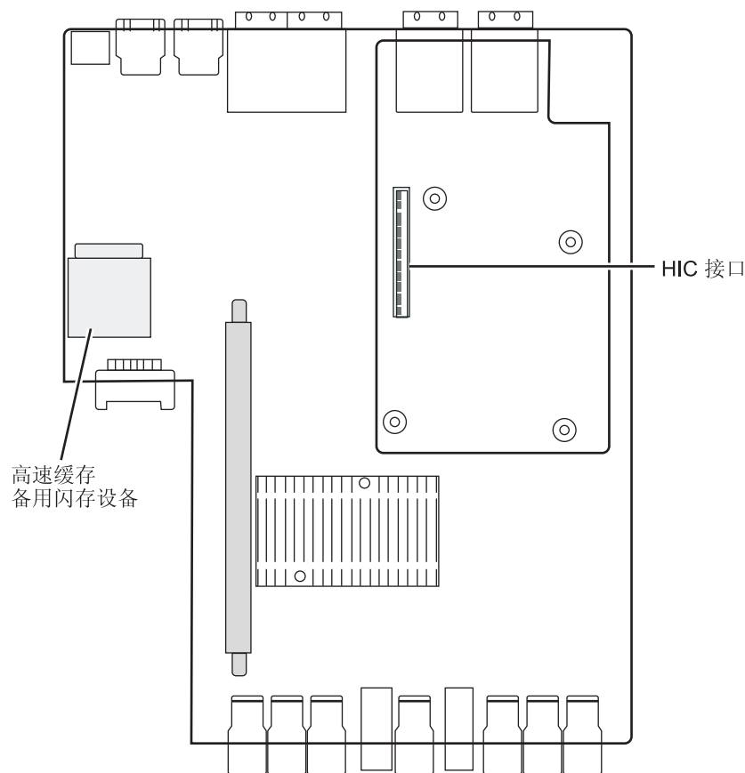
图 72. 对齐 HIC 接口
