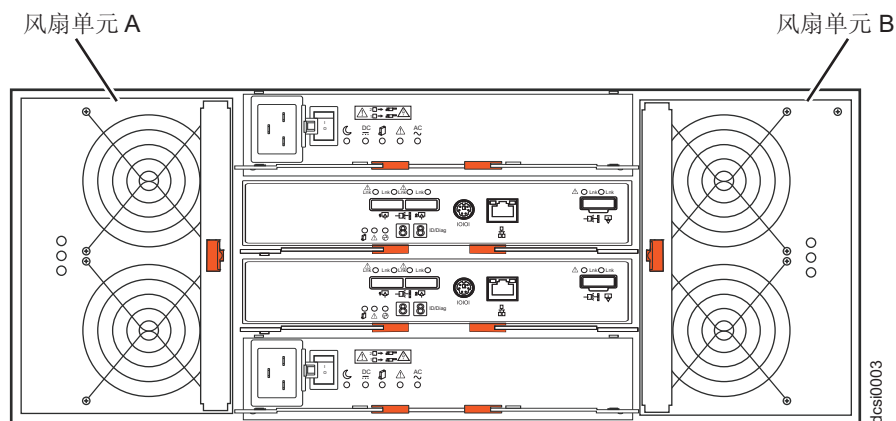
图 11. 风扇组合件组件
