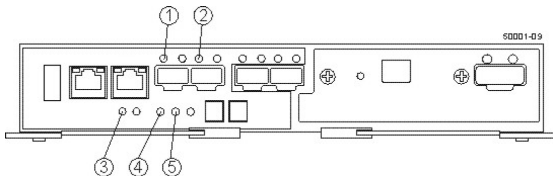
图 108. 控制器指示灯
