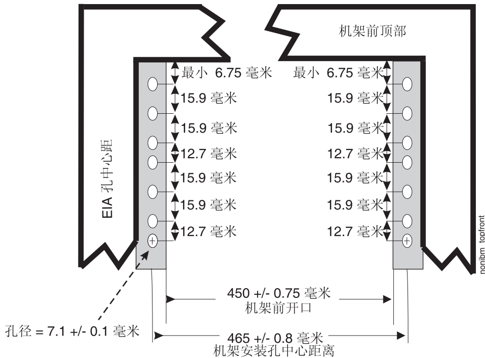
图 127. 机架规格尺寸，顶视图（前部）
