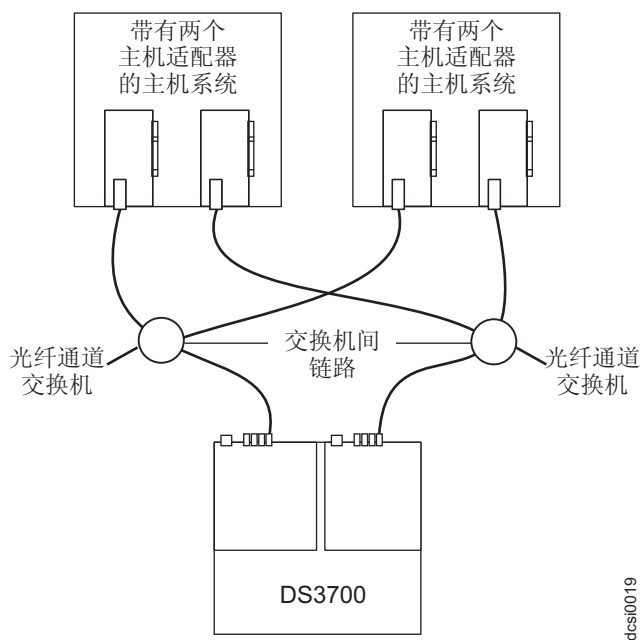
图 47. 单光纤通道 SAN 光纤网配置的示例
