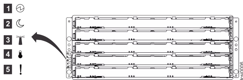
图 52. DCS3700 前部指示灯和控件
