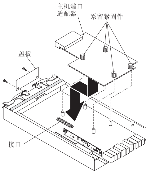
图 71. 安装主机端口适配器
