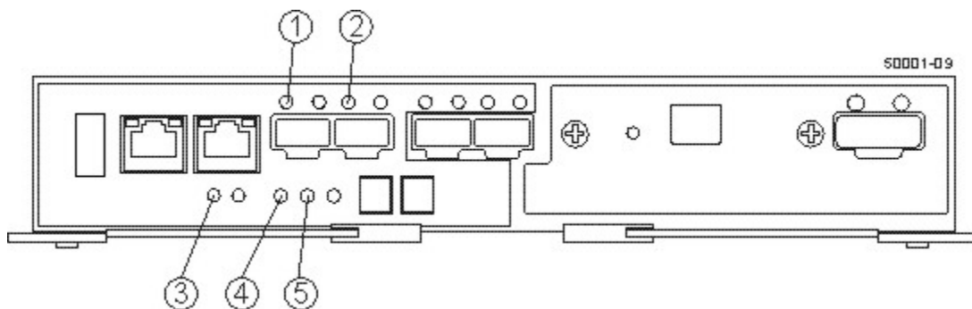
図 115. コントローラー LED
