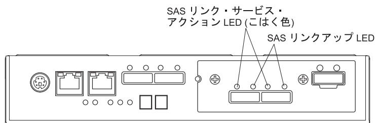
図 57. SAS ホスト・ポート・アダプター LED
