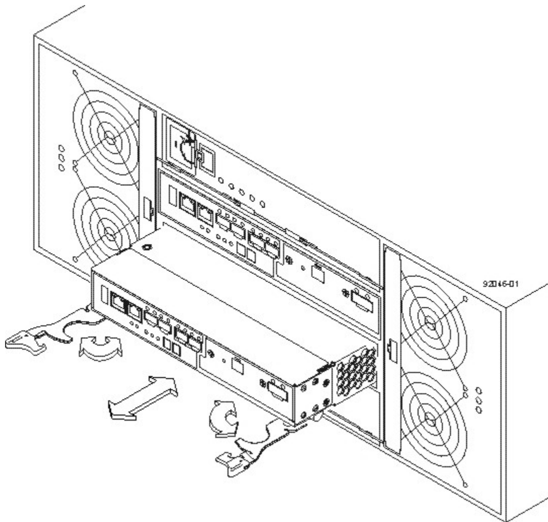
図 116. コントローラーの取り外しおよび再取り付け
