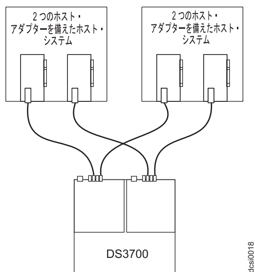
図 46. 複数のホスト内の複数の HBA へのデュアル・コントローラー直接ファイバー・チャンネル接続による接続
