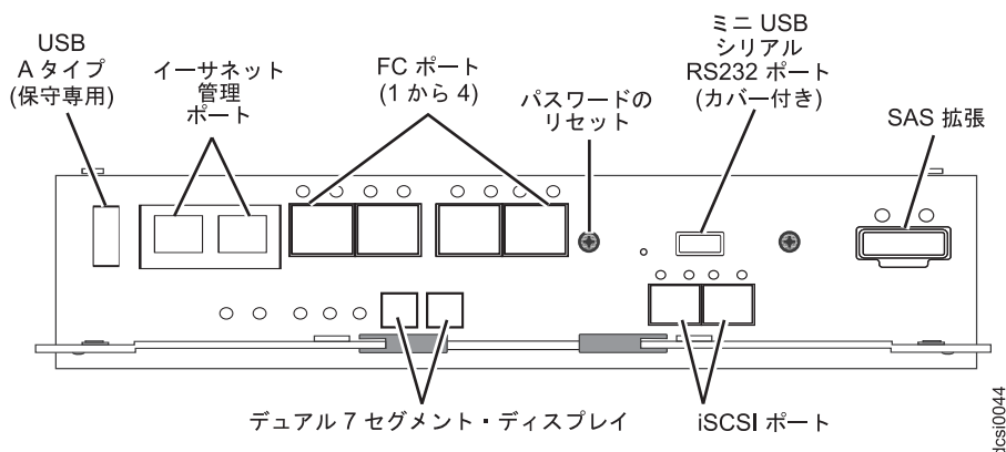
図 21. パフォーマンス・モジュール・コントローラー搭載の DCS3700 ストレージ・サブシステム (FC ポートを一覧)
