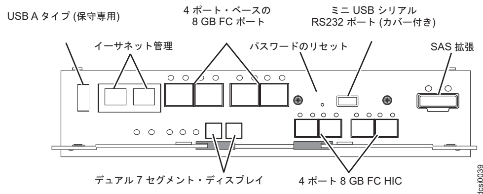
図 6. パフォーマンス・モジュール・コントローラー搭載の DCS3700 ストレージ・サブシステム上のコネクタ
