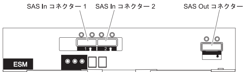
図 37. ESM のコネクター
