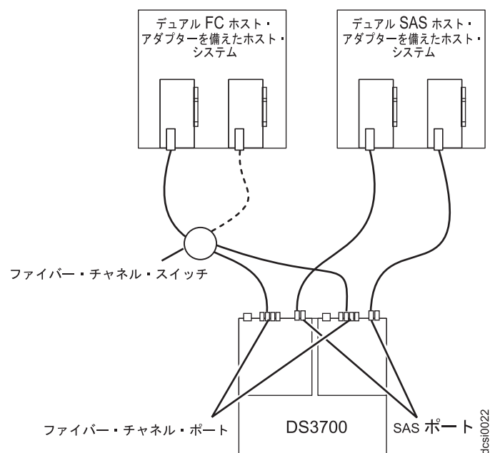
図 50. 複数ホスト、複数ポート、および複数ファブリック（ファイバー・チャンネルおよび SAS）構成の例
