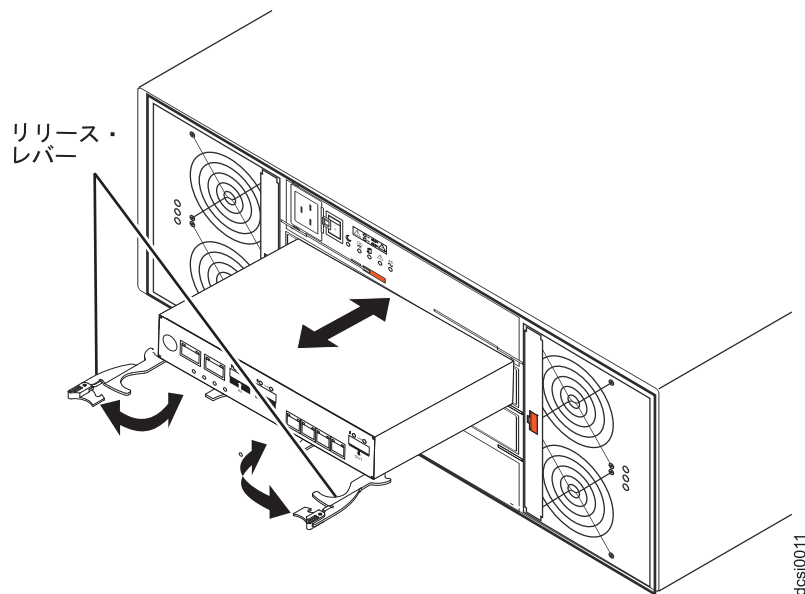
図 64. コントローラーの取り外し
