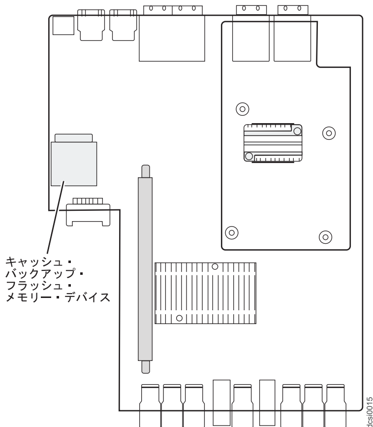
図 85. キャッシュ・バックアップ・フラッシュ・メモリー・デバイス
