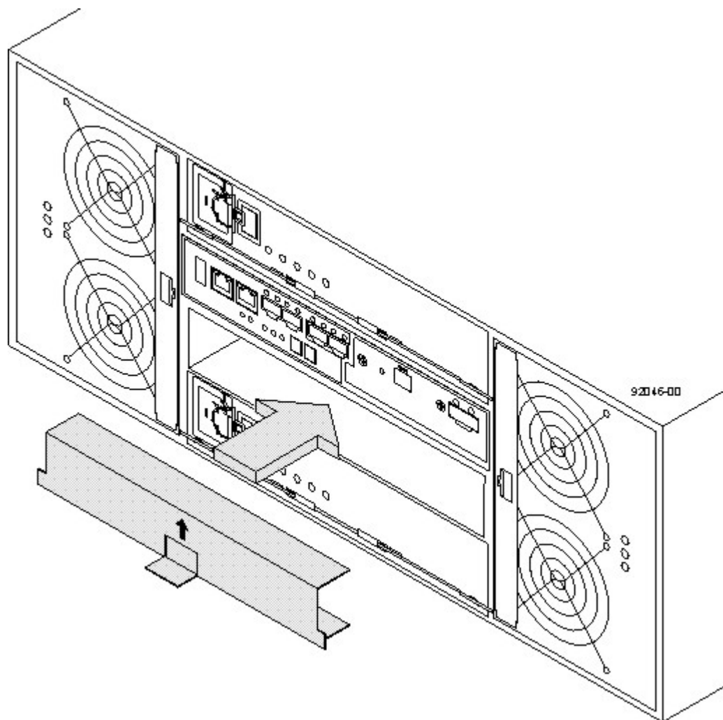
図 104. 開いたコントローラー・スロットへのコントローラー・エアー・セパレーターの挿入
