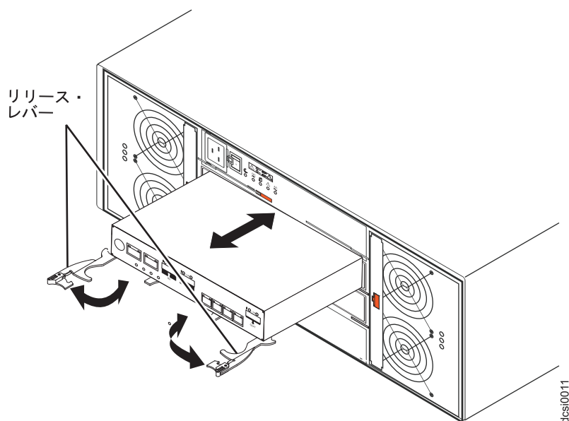
図 79. コントローラーの取り外し
