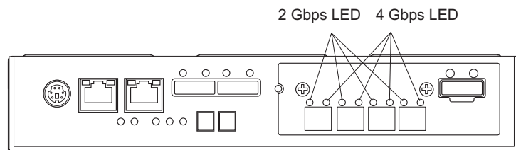
図 56. ファイバー・チャネル・ホスト・ポート・アダプター LED
