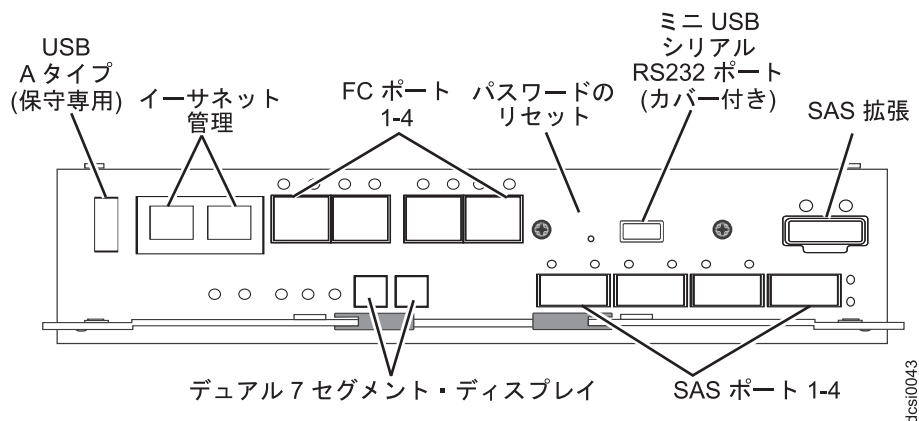
図 20. パフォーマンス・モジュール・コントローラー搭載の DCS3700 ストレージ・サブシステム (SAS 拡張として SAS ポートを一覧)
