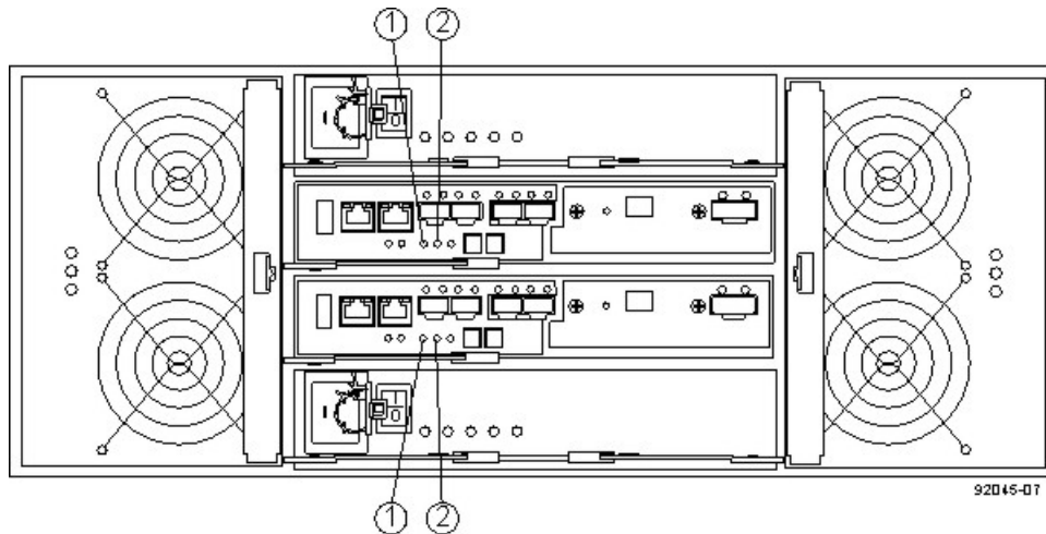
図 114. コントローラー保守処置 LED
