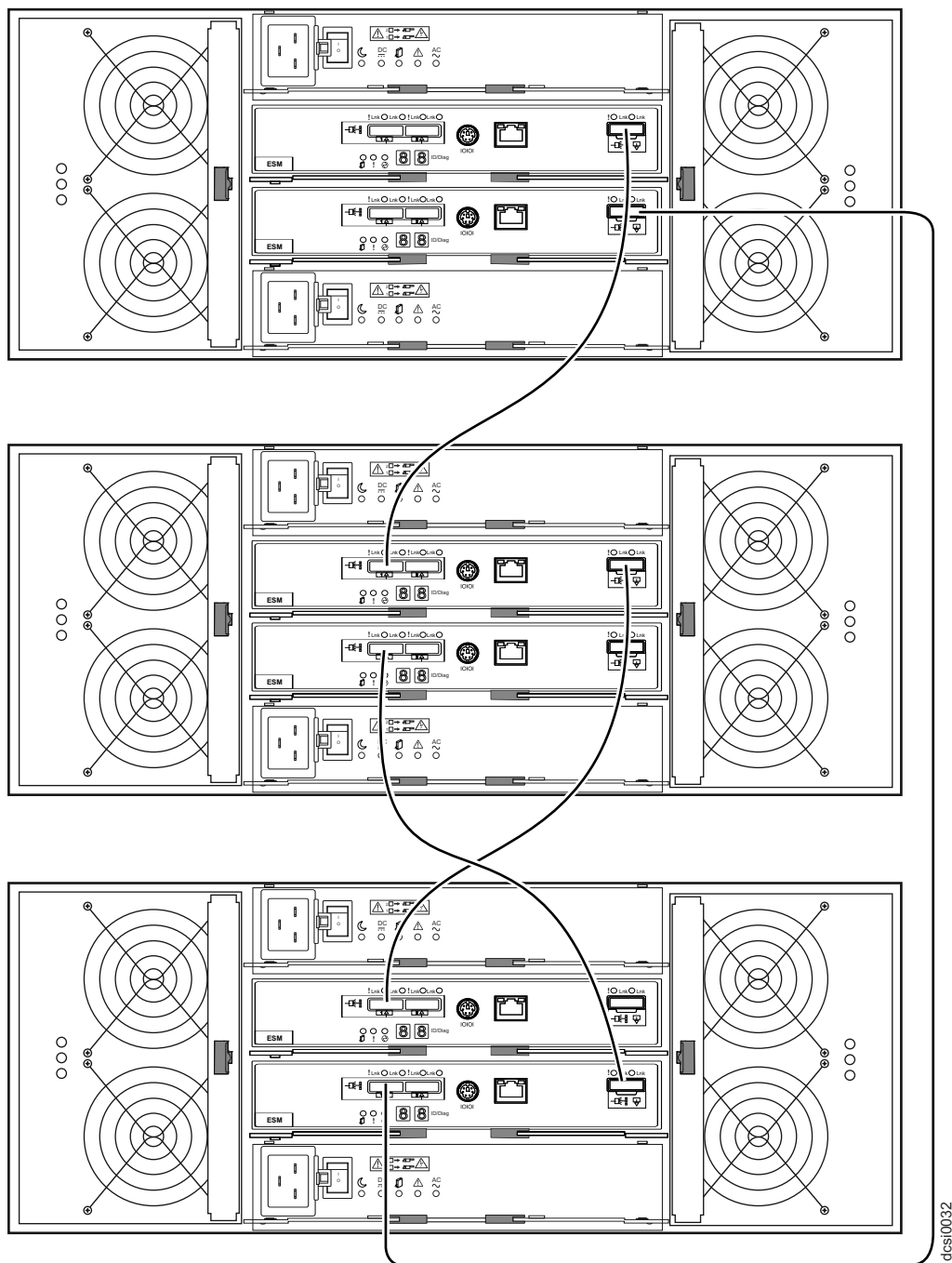
図 39. デュアル拡張エンクロージャー
