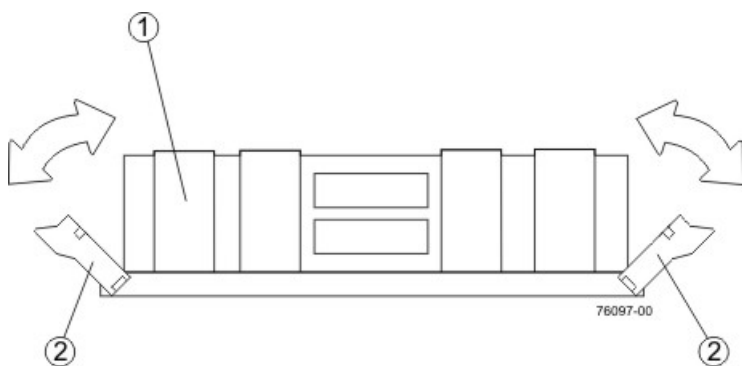
図 106. キャッシュ・メモリー DIMM の取り外し
