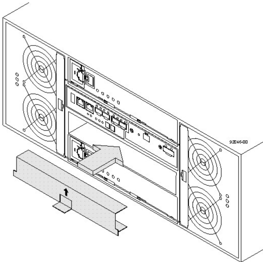
図 111. 開いたコントローラー・スロットへのコントローラー・エアー・セパレーターの挿入
