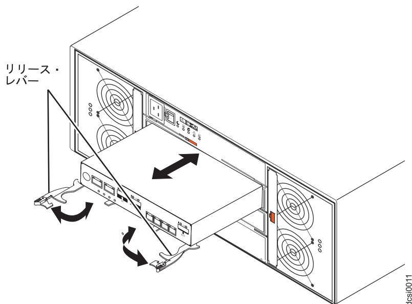
図 66. コントローラーの取り外しと交換
