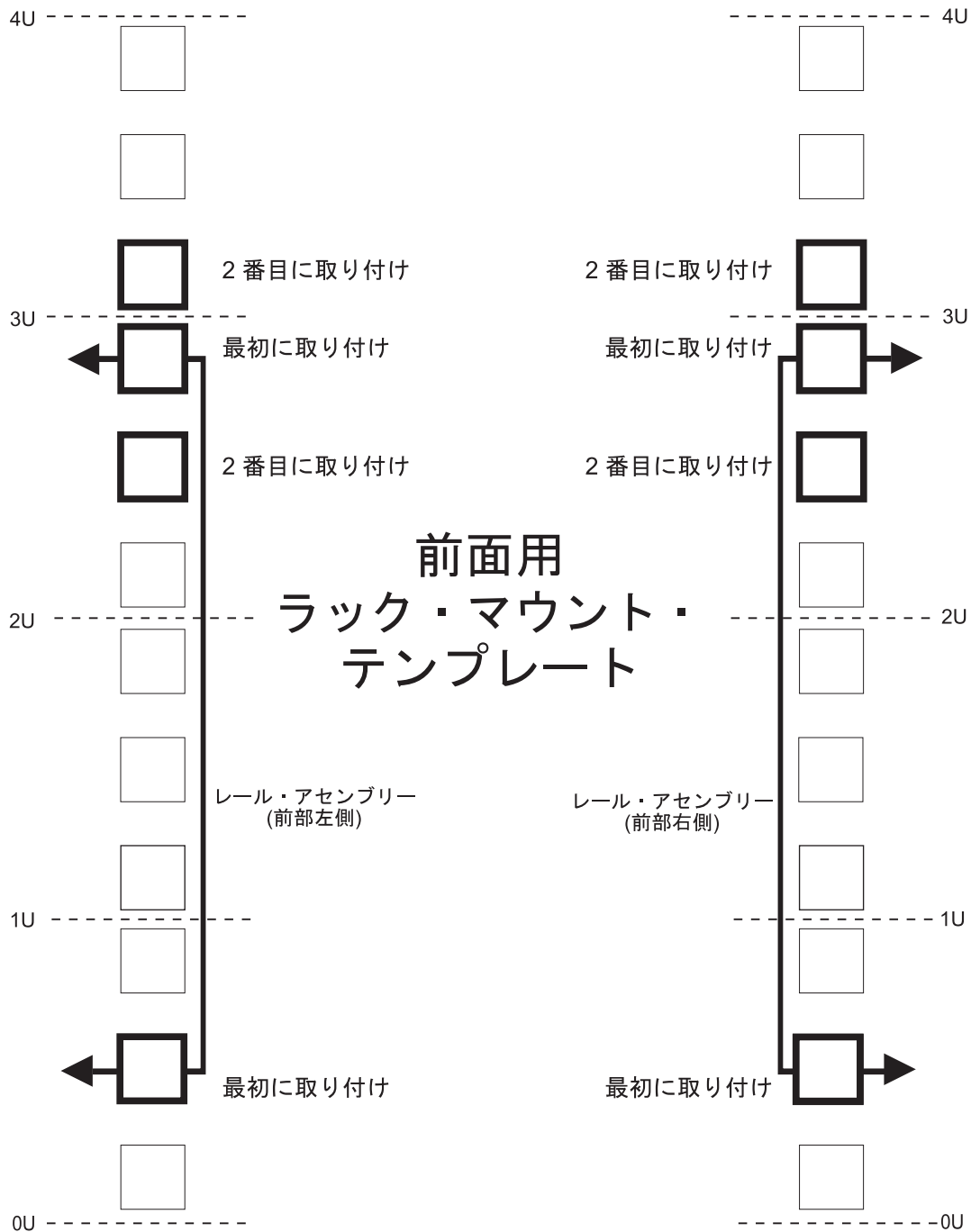
図 124. 前面用ラック・マウント・テンプレート
