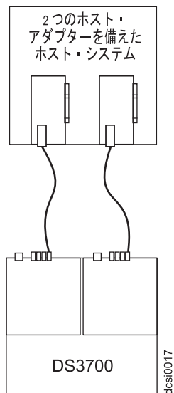
図 45. 同一ホスト内の 2 つの HBA へのデュアル・コントローラー直接ファイバー・チャンネル接続による接続 (冗長ホスト接続)
