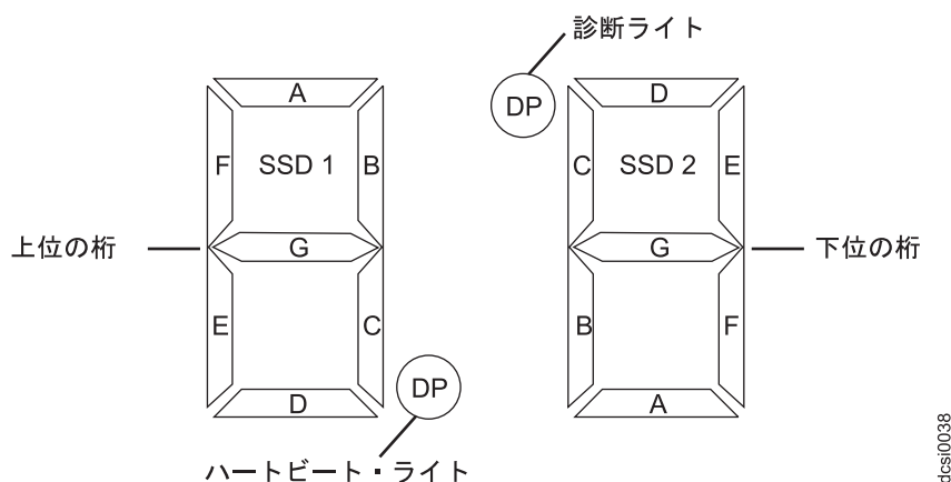
図 63. 数値ディスプレイ LED
