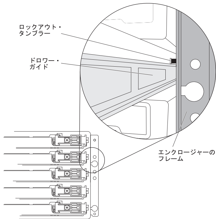
図 99. ロック・タンブラーがドロワー・ガイドより上にある場合
