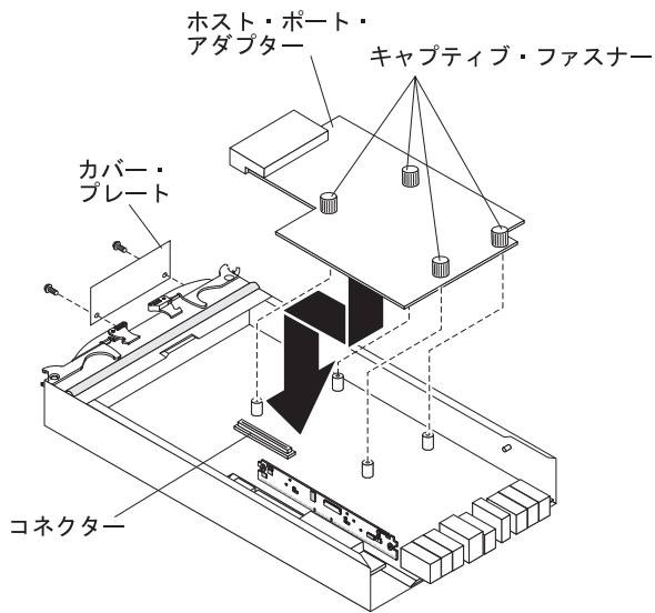
図 71. ホスト・ポート・アダプターの取り付け
