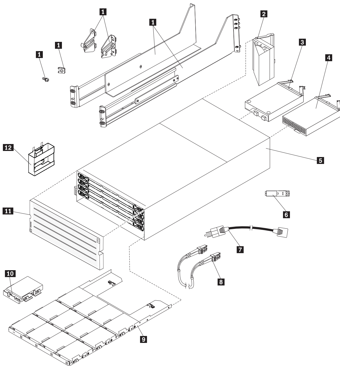
図 121. DCS3700 ストレージ・サブシステム・エンクロージャー部品リスト
