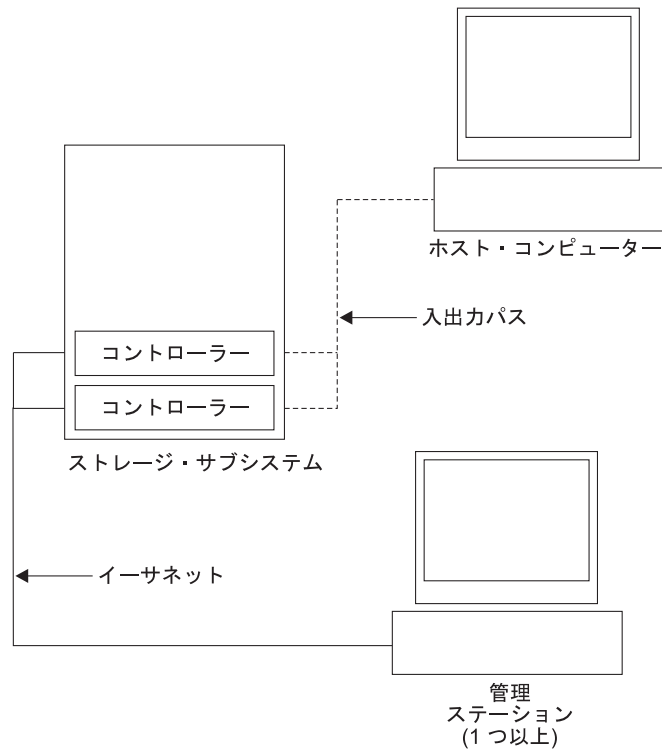
図 41. 直接 (アウト・オブ・バンド) 管理方式
