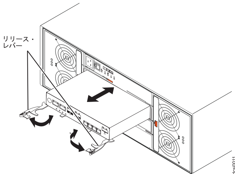
図 87. 環境サービス・モジュールの取り外し
