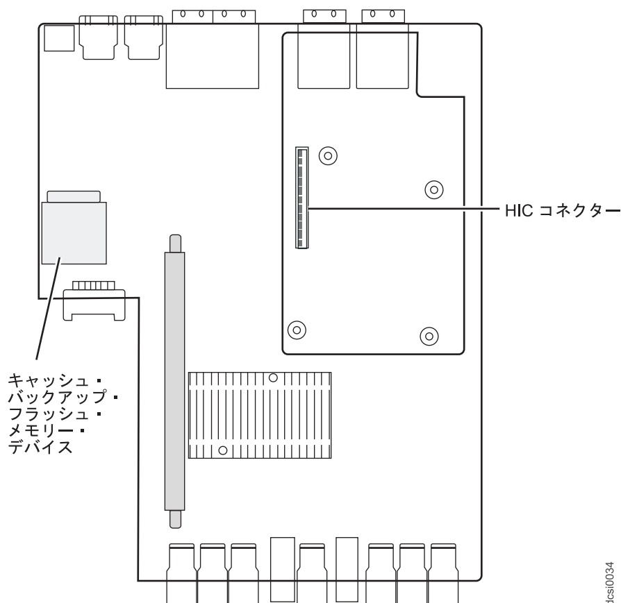
図 72. HIC コネクターの位置合わせ
