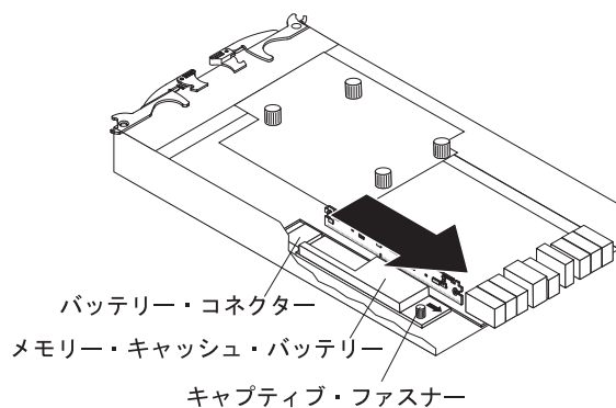
図 67. コントローラーからのバッテリー・ユニットの取り外し
