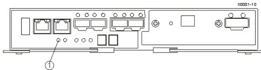
図 107. コントローラー上のバッテリーの要保守処置 LED
