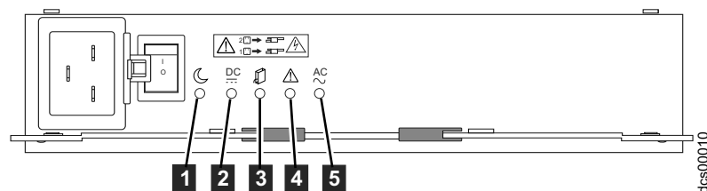
図 60. AC 電源機構 LED
