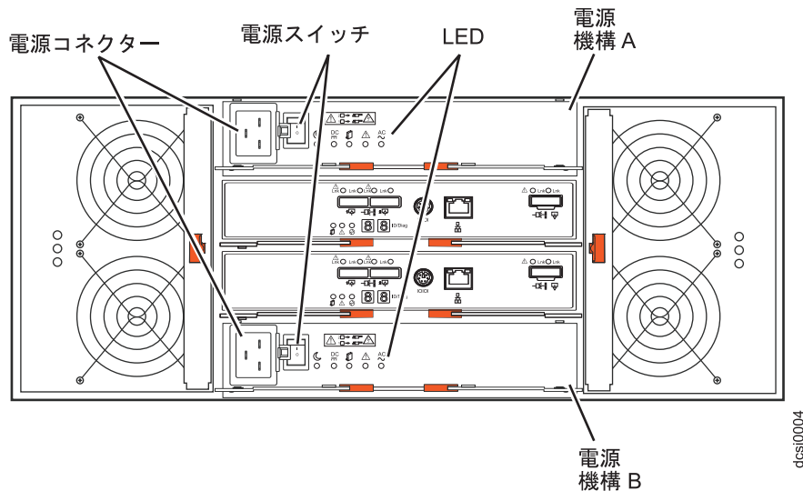
図 51. DCS3500 DC モデルの電源機構のスイッチとコネクタ
