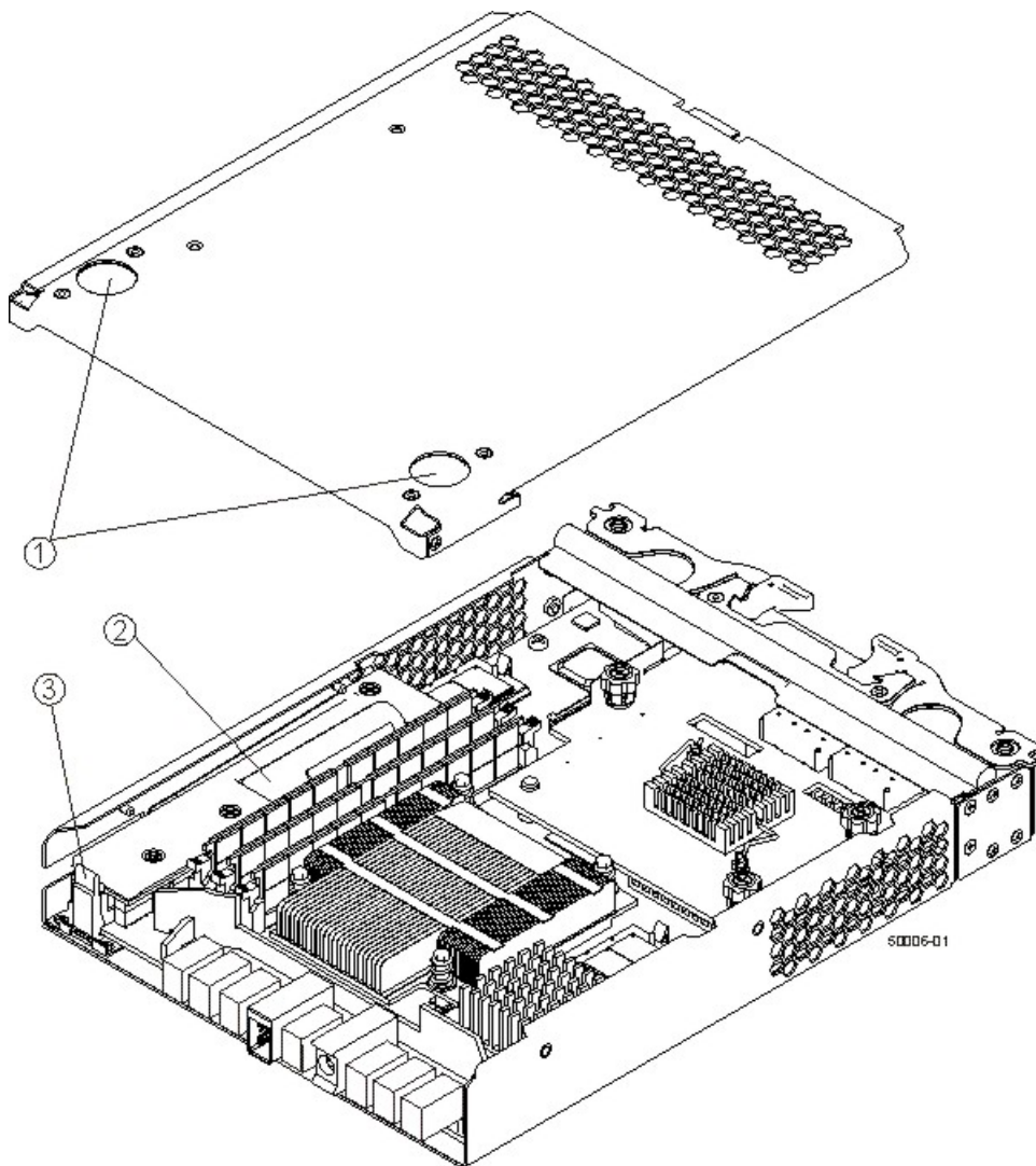
図 112. コントローラーの上部カバー・ラッチ・ボタン
