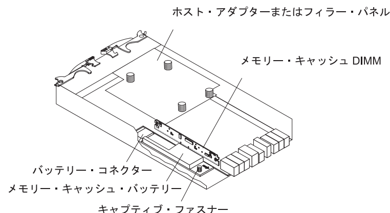
図 81. メモリー・キャッシュ DIMM の位置
