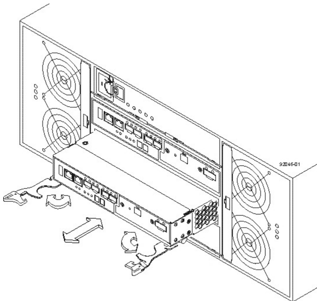
図 109. コントローラーの取り外しと交換
