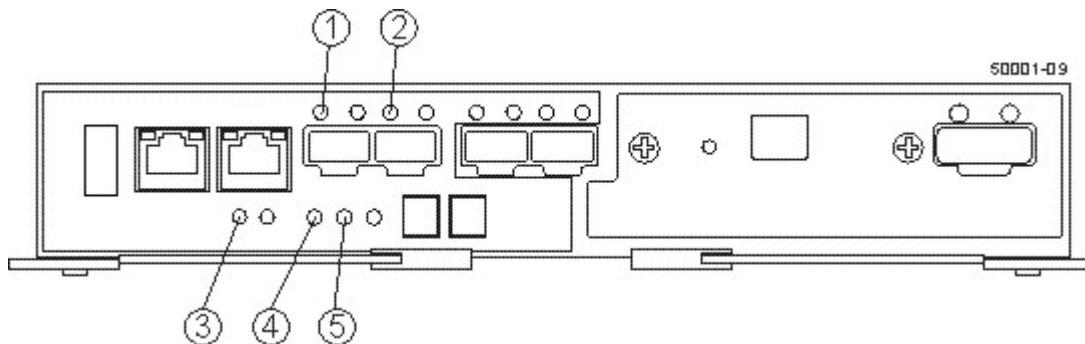
図 120. コントローラー LED
