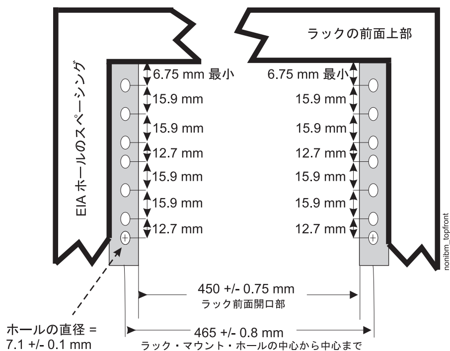
図 127. ラックの仕様寸法 (正面図)
