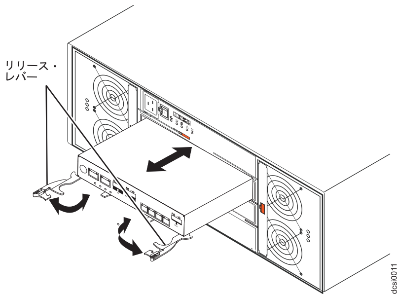
図 100. コントローラーの取り外しと交換
