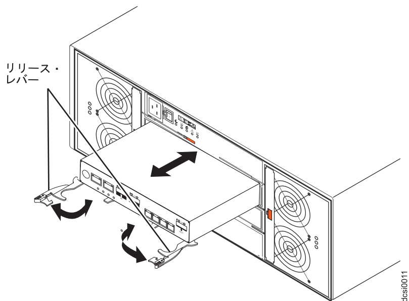
図 69. コントローラーの取り外し
