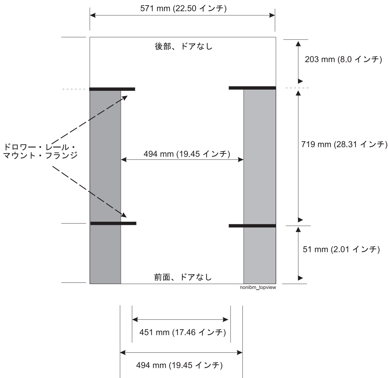
図 126. IBM 以外のラックの仕様寸法の平面図
