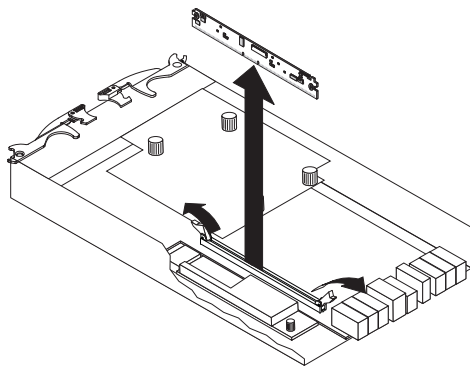
図 84. コントローラーへの DIMM のインストール
