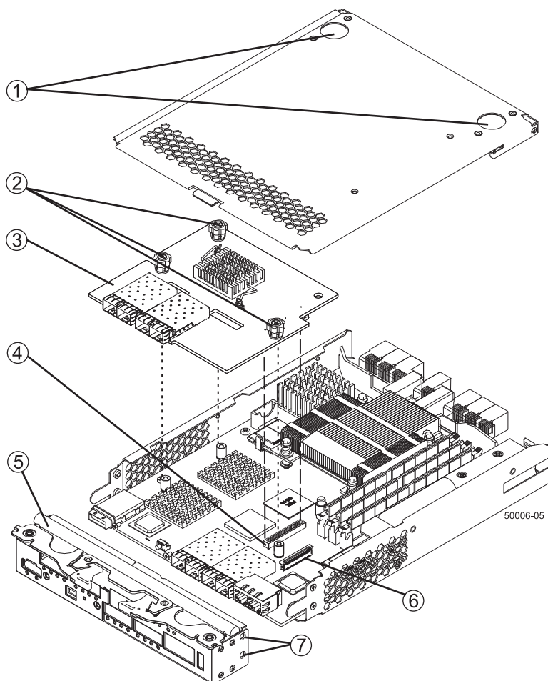
図 119. ホスト・インターフェース・カードの交換
