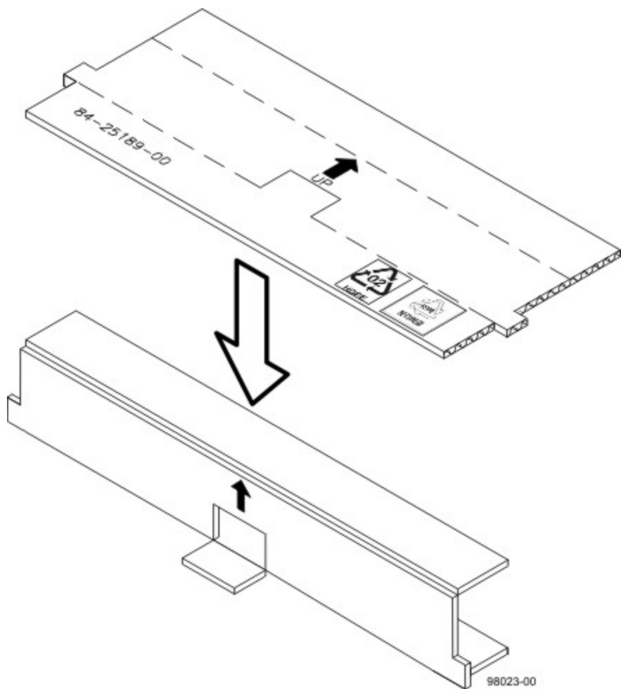
図 103. コントローラー・エアー・セパレーター
