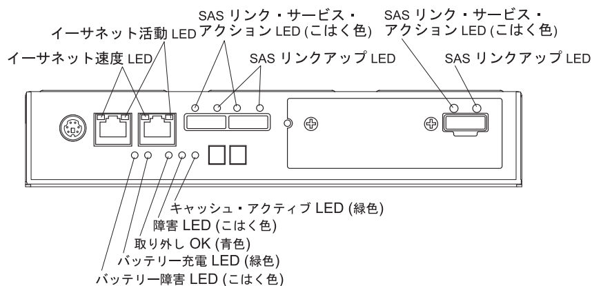
図 54. コントローラー LED
