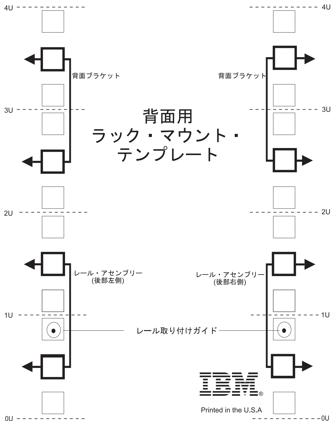
図 125. 背面用ラック・マウント・テンプレート
