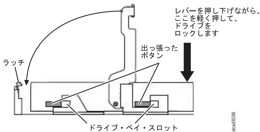
図 74. ハード・ディスクのコネクタへの挿入
