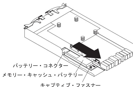
図 80. コントローラーからのバッテリー・ユニットの取り外し
