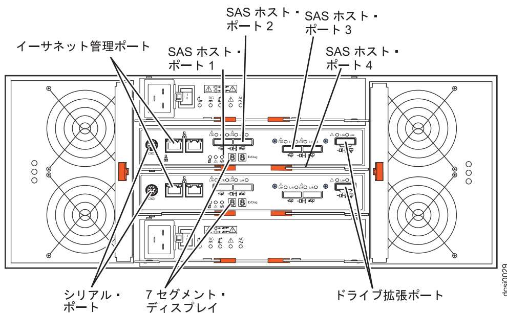
図 19. デュアル・コントローラー DCS3700 ストレージ・サブシステムのポートとコントローラー (オプションの SAS ホスト・ポート・アダプターを装備)
