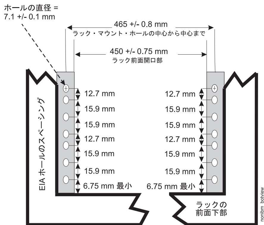
図 128. ラックの仕様寸法 (下部正面図)
