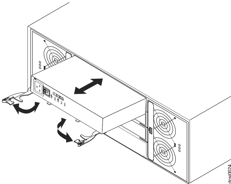
図 78. 電源機構の交換
