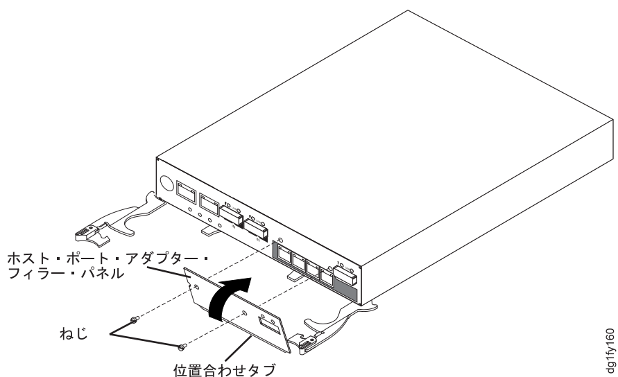
図 70. ホスト・ポート・アダプター・フィラー・パネルの取り外し
