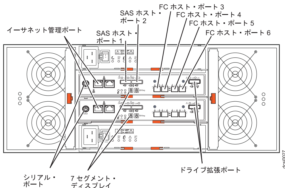
図 22. デュアル・コントローラー DCS3700 ストレージ・サブシステムのポートとコントローラー (オプションのファイバー・チャネル・ホスト・ポート・アダプターを装備)
