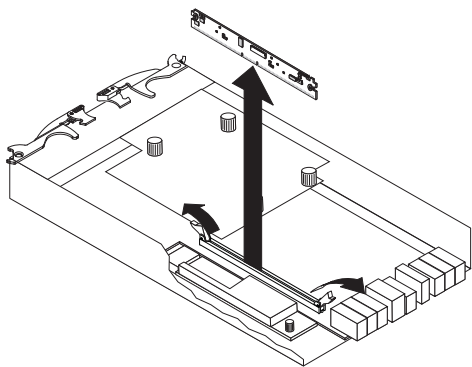
図 83. コントローラーからの DIMM の取り外し
