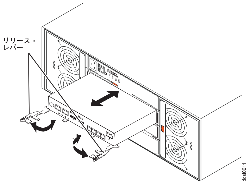
図 82. コントローラーの取り外し
