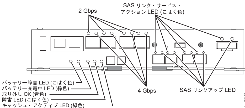
図 55. パフォーマンス・モジュール・コントローラー搭載のサブシステムのコントローラー LED
