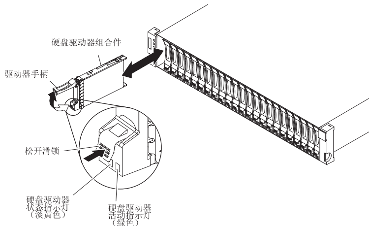
图 5-16. 在 DS3524 或 EXP3524 中安装驱动器
