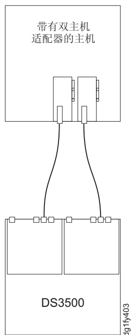
图 3-34. 与同一主机中两个 HBA 的双控制器直接连接的 SAS 连接（冗余主机连接）
