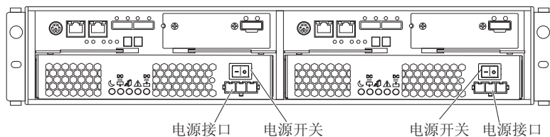
图 5-24. DS3500 直流型号电源开关和接口
