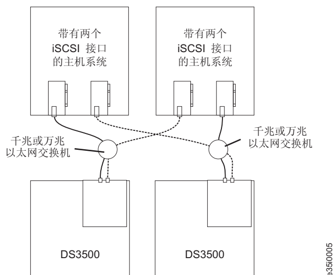
图 3-53. 多主机、多端口、多存储子系统的 iSCSI 配置
