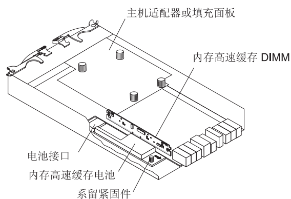
图 5-28. 内存高速缓存 DIMM 的位置
