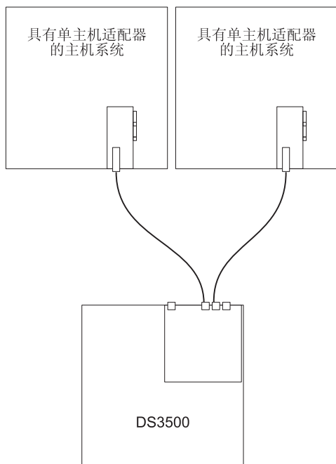
图 3-33. 与多主机中单 HBA 的单控制器直接连接的 SAS 连接
