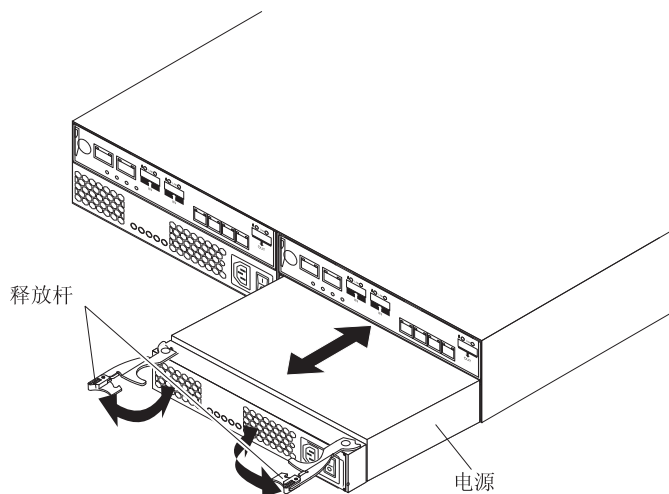
图 5-25. 更换电源
