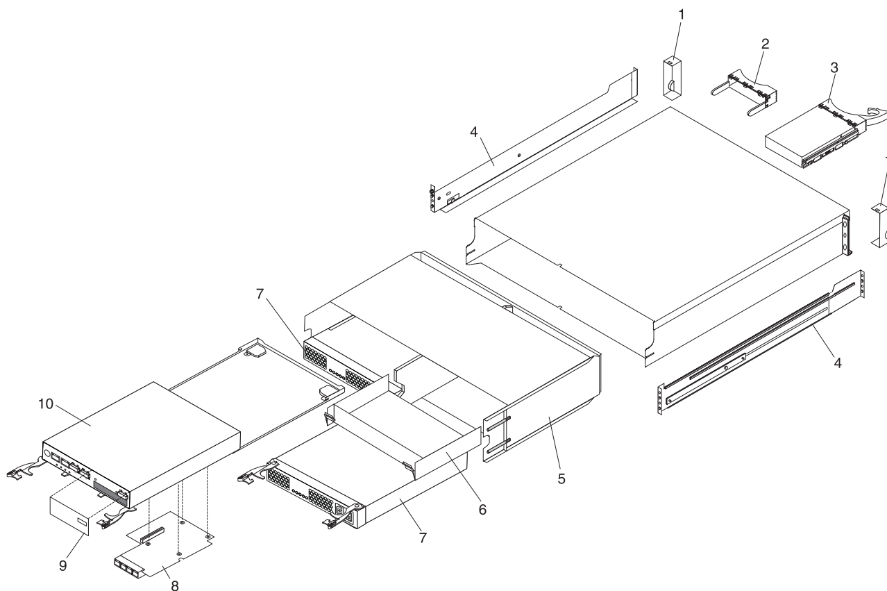
图 7-1. DS3512 存储子系统和 EXP3512 存储机柜的部件
