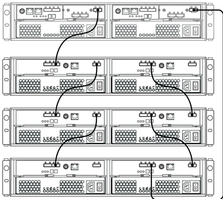
图 3-23. 冗余驱动器路径的示例
