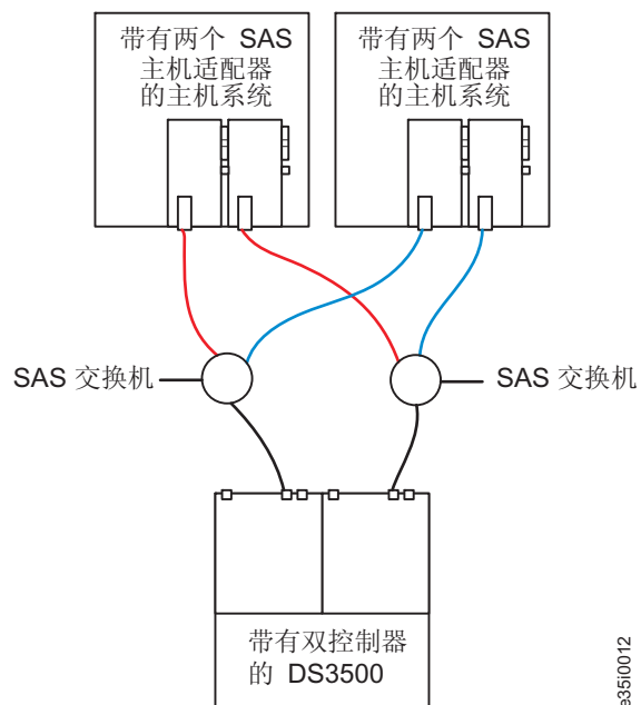
图 3-37. 使用两个独立的 SAS 交换机从双控制器 DS3500 SAS 到多个主机的连接
