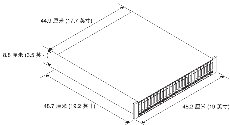
图 1-14. DS3524 存储子系统和 EXP3524 存储机柜的尺寸
