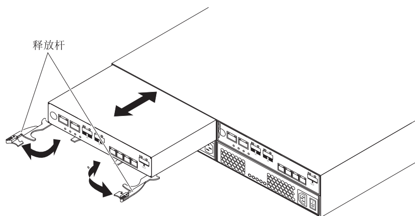
图 5-1. 卸下控制器
