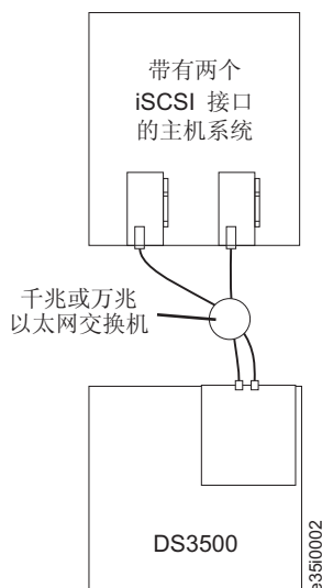
图 3-50. 多端口、单控制器的 iSCSI 配置
