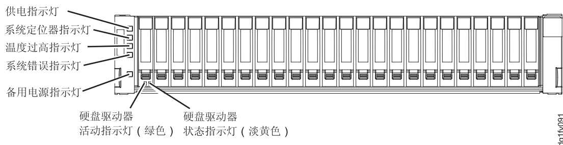
图 5-32. DS3524 存储子系统和 EXP3524 存储机柜前部指示灯
