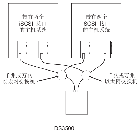
图 3-52. 多主机、多端口、单控制器和冗余路径的 iSCSI 配置
