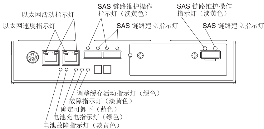
图 5-33. 控制器指示灯
