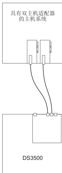
图 3-32. 与单主机中双 HBA 的单控制器直接连接的 SAS 连接（冗余主机连接）
