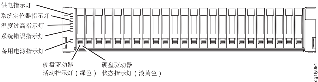
图 4-6. DS3524 存储子系统和 EXP3524 存储机柜前部指示灯
