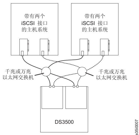
图 3-55. 多主机、多端口、双控制器的 iSCSI 配置
