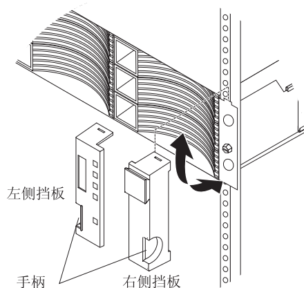
图 5-35. 卸下挡板
