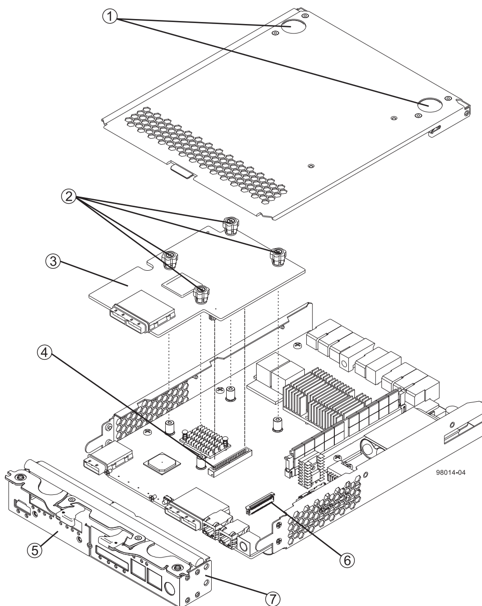
图 5-7. 卸下控制器组件的顺序
