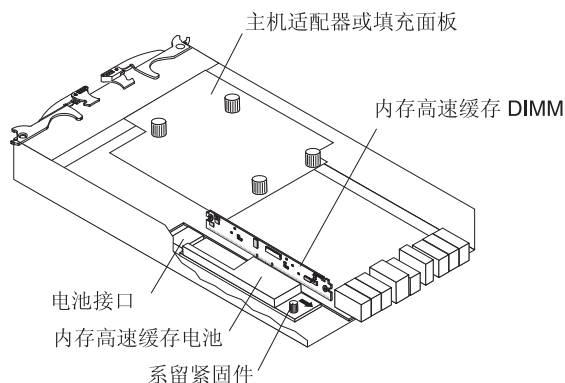
图 1-12. 电池单元
