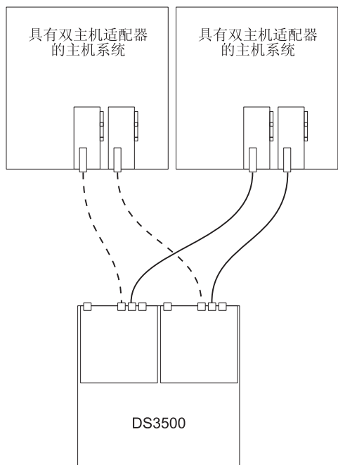
图 3-35. 与多主机中多个 HBA 的双控制器直接连接的 SAS 连接
