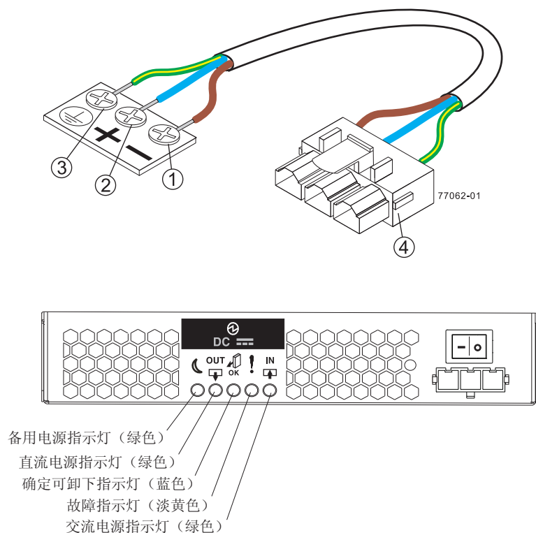
图 5-23. DS3500 直流型号的直流电源接口
