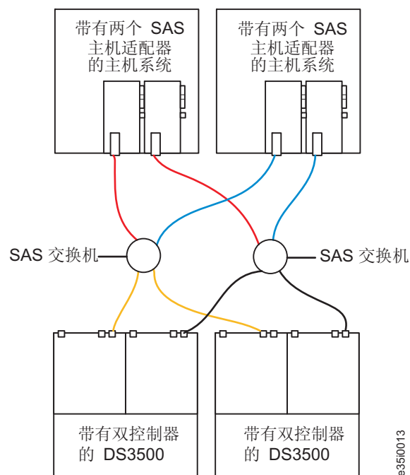
图 3-38. 使用两个独立的 SAS 交换机从多个双控制器 DS3500 SAS 到多个主机的连接
