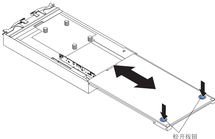
图 5-2. 卸下外盖
