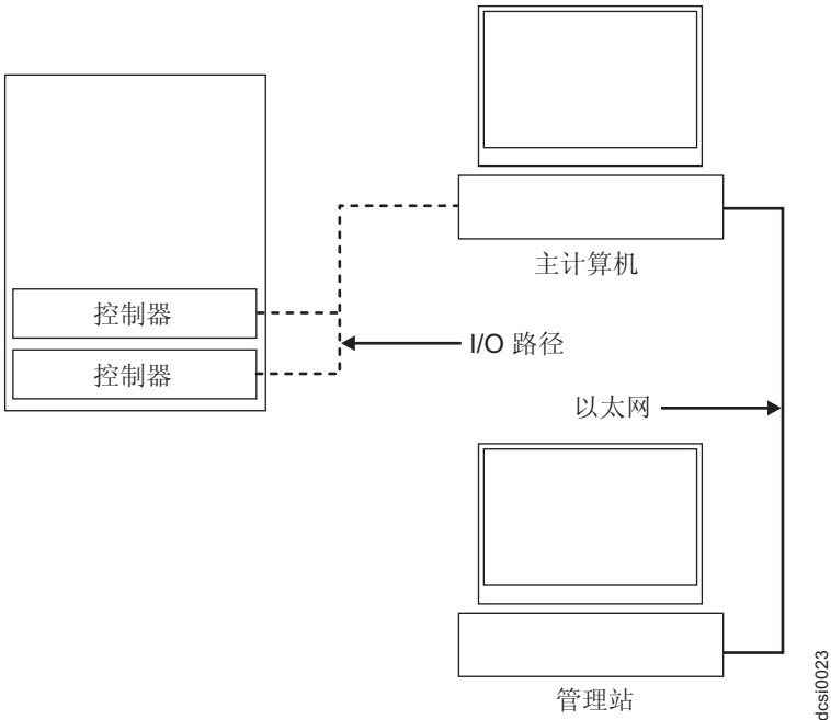
图 3-29. 主机代理（频带内）受管存储子系统
