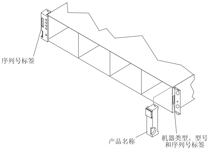
图 A-1. DS3500 上的序列号位置
