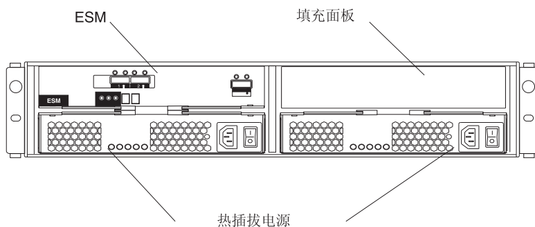
图 1-8. 后视图，单个 ESM 型存储机柜
