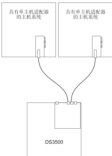
图 3-43. 与多主机中单 HBA 的单控制器直接连接的光纤通道连接
