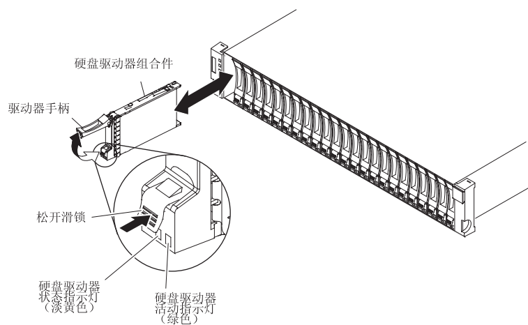
图 5-14. 从 DS3524 或 EXP3524 中卸下驱动器
