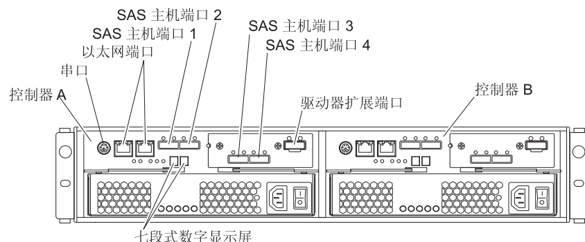
图 3-4. 双控制器 DS3500 存储子系统端口和控制器（带有可选 SAS 主机端口适配器）
