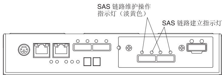
图 4-10. SAS 主机端口适配器指示灯
