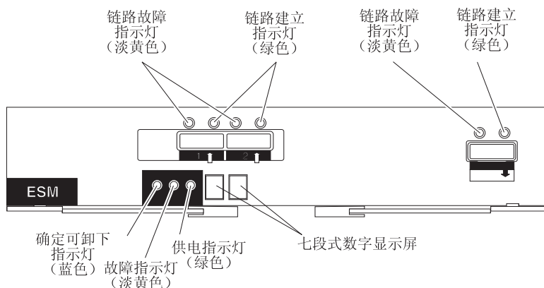
图 4-13. ESM 指示灯
