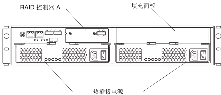
图 1-7. 后视图，单控制器型（未安装可选主机端口适配器）
