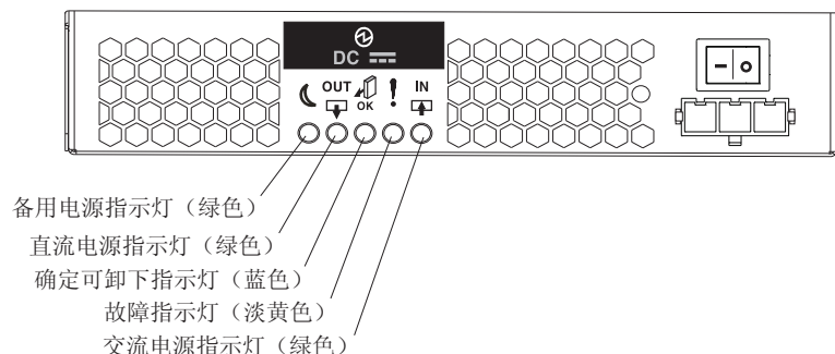
图 5-22. 直流电源指示灯
