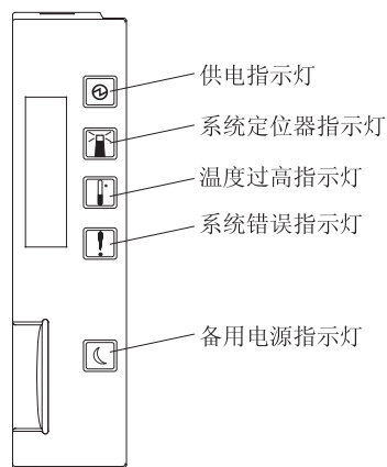
图 1-4. 左侧挡板
