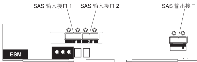
图 3-22. ESM 接口
