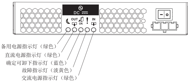
图 4-4. 直流电源指示灯
