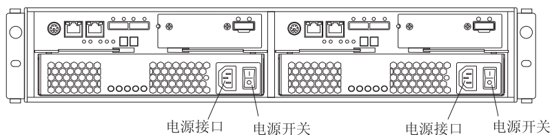
图 5-20. DS3500 交流型号电源开关和接口
