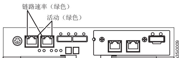
图 4-11. 10 Gbps iSCSI 端口指示灯
