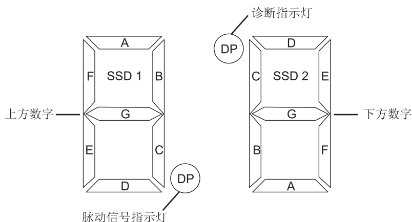
图 4-12. 数字显示屏指示灯
