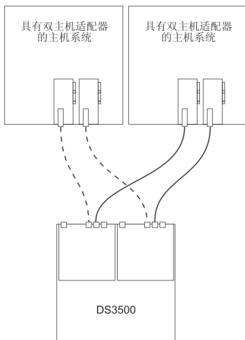
图 3-45. 与多主机中多个 HBA 的双控制器直接连接的光纤通道连接
