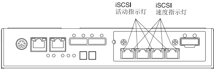
图 4-8. iSCSI 主机端口适配器指示灯
