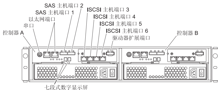
图 3-2. 双控制器 DS3500 存储子系统端口和控制器（带有可选 iSCSI 主机端口适配器）
