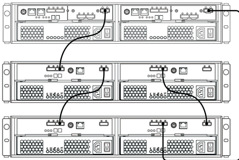
图 3-26. 一个双控制器 DS3500 和两个存储机柜
