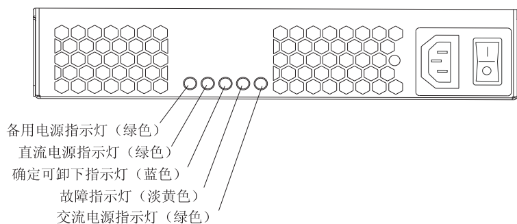
图 5-19. 交流电源指示灯
