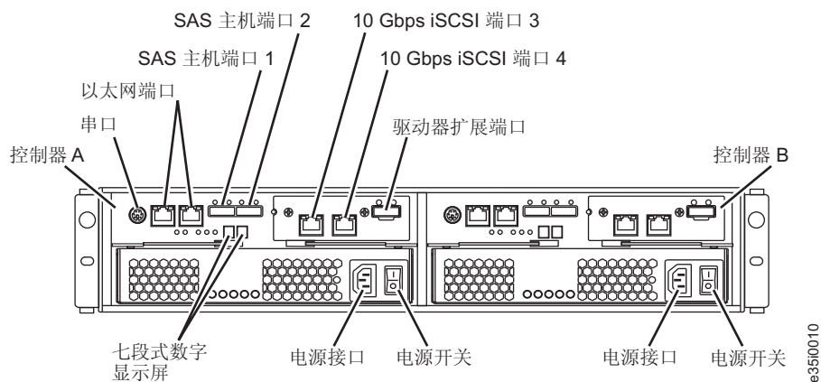
图 3-3. 双控制器 DS3500 存储子系统端口和控制器（带有可选 10 iSCSI 主机端口适配器）
