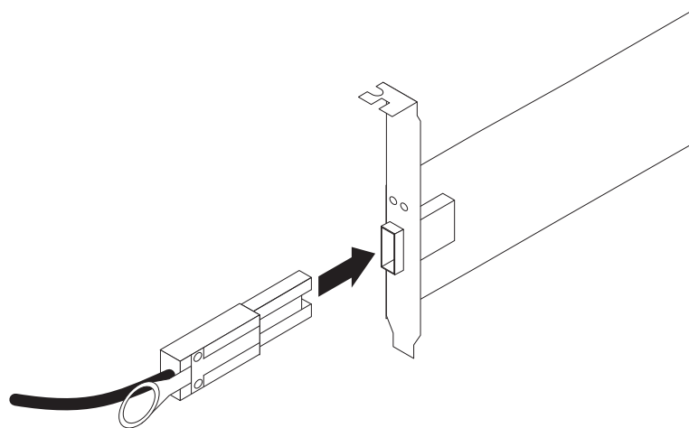
图 3-6. 连接迷你 SAS 电缆
