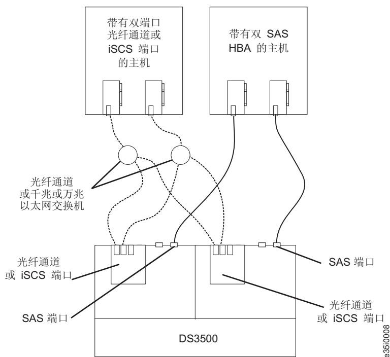
图 3-56. 多主机、多端口和多光纤网（光纤通道或 iSCSI 和 SAS）配置的示例
