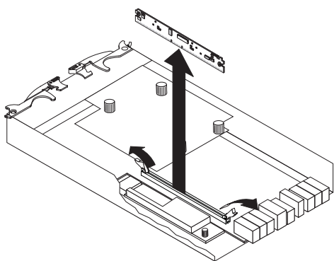
图 5-30. 从控制器上卸下 DIMM
