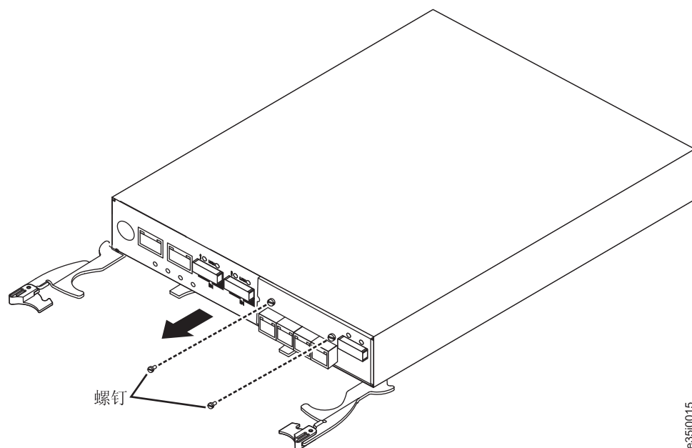
图 5-10. 安装主机端口适配器
