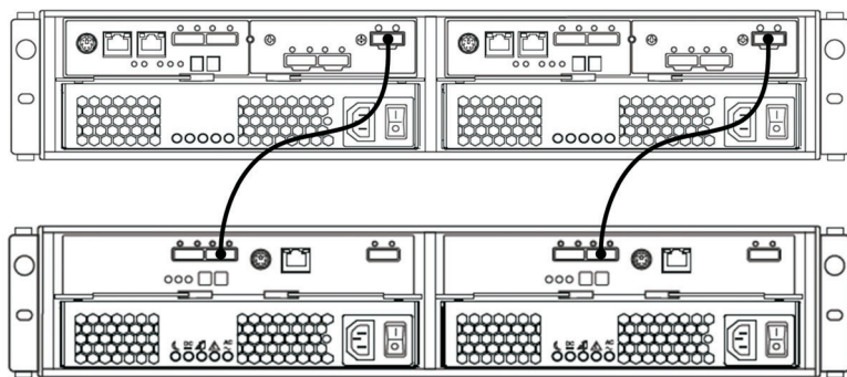
图 3-25. 一个双控制器 DS3500 和一个存储机柜
