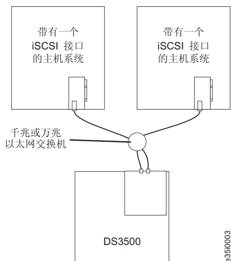
图 3-51. 多个单端口主机、单控制器的 iSCSI 配置
