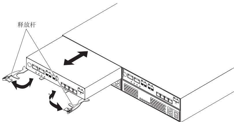
图 5-8. 卸下控制器
