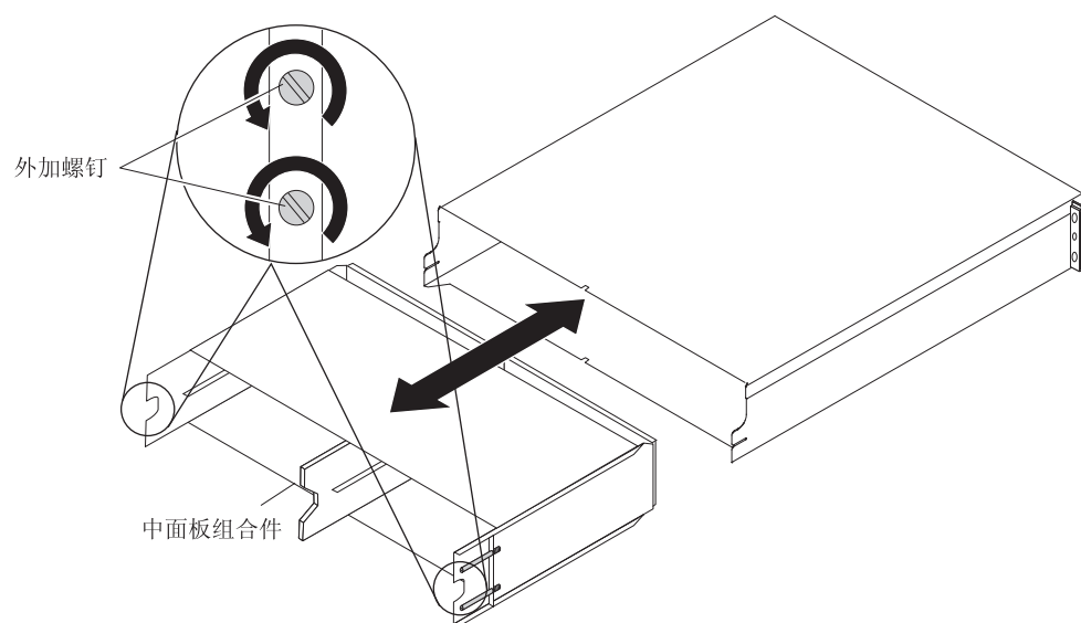
图 5-37. 更换 DS3512 或 EXP3512 中的中面板组合件
