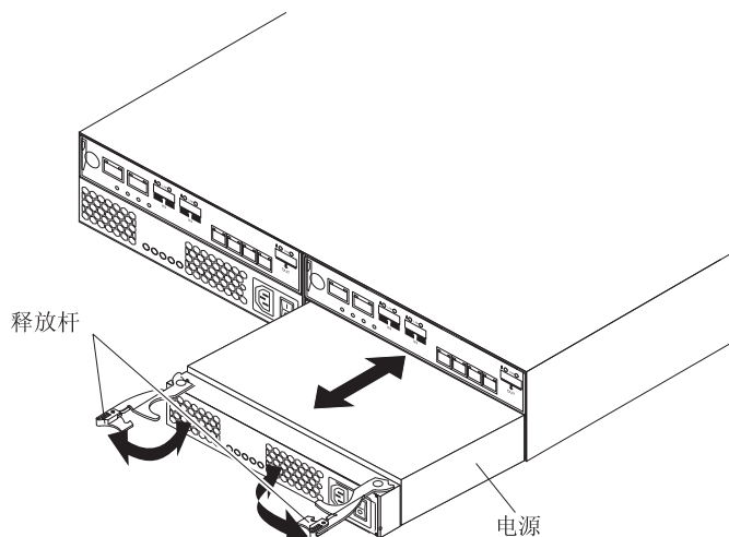
图 5-17. 更换电源
