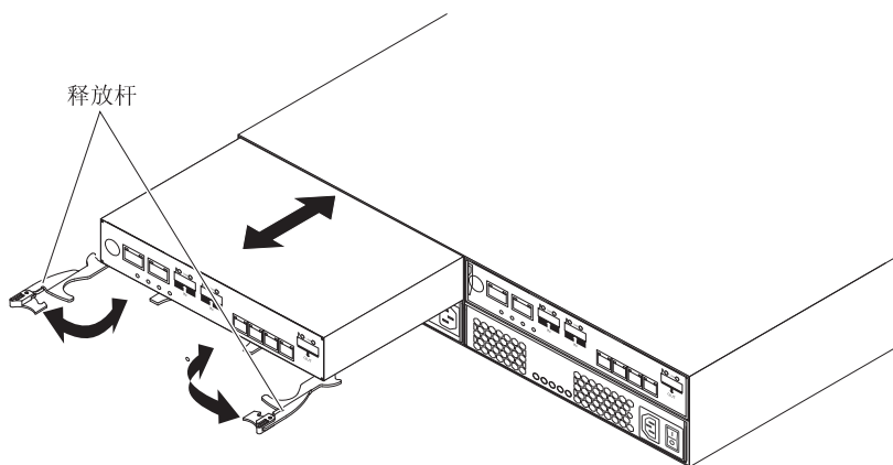
图 5-4. 卸下并重新安装控制器
