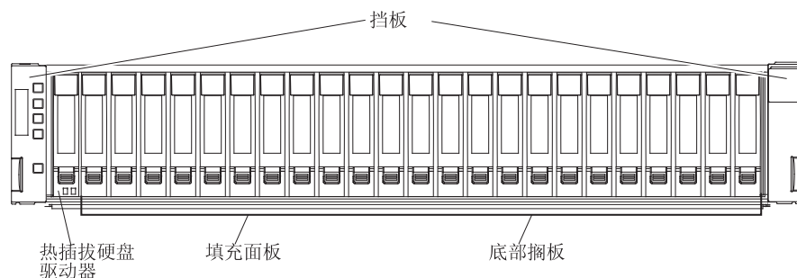
图 1-3. DS3524 存储子系统和 EXP3524 存储机柜的热插拔驱动器托架和挡板
