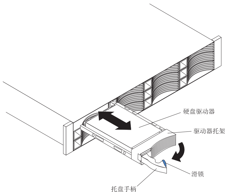
图 5-13. 从 DS3512 或 EXP3512 中卸下驱动器
