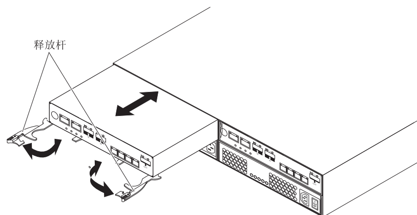
图 5-26. 卸下控制器
