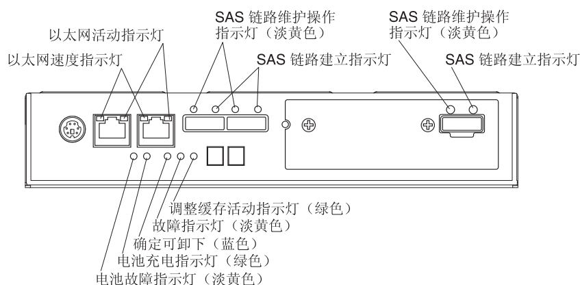
图 4-7. 控制器指示灯
