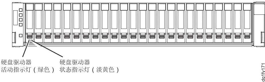
图 5-12. DS3524 存储子系统和 EXP3524 存储机柜驱动器指示灯
