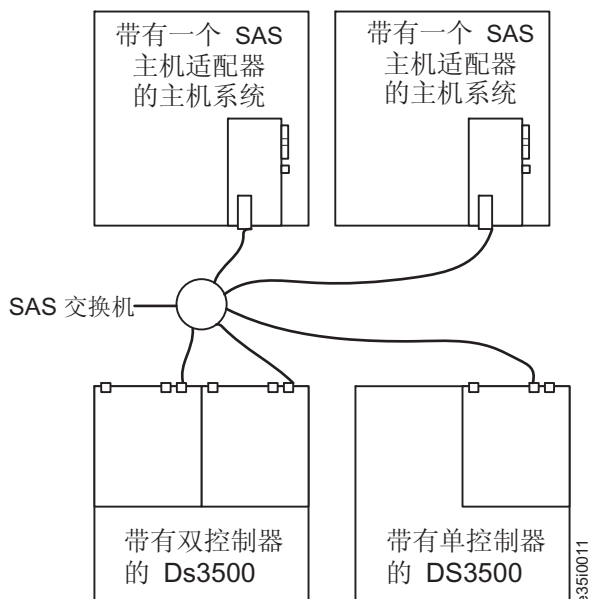
图 3-36. 使用一个 SAS 交换机的双控制器 DS3500 或单控制器 DS3500 SAS 到多个主机的连接
