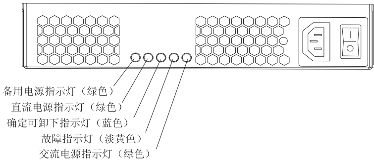
图 4-3. 交流电源指示灯
