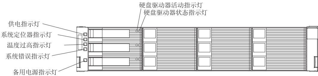
图 4-5. DS3512 存储子系统和 EXP3512 存储机柜前部指示灯和控件
