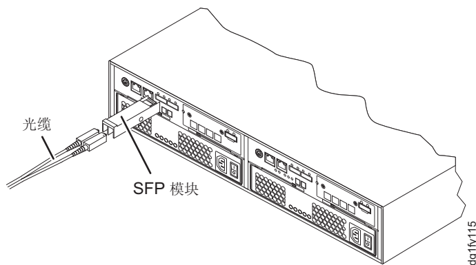
图 5-34. 将 SFP 模块安装到主机端口中
