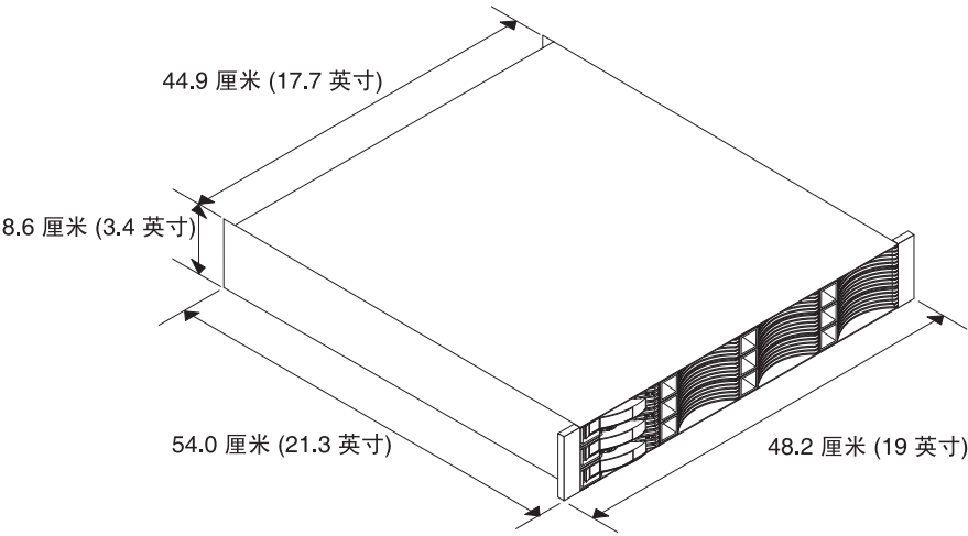
图 1-13. DS3512 存储子系统和 EXP3512 存储机柜的尺寸
