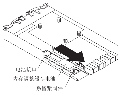
图 5-5. 从控制器上卸下电池单元
