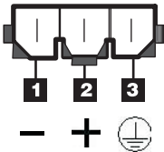
图 1-11. 直流电源接口 - 插脚位置
