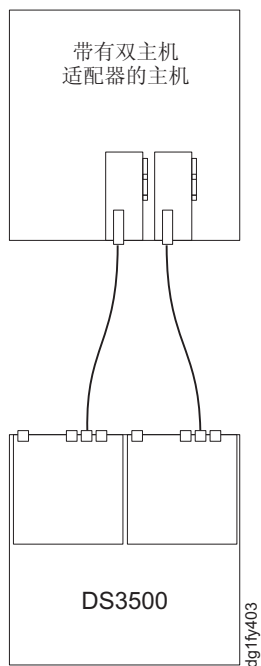
图 3-44. 与同一主机中两个 HBA 的双控制器直接连接的光纤通道连接（冗余主机连接）
