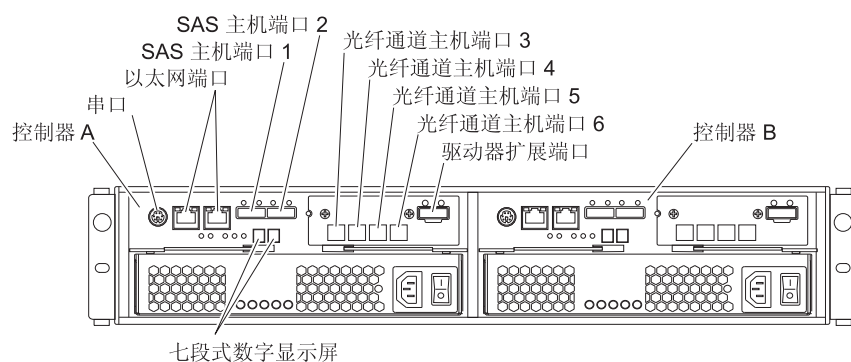
图 3-1. 双控制器 DS3500 存储子系统端口和控制器（带有可选光纤通道主机端口适配器）
