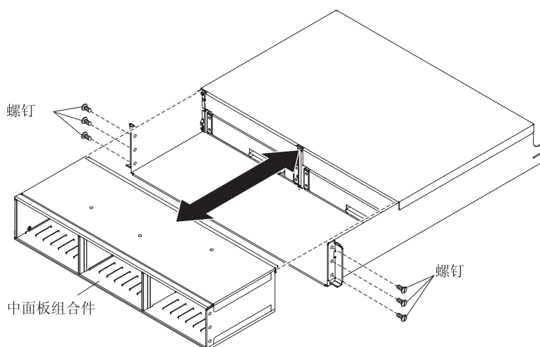
图 5-38. 更换 DS3524 或 EXP3524 中的中面板组合件
