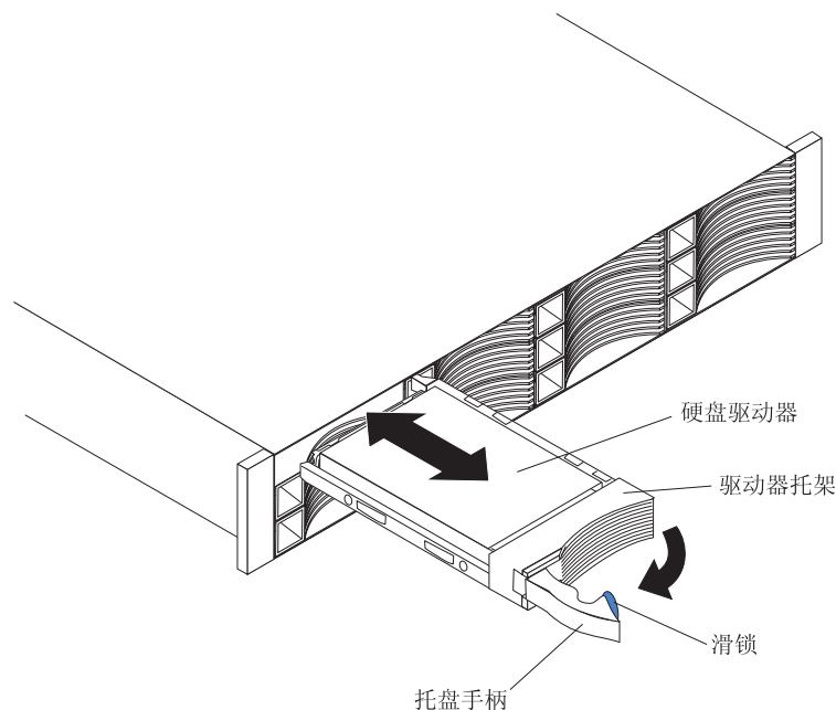
图 5-15. 在 DS3512 或 EXP3512 中安装驱动器
