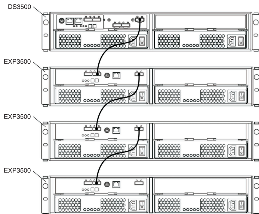
图 3-24. 一个单控制器 DS3500 和多个单 ESM 存储机柜
