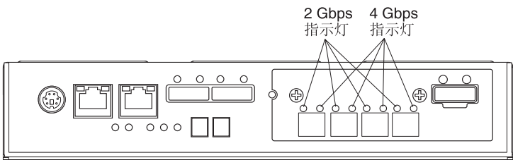
图 4-9. 光纤通道主机端口适配器指示灯
