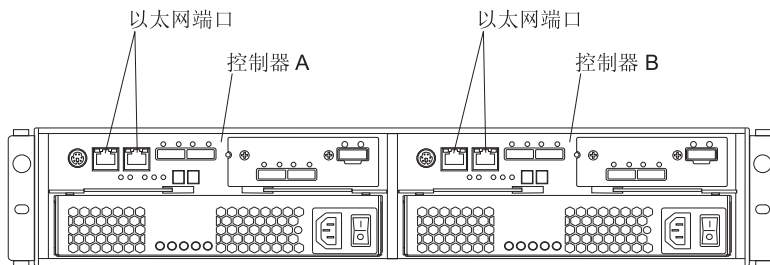
图 3-28. 双控制器 DS3500 上的以太网端口位置
