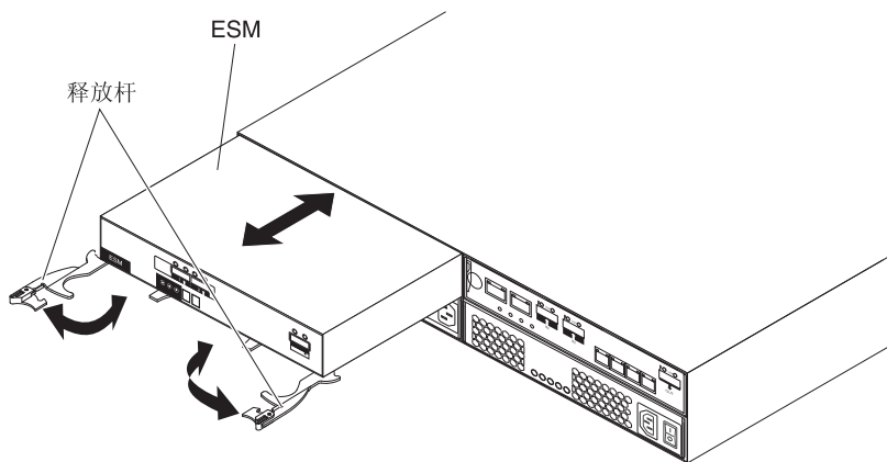
图 5-36. 卸下环境维护模块
