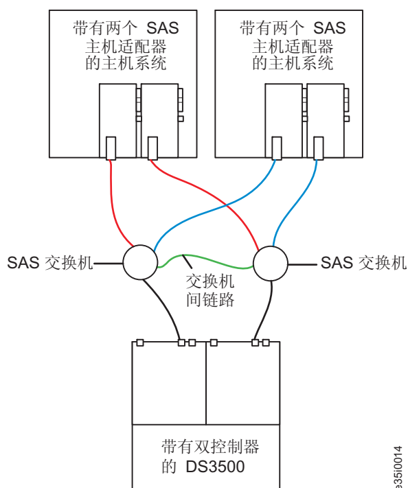
图 3-39. 使用两个通过互相链接的交换机彼此连接的 SAS 交换机从双控制器 DS3500 SAS 到多个主机的连接
