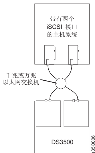
图 3-54. 单主机、多端口、双控制器的 iSCSI 配置
