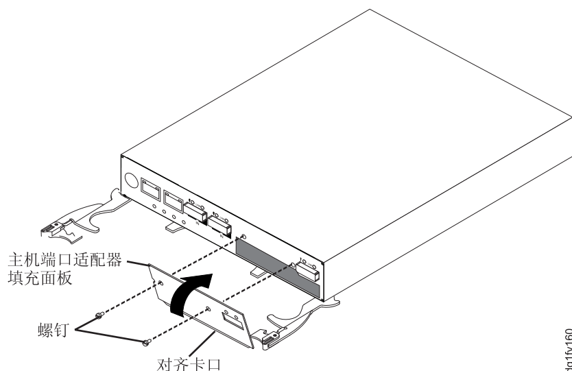
图 5-9. 卸下主机端口适配器填充面板
