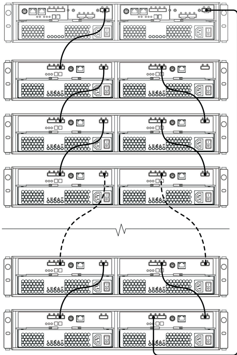
图 3-27. 一个双控制器 DS3500 和八个存储机柜
