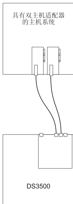
图 3-42. 与双 HBA 的单控制器直接连接的光纤通道连接（冗余主机连接）
