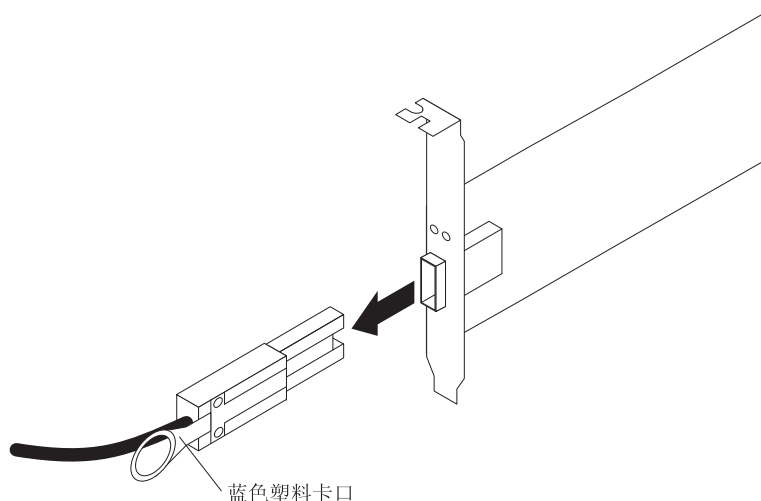
图 3-7. 拔下迷你 SAS 电缆
