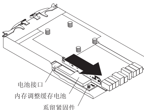
图 5-27. 从控制器上卸下电池单元
