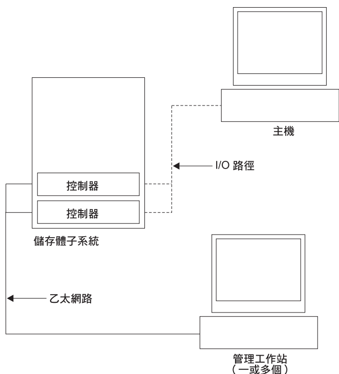
圖 3-30. 直接（頻外）管理的儲存體子系統
