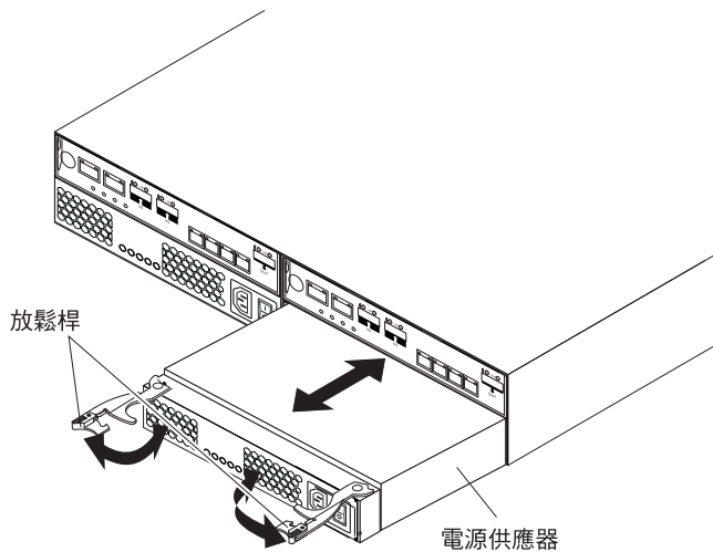
圖 5-19. 更換電源供應器
