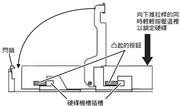
圖 5-15. 將硬碟插入接頭
