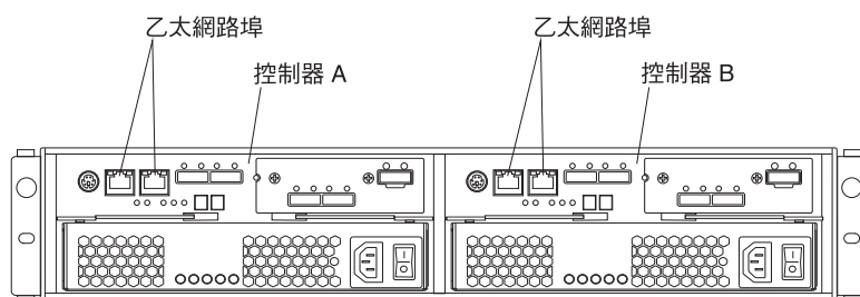
圖 3-28. 雙控制器 DS3500 上的乙太網路埠位置
