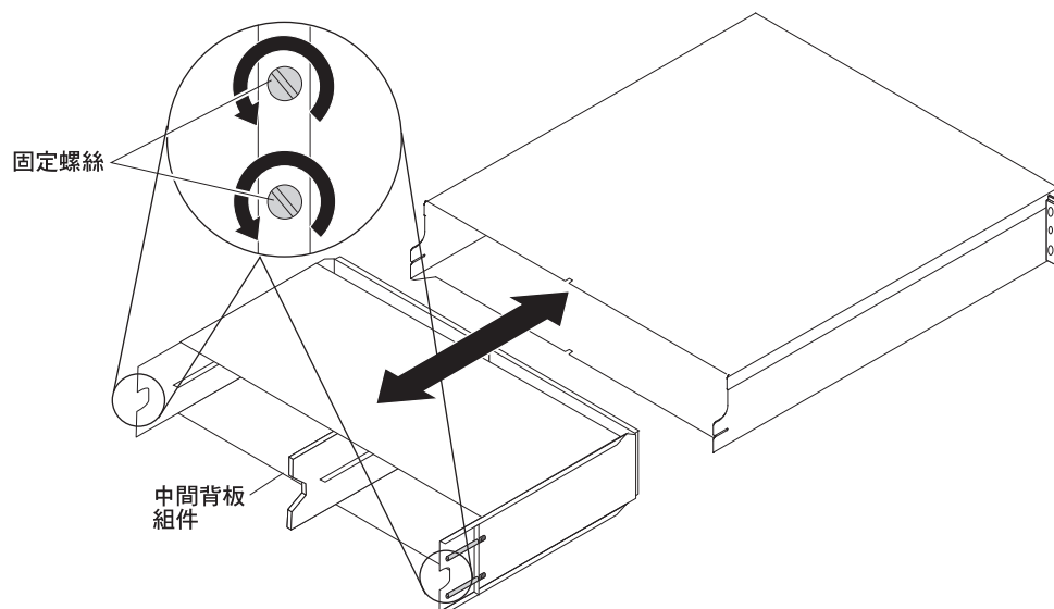
圖 5-28. 更換 DS3512 或 EXP3512 中的中間背板組件
