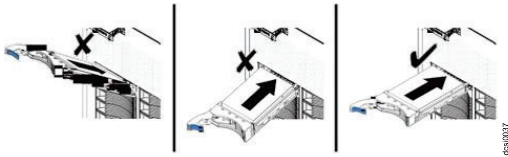
圖 5-14. 將硬碟插入硬碟插槽
