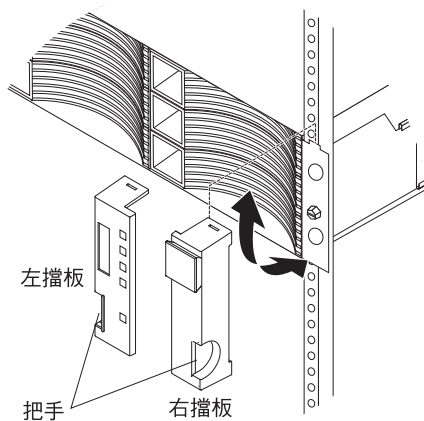
圖 5-26. 卸下隔板
