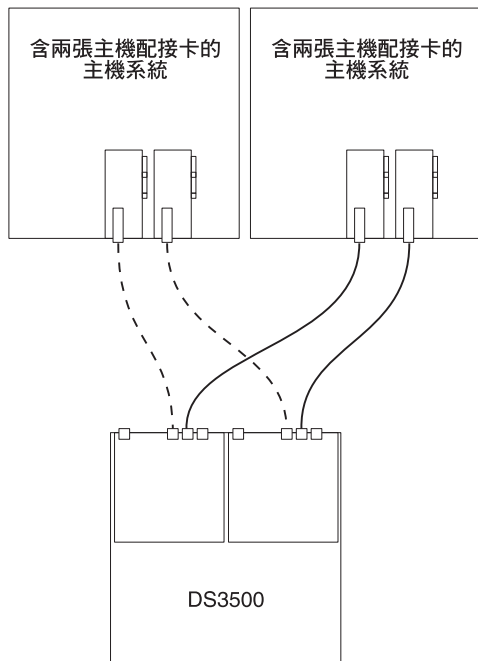
圖 3-45. 多個主機中多個 HBA 的雙控制器直接連接型「光纖通道」連線
