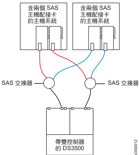
圖 3-37. 使用兩個獨立的 SAS 交換器連接至多部主機的双控制器 DS3500 SAS 連線
