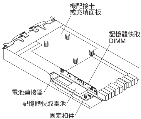
圖 5-22. 記憶體快取 DIMM 位置
