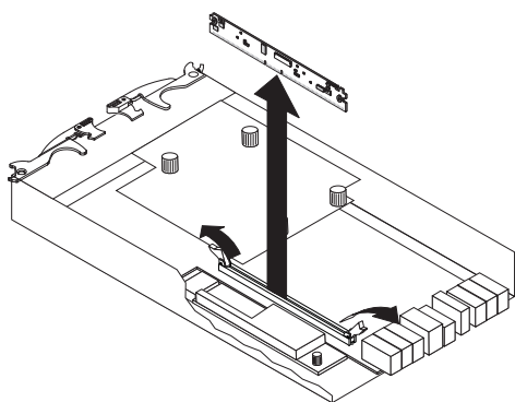
圖 5-25. 在控制器中安裝 DIMM
