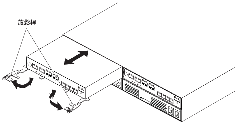
圖 5-20. 卸下控制器
