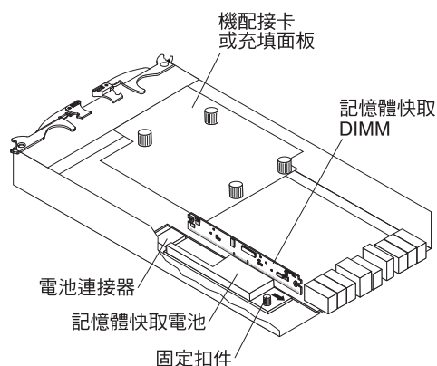
圖 1-12. 電池裝置
