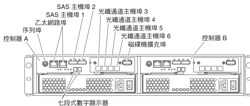
圖 3-40. 儲存體控制器上的主機接頭位置
