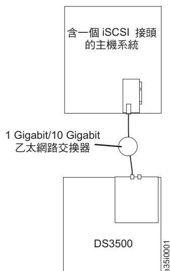
圖 3-49. 單一主機、單控制器 iSCSI 配置
