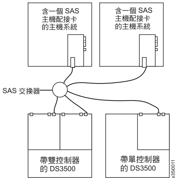
圖 3-36. 使用一個 SAS 交換器連接至多部主機的双控制器 DS3500 或單控制器 DS3500 SAS 連線
