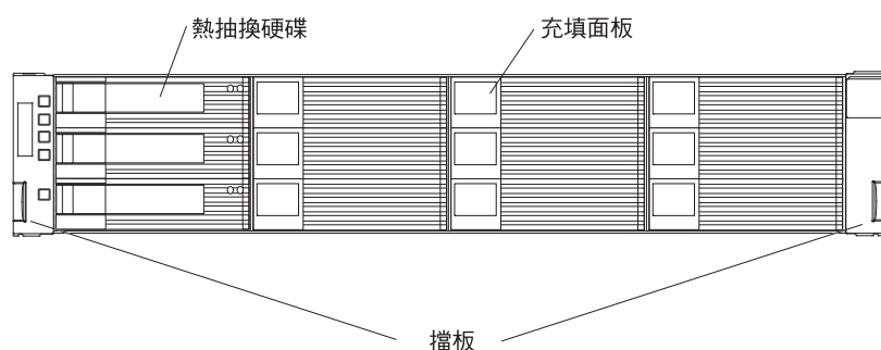
圖 1-2. DS3512 儲存體子系統和 EXP3512 儲存體機體熱抽換硬碟機槽和隔板
