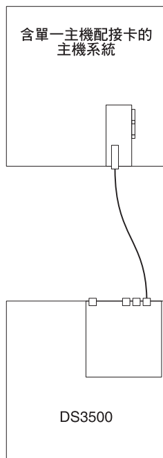
圖 3-31. 單一主機 HBA 的單控制器直接連接型 SAS 連線
