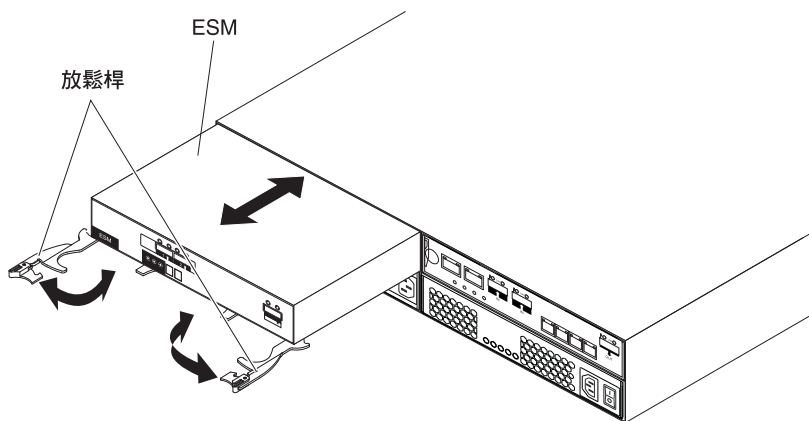
圖 5-27. 卸下環境服務模組
