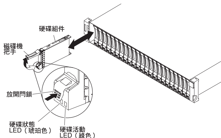
圖 5-13. 從 DS3524 或 EXP3524 卸下硬碟
