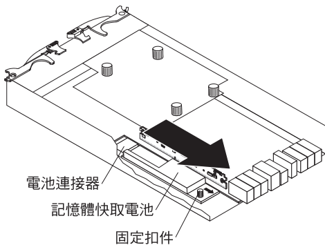
圖 5-21. 卸下控制器中的電池裝置
