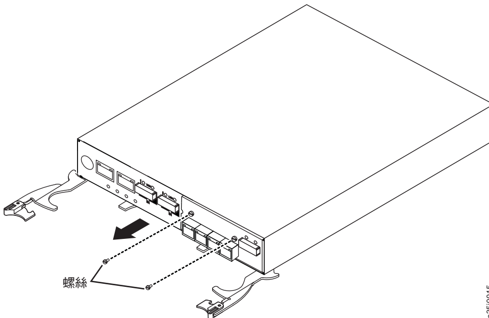
圖 5-9. 安裝主機埠配接卡
