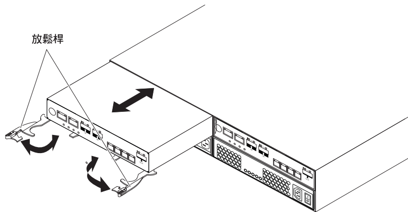
圖 5-23. 卸下控制器
