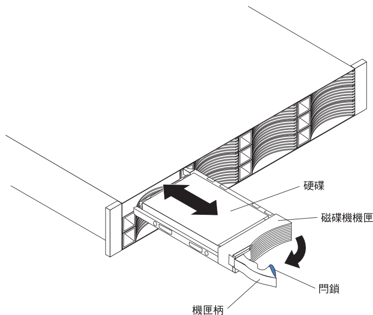
圖 5-12. 從 DS3512 或 EXP3512 卸下硬碟
