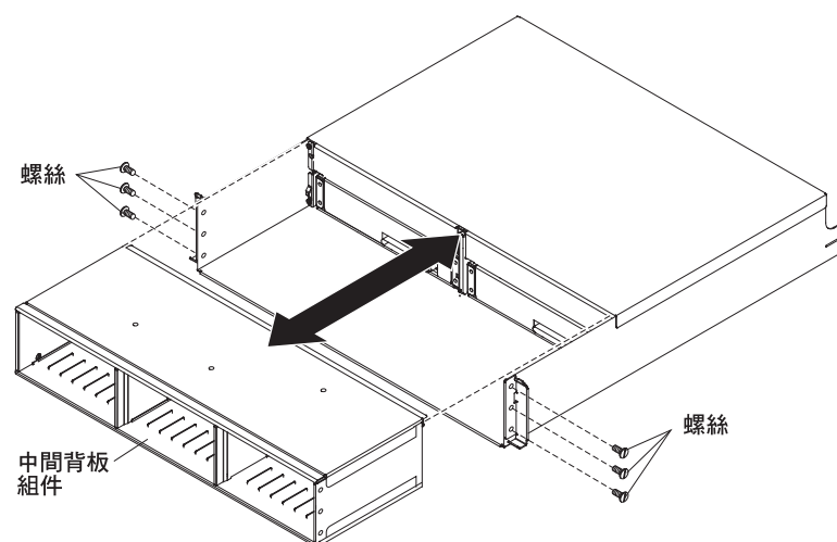
圖 5-29. 更換 DS3524 或 EXP3524 中的中間背板組件
