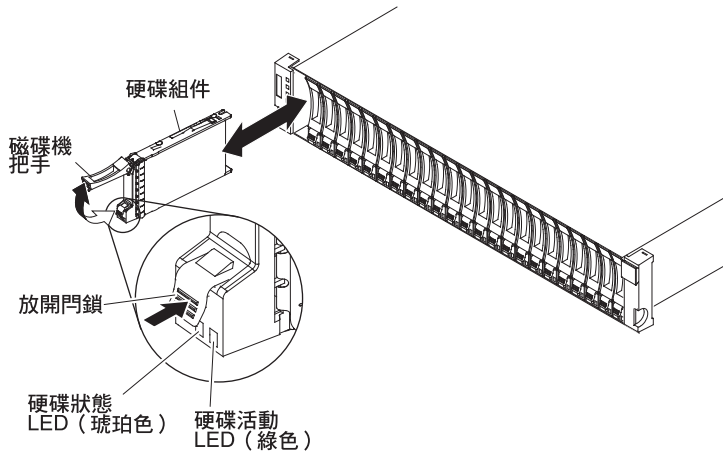
圖 5-17. 在 DS3524 或 EXP3524 中安裝硬碟
