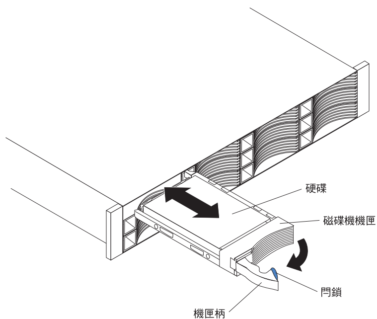
圖 5-16. 在 DS3512 或 EXP3512 中安裝硬碟
