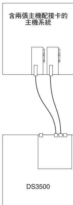
圖 3-32. 單一主機中雙重 HBA 的單控制器直接連接型 SAS 連線（備用主機連線）
