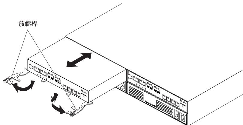
圖 5-7. 卸下控制器
