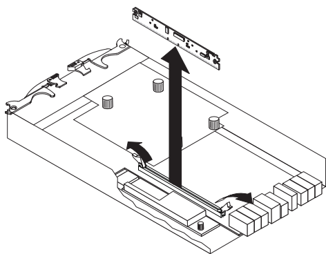
圖 5-24. 從控制器卸下 DIMM
