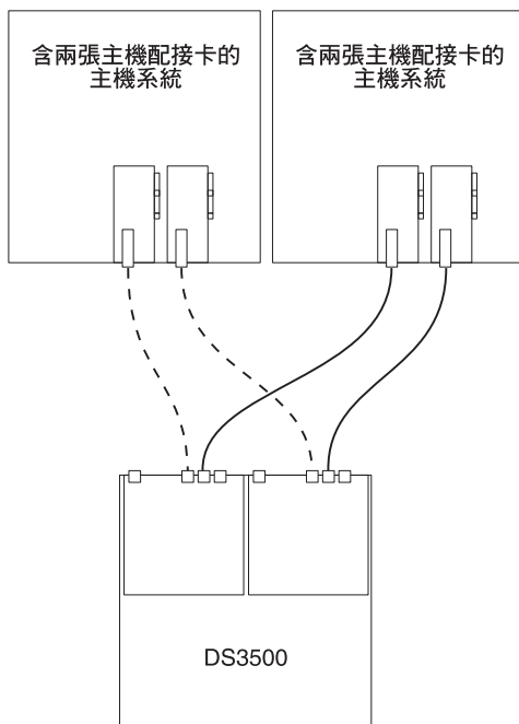
圖 3-35. 多個主機中多個 HBA 的雙控制器直接連接的 SAS 連線
