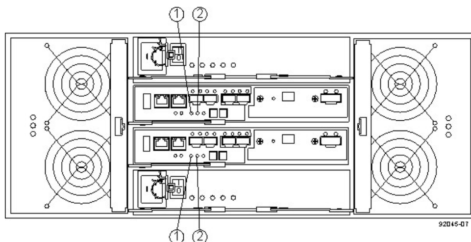
圖 110. 控制器維修動作 LED
