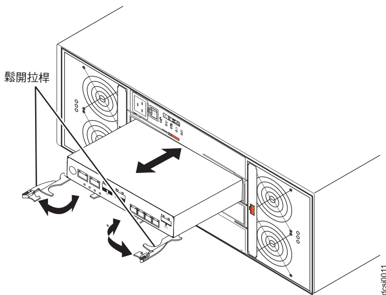
圖 96. 卸下及更換控制器
