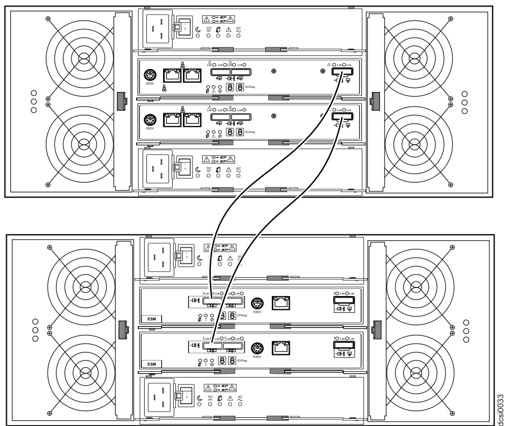
圖 36. 單一擴充機體
