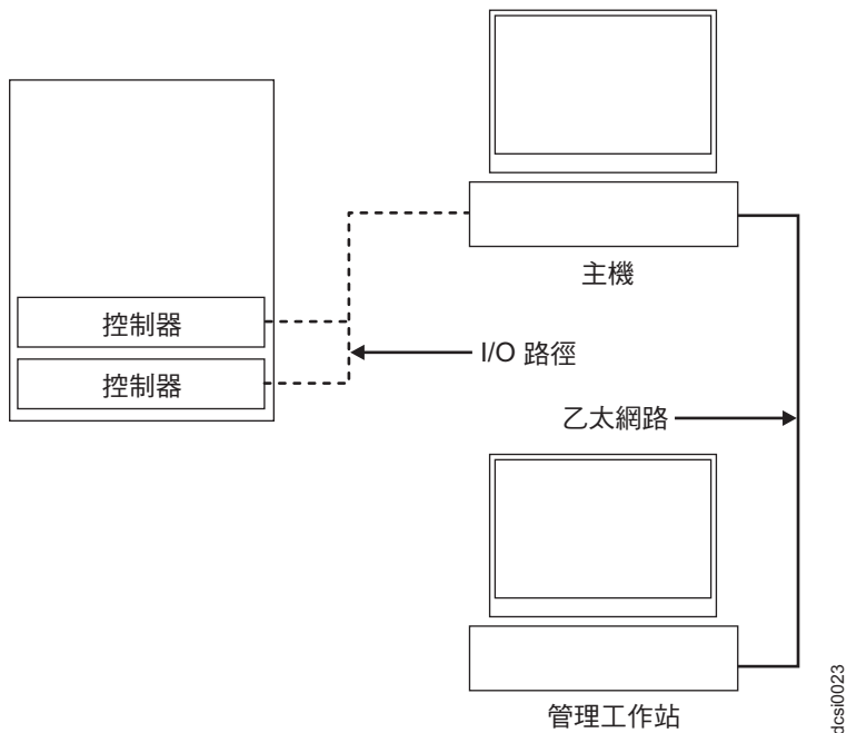
圖 38. 主機代理程式（頻內）管理
