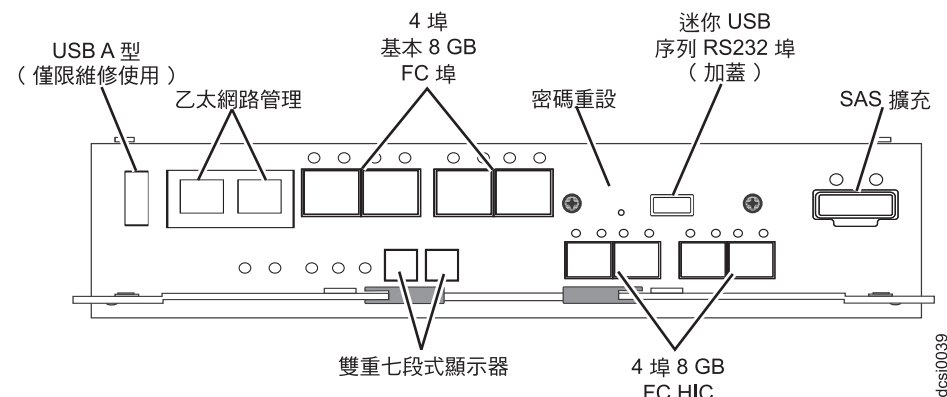
圖 21. 含有效能模組控制器的 DCS3700 儲存體系統（列出 FC 埠）
