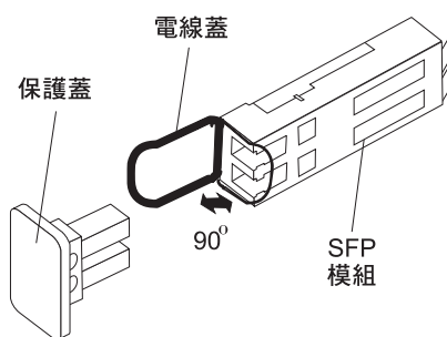
圖 25. SFP 模組及保護蓋
