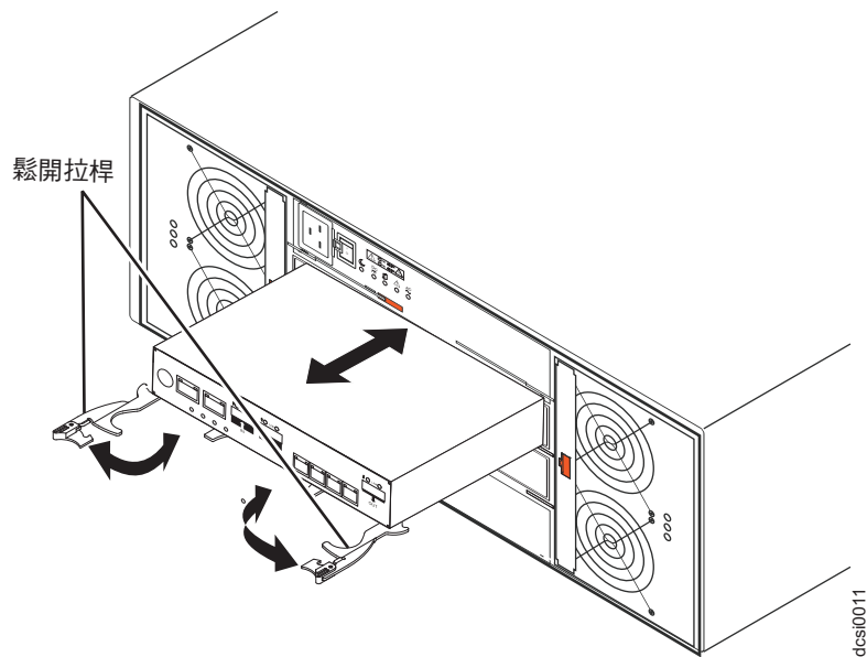
圖 63. 卸下及更換控制器
