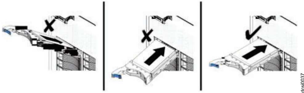
圖 69. 將硬碟插入磁碟機槽中
