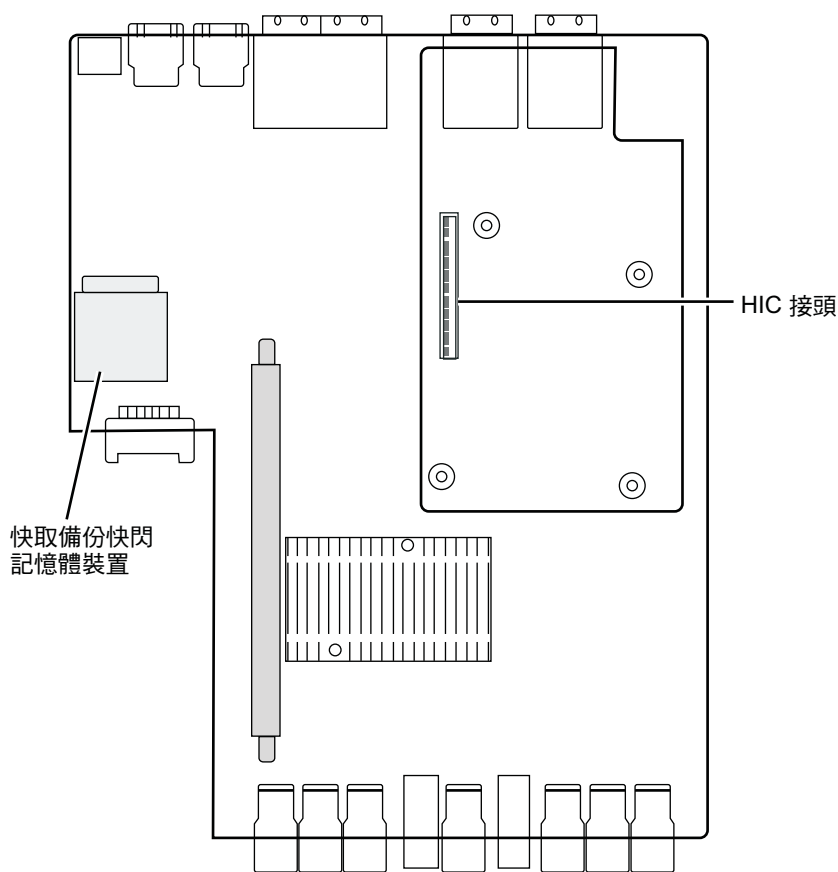
圖 67. 對齊 HIC 接頭
