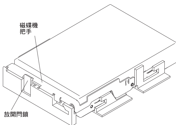
圖 73. 將磁碟機鎖在定位
