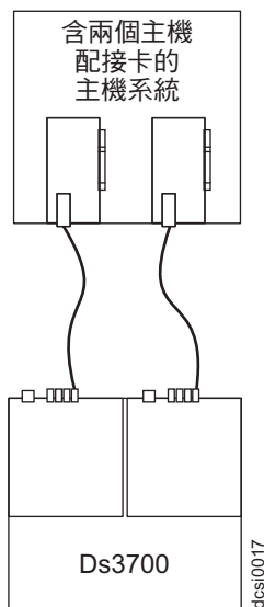
圖 40. 相同主機中兩個 HBA 的雙控制器直接連接型光纖通道連線（備用主機連線）
