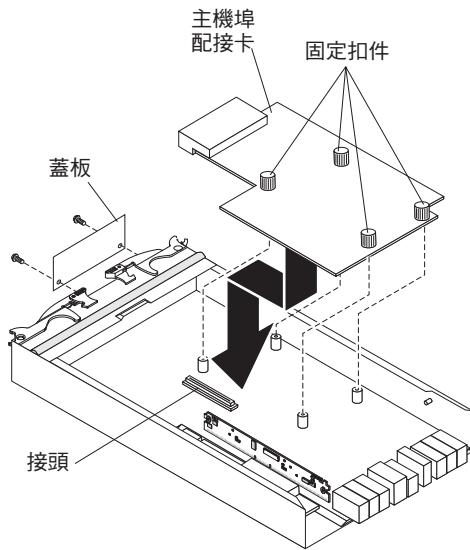
圖 66. 安裝主機埠配接卡
