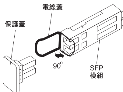
圖 27. 鬆開 SFP 模組門鎖 - 塑膠種類
