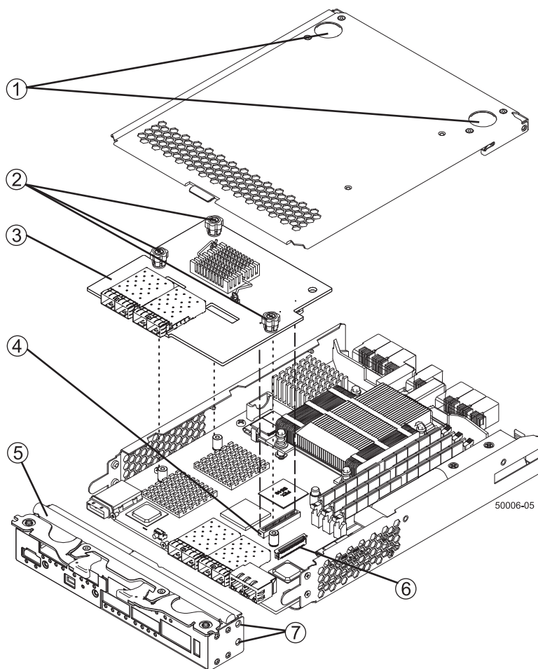
圖 115. 更換主機介面卡
