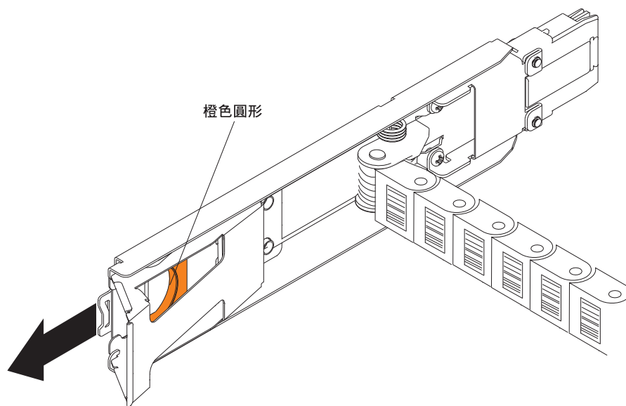
圖 92. 連接至中間背板的垂直裝載托架
