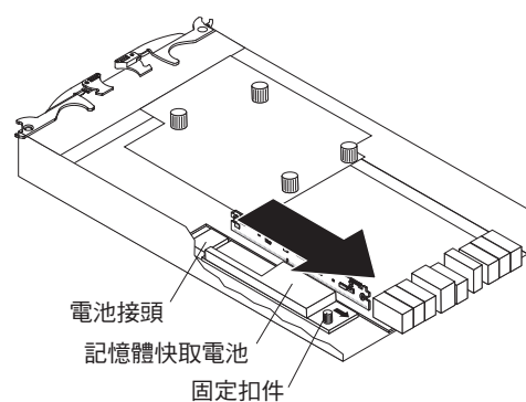
圖 76. 從控制器卸下電池裝置
