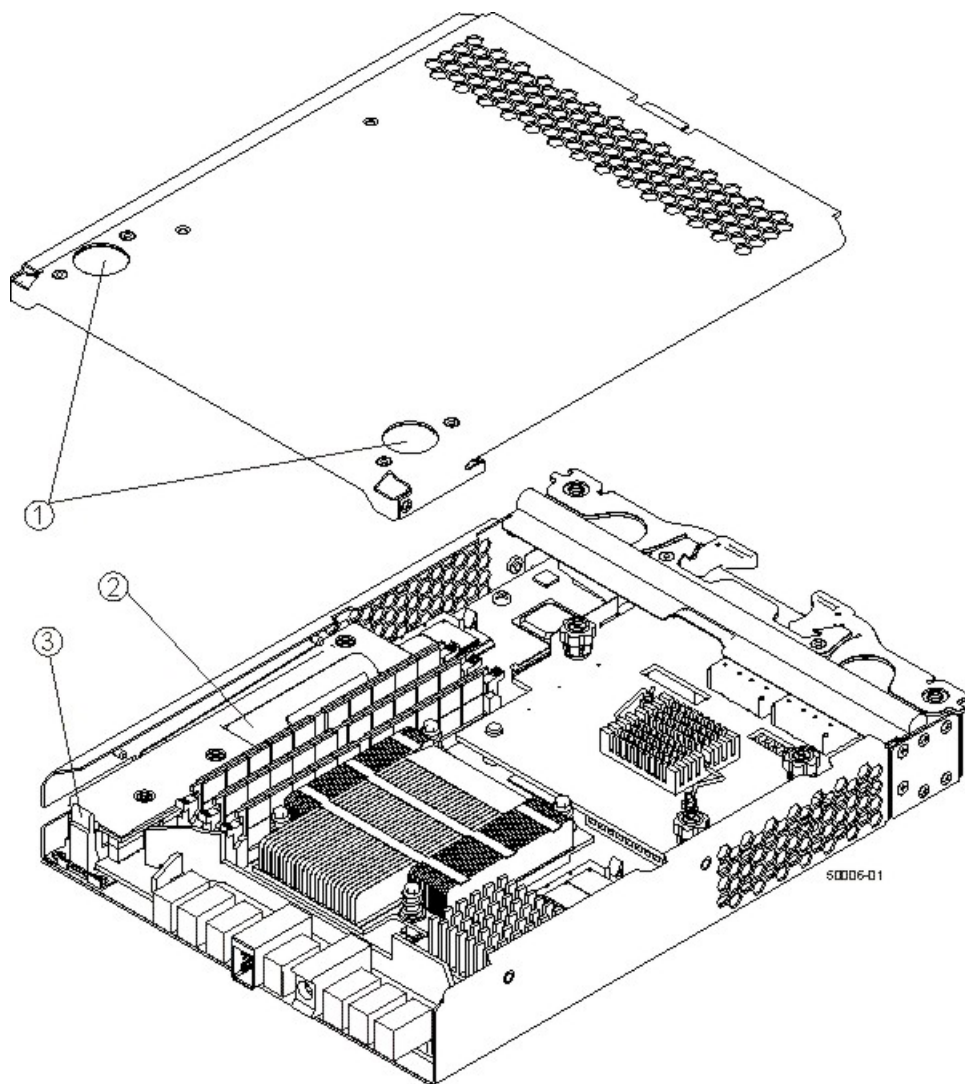
圖 108. 控制器上蓋板門鎖按鈕
