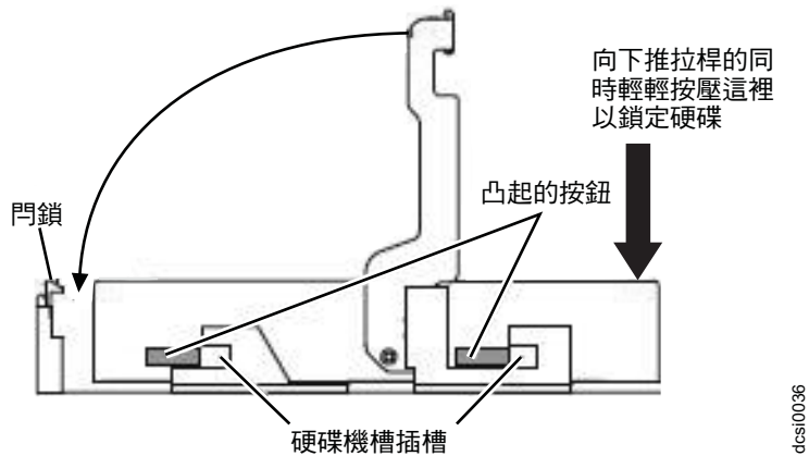
圖 70. 將硬碟插入接頭中
