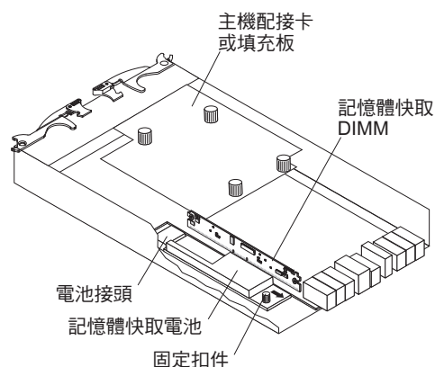
圖 77. 記憶體快取 DIMM 位置
