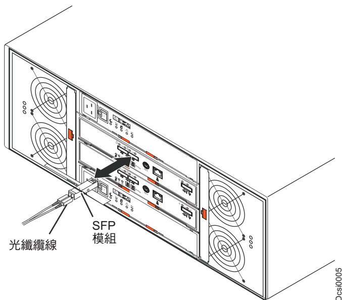
圖 13. SFP 模組與光纖纜線
