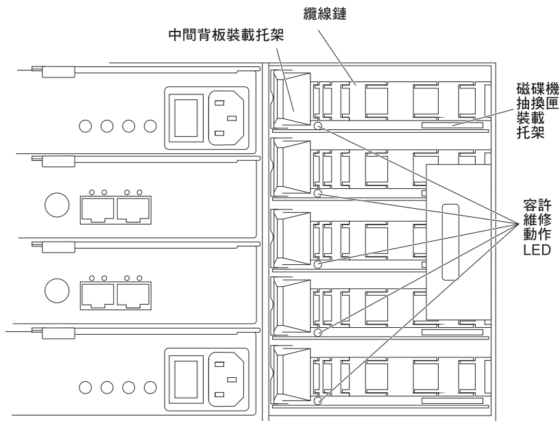
圖 85. 已卸下右側風扇組件的儲存體擴充機體背面視圖
