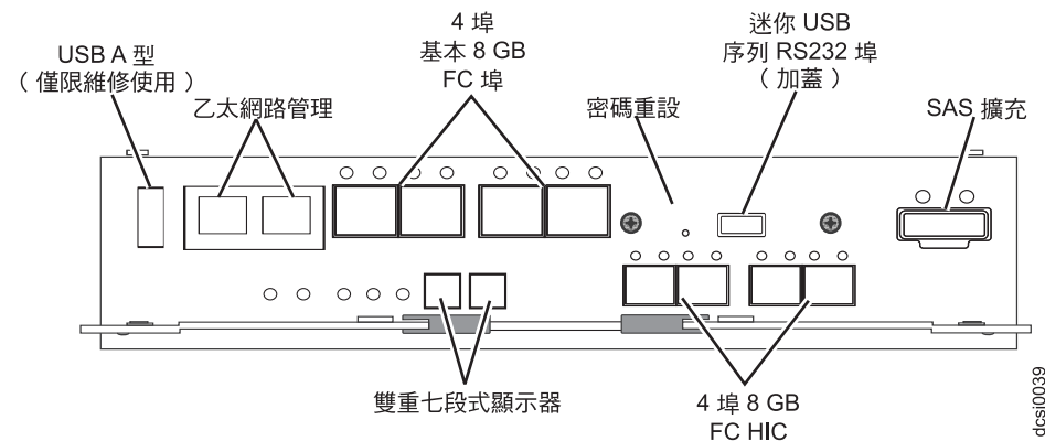
圖 6. 含有效能模組控制器的 DCS3700 儲存體系系統上的接頭
