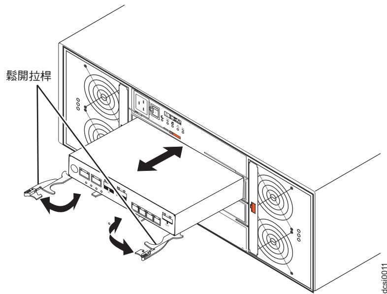
圖 83. 卸下環境服務模組
