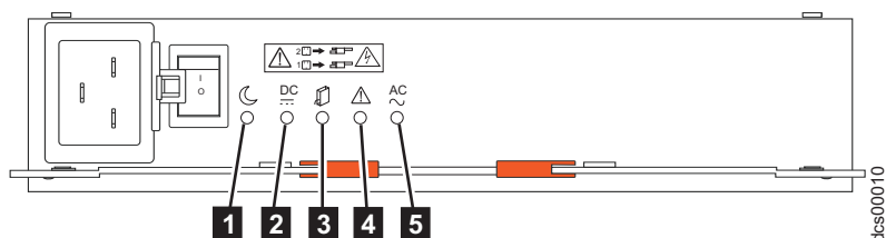
圖 57. AC 電源供應器 LED
