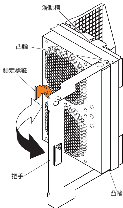
圖 90. 卸下風扇組件
