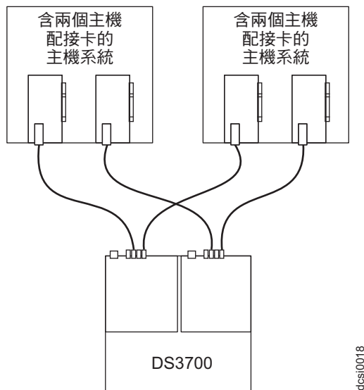
圖 41. 多部主機中多個 HBA 的雙控制器直接連接型光纖通道連線
