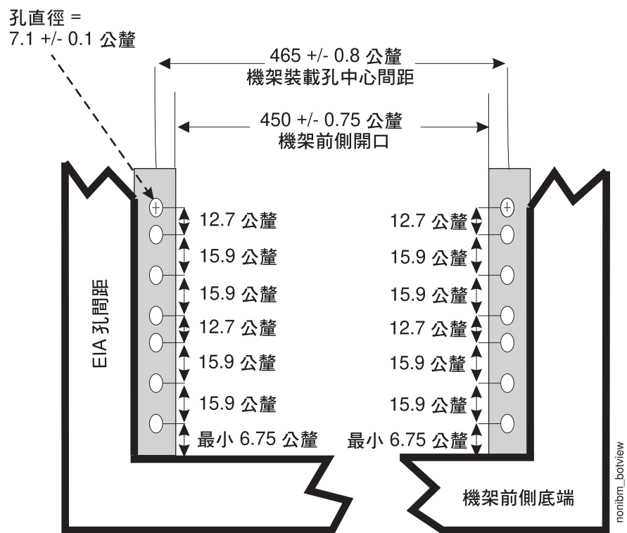
圖 124. 機架規格尺寸，底端前視圖
