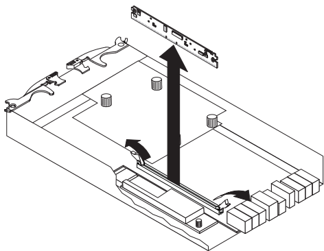
圖 79. 從控制器卸下 DIMM
