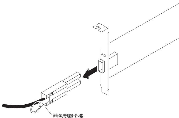
圖 24. 拔掉迷你 SAS 纜線
