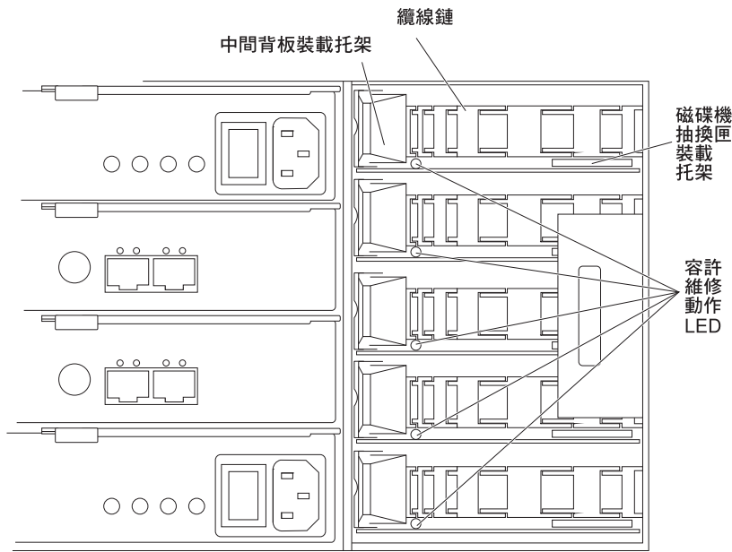
圖 91. 已卸下右側風扇組件的儲存體擴充機體背面視圖
