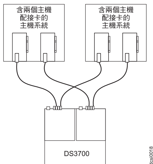
圖 44. 多部主機中多個 HBA 的雙控制器直接連接型光纖通道連線
