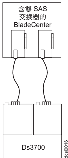
圖 42. 連接至單一 BladeCenter 裝置的 DCS3700 範例
