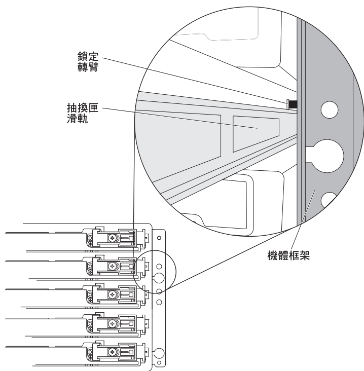
圖 95. 位於抽換匣導軌上面的鎖定桿鎖簧
