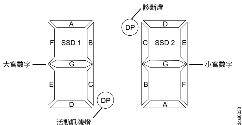
圖 60. 數字顯示器 LED
