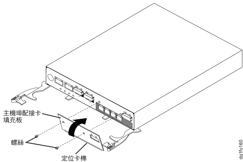
圖 65. 卸下主機埠配接卡填充板
