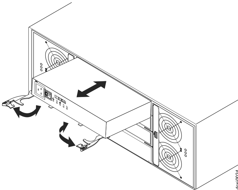
圖 74. 更換電源供應器
