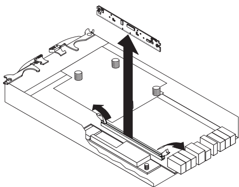
圖 80. 在控制器中安裝 DIMM
