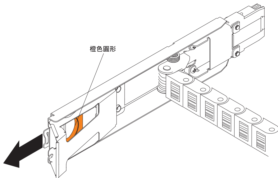
圖 86. 連接至中間背板的垂直裝載托架
