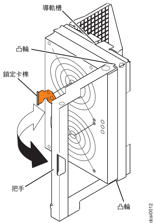
圖 84. 卸下風扇組件
