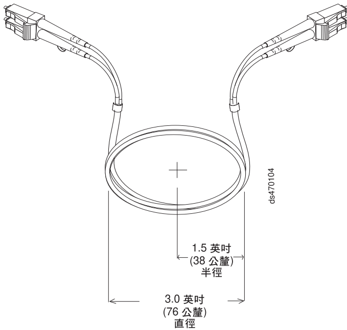
圖 29. 建議的光纖纜線彎曲及線圈規格
