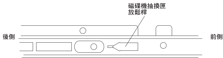
圖 88. 磁碟機抽換匣側面的磁碟機抽換匣鬆開拉桿
