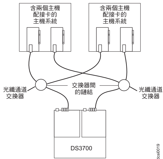
圖 45. 單一光纖通道 SAN 光纖配置的範例
