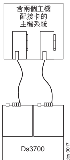
圖 43. 相同主機中兩個 HBA 的雙控制器直接連接型光纖通道連線（備用主機連線）
