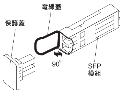
圖 28. 鬆開 SFP 模組門鎖 - 金屬種類
