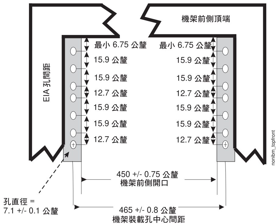
圖 123. 機架規格尺寸，頂端前視圖
