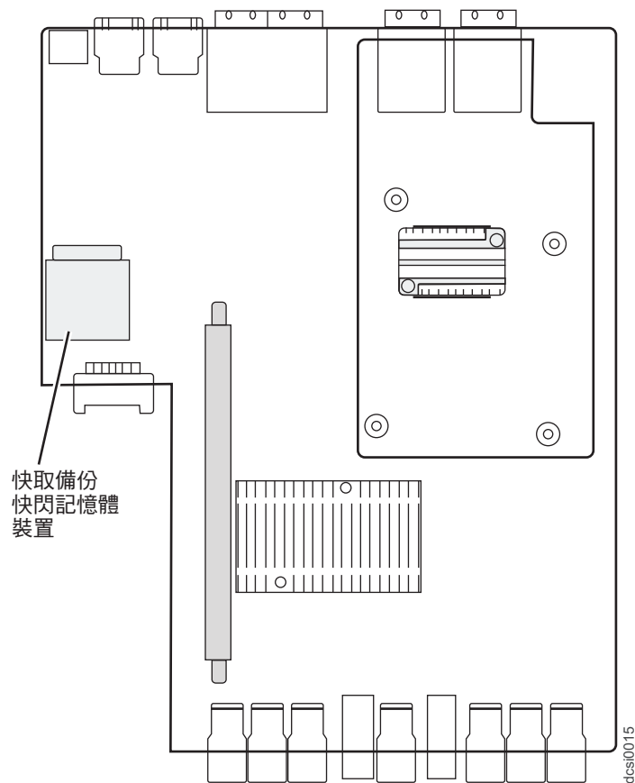
圖 81. 快取備份快閃記憶體裝置
