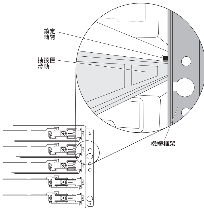
圖 89. 位於抽換匣導軌上面的鎖定桿鎖簧
