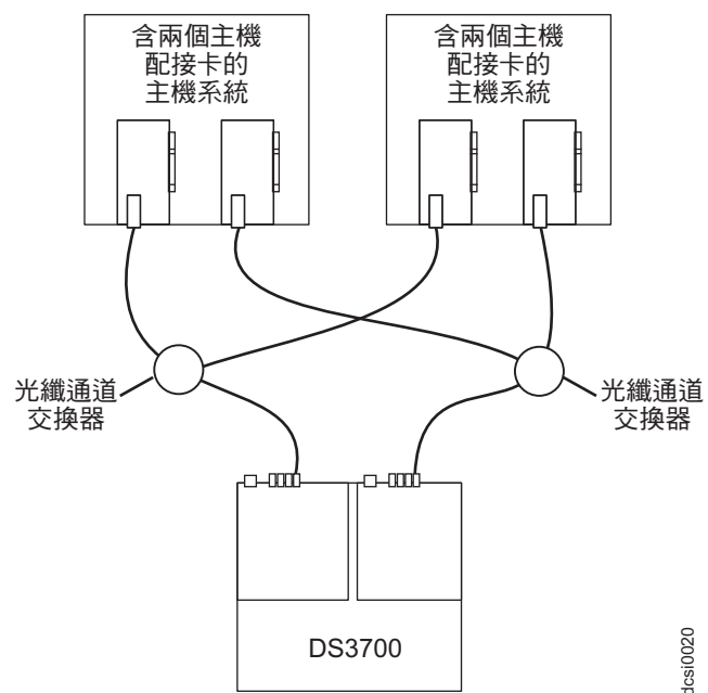
圖 46. 雙光纖通道 SAN 光纖配置的範例
