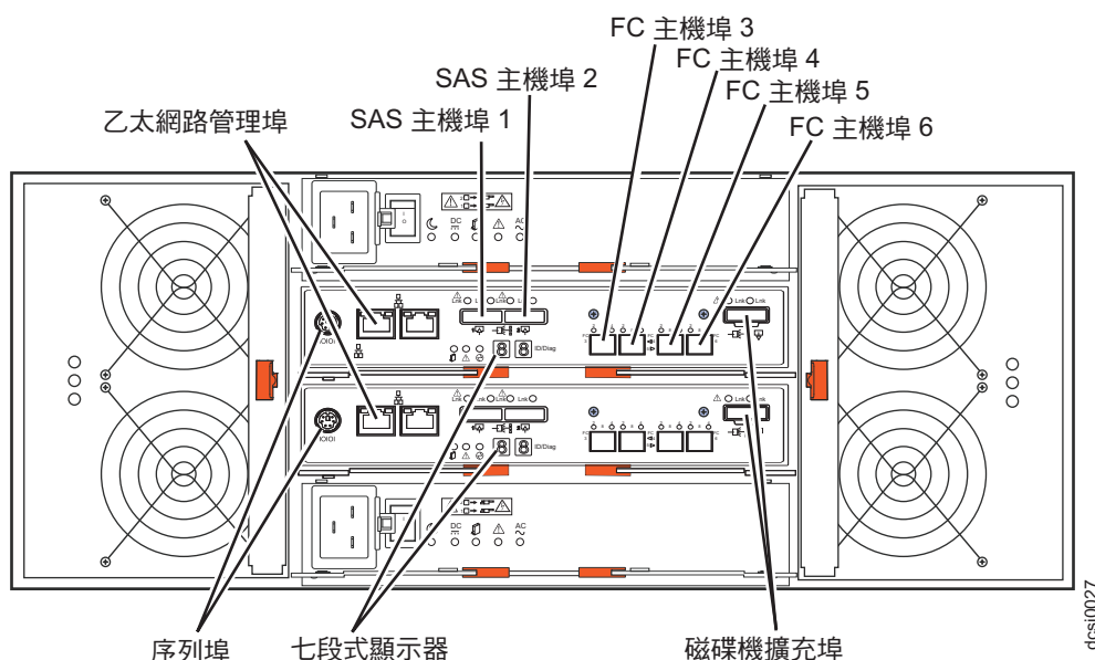
圖 20. 雙控制器 DCS3700 儲存體系統埠及控制器（含選用光纖通道主機埠配接卡）
