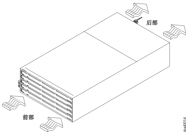
图 12. 穿过存储扩展机柜的气流
