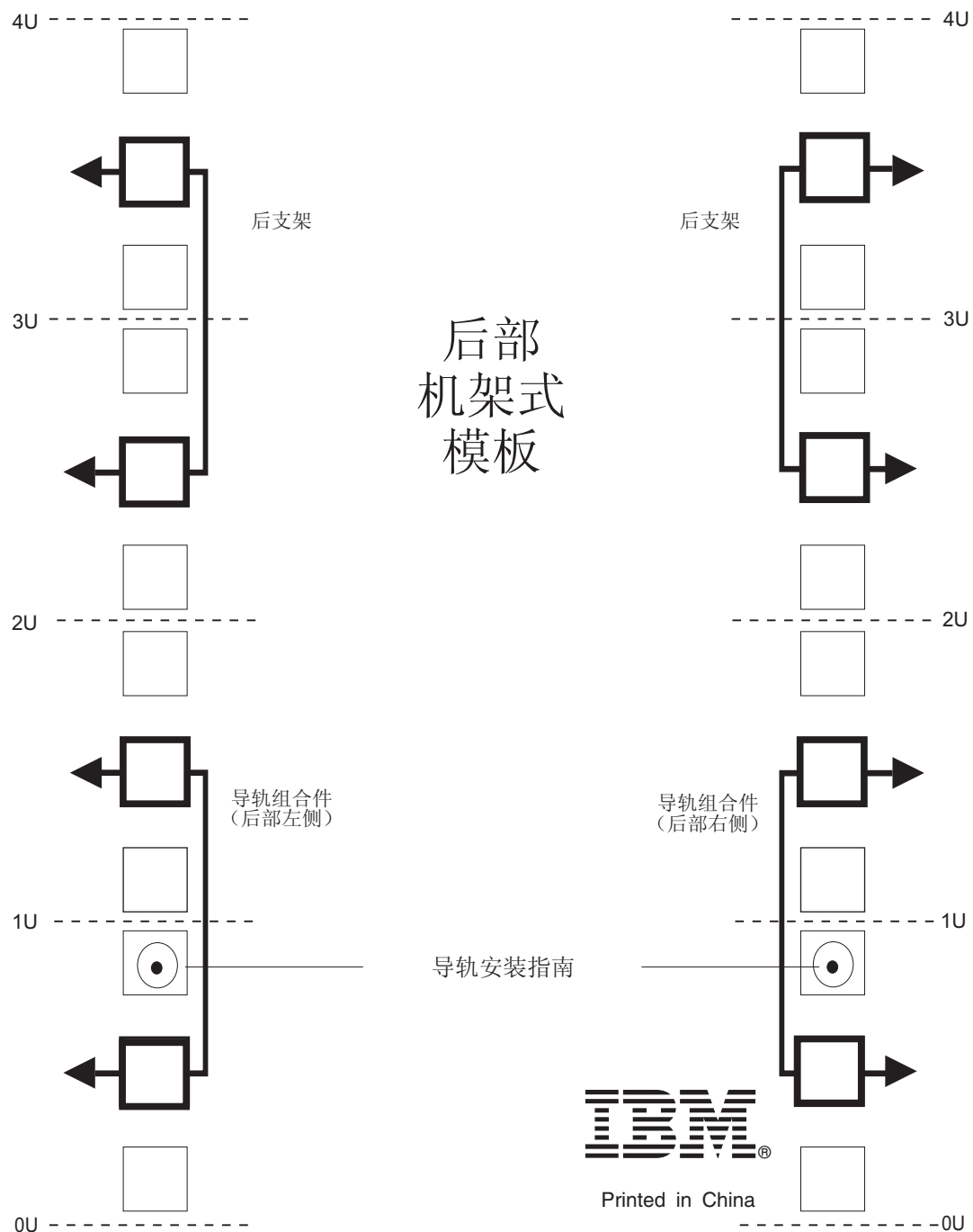
图 121. 后部机架安装模板
