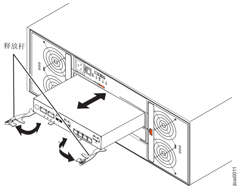
图 75. 卸下控制器
