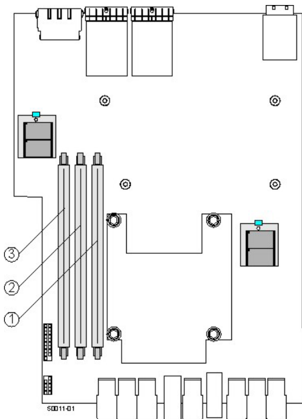
图 101. 三个高速缓存内存 DIMM 插槽
