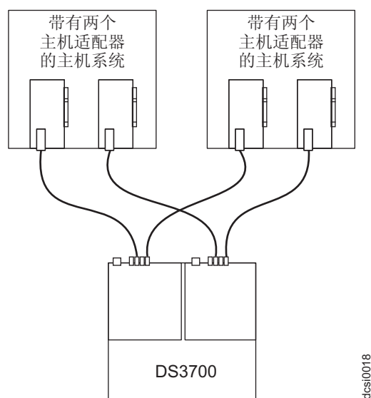
图 44. 与多主机中多个 HBA 的双控制器直接连接的光纤通道连接
