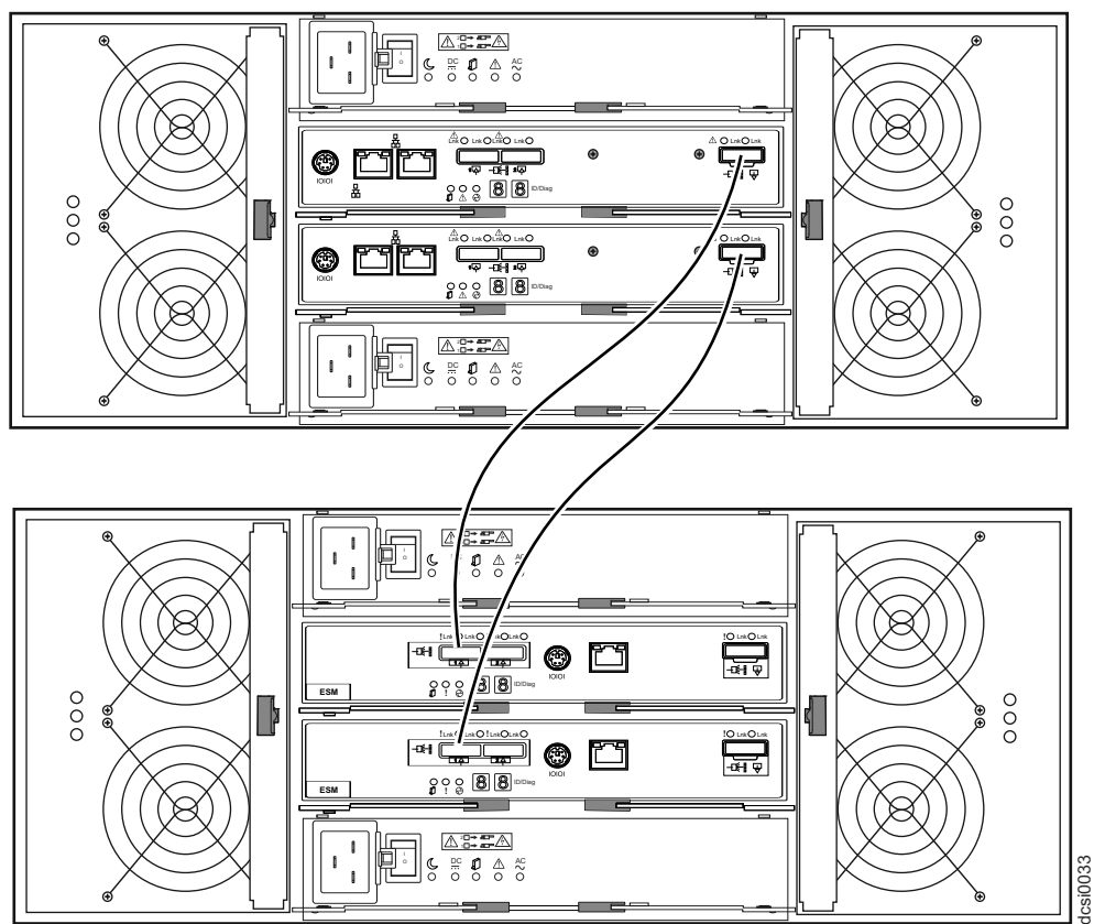
图 36. 单扩展机柜
