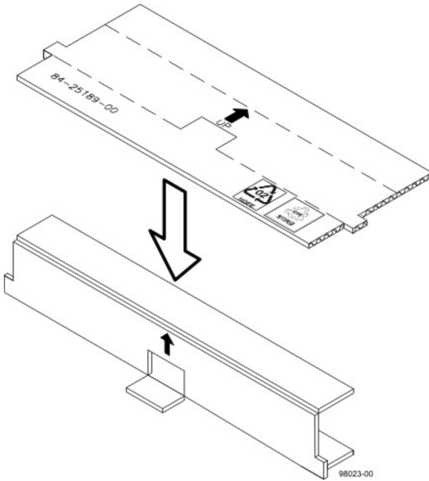
图 113. 控制器空气分流器
