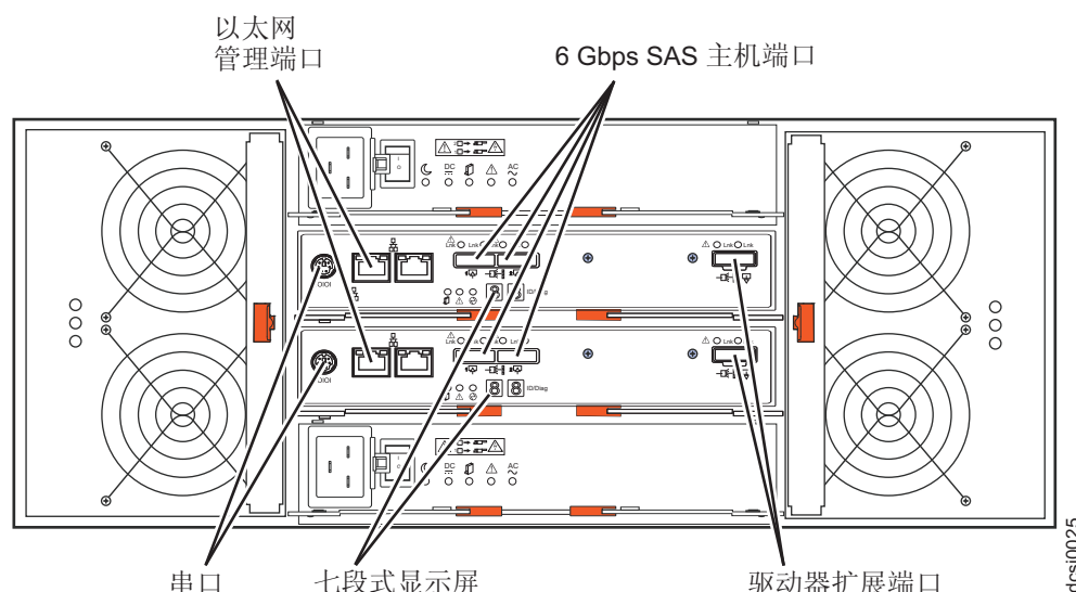
图 5. DCS3700 接口
