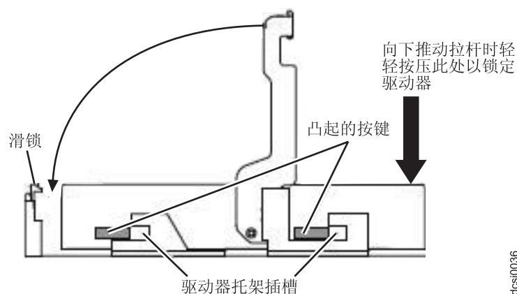
图 70. 将硬盘驱动器插入接口
