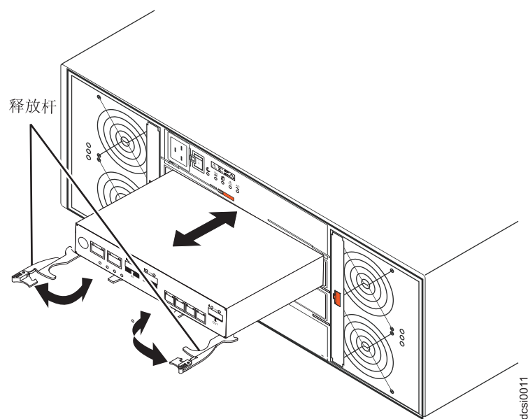
图 78. 卸下控制器
