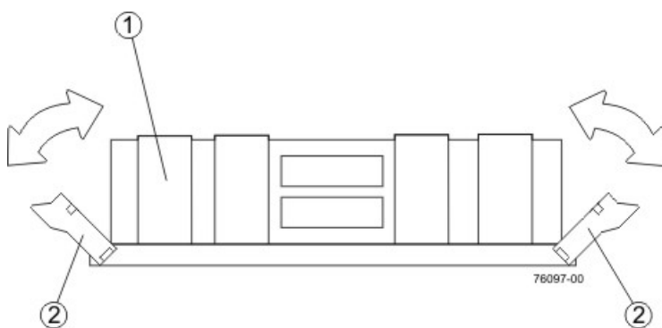
图 102. 卸下高速缓存内存 DIMM
