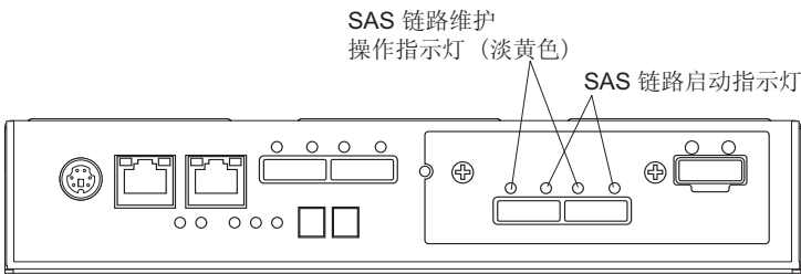
图 54. SAS 主机端口适配器指示灯
