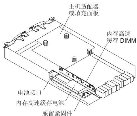
图 77. 内存高速缓存 DIMM 的位置
