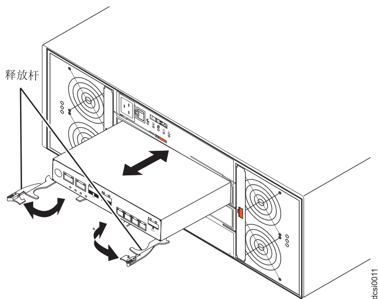
图 61. 卸下控制器
