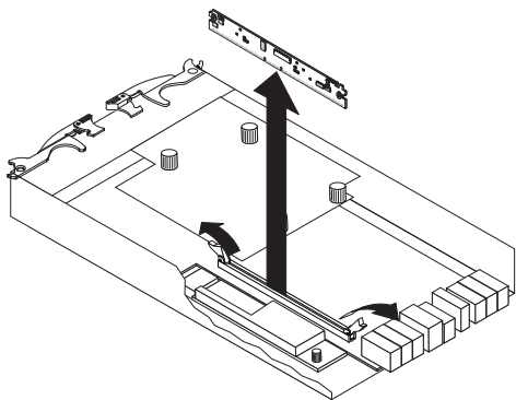
图 79. 从控制器上卸下 DIMM
