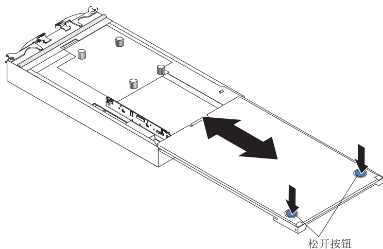
图 62. 卸下外盖
