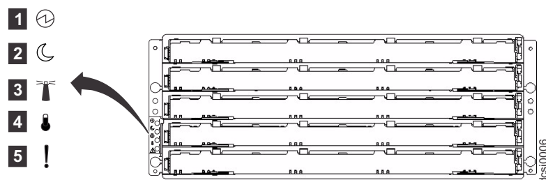
图 50. DCS3700 前部指示灯和控件
