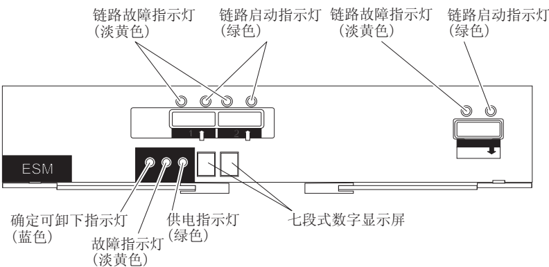
图 55. ESM 指示灯
