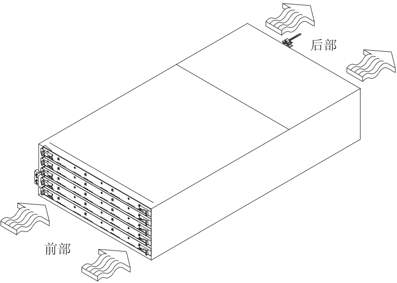
图 14. DCS3700 气流
