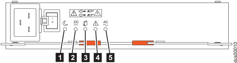
图 57. 交流电源指示灯
