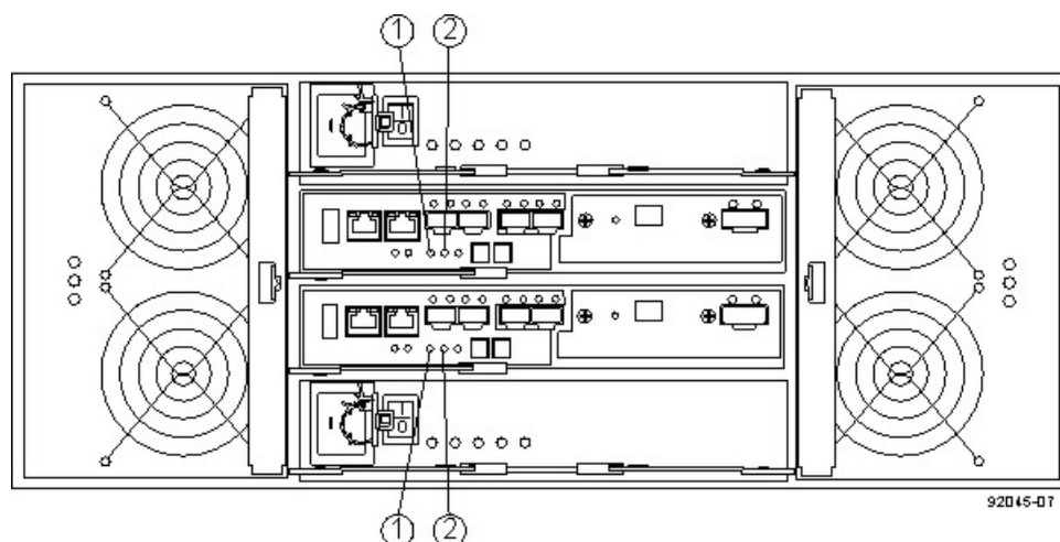
图 110. “控制器维护操作”指示灯
