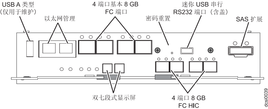
图 21. 带有性能模块控制器的 DCS3700 存储子系统（已列出 FC 端口）
