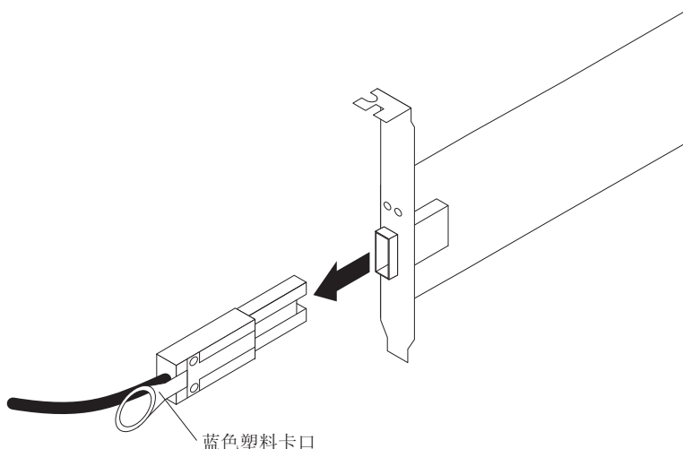
图 24. 拔出迷你 SAS 电缆
