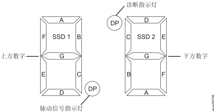
图 60. 数字显示屏指示灯
