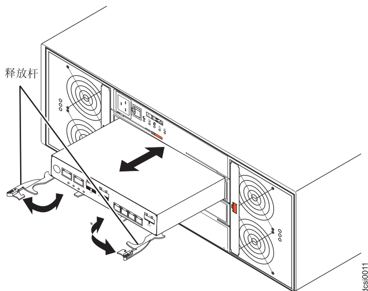
图 83. 卸下环境维护模块
