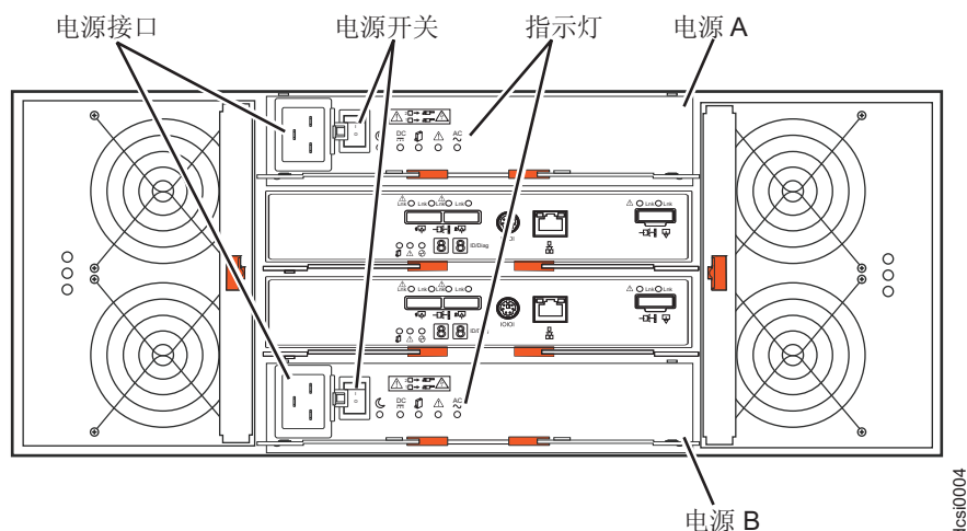
图 49. DS3500 直流型号的电源开关和接口
