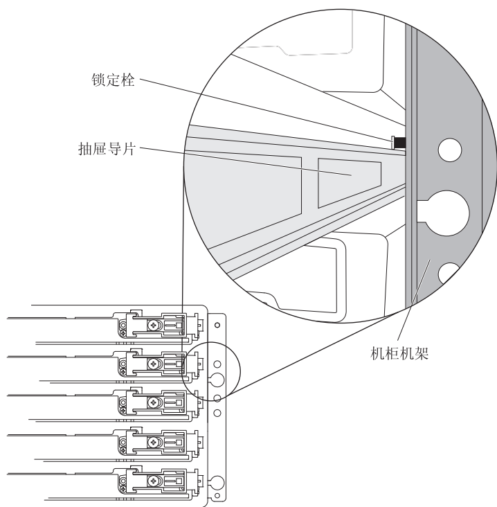
图 95. 位于抽屉导销上方的锁定滚轮
