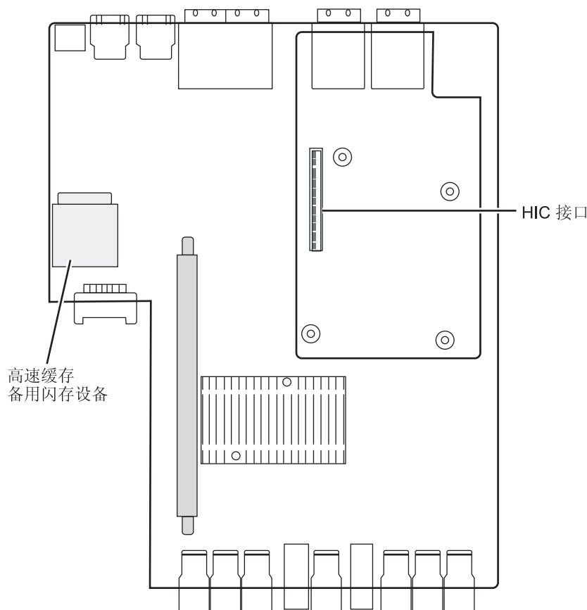
图 67. 对齐 HIC 接口
