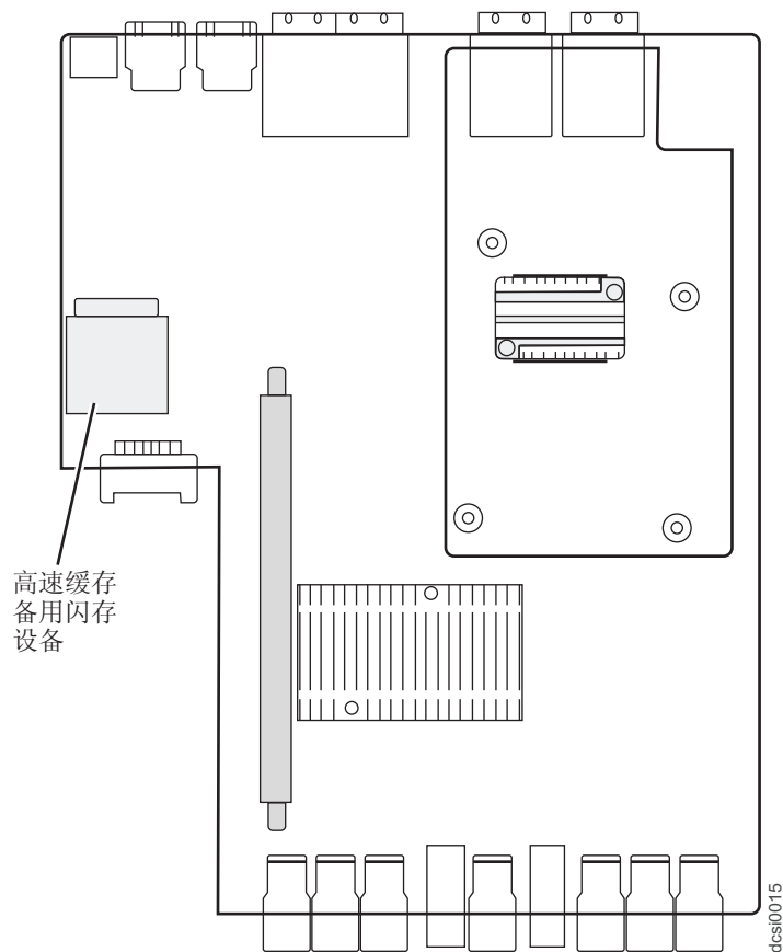
图 81. 高速缓存备用闪存设备
