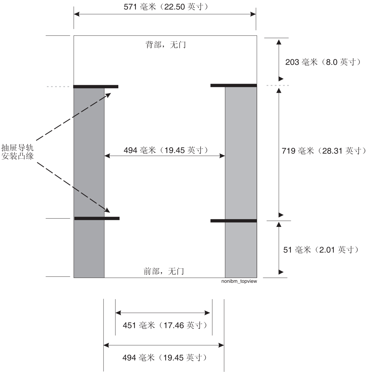
图 122. 非 IBM 机架规格尺寸的顶视图
