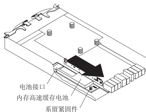
图 76. 从控制器上卸下电池单元
