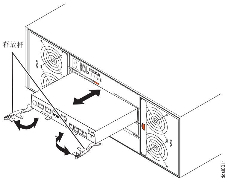
图 63. 卸下并重新安装控制器
