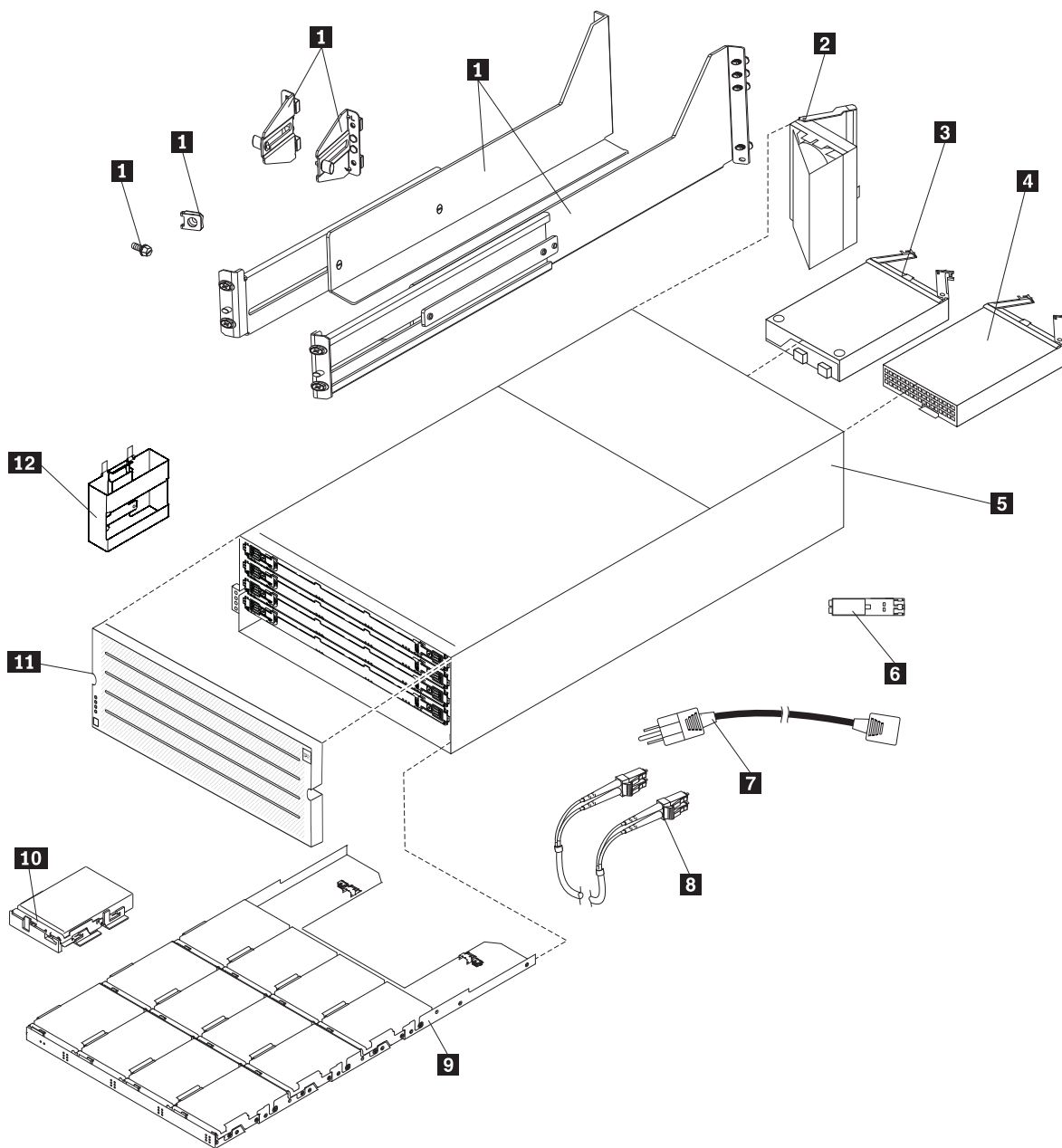
图 117. DCS3700 存储子系统机柜部件列表
