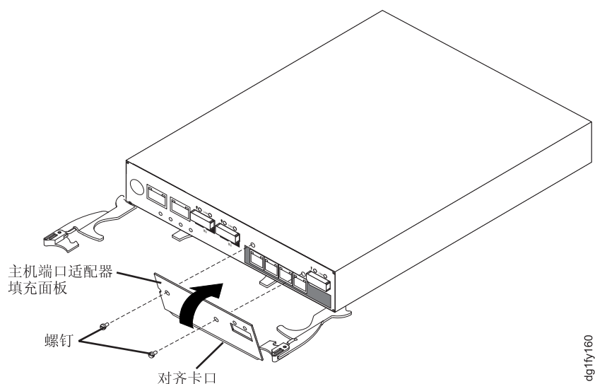
图 65. 卸下主机端口适配器填充面板
