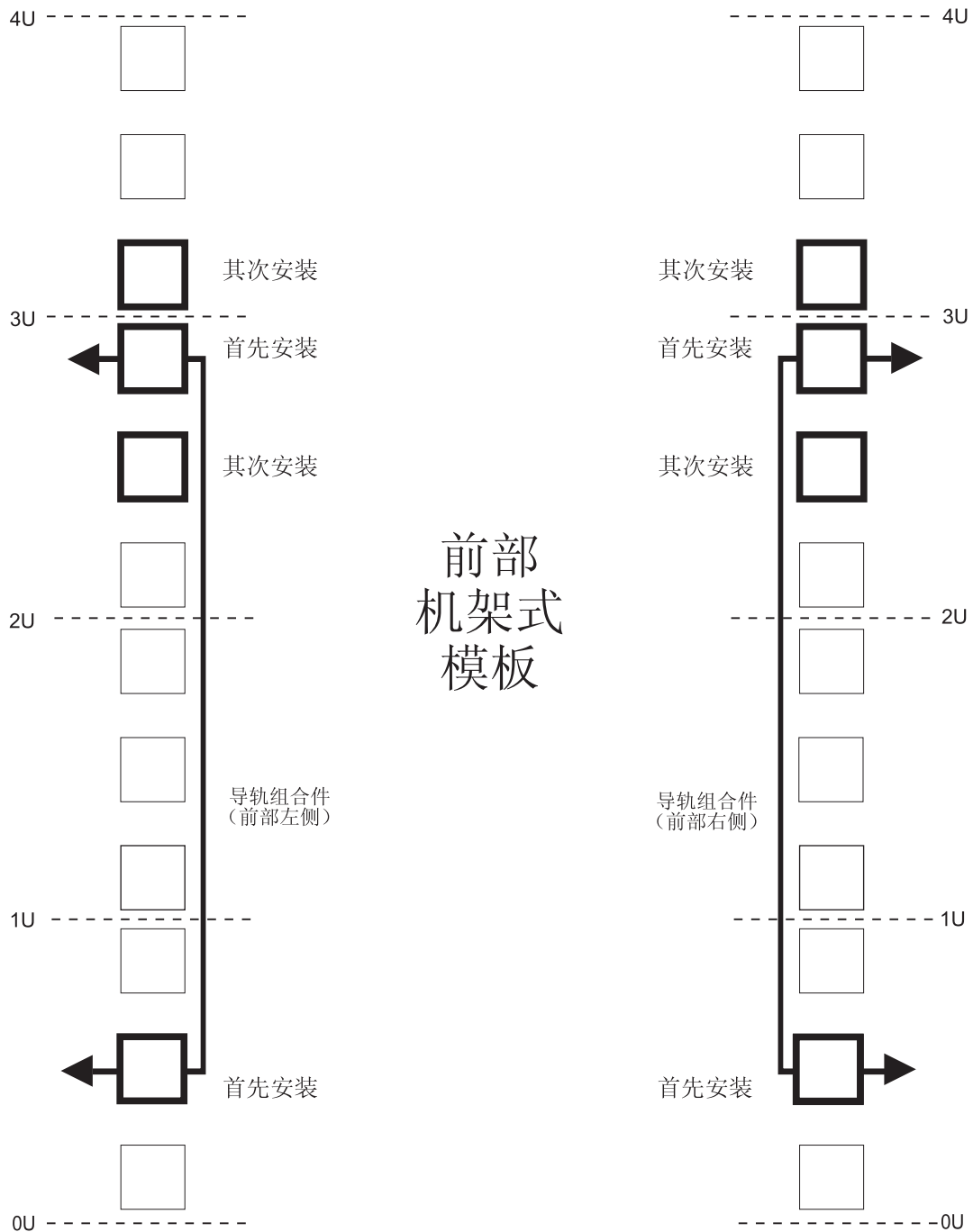
图 120. 前部机架安装模板
