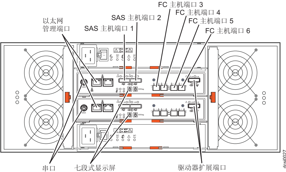
图 20. 双控制器 DCS3700 存储子系统端口和控制器（带有可选光纤通道主机端口适配器）
