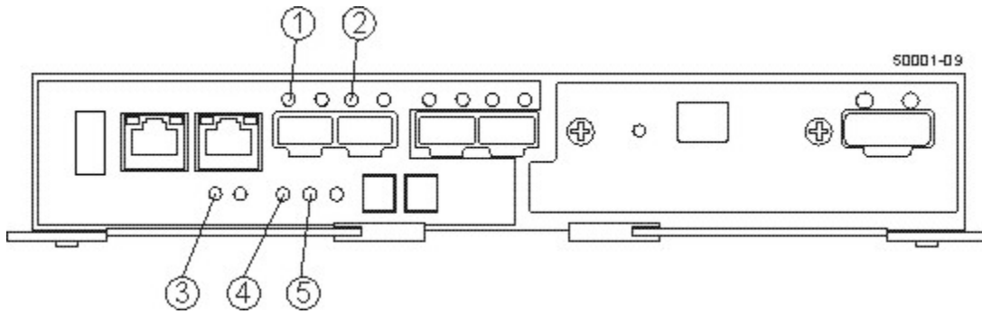
图 109. 控制器指示灯
