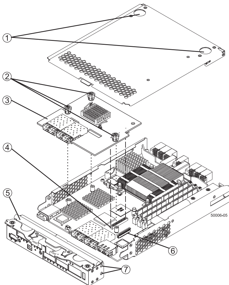
图 115. 主机接口卡更换
