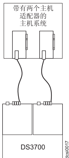
图 43. 与同一主机中两个 HBA 的双控制器直接连接的光纤通道连接（冗余主机连接）
