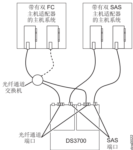
图 48. 多主机、多端口和多光纤网（光纤通道和 SAS）配置的示例
