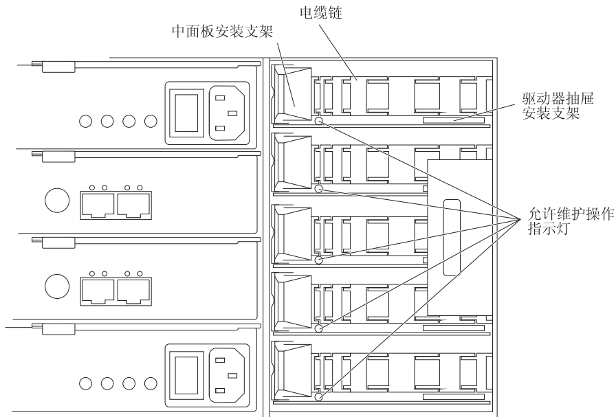
图 91. 已卸下右侧风扇组合件的存储扩展机柜的后视图
