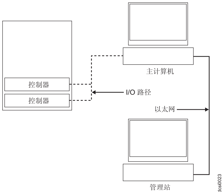
图 38. 主机代理程序（频带内）管理
