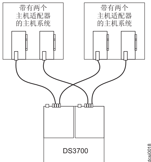
图 41. 与多主机中多个 HBA 的双控制器直接连接的光纤通道连接
