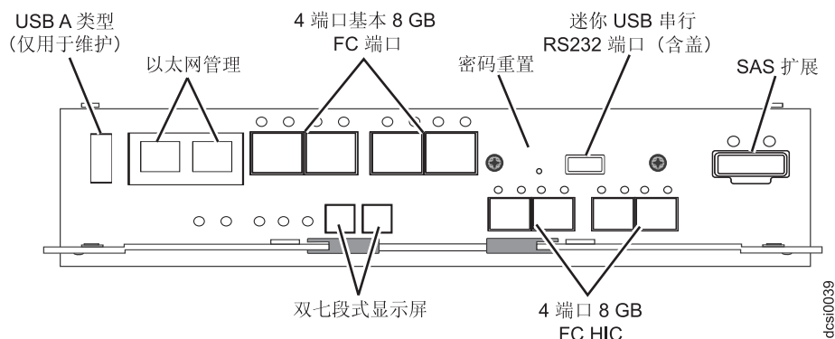
图 6. 带有性能模块控制器的 DCS3700 存储子系统上的接口
