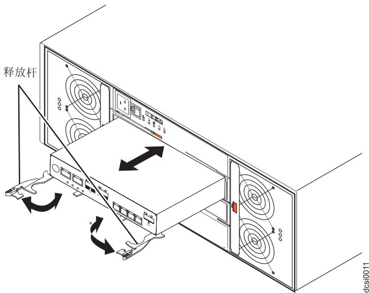
图 96. 卸下并重新安装控制器
