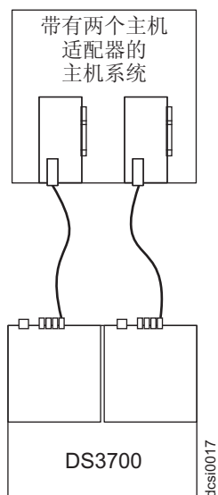
图 40. 与同一主机中两个 HBA 的双控制器直接连接的光纤通道连接（冗余主机连接）
