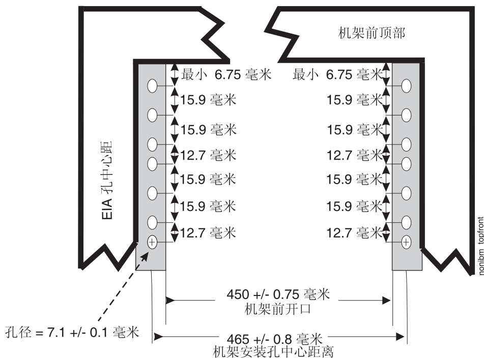
图 123. 机架规格尺寸, 顶视图 (前部)
