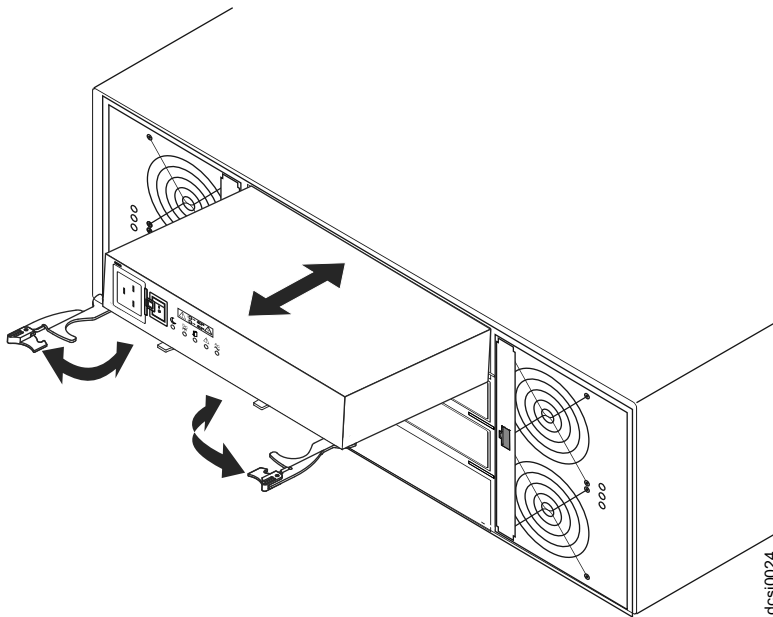
图 74. 更换电源
