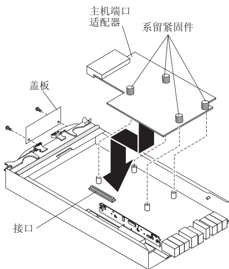
图 66. 安装主机端口适配器
