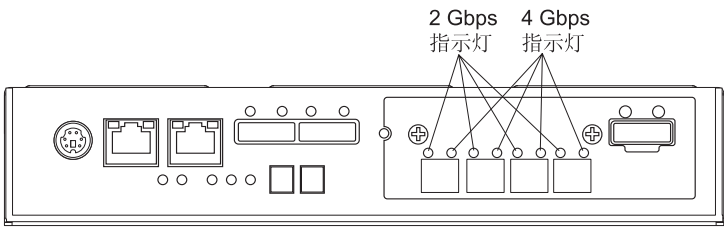
图 53. 光纤通道主机端口适配器指示灯
