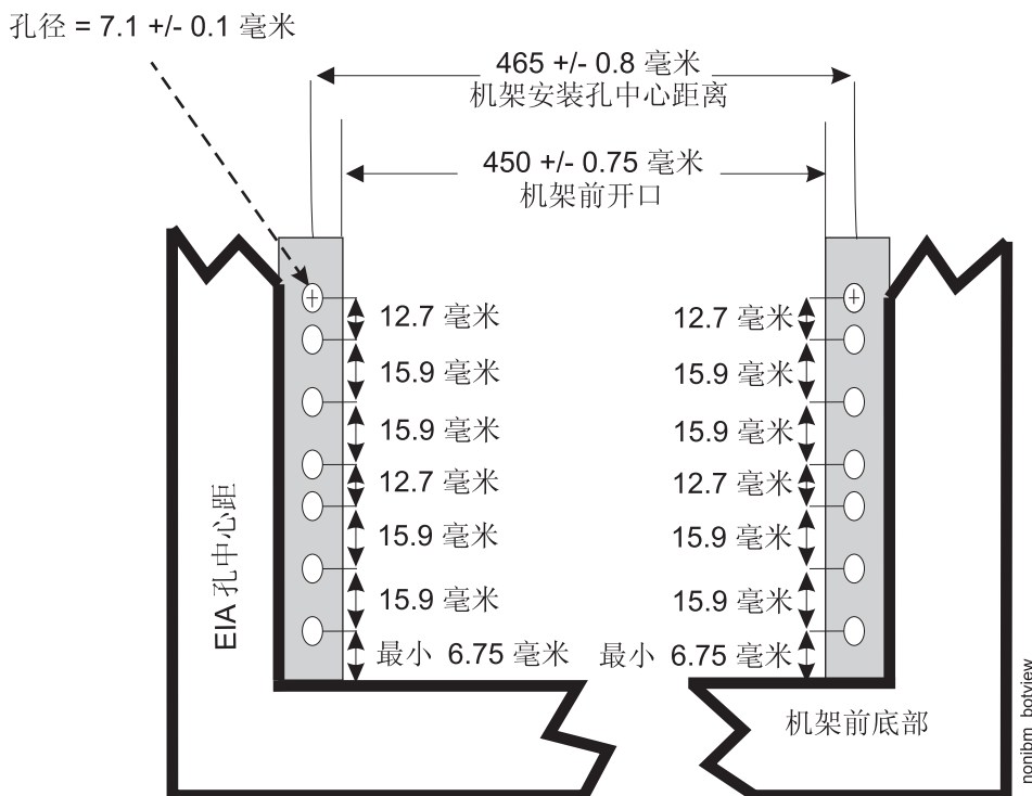
图 124. 机架规格尺寸, 底视图 (前部)
