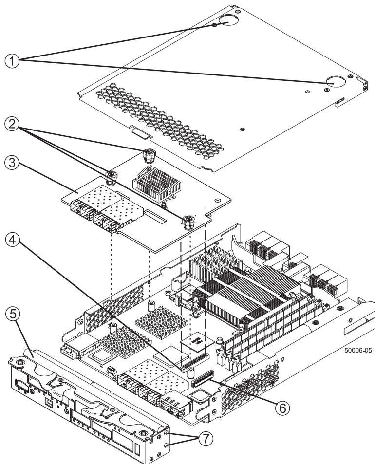
図 115. ホスト・インターフェース・カードの交換
