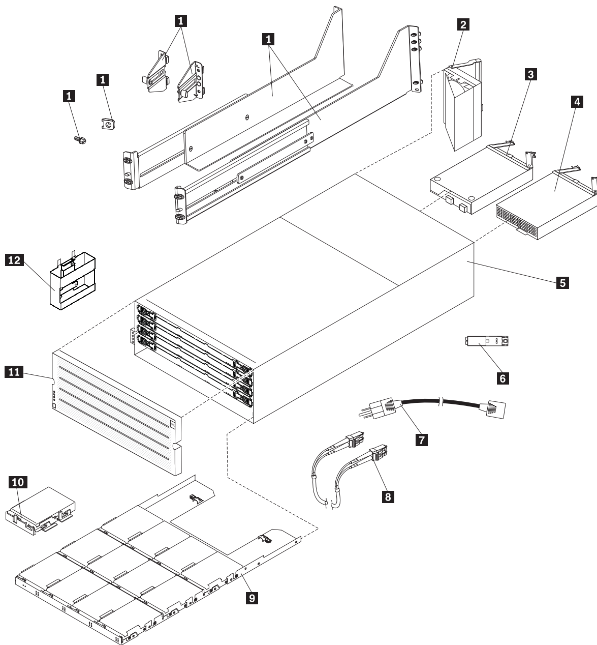
図 117. DCS3700 ストレージ・サブシステム・エンクロージャー部品リスト
