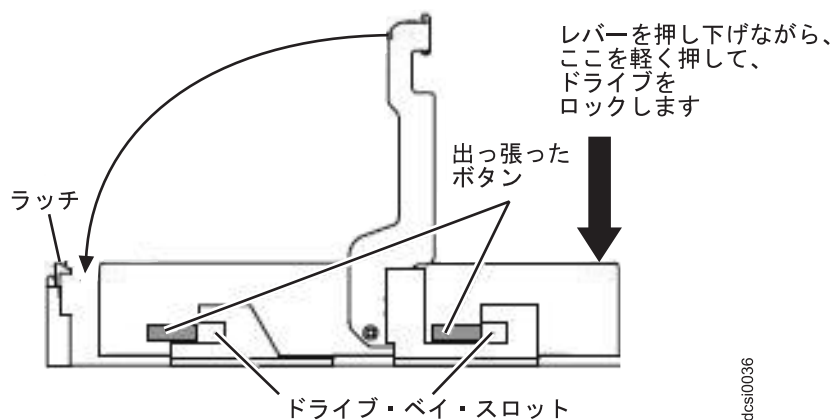
図 70. ハード・ディスクのコネクタへの挿入
