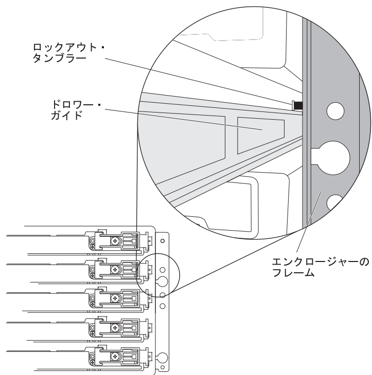
図 95. ロック・タンブラーがドロワー・ガイドより上にある場合
