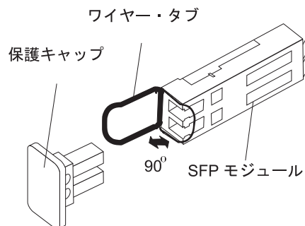
図 27. SFP モジュール・ラッチのアンロック - プラスチック・タブの場合
