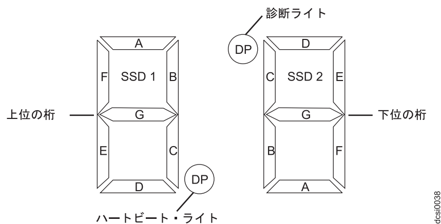
図 60. 数値ディスプレイ LED
