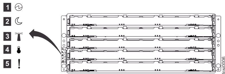
図 50. DCS3700 前面 LED およびコントロール
