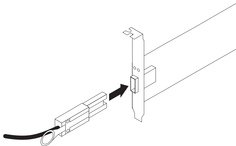
図 23. ミニ SAS ケーブルの接続
