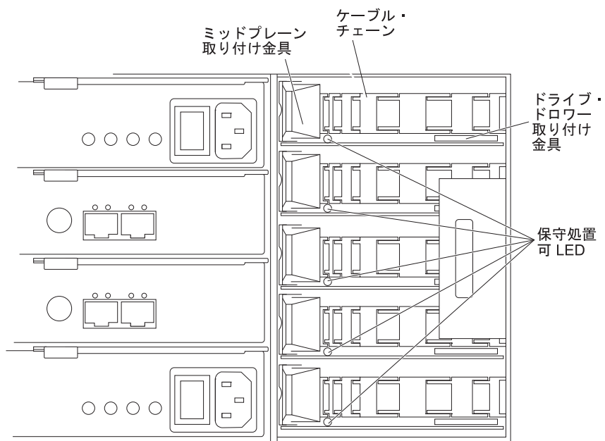
図 91. 右のファン・アセンブリーを取り外したストレージ拡張エンクロージャの背面図
