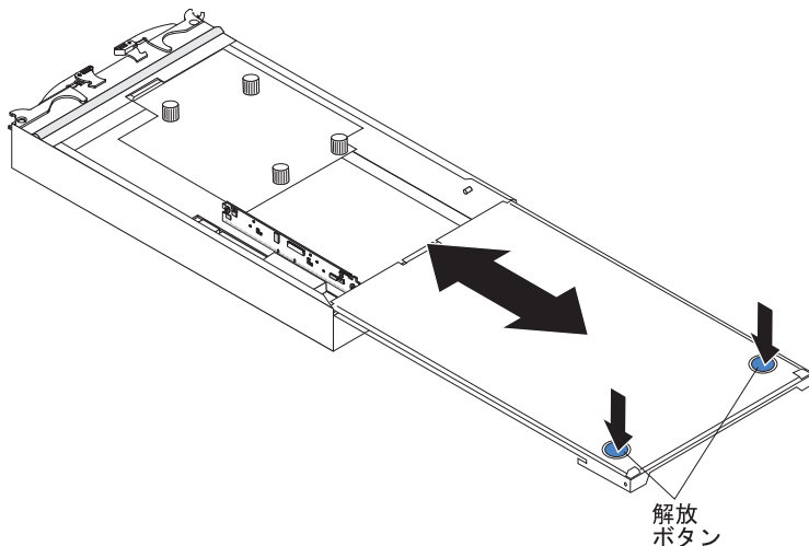
図 62. カバーの取り外し
