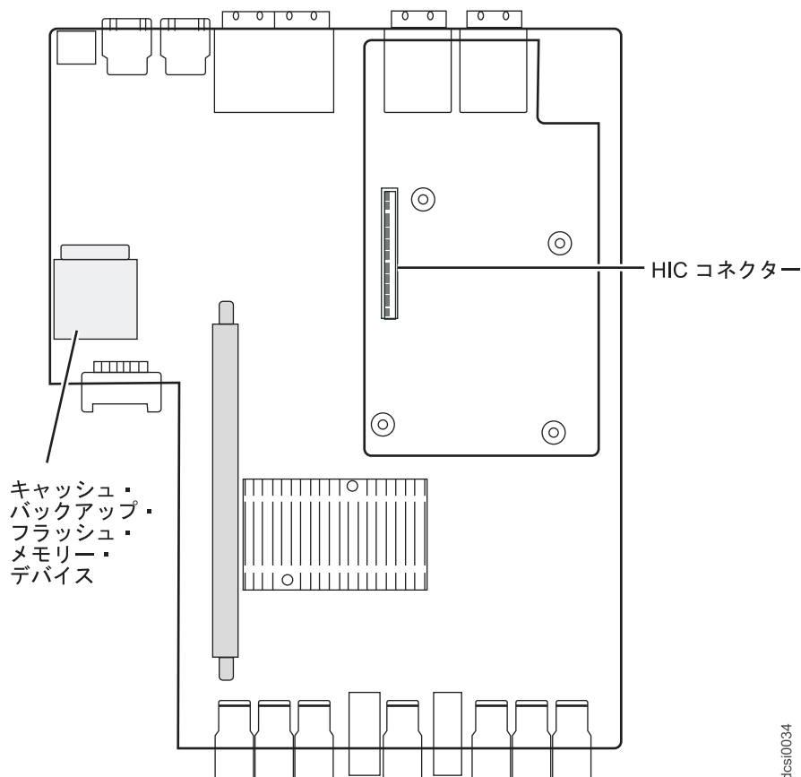
図 67. HIC コネクターの位置合わせ
