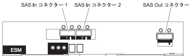
図 35. ESM のコネクター
