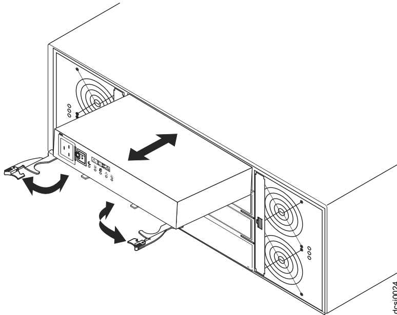
図 74. 電源機構の交換
