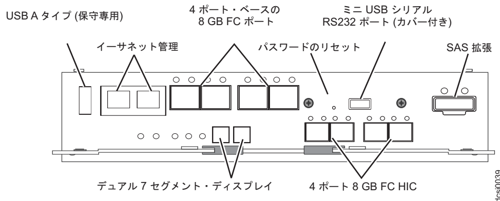
図 21. パフォーマンス・モジュール・コントローラー搭載の DCS3700 ストレージ・サブシステム (FC ポートをリスト)
