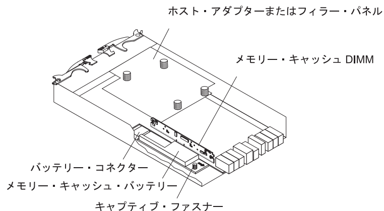
図 77. メモリー・キャッシュ DIMM の位置
