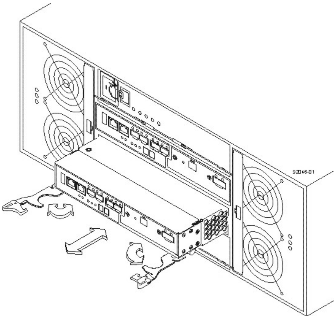
図 105. コントローラーの取り外しと交換
