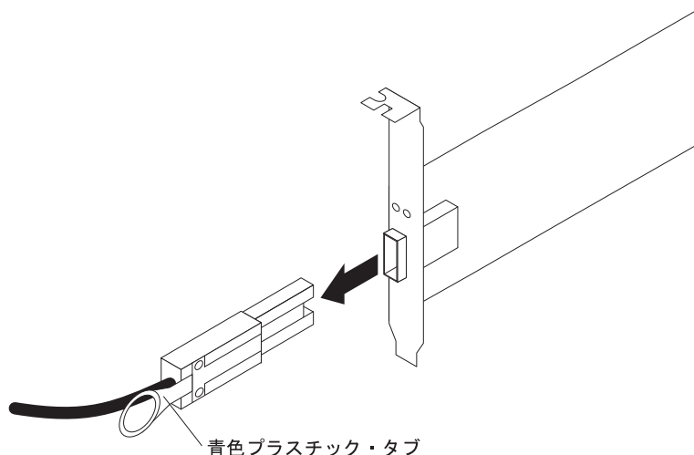
図 24. ミニ SAS ケーブルの取り外し
