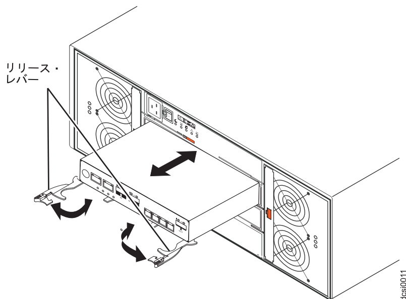
図 61. コントローラーの取り外し
