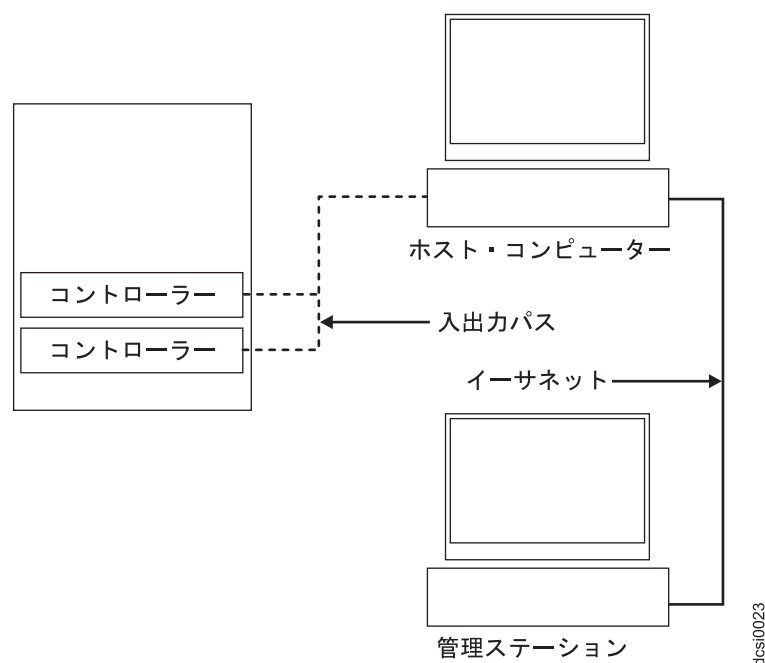
図 38. ホスト・エージェント (インバンド) 管理
