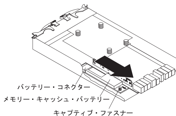
図 76. コントローラーからのバッテリー・ユニットの取り外し
