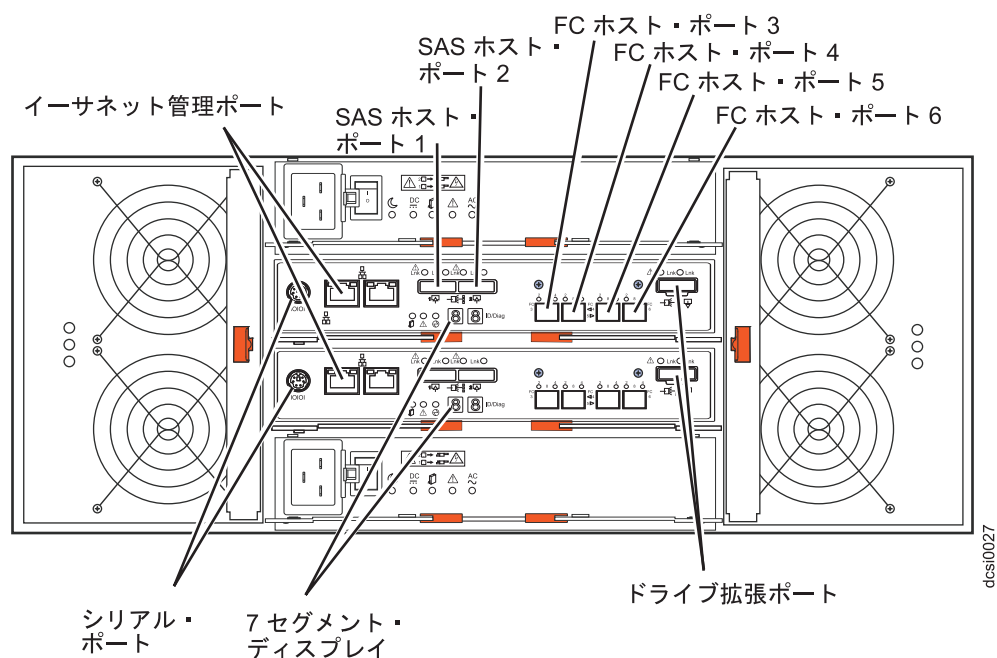
図 20. デュアル・コントローラー DCS3700 ストレージ・サブシステムのポートとコントローラー (オプションのファイバー・チャネル・ホスト・ポート・アダプターを装備)
