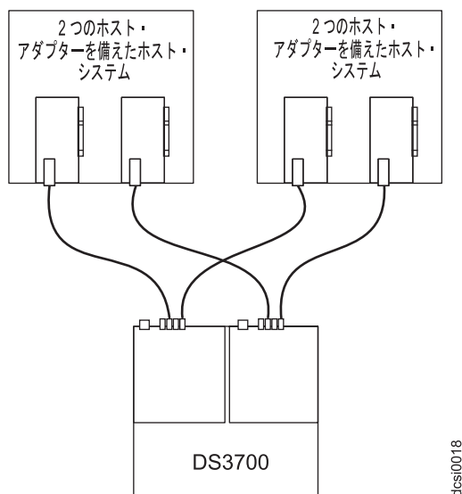
図 41. 複数のホスト内の複数の HBA へのデュアル・コントローラー直接ファイバー・チャンネル接続による接続
