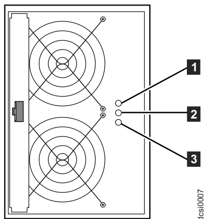
図 56. ファン・アセンブリーの LED
