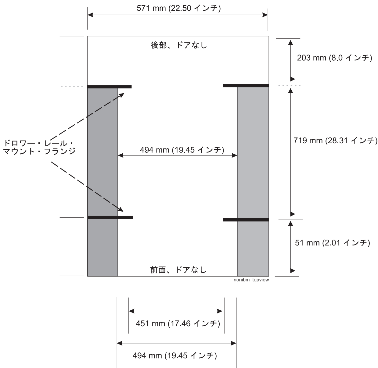
図 122. IBM 以外のラックの仕様寸法の平面図
