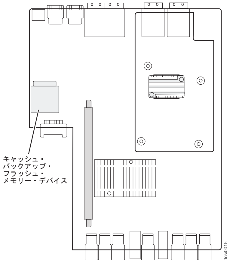
図 8I. キャッシュ・バックアップ・フラッシュ・メモリー・デバイス
