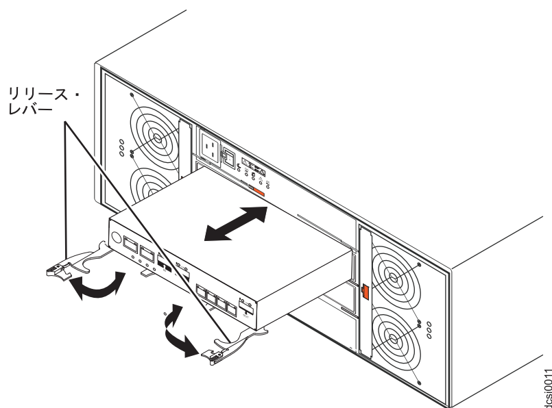
図 75. コントローラーの取り外し
