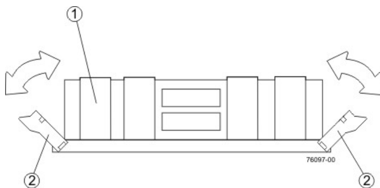
図 102. キャッシュ・メモリー DIMM の取り外し
