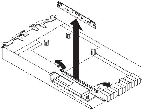
図 79. コントローラーからの DIMM の取り外し
