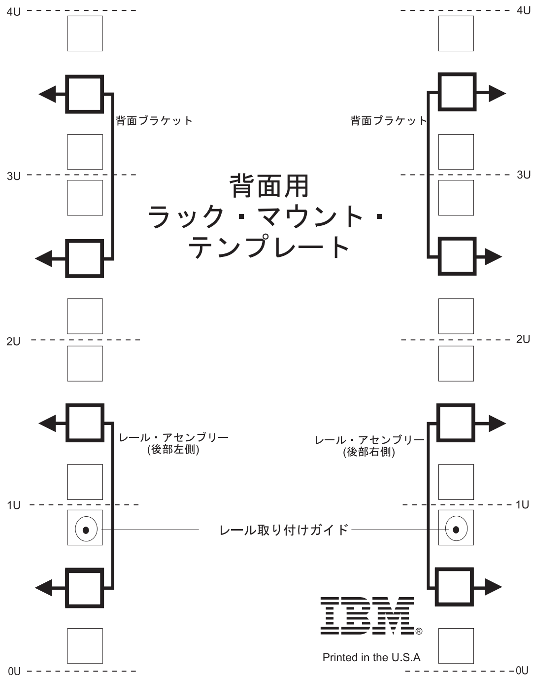
図 121. 背面用ラック・マウント・テンプレート
