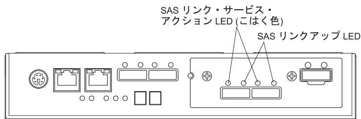
図 54. SAS ホスト・ポート・アダプター LED
