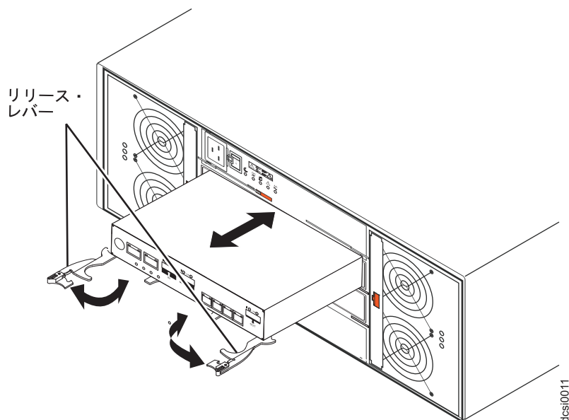
図 63. コントローラーの取り外しと交換
