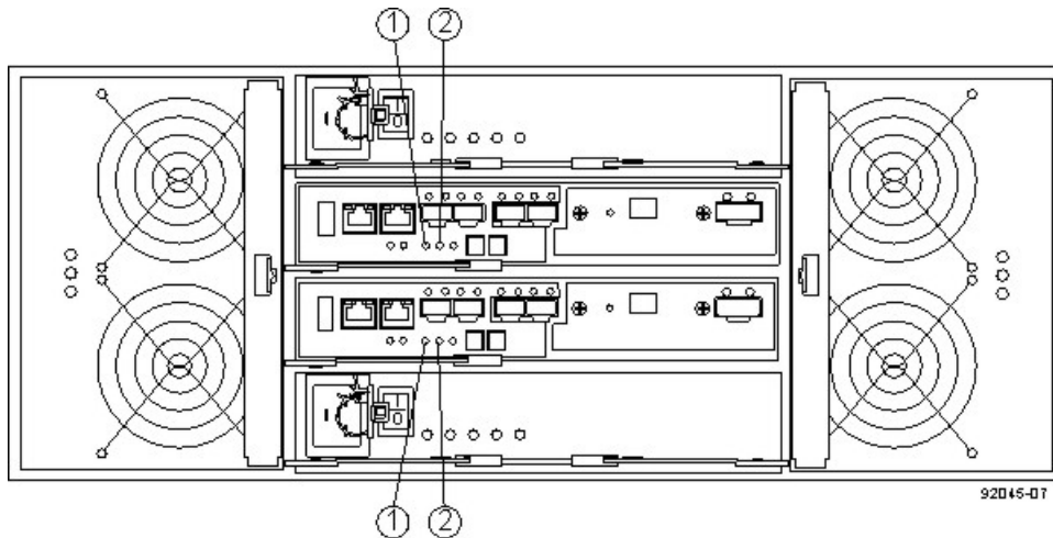
図 110. コントローラー保守処置 LED
