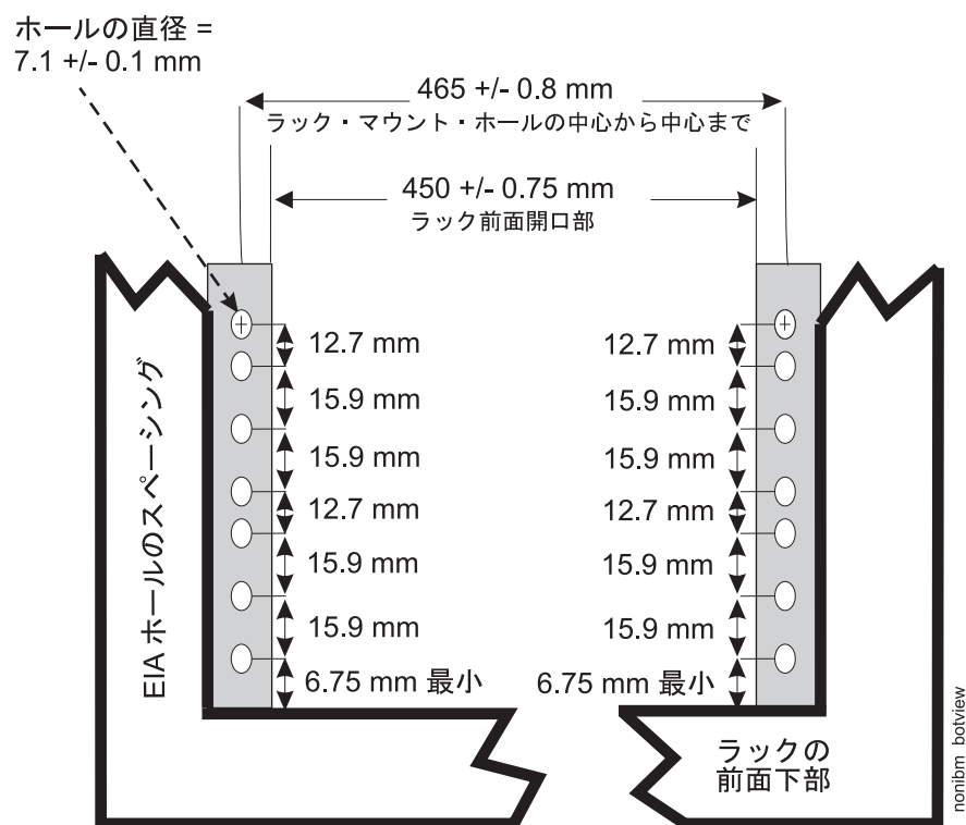
図 124. ラックの仕様寸法 (下部正面図)
