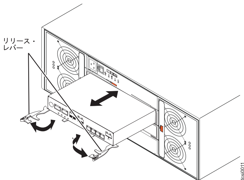
図 83. 環境サービス・モジュールの取り外し
