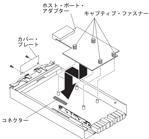
図 66. ホスト・ポート・アダプターの取り付け
