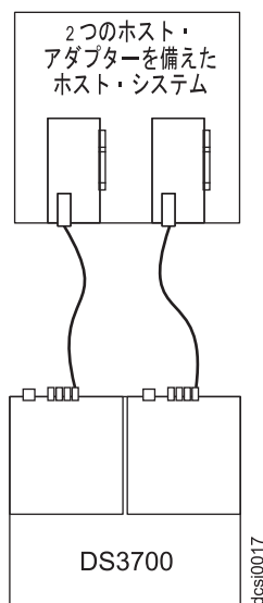
図 40. 同一ホスト内の 2 つの HBA へのデュアル・コントローラー直接ファイバー・チャンネル接続による接続 (冗長ホスト接続)
