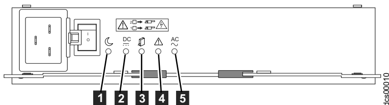
図 57. AC 電源機構 LED
