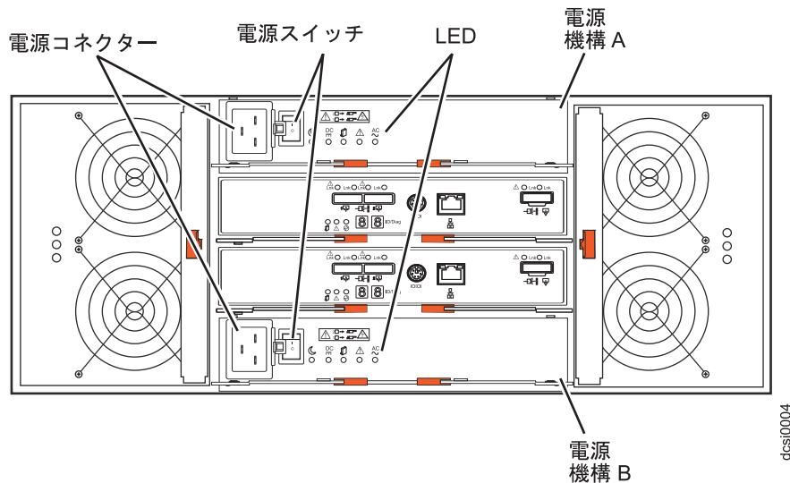
図 49. DCS3500 DC モデルの電源機構のスイッチとコネクタ
