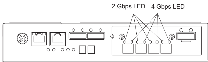
図 53. ファイバー・チャネル・ホスト・ポート・アダプター LED
