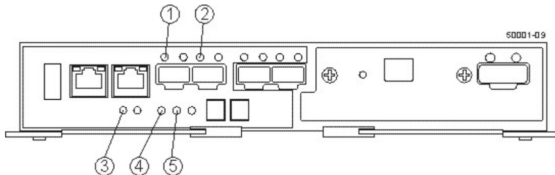
図 116. コントローラー LED
