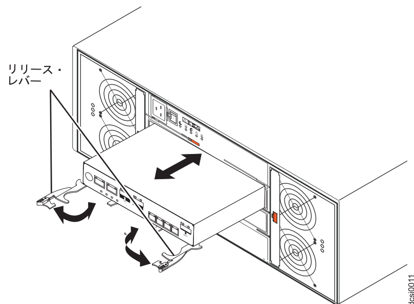
図 78. コントローラーの取り外し
