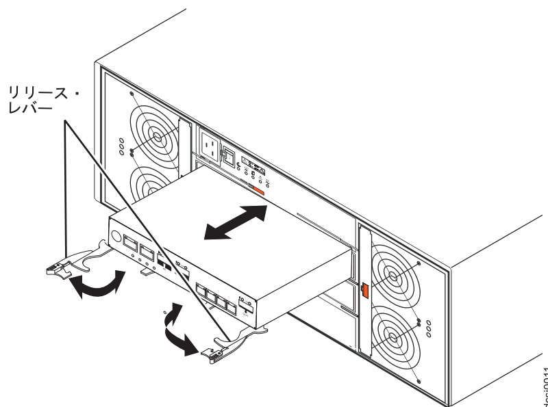
図 64. コントローラーの取り外し
