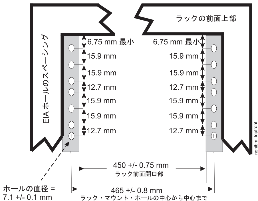
図 123. ラックの仕様寸法 (正面図)
