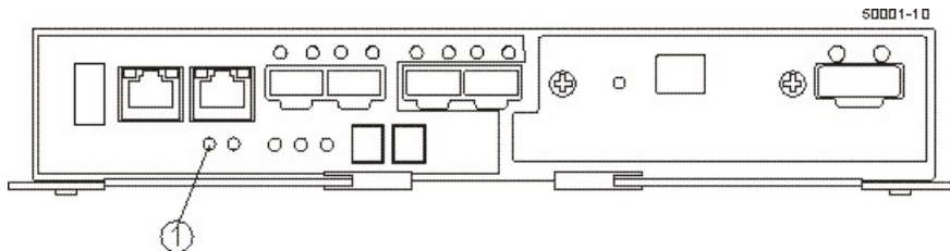
図 103. コントローラー上のバッテリーの要保守処置 LED
