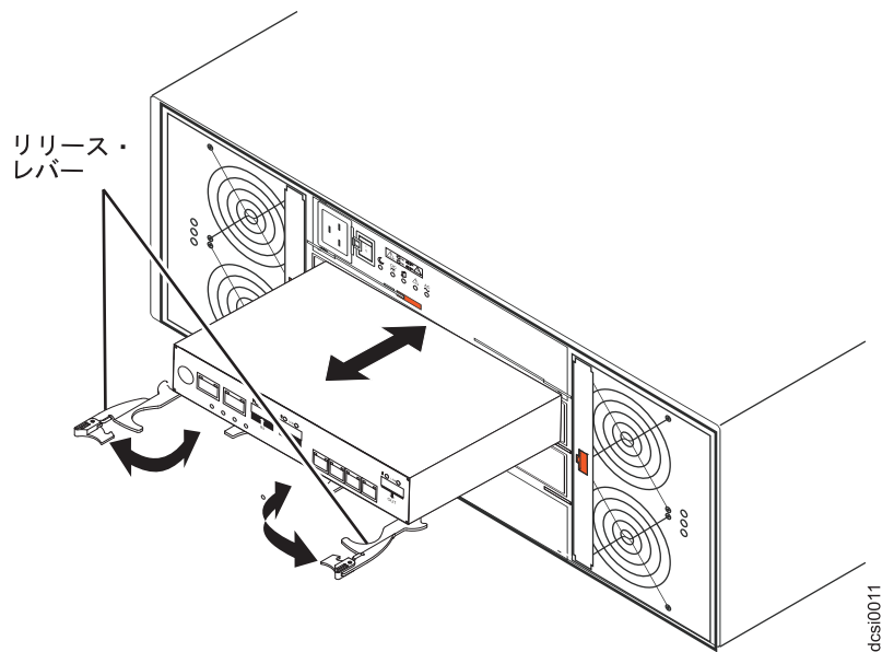
図 96. コントローラーの取り外しと交換
