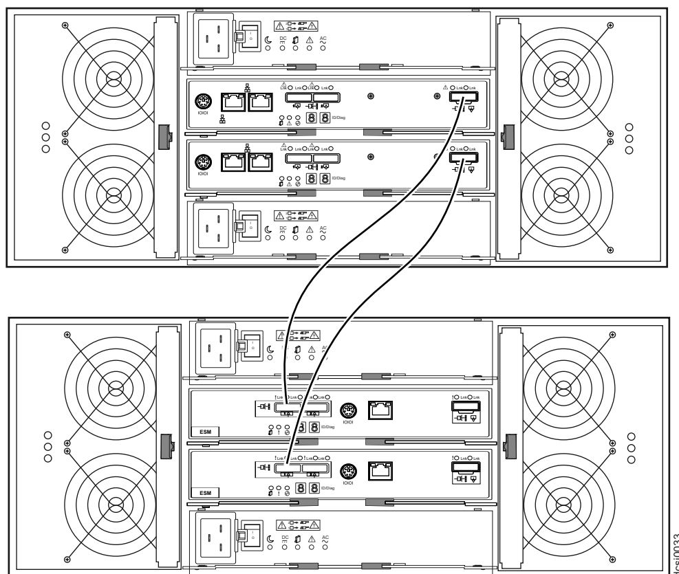
図 36. 単一の拡張エンクロージャー
