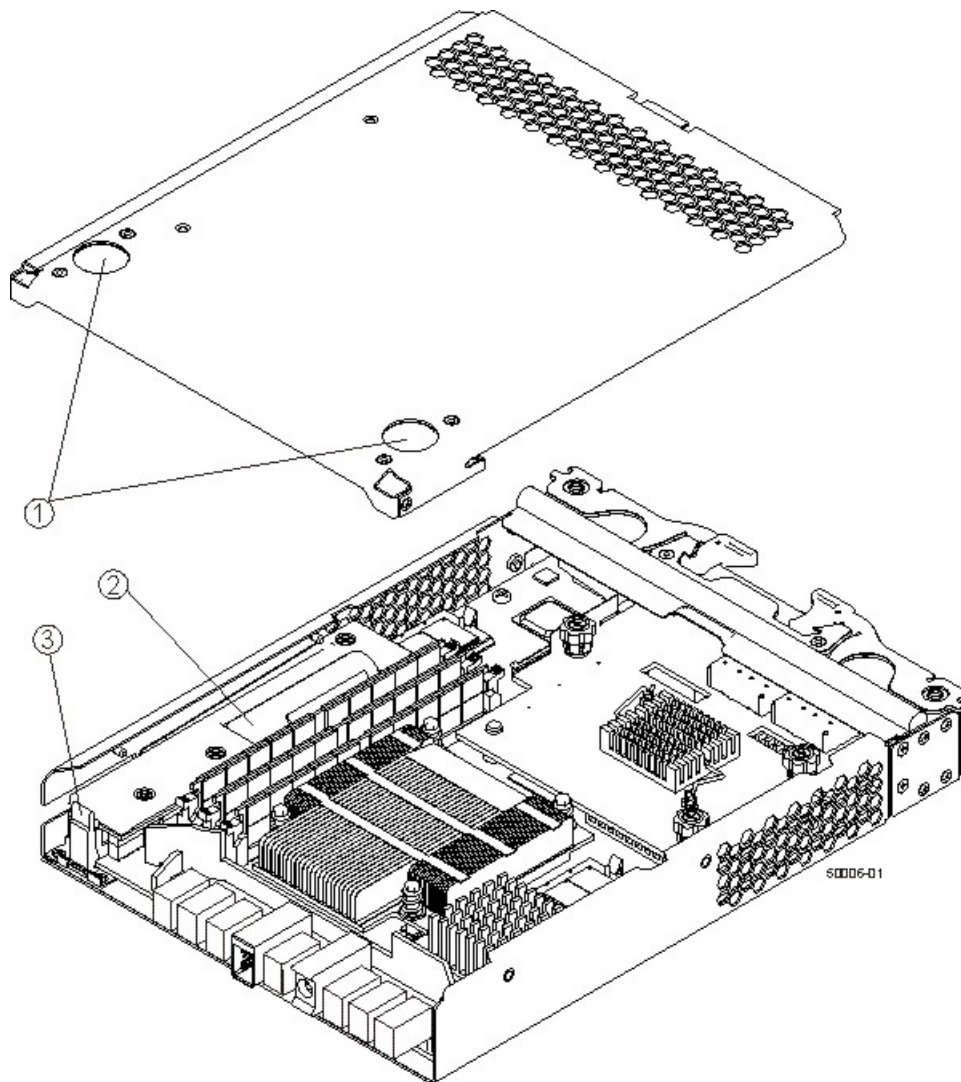
図 108. コントローラーの上部カバー・ラッチ・ボタン
