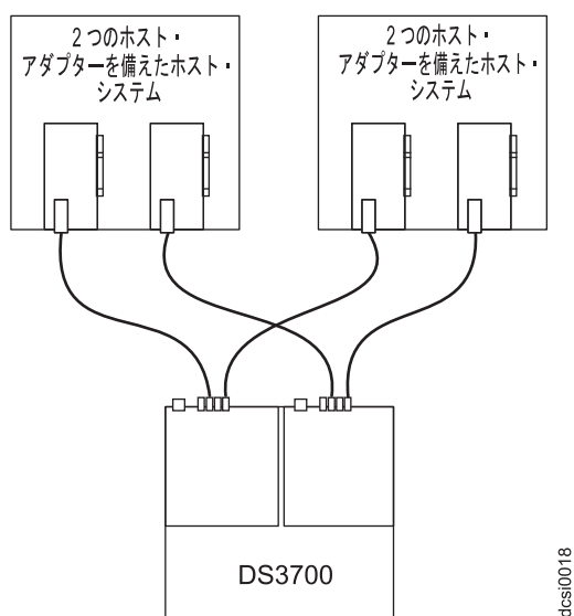
図 44. 複数のホスト内の複数の HBA へのデュアル・コントローラー直接ファイバー・チャンネル接続による接続
