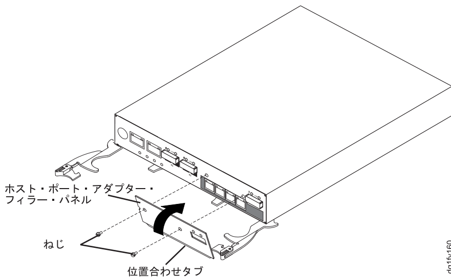
図 65. ホスト・ポート・アダプター・フィラー・パネルの取り外し
