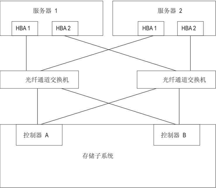
要了解更多信息，请参阅第 50 页的『IBM System Storage DS Storage Manager 支持的磁盘驱动器』。 图 18. 所有多路径驱动程序（不包括 AIX fcp_array 和 Solaris RDAC）的主机 HBA 到存储子系统控制器多路径样本配置
