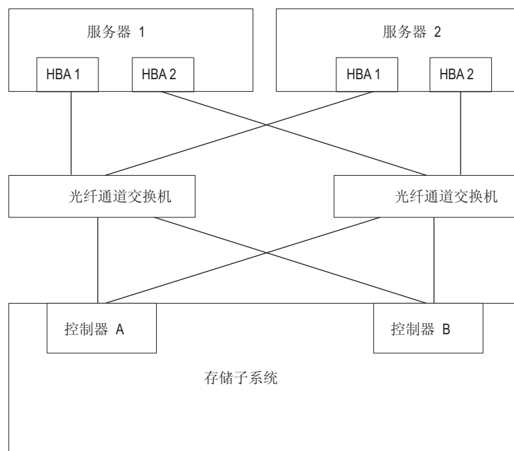
图 33. VMware 连接的交叉连接配置
