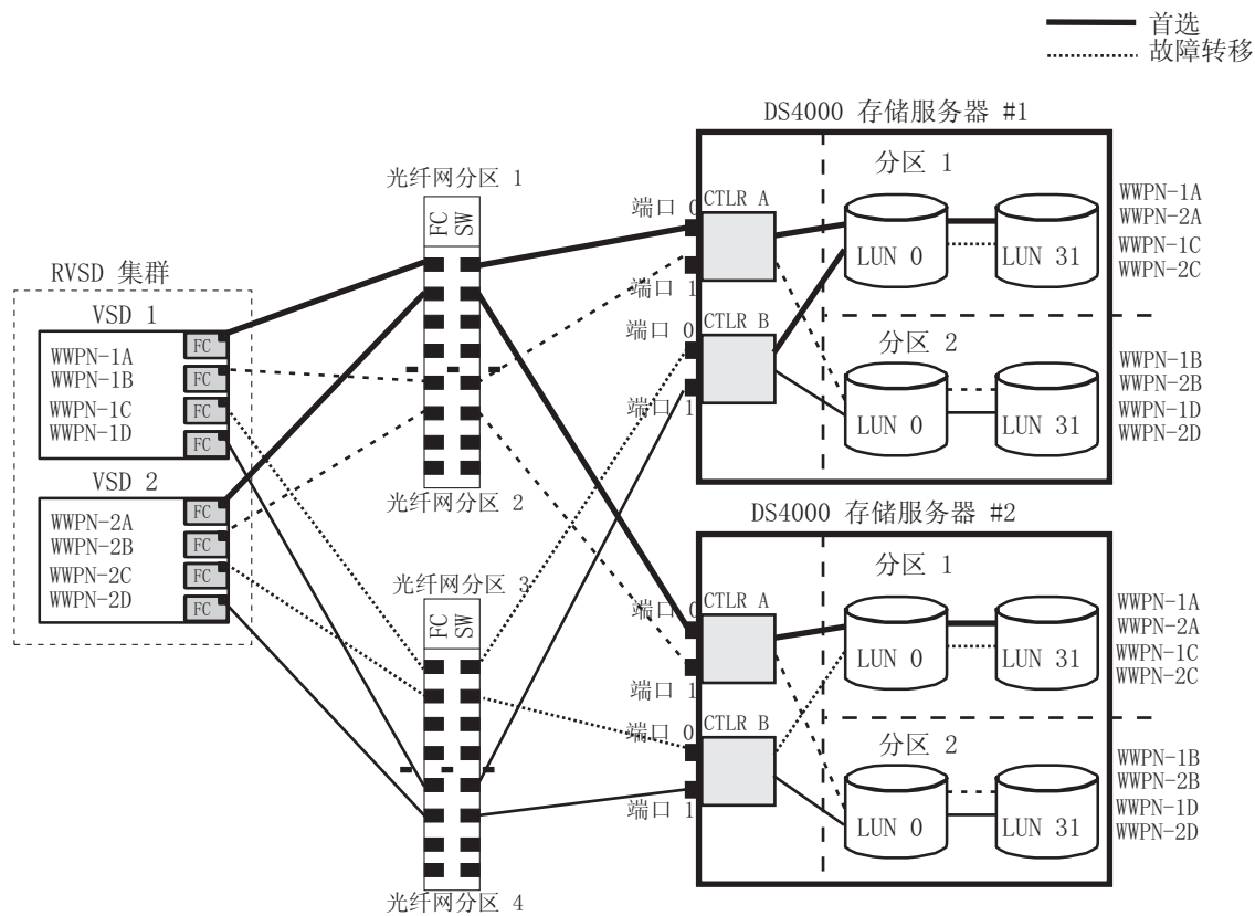
图 37. 包含两个存储子系统（每个子系统两个分区）的 RVSD 集群配置
