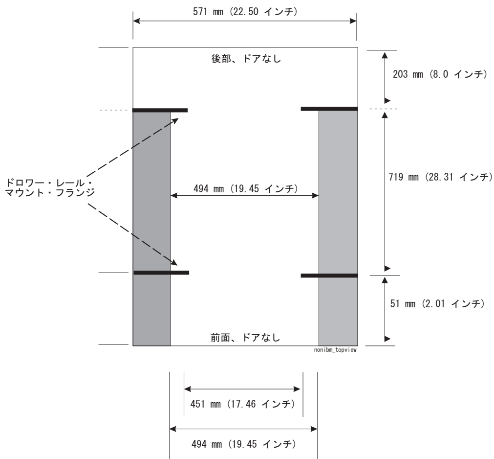
図 94. IBM 以外のラックの仕様寸法の平面図
