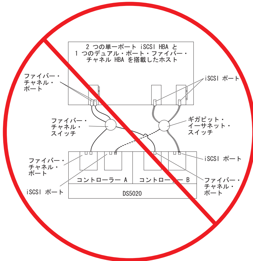
図 64. 誤った構成の例: 単一ホスト、iSCSI およびファイバー・チャネル
