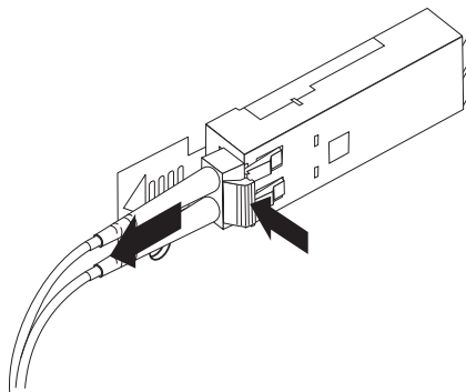
図 34. LC-LC ファイバー・チャネル・ケーブルの取り外し
