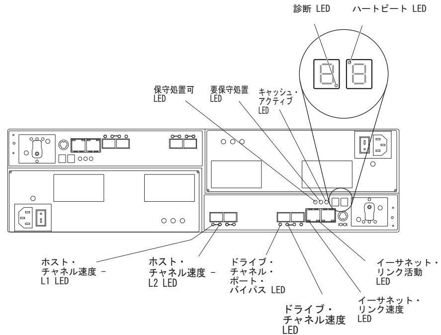
図 69. 2 つの標準ファイバー・チャンネル・ホスト拡張チャンネルを搭載したコントローラーの LED、制御、およびコネクター
