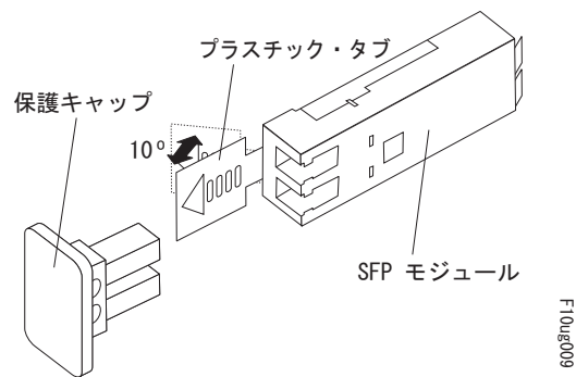
図 75. SFP モジュール・ラッチのアンロック - プラスチック・タブの場合
