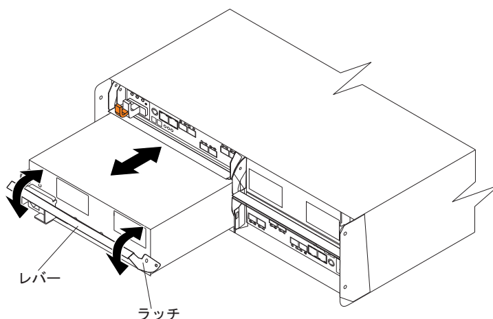
図 22. 電源機構およびファン・ユニットの再取り付け
