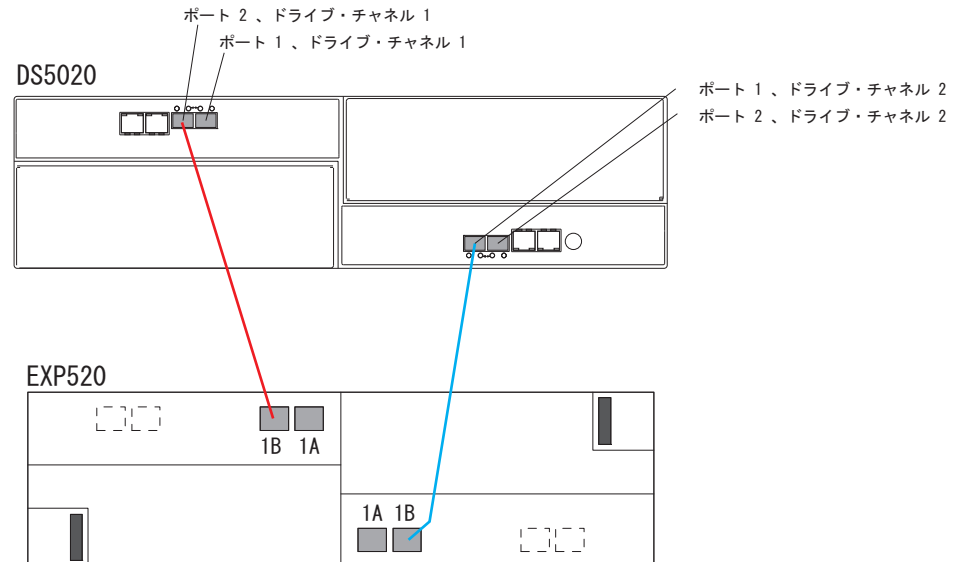
図 46. 1 つの DS5020 と 1 つの EXP520 ストレージ拡張エンクロージャのケーブル接続
