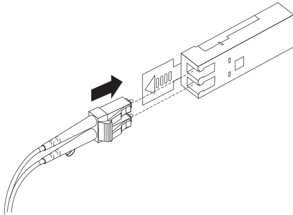
図 32. LC-LC ファイバー・チャンネル・ケーブルの SFP モジュールへの挿入
