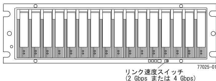
図 84. リンク速度スイッチ
