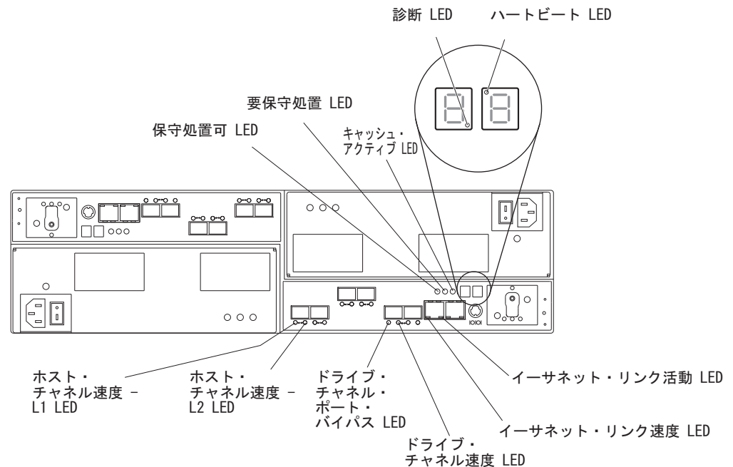
図 70. 2 つの標準および 2 つのオプションのファイバー・チャンネル・ホスト拡張チャンネルを搭載したコントローラーの LED、制御、およびコネクター
