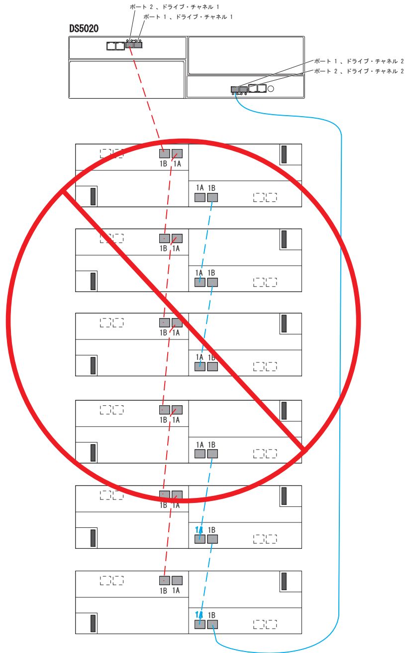
図 43. 1 つの DS5020 と最大 6 つのストレージ拡張エンクロージャーのケーブル接続
