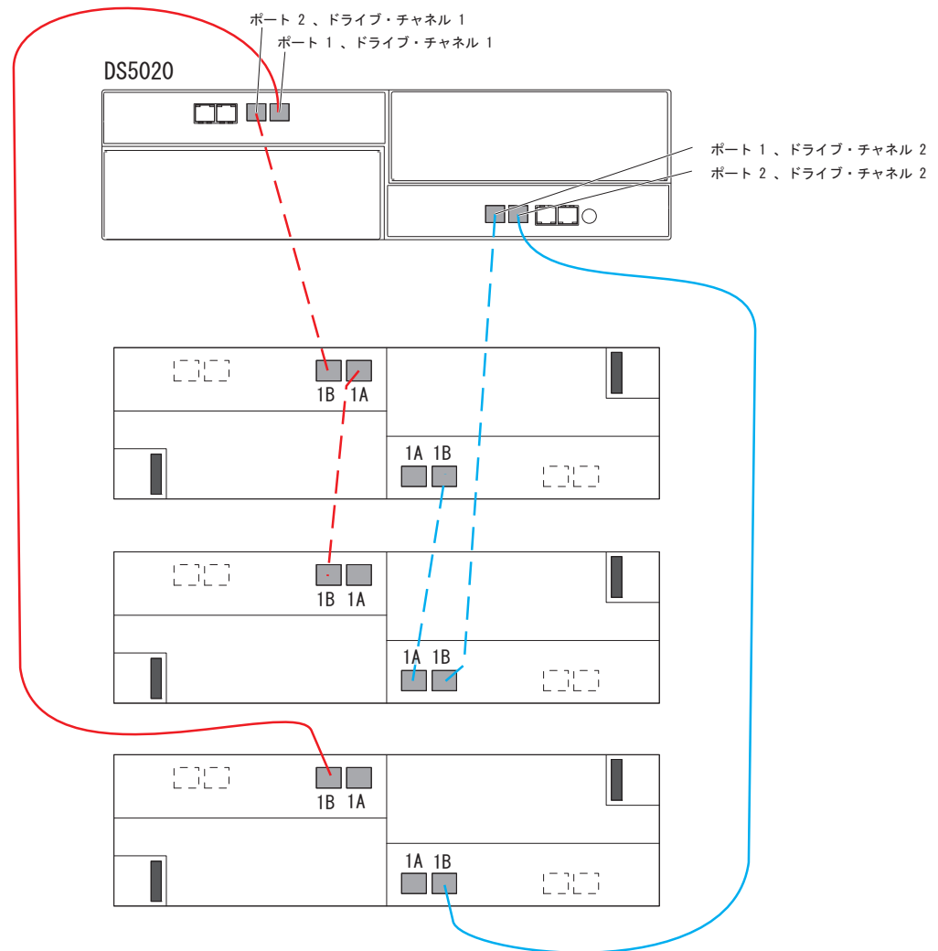
図 40. 1 つの DS5020 と 3 つのストレージ拡張エンクロージャのケーブル接続
