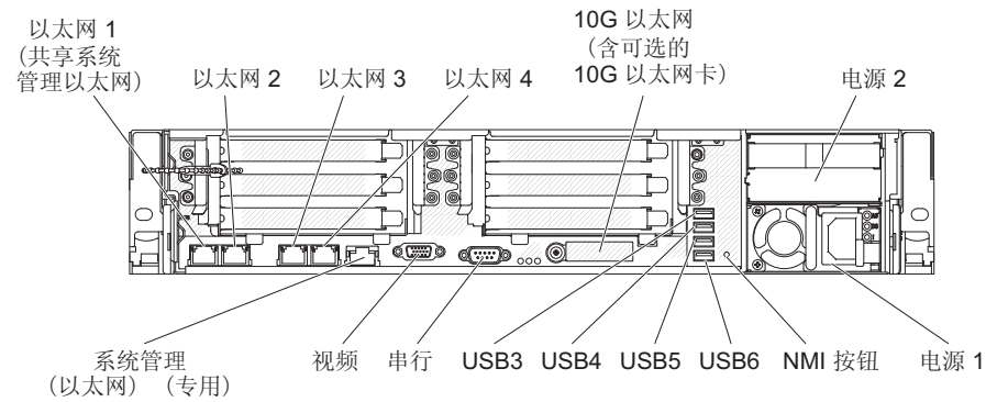
后视图
